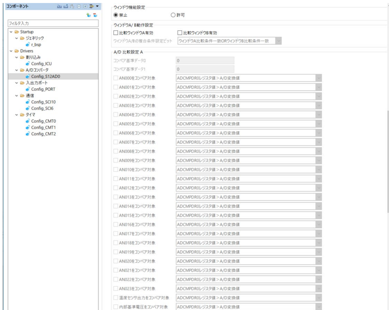
図 4-46 Config_S12AD0 設定(2)
