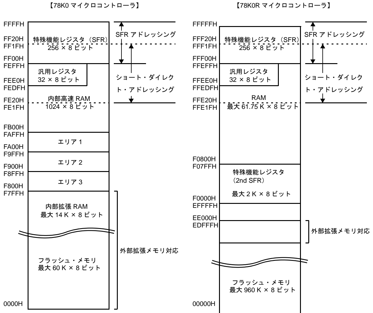
図4-8 78K0 マイクロコントローラと78K0R マイクロコントローラのメモリ・マップ
