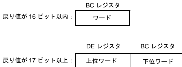
図 9—5 戻り値の参照
