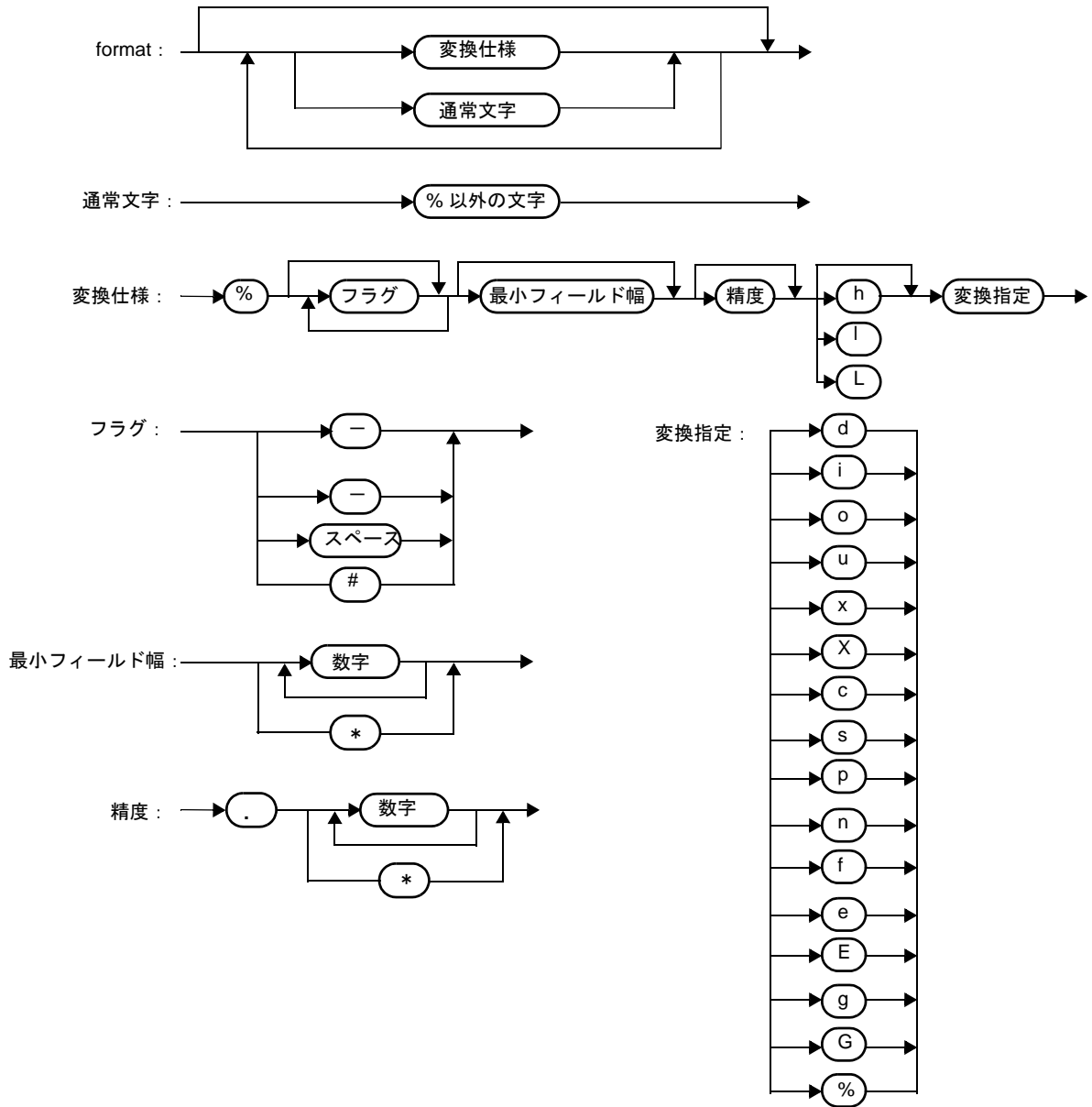
図 6—2 format の構文図
