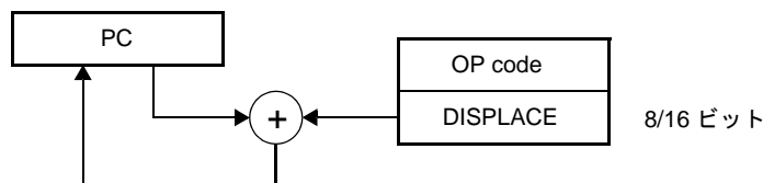
図4—16 レラティブ・アドレッシングの概略
