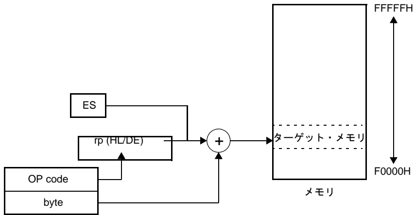
図4—33 ES:[HL+byte], ES:[DE+byte] の例
