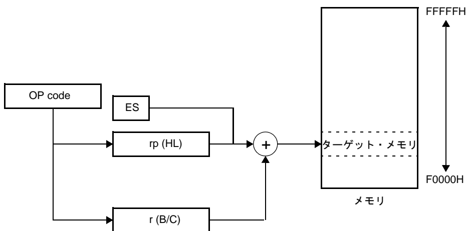
図 4—37 ES:[HL+B], ES:[HL+C] の例
