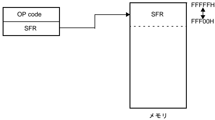
図4-26 SFR アドレッシングの概略
