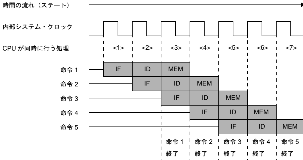
図4—38 標準的な命令を5つ続けて実行する例
