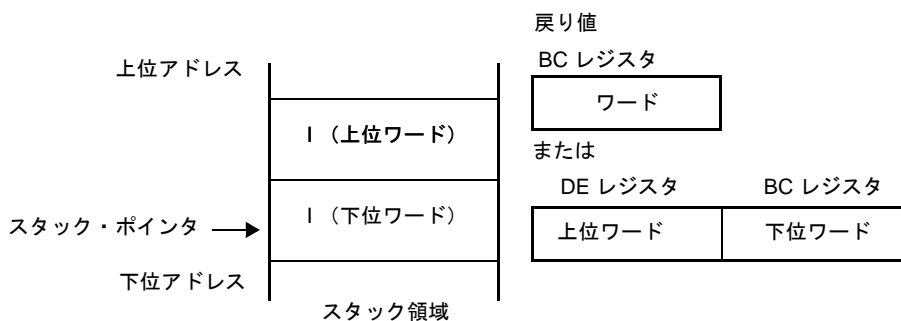
図9—3 関数 main へのリターン
