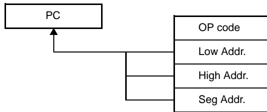
図4-17 CALL !!addr20/BR !!addr20 の例
