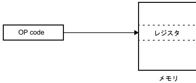
図 4—22 レジスタ・アドレッシングの概略
