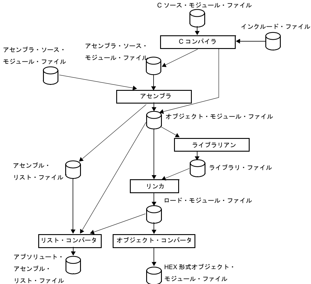
図 1—5 コンパイラ／アセンブラの処理の流れ
