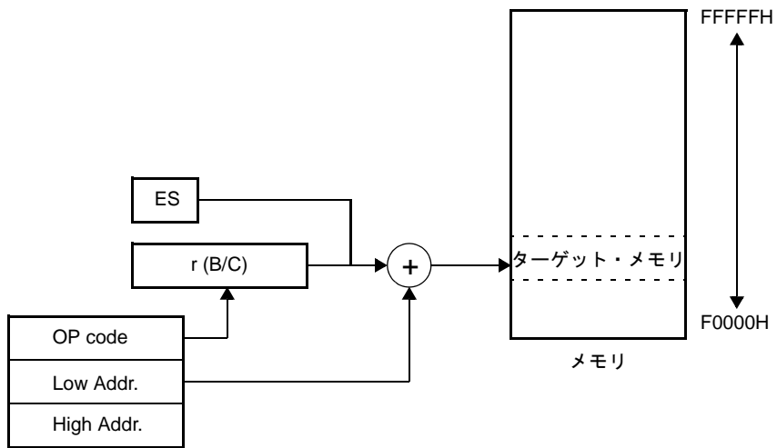
図4—34 ES:word[B], ES:word[C] の例
