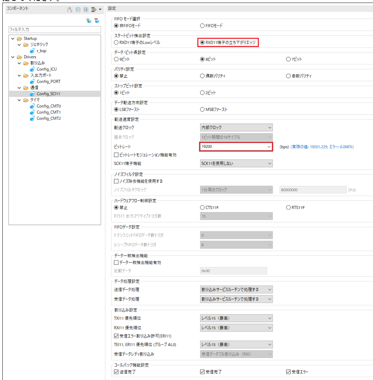
図 4-31: Config_SCI11 設定
