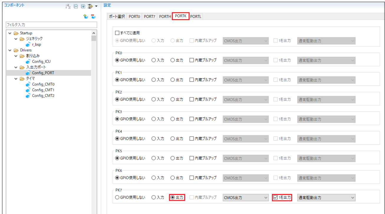
図 4-27: PORTC タブ選択
