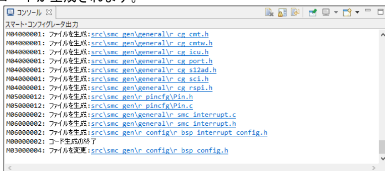
図 4-51: コード生成
