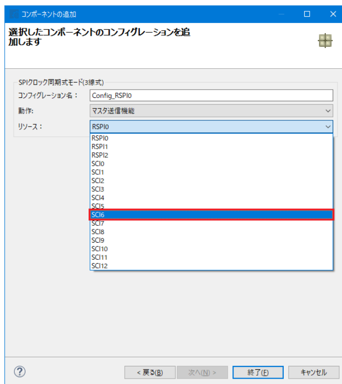
図 4-38: リソース選択 – SCI6
