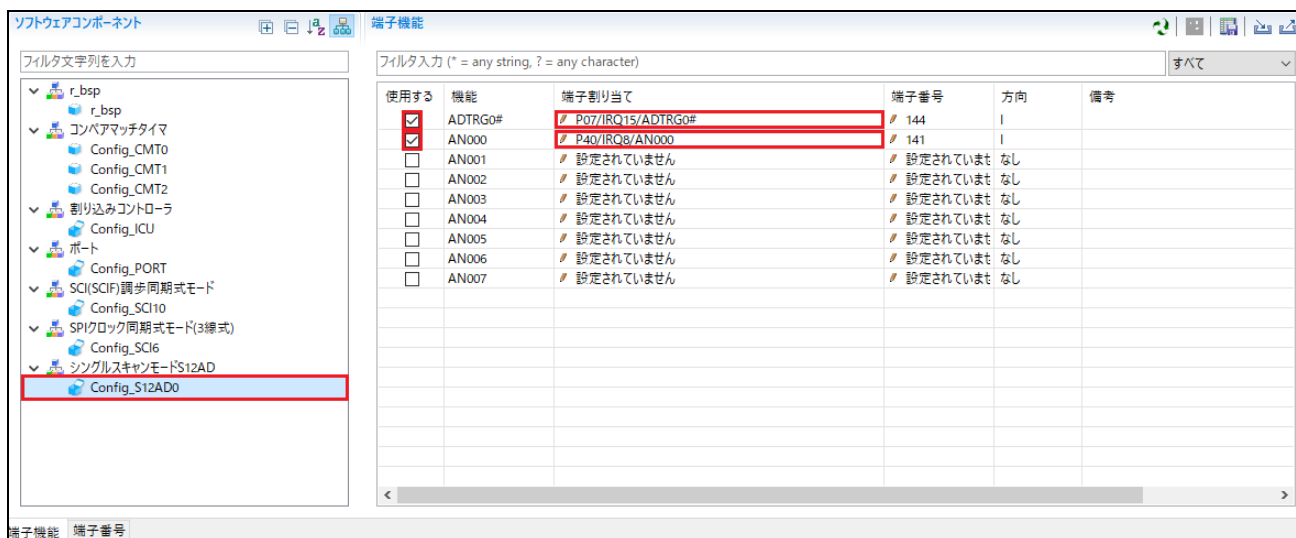
図 4-50: 端子設定 – Config_S12AD0
