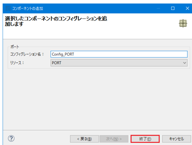
図 4-24: リソース選択 – PORT
