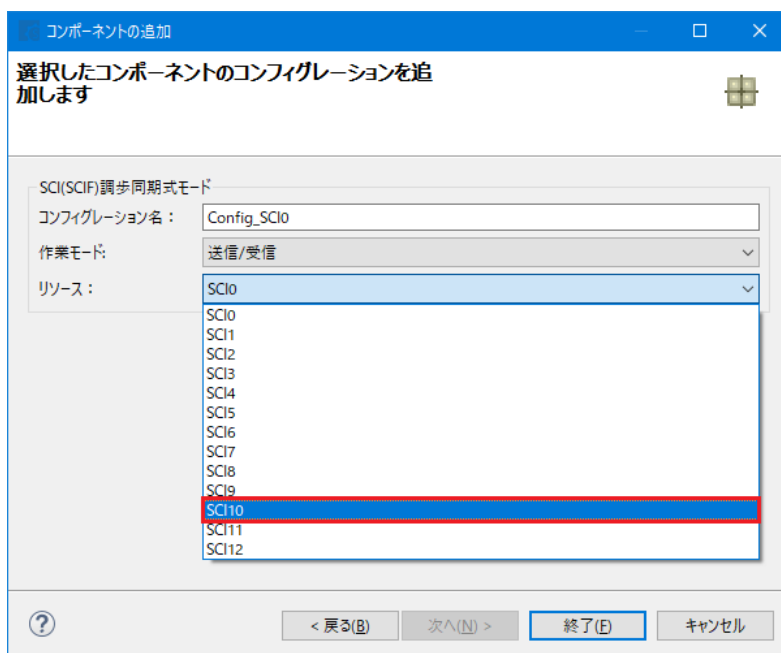
図 4-33: リソース選択 – SCI10
