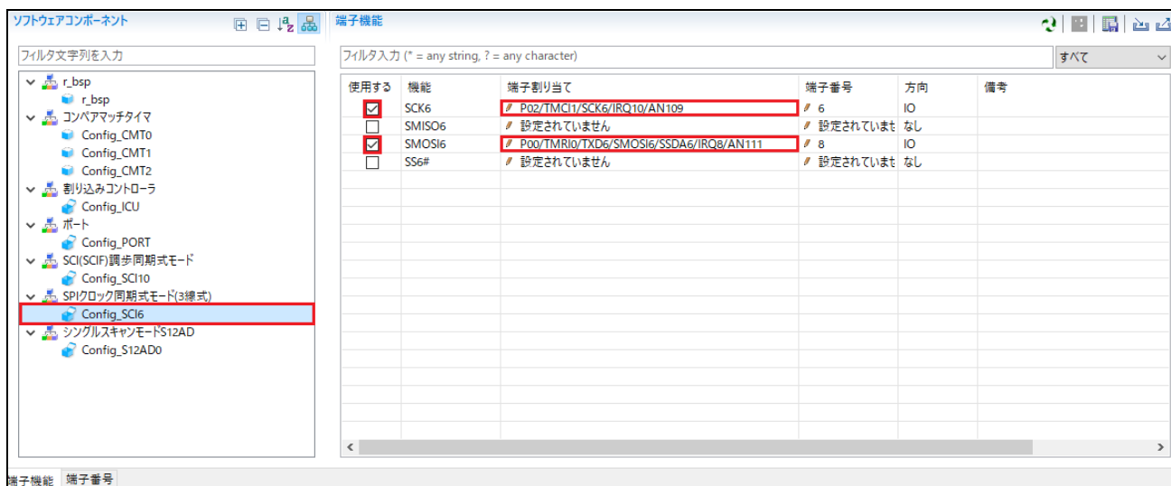
図 4-49: 端子設定 – Config_SCI6
