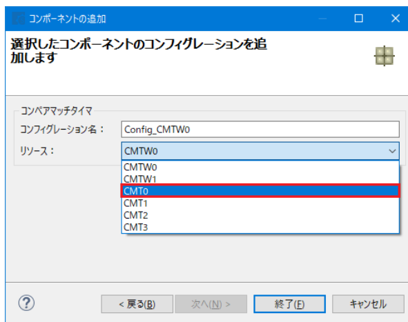
図 4-11: リソース選択 – CMT0
