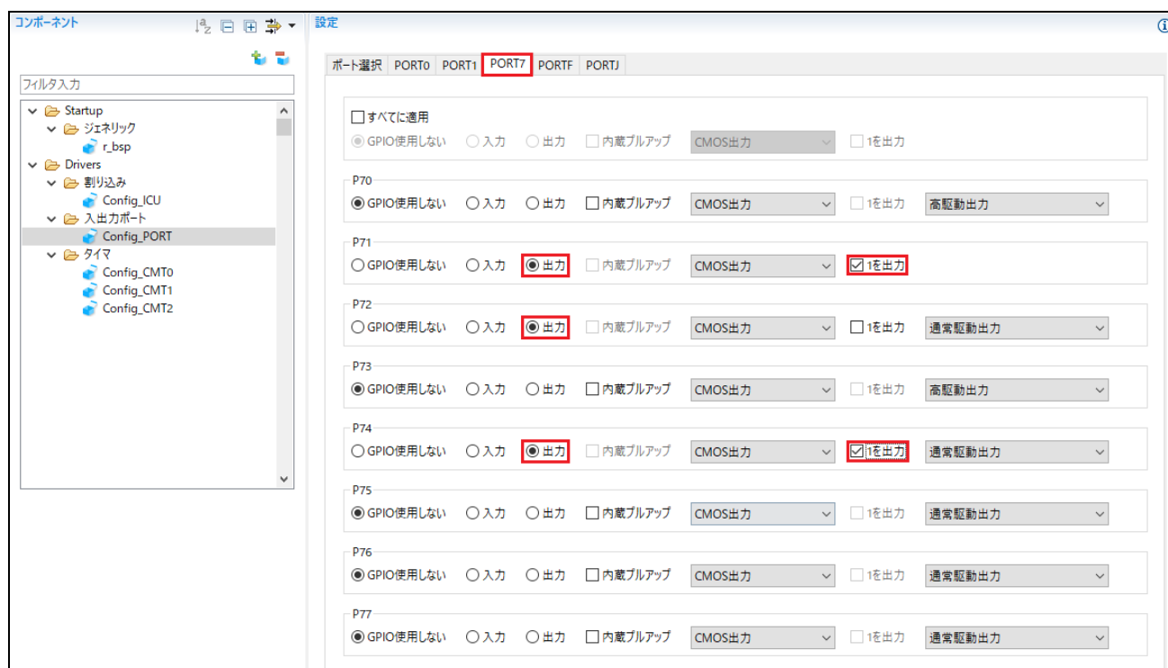
図 4-28: PORT7 タブ選択
