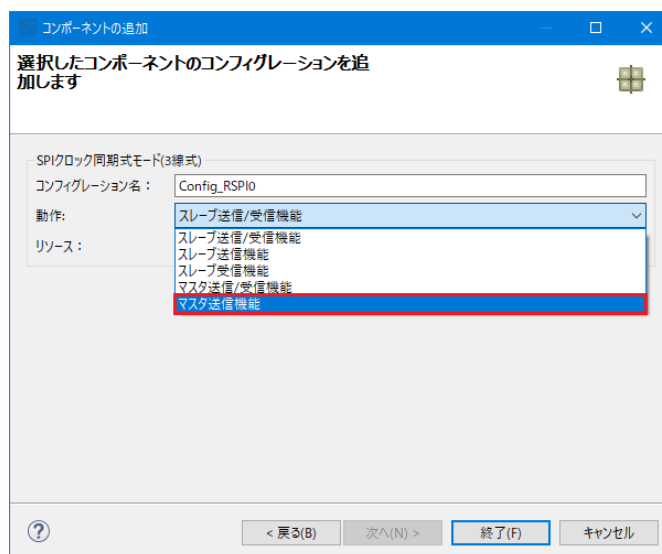
図 4-37: 動作選択 – マスタ送信機能
