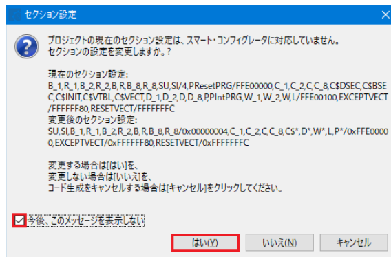
図 4-52: セクション設定ダイアログ
