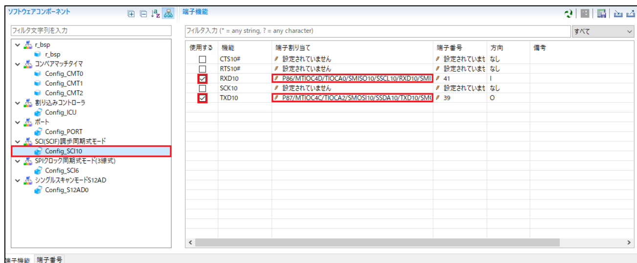
図 4-48: 端子設定 – Config_SCI10
