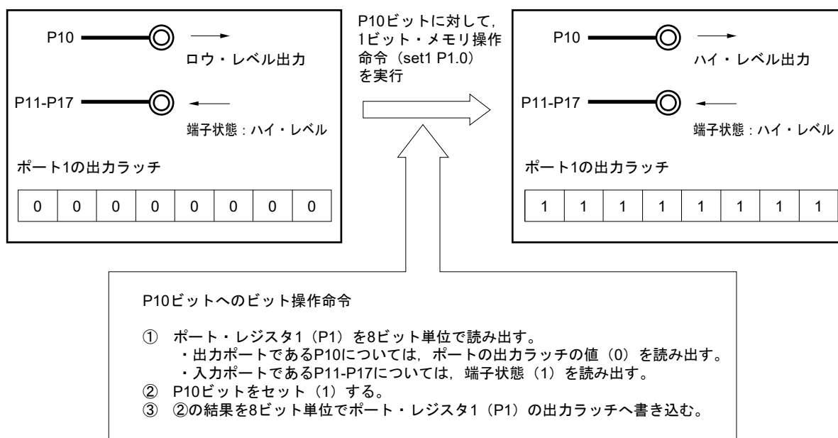
図4-14 1ビット・メモリ操作命令（P10の場合）
