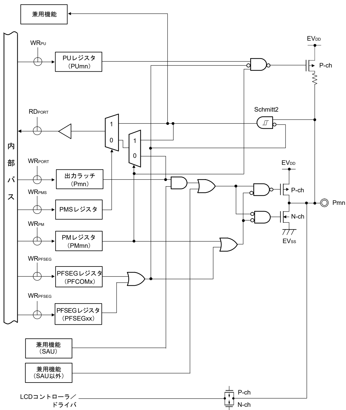
図2-13 端子タイプ7-5-29の端子ブロック図
