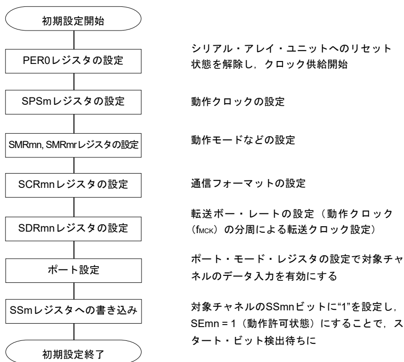
図20-87 UART受信の初期設定手順
