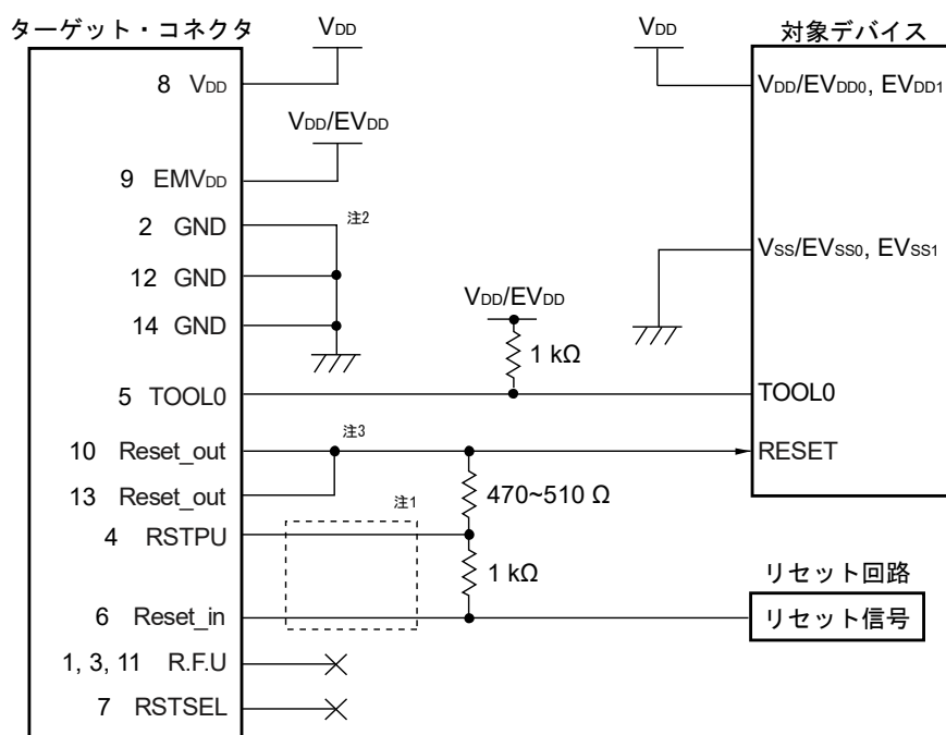
図39-1 E1オンチップデバッキングエミュレータとの接続例
