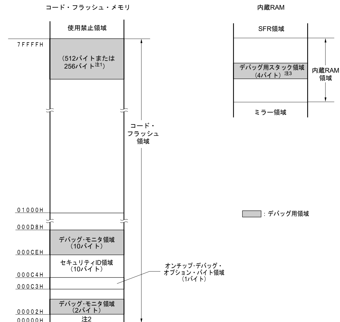
図39-2 デバッグ用モニタ・プログラムが配置されるメモリ空間
