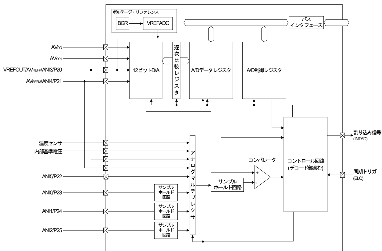
図17-1 12ビットA/Dコンバータのブロック図
