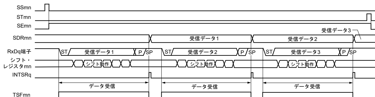
図20-90 UART受信のタイミング・チャート
