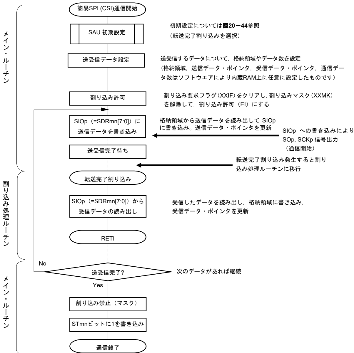
図20-48 マスタ送受信（シングル送受信モード時）のフロー・チャート
