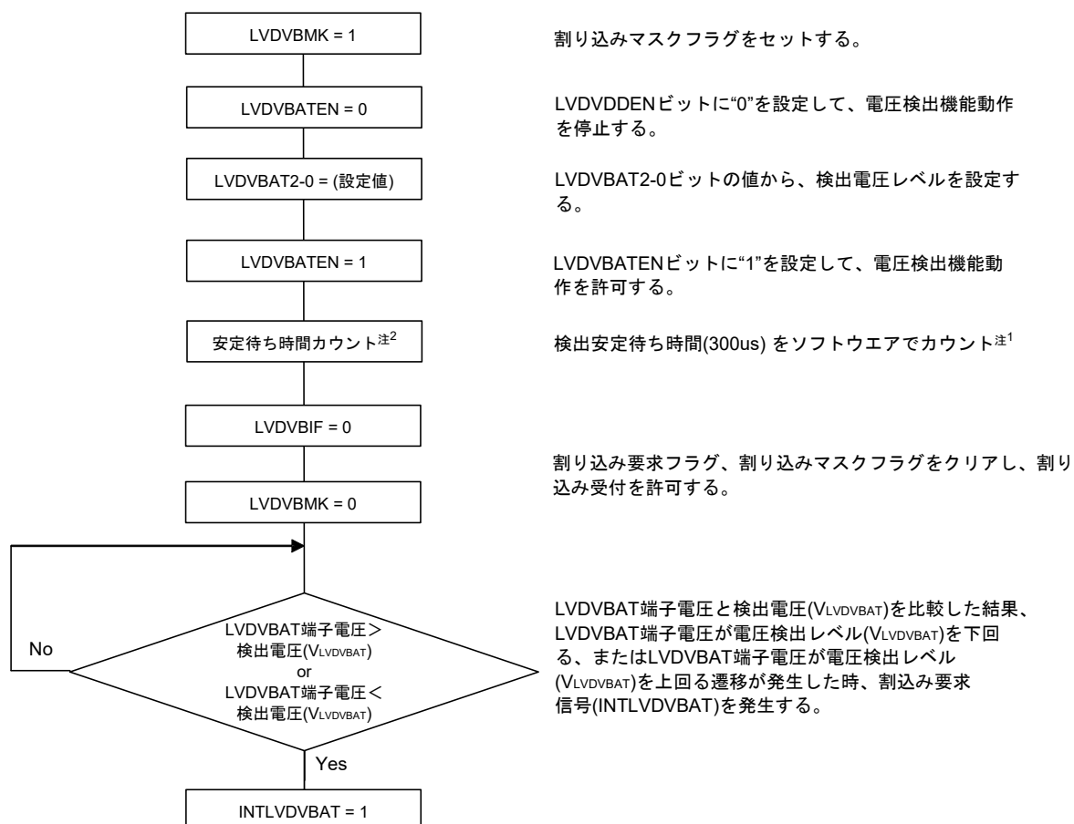
図32-22 LVDVBAT端子電圧検出の設定手順
