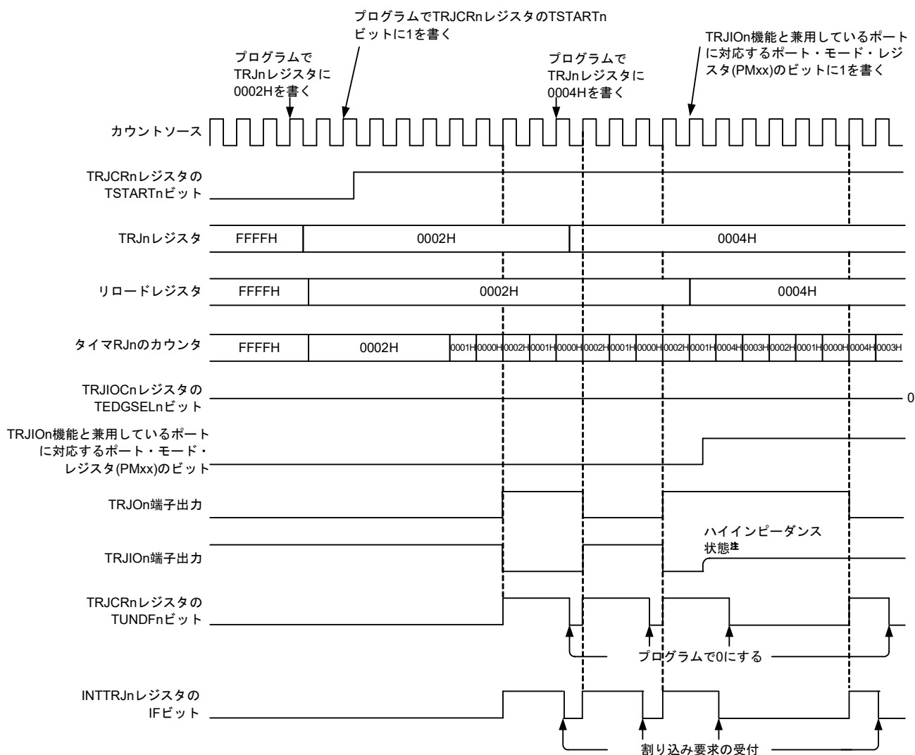
図13-13 パルス出力モードの動作例
