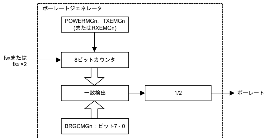
図22-23 ポー・レート・ジェネレータ構成
