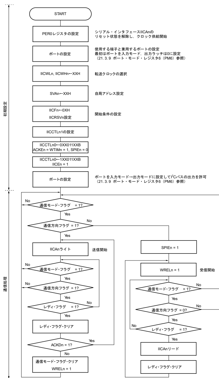
図21-31 スレーブ動作手順 (1)
