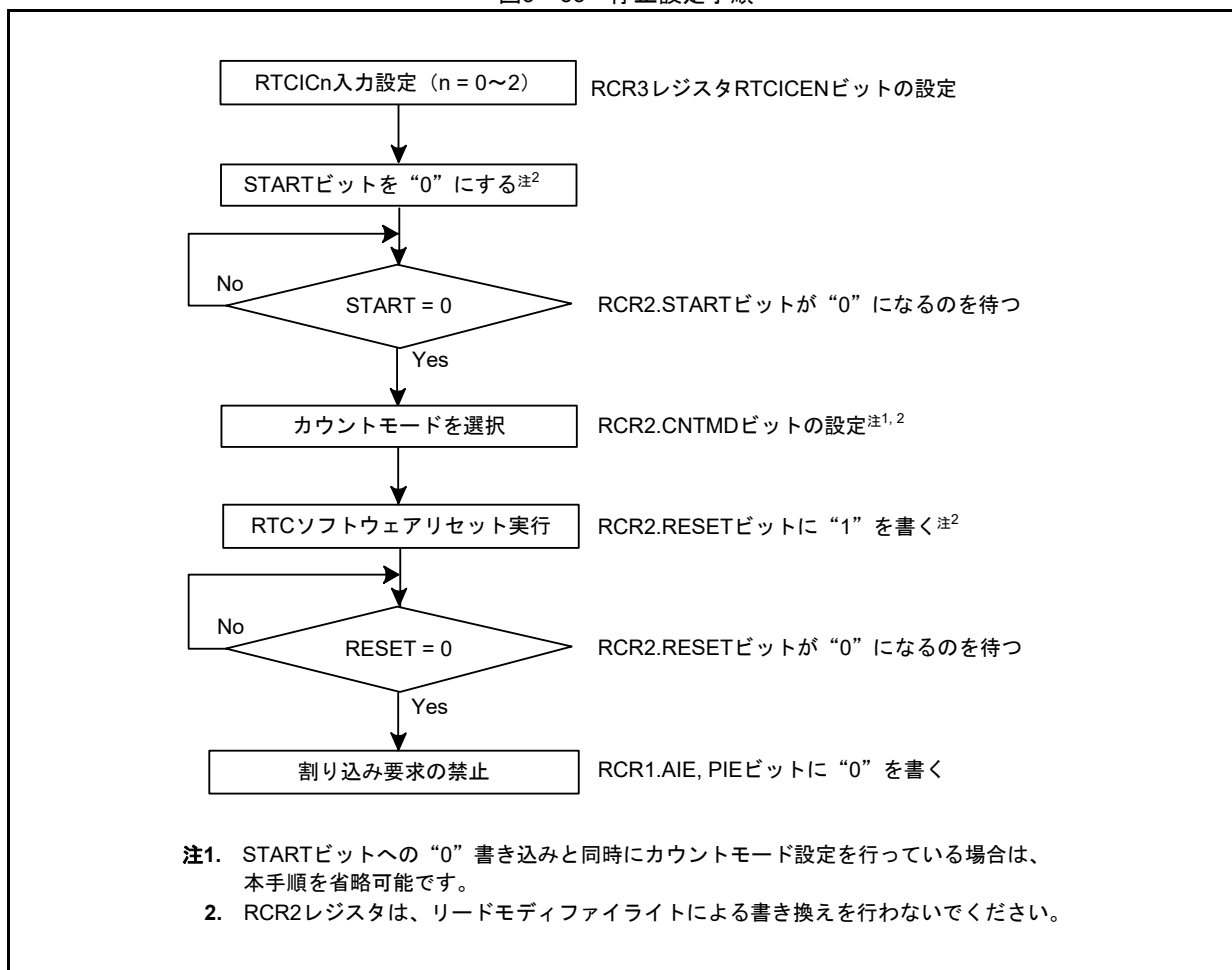
図9-66 停止設定手順
