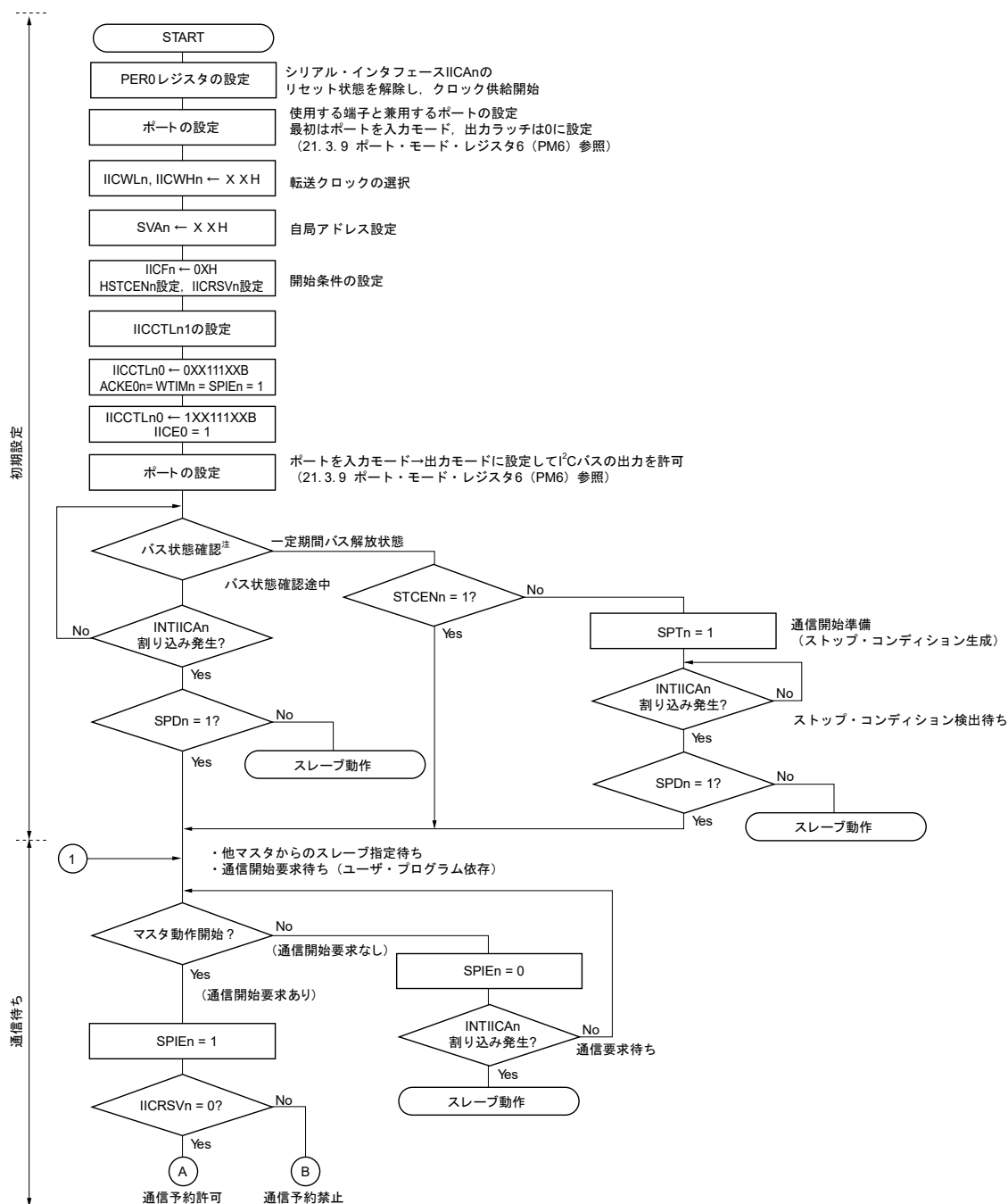
図21-30 マルチマスタ・システムでのマスタ動作 (1/3)
