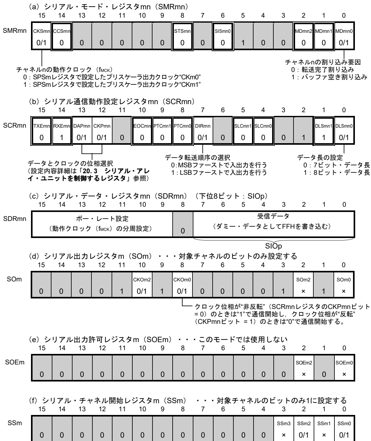
図20-35 簡易SPI (CSI00, CSI10, CSI30) のマスタ受信時のレジスタ設定内容例
