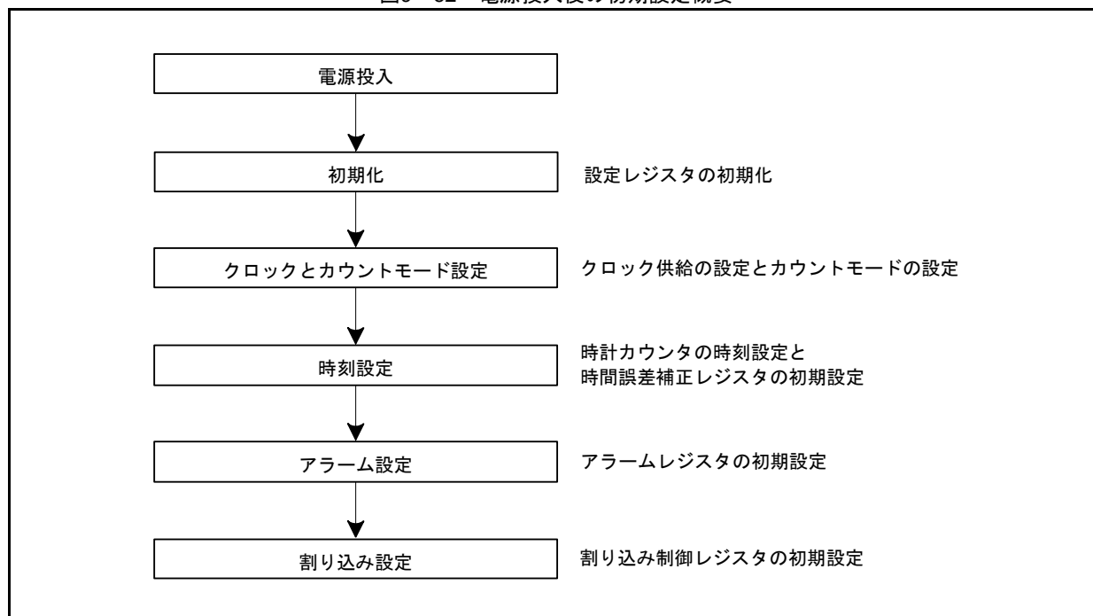
図9-52 電源投入後の初期設定概要
