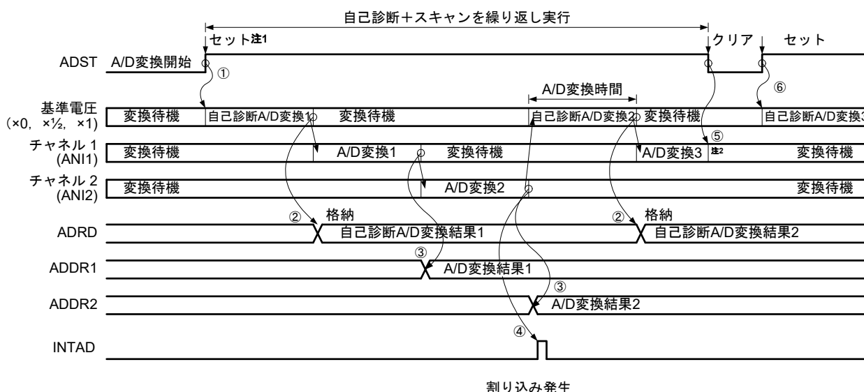
図17-26 連続スキャンモードの動作例（基本動作：ANI1, ANI2選択 + 自己診断）
