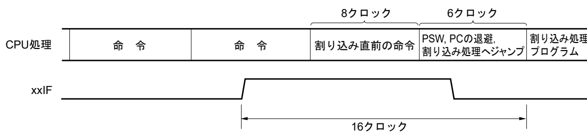
図27-9 割り込み要求の受け付けタイミング（最大時間）
