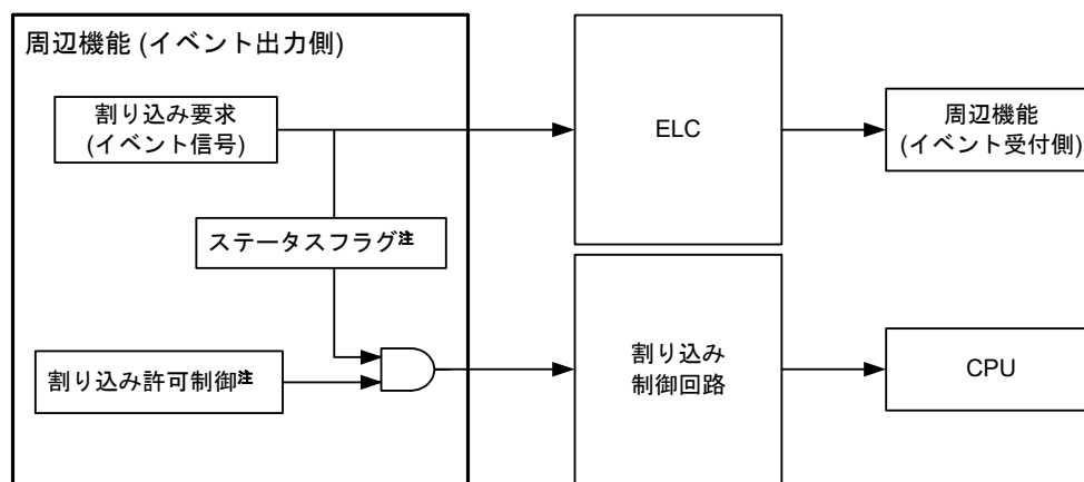
図26-5 割り込み処理とELCの関係
