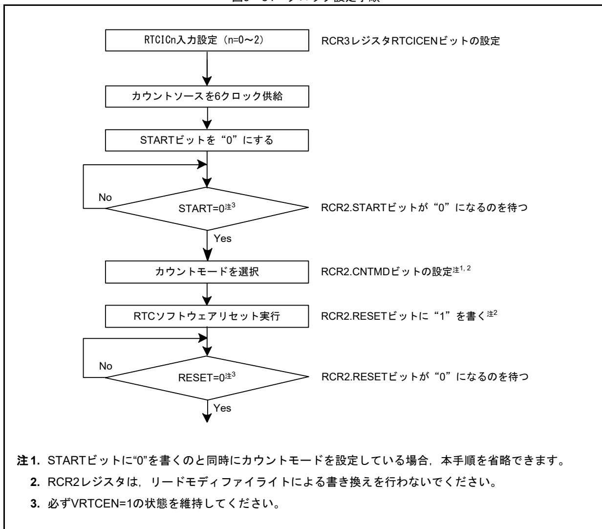
図9-54 クロック設定手順
