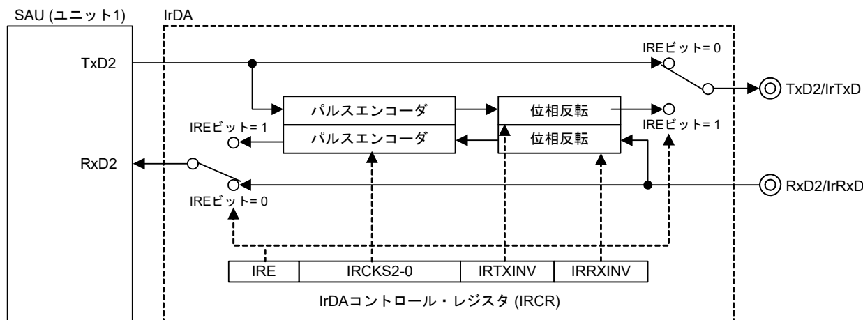
図23-1 IrDAとSAUの連携イメージのブロック図
