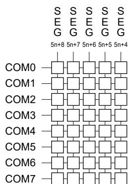
図24-41 8時分割LCD表示パターンと電極結線
