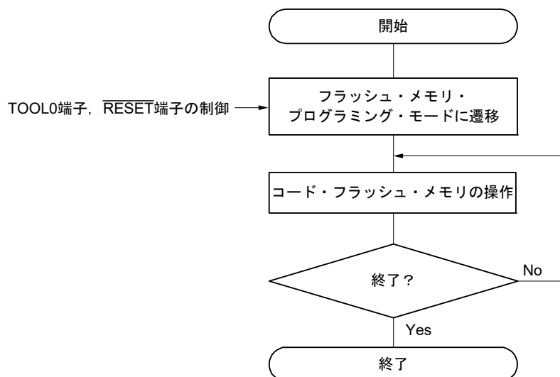
図38-6 コード・フラッシュメモリの操作手順
