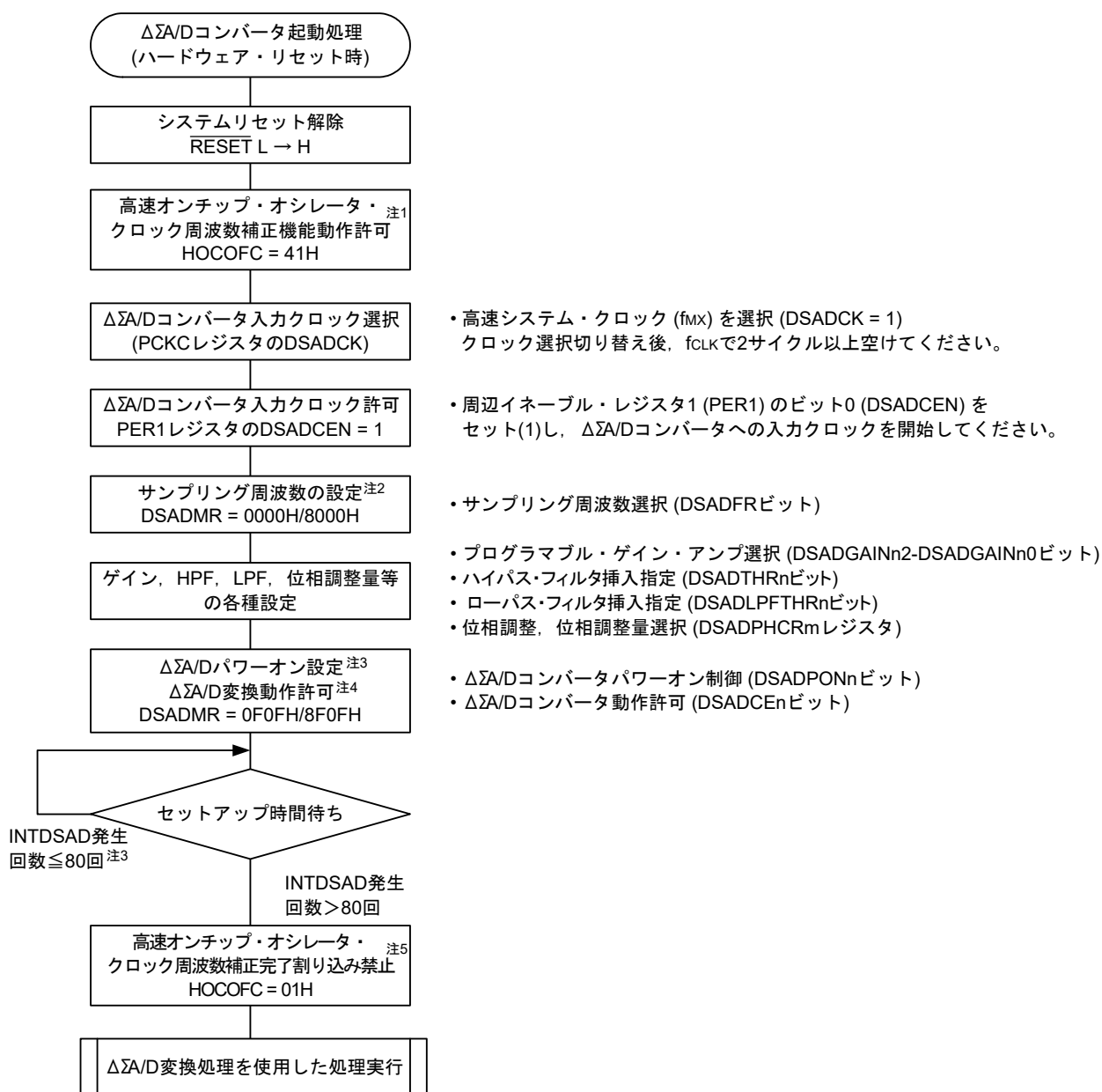
図19-16 初期設定フロー図
