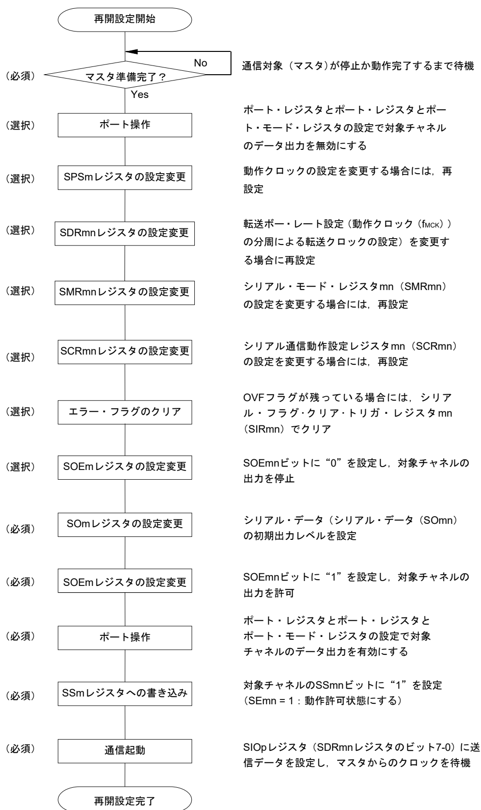
図20-54 スレーブ送信の再開設定手順
