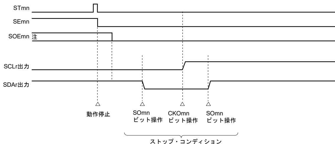
図20-115 ストップ・コンディション発生のタイミング・チャート
