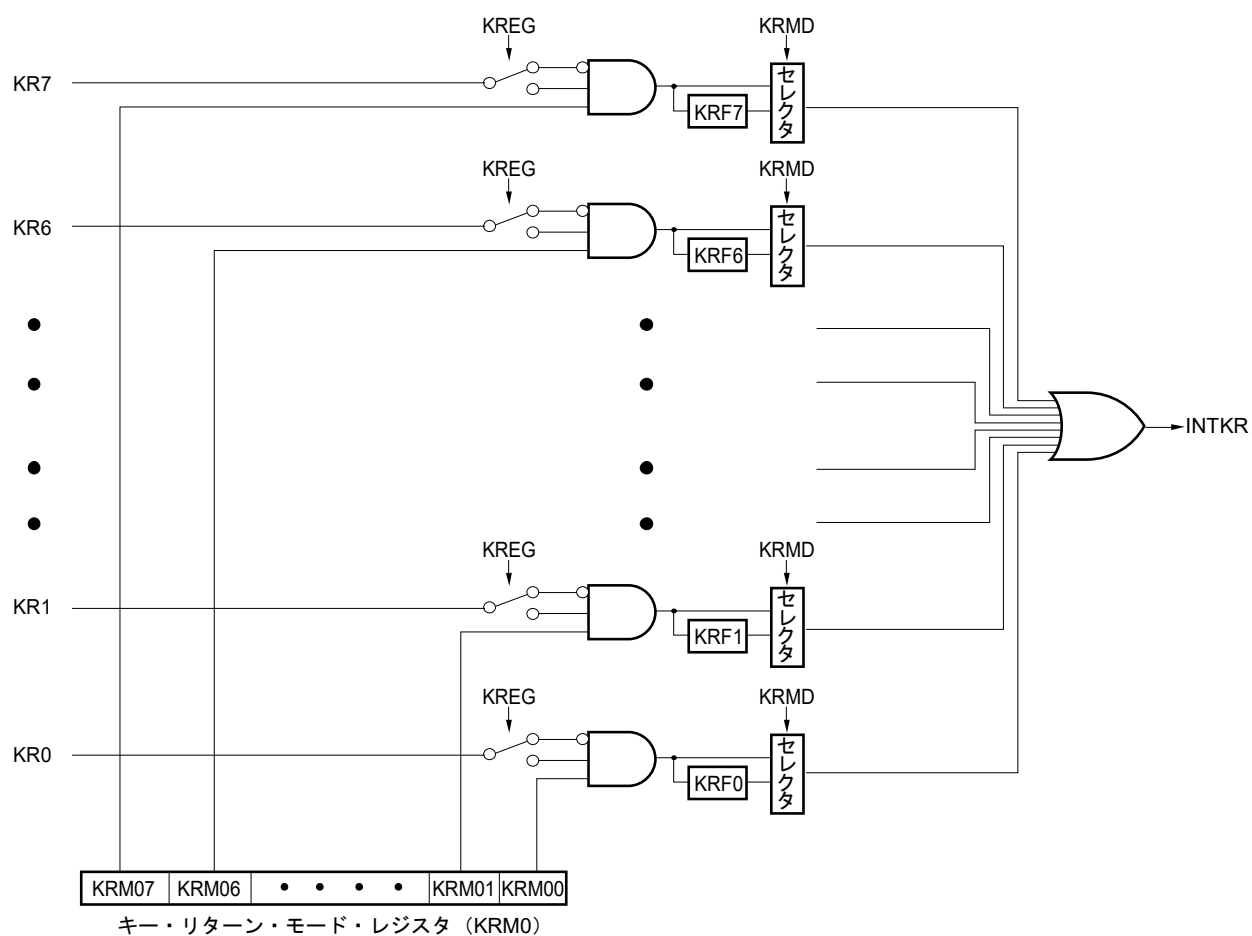
図28-1 キー割り込みのブロック図
