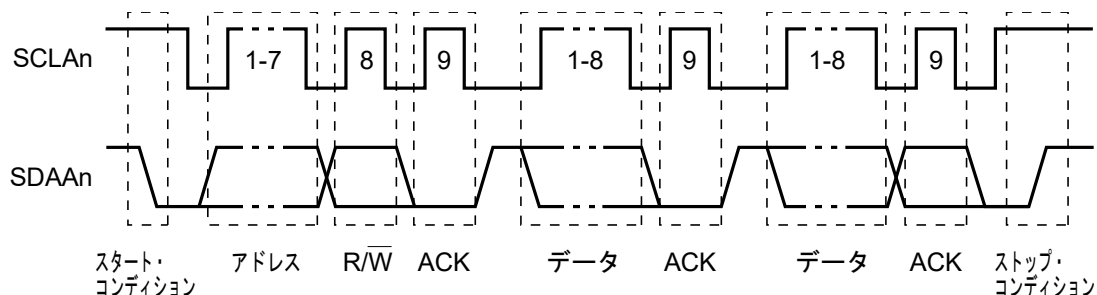
図21-15 I 2 Cバスのシリアル・データ転送タイミング
