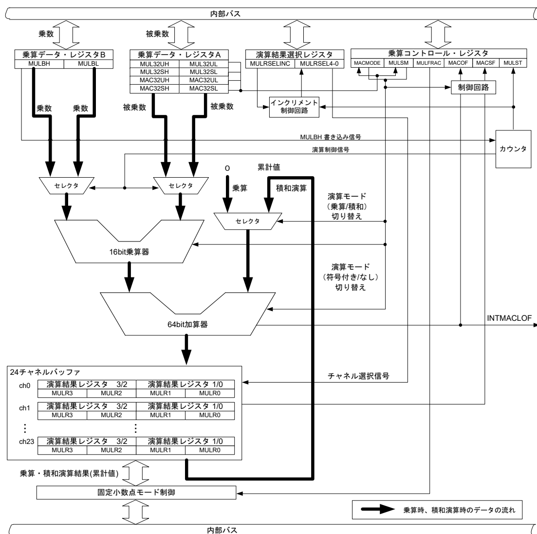
図41-1 32ビット積和演算回路のブロック図
