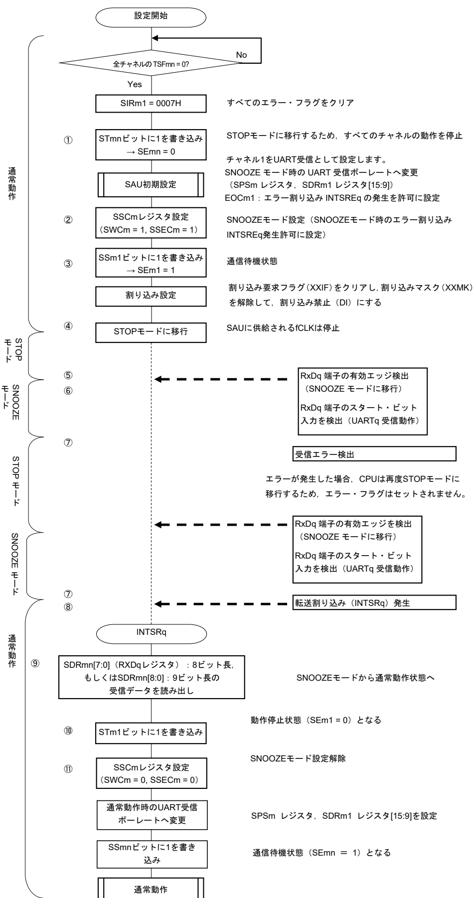
図20-96 SNOOZEモード動作 (EOCm1 = 1, SSECm = 1) 時のフロー・チャート
