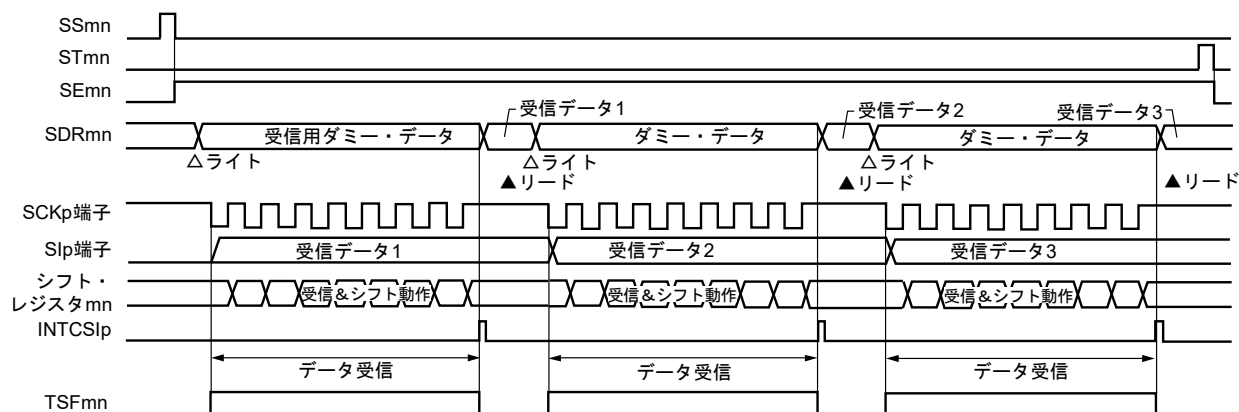
図20-39 マスタ受信 (シングル受信モード時) のタイミング・チャート (タイプ1: DAPmn = 0, CKPmn = 0)
