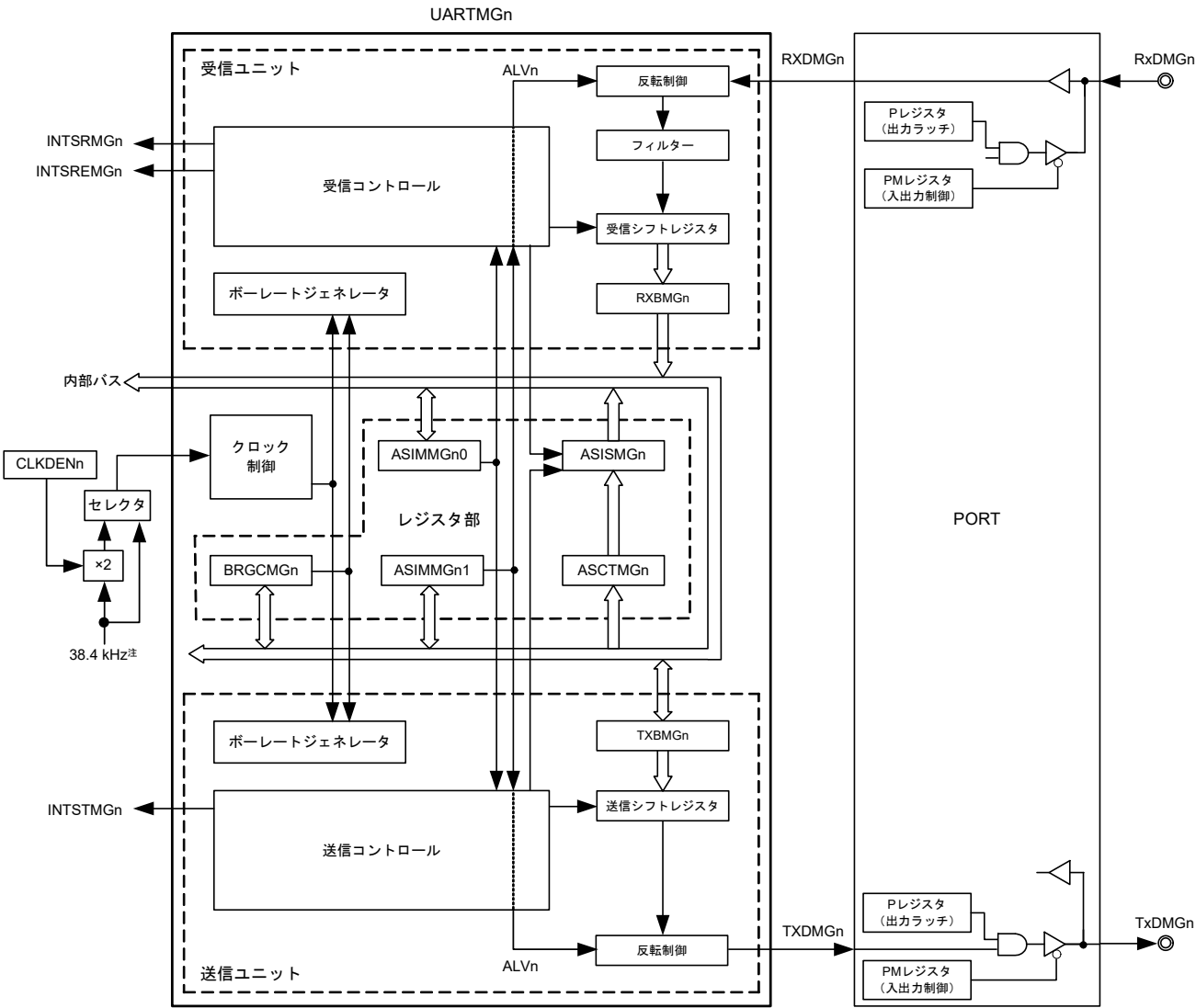
図22-1 UARTMGnのブロック図
