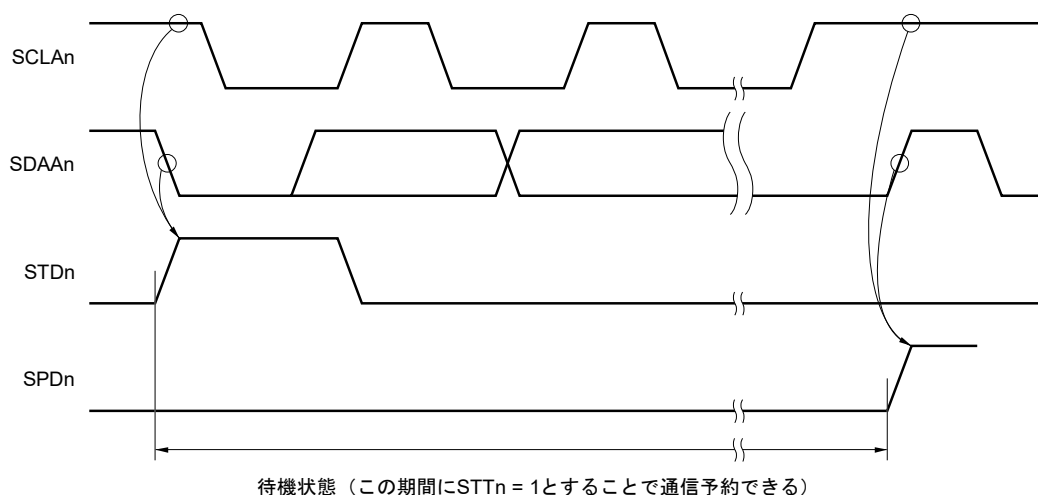
図21-27 通信予約受け付けタイミング
