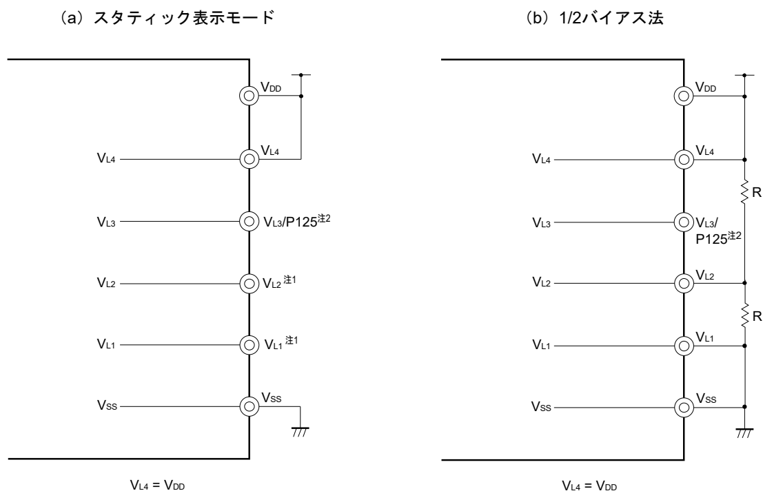
図24-20 LCD駆動用電源の接続例（外部抵抗分割方式）（1/2）
