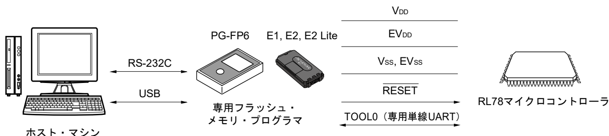
図38-1 フラッシュ・メモリにプログラムを書き込むための環境
