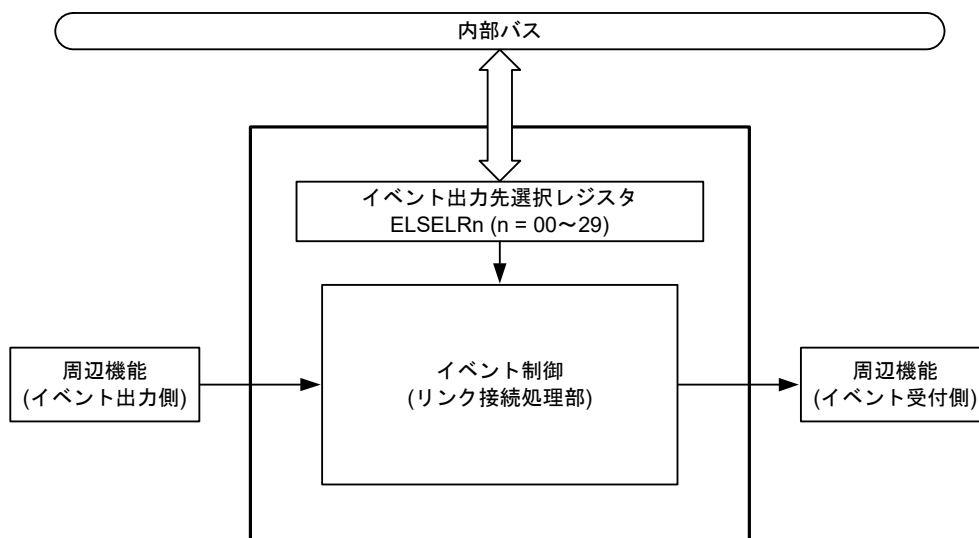
図26-1 ELCのブロック図
