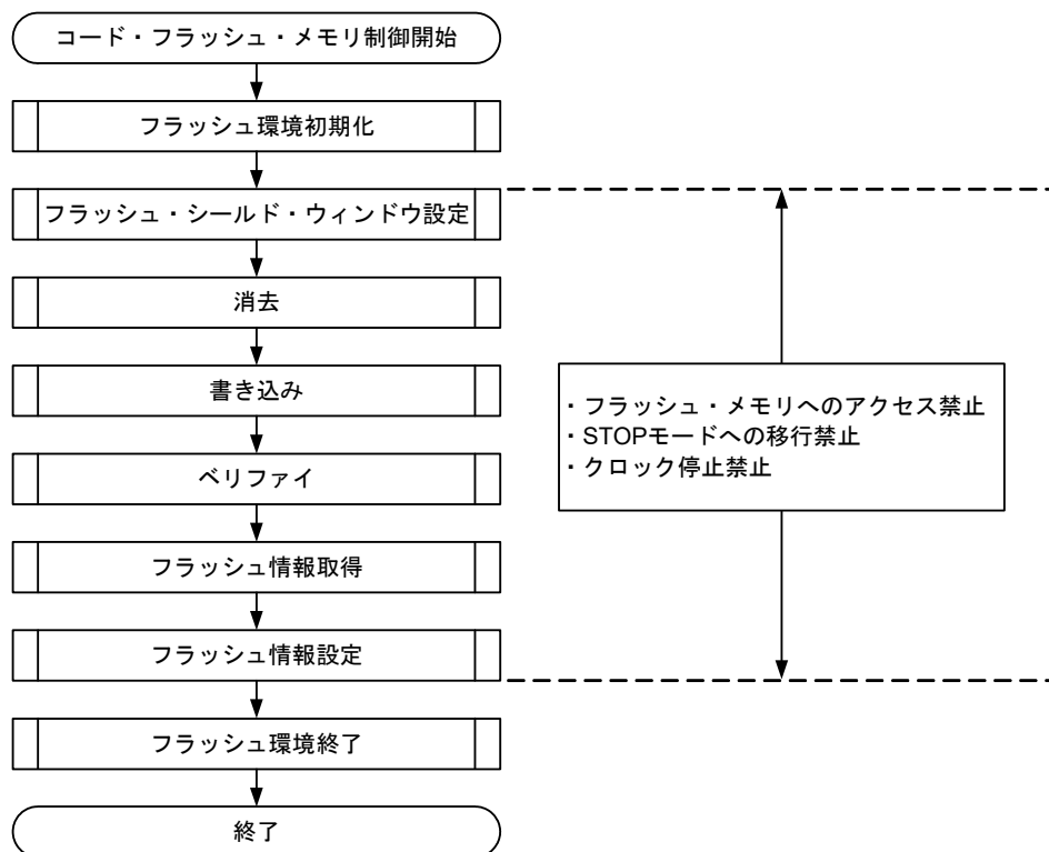
図38-8 セルフ・プログラミング（フラッシュ・メモリの書き換え）の流れ
