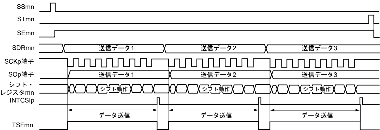
図20-31 マスタ送信（シングル送信モード時）のタイミング・チャート（タイプ1：DAPmn = 0, CKPmn = 0）
