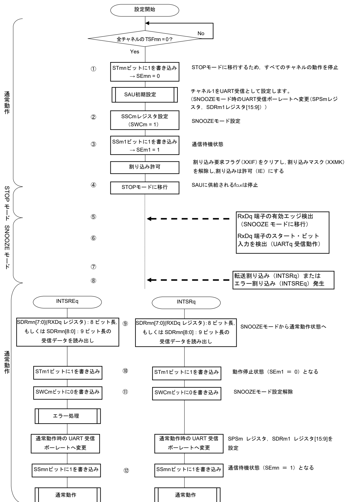
図20-94 SNOOZEモード動作 (EOCm1 = 0, SSECm = 0/1もしくはEOCm1 = 1, SSECm = 0) 時の フロー・チャート
