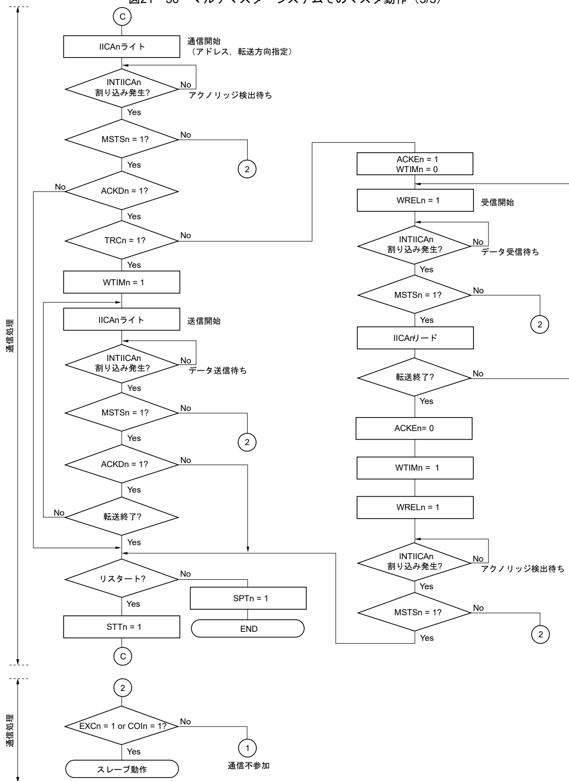
図21-30 マルチマスタ・システムでのマスタ動作 (3/3)
