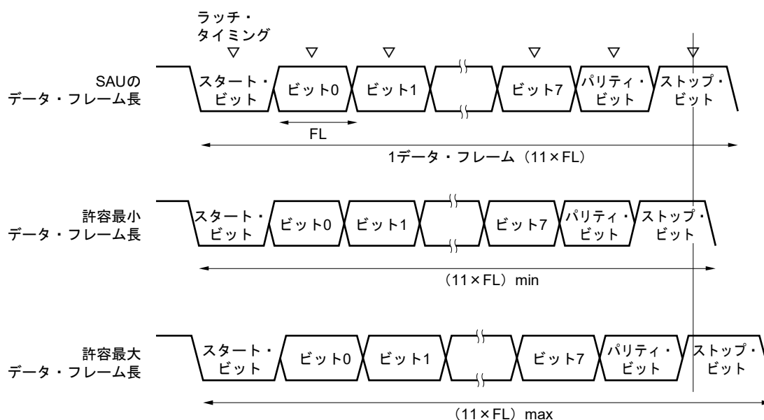
図20-97 受信時の許容ボー・レート範囲 (1データ・フレーム長 = 11ビットの場合)
