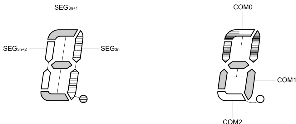
図24-31 3時分割LCD表示パターンと電極結線
