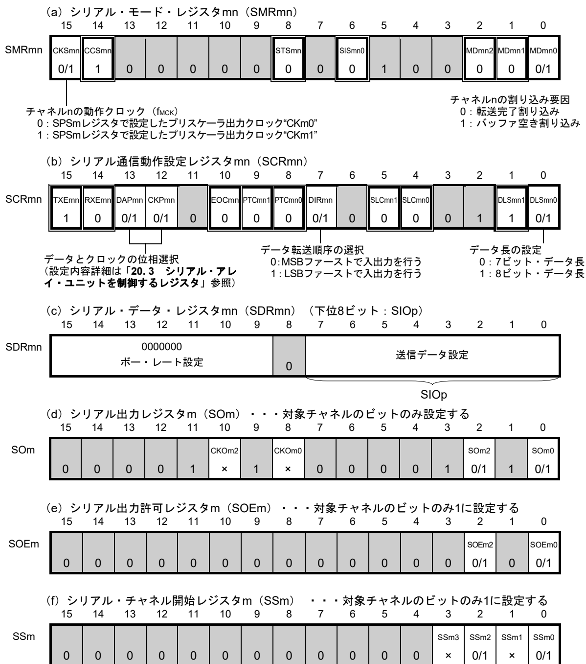
図20-51 簡易SPI (CSI00, CSI10, CSI30) のスレーブ送信時のレジスタ設定内容例
