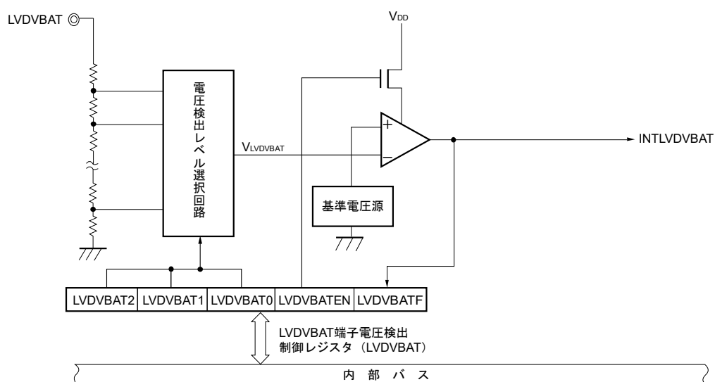
図32-3 LVDVBAT端子電圧検出回路のブロック図
