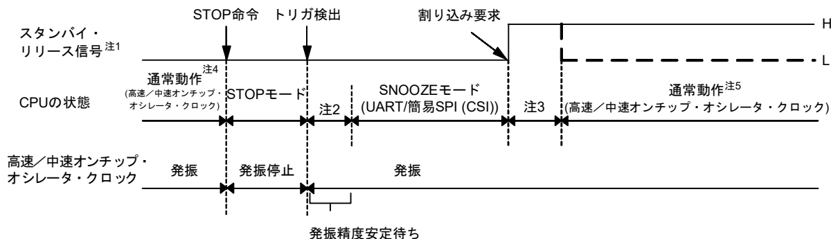
図29-5 SNOOZEモードの割り込み要求が発生する場合
