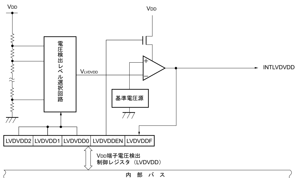
図32-2 V DD 端子電圧検出回路のブロック図
