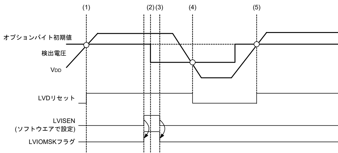
図32-26 LVDリセット・モード時のLVD検出電圧設定変更タイミング例
