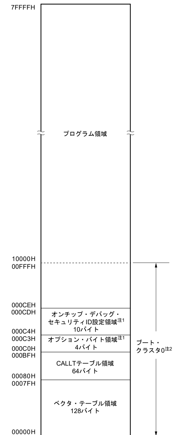
(A) ユーザモードのメモリマップ
