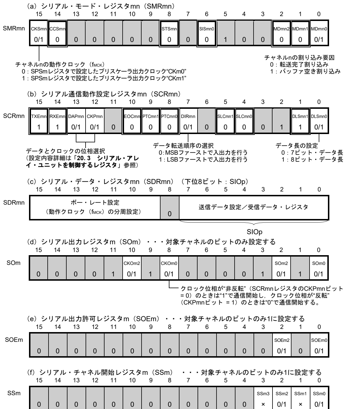
図20-43 簡易SPI (CSI00, CSI10, CSI30) のマスタ送受信時のレジスタ設定内容例
