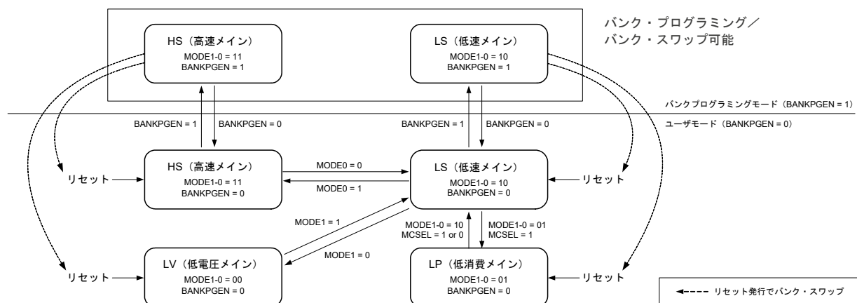
図38-11 バンクプログラミング時のFLASH状態遷移図
