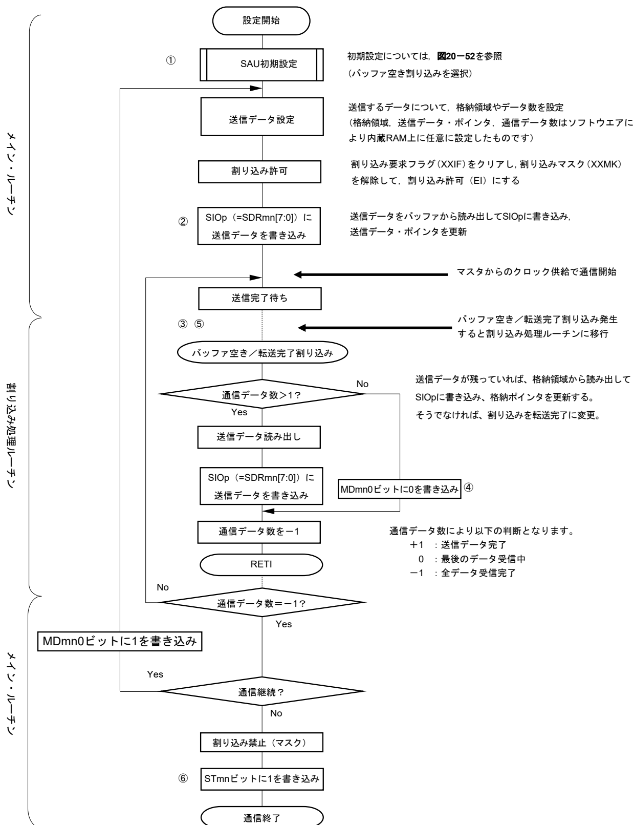
図20-58 スレーブ送信（連続送信モード時）のフロー・チャート
