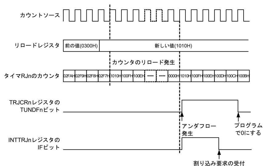
図13-12 タイマモードの動作例
