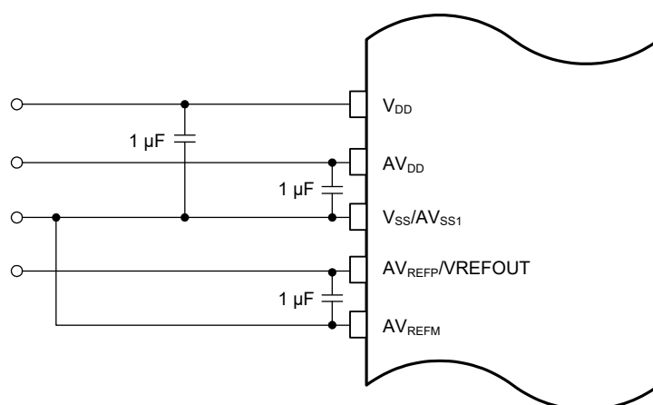
図17-32 各電源端子の接続例
