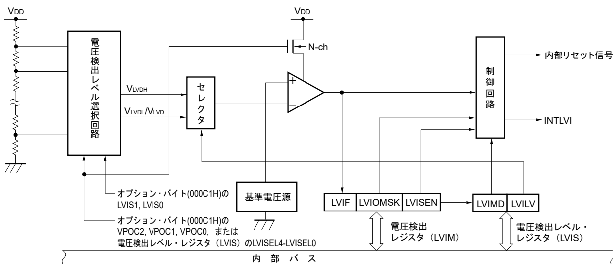
図32-1 電圧検出 (LVD) 回路のブロック図
