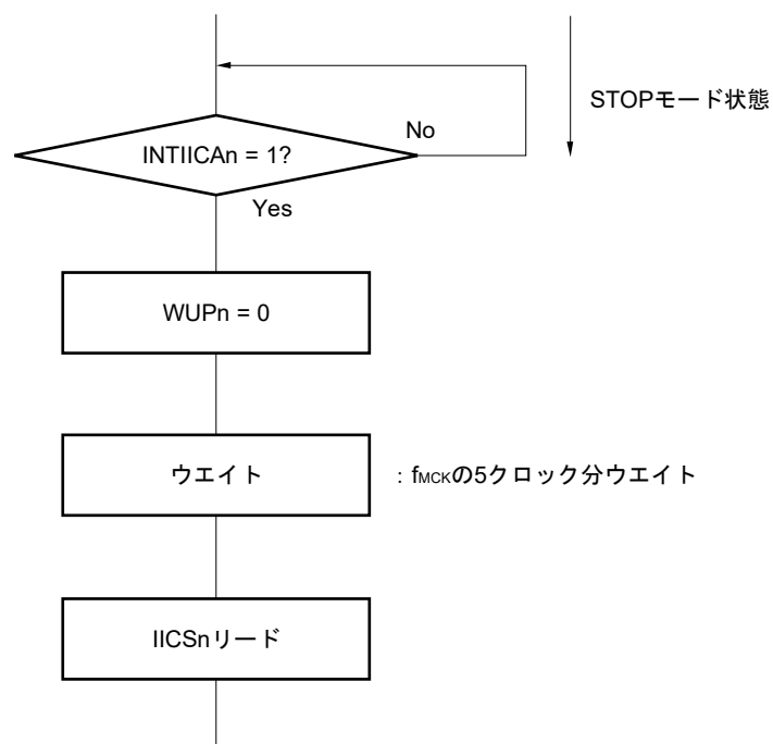
図21-24 アドレス一致によりWUPn = 0に設定する場合のフロー（拡張コード受信含む）
