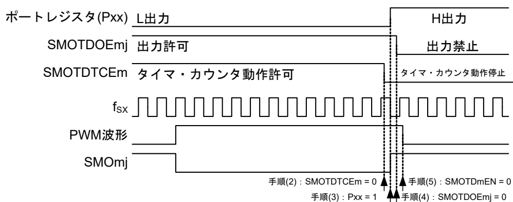
図14-25 SMOMj端子をロウ・アクティブで使用時の動作停止タイミング(SMOTDPOLm = 1の場合)
