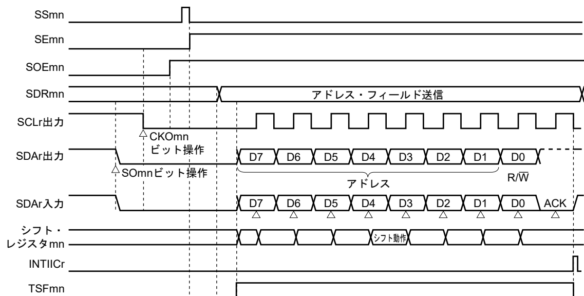
図20-107 アドレス・フィールド送信のタイミング・チャート
