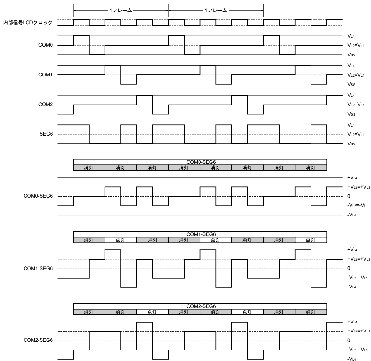
図24-33 SEG6と各コモン信号間の3時分割LCD駆動波形例（1/2バイアス法）
