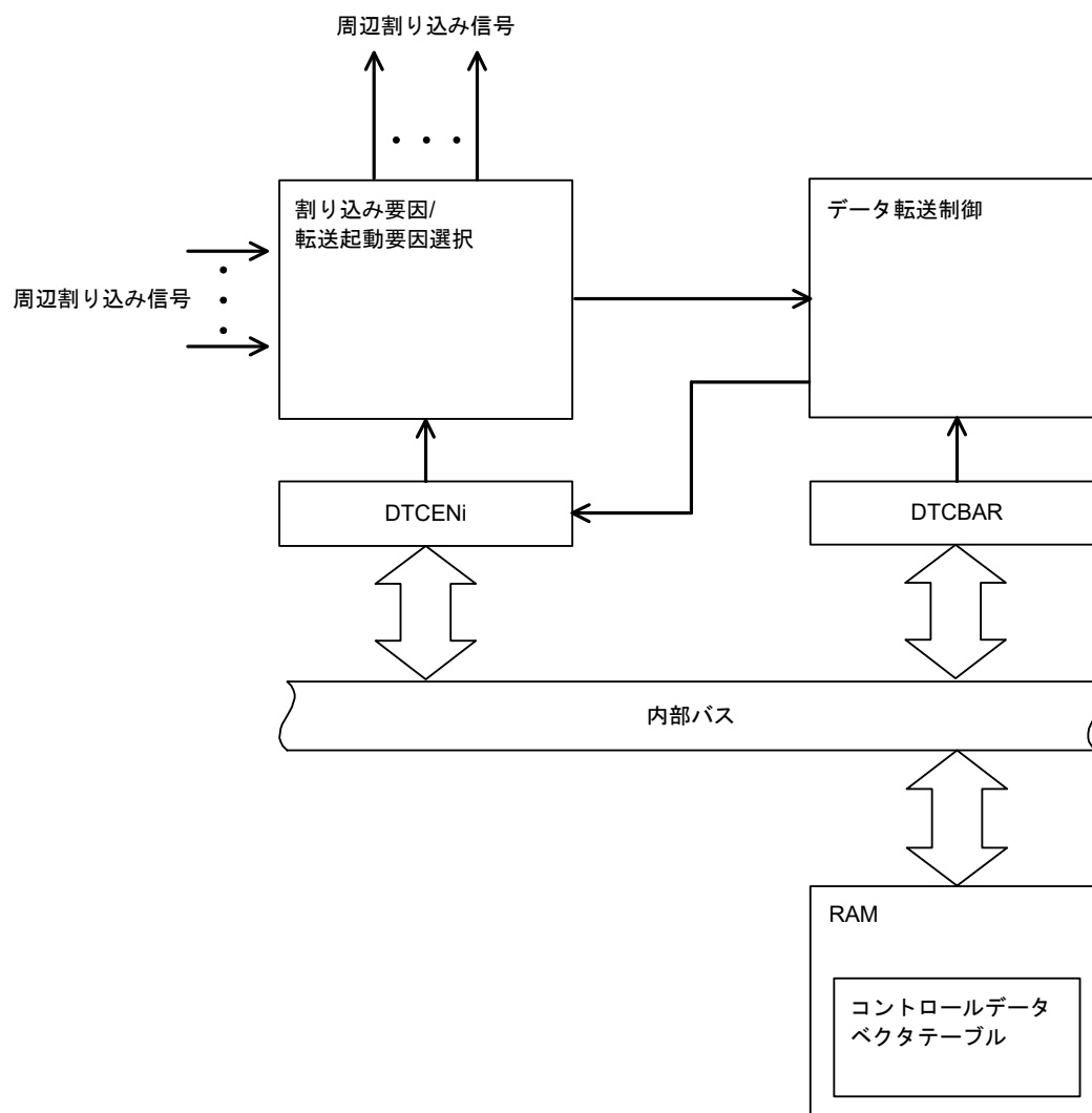
図25-1 DTCのブロック図
