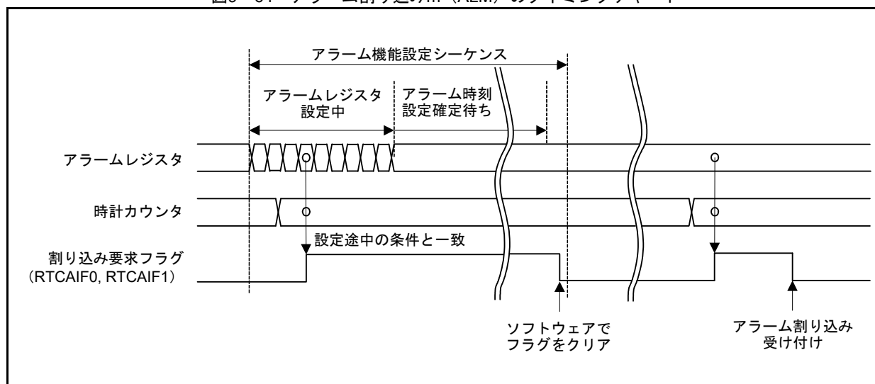
図9-64 アラーム割り込みm (ALM) のタイミングチャート
