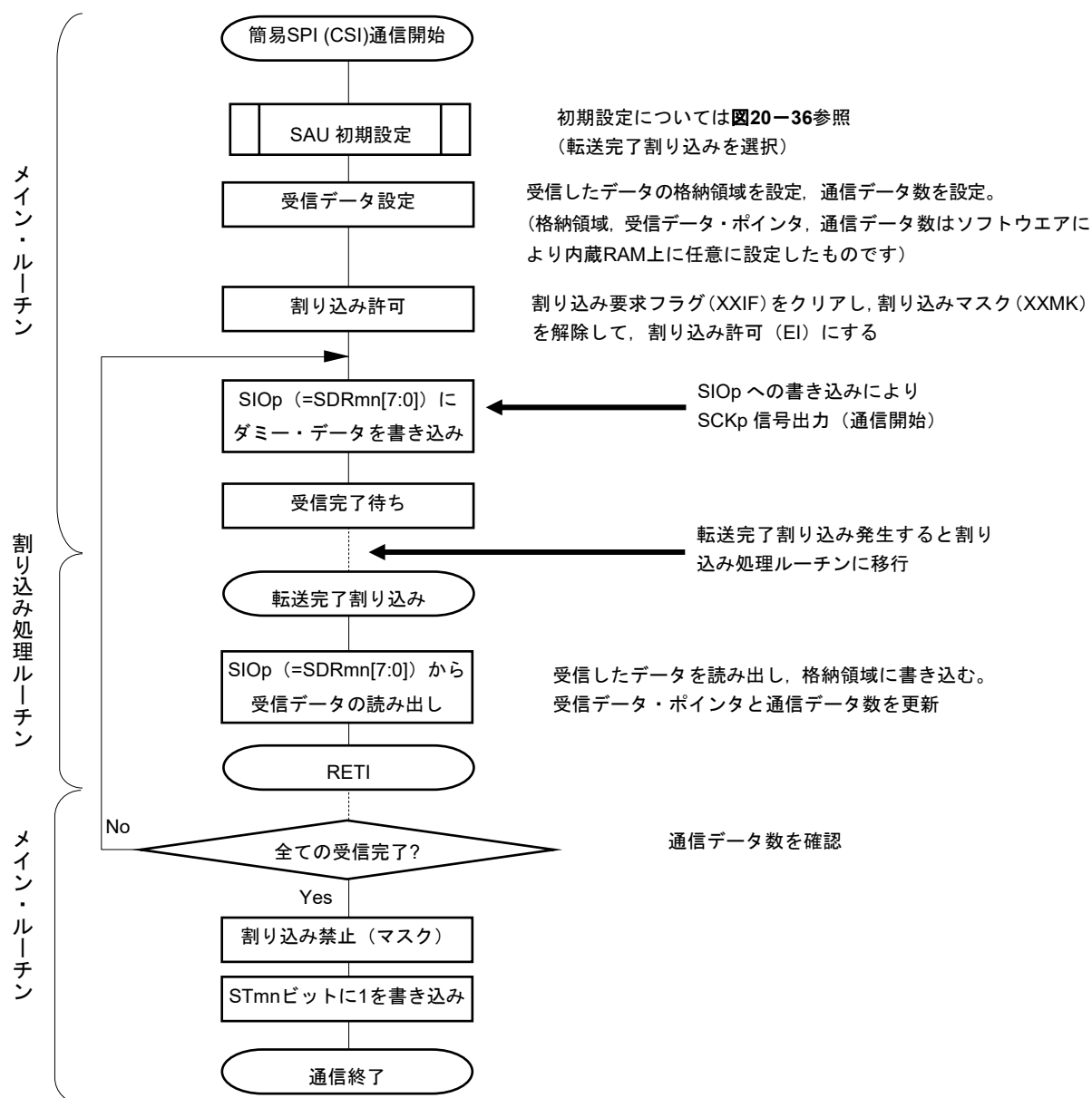
図20-40 マスタ受信（シングル受信モード時）のフロー・チャート
