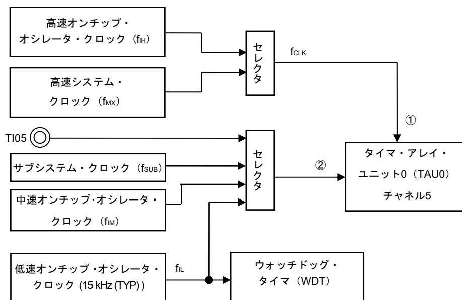
図34-13 周波数検出機能の構成
