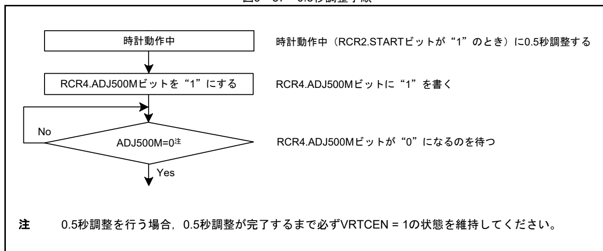
図9-57 0.5秒調整手順
