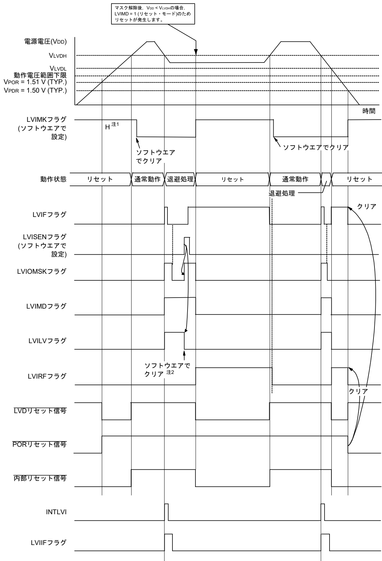
図32-19 割り込み&amp;リセット信号発生タイミング (オプション・バイトLVIMDS1, LVIMDS0 = 1, 0) (2/2)
