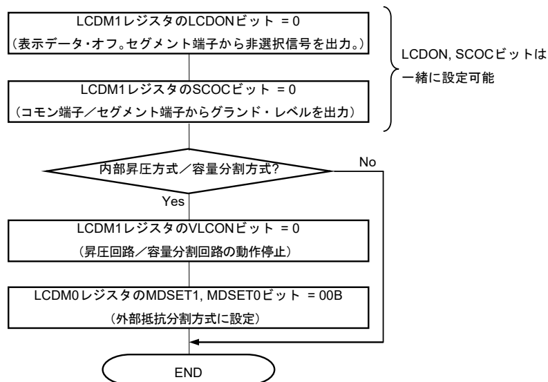
図24-19 動作停止手順
