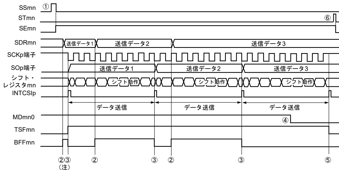
図20-33 マスタ送信（連続送信モード時）のタイミング・チャート（タイプ1：DAPmn = 0, CKPmn = 0）
