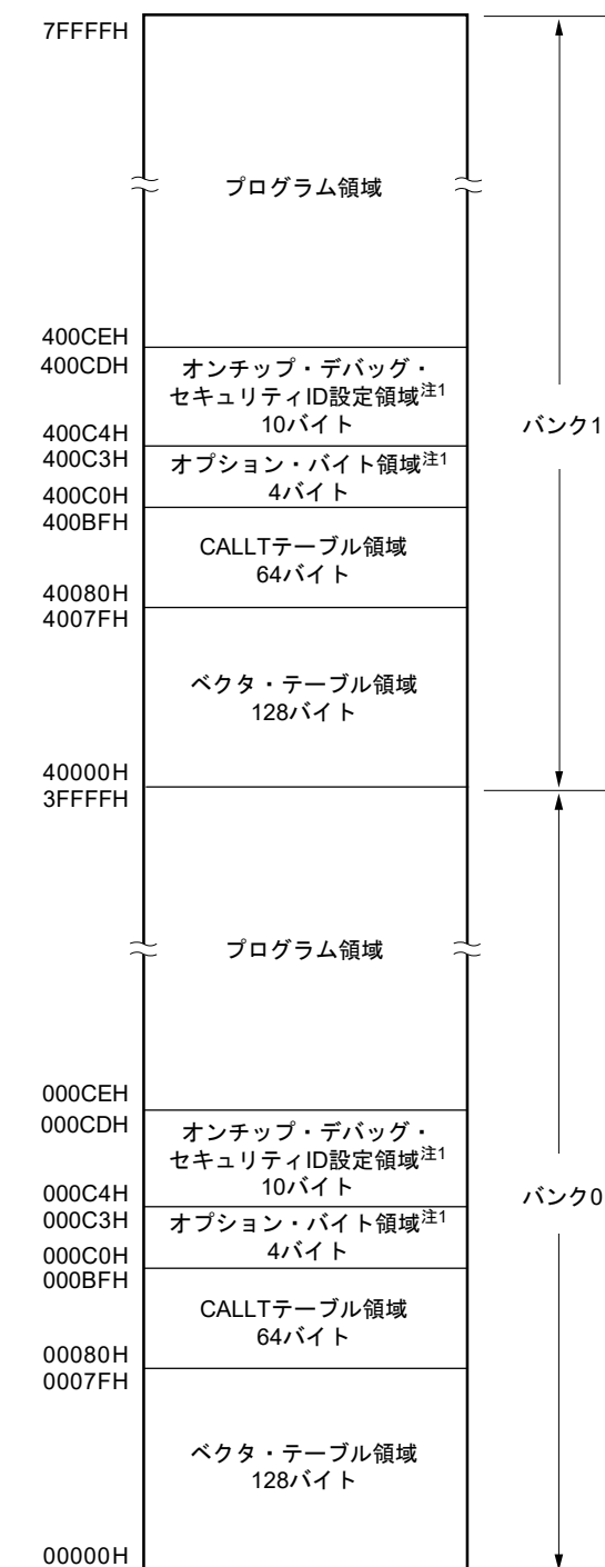
(B) バンクプログラミングモードのメモリマップ
