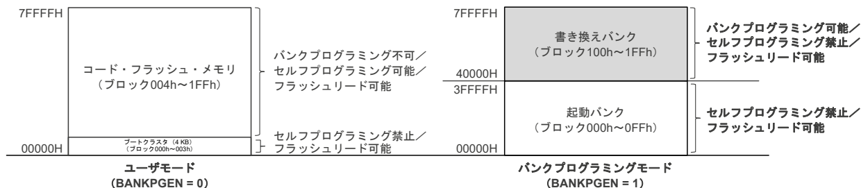
図38-10 バンクプログラミング機能
