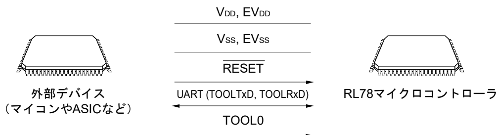
図38-3 フラッシュ・メモリにプログラムを書き込むための環境
