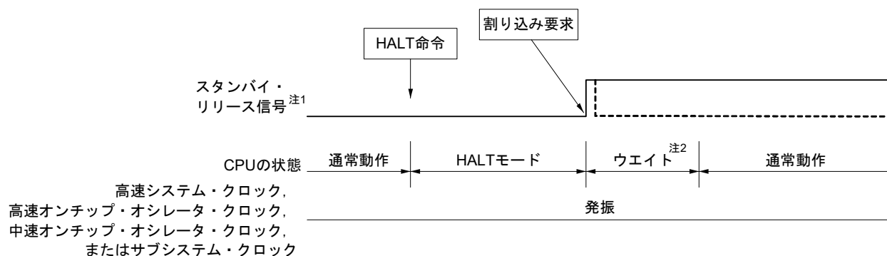
図29-1 HALTモードの割り込み要求発生による解除
