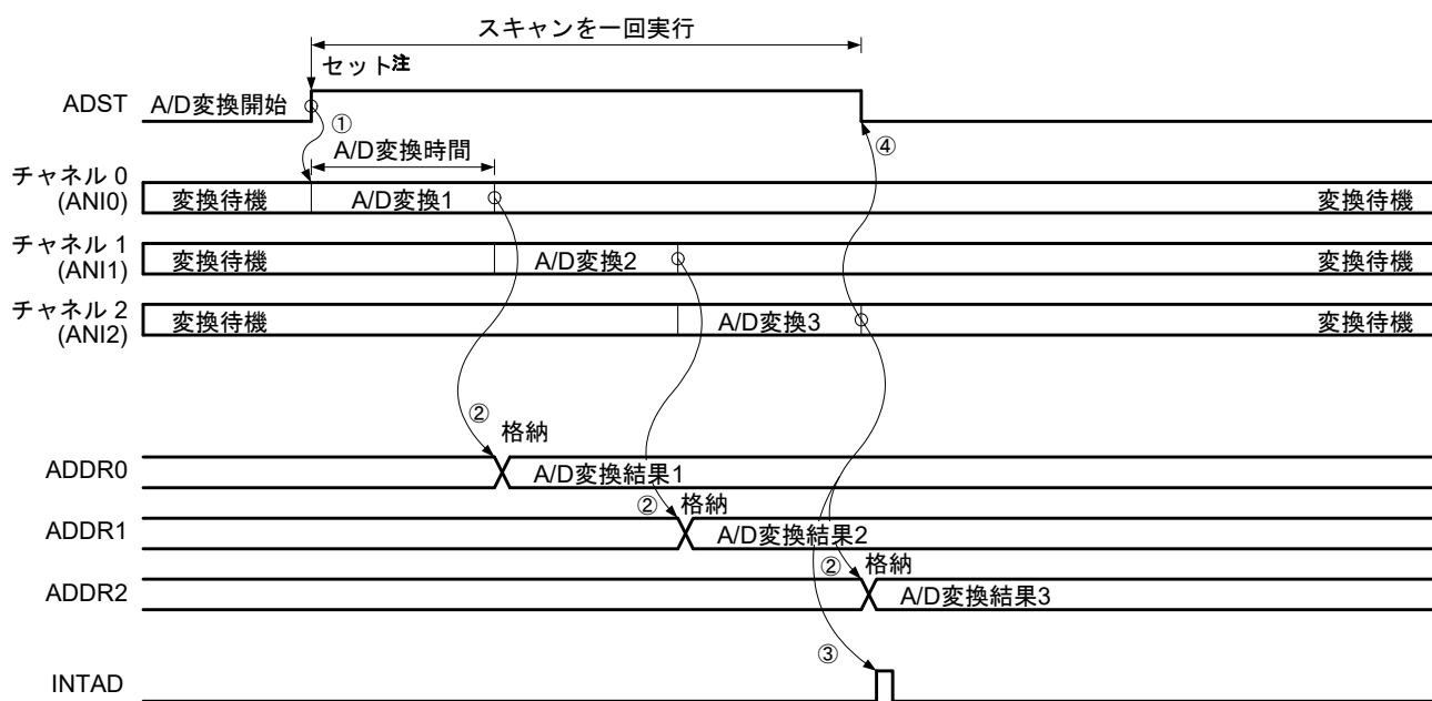
図17-19 シングルスキャンモードの動作例（基本動作：ANI0, ANI1, ANI2選択）
