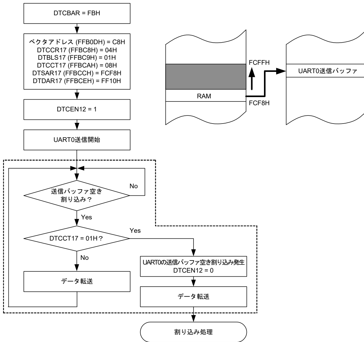
図25-17 ノーマルモードの使用例2 : UART0連続送信
