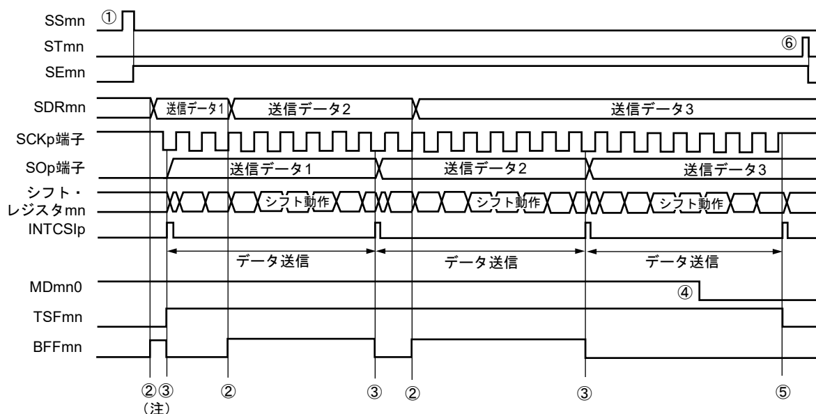
図20-57 スレーブ送信（連続送信モード時）のタイミング・チャート（タイプ1：DAPmn = 0, CKPmn = 0）
