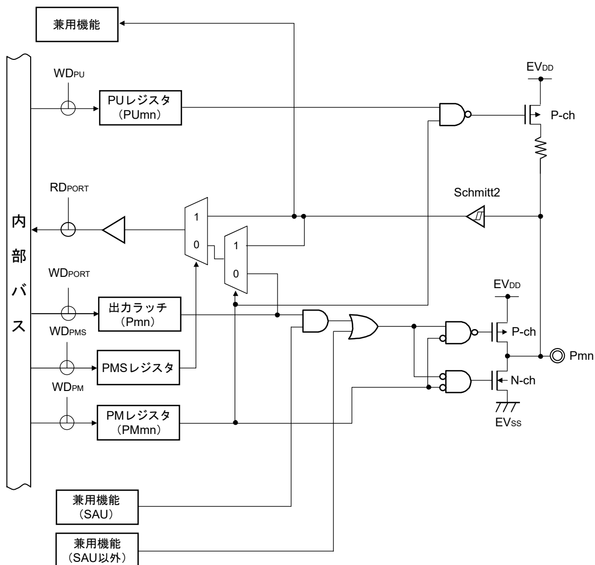
図2-8 端子タイプ7-1-3の端子ブロック図
