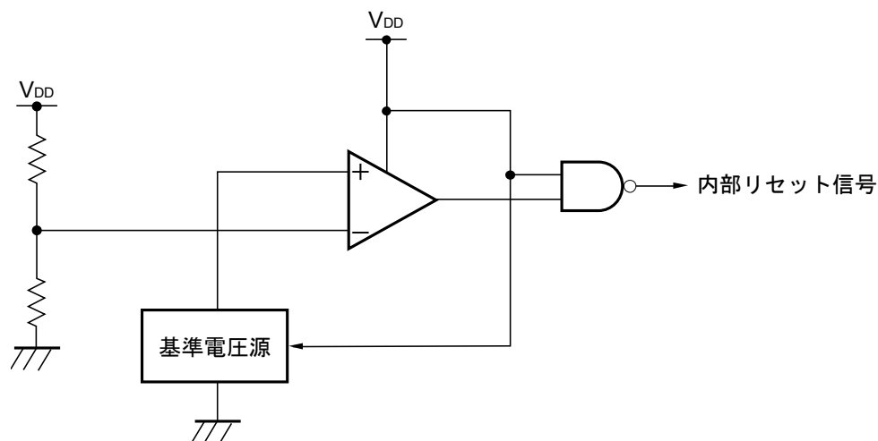
図31-1 パワーオン・リセット回路のブロック図
