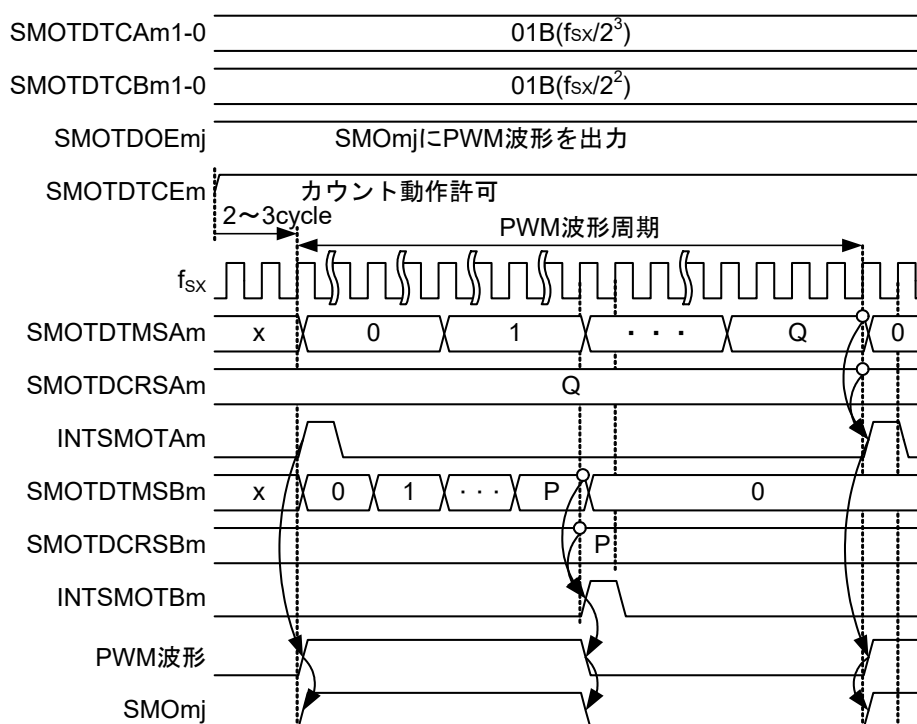
図14-18 サンプリング・クロック出力(分周あり)
