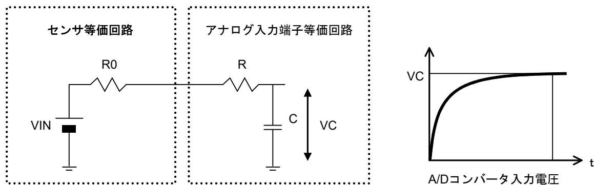
図17-30 アナログ入力端子と外部センサの等価回路
