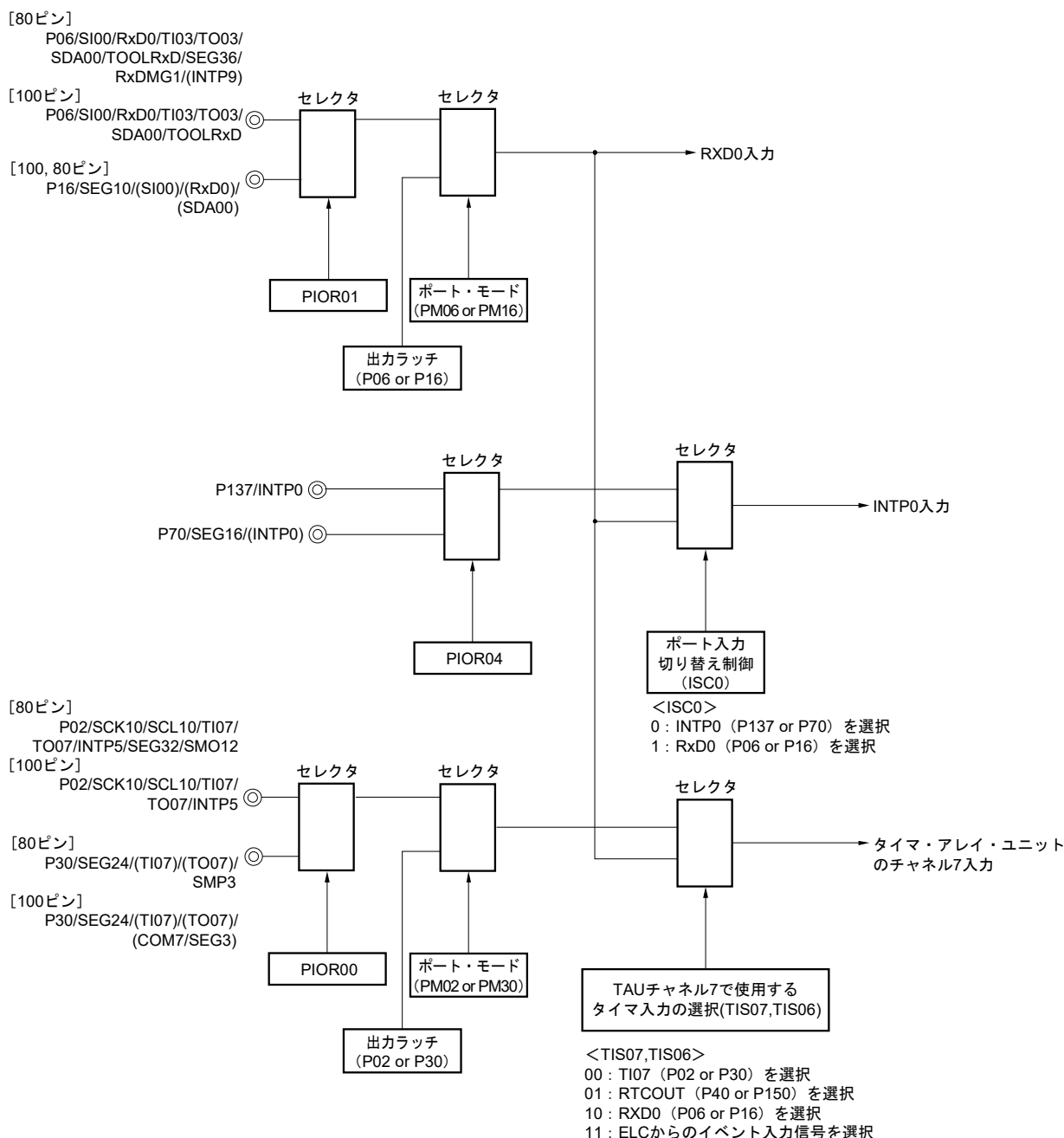
図20-104 LINの受信操作のポート構成図
