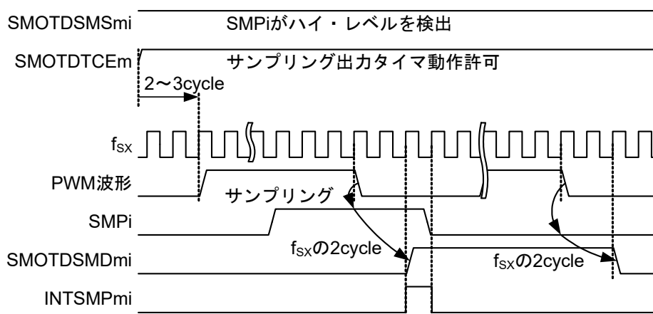
図14-19 サンプリング・クロック出力機能
