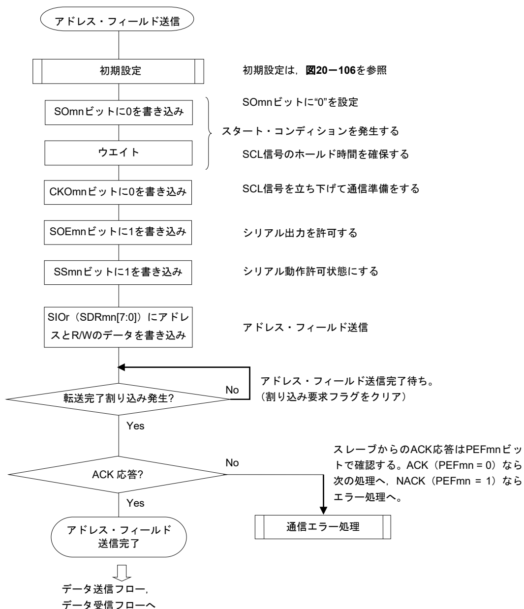
図20-108 簡易I 2 Cアドレス・フィールド送信のフロー・チャート
