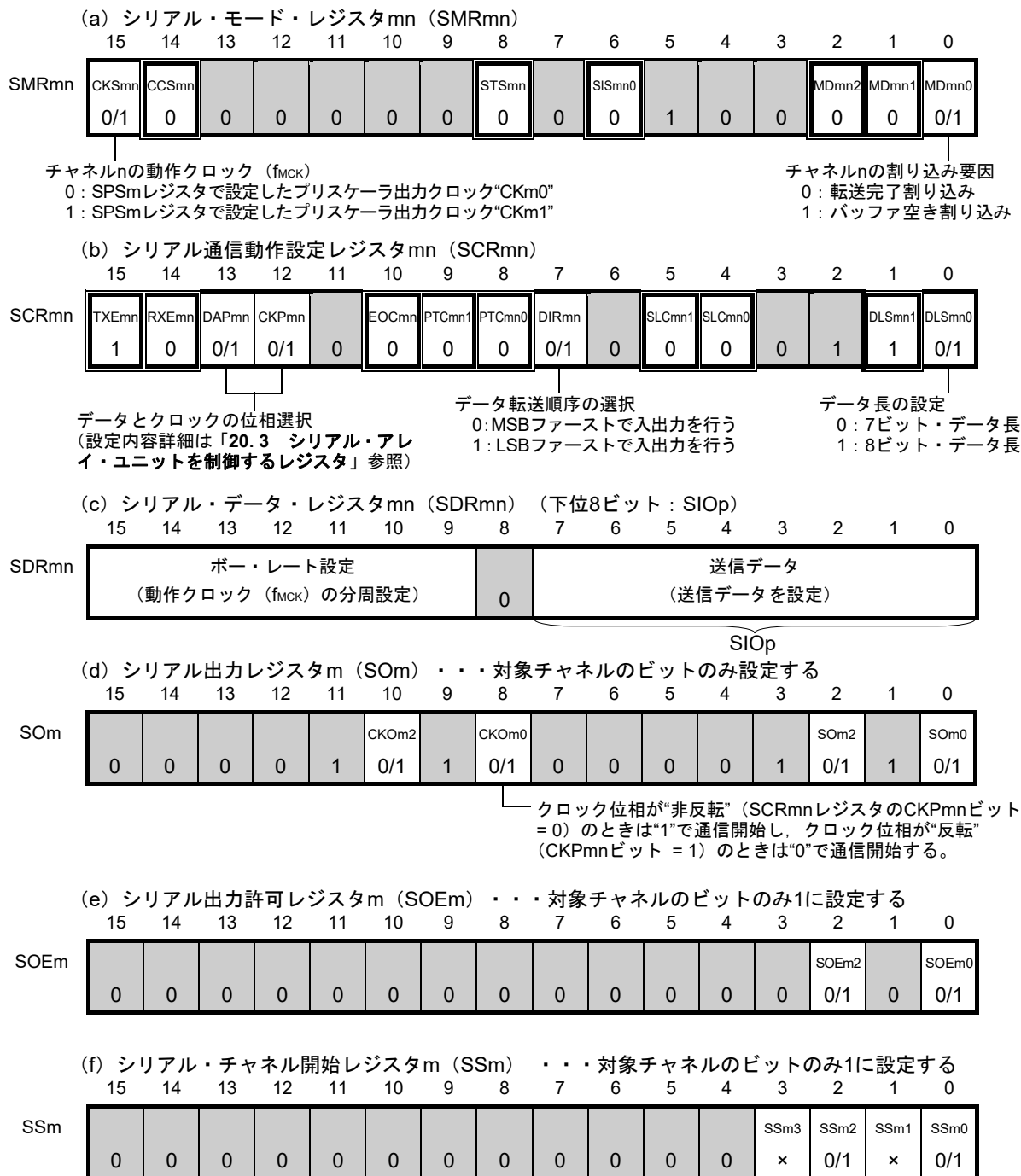
図20-27 簡易SPI (CSI00, CSI10, CSI30) のマスタ送信時のレジスタ設定内容例
