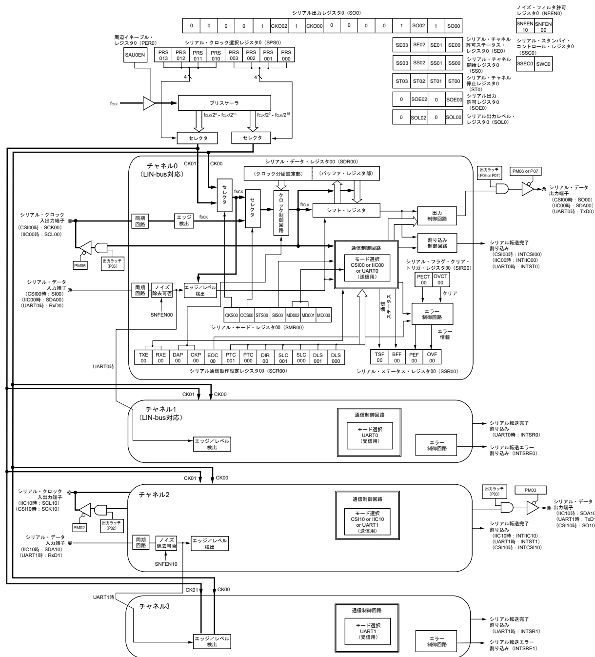
図20-1 シリアル・アレイ・ユニット0のブロック図
