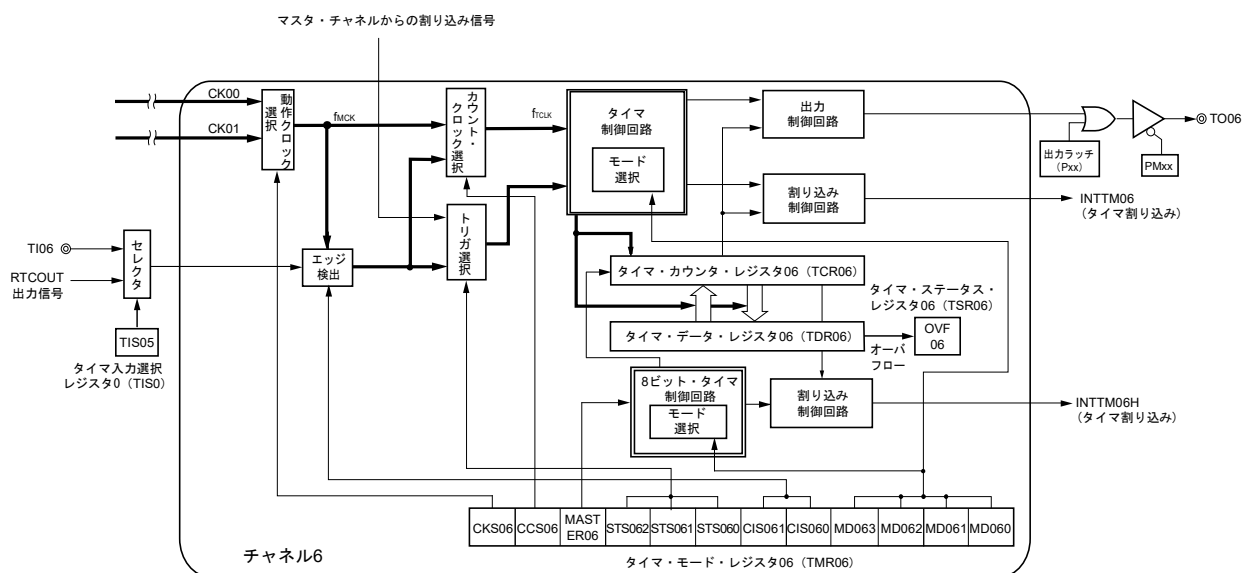
図8-7 タイマ・アレイ・ユニットのチャンネル6内部ブロック図
