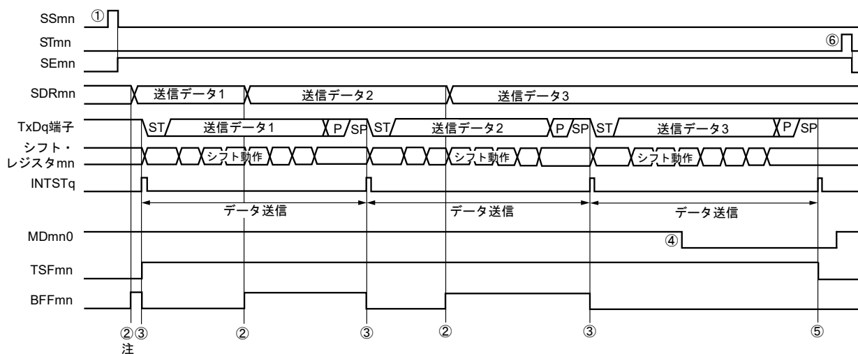
図20-84 UART送信（連続送信モード時）のタイミング・チャート
