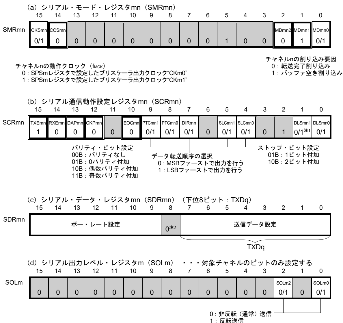
図20-78 UART (UART0-UART4) のUART送信時のレジスタ設定内容例 (1/2)
