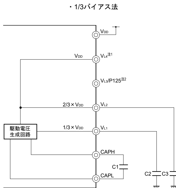
図24-22 LCD駆動用電源の接続例（容量分割方式）
