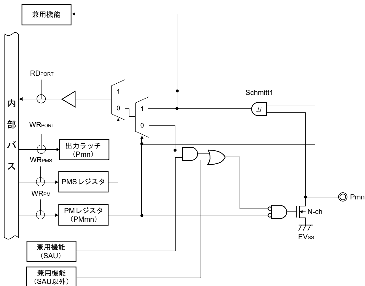
図2-16 端子タイプ12-1-2の端子ブロック図
