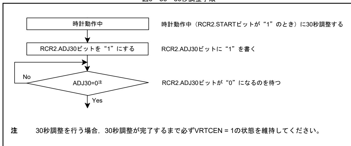
図9-56 30秒調整手順
