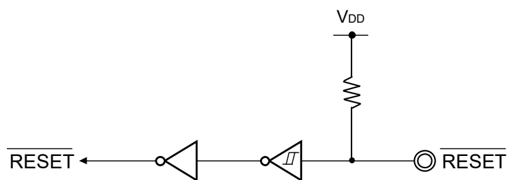
図2-3 端子タイプ3-1-1の端子ブロック図
