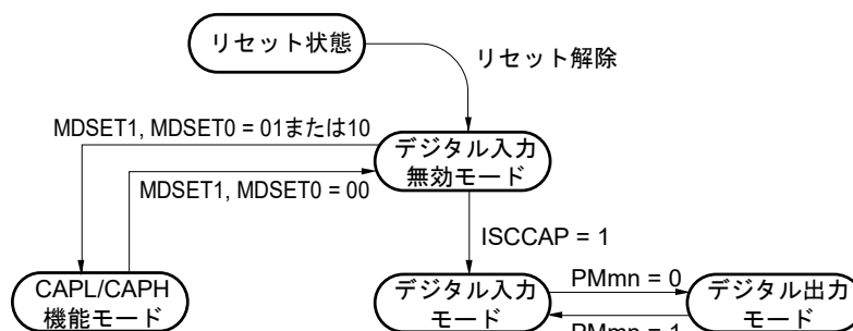
図24－9 CAPL/P126, CAPH/P127端子機能の状態遷移図
