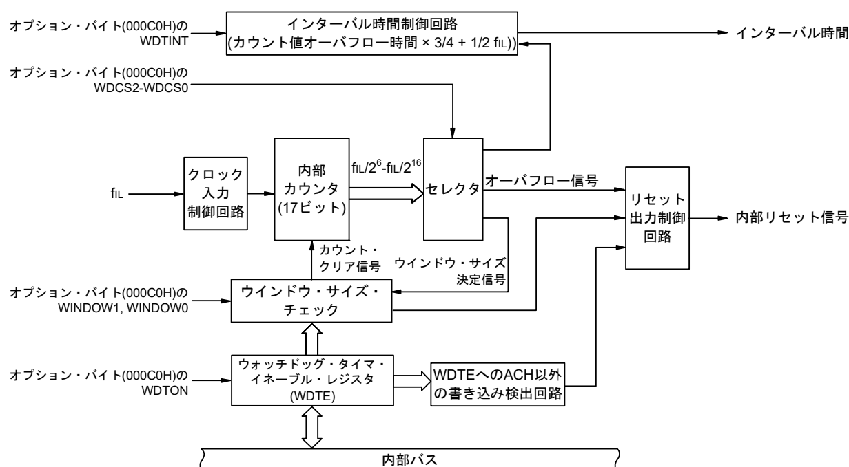
図16-1 ウォッチドッグ・タイマのブロック図
