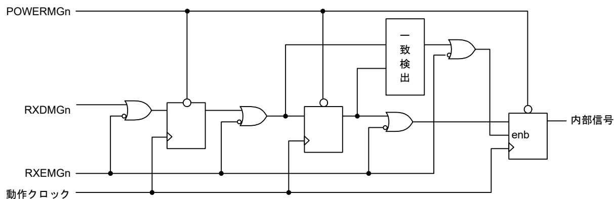
図22-22 ノイズフィルタ
