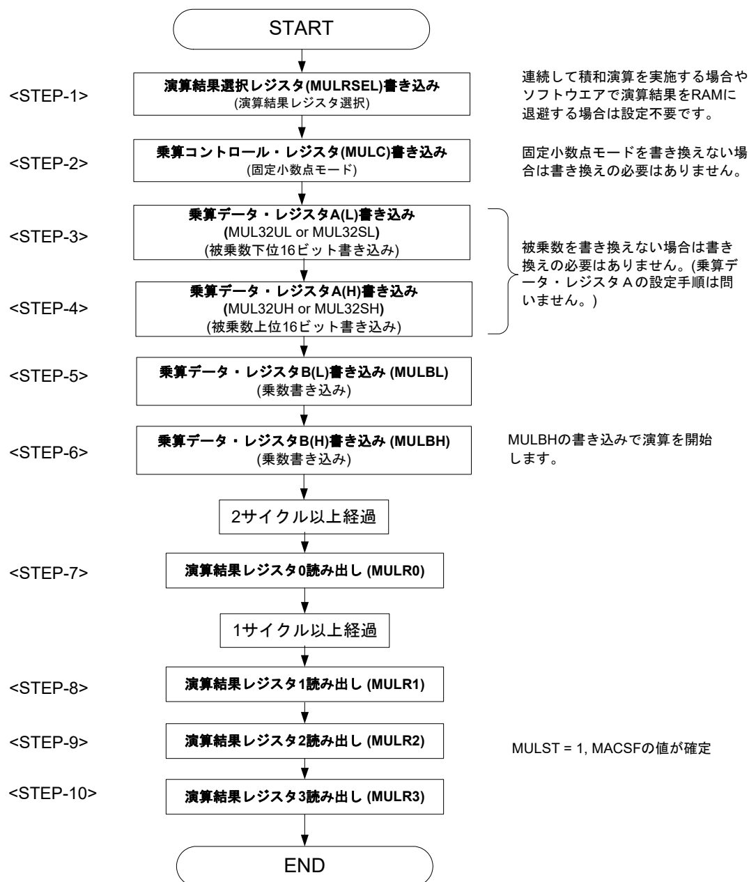
図41-9 32ビット積和演算回路の動作フロー（乗算時）
