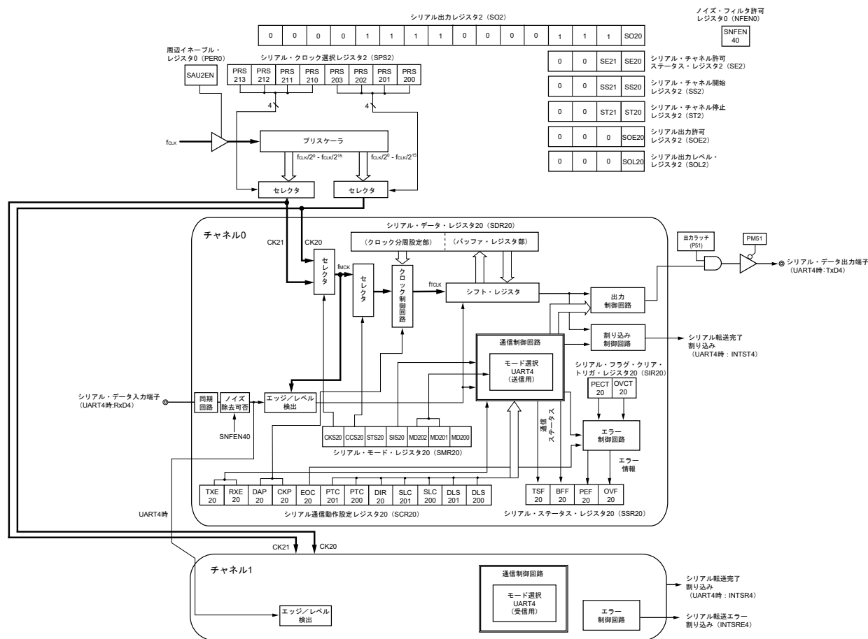
図20-3 シリアル・アレイ・ユニット2のブロック図
