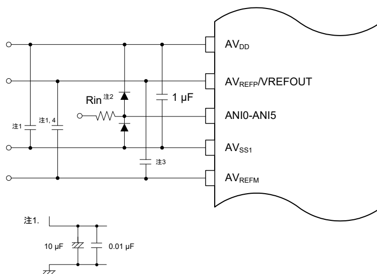
図 17-33 アナログ入力保護回路の例
