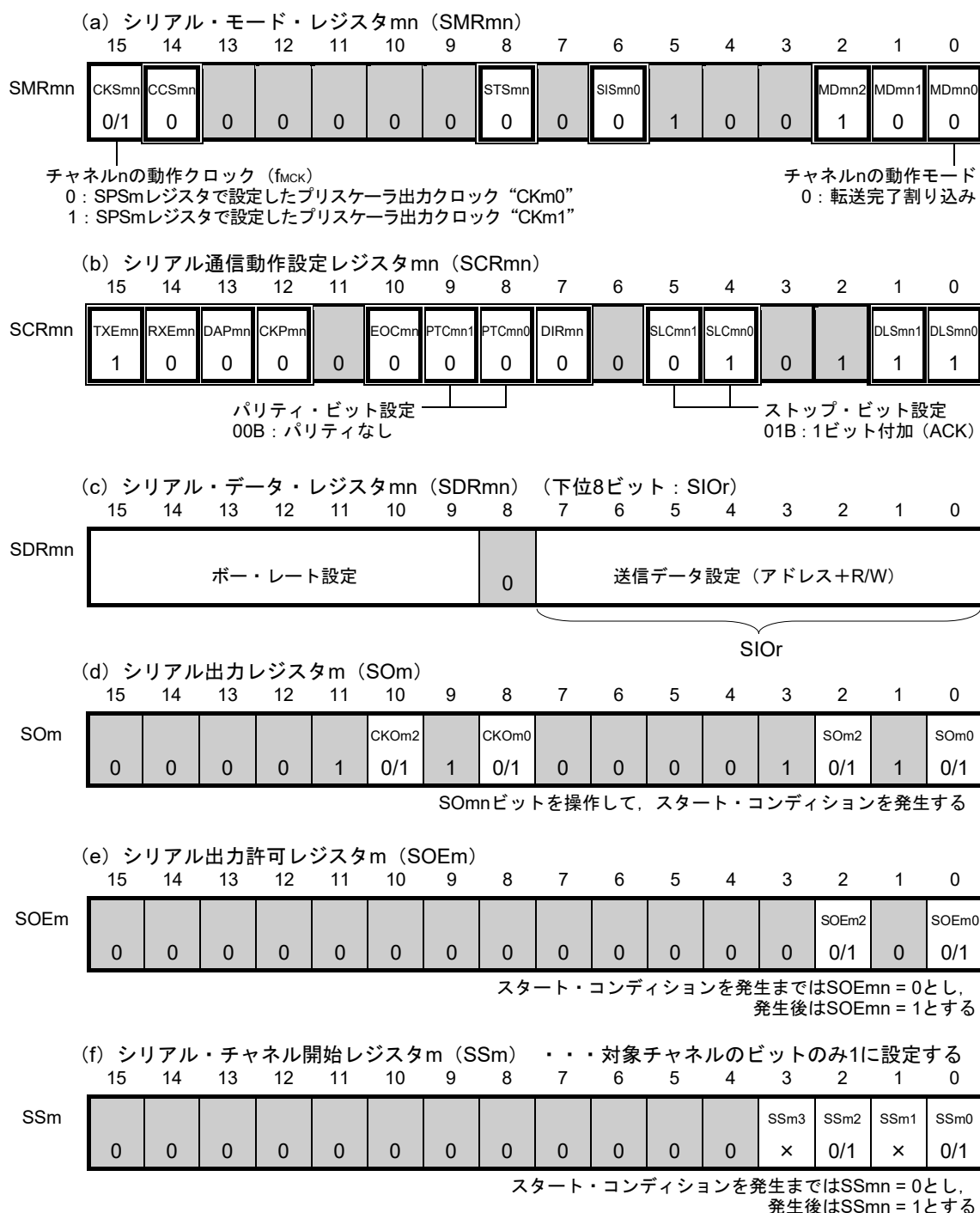
図20-105 簡易I 2 C (IIC00, IIC10, IIC30) のアドレス・フィールド送信時のレジスタ設定内容例
