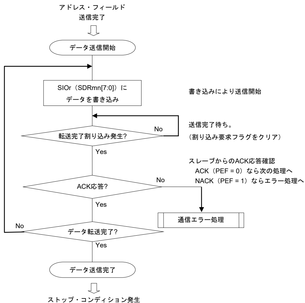
図20-111 簡易I 2 Cデータ送信のフロー・チャート
