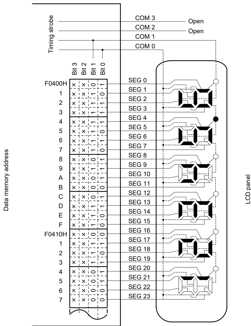
図24-29 2時分割LCDパネルの結線例
