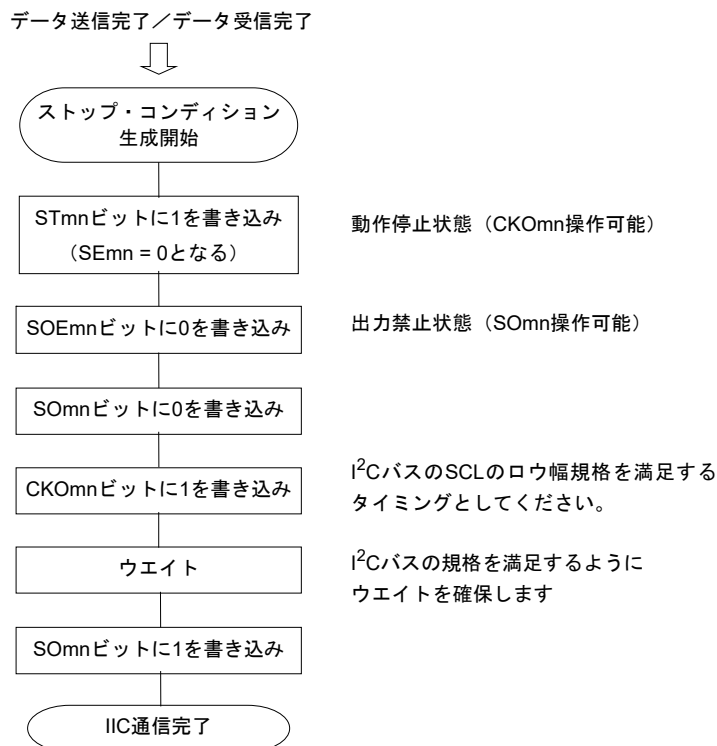
図20-116 ストップ・コンディション発生のフロー・チャート
