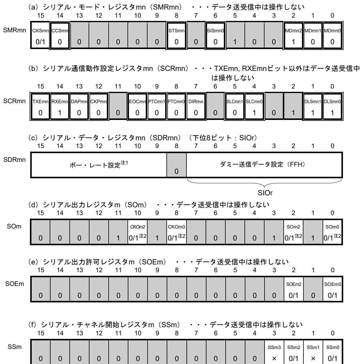
図20-112 簡易I 2 C (IIC00, IIC10, IIC30) のデータ受信時のレジスタ設定内容例
