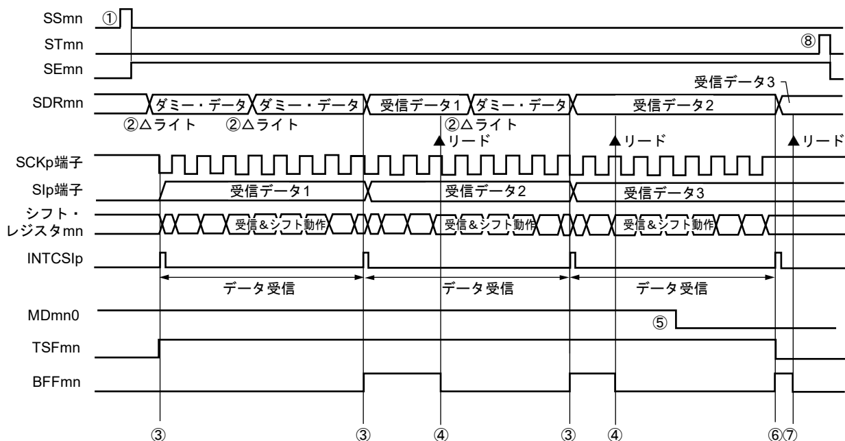
図20-41 マスタ受信（連続受信モード時）のタイミング・チャート（タイプ1：DAPmn = 0, CKPmn = 0）
