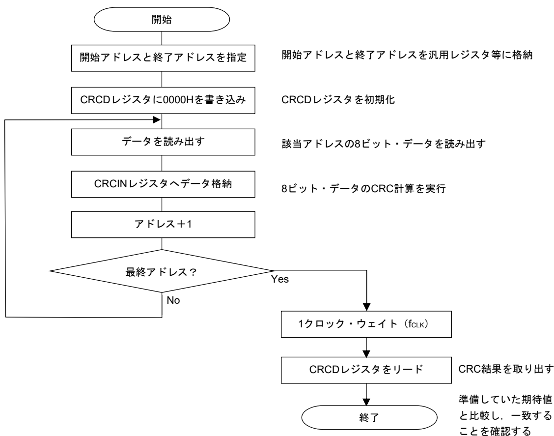
図34-6 CRC演算機能 (汎用CRC) のフロー・チャート
