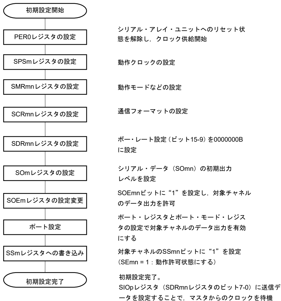
図20-66 スレーブ送受信の初期設定手順
