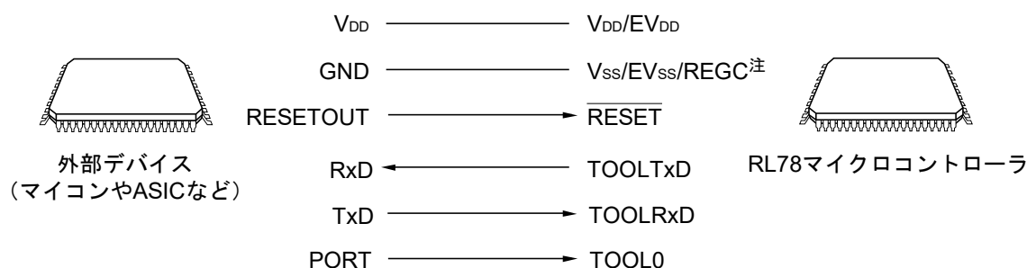
図38-4 外部デバイスとの通信
