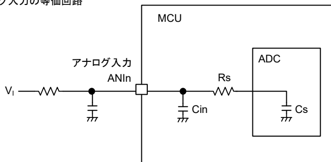
アナログ入力の等価回路
