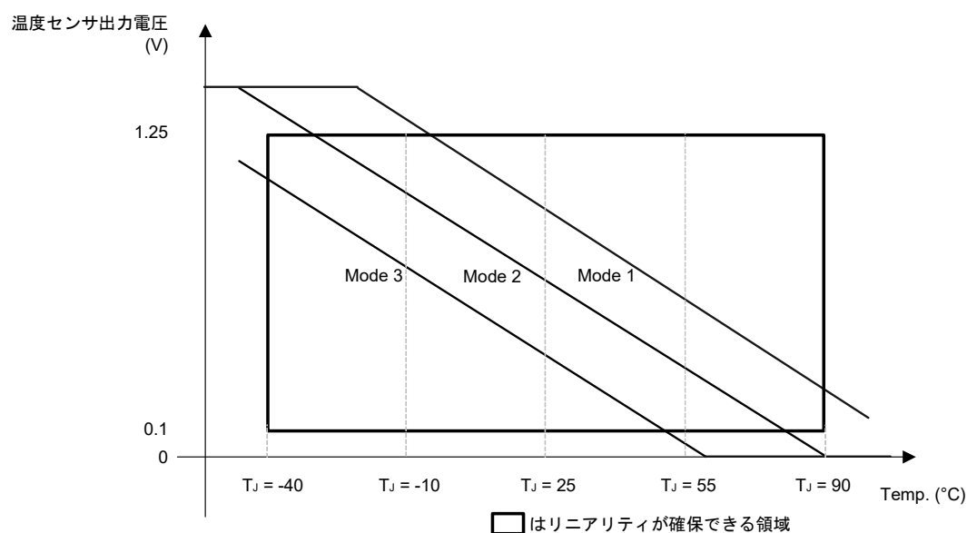
図18-2 出力イメージ図
