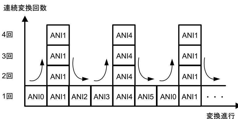
図17-9 ADADC.ADC[2:0] = 011b, ADADC.AVEE=0, ADS0[1] = 1, ADS0[4] = 1選択時のスキャン変換シーケンス
