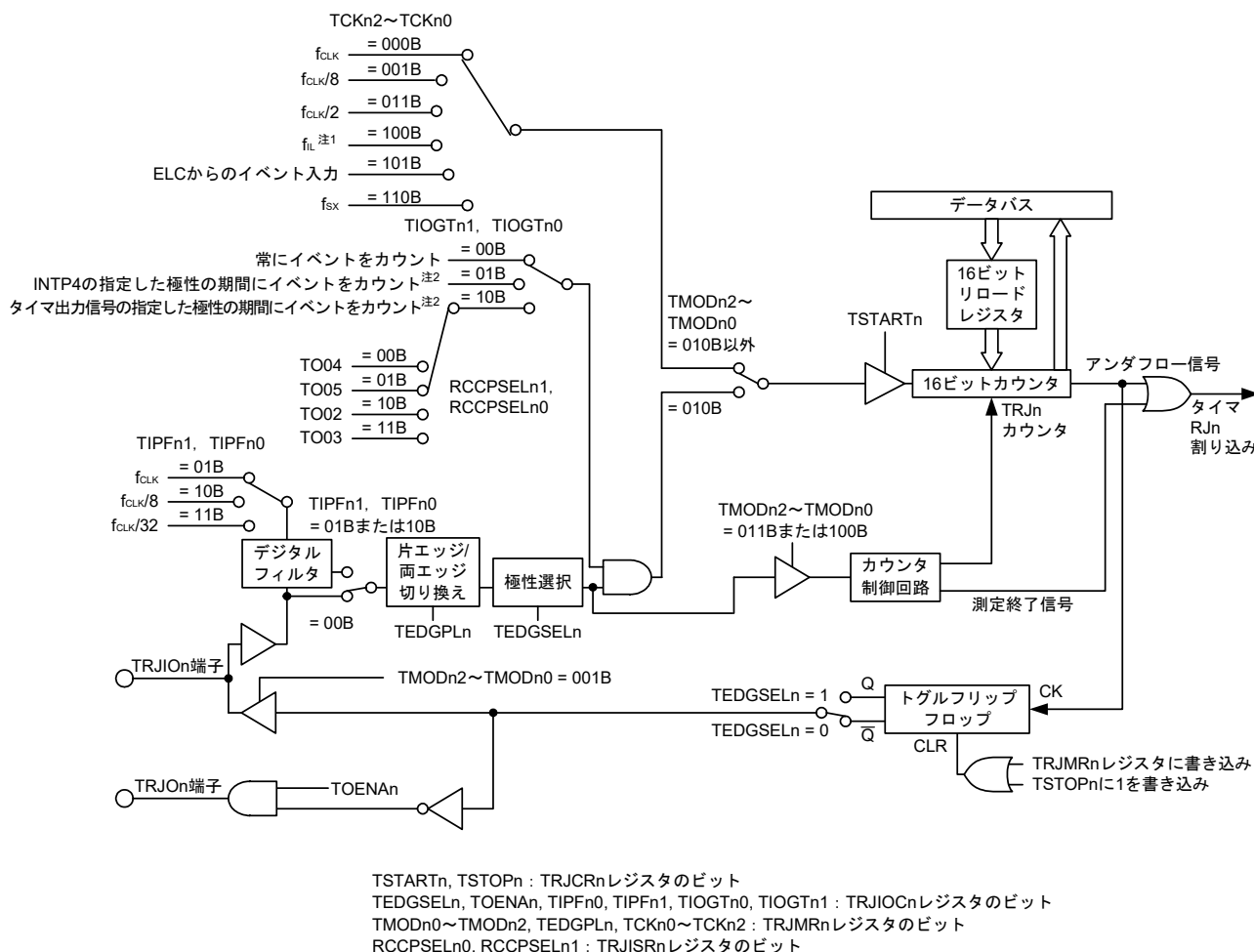
図13-1 タイマRJnのブロック図
