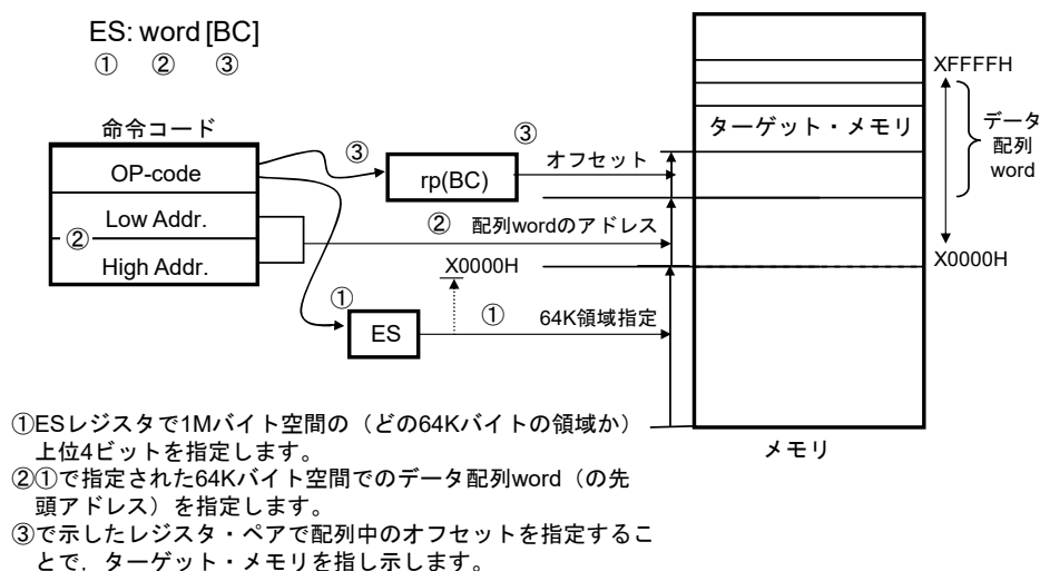
図3-30 ES:word[BC]の例
