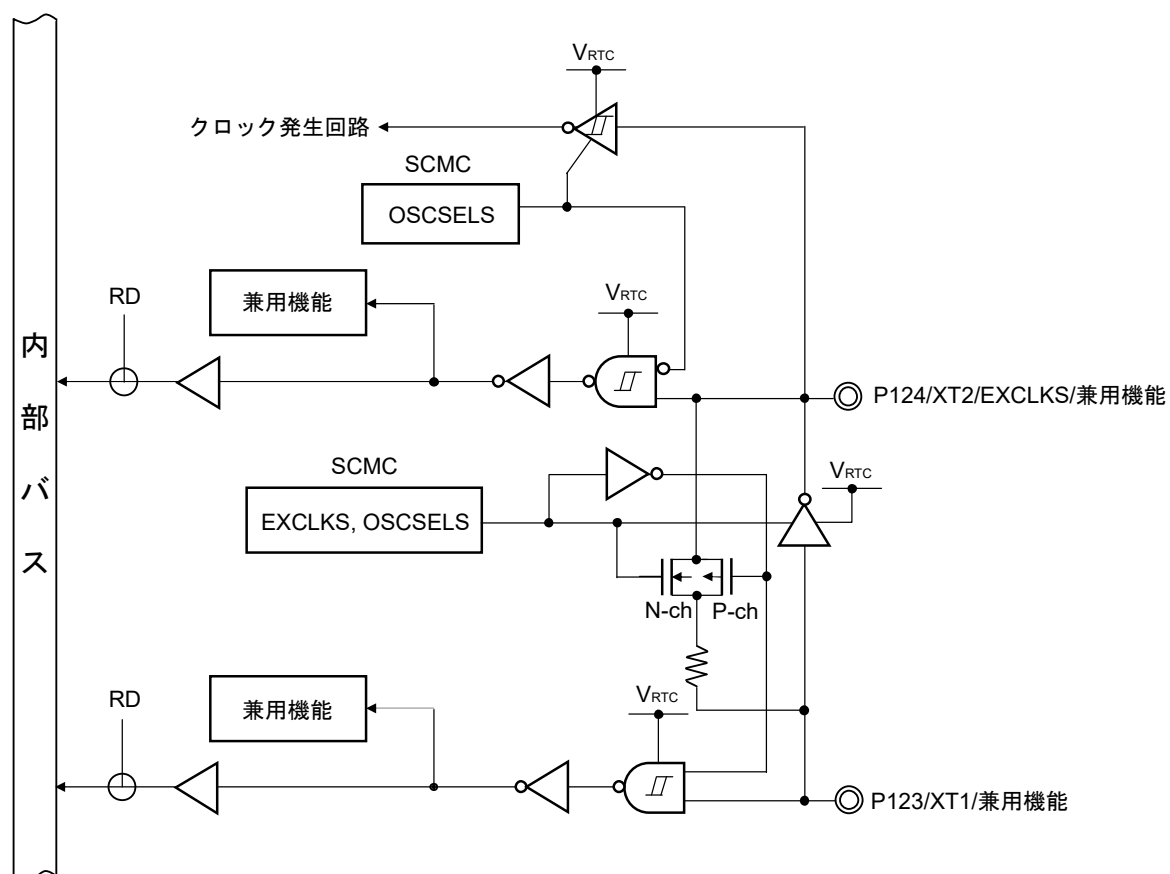
図2-5 端子タイプ2-2-2の端子ブロック図
