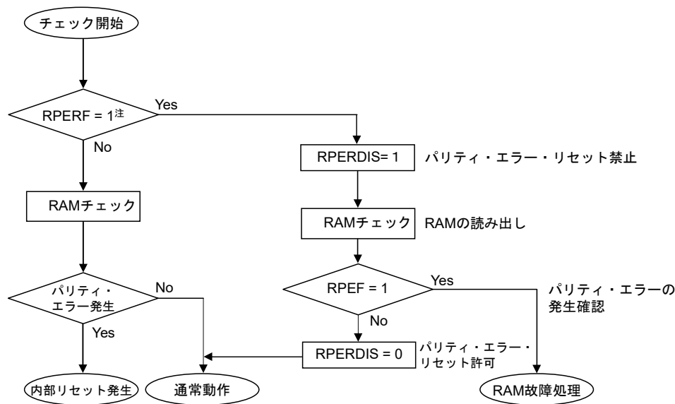
図34-8 RAMパリティ・チェックのフローチャート
