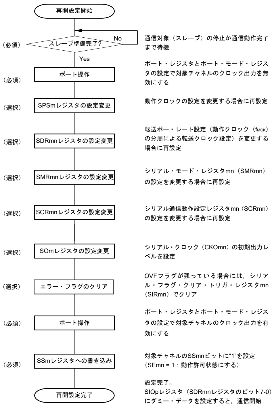
図20-38 マスタ受信の再開設定手順
