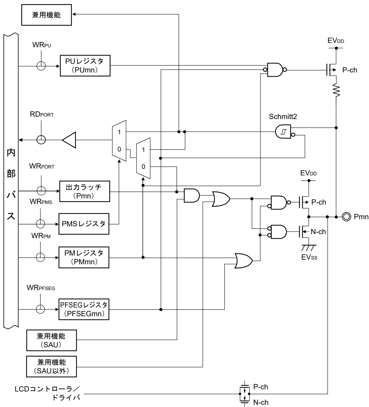
図2-9 端子タイプ7-5-4の端子ブロック図
