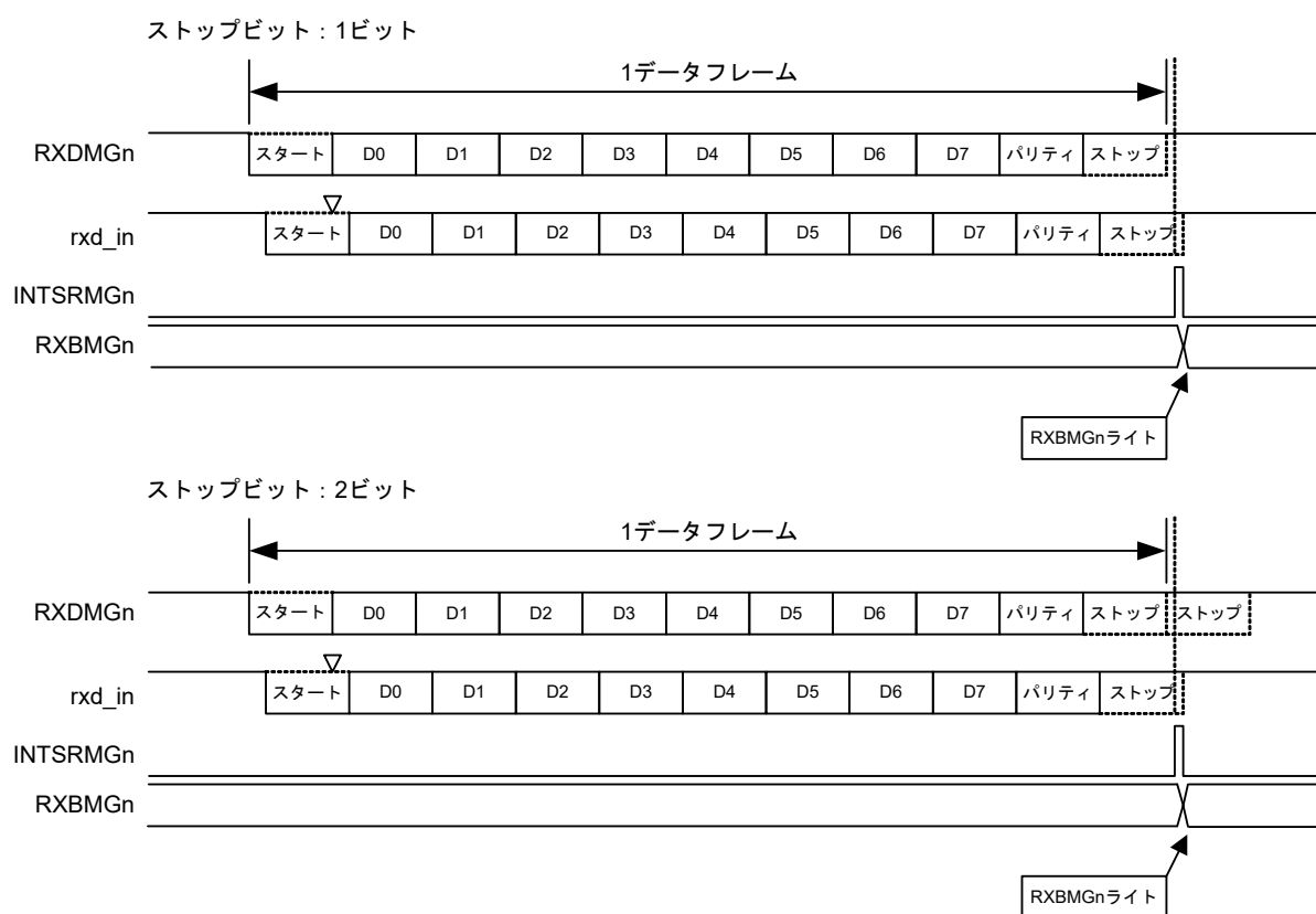
図22-20 UART受信動作タイミング
