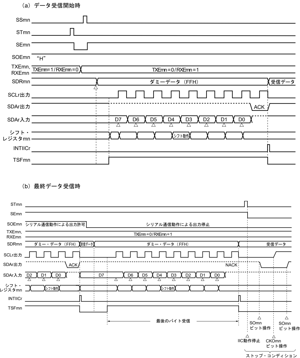
図20-113 データ受信のタイミング・チャート
