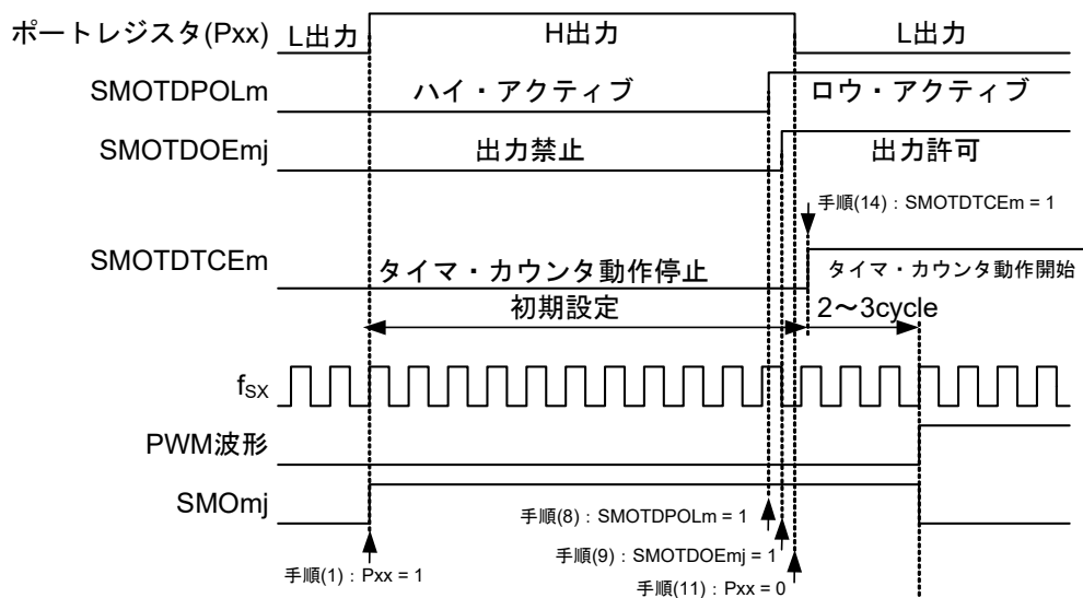
図14-22 SMO m j端子をロウ・アクティブで使用する時の動作開始(SMOTDPO Lm = 1 の場合)
