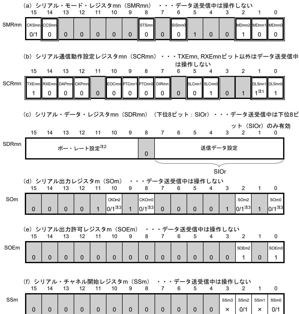
図20-109 簡易I 2 C (IIC00, IIC10, IIC30) のデータ送信時のレジスタ設定内容例
