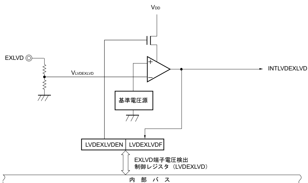
図32-5 EXLVD端子電圧検出回路のブロック図
