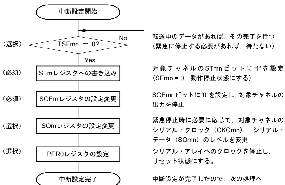
図20-29 マスタ送信の中断手順
