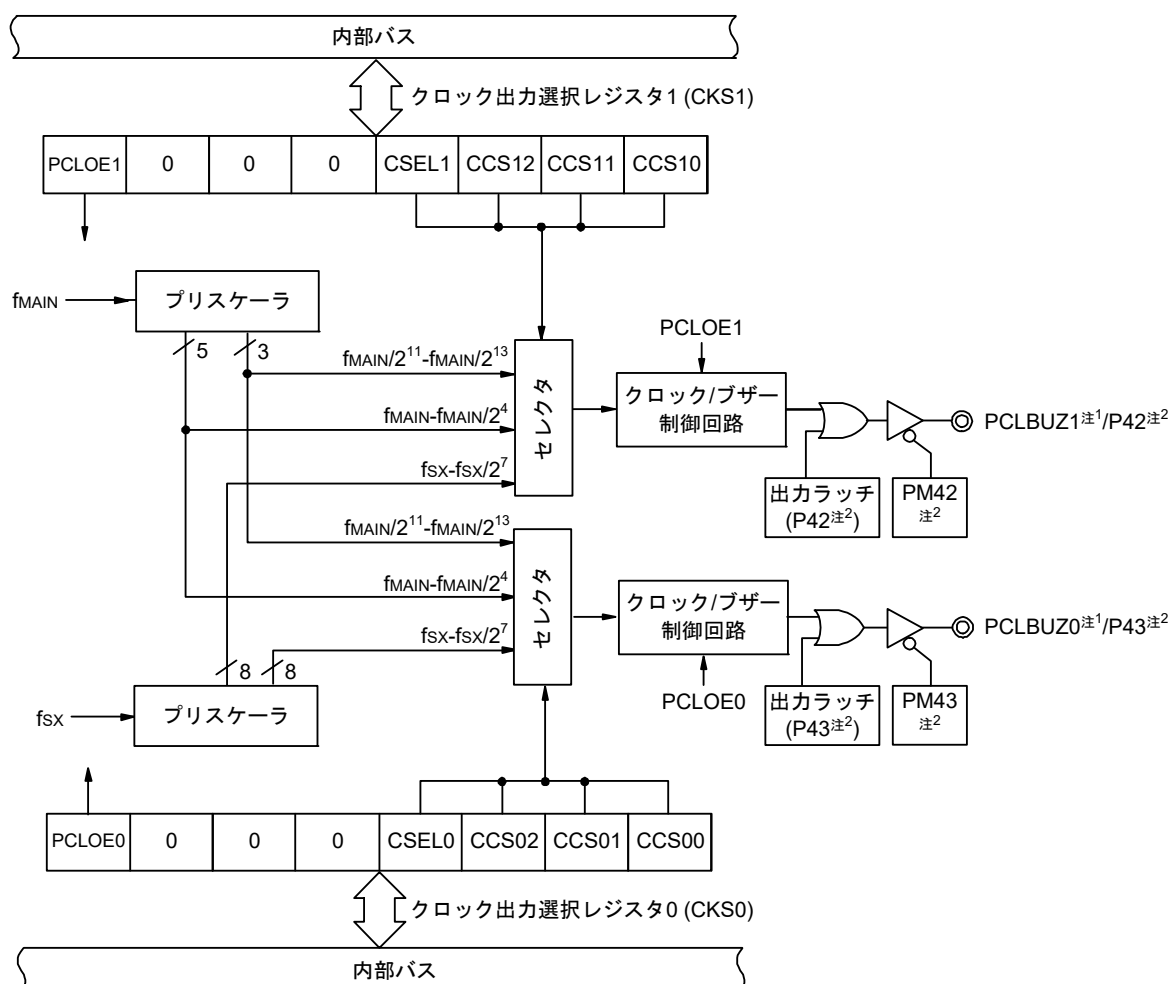
図15-1 クロック出力／ブザー出力制御回路のブロック図
