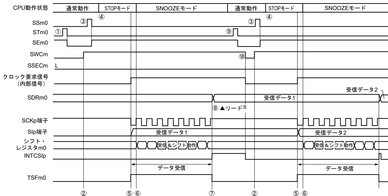
図20-75 SNOOZEモード動作 (連続起動) 時のタイミング・チャート (タイプ1: DAPm0 = 0, CKPm0 = 0)
