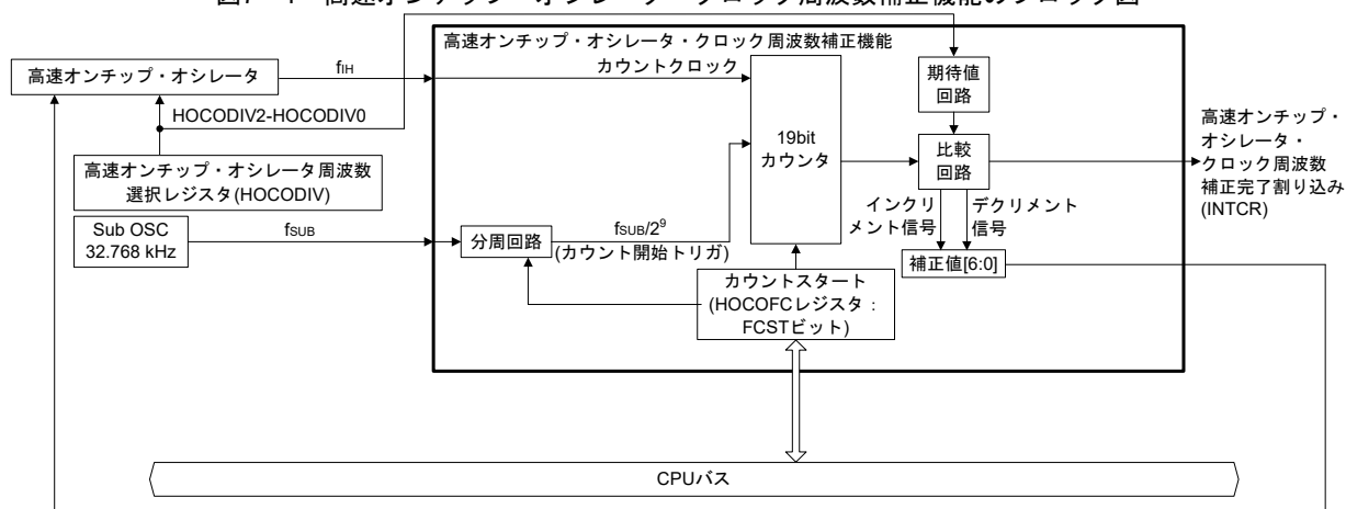
図7-1 高速オンチップ・オシレータ・クロック周波数補正機能のブロック図
