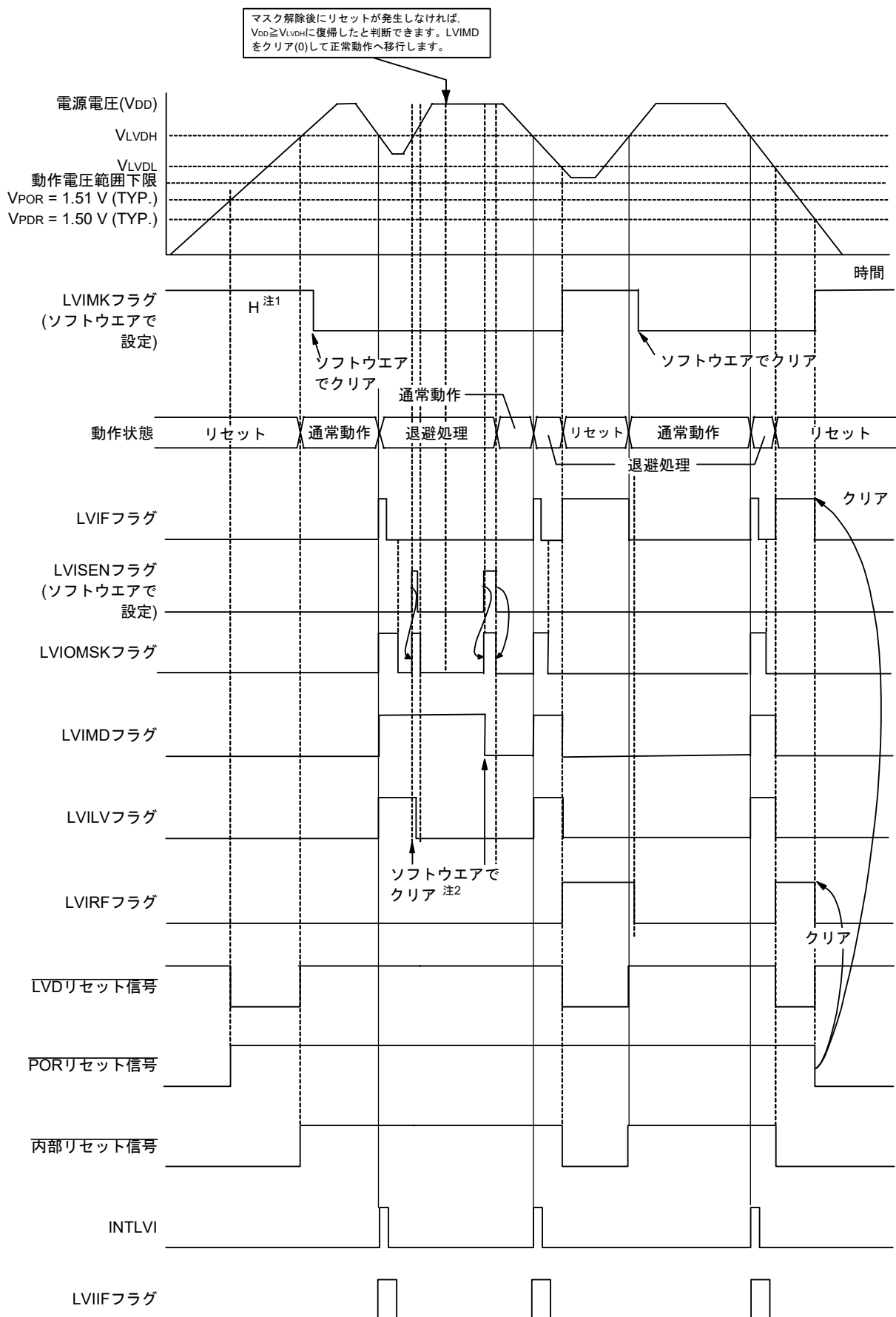
図32-19 割り込み&amp;リセット信号発生タイミング (オプション・バイトLVIMDS1, LVIMDS0 = 1, 0) (1/2)
