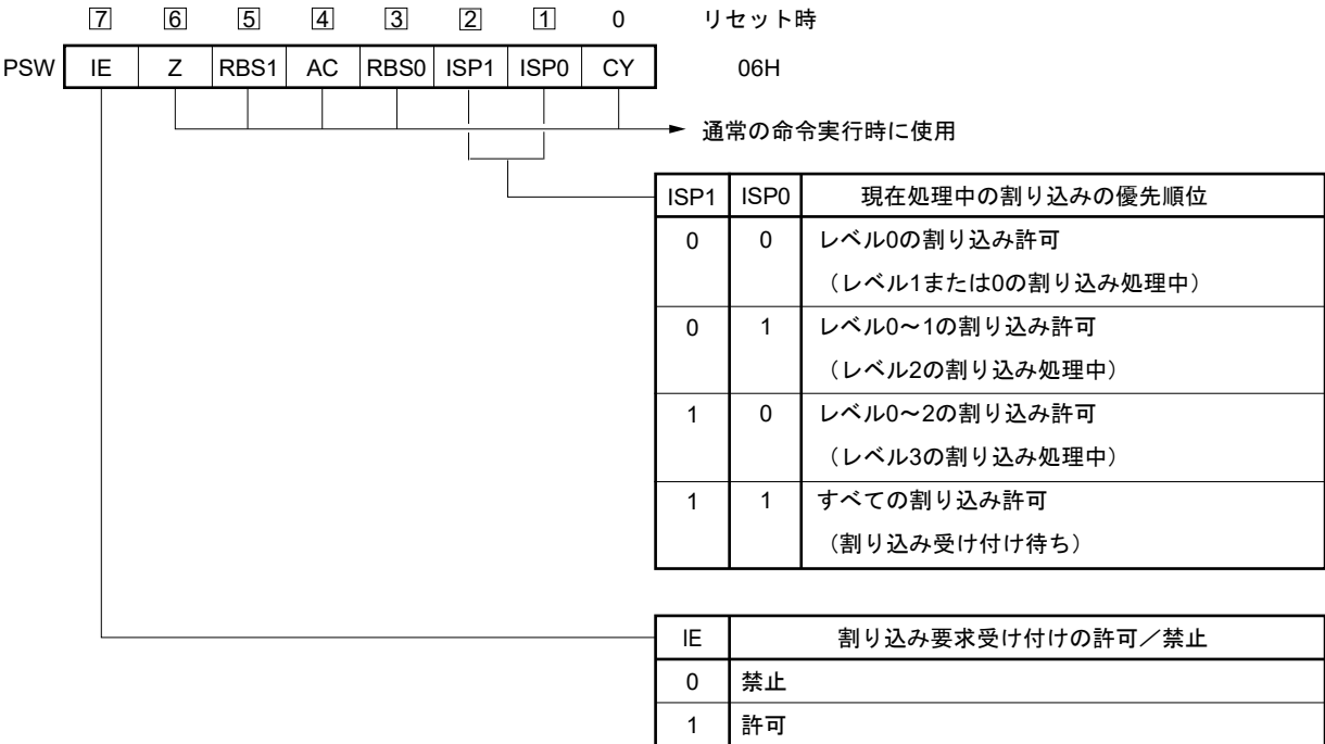
図27-6 プログラム・ステータス・ワードの構成
