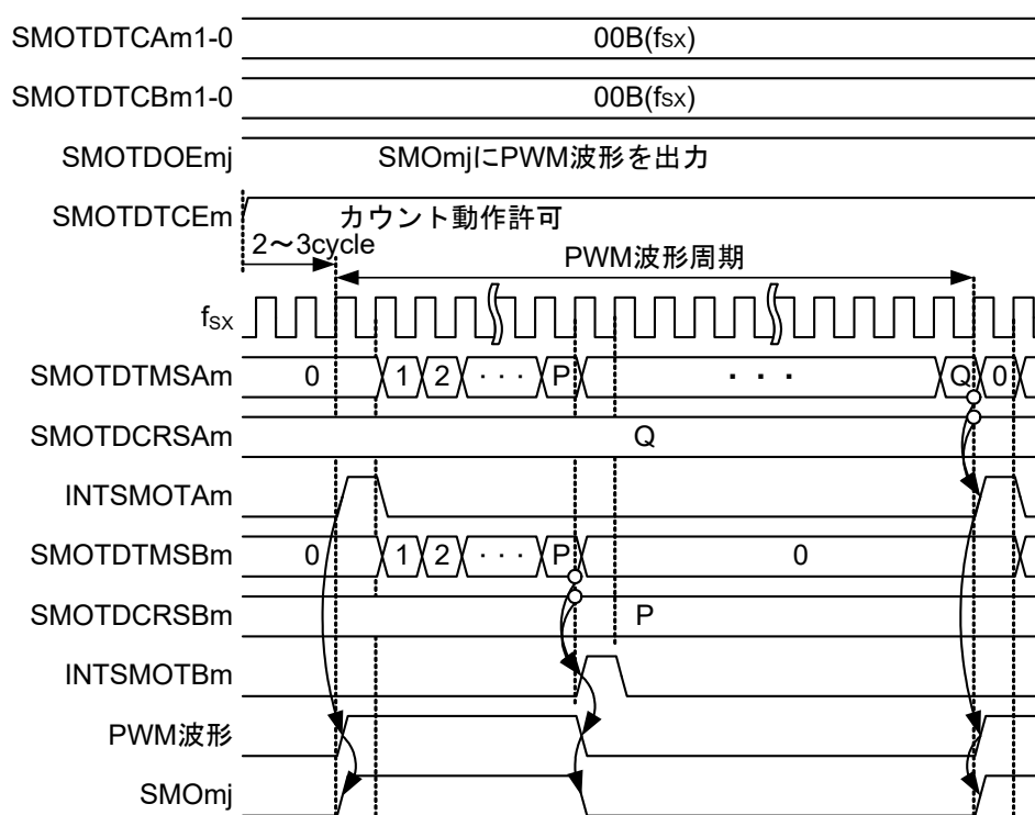
図14-17 サンプルング・クロック出力(分周なし)
