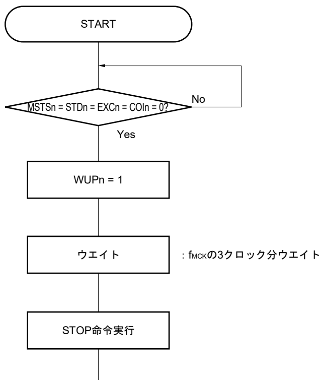
図21-23 WUPn = 1を設定する場合のフロー
