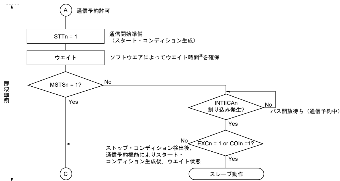
図21-30 マルチマスタ・システムでのマスタ動作 (2/3)
