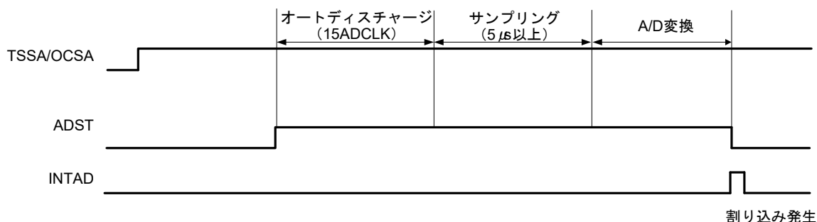
図17-23 シングルスキャンモードの動作例 (温度センサ出力, 内部基準電圧 ( V_{BGR} ) 選択)
