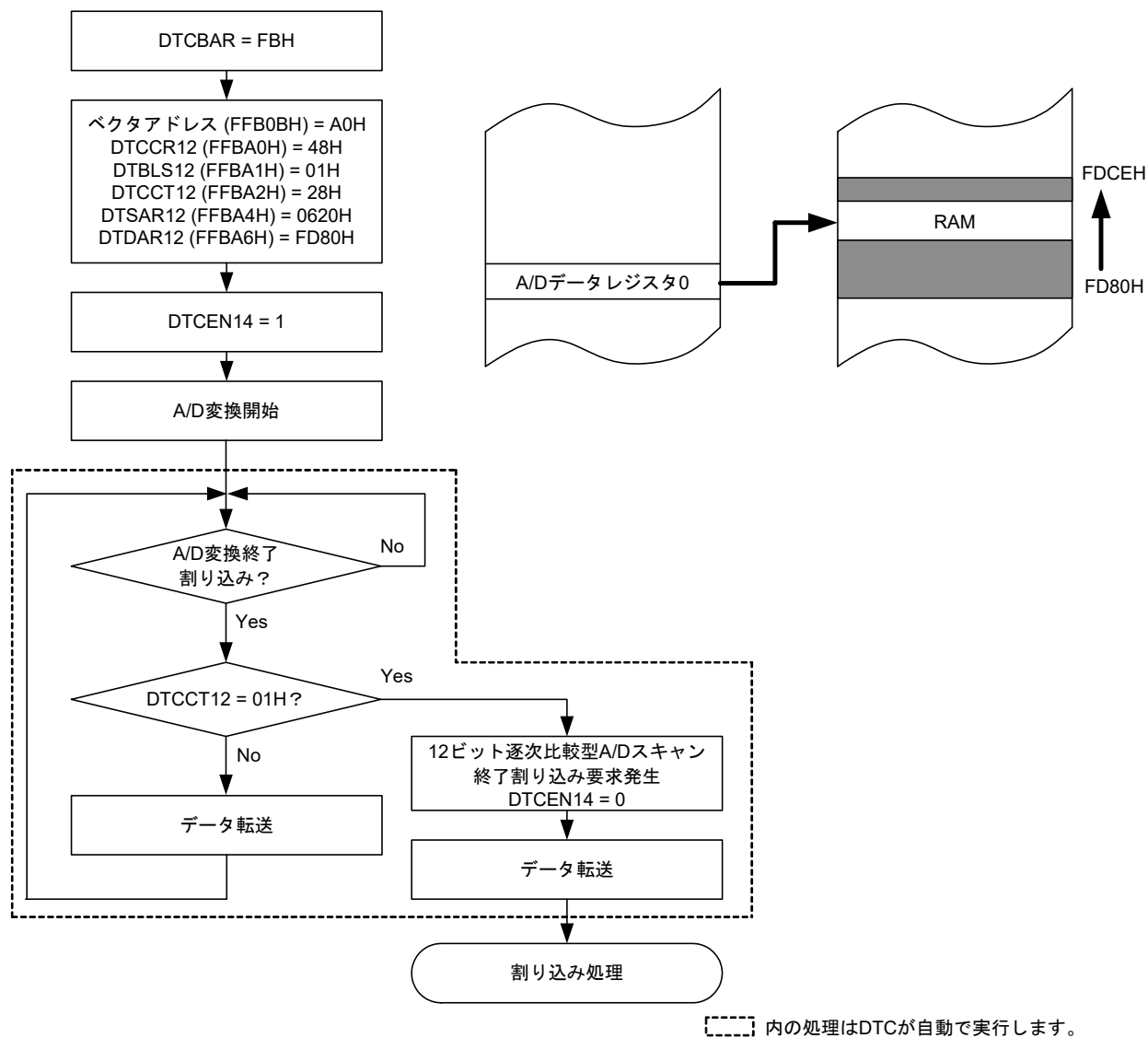
図25-16 ノーマルモードの使用例1：12ビットA/D変換結果の連続取り込み
