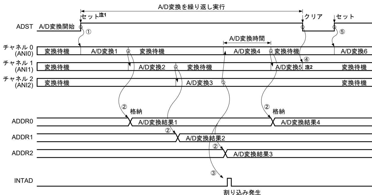
図17-24 連続スキャンモードの動作例（基本動作：ANI0, ANI1, ANI2選択）
