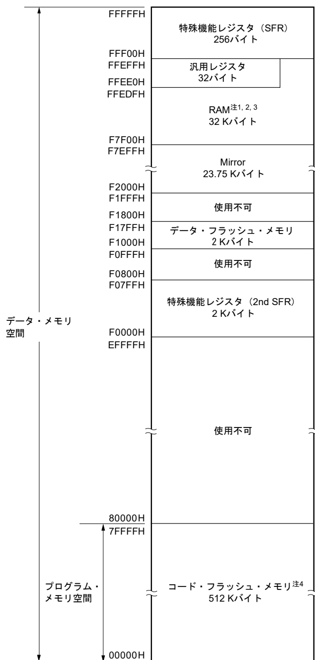
図3-1 メモリ・マップ (R5F10NPL, R5F10NML)
