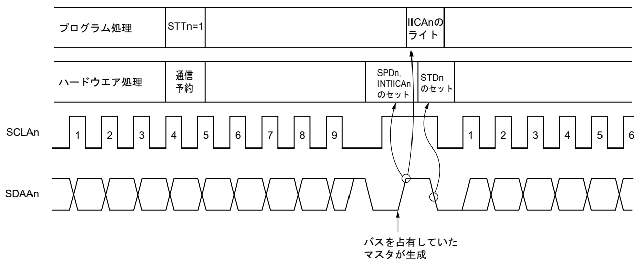
図21-26 通信予約のタイミング
