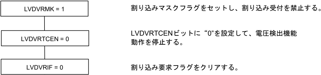
図32-14 VRTC端子電圧検出機能禁止時の設定手順
