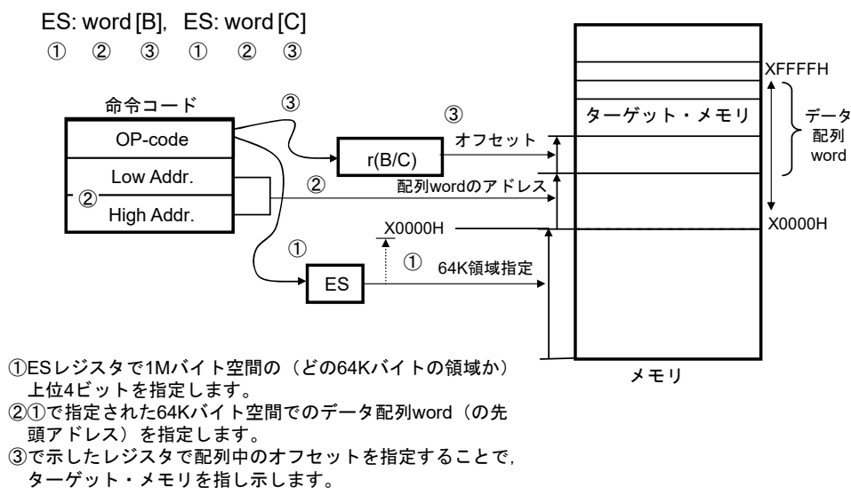
図3-30 ES:word[BC]の例
