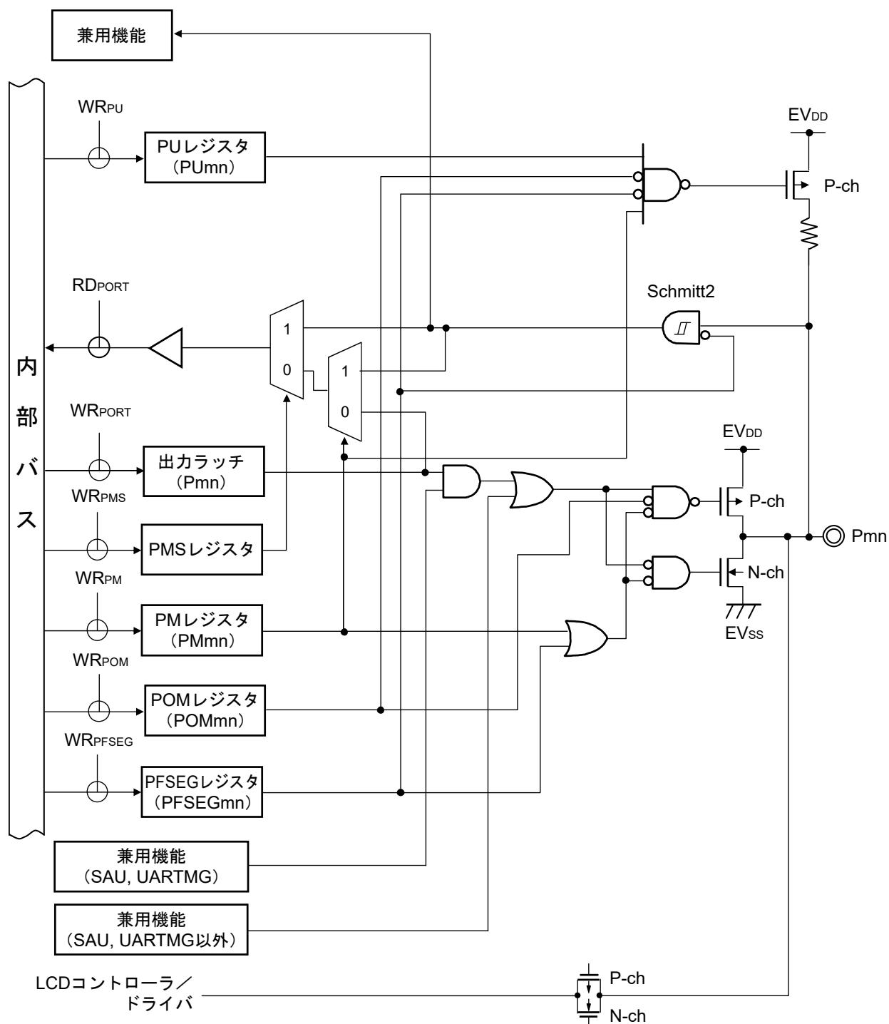
図2-12 端子タイプ7-5-10の端子ブロック図
