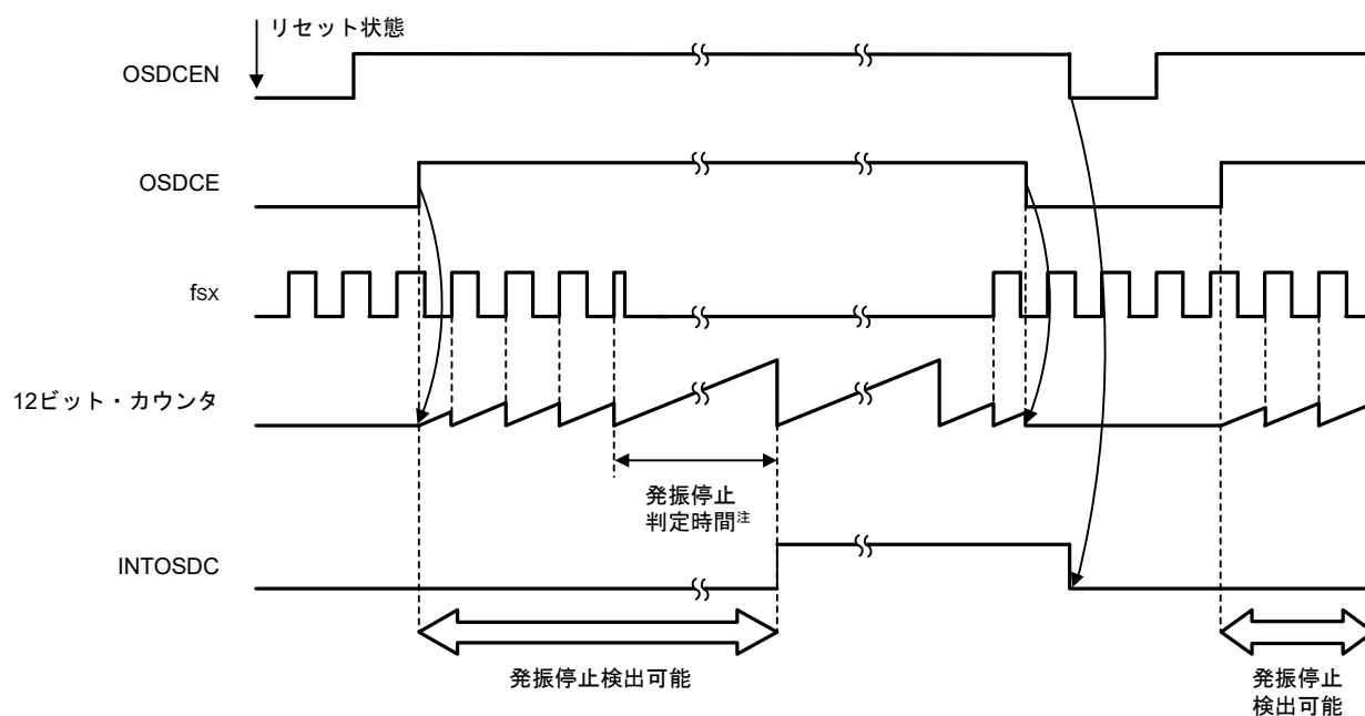
図33-6 発振停止検出回路のタイミング
