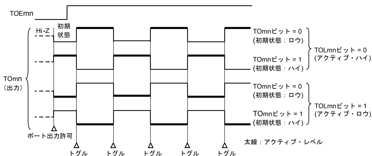
図8-36 トグル出力時 (TOMmn = 0) のT0mn端子出力状態
