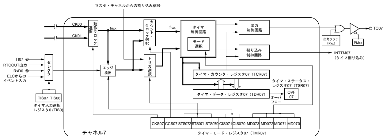
図8-8 タイマ・アレイ・ユニットのチャンネル7内部ブロック図
