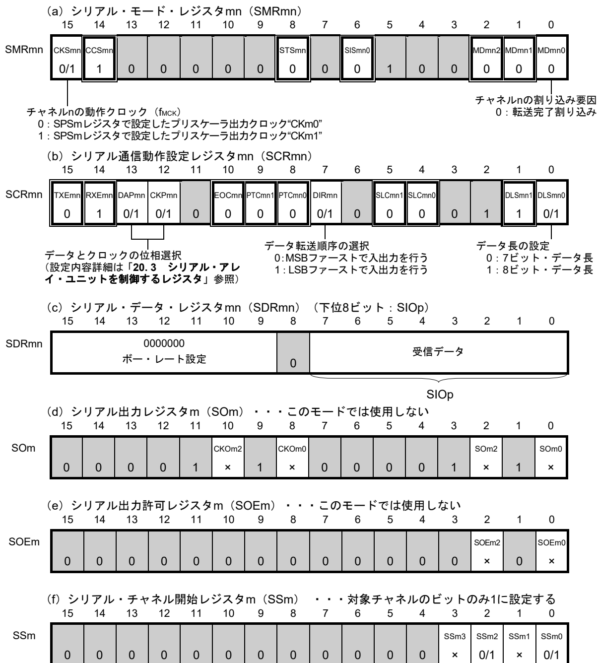
図20-59 簡易SPI (CSI00, CSI10, CSI30) のスレーブ受信時のレジスタ設定内容例
