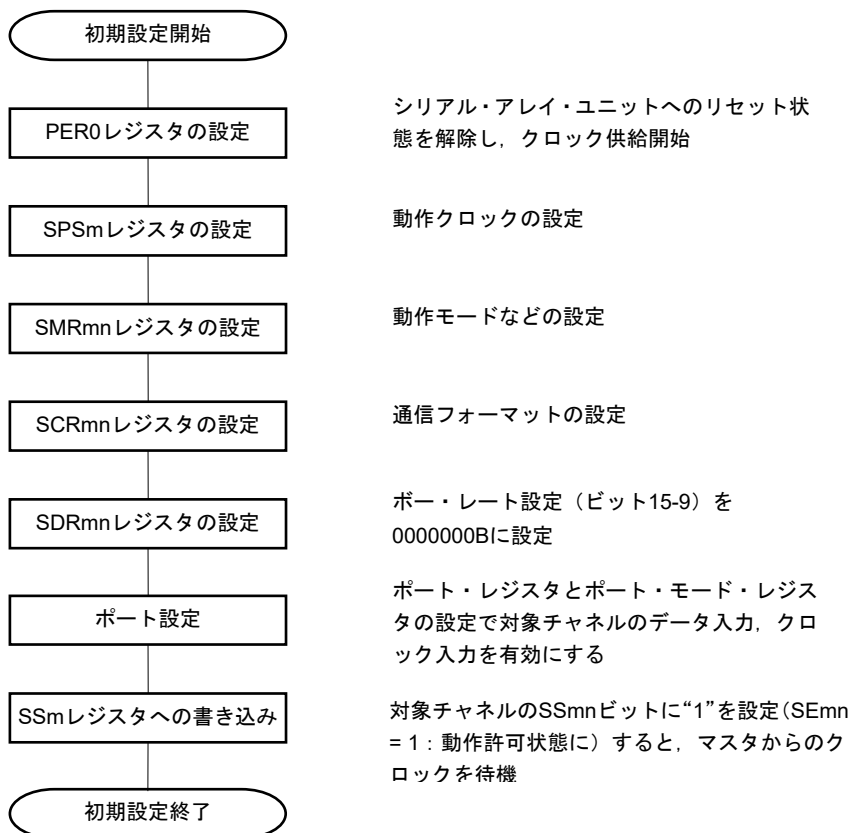
図20-60 スレーブ受信の初期設定手順
