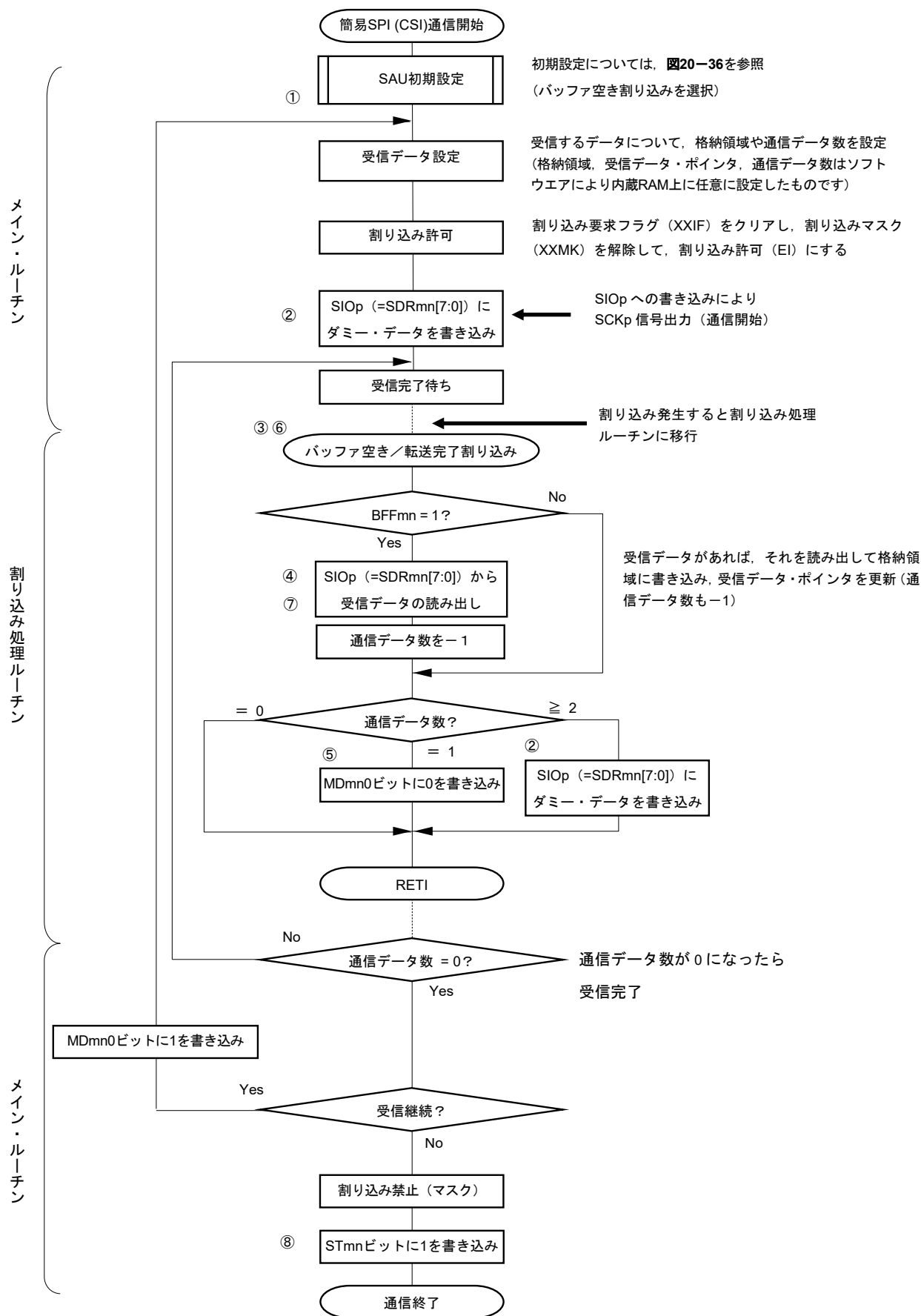
図20-42 マスタ受信（連続受信モード時）のフロー・チャート
