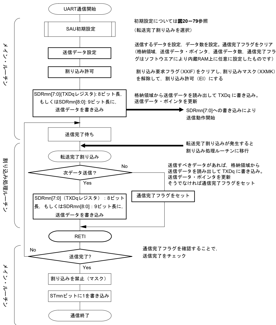
図20-83 UART送信（シングル送信モード時）のフロー・チャート
