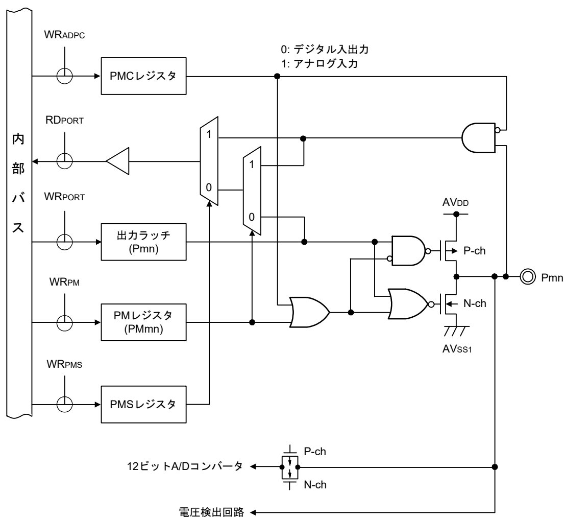
図2-7 端子タイプ4-15-3の端子ブロック図
