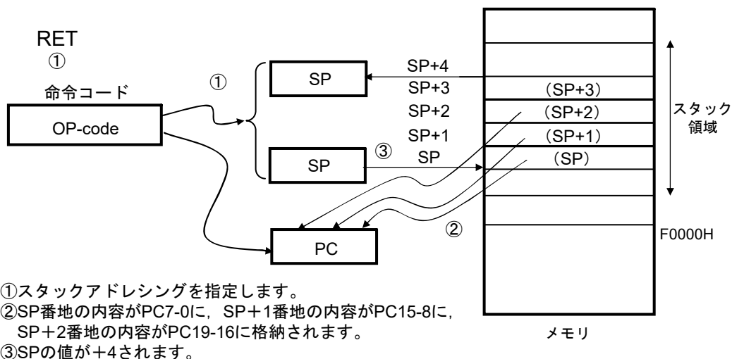
図3-36 RETの例
