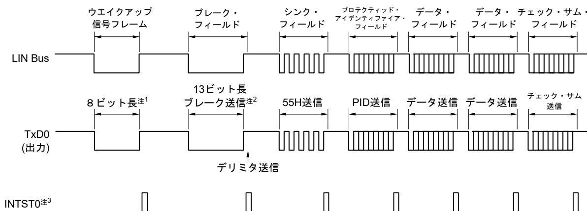
図20-100 LINの送信操作
