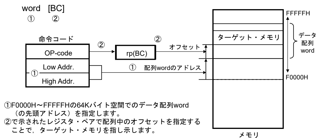
図3-27 word[BC]の例
