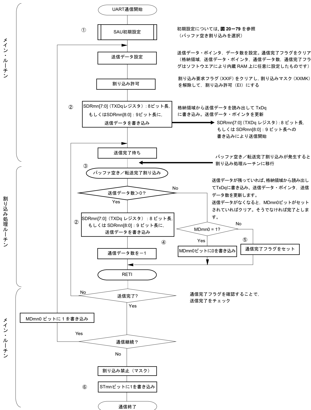
図20-85 UART送信（連続送信モード時）のフロー・チャート
