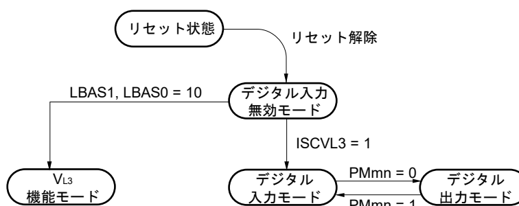
図4-12 VL 3 /P125端子機能の状態遷移図
