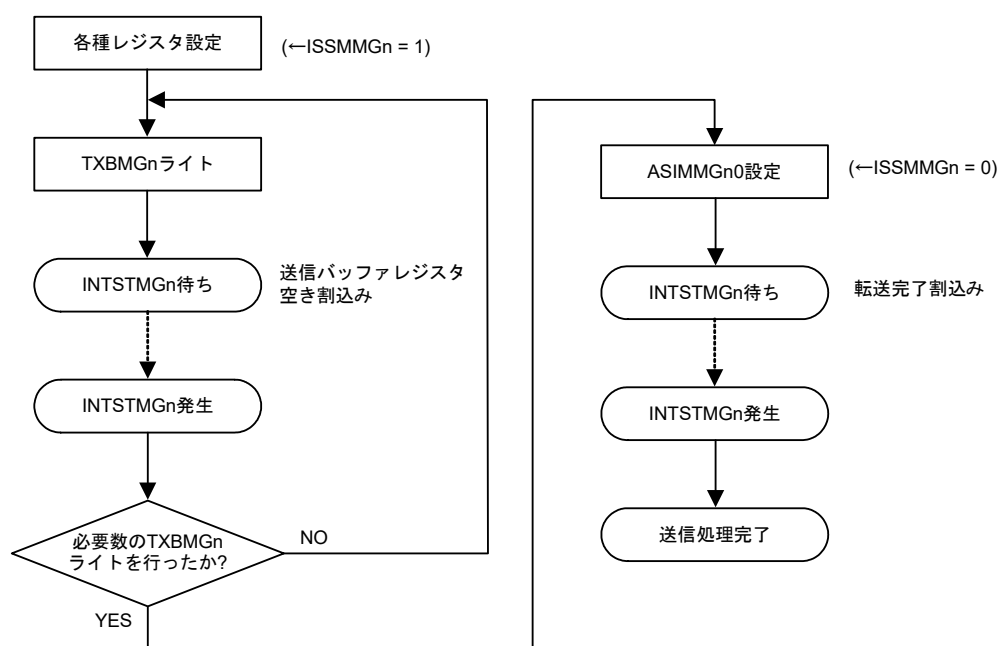
図22-17 割り込みによる連続送信処理フロー例
