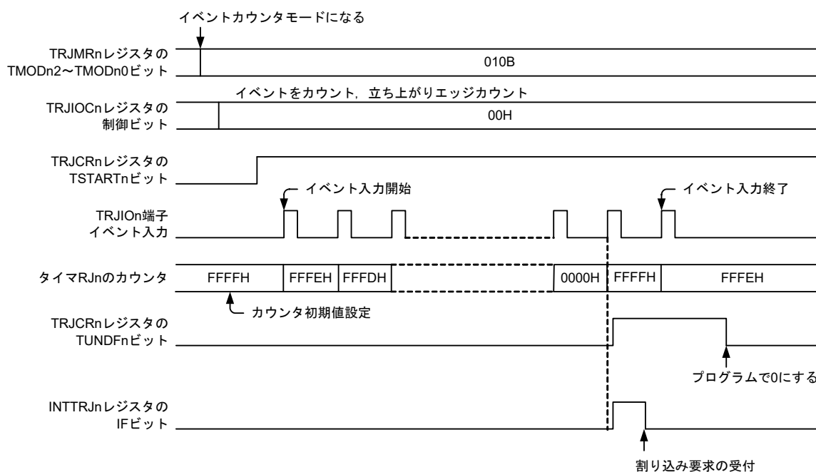
図13-14 イベントカウンタモードの動作例1
