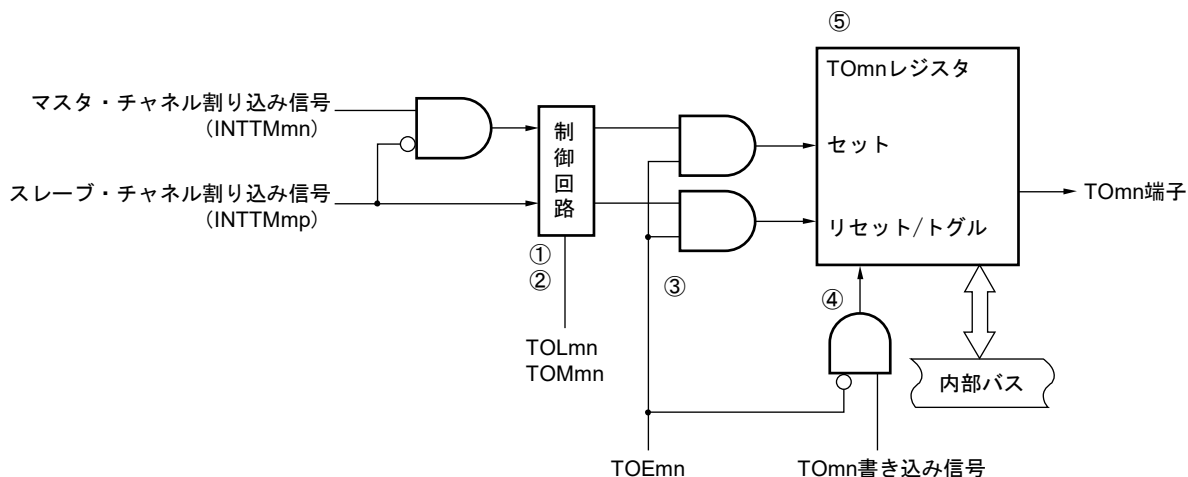
図8-34 出力回路構成図
