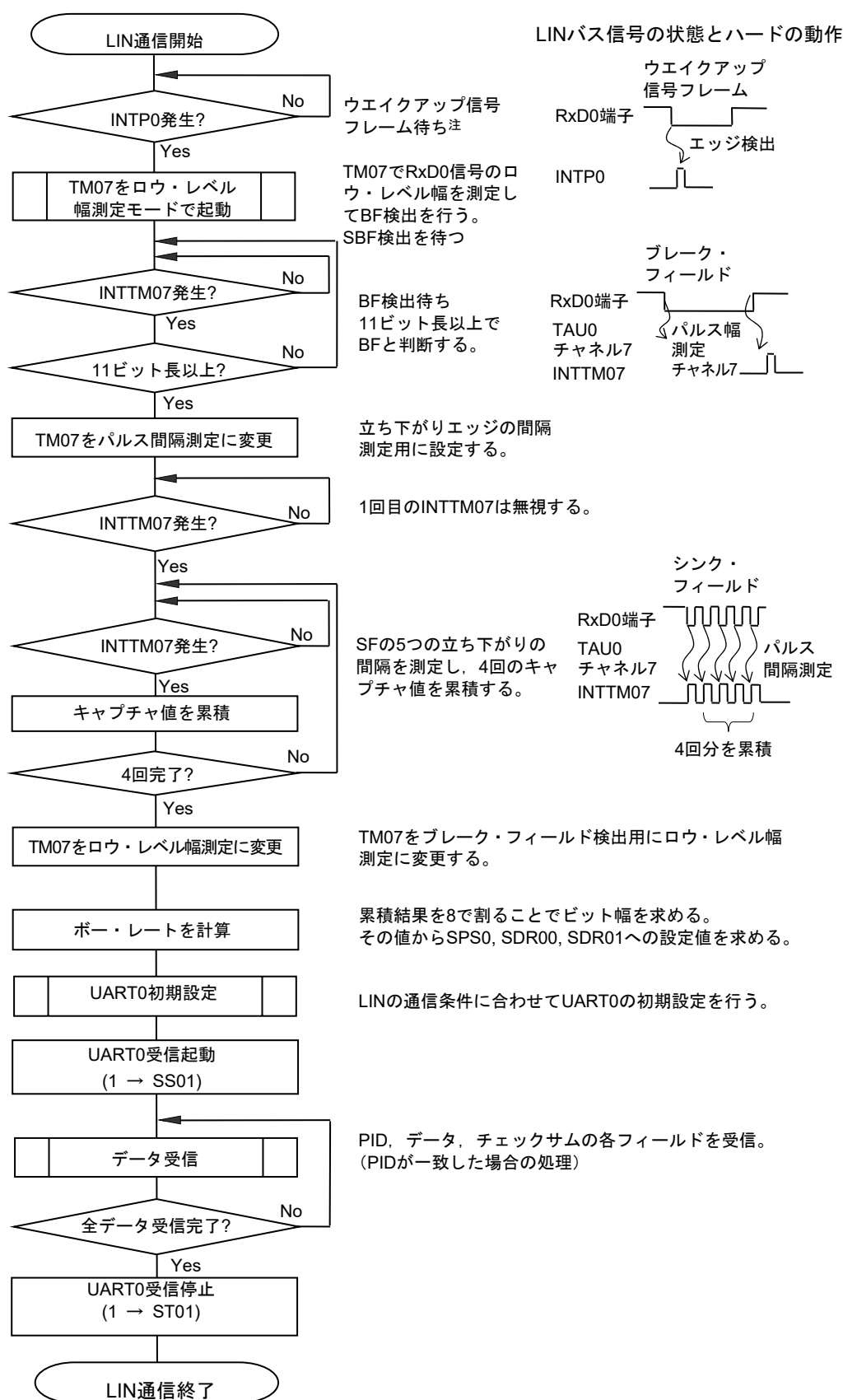
図20-103 LIN受信のフロー・チャート
