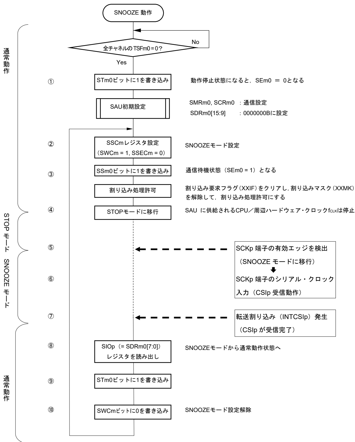
図20-76 SNOOZEモード動作（連続起動）時のフロー・チャート
