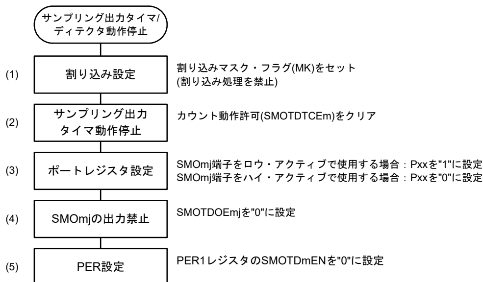
図14-23 動作停止手順
