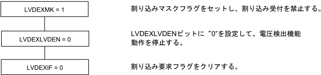
図32-16 EXLVD端子電圧検出機能禁止時の設定手順
