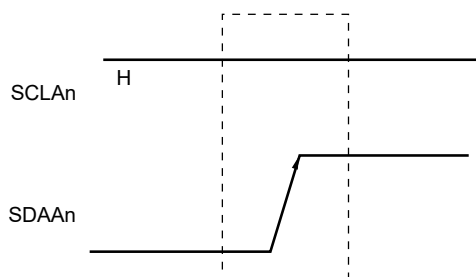
図21-20 ストップ・コンディション
