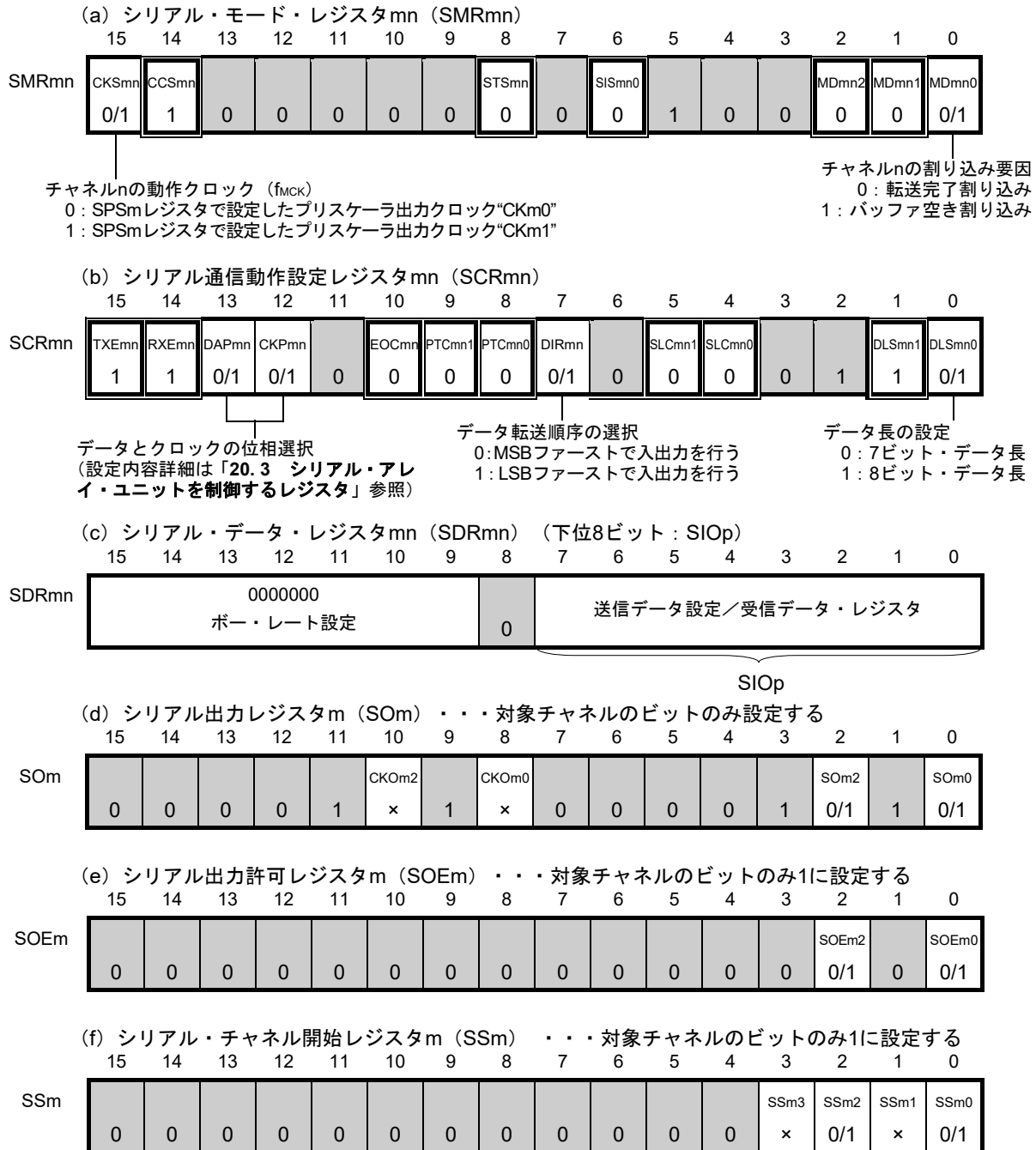
図20-65 簡易SPI (CSI00, CSI10, CSI30) のスレーブ送受信時のレジスタ設定内容例
