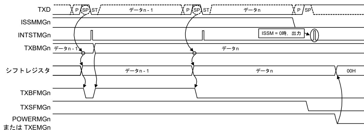
図22-19 連続送信終了タイミング
