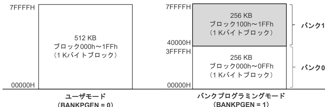
図38-9 バンクモード切り替え機能
