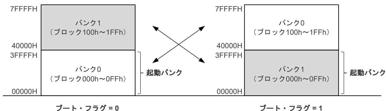
図38-12 バンクスワップ機能 (ユーザモード/バンクプログラミングモード)
