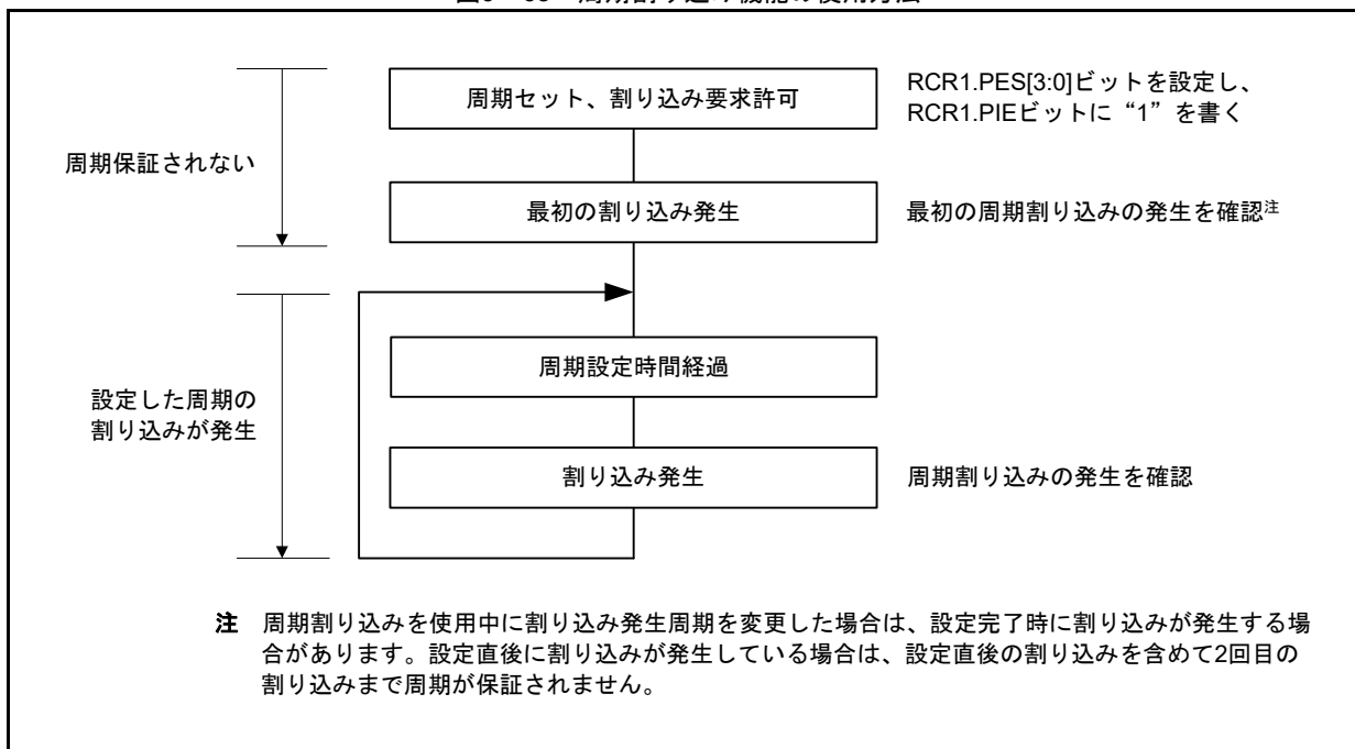
図9-65 周期割り込み機能の使用方法
