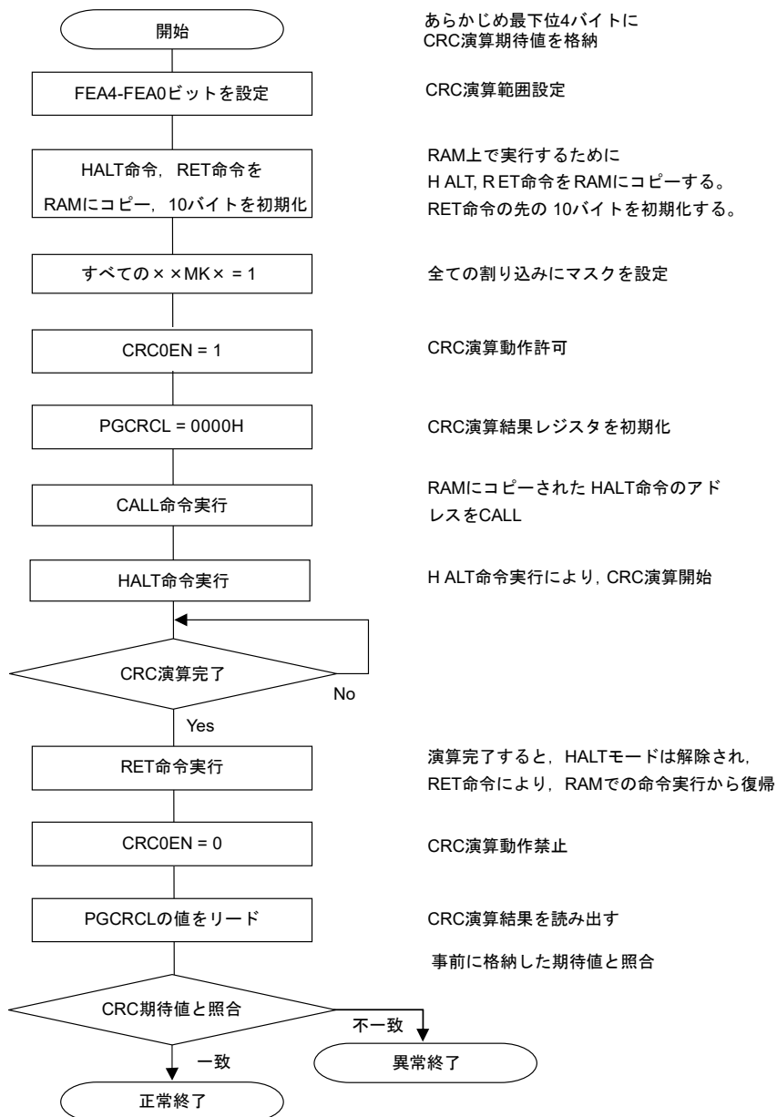
図34-3 フラッシュ・メモリCRC演算機能（高速CRC）のフロー・チャート
