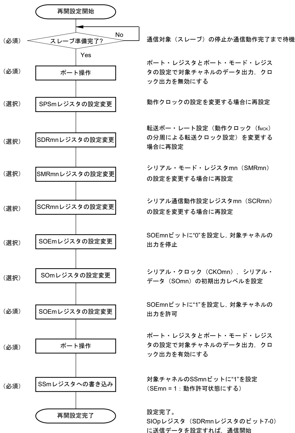
図20-30 マスタ送信の再開設定手順
