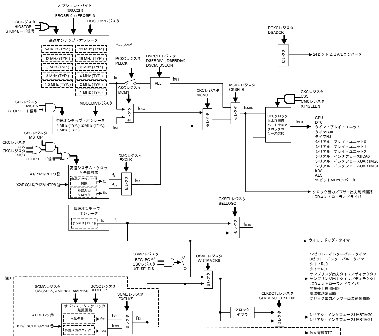
図6-1 クロック発生回路のブロック図
