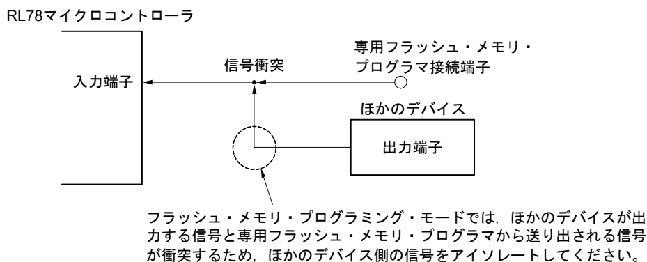
図38-5 信号の衝突 (RESET端子)
