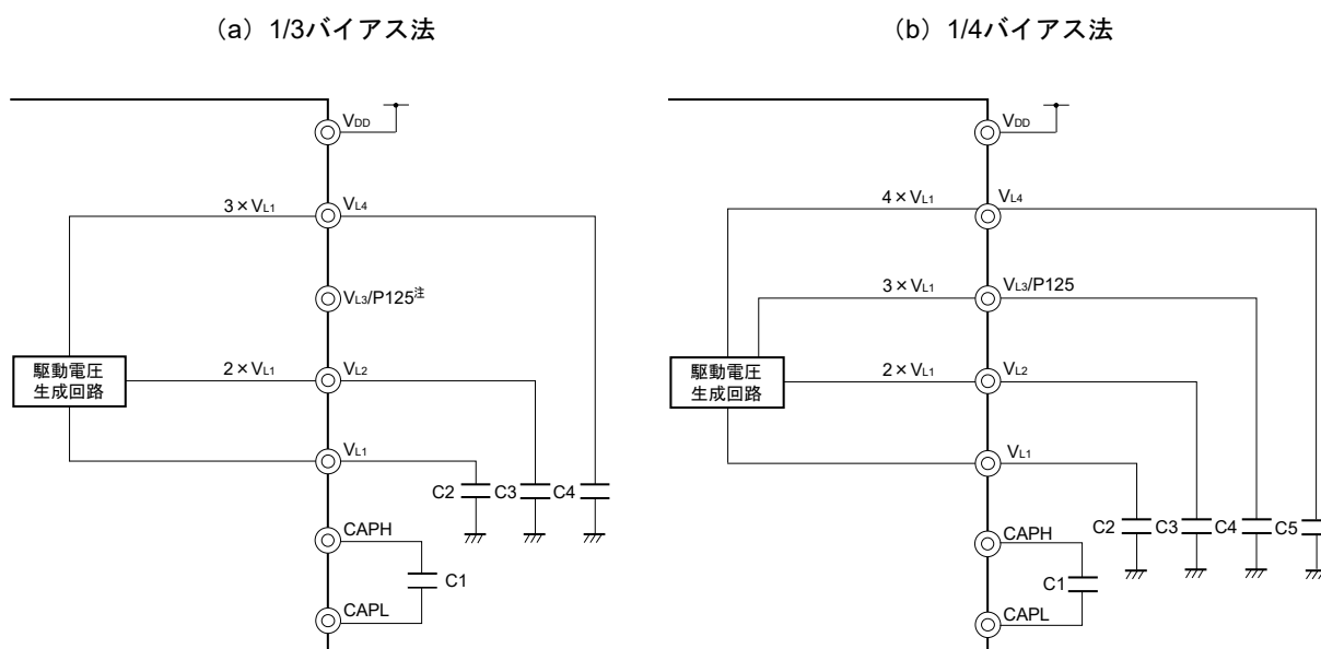
図24-21 LCD駆動用電源の接続例 (内部昇圧方式)
