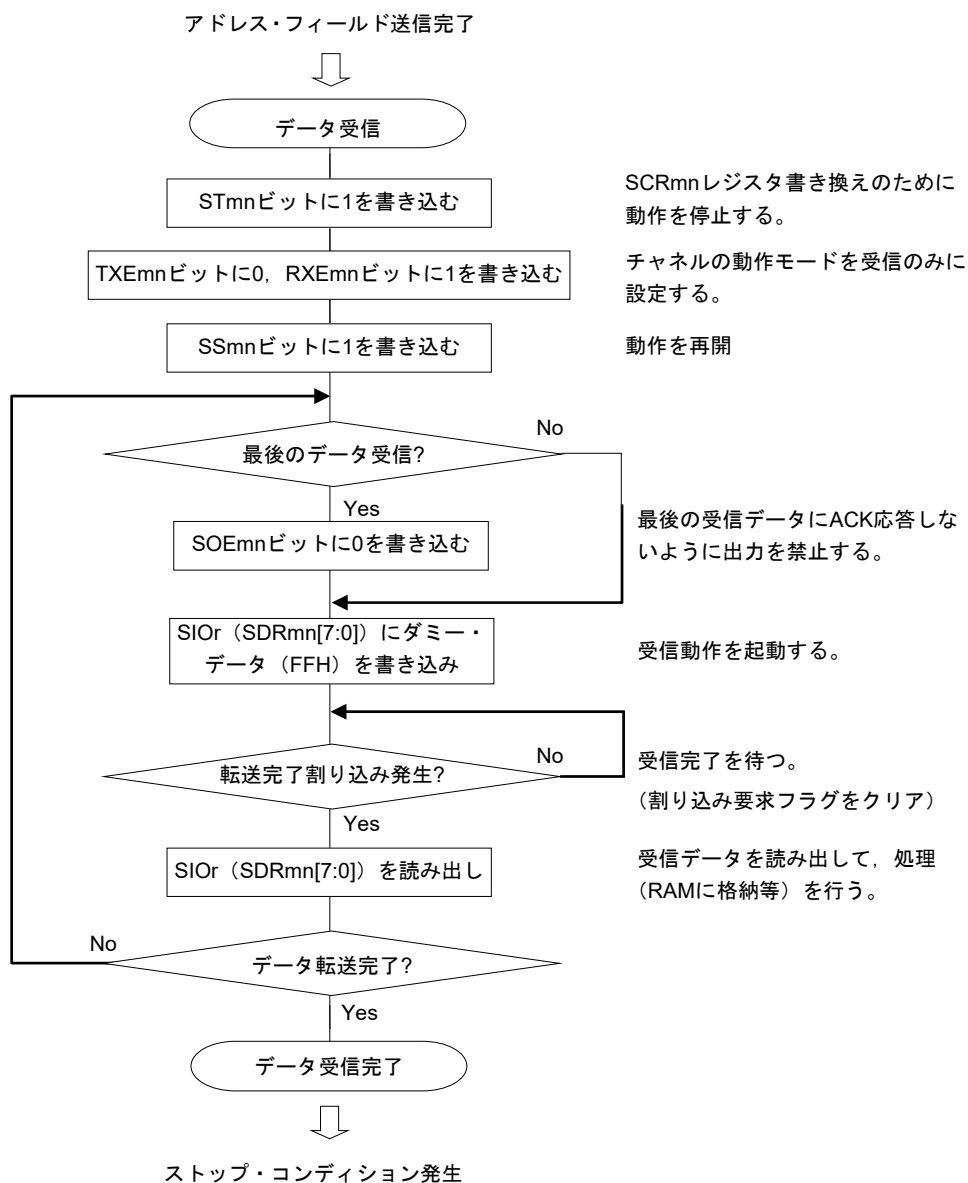
図20-114 データ受信のフロー・チャート
