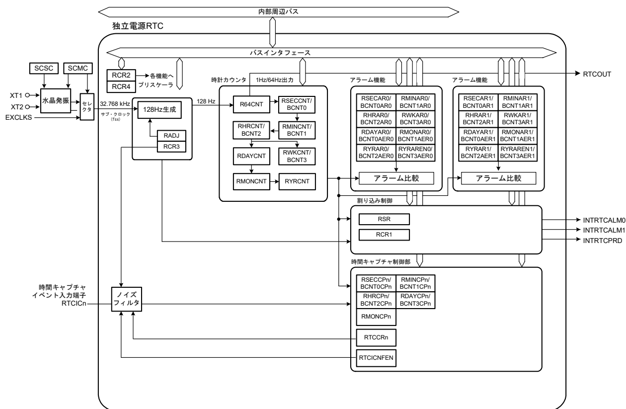
図9-1 RTCのブロック図
