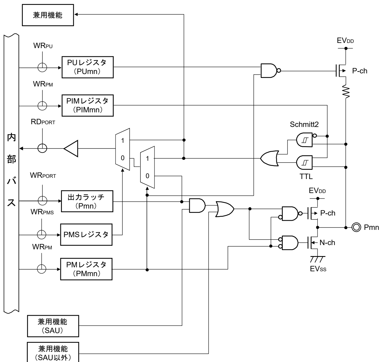
図2-14 端子タイプ8-1-3の端子ブロック図
