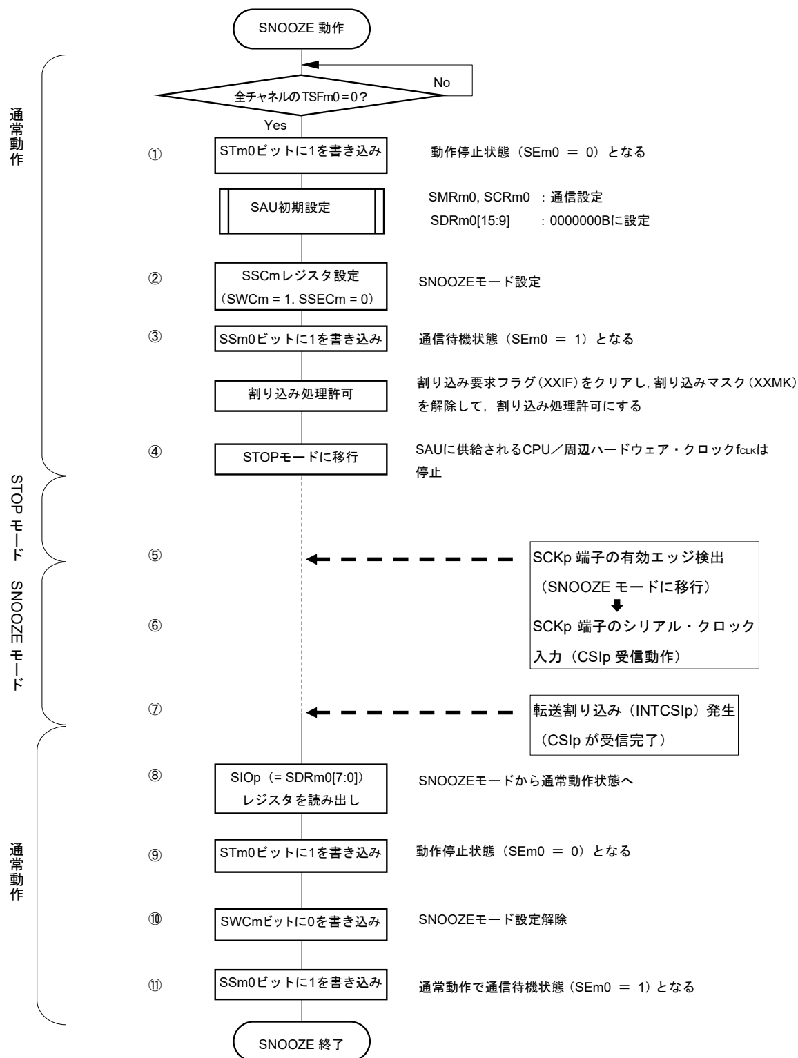
図20-74 SNOOZEモード動作（1回起動）時のフロー・チャート
