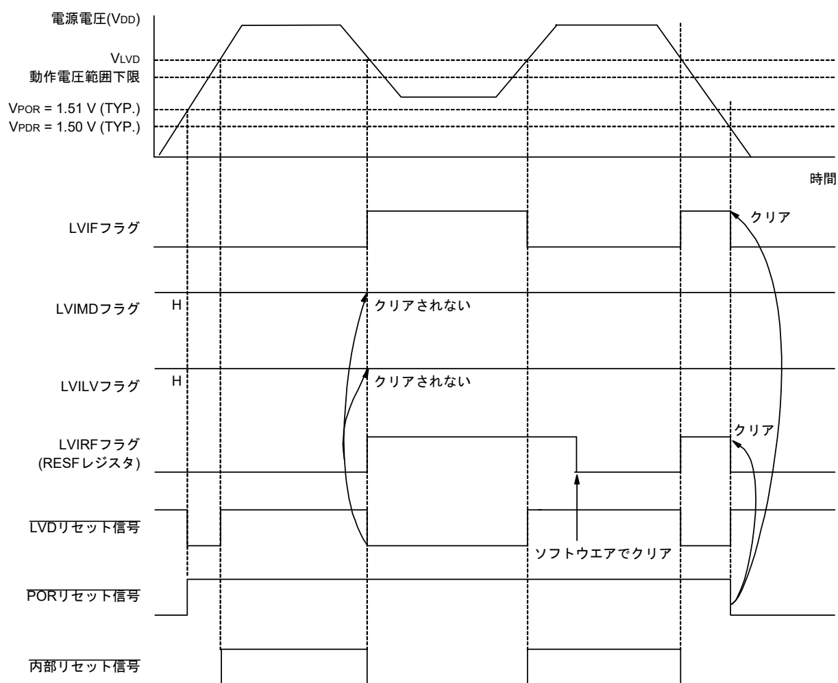
図32-17 内部リセット信号発生タイミング (オプション・バイトLVIMDS1, LVIMDS0 = 1, 1)
