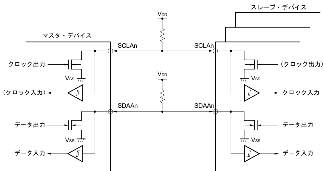
図21-14 端子構成図
