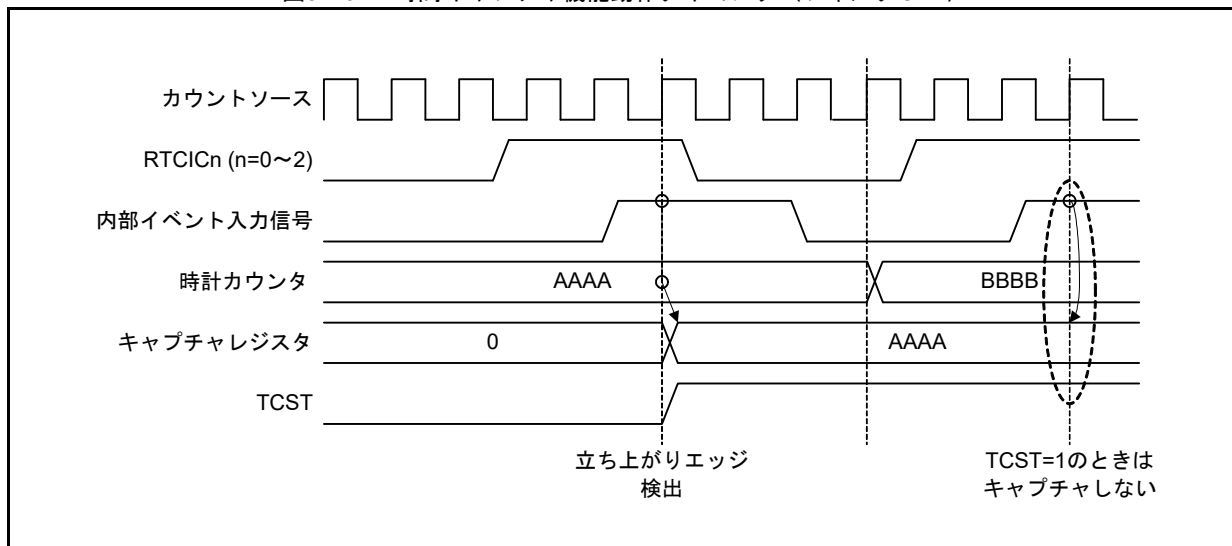
図9-61 時間キャプチャ機能動作タイミング（フィルタOFF）
