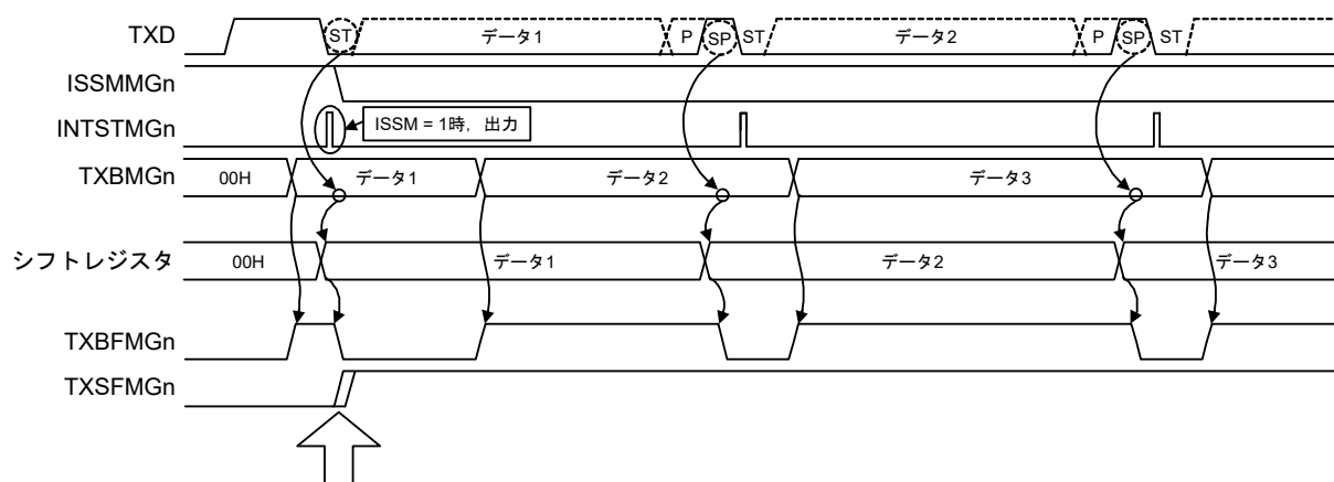
図22-18 連続送信開始タイミング
