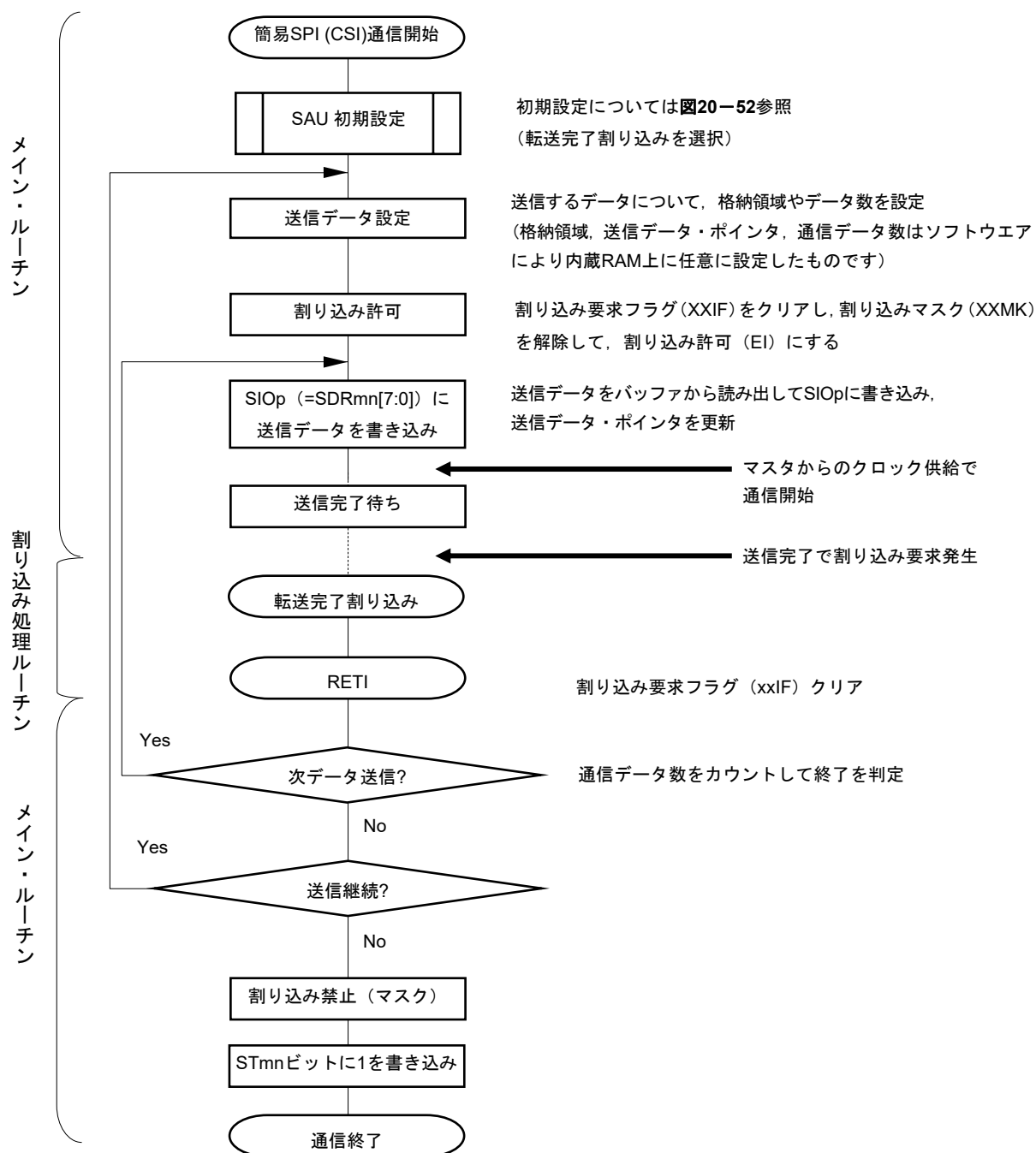
図20-56 スレーブ送信（シングル送信モード時）のフロー・チャート
