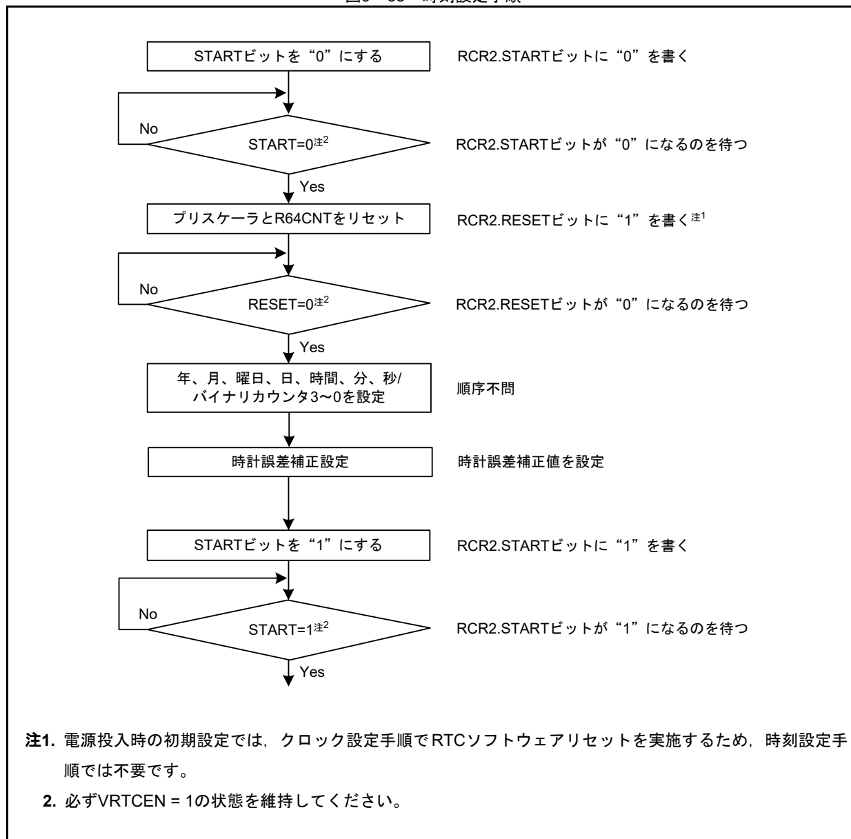
図9-55 時刻設定手順
