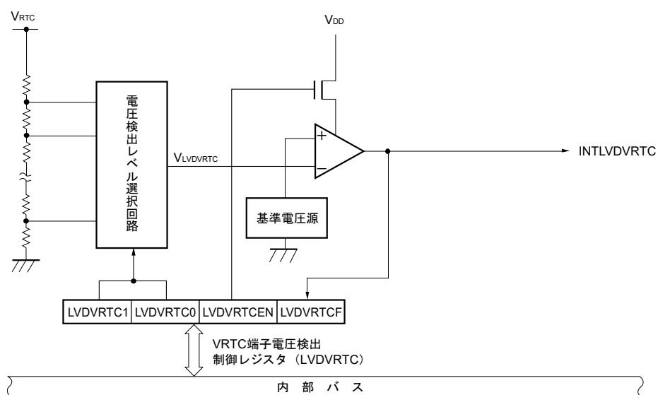
図32-4 VRTC端子電圧検出回路のブロック図
