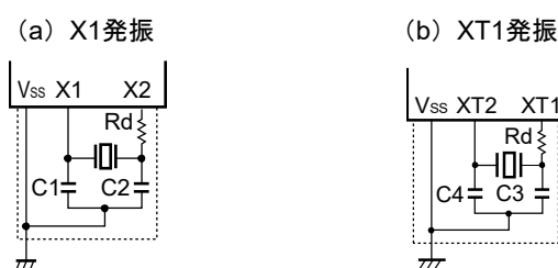
図6-25 外付け回路例
