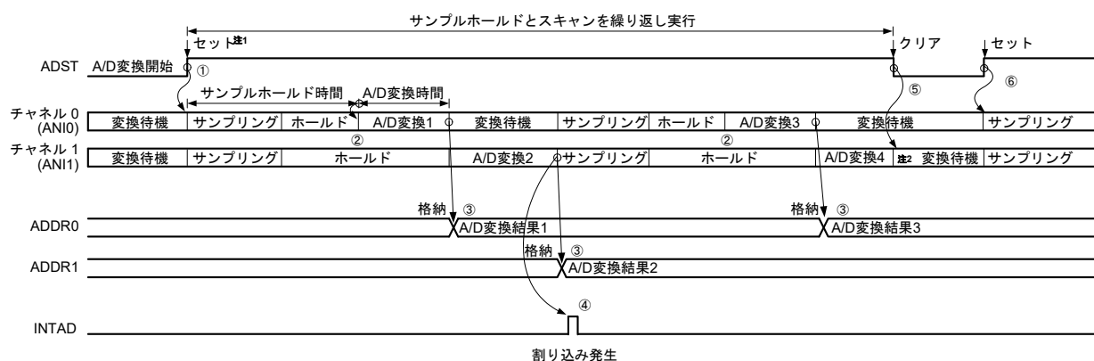
図17-25 連続スキャンモードの動作例（チャンネル専用サンプル&ホールド回路あり）
