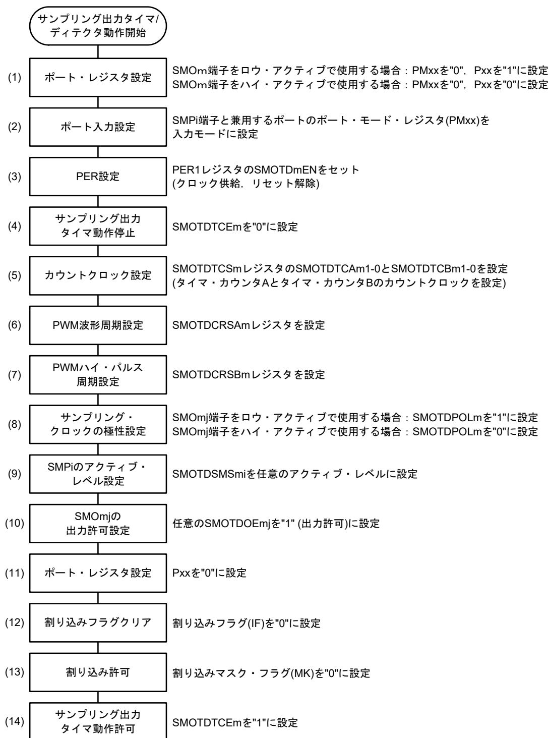
図14-20 動作開始手順
