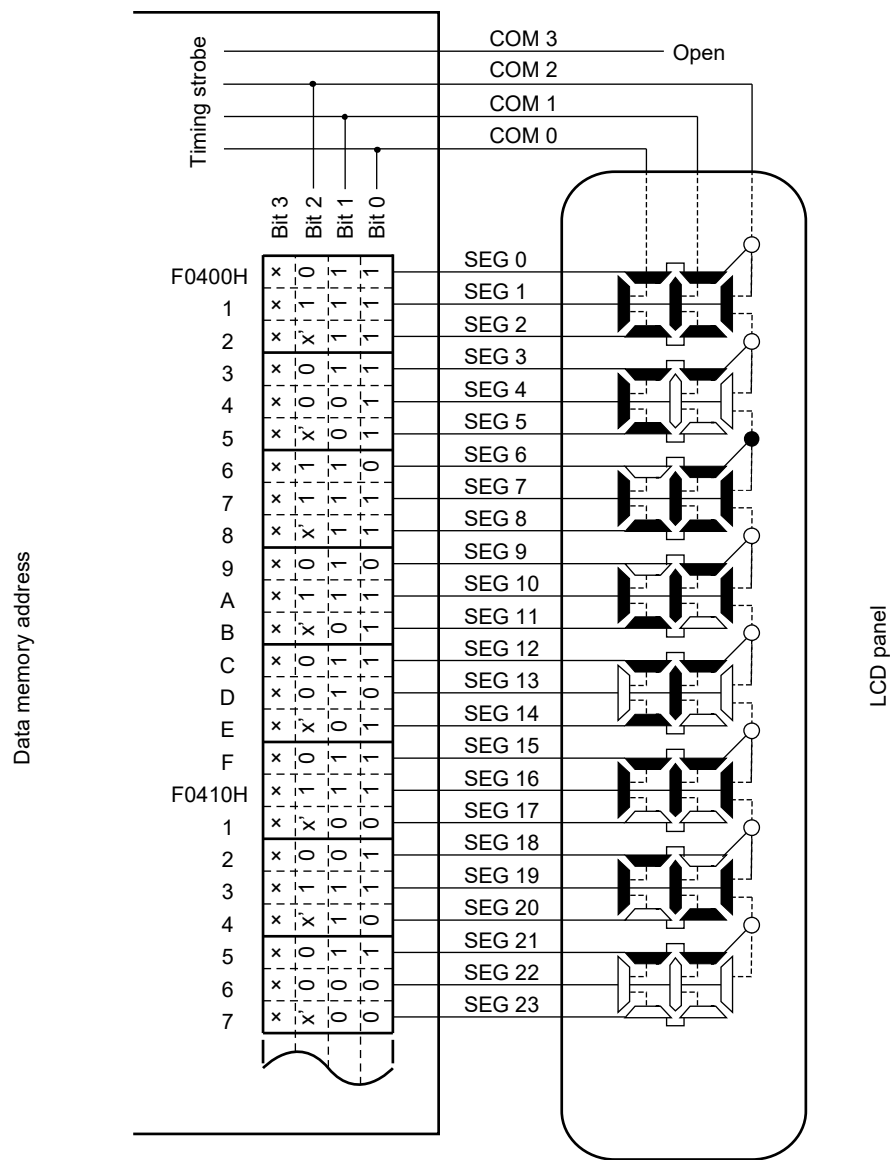
図24-32 3時分割LCDパネルの結線例
