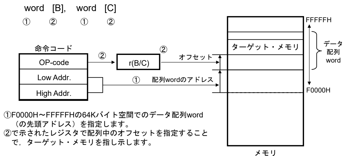
図3-27 word[BC]の例
