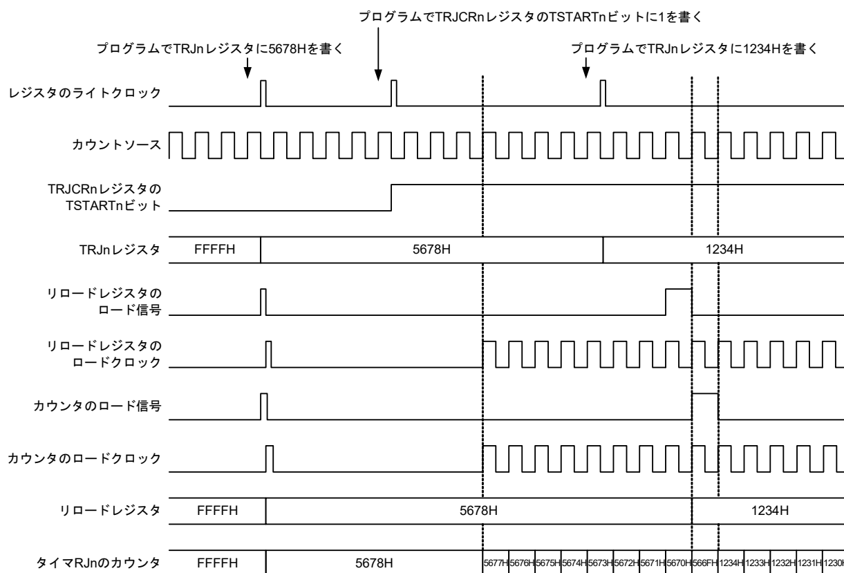
図13-11 TSTARTnビットの値による書き換え動作のタイミング図
