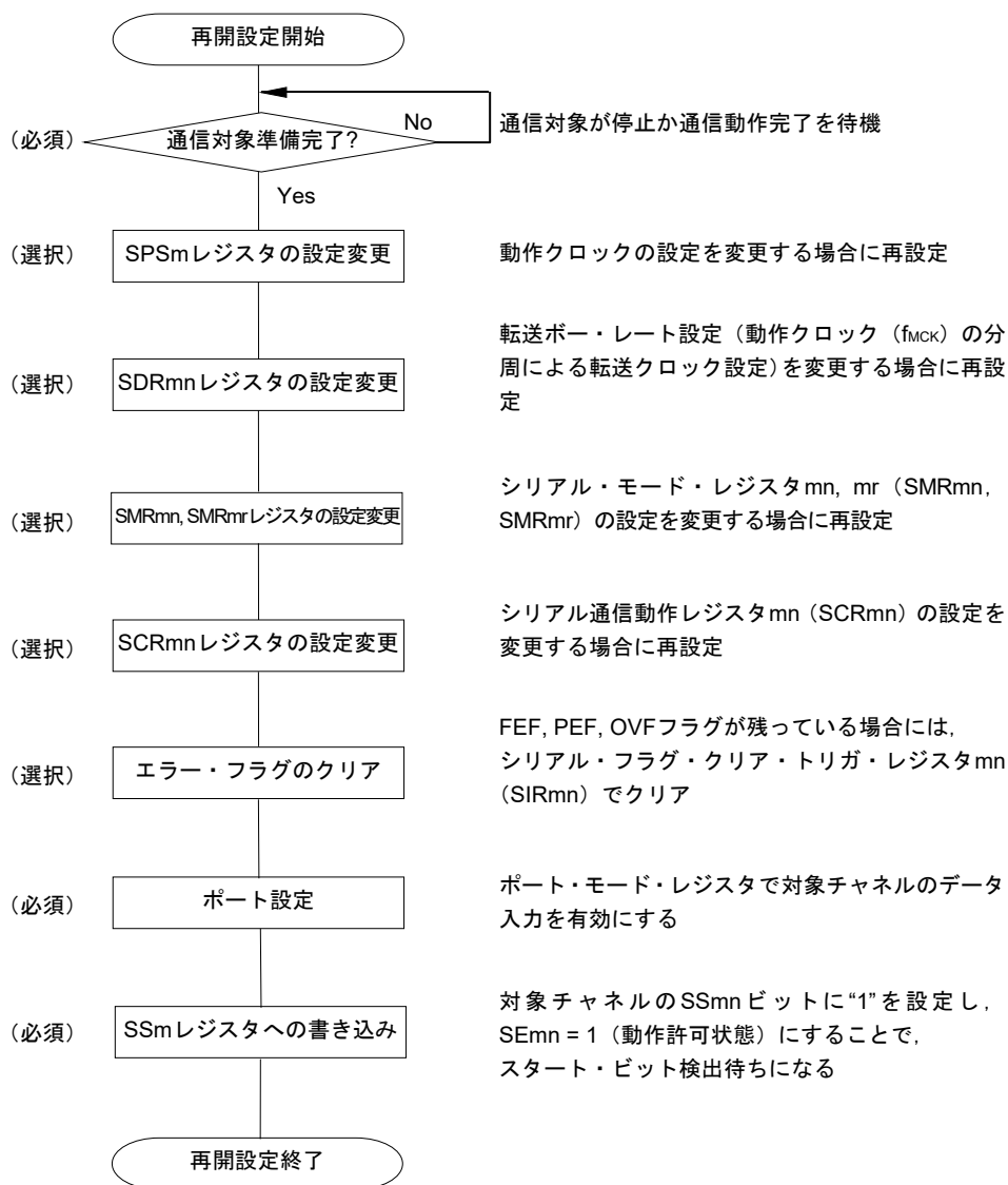
図20-89 UART受信の再開設定手順
