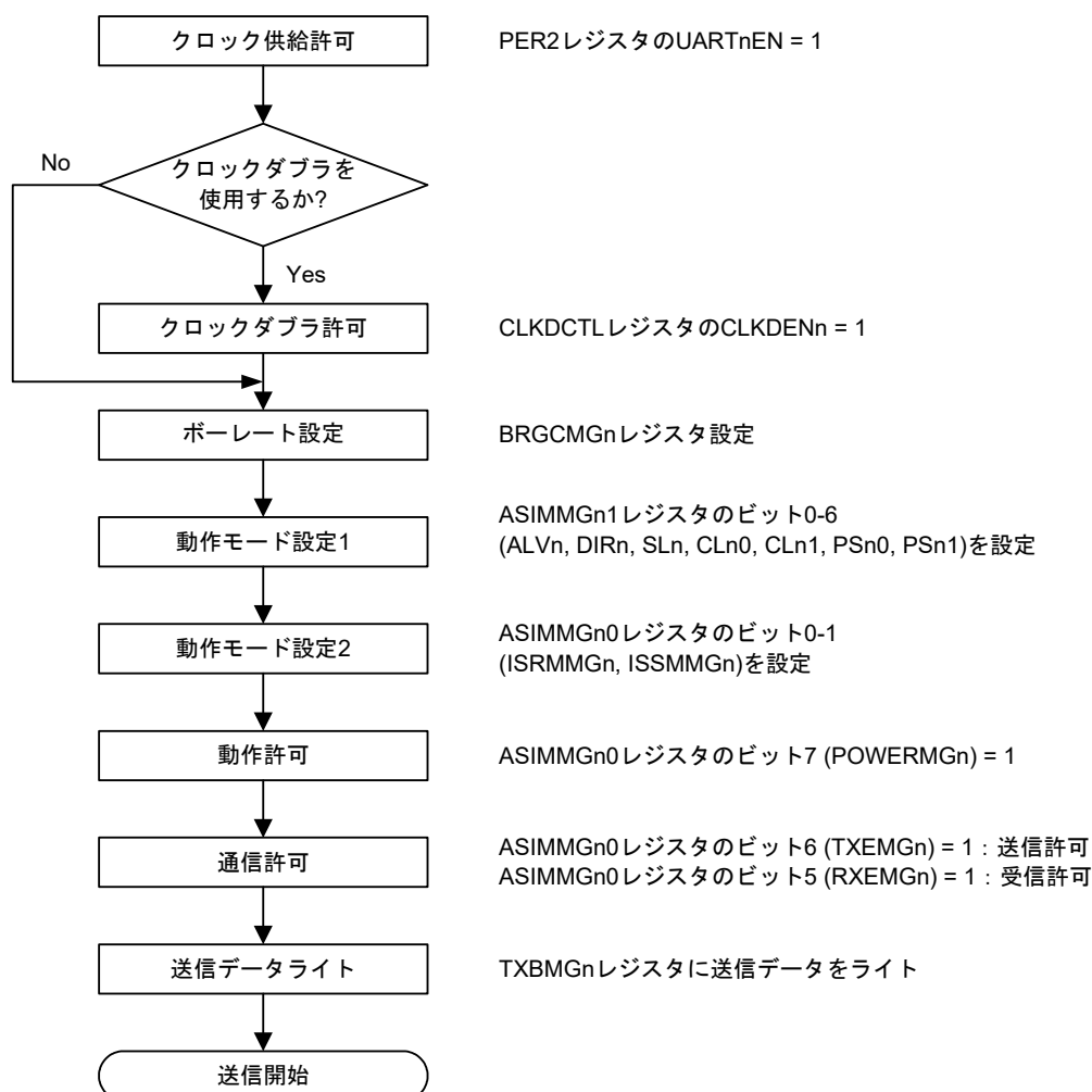
図22-12 通信手順フロー
