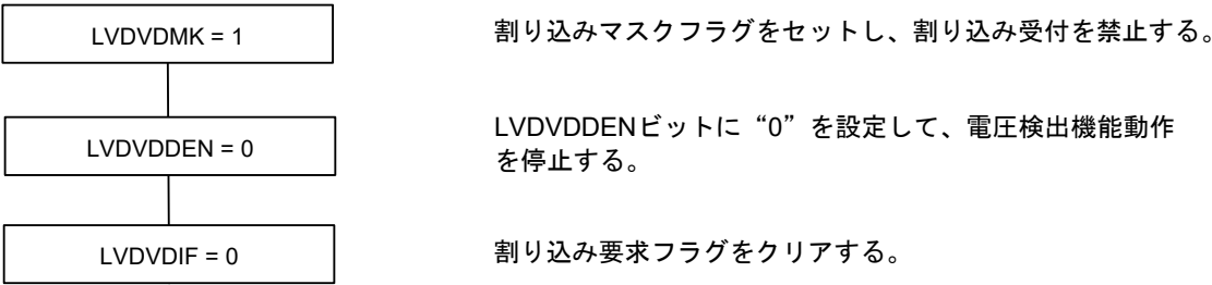
図32-10 V DD 端子電圧検出機能禁止時の設定手順
