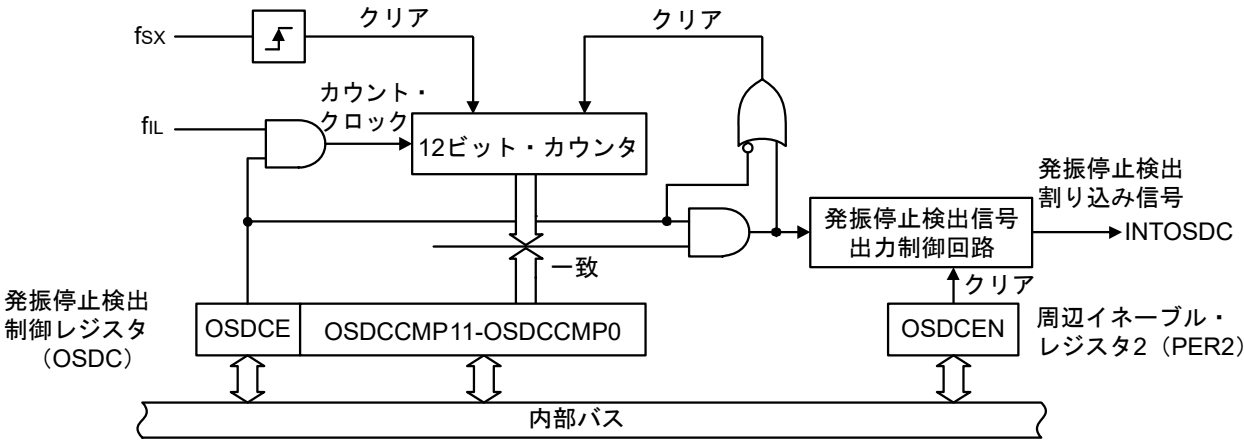
図33-1 発振停止検出回路のブロック図
