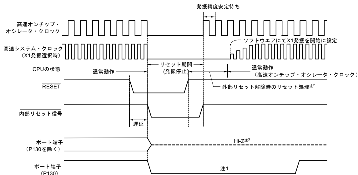
図30-2 RESET入力によるリセット・タイミング
