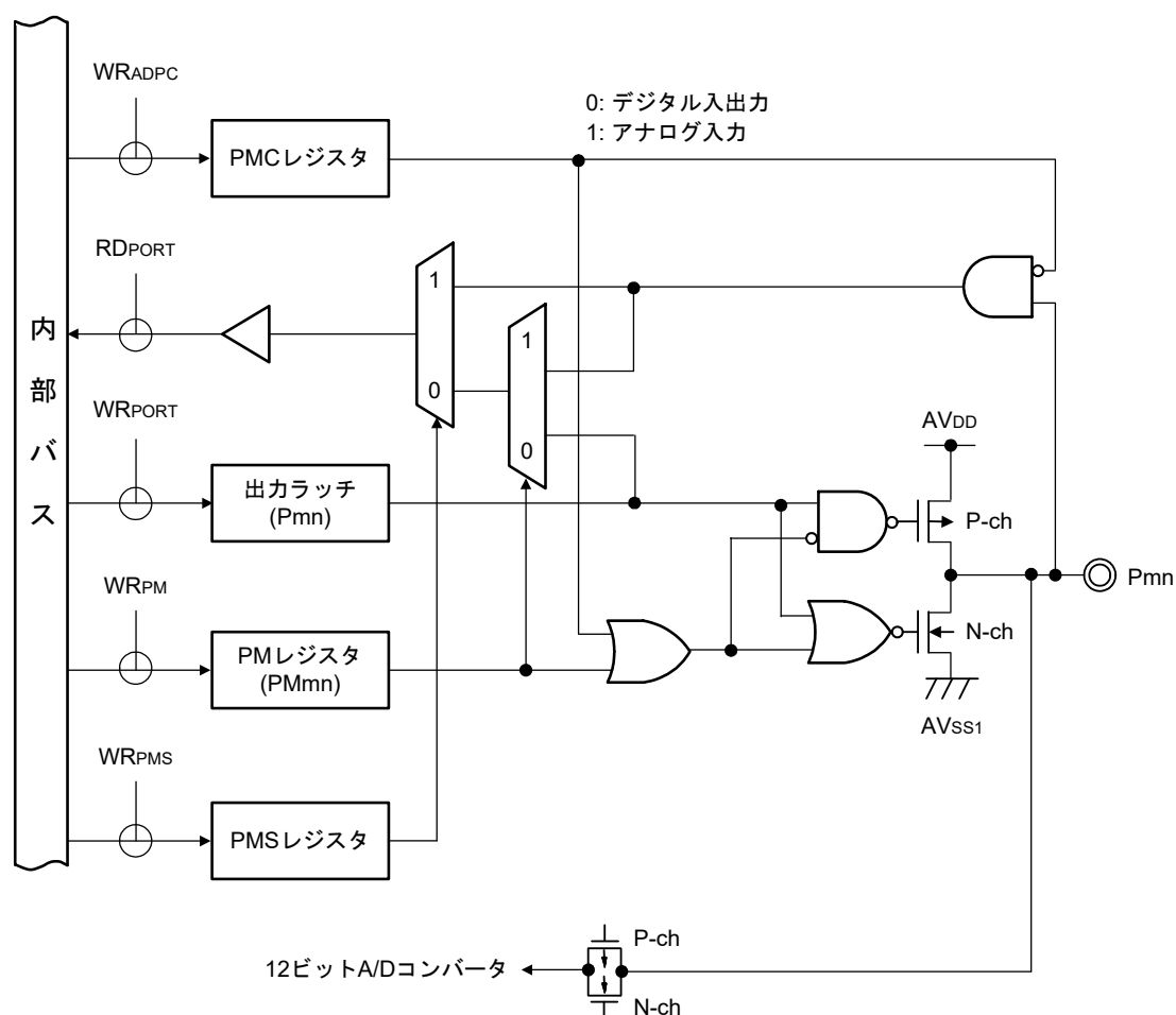
図2-6 端子タイプ4-3-5の端子ブロック図
