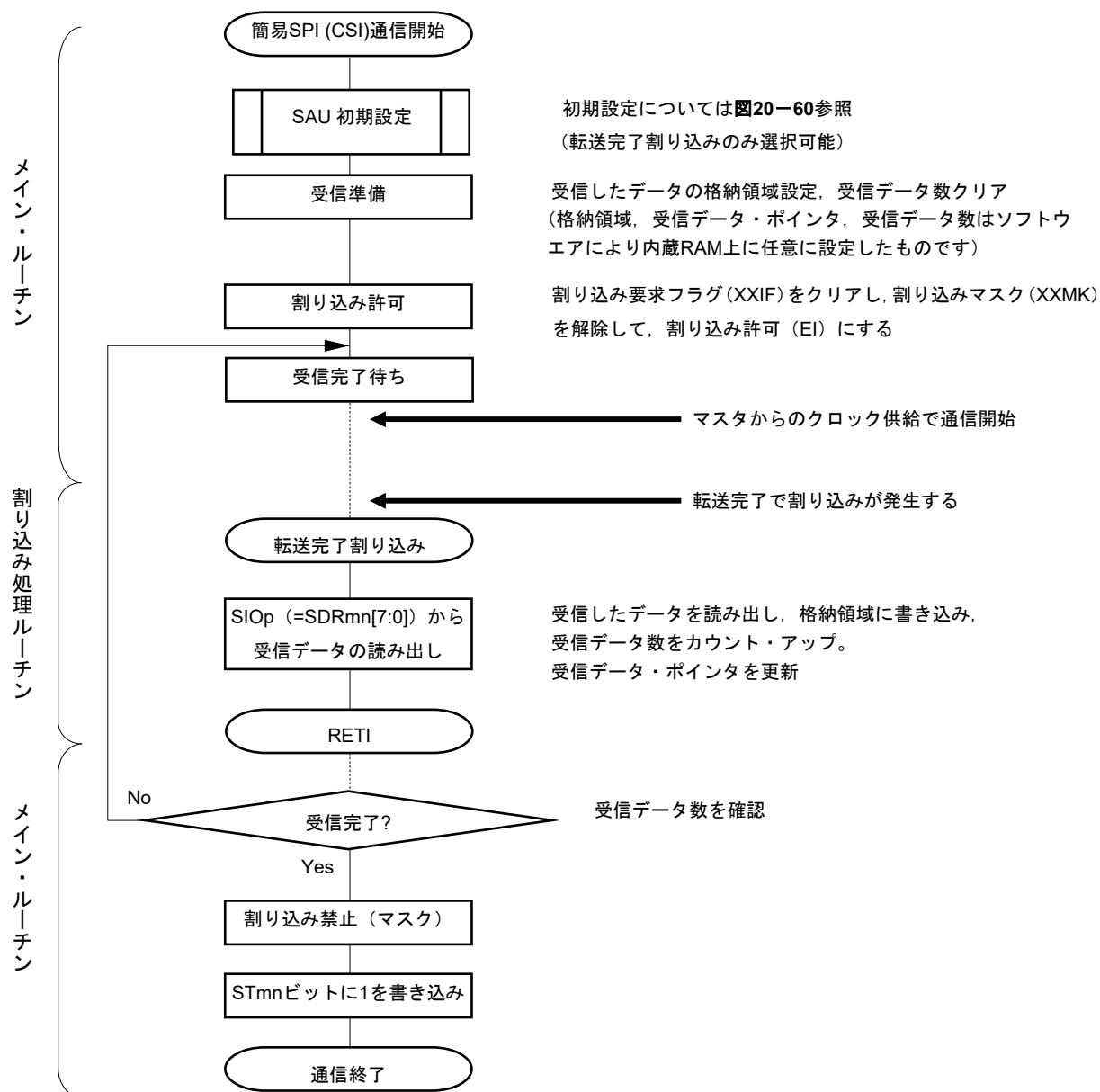
図20-64 スレーブ受信（シングル受信モード時）のフロー・チャート
