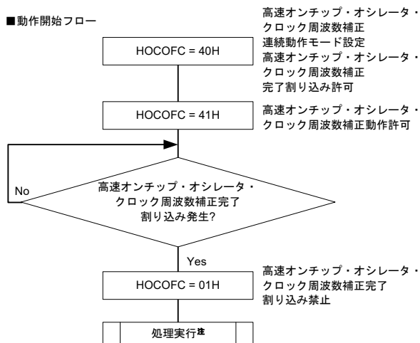
図7-6 動作モード設定手順例
