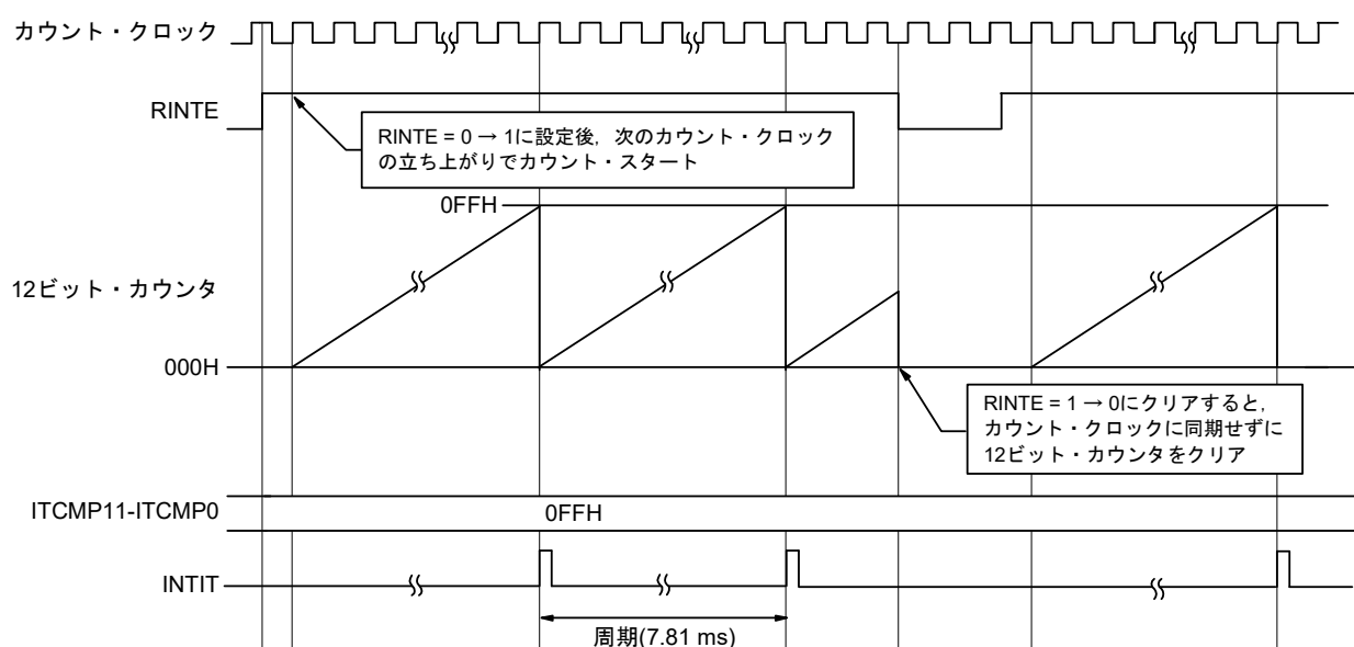
図11-6 12ビット・インターバル・タイマ動作のタイミング (ITCMP11-ITCMP0 = 0FFH, カウント・クロック : f_{sx} = 32.768 \text{ kHz} )
