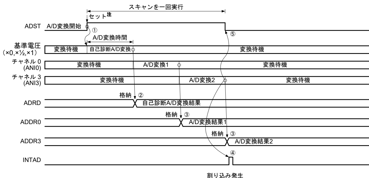
図17-21 シングルスキャンモードの動作例（基本動作：ANI0, ANI3選択 + 自己診断）
