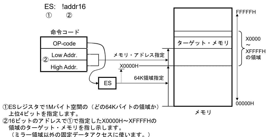
図3-19 ES:!addr16の例
