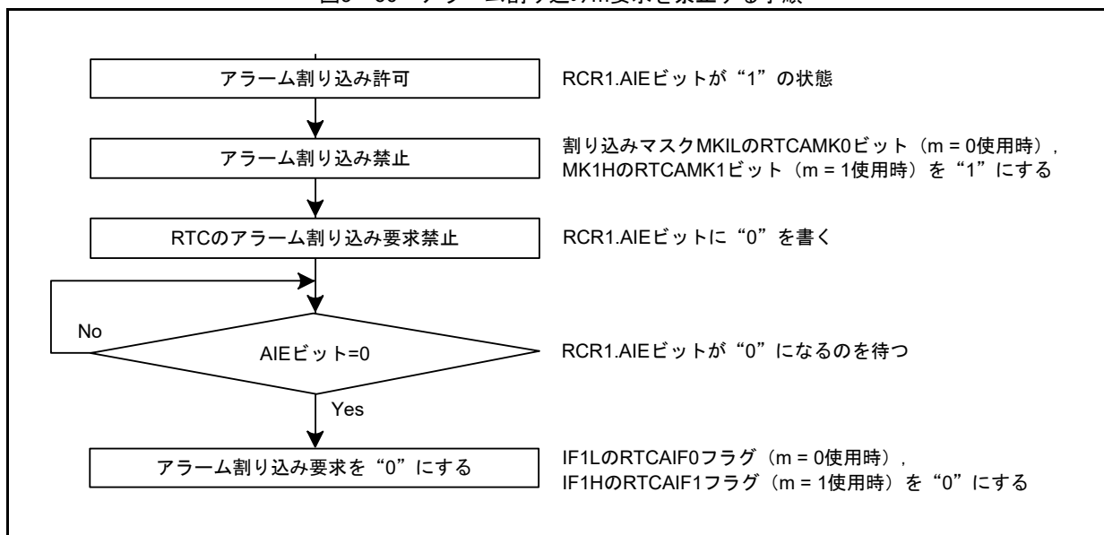
図9-60 アラーム割り込みm要求を禁止する手順
