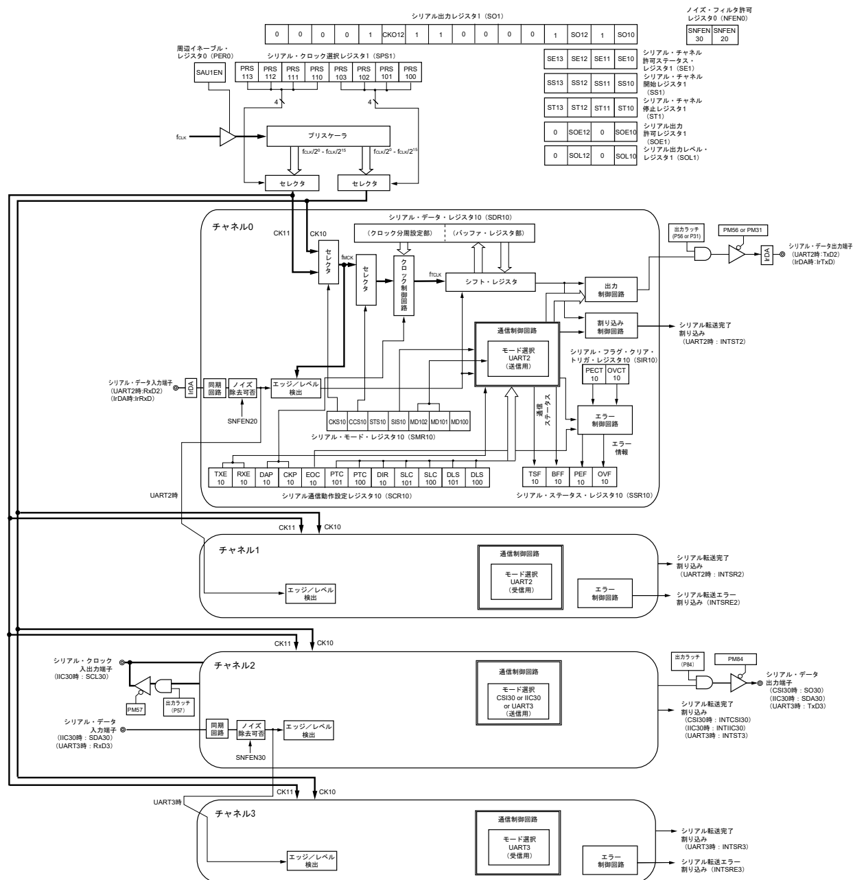
図20-2 シリアル・アレイ・ユニット1のブロック図
