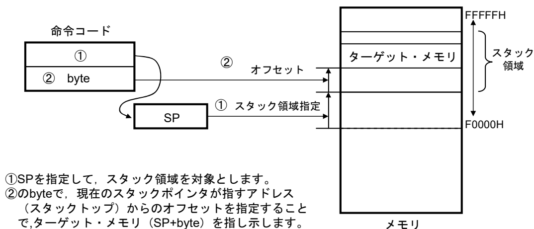
図3-24 [SP+byte]の例
