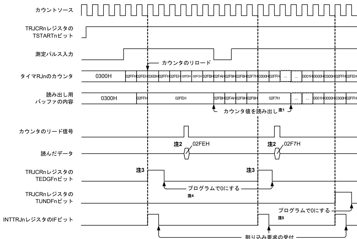
図13-17 パルス周期測定モードの動作例
