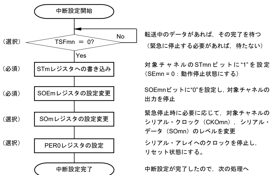
図20-45 マスタ送受信の中断手順
