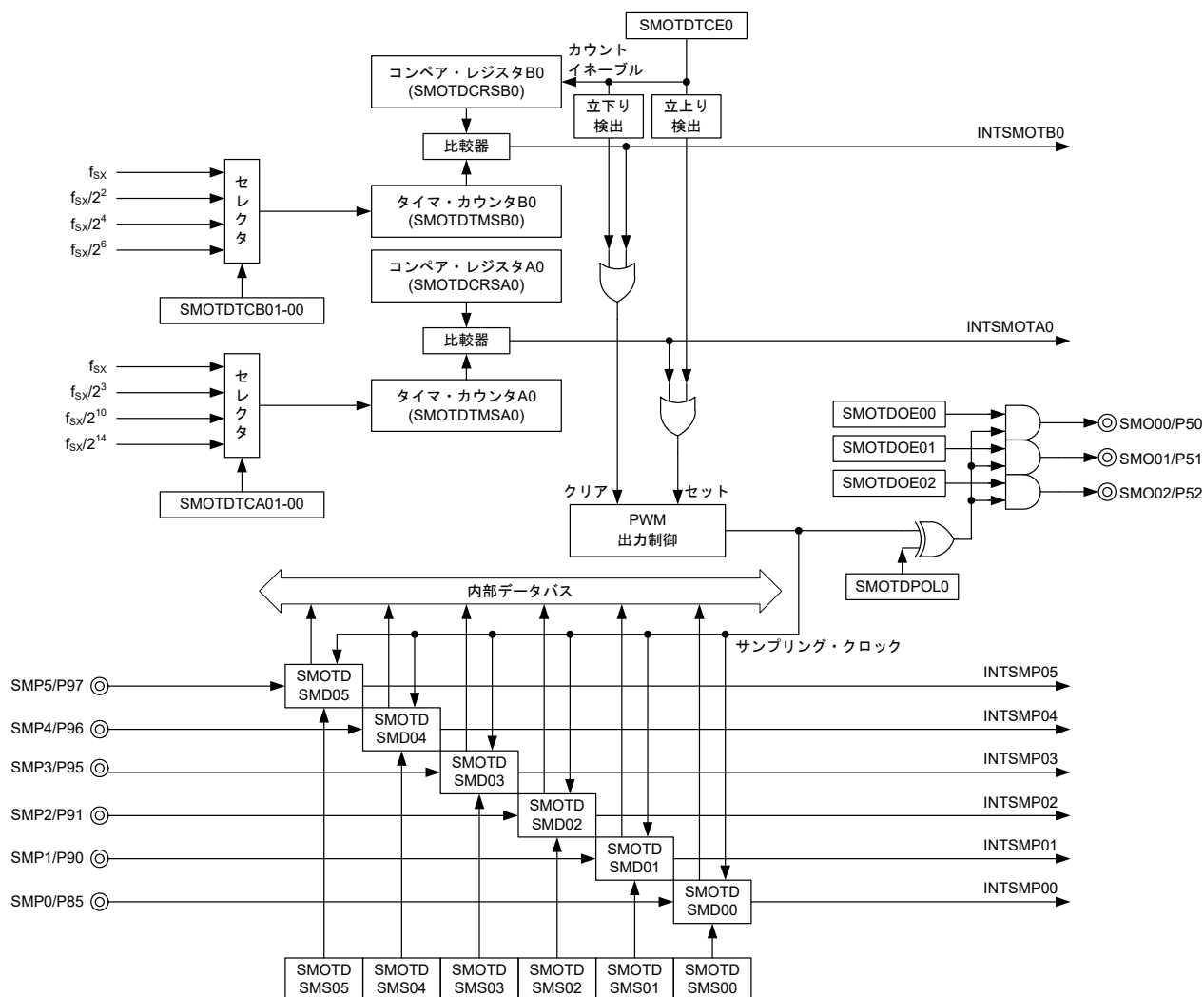
図14-1 サンプリング出力タイマ/ディテクタ0のブロック図
