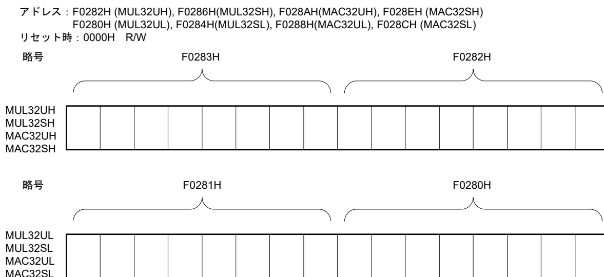
図41-2 乗算データ・レジスタA(MUL32UH, MUL32UL, MUL32SH, MUL32SL, MAC32UH, MAC32UL, MAC32SH, MAC32SL) のフォーマット
