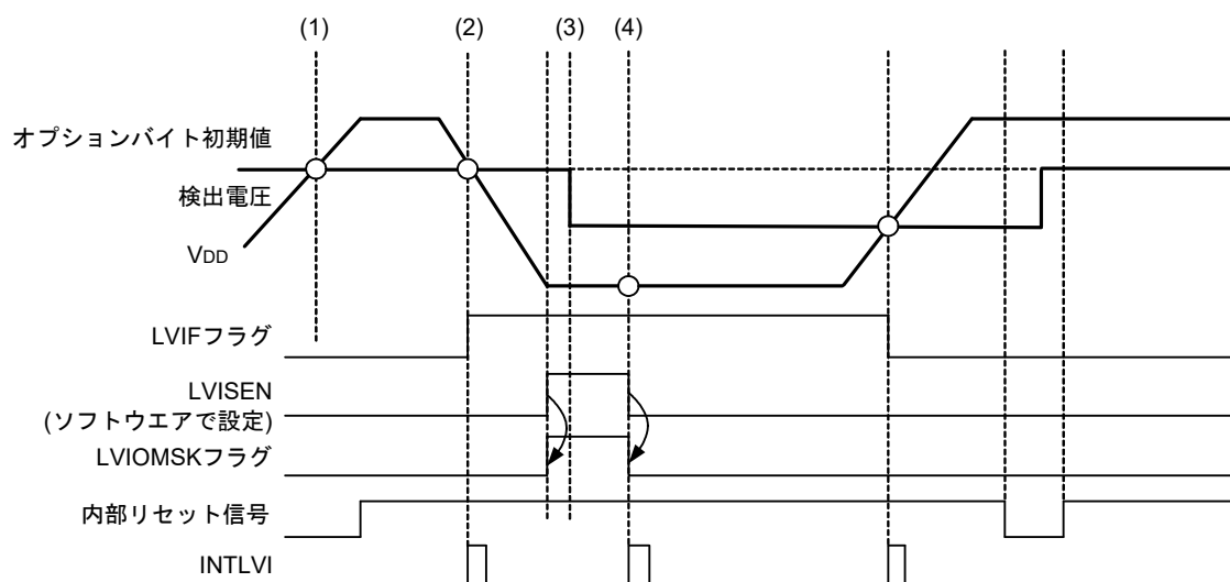
図32-28 V_{DD} < V_{LVD} 時, LVISによるLVD検出電圧の設定変更タイミング例
