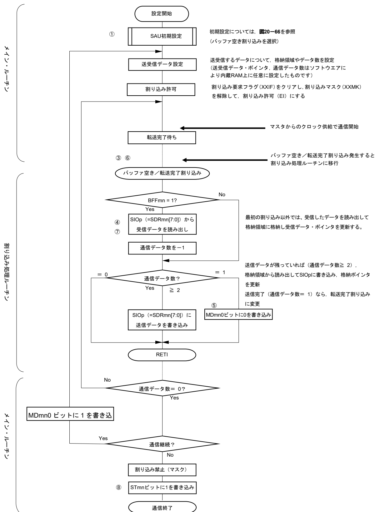
図20-72 スレーブ送受信（連続送受信モード時）のフロー・チャート
