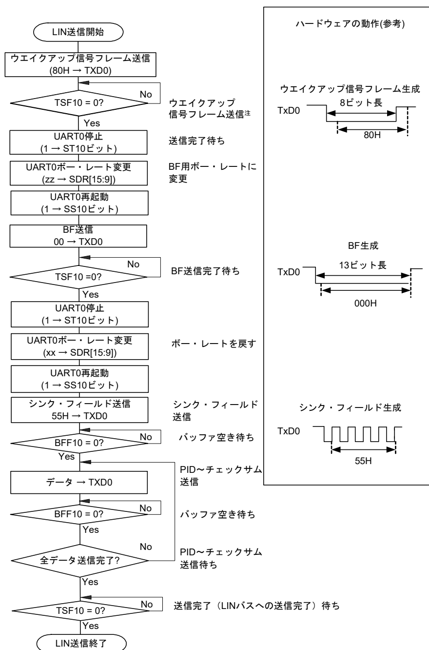
図20-101 LIN送信のフロー・チャート
