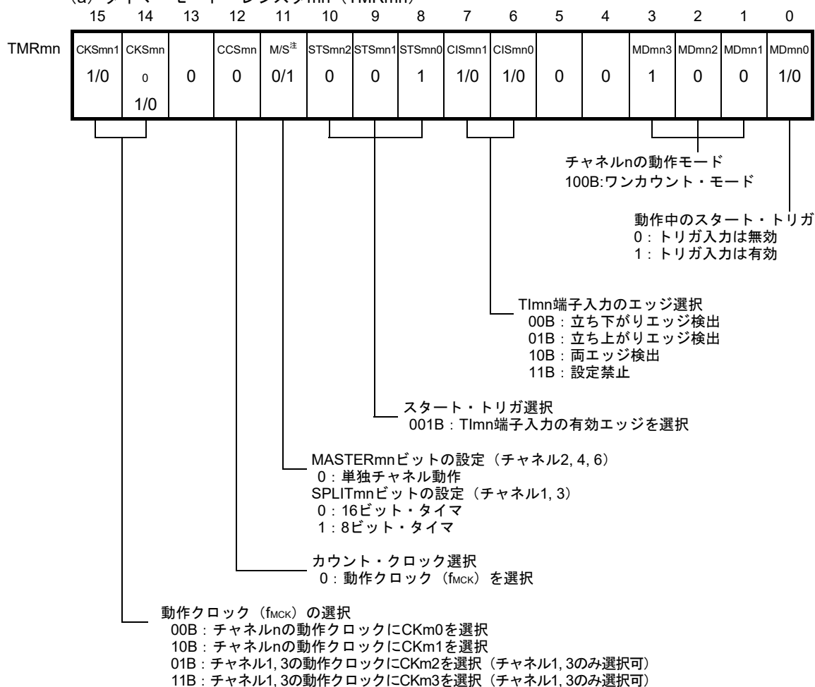
図8-63 ディレイ・カウンタ機能時のレジスタ設定内容例
