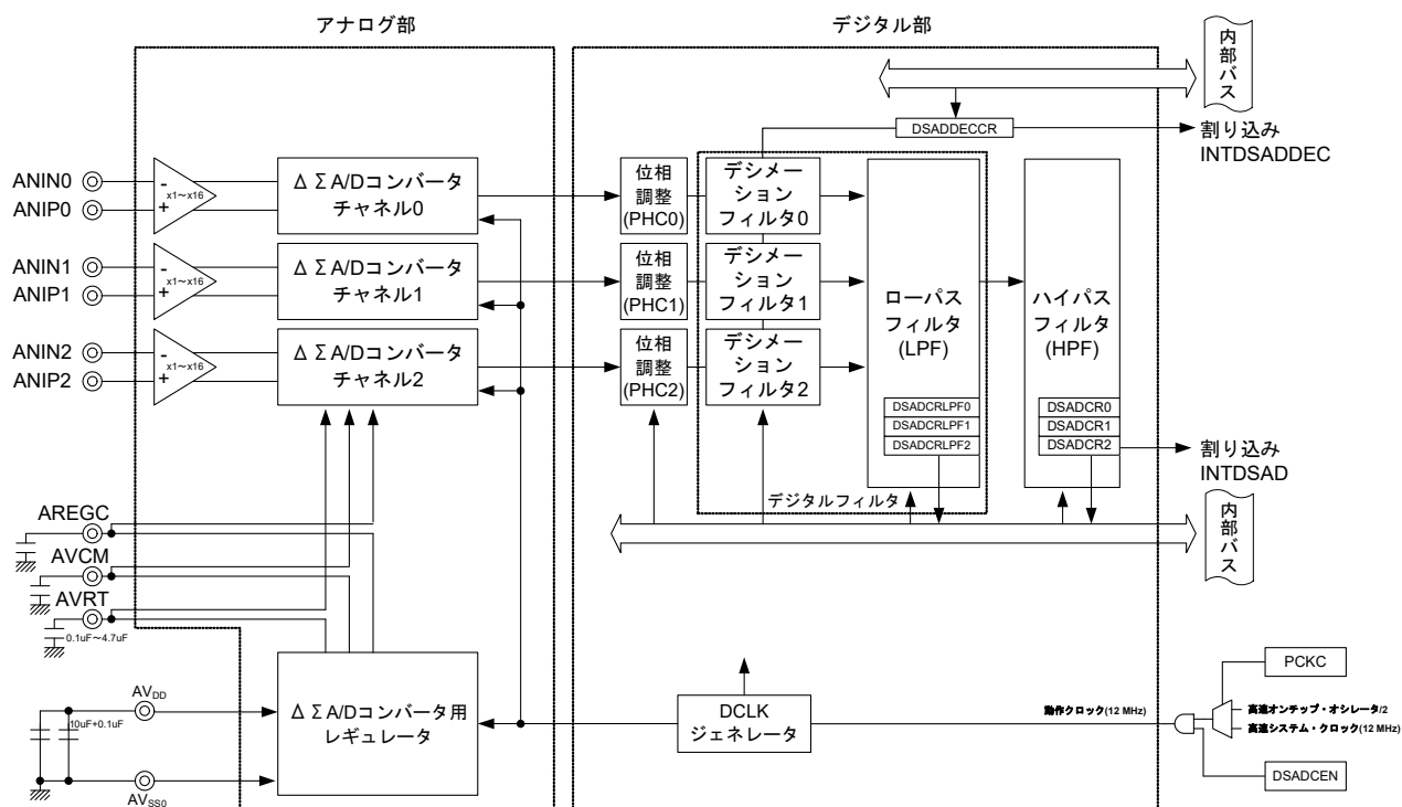
図19-2 24ビット \Delta\Sigma A/Dコンバータのブロック図 (80ピン製品)
