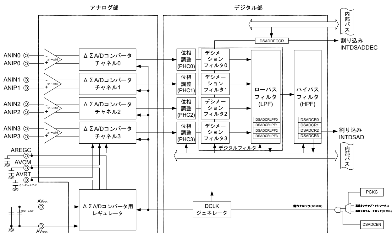
図19-1 24ビット \Delta\Sigma A/Dコンバータのブロック図 (100ピン製品)
