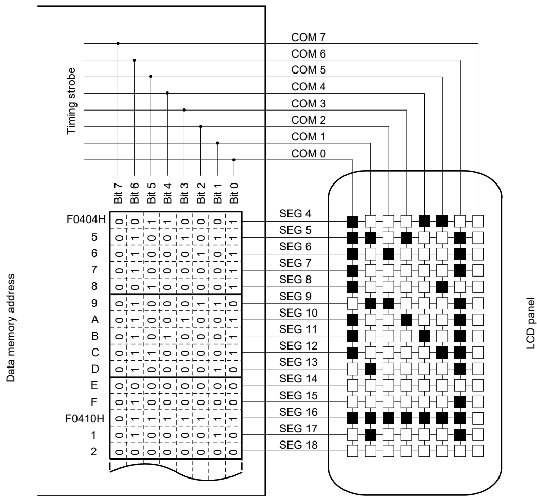
図24-42 8時分割LCDパネルの結線例
