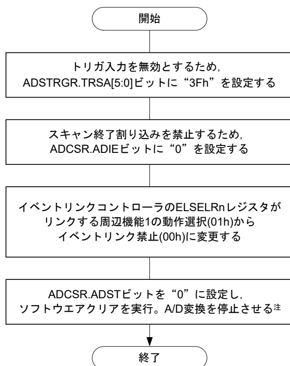
図17-31 ADCSR.ADSTビットによるソフトウェアクリア実行の設定フロー
