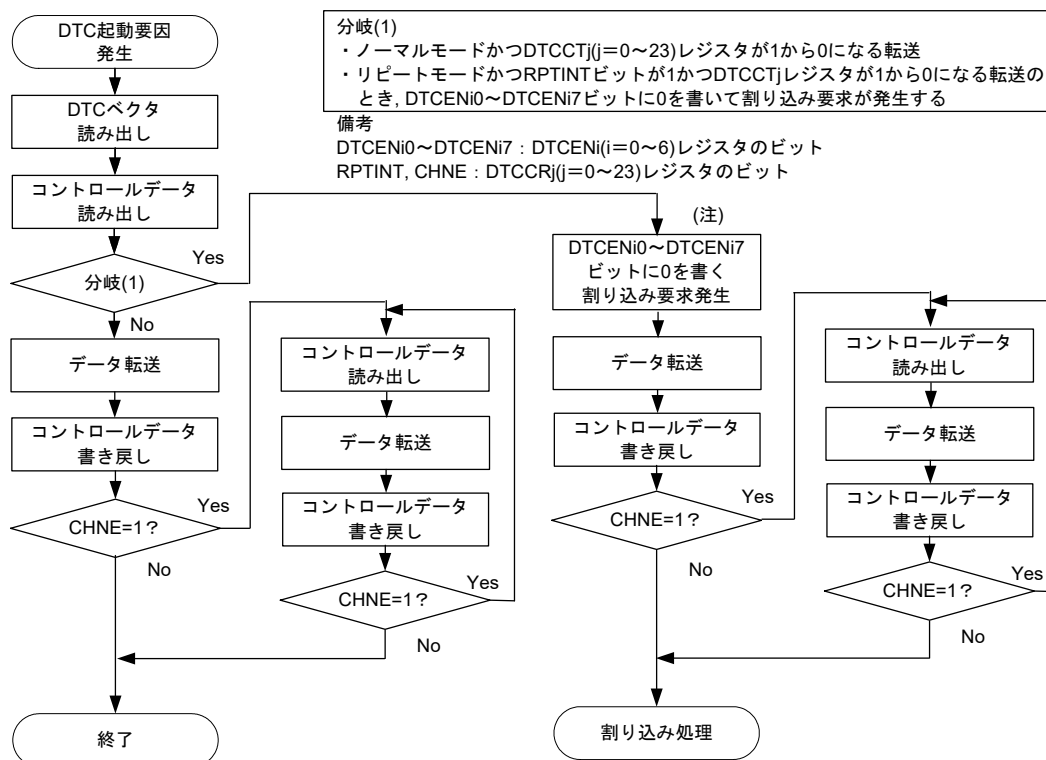
図25-14 DTC内部動作フローチャート
