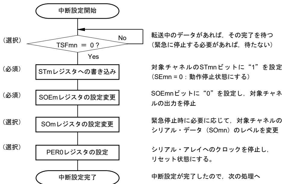
図20-67 スレーブ送受信の中断手順
