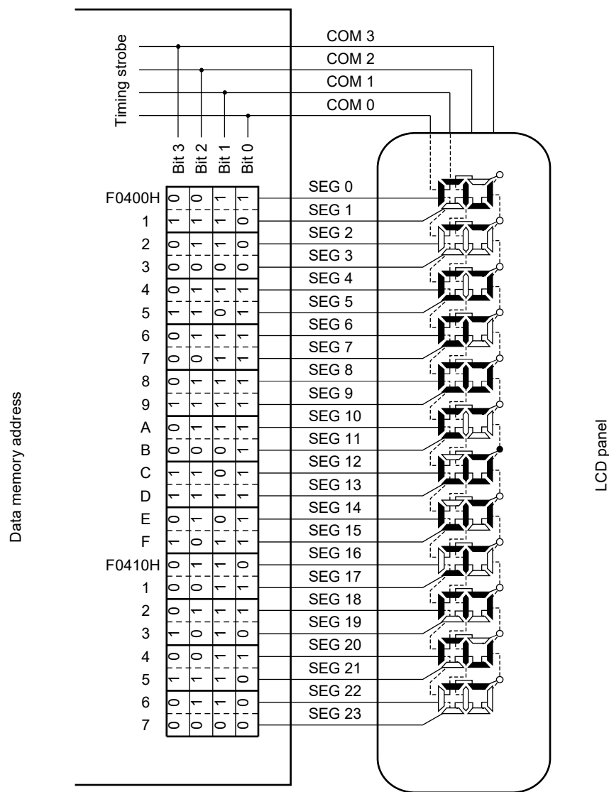
図24-36 4時分割LCDパネルの結線例
