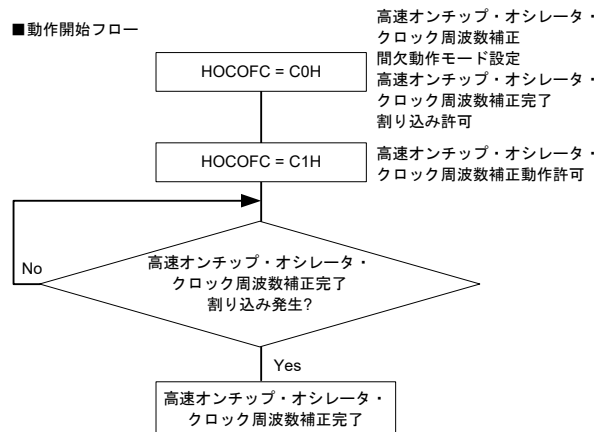
図7-6 動作モード設定手順例
