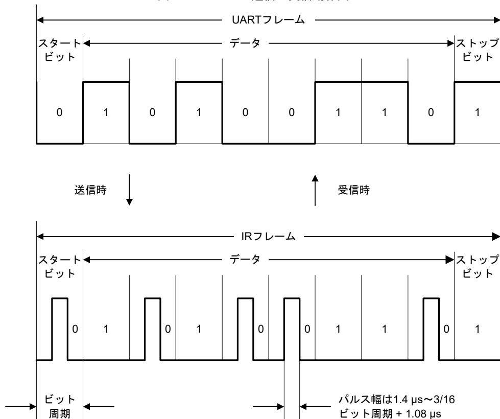
図23-5 IrDAの送信/受信動作図
