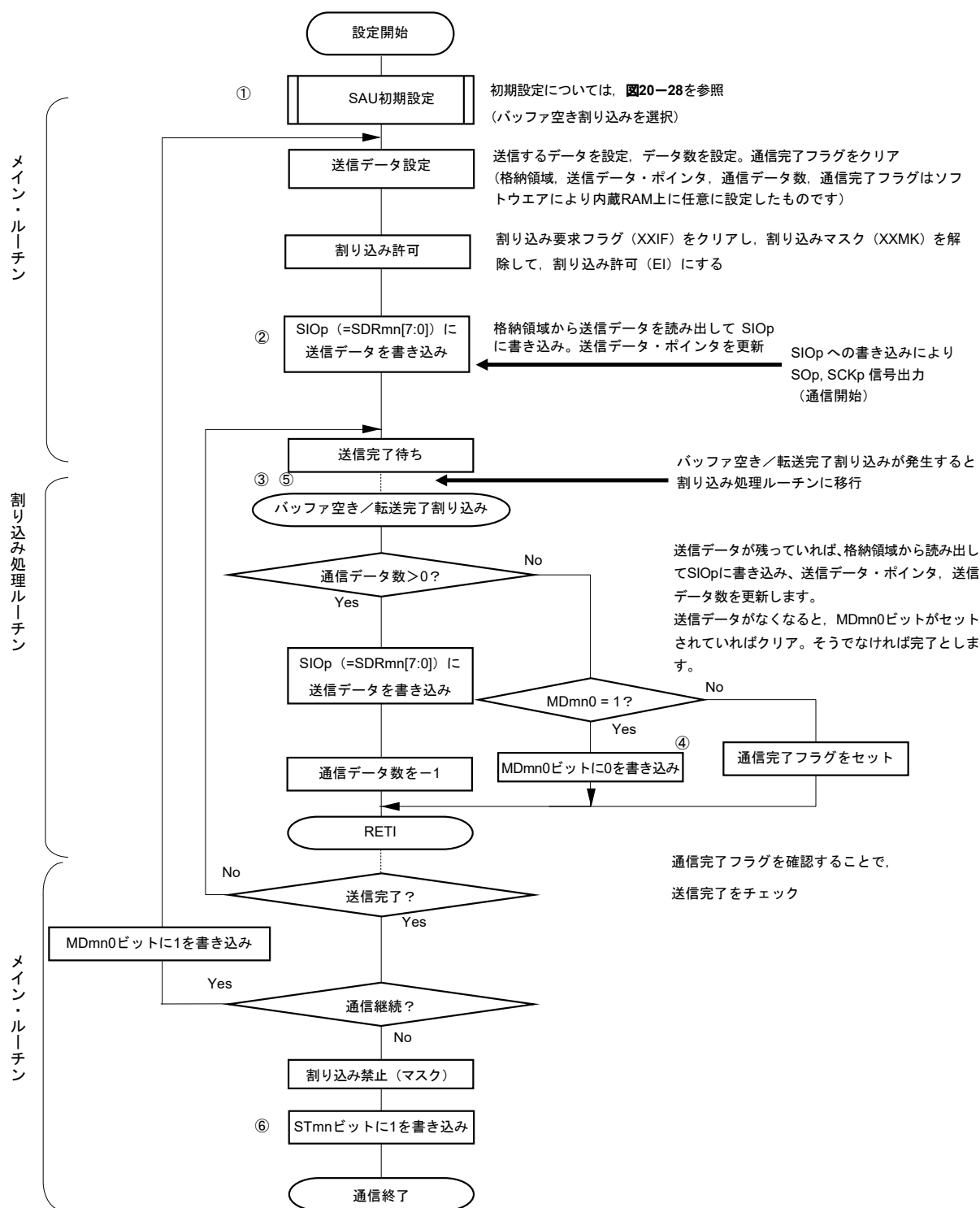
図20-34 マスタ送信（連続送信モード時）のフロー・チャート
