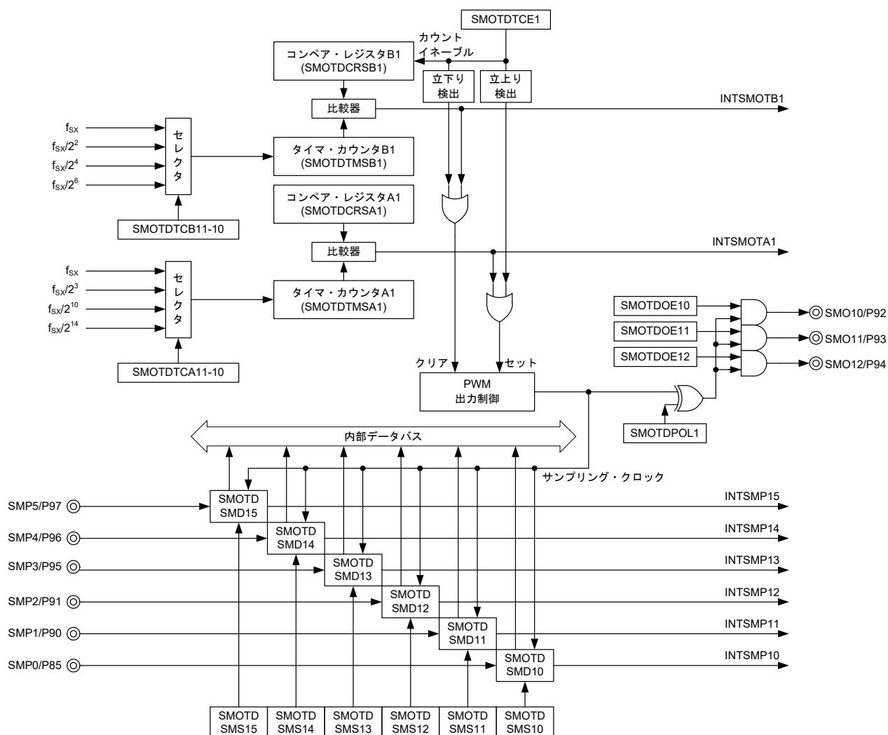
図14-2 サンプリング出力タイマ/ディテクタ1のブロック図
