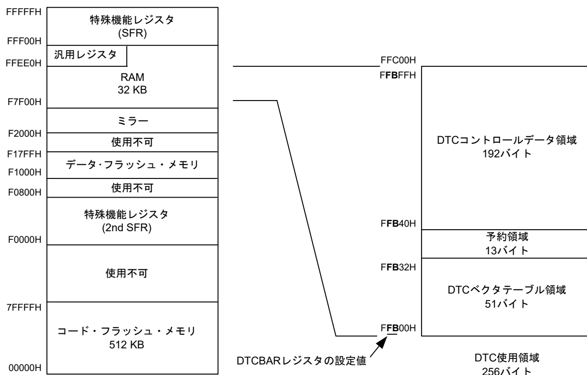
図25-2 DTCBARレジスタにFBHを設定したときのメモリマップ例 (R5F10NPLDFB, R5F10NMLDFB)
