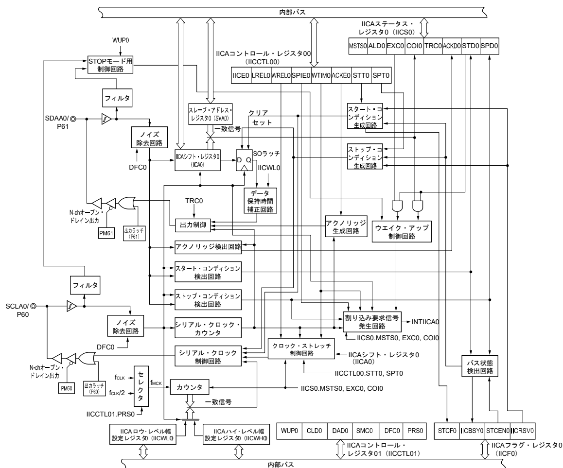
図21-1 シリアル・インタフェースIICA0のブロック図
