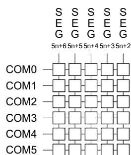
図24－38 6時分割LCD表示パターンと電極結線
