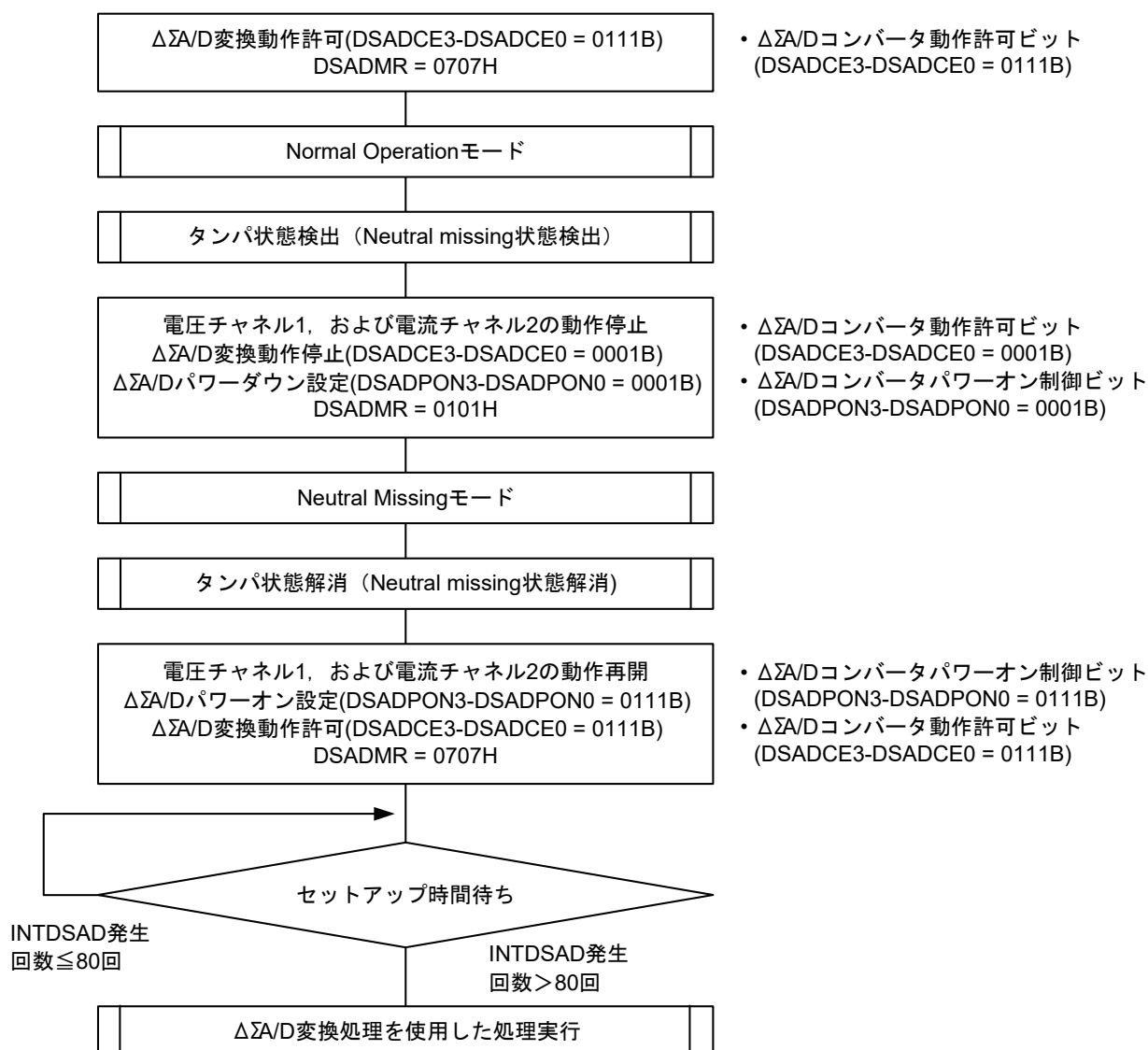
図19-17 Normal OperationからNeutral Missingモードへの切替手順
