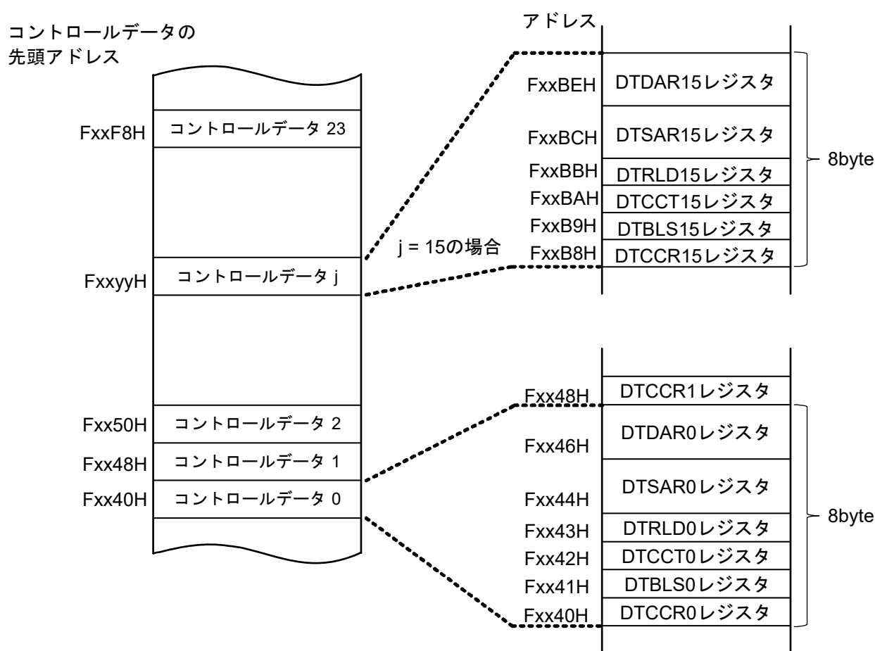
図25-3 コントロールデータの配置
