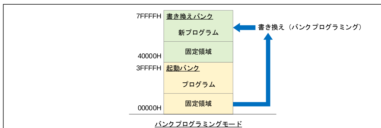
図 2-3 バンクプログラミング機能の概念図
