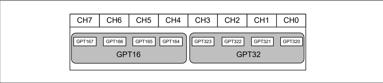
図 21.2 GPT チャンネルとモジュール名の関係
