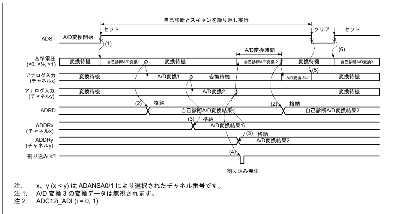
図 37.14 連続スキャンモードの基本動作例（アナログ入力（チャンネル x、y）選択+自己診断）
