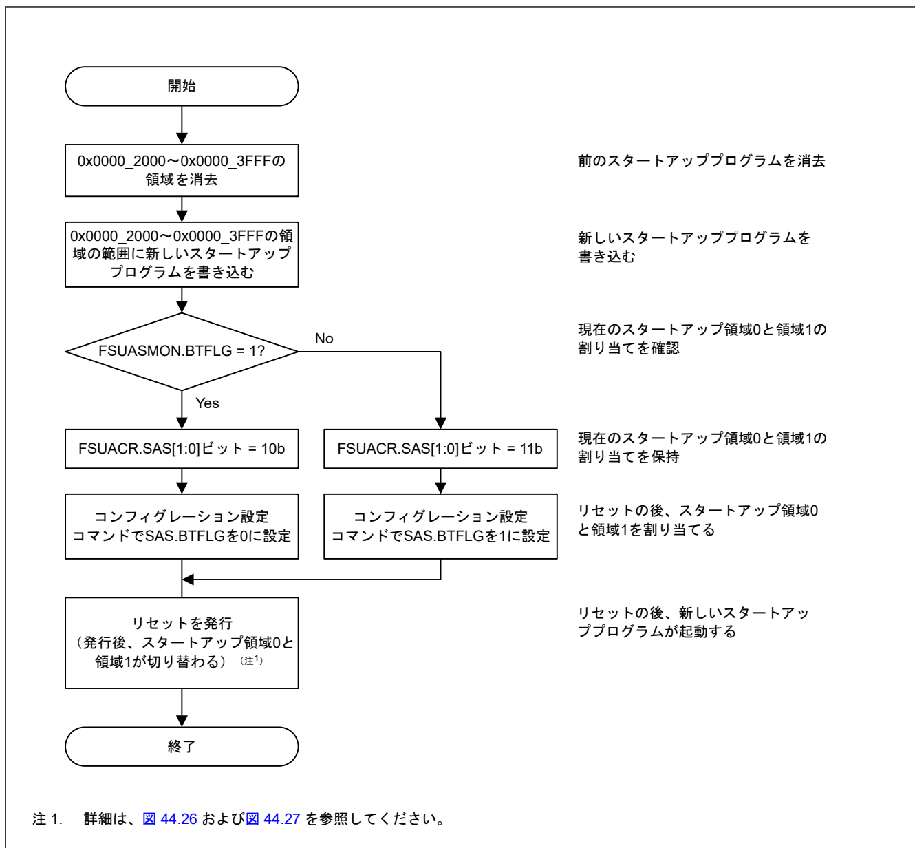
図 44.28 スタートアッププログラムプロテクションの概念
