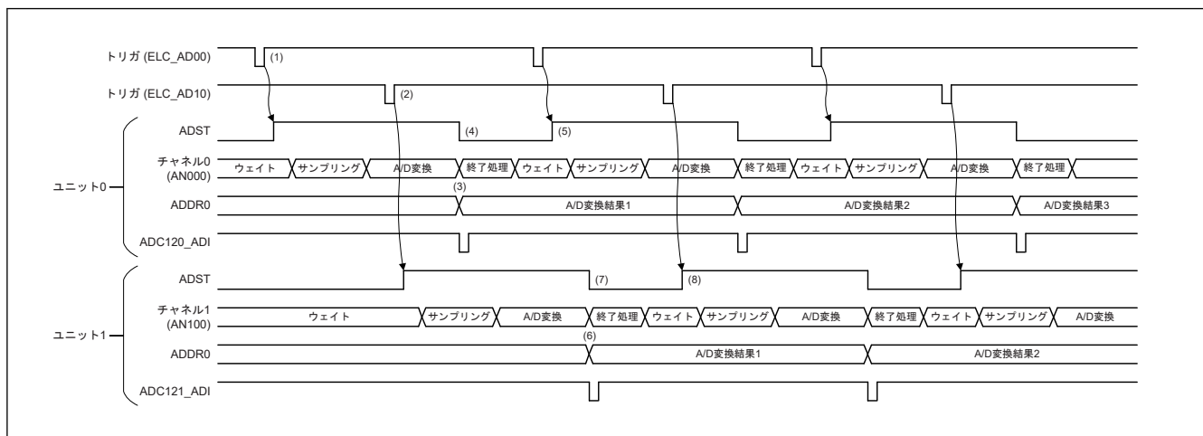
図 37.26 シングルスキャンモードの動作例 (AN000 および AN100 選択、インターリーブ動作)
