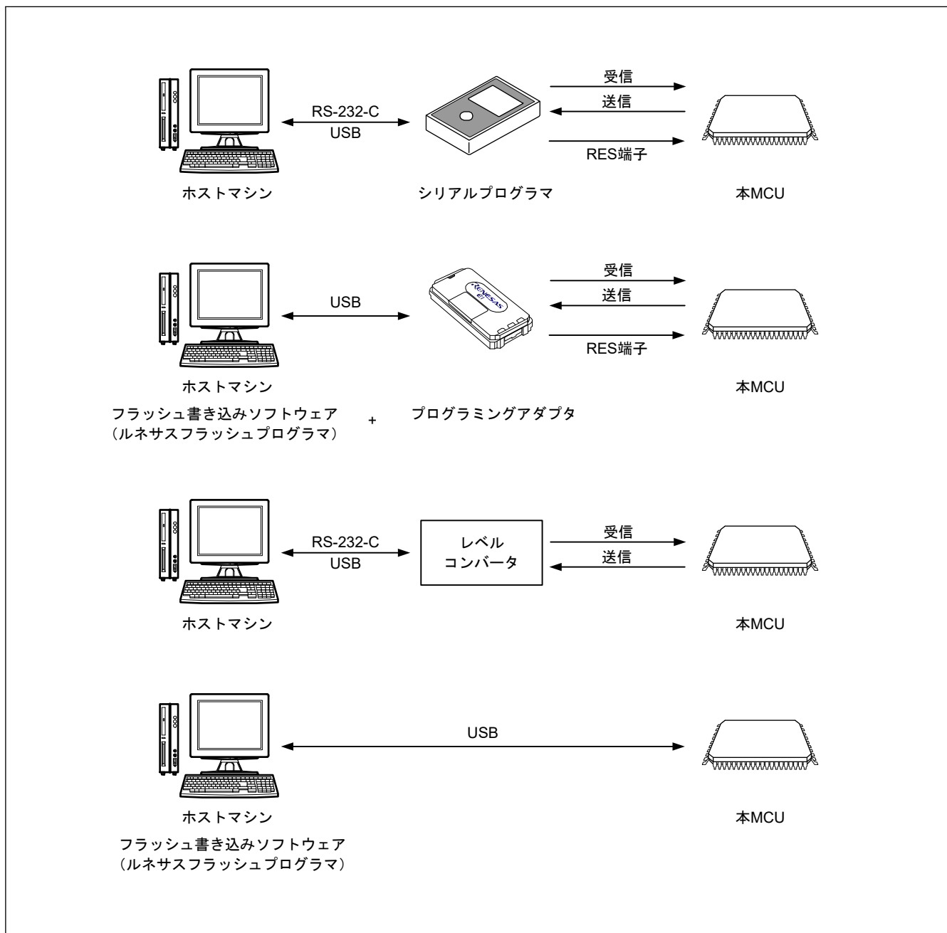
図 44.42 フラッシュメモリを書き換えるための環境
