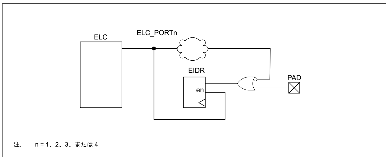
図 19.2 イベントポート入力データ
