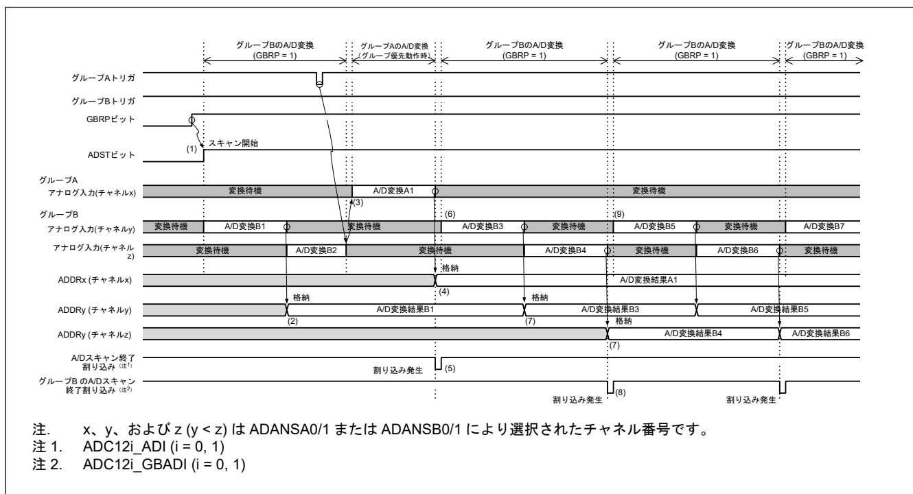
図 37.23 グループ優先動作の例 1-5 : グループ B のシングルスキャン連続動作 (ADGSPCR.GBRP = 1、ADGSPCR.LGRRS = 0 の場合)
