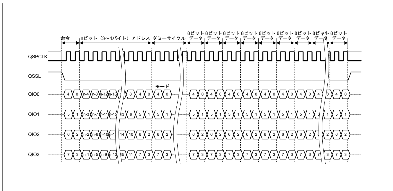
図 31.7 Quad-SPI プロトコル例 (ファストリード Quad I/O)
