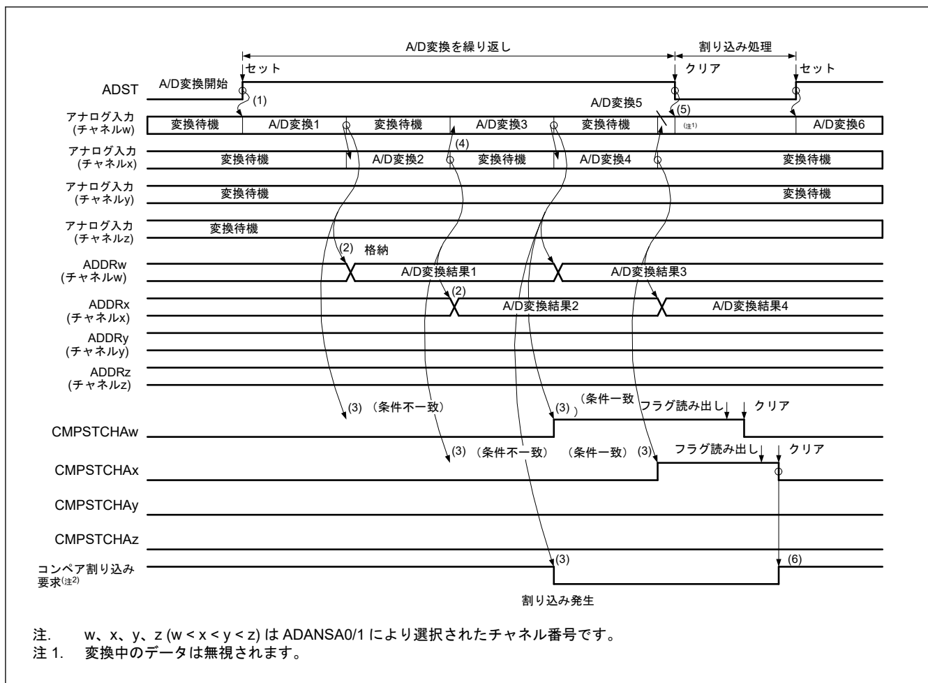
図 37.28 コンペア機能の動作例 (アナログ入力 (チャンネル w~z) を比較)
