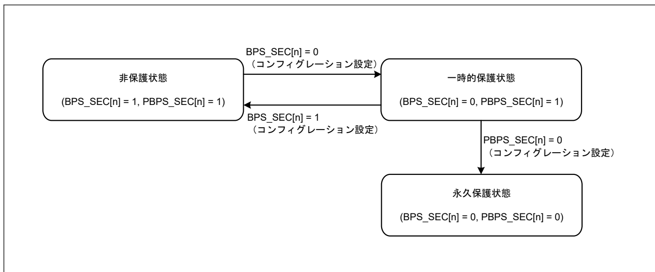
図 44.32 BPS_SEC[n]ビットおよび PBPS_SEC[n]ビットによるフラッシュシーケンサの状態遷移
