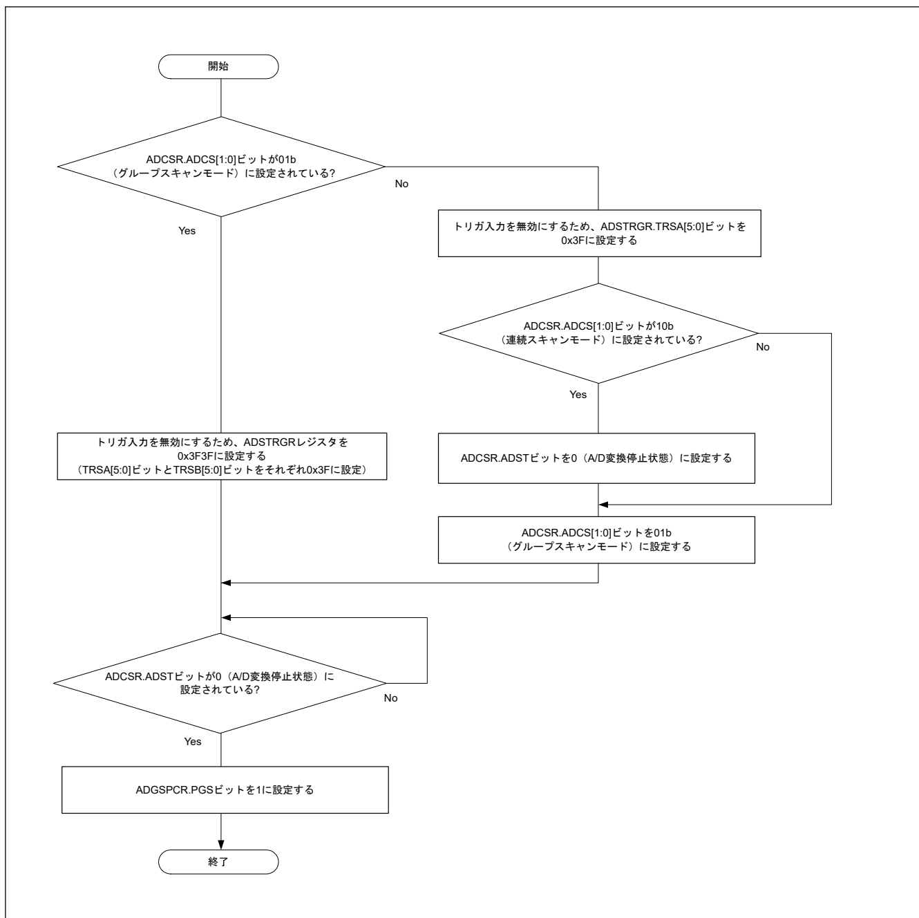
図 37.18 ADGSPCR.PGS ビット設定時のフローチャート
