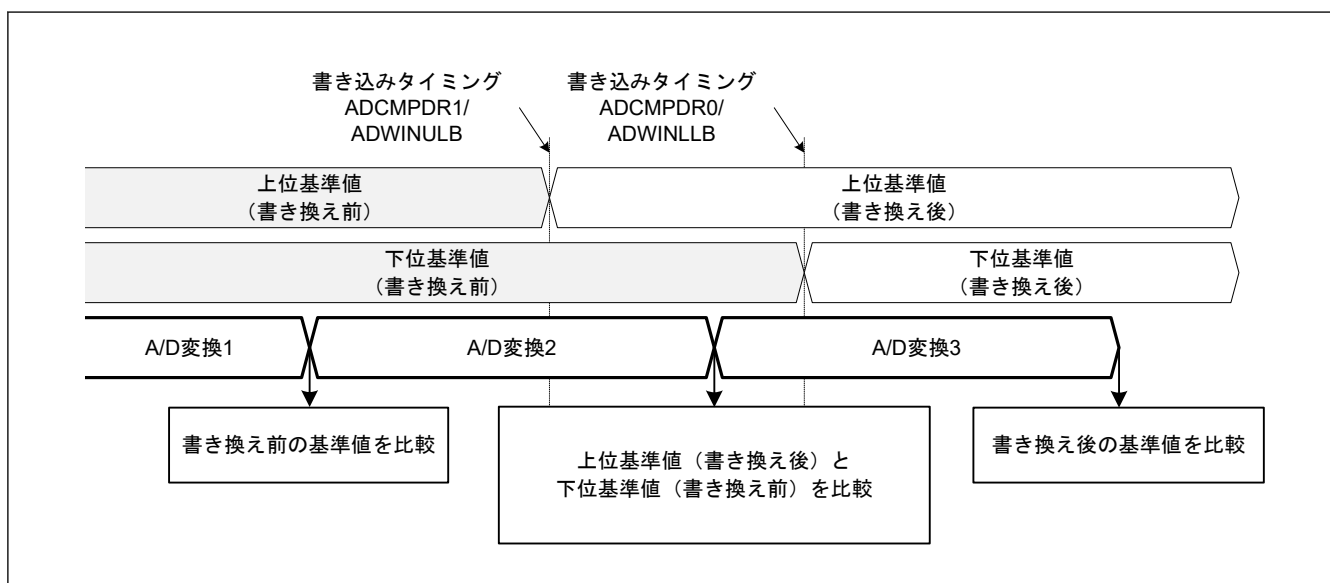
図 37.6 書き換え前後の上側基準値と下側基準値の比較
