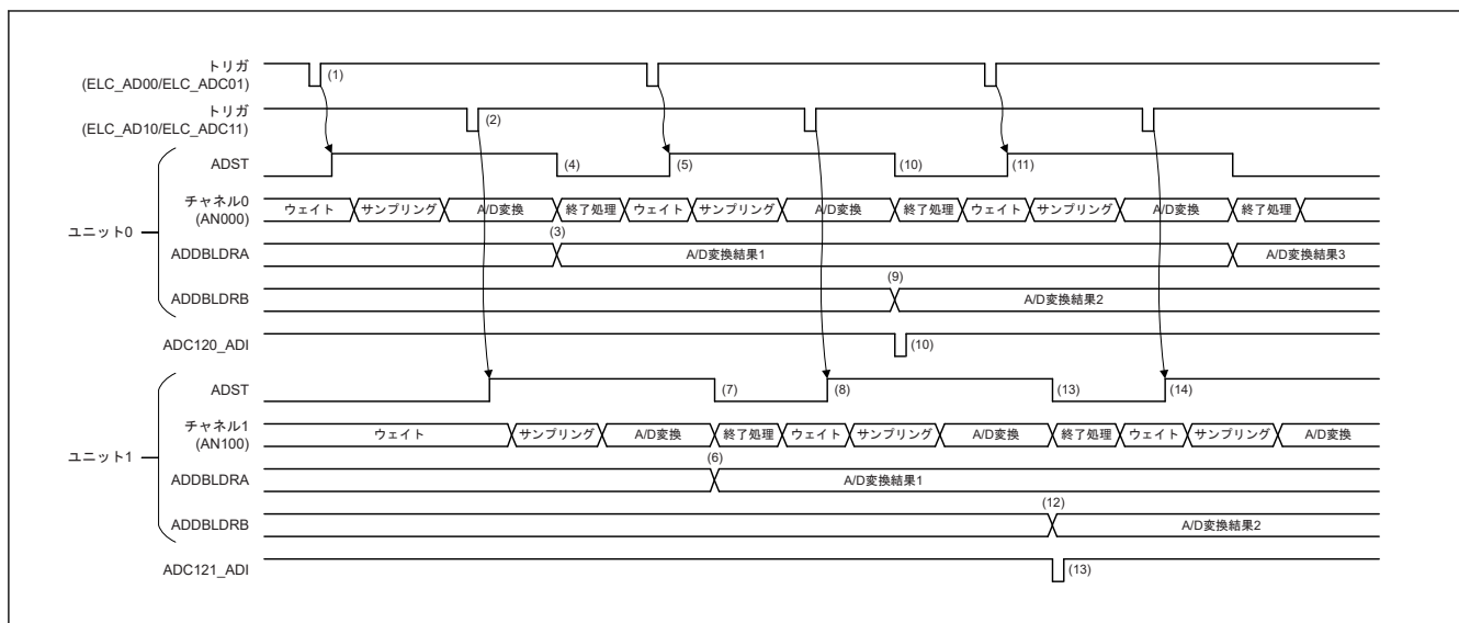
図 37.27 シングルスキャンモードの動作例（ダブルトリガ拡張モード選択、AN000 および AN100 選択、インターリーブ動作）
