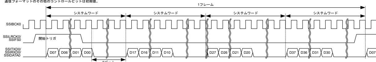
図 32.42 TDM フォーマット（パディングあり、システムワード長 > データワード長）
