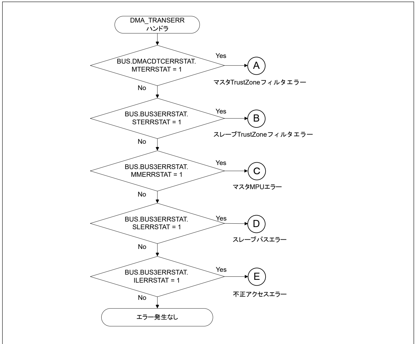
図 16.27 エラー応答検出割り込み (DMA_TRANSERR) 発生時の転送エラー要因判定
