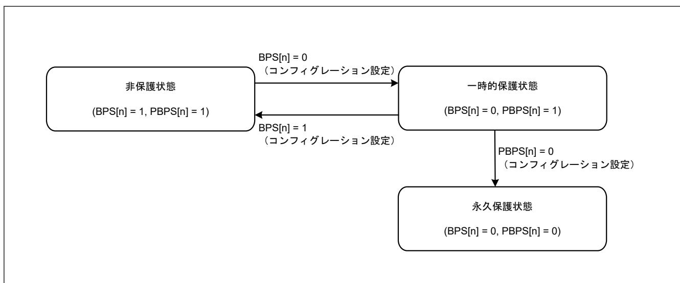
図 44.31 BPS[n]ビットおよび PBPS[n]ビットによるフラッシュシーケンサの状態遷移
