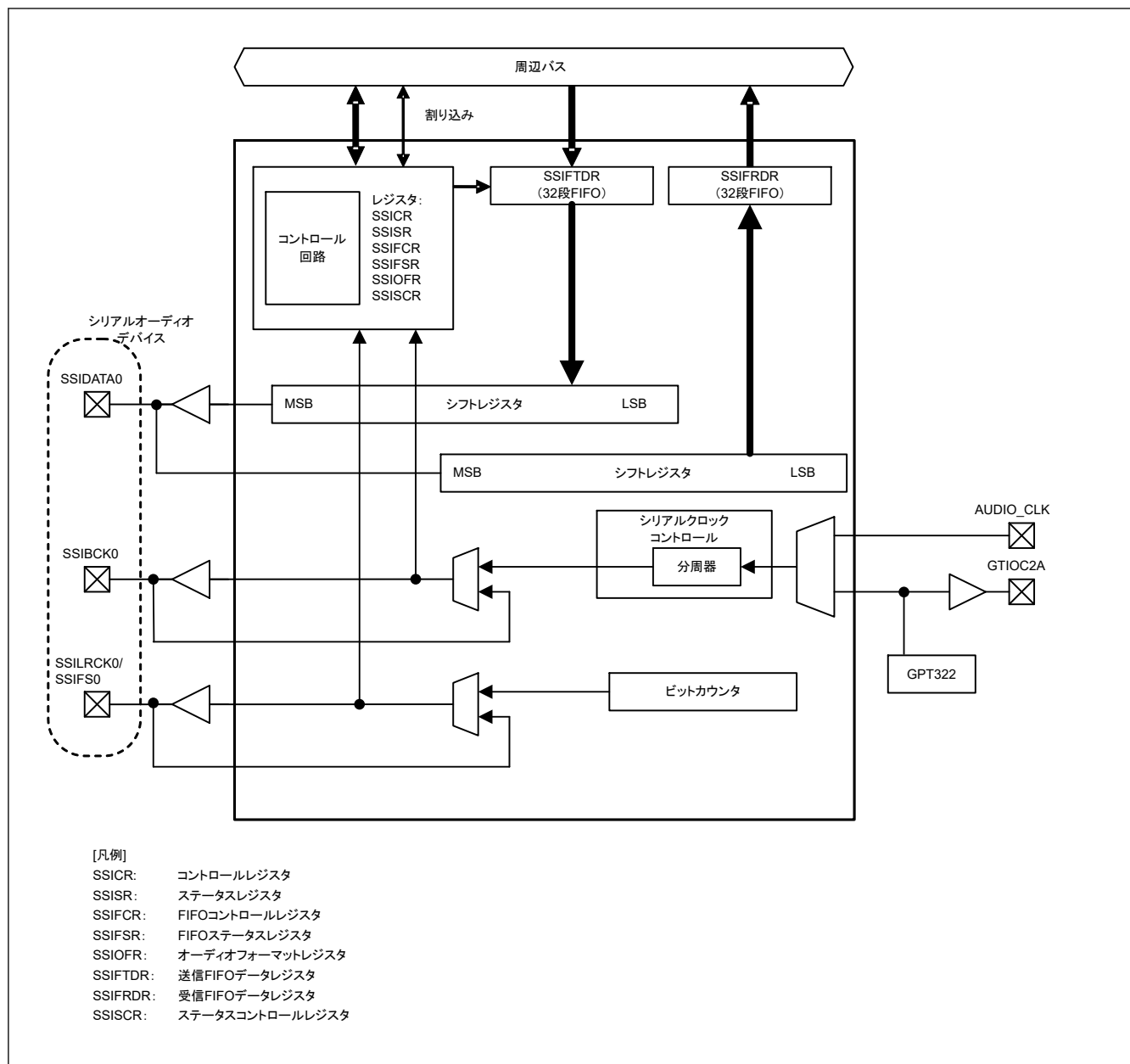
図 32.3 半二重通信の SSIE ブロック図
