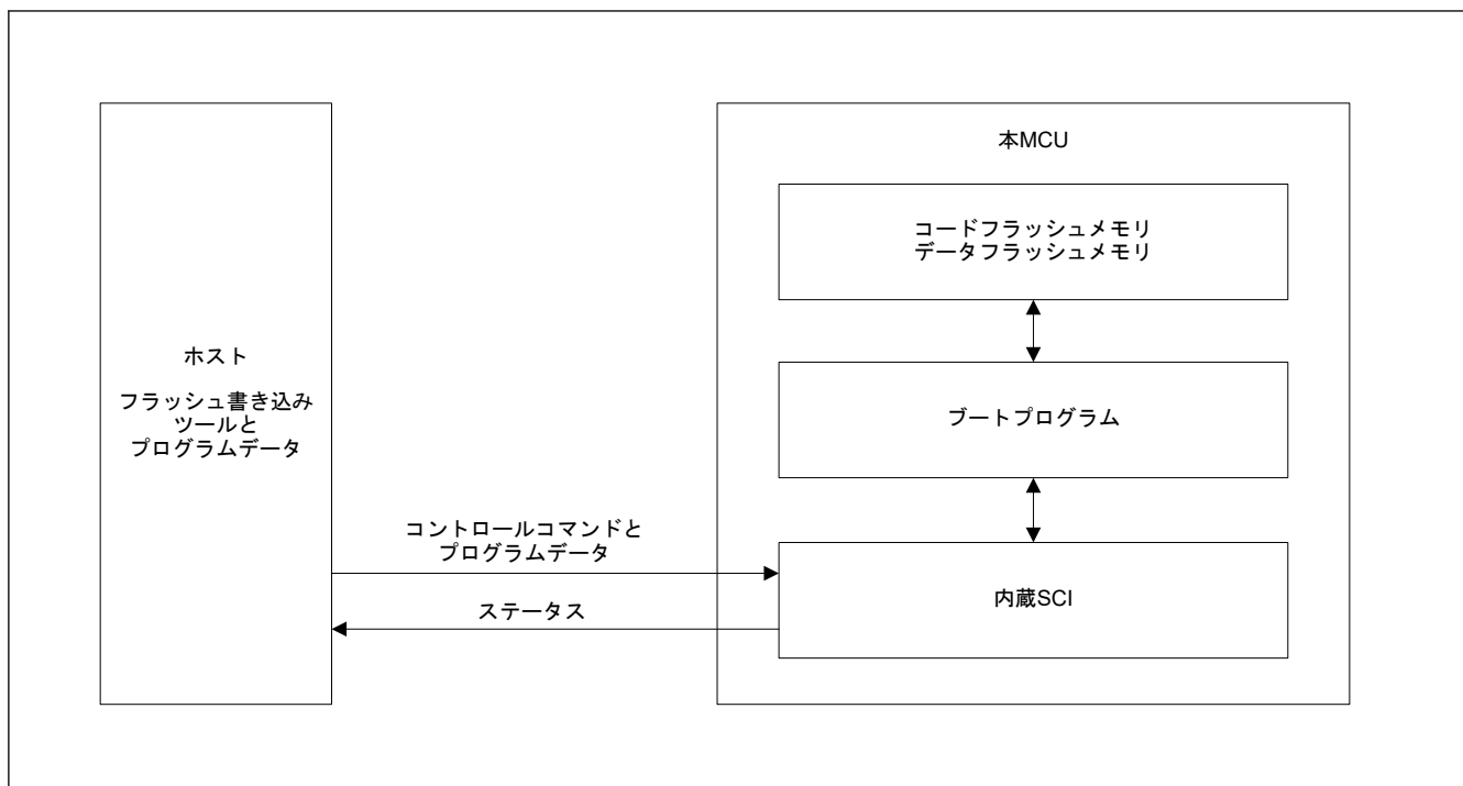
図 44.40 ブートモード（SCI インタフェース）時のシステム構成
