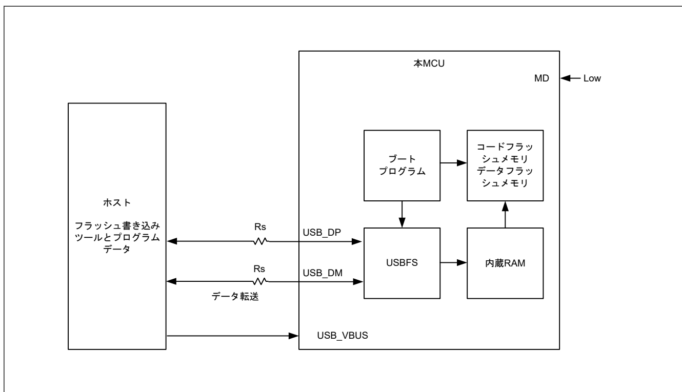
図 44.41 ブートモード（USB インタフェース）のシステム構成図
