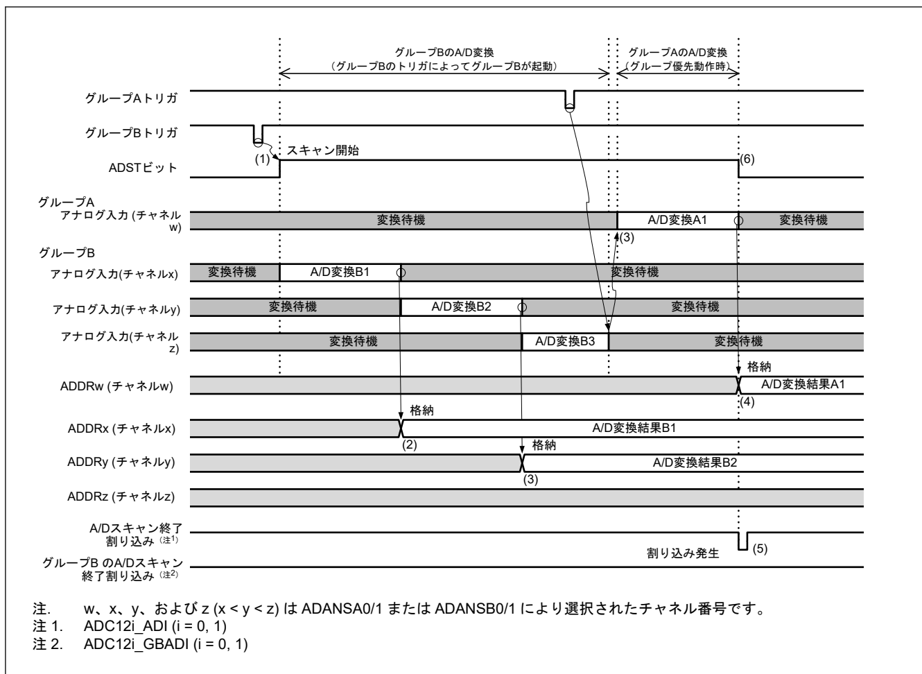
図 37.22 グループ優先動作の例 1-4 : グループ B スキャン中のグループ A トリガ入力、再スキャンなし (ADGSPCR.GBRSCN = 0、ADGSPCR.GBRP = 0、および ADGSPCR.LGRRS = 0 の場合)
