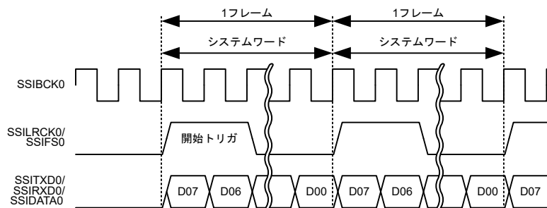
図 32.40 モノラルフォーマットにおけるロングフレーム（パディングなし）
