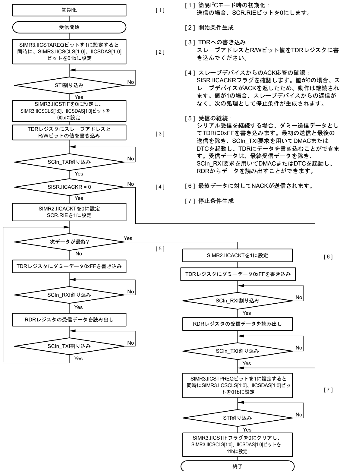
図 27.97 簡易 IIC モードにおけるマスタ受信のフローチャート例（送信割り込み、受信割り込み使用時）
