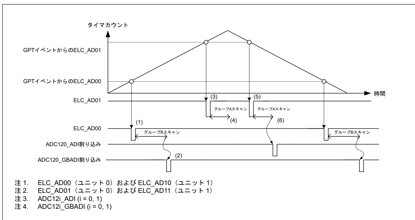
図 37.17 グループスキャンモードでダブルトリガモードを使用する場合の基本動作例 (ELC からの同期トリガ使用時)
