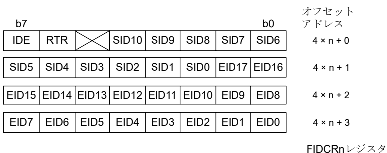
図 29.15 FIDCRn レジスタの構成 ( n = 0, 1 )
