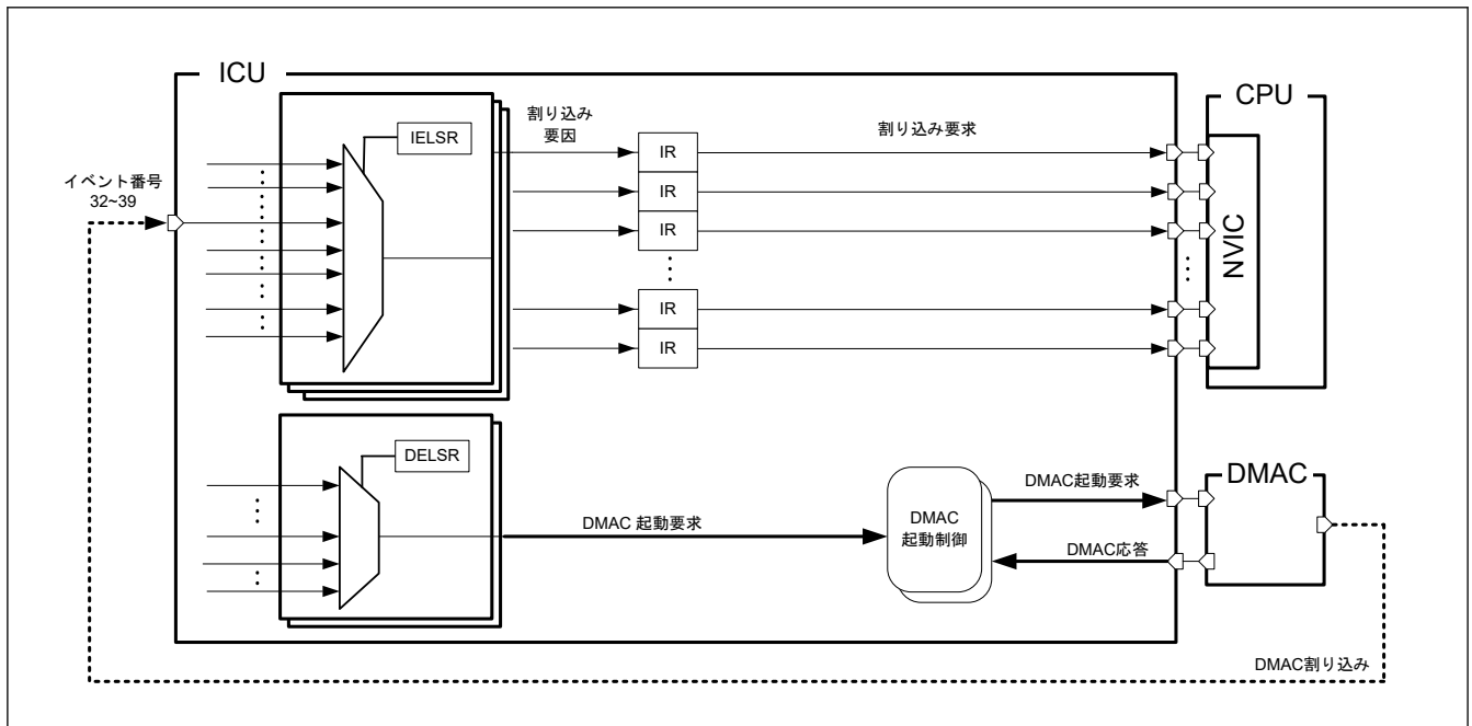
図 13.3 DMAC 要求トリガと割り込み経路
