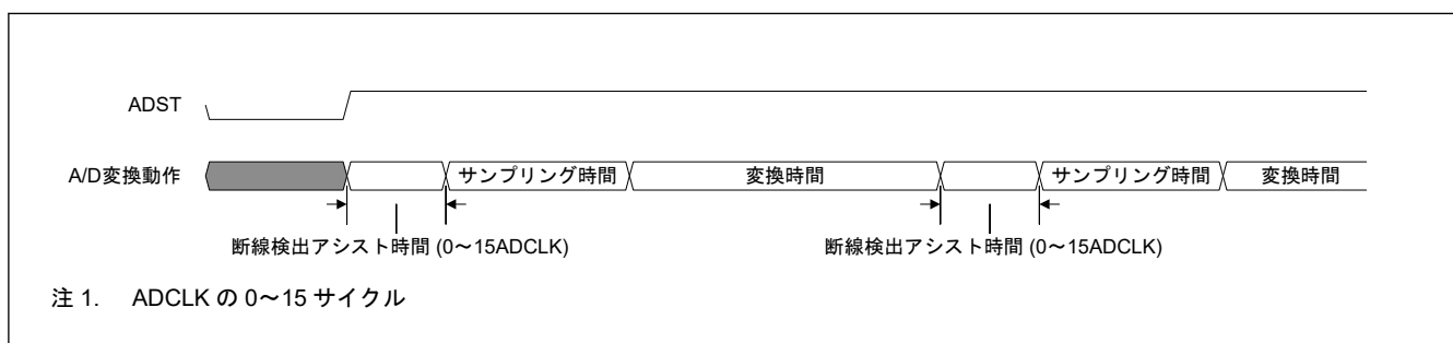
図 37.33 断線検出アシスト機能を使用した場合の A/D 変換動作図
