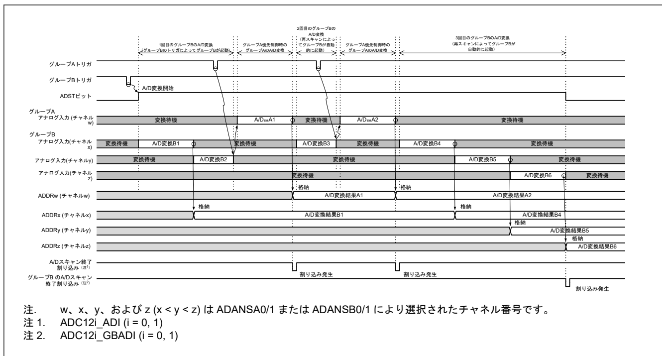
図 37.20 グループ優先動作の例 1-2: グループ B 再スキャン中のグループ A トリガ入力、再スキャンあり (ADGSPCR.GBRSCN = 1、ADGSPCR.GBRP = 0、および ADGSPCR.LGRRS = 0 の場合)
