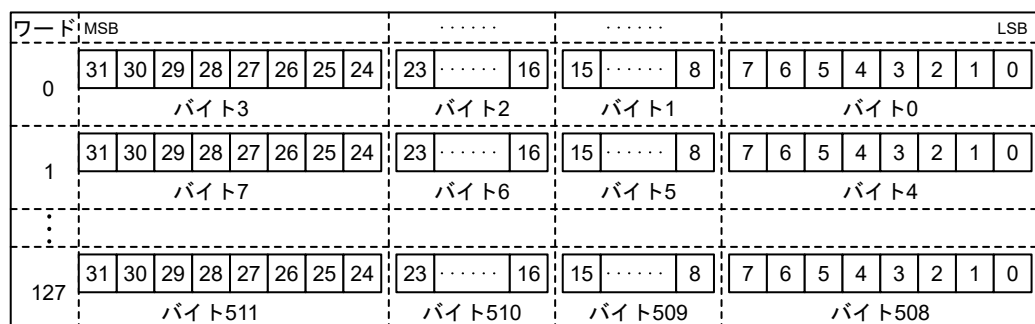
図 33.5 SD_BUF 格納データ
