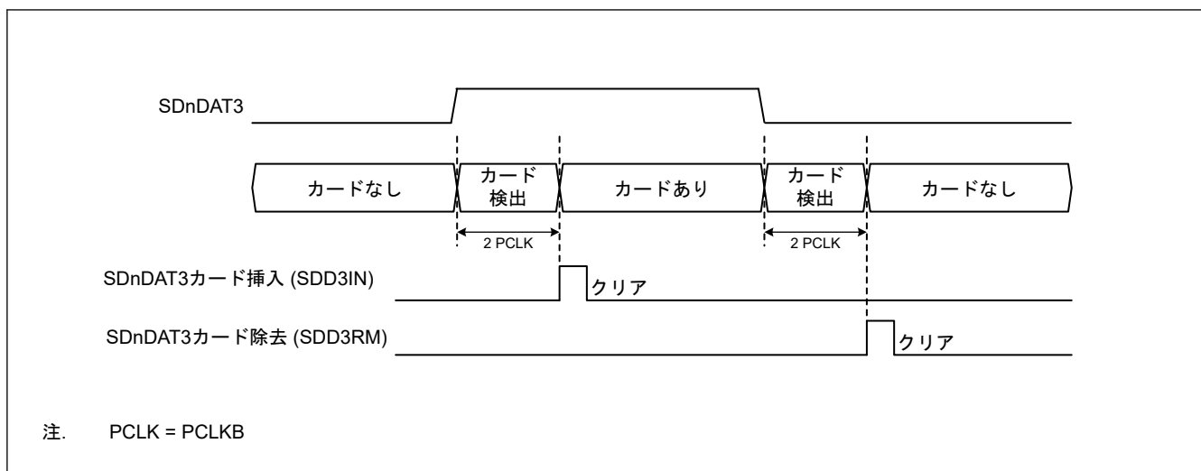
図 33.8 SDnDAT3 による SD カード検出
