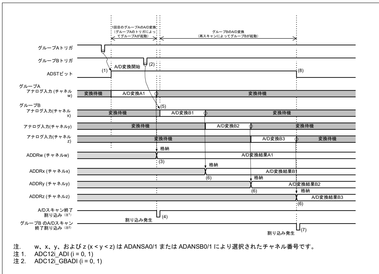
図 37.21 グループ優先動作の例 1-3: グループ A スキャン中のグループ B トリガ入力、再スキャンあり (ADGSPCR.GBRSCN = 1、ADGSPCR.GBRP = 0、および ADGSPCR.LGRRS = 0 の場合)
