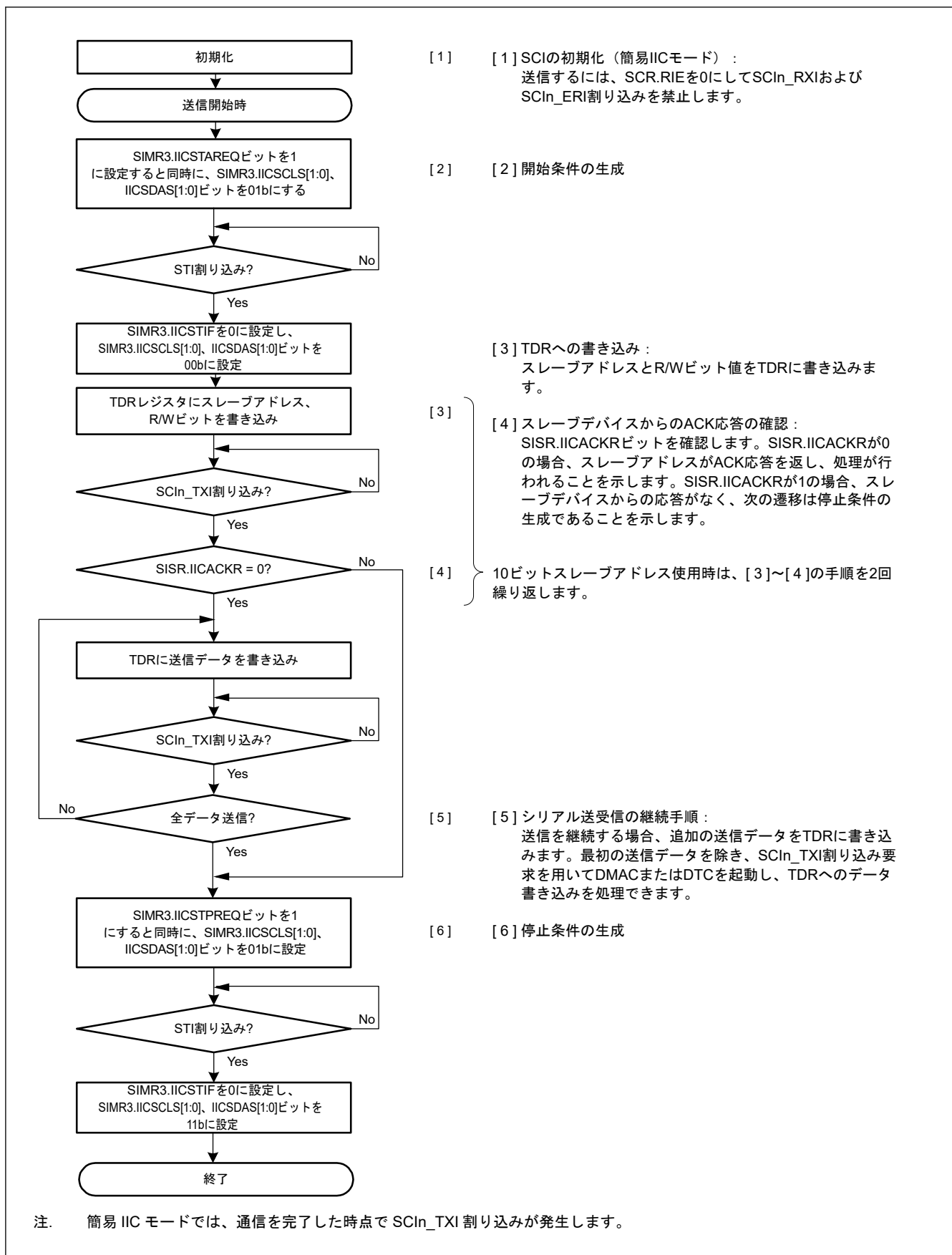
図 27.95 簡易 IIC モードにおけるマスタ送信のフローチャート例（送信割り込み、受信割り込み使用時）
