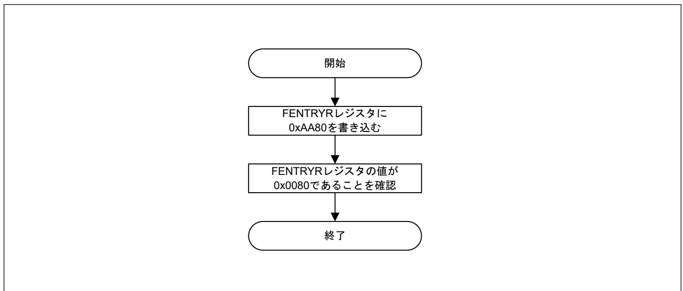
図 44.10 データフラッシュ P/E モードへの遷移手順
