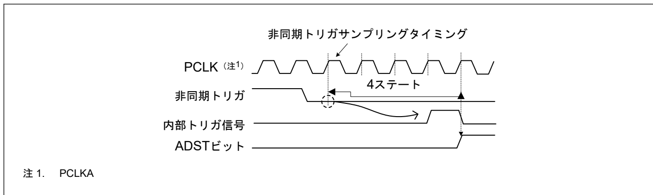
図 37.36 非同期トリガ入力タイミング
