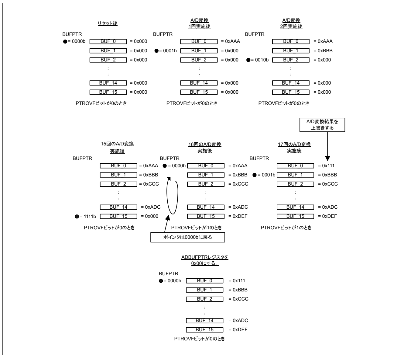
図 37.37 データバッファ、ポインタ、およびオーバーフローフラグの動作概略図
