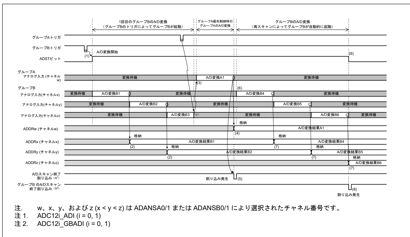
図 37.19 グループ優先動作の例 1-1：グループ B スキャン中のグループ A トリガ入力、再スキャンあり (ADGSPCR.GBRSCN = 1、ADGSPCR.GBRP = 0、および ADGSPCR.LGRRS = 0 の場合)
