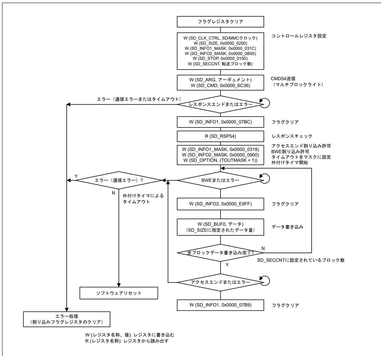
図 33.15 外付けタイマによるマルチブロックライト動作の例
