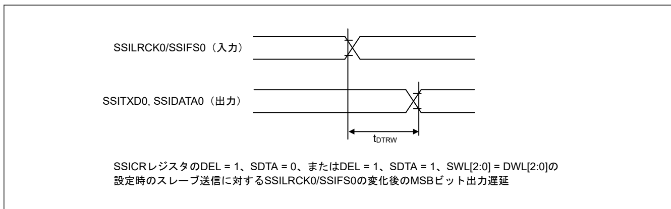
図 47.48 SSILRCK0/SSIFS0 変化時からの SSIE データ出力遅延
