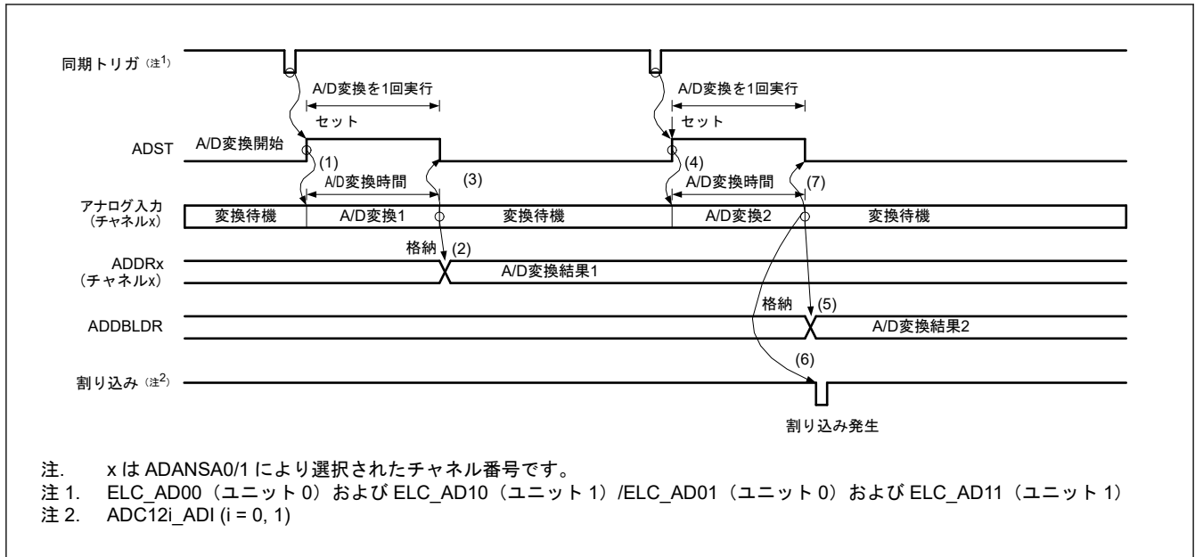
図 37.11 シングルスキャンモードの動作例 (ダブルトリガモード選択、アナログ入力 (チャネル x) を 2 重化)
