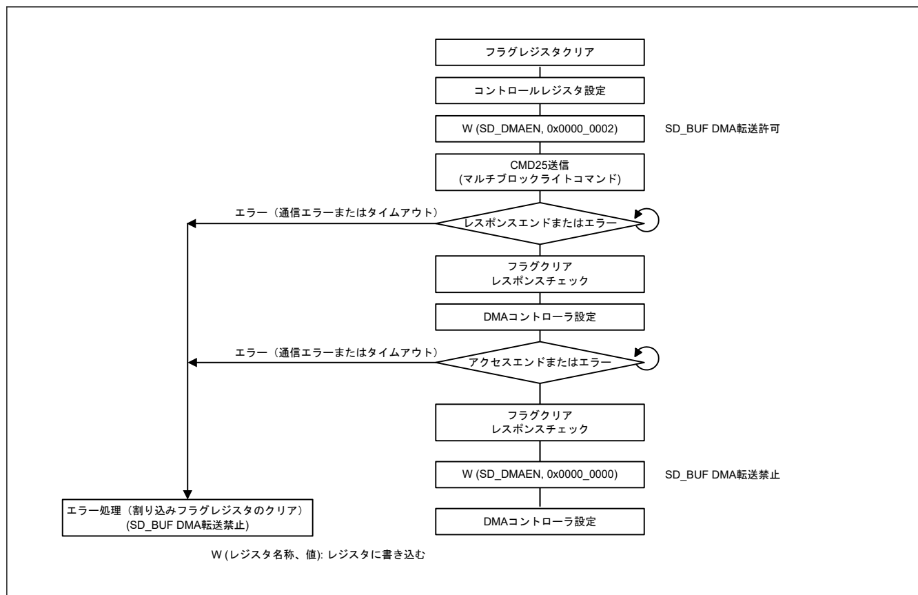
図 33.24 SD_BUF_DMA ライト動作の例
