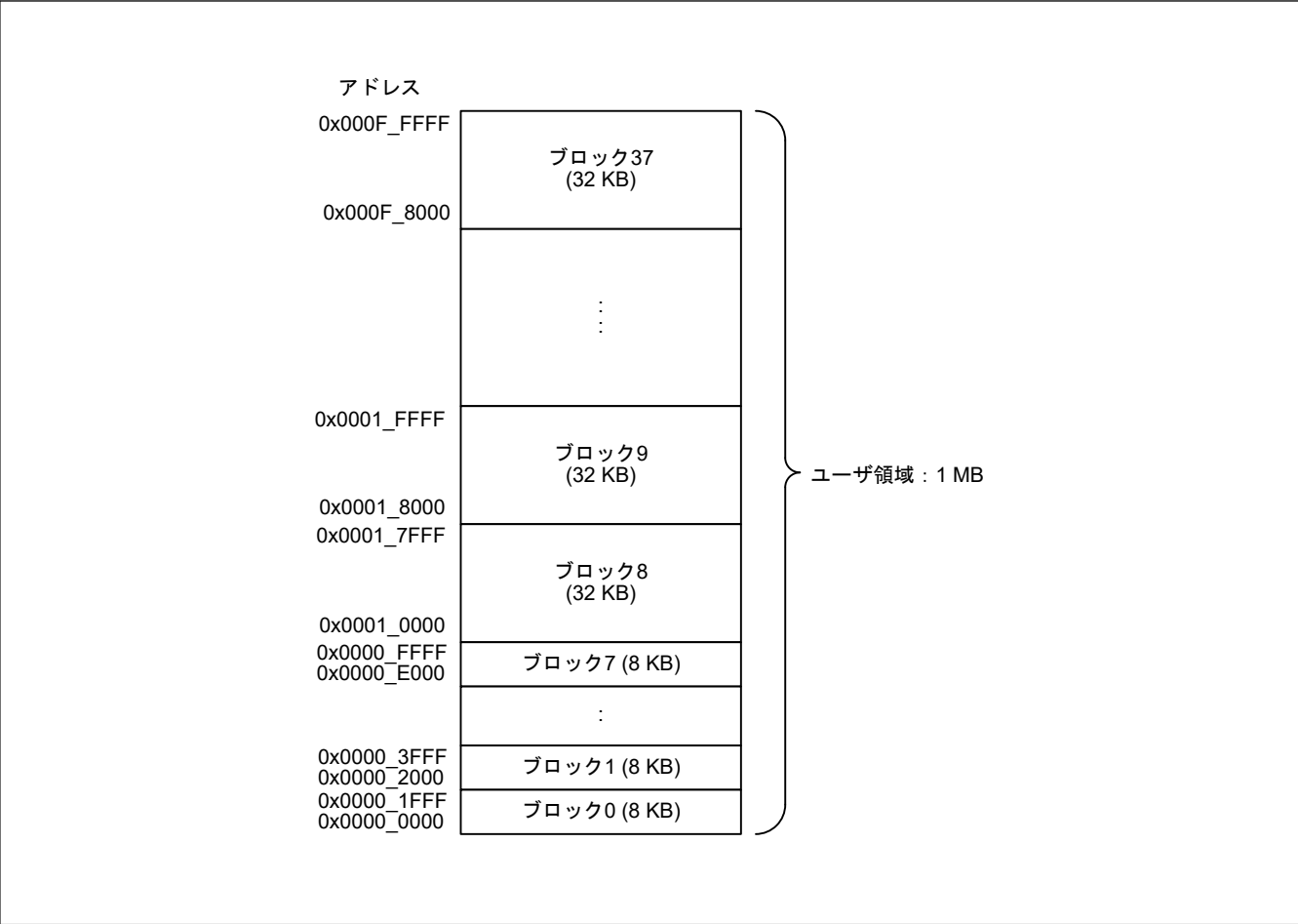
図 44.2 コードフラッシュメモリのマップ
