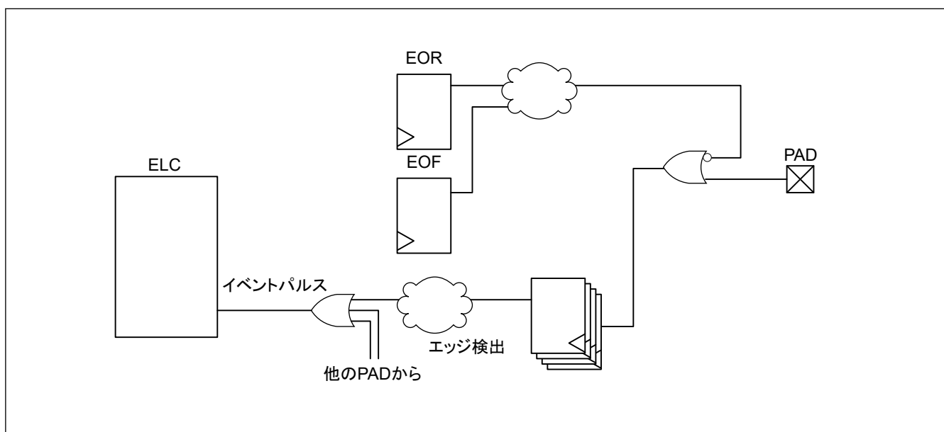
図 19.4 イベントパルスの発生
