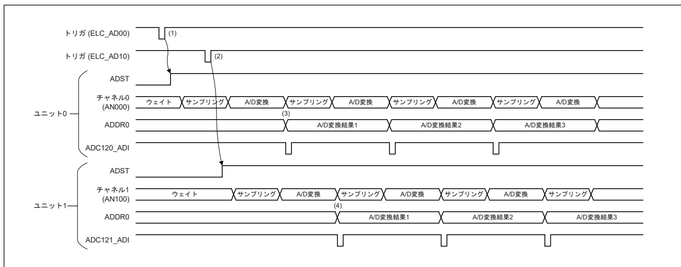
図 37.25 連続スキャンモードの動作例 (AN000 および AN100 選択、インターリーブ動作)
