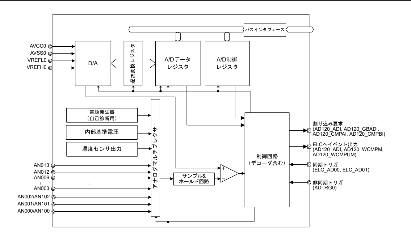
図 37.1 ADC12 のブロック図 (ユニット 0)
