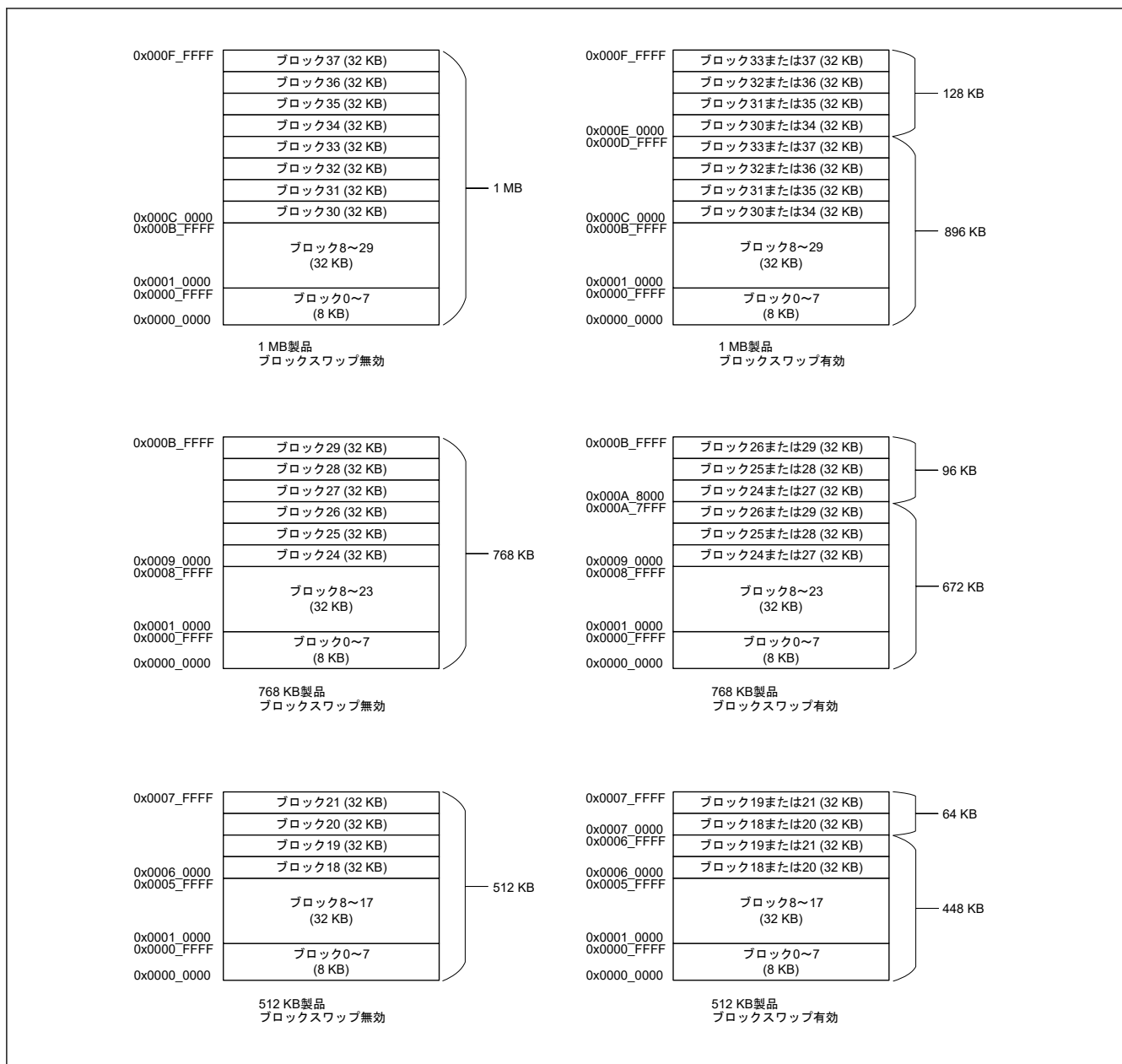
図 6.2 フラッシュメモリのマッピング
