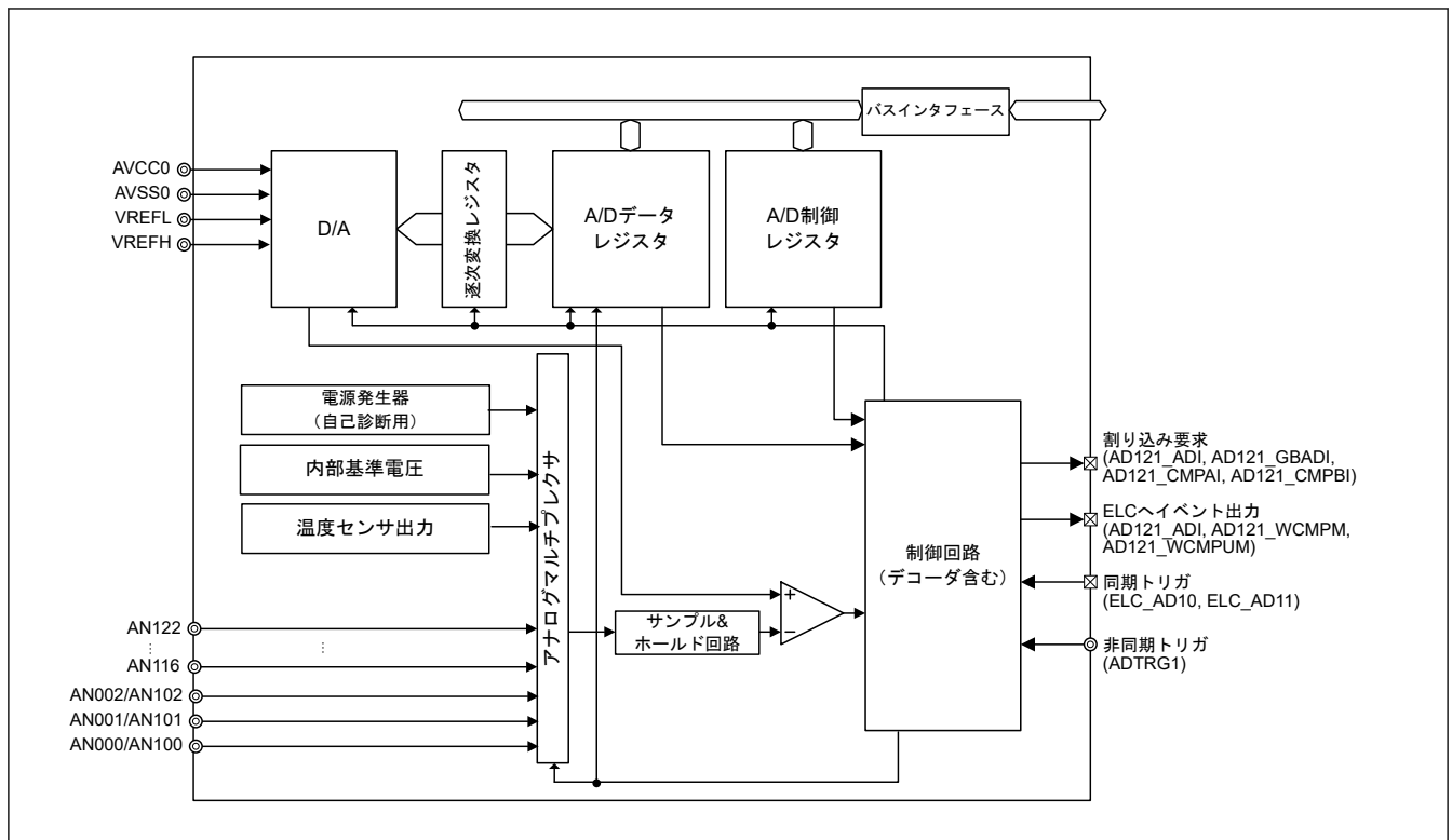
図 37.2 ADC12 のブロック図 (ユニット 1)
