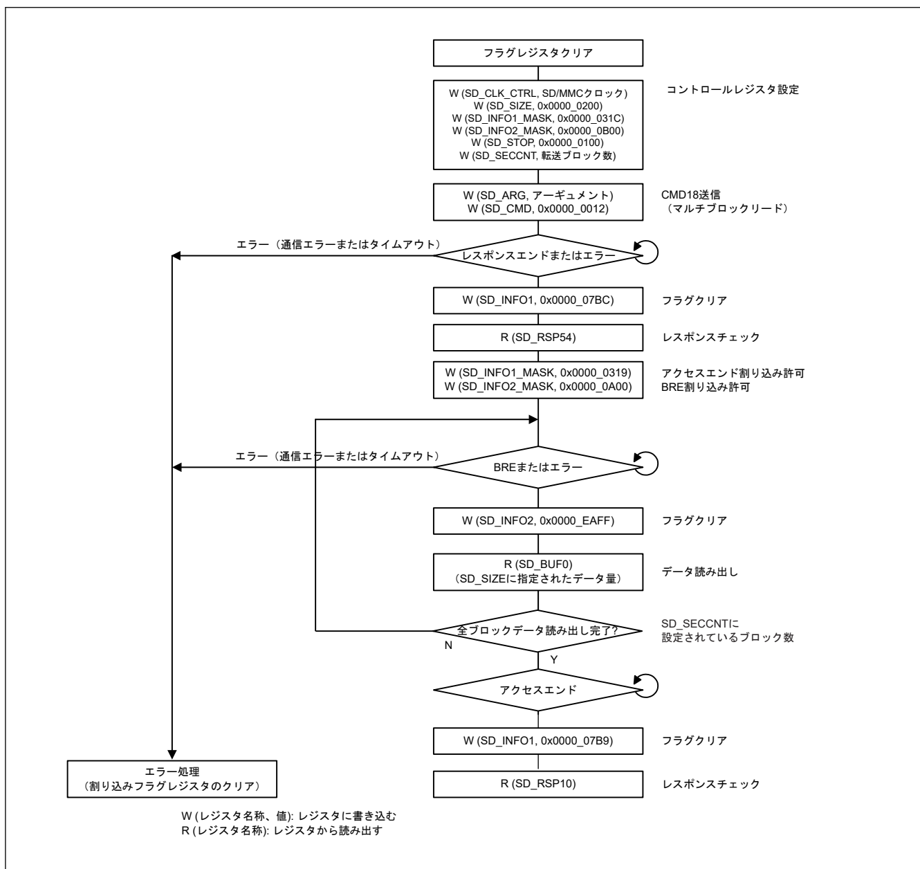
図 33.13 マルチブロックリード動作の例
