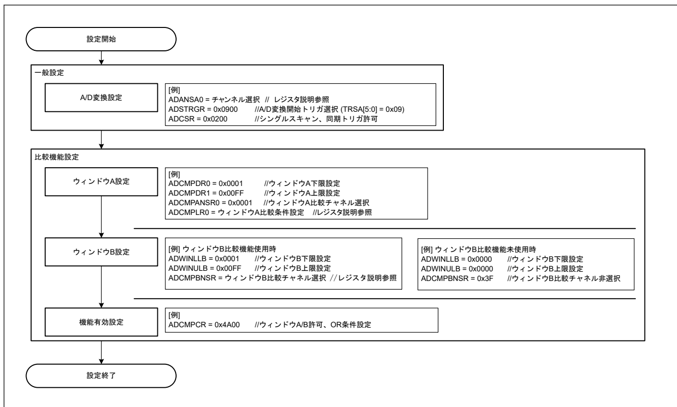
図 37.29 コンペア機能のイベント出力使用時の設定例
