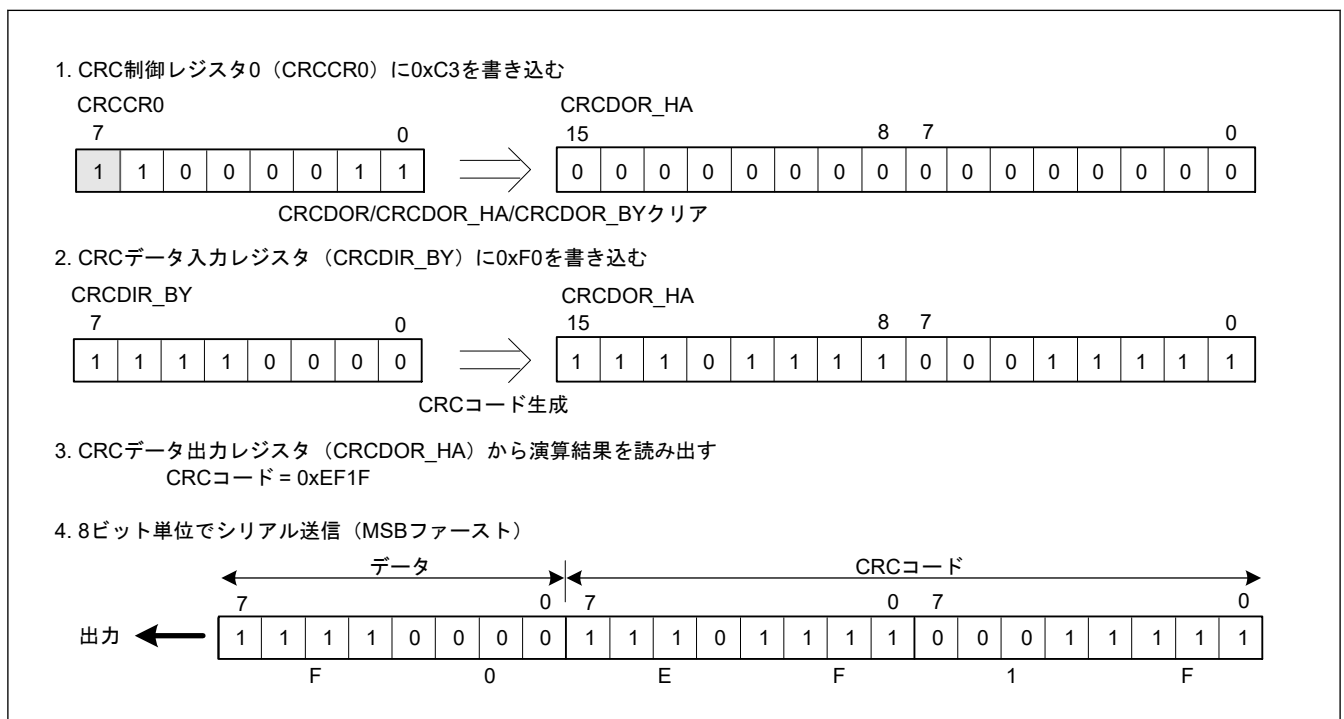
図 34.3 MSB ファーストのデータ送信
