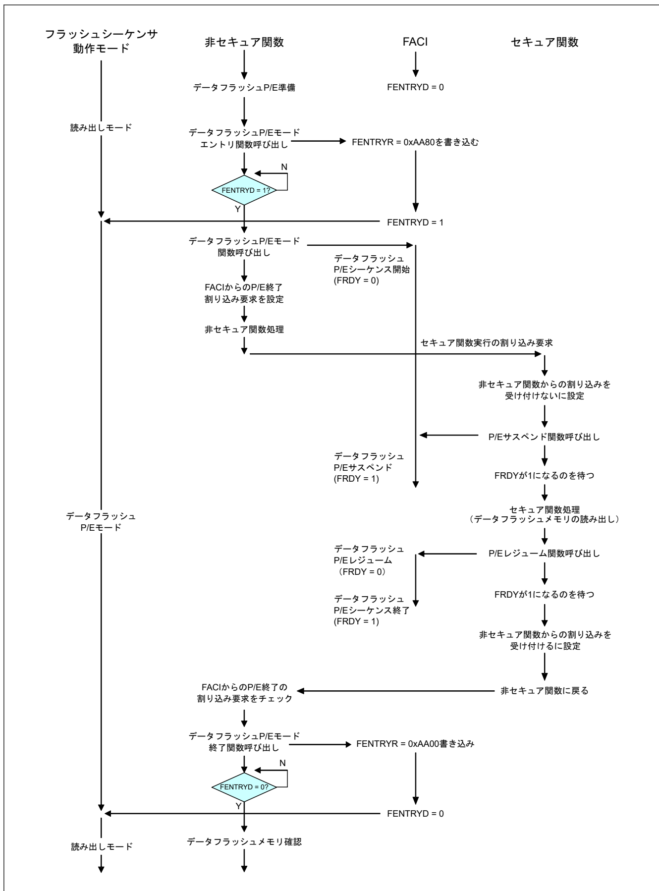
図 44.38 セキュア関数のデータフラッシュ P/E サスペンド例 (P/E 終了を検出するには割り込み要求を確認)
