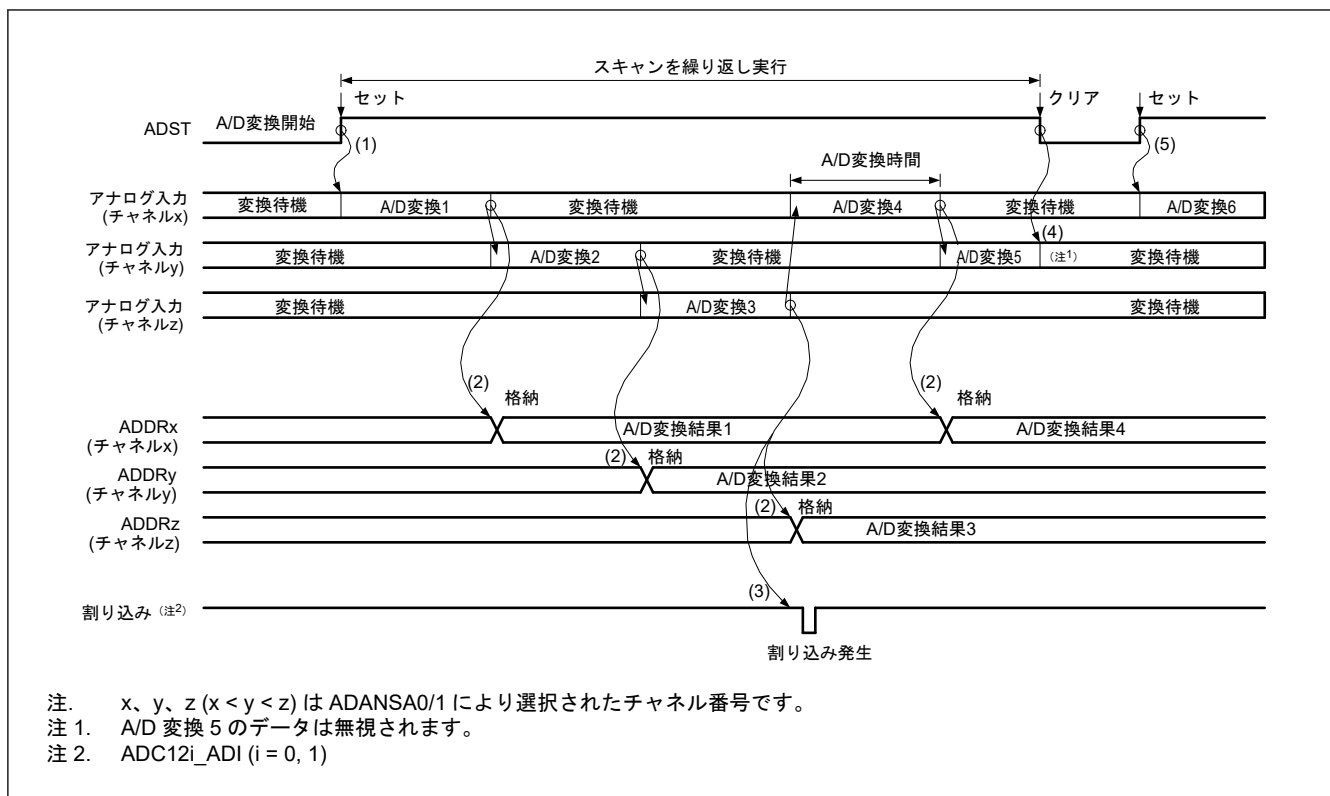
図 37.13 連続スキャンモードの基本動作例（アナログ入力（チャンネル x~z）選択）
