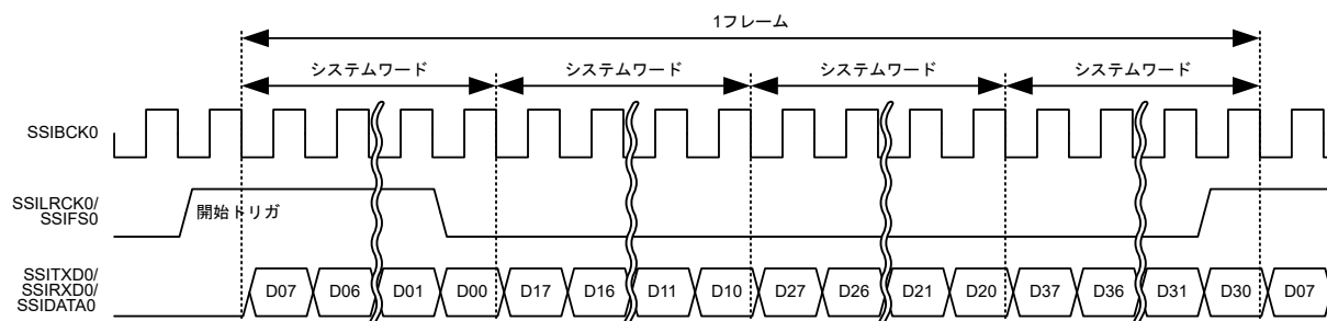
図 32.41 TDM フォーマット（パディングなし、システムワード長 = データワード長）
