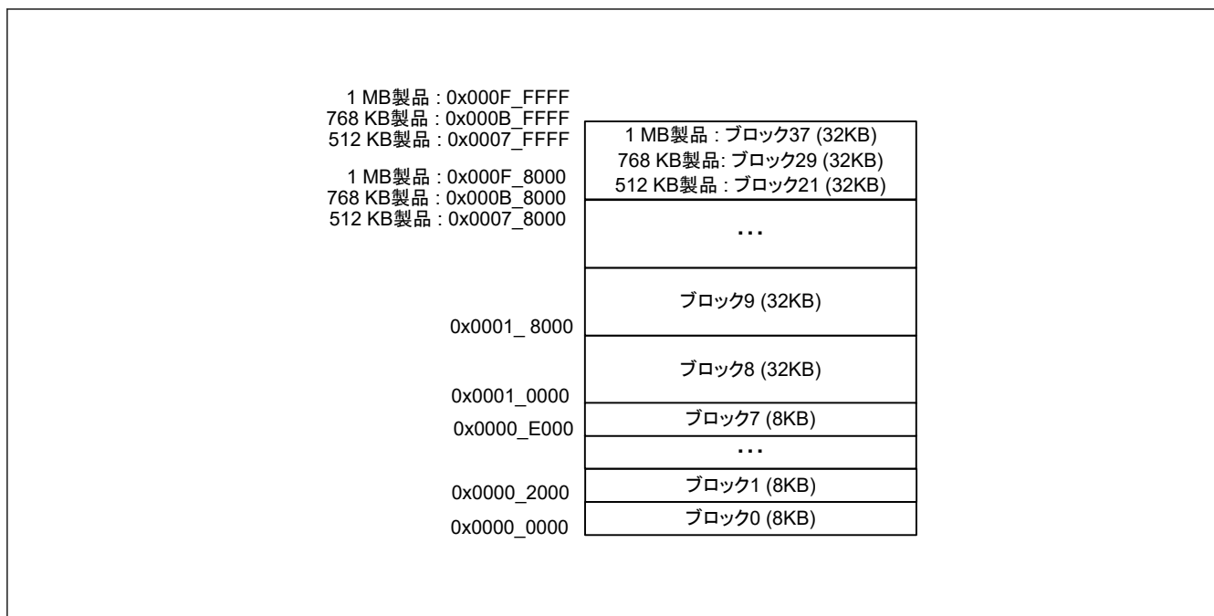
図 6.3 コードフラッシュのブロック構成
