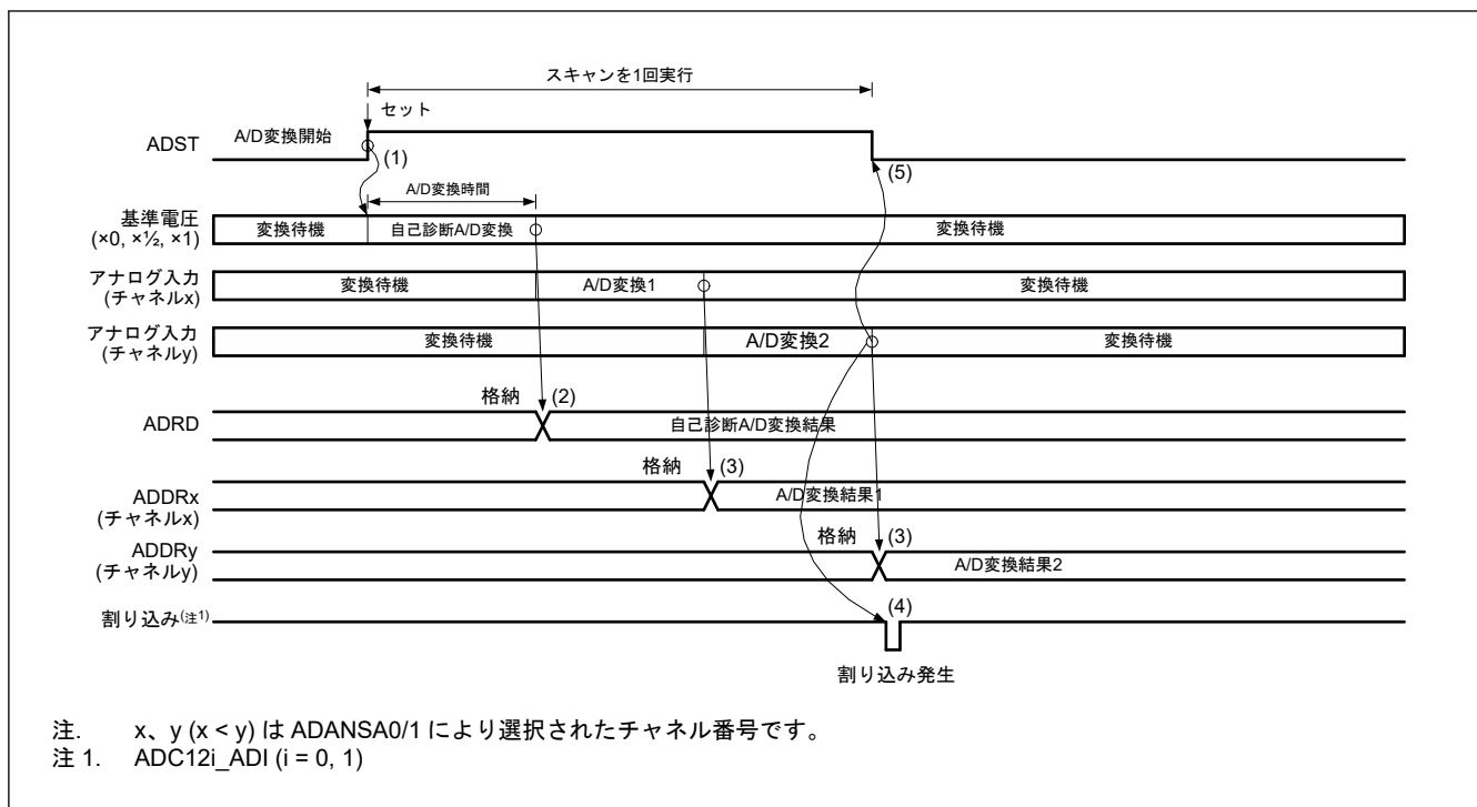
図 37.9 シングルスキャンモードの基本動作例（アナログ入力（チャンネル x、y）選択+自己診断）
