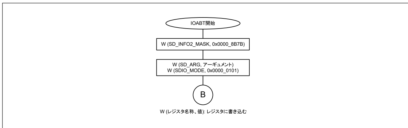
図 33.21 CMD53 マルチブロックライト時に CMD52 (SDIO abort) が送信される場合のフロー
