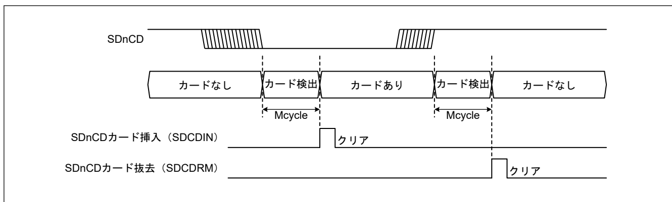
図 33.7 SDnCD によるカード検出例
