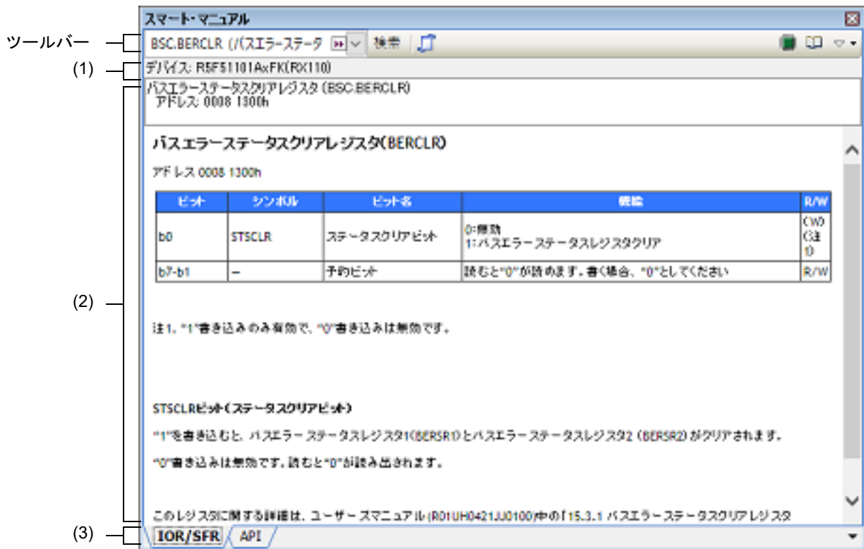
図 A.19 スマート・マニュアルパネル【RX】
