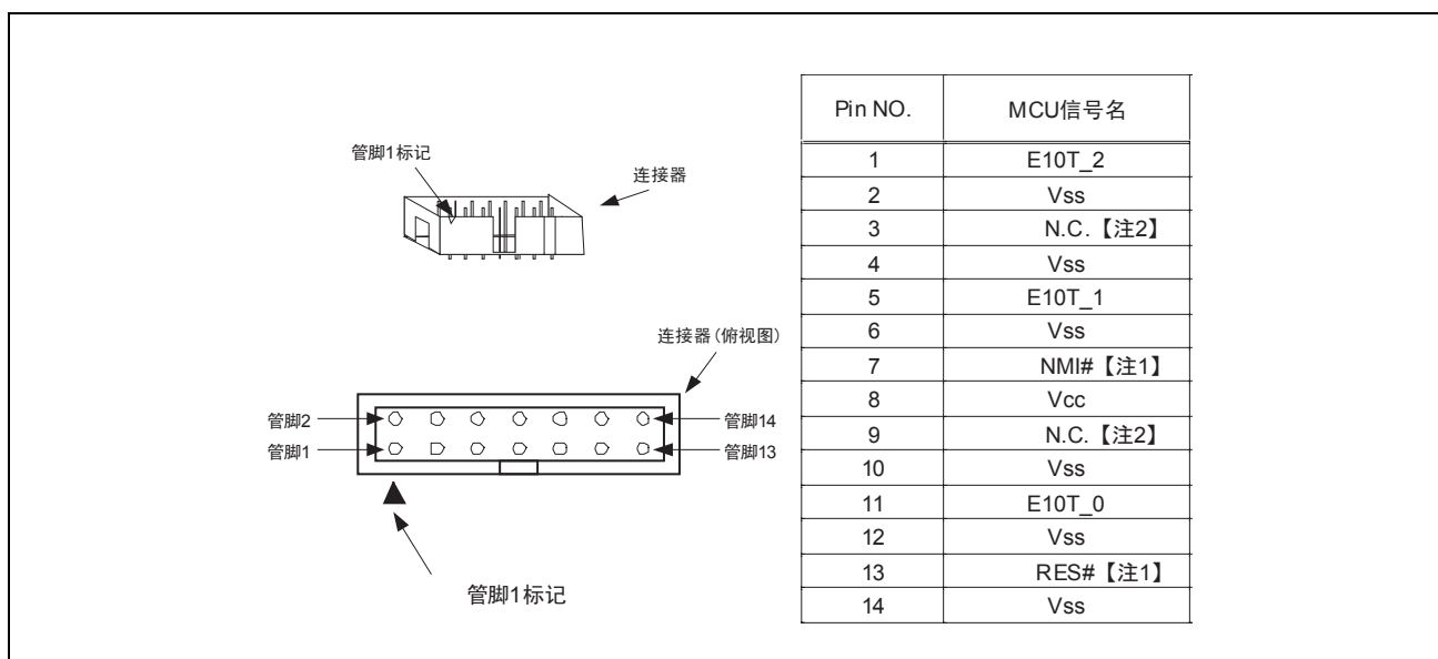
图 2.1 E8 连接器的管脚配置
