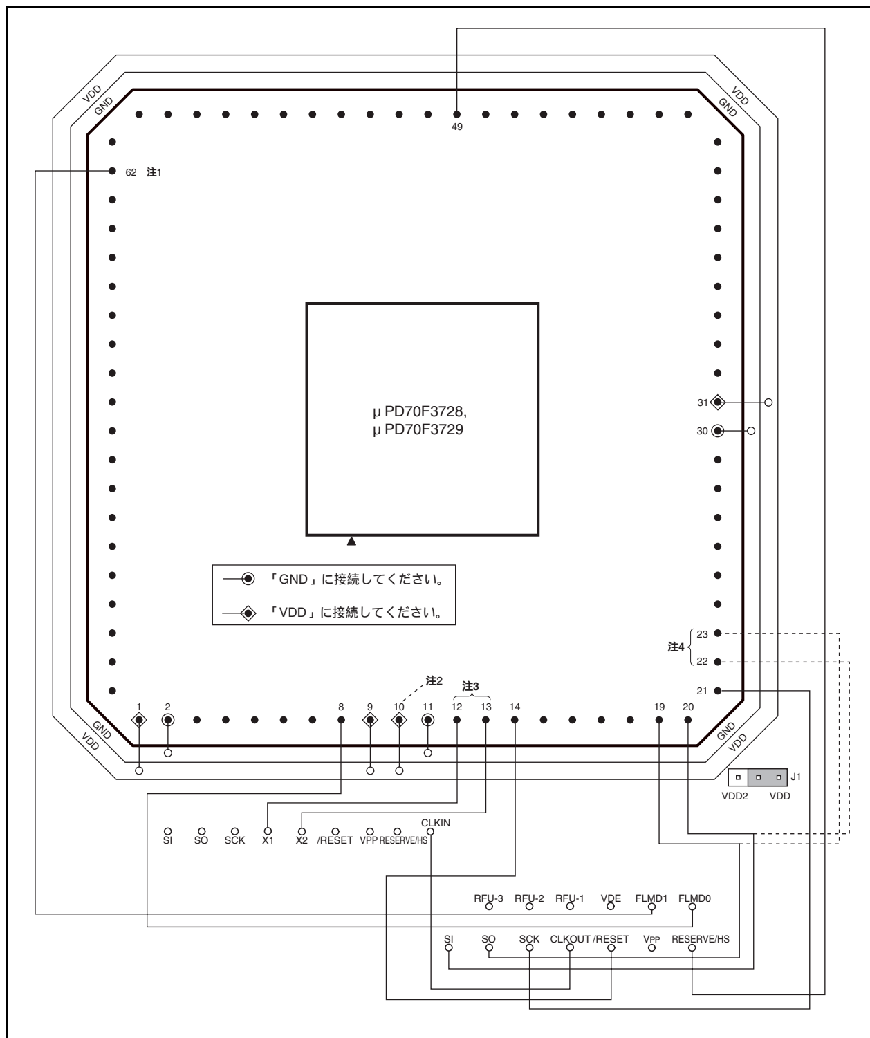
図24 - 6 V850ES/KF2フラッシュ書き込み用アダプタ (FA-80GC-8BT-A) の配線例 (1/2)
