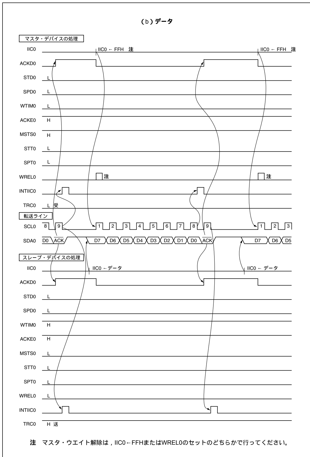
図18 - 21 スレーブ→マスタ通信例（マスタ：8クロック，スレーブ：9クロックでウェイト選択時）（2/3）
