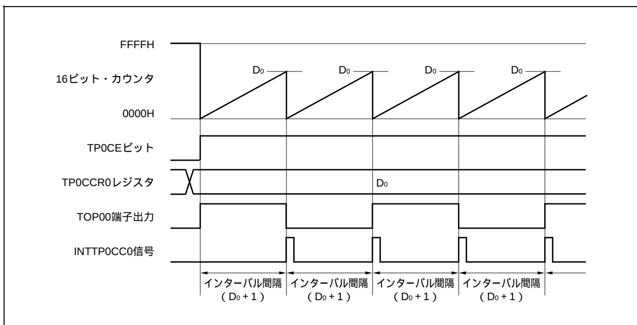
図7-3 インターバル・タイマ・モード動作の基本タイミング
