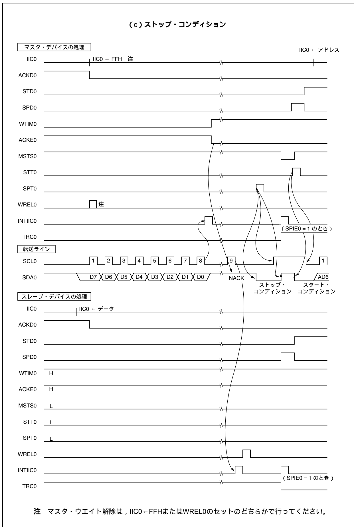
図18 - 21 スレーブ→マスタ通信例（マスタ：8→9クロック，スレーブ：9クロックでウェイト選択時）（3/3）
