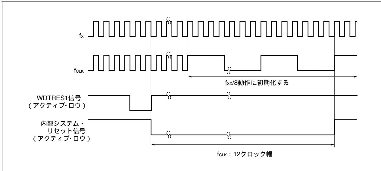
図22 - 5 ウォッチドッグ・タイマ2によるリセット動作のタイミング
