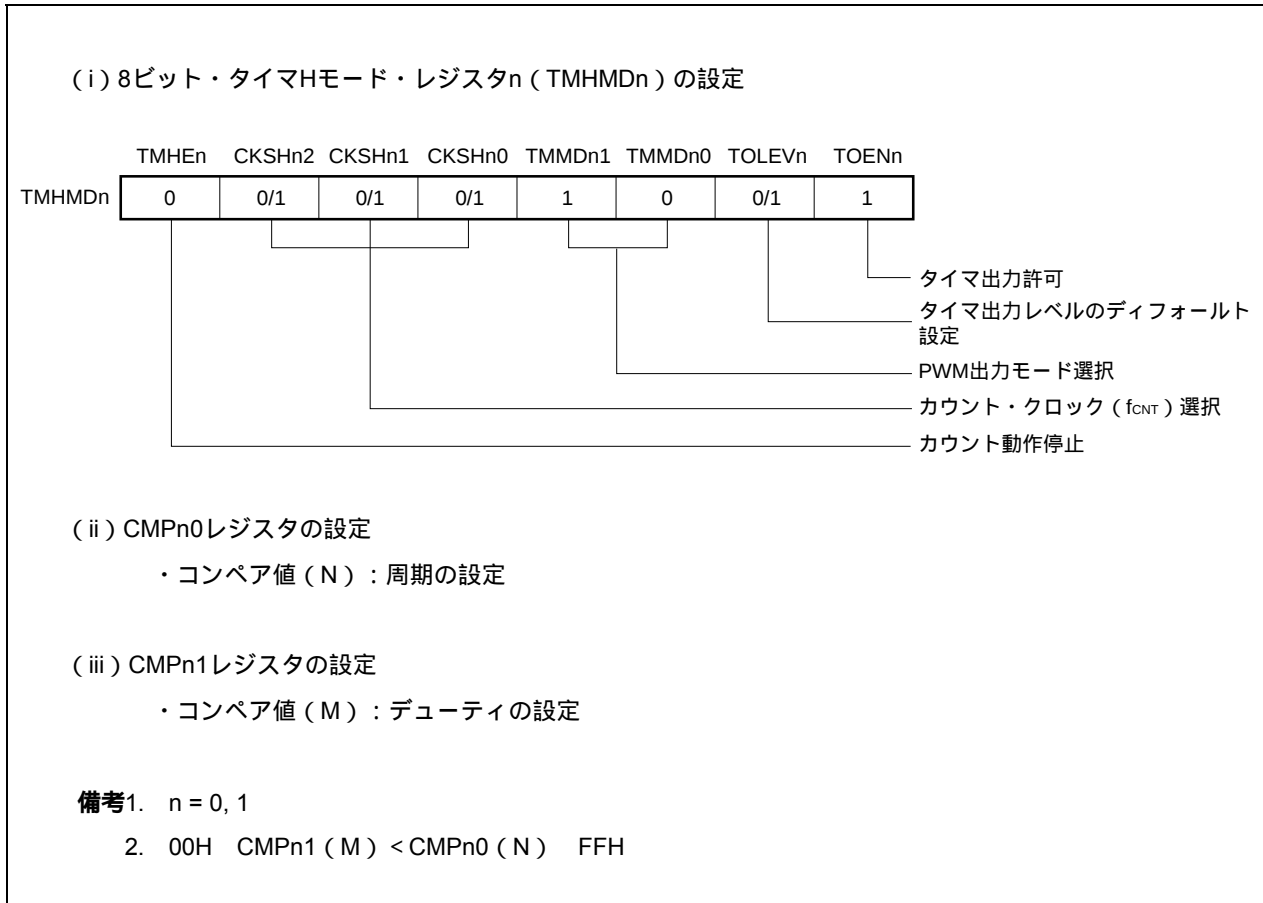
図10 - 4 PWM出力モード時のレジスタの設定
