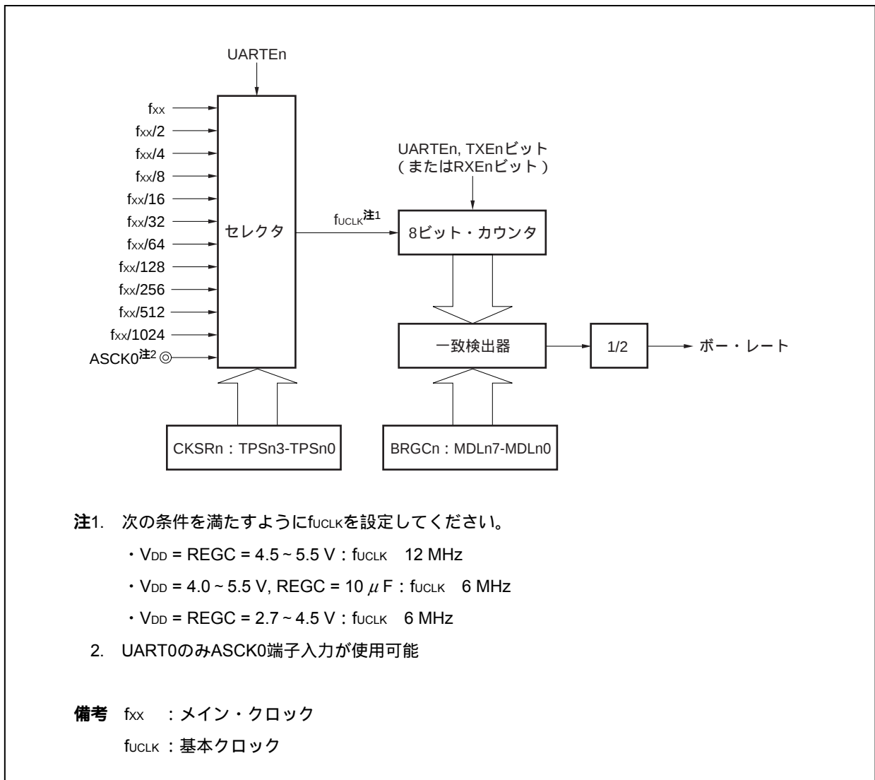
図15 - 12 ボー・レート・ジェネレータ n (BRG n ) の構成
