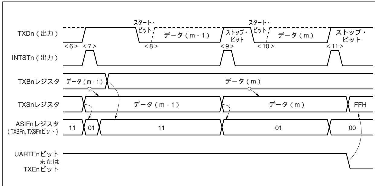
図15 - 6 連続送信の終了手順
