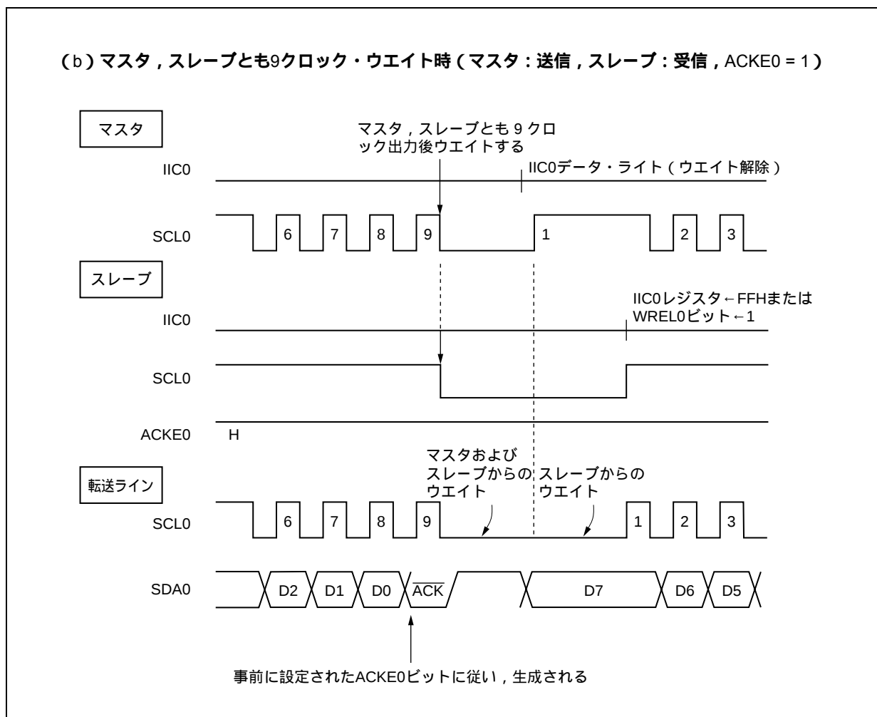
図18 - 10 ウェイト (2/2)
