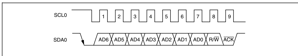
図18 - 8 アクノリッジ (ACK)
