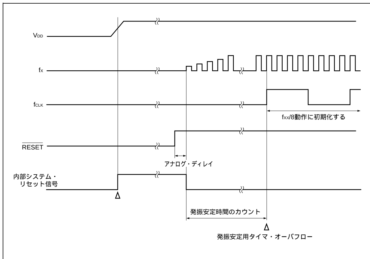
図22 - 3 パワーオン時の動作
