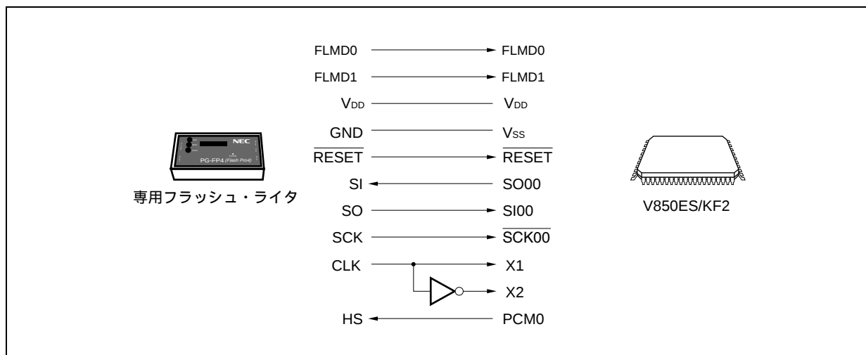
図24 - 5 専用フラッシュ・ライタとの通信 (CSI00 + HS)
