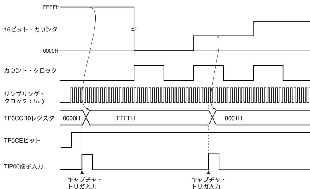
(b) パルス幅測定モード
