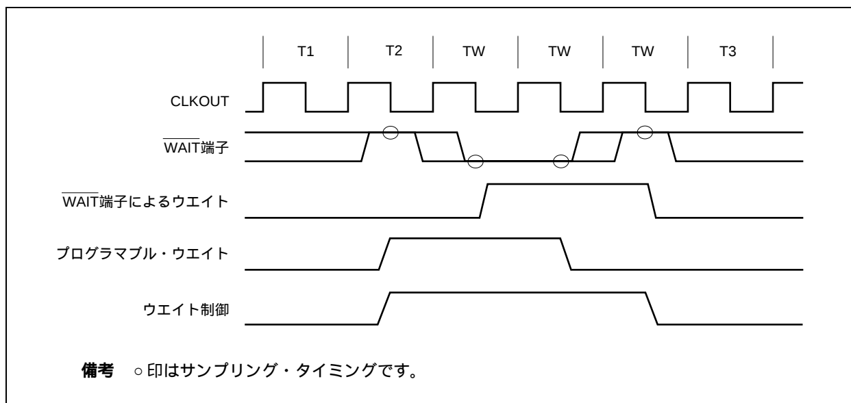
図5-3 ウェイト挿入例
