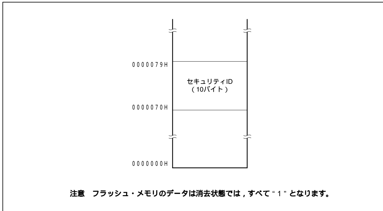
図25 - 3 セキュリティID領域
