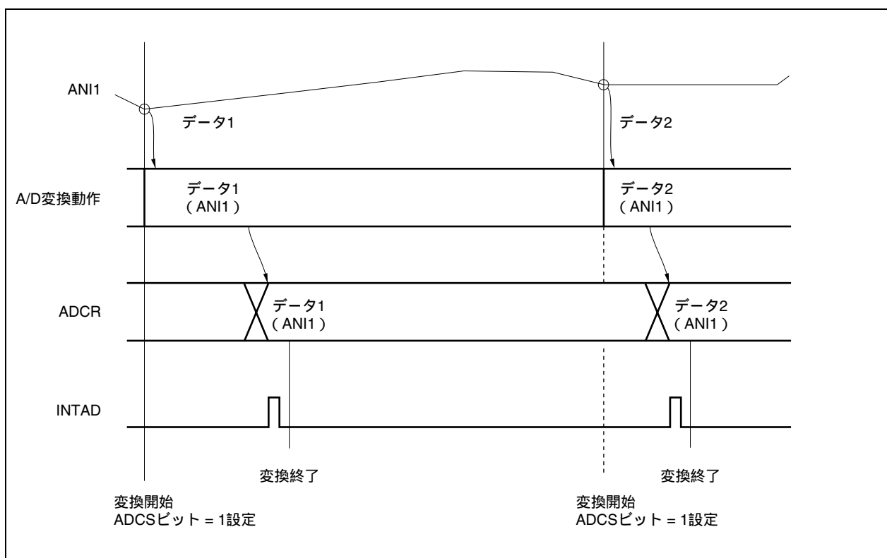
図14-4 セレクト・モード動作タイミング例 (ADS.ADS2-ADS0ビット = 001B)
