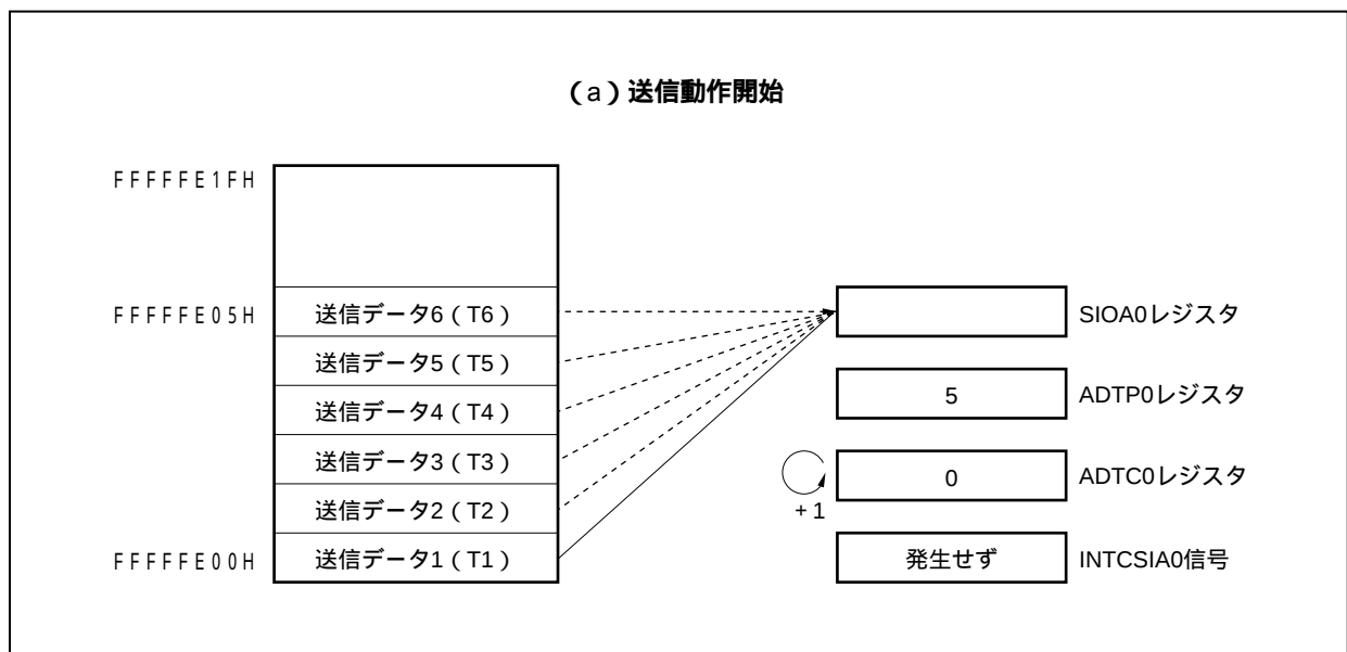
図17 - 13 6バイト分送信するときのバッファRAMの動作 (繰り返し送信モード時) (1/2)
