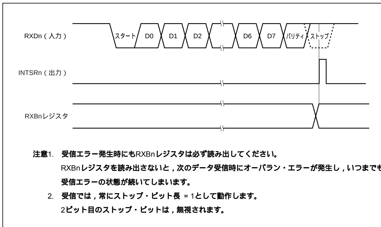
図15 - 7 UART n 受信完了割り込みタイミング
