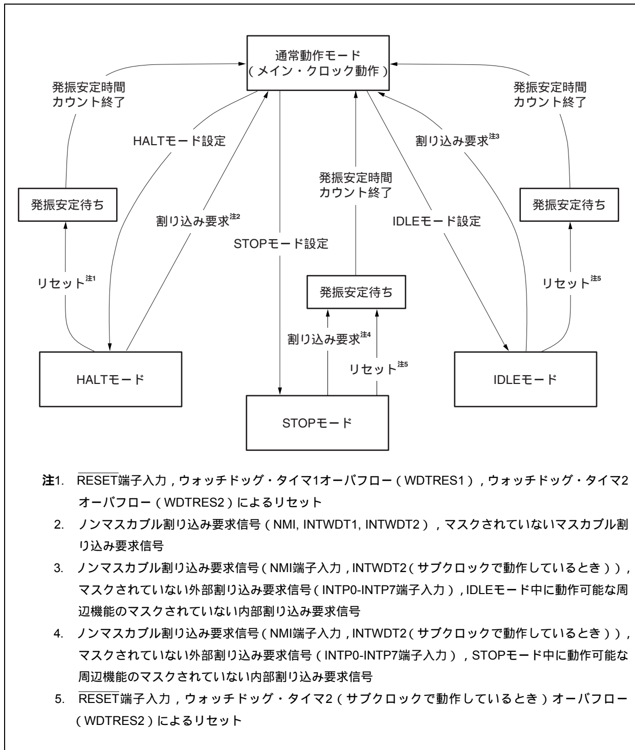
図21 - 1 状態遷移図 (1/2)
