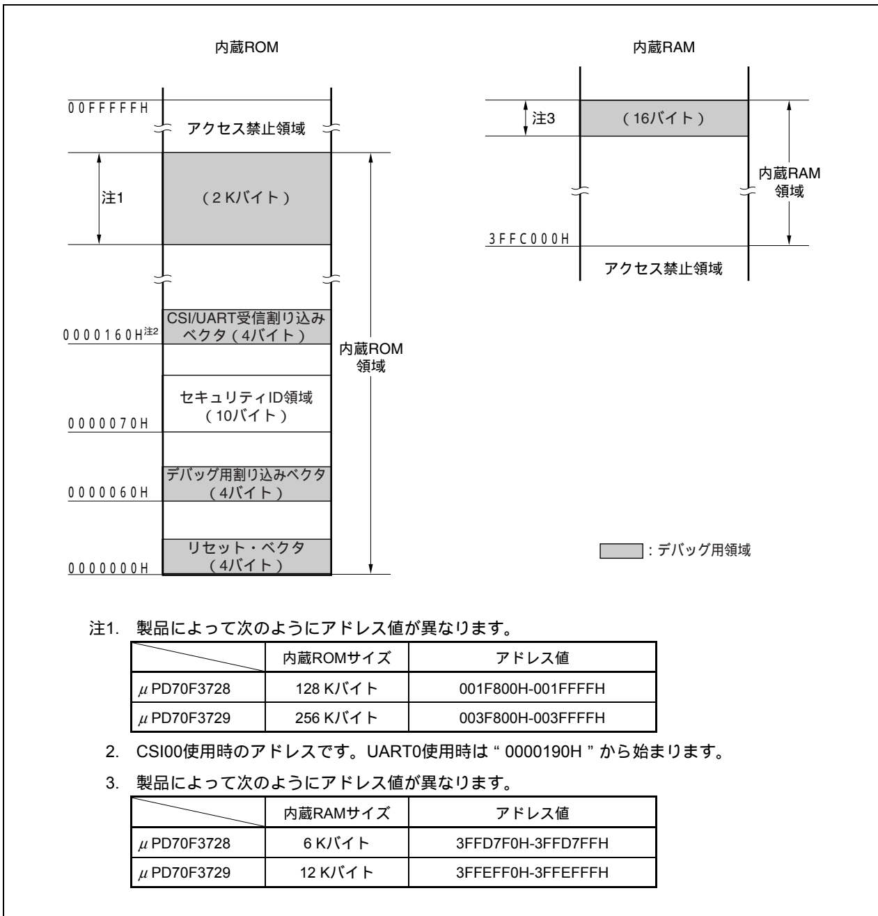
図25 - 2 デバッグ用モニタ・プログラムが配置されるメモリ空間
