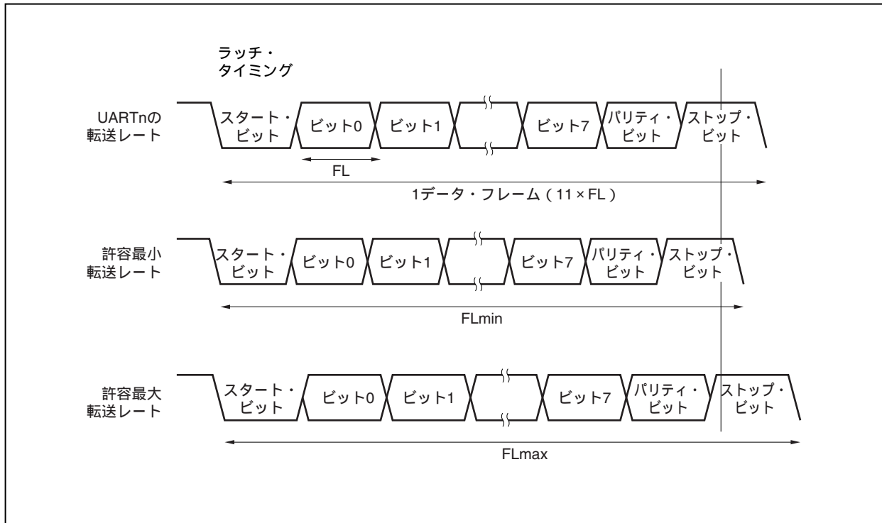
図15 - 13 受信時の許容ボー・レート範囲
