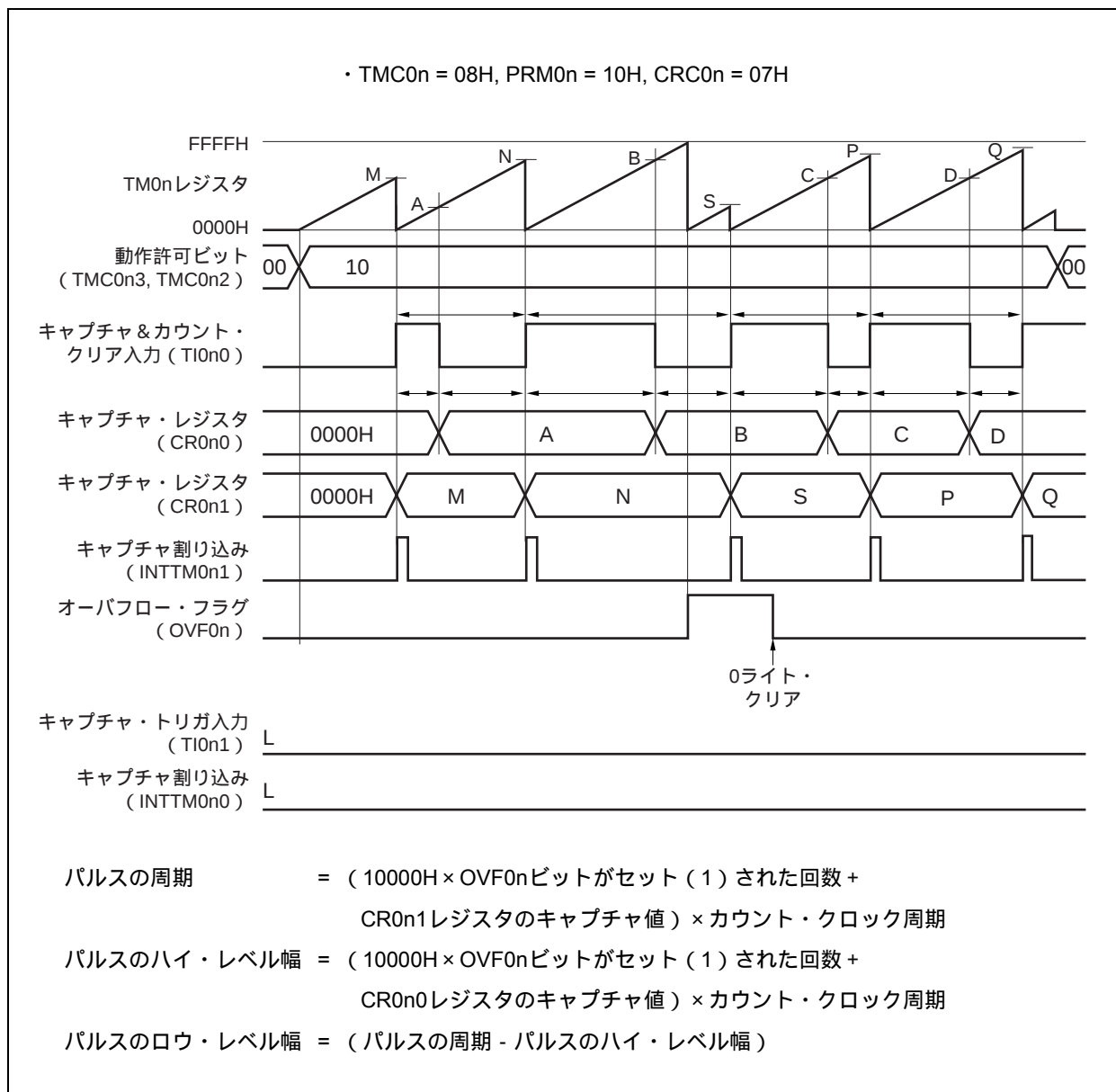
図8 - 41 パルス幅測定のタイミング例(3)
