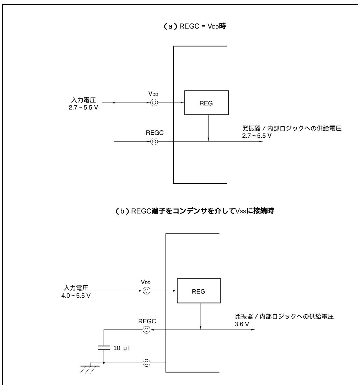
図23 - 2 REGC 端子の接続
