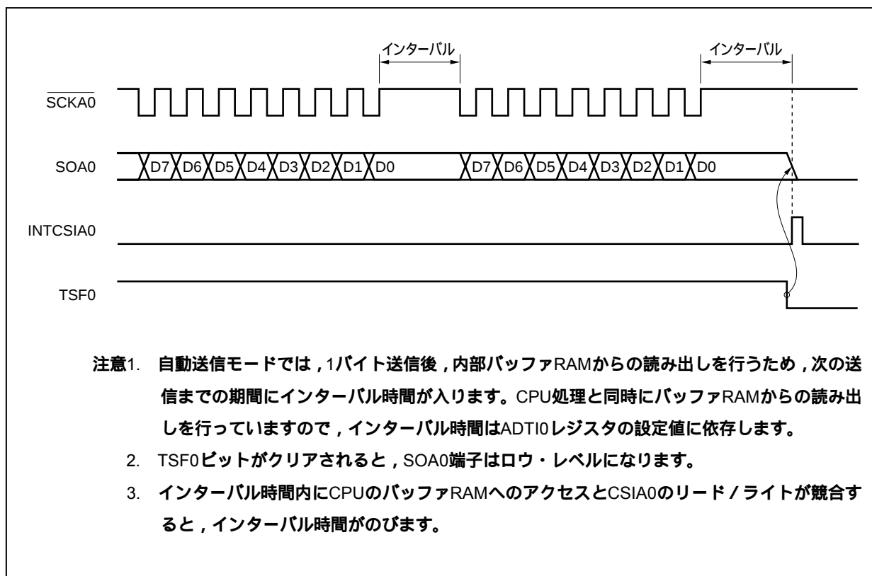
図17 - 8 自動送信モードの動作タイミング
