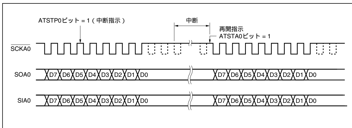
図17 - 15 自動送受信の中断と再開
