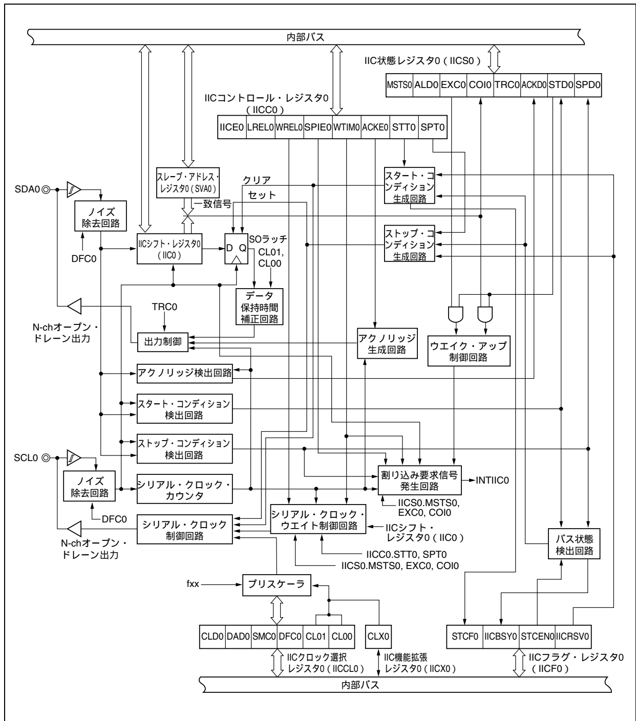
図18 - 1 I 2 C0のブロック図
