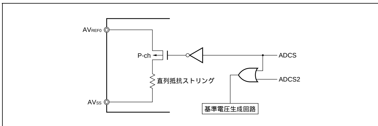
図14 - 7 スタンバイ・モード時の消費電力を低減させる方法例
