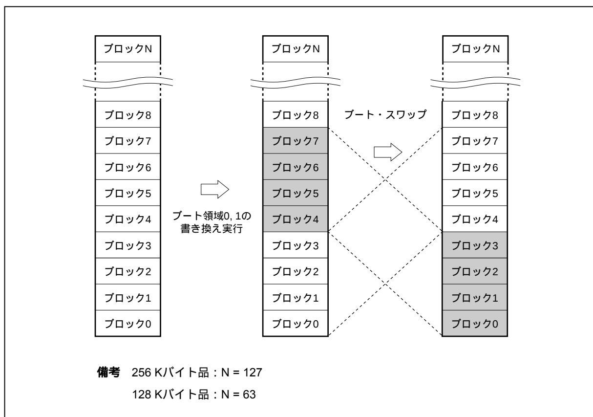
図24 - 16 全メモリ領域の書き換え (ブート・スワップ対応)
