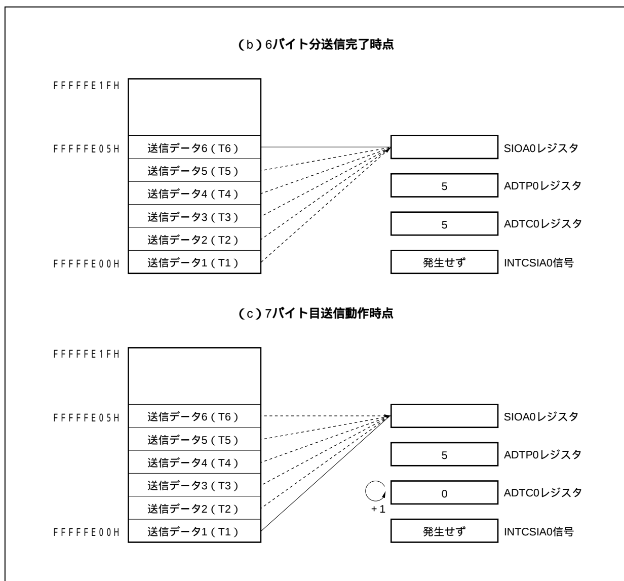
図17 - 13 6バイト分送信するときのバッファRAMの動作（繰り返し送信モード時）（2/2）
