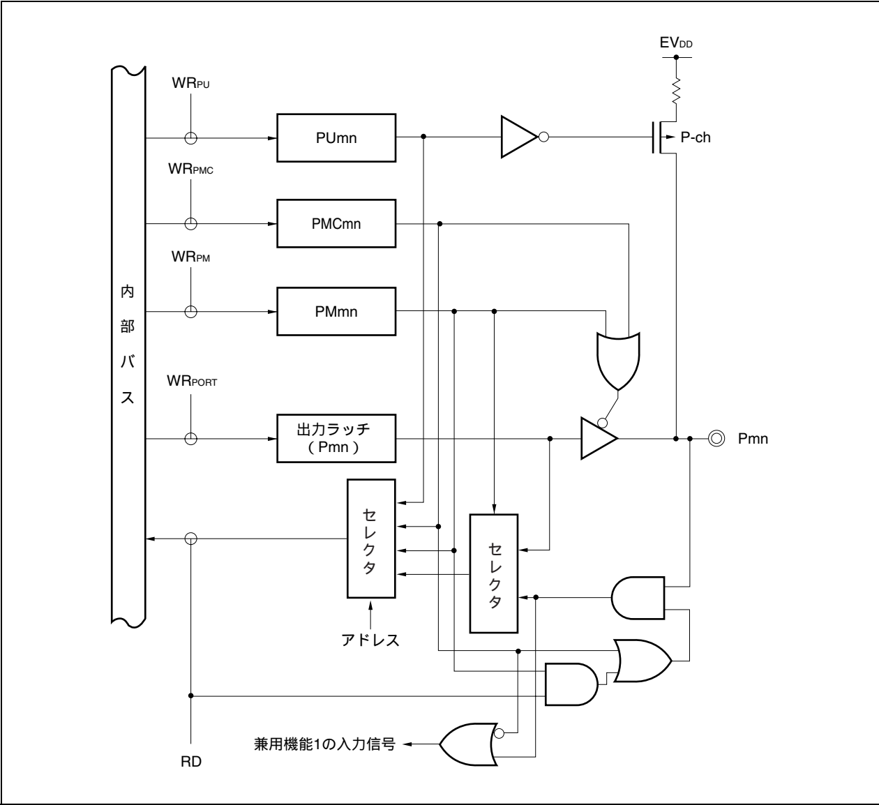
図4-9 タイプD1-UHのブロック図
