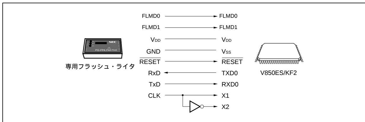
図24 - 3 専用フラッシュ・ライタとの通信 (UART0)
