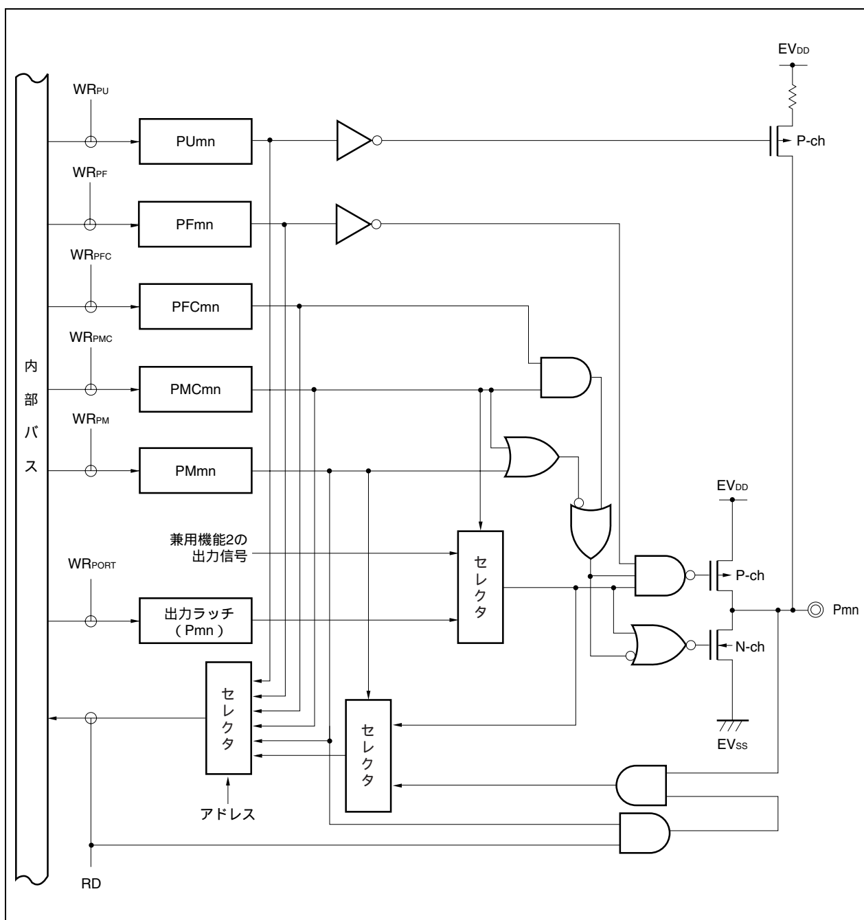
図4 - 19 タイプEx0-UFのブロック図
