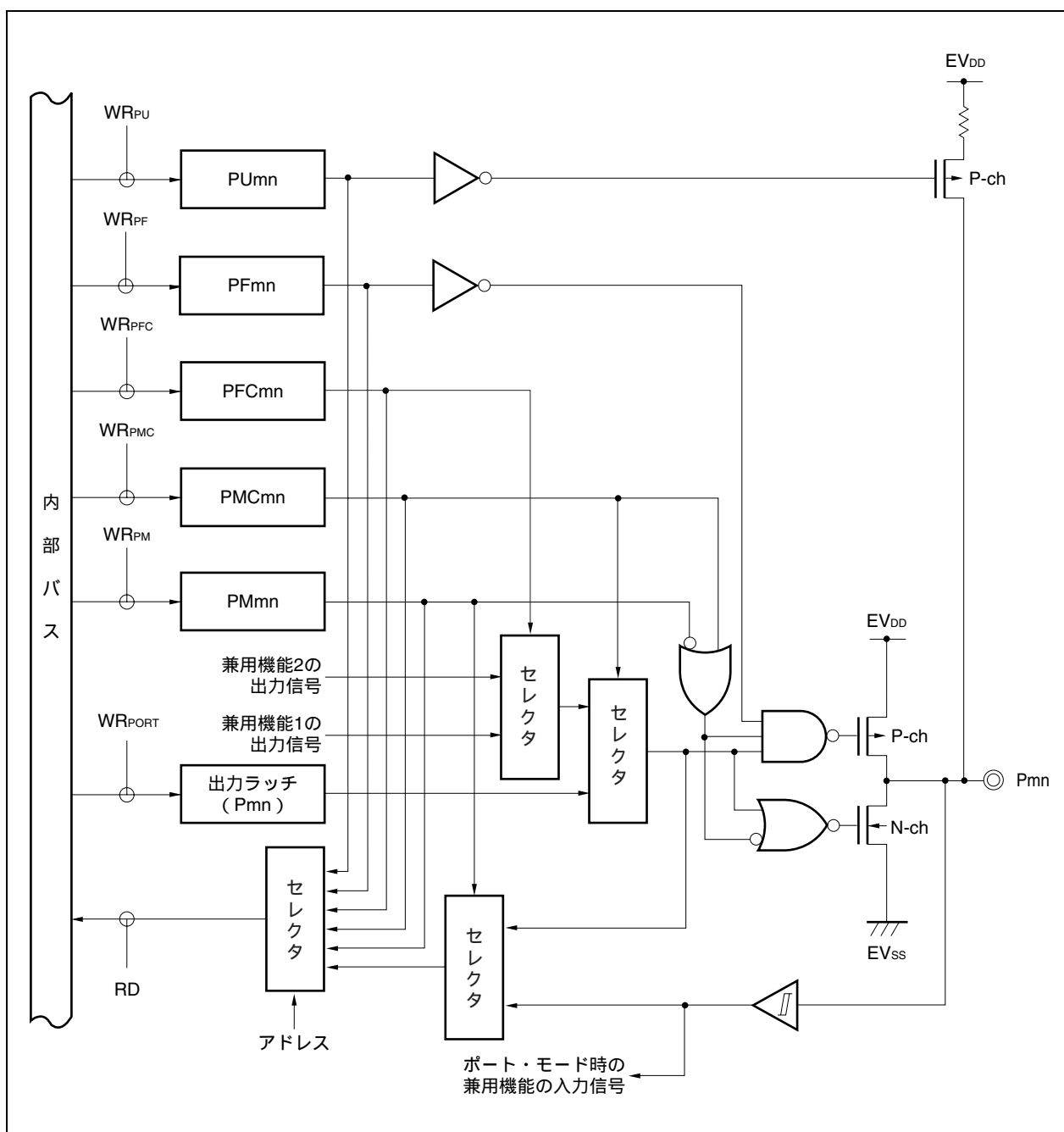
図4 - 13 タイプE00-SUFTのブロック図
