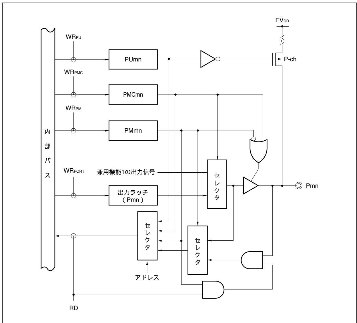
図4 - 3 タイプD0-Uのブロック図
