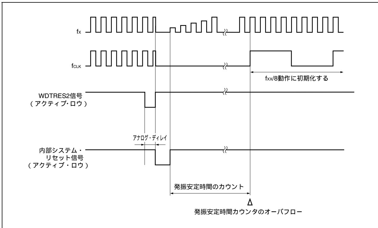
図22 - 5 ウォッチドッグ・タイマ2によるリセット動作のタイミング
