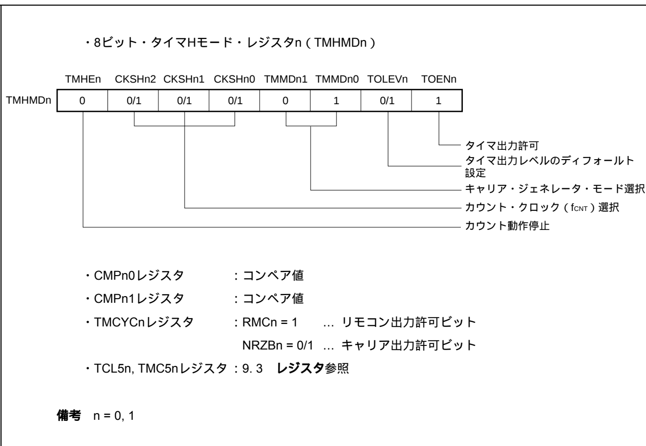
図10-7 キャリア・ジェネレータ・モード時のレジスタの設定
