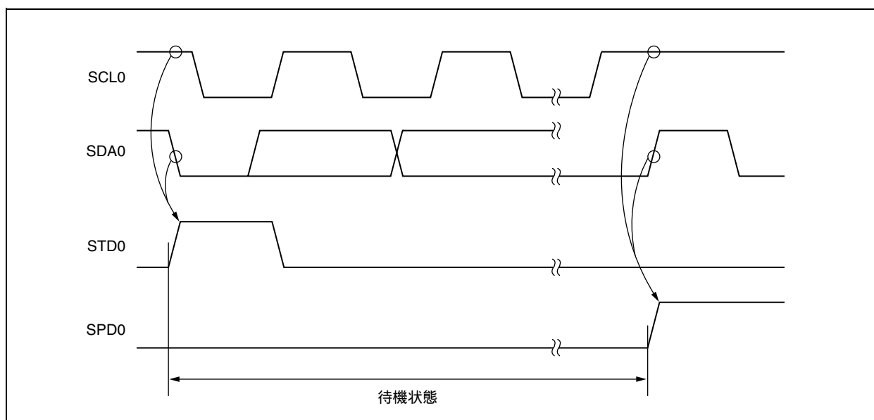
図18 - 13 通信予約受け付けタイミング
