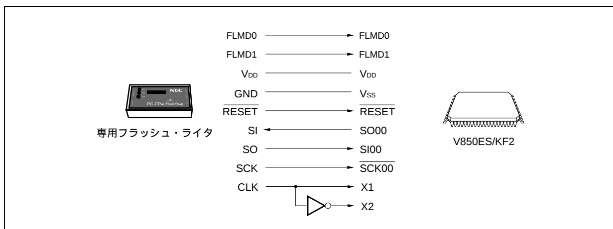
図24 - 4 専用フラッシュ・ライタとの通信 (CSI00)
