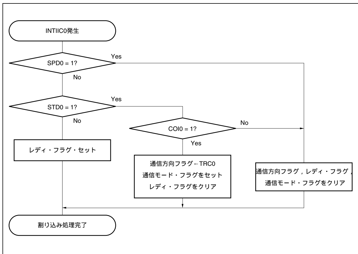
図18 - 19 スレーブ動作手順(2)
