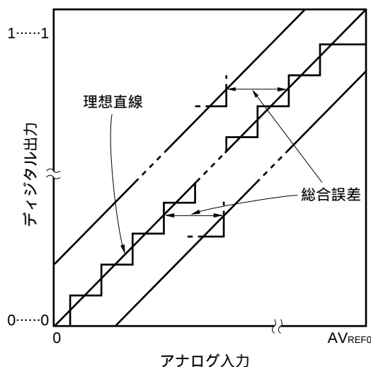
図14 - 12 総合誤差
