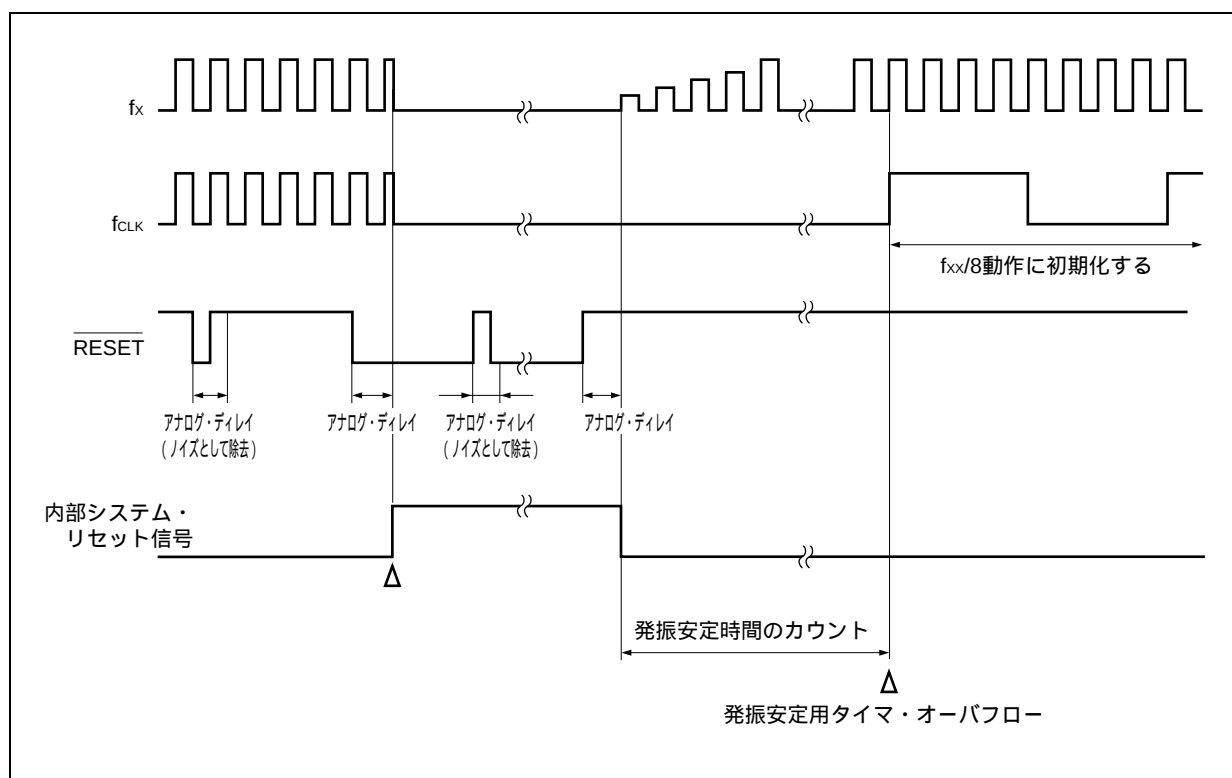
図22 - 3 パワーオン時の動作
