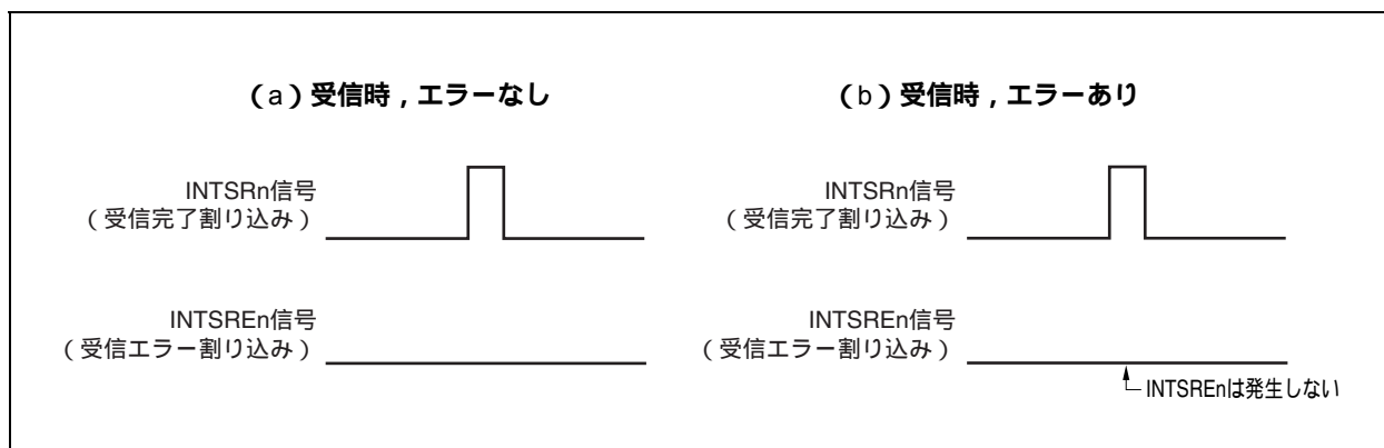
図15 - 9 受信エラー割り込み要求信号もINTSRn信号に含める場合（ISRMnビット = 1）
