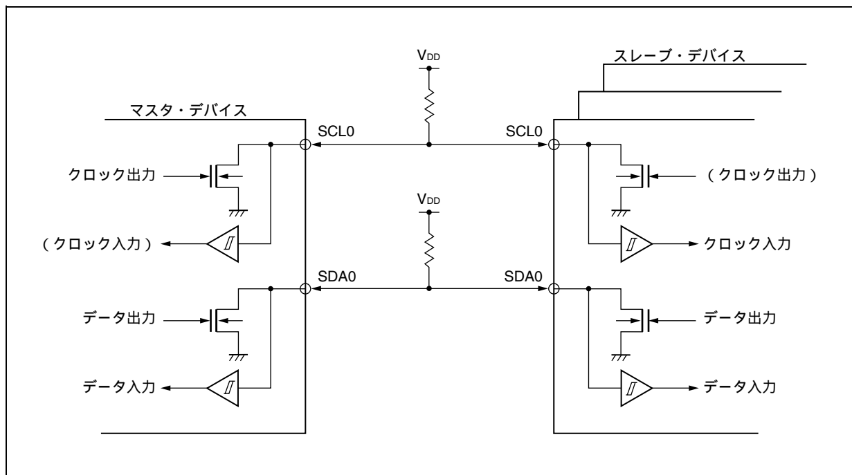
図18 - 3 端子構成図
