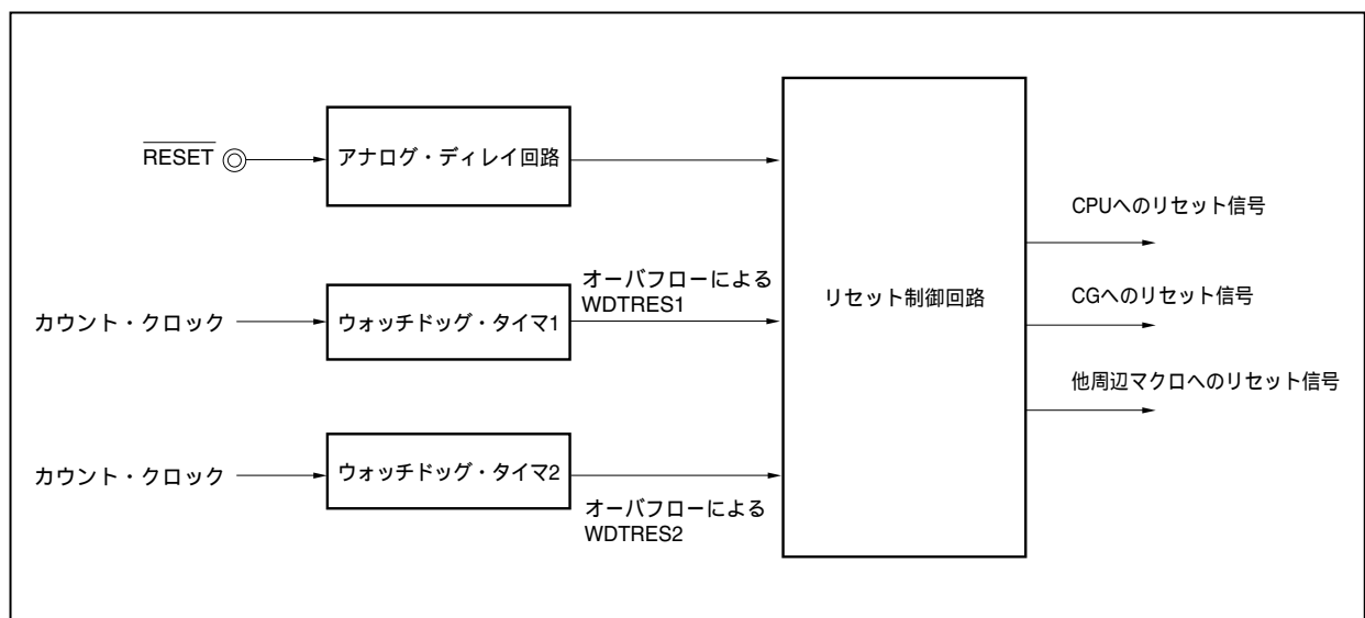
図22 - 1 リセットのブロック図
