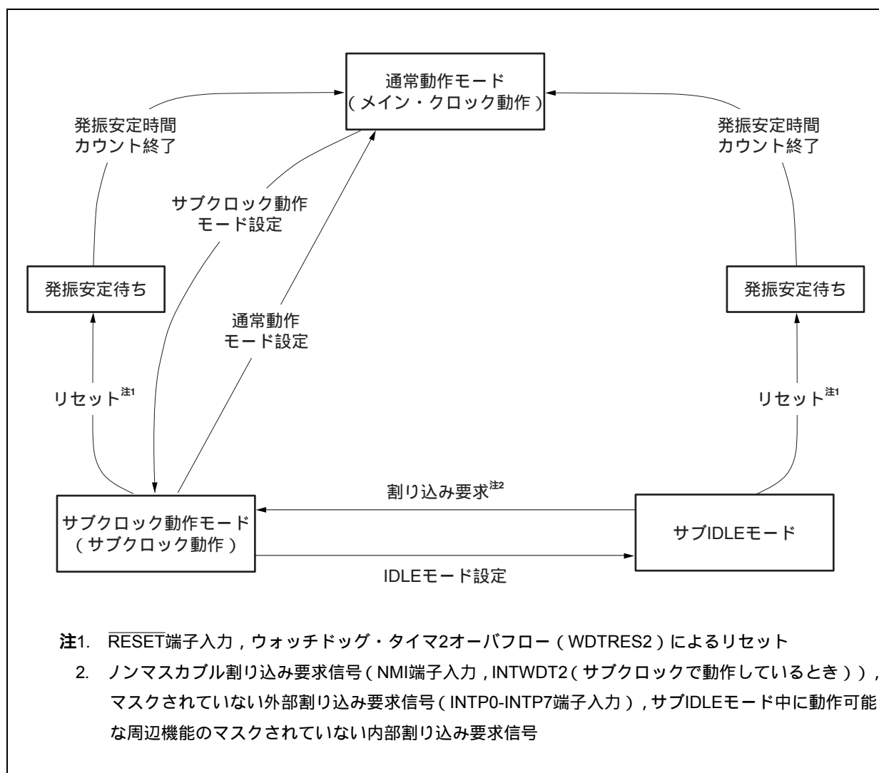
図21 - 1 状態遷移図 (2/2)
