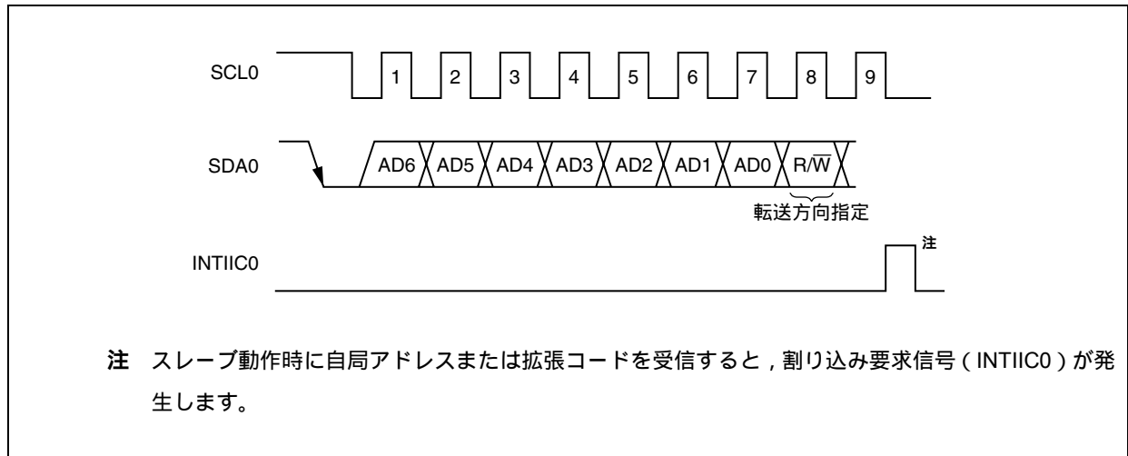
図18 - 7 転送方向指定
