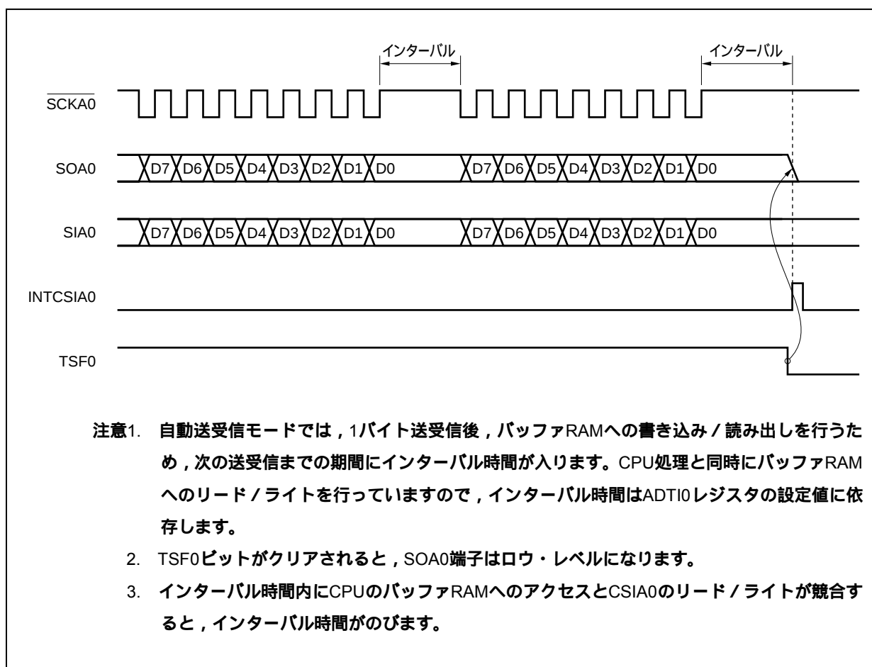
図17 - 5 自動送受信モードの動作タイミング
