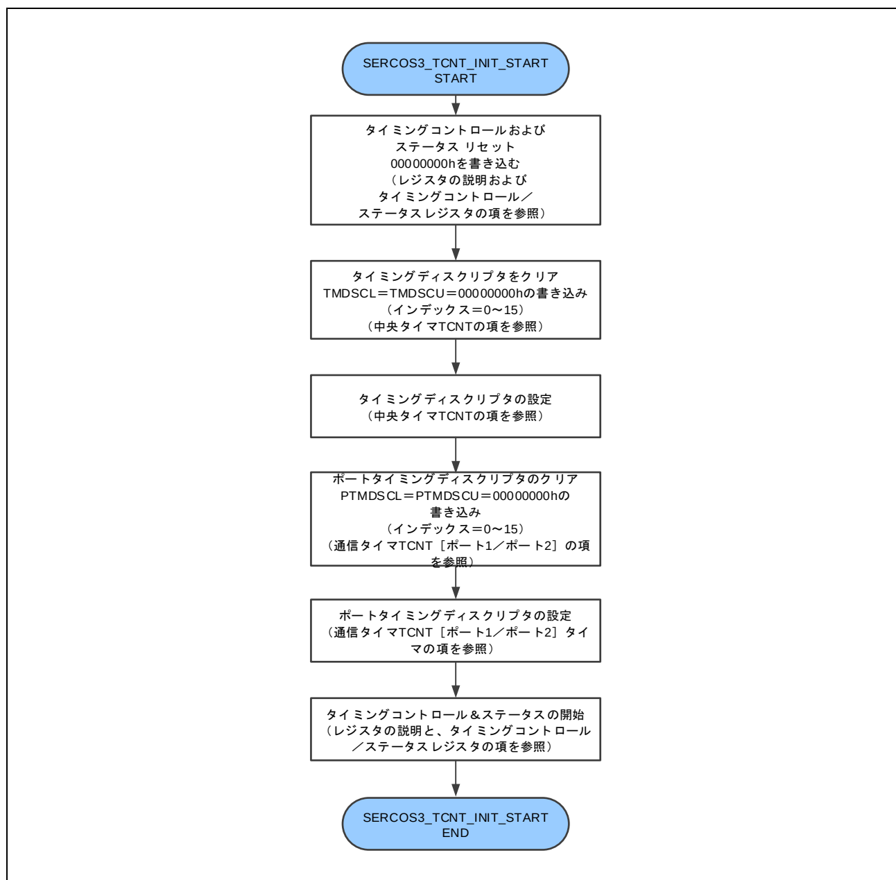
図 8.5 SERCOS3_TCNT_INIT_START フローチャート
