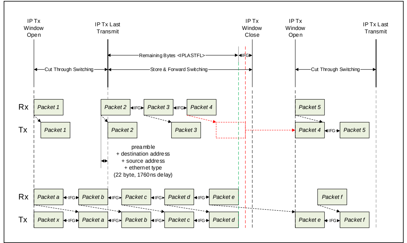
図 8.21 IPLASTFL の効果
