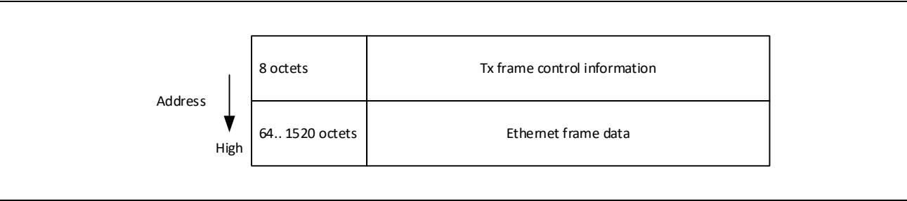
図 3.13 TX データフォーマット
