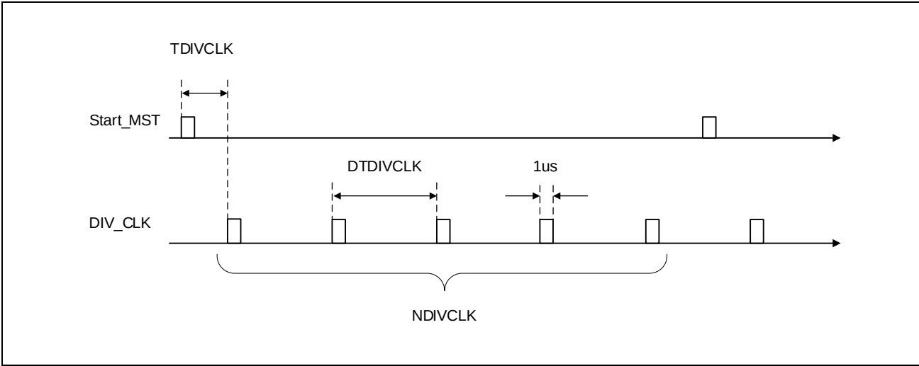
図 8.12 DIV_CLK モード 0 における TDIVCLK および DTDIVCLK
