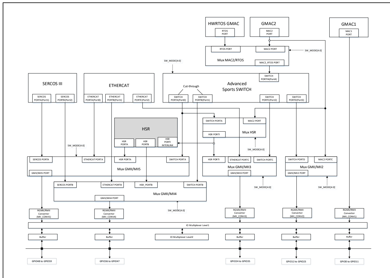
図 7.1 HSR のブロック図
