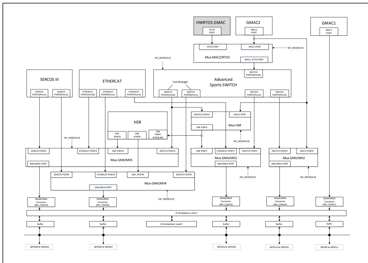
図 3.1 HW-RTOS GMAC のブロック図
