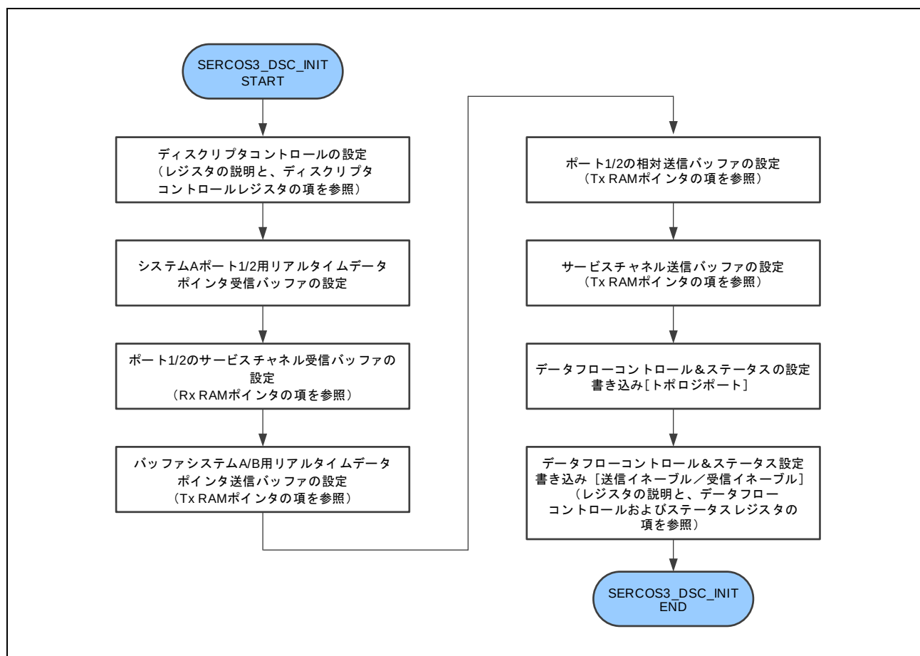
図 8.4 SERCOS3_DSC_INIT フローチャート
