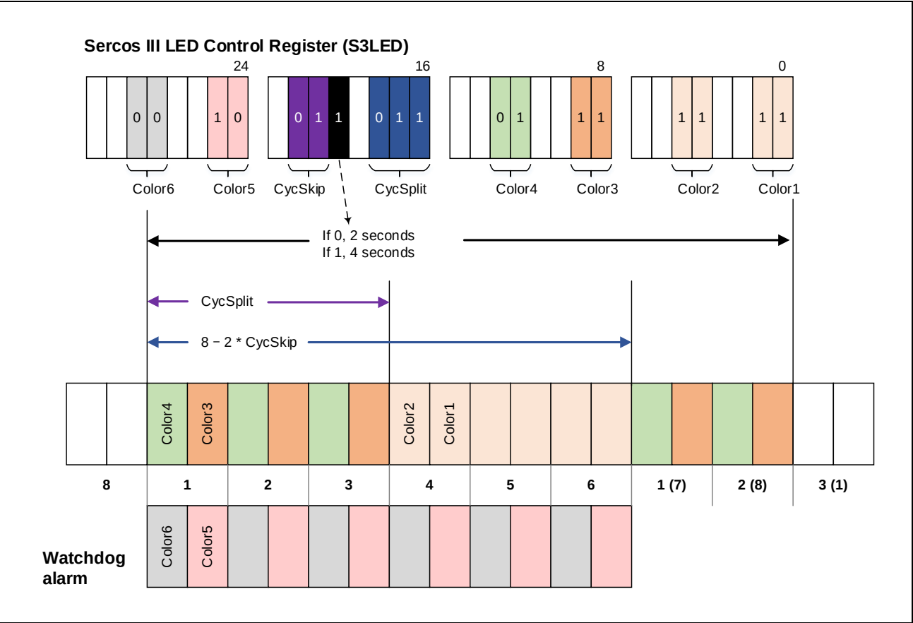
図 8.22 LED コントロール
