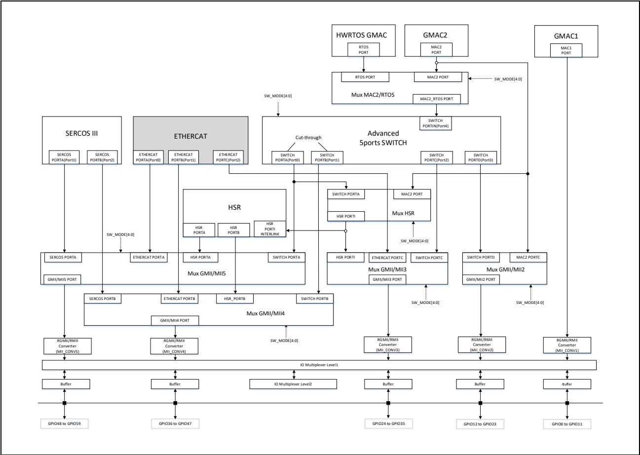
図 5.1 EtherCAT スレーブ接続
