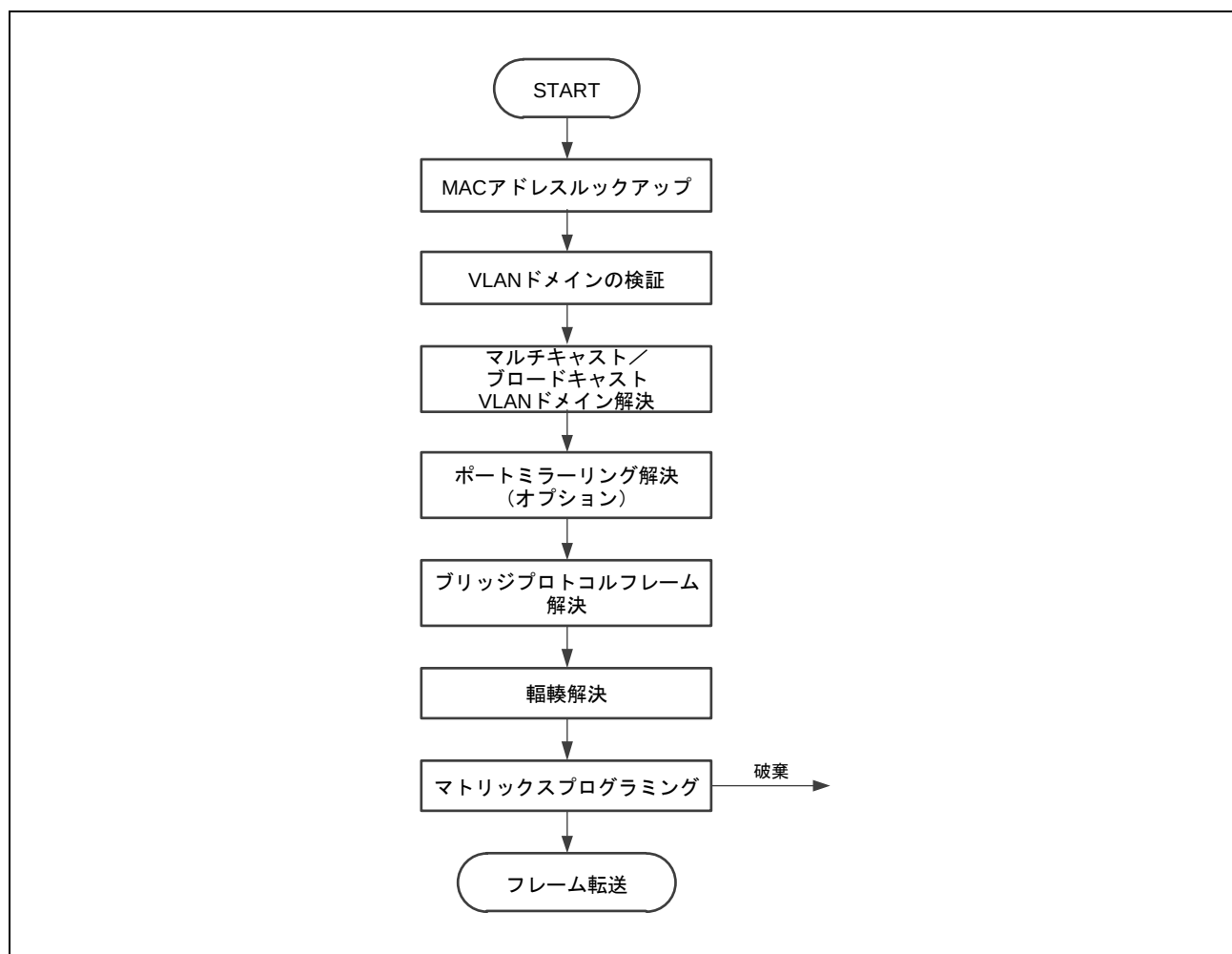
図 4.15 フレーム転送タスクの概要
