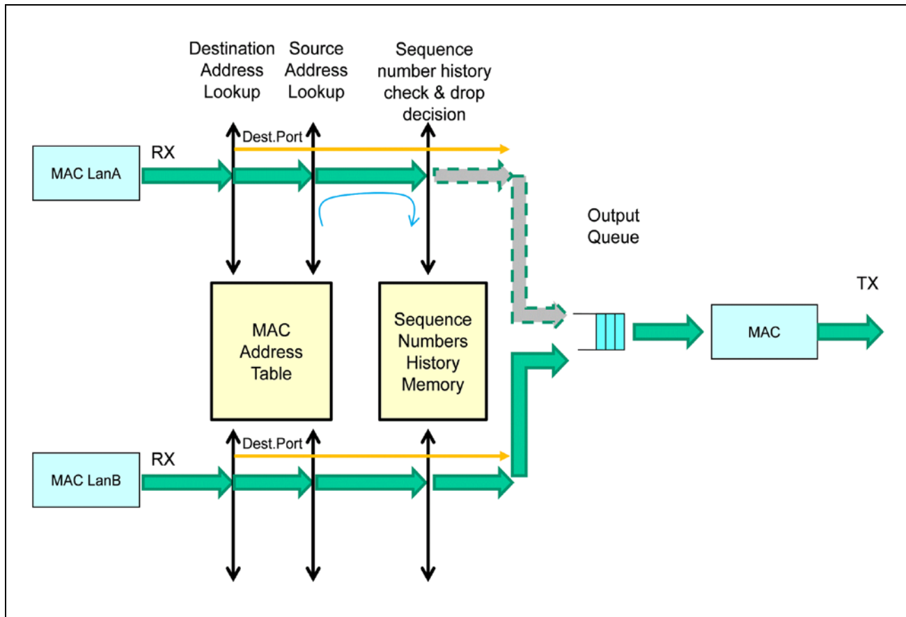
図 4.28 冗長ネットワークからの受信
