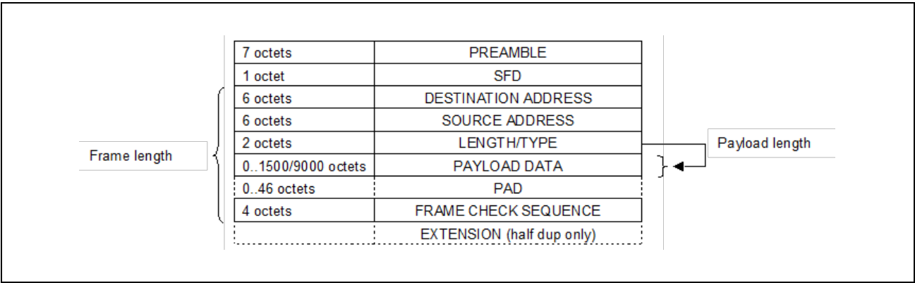
図 4.2 MAC フレームフォーマットの概要
