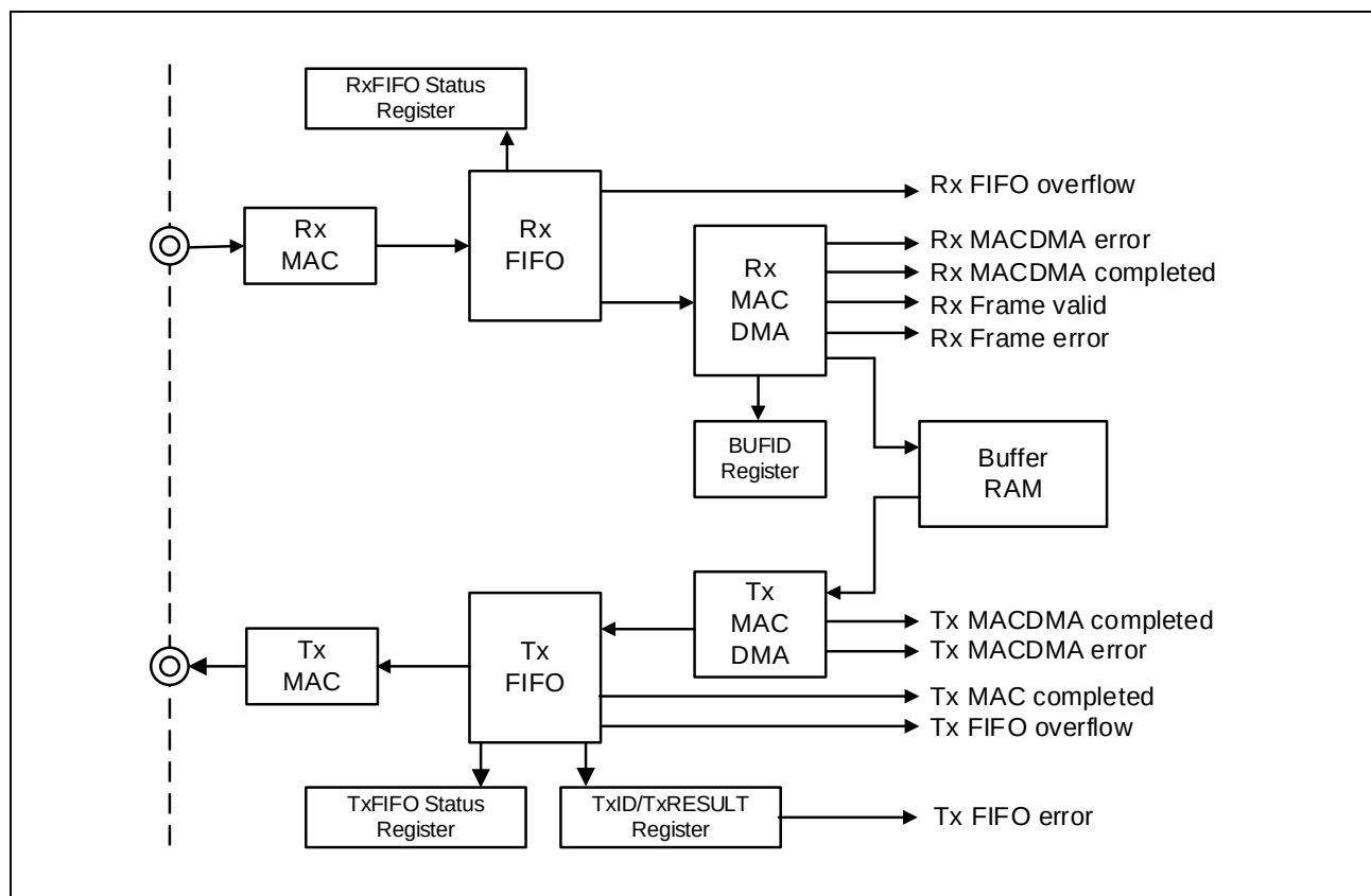
図 3.8 MACDMAC 周辺と割り込み信号のブロック図
