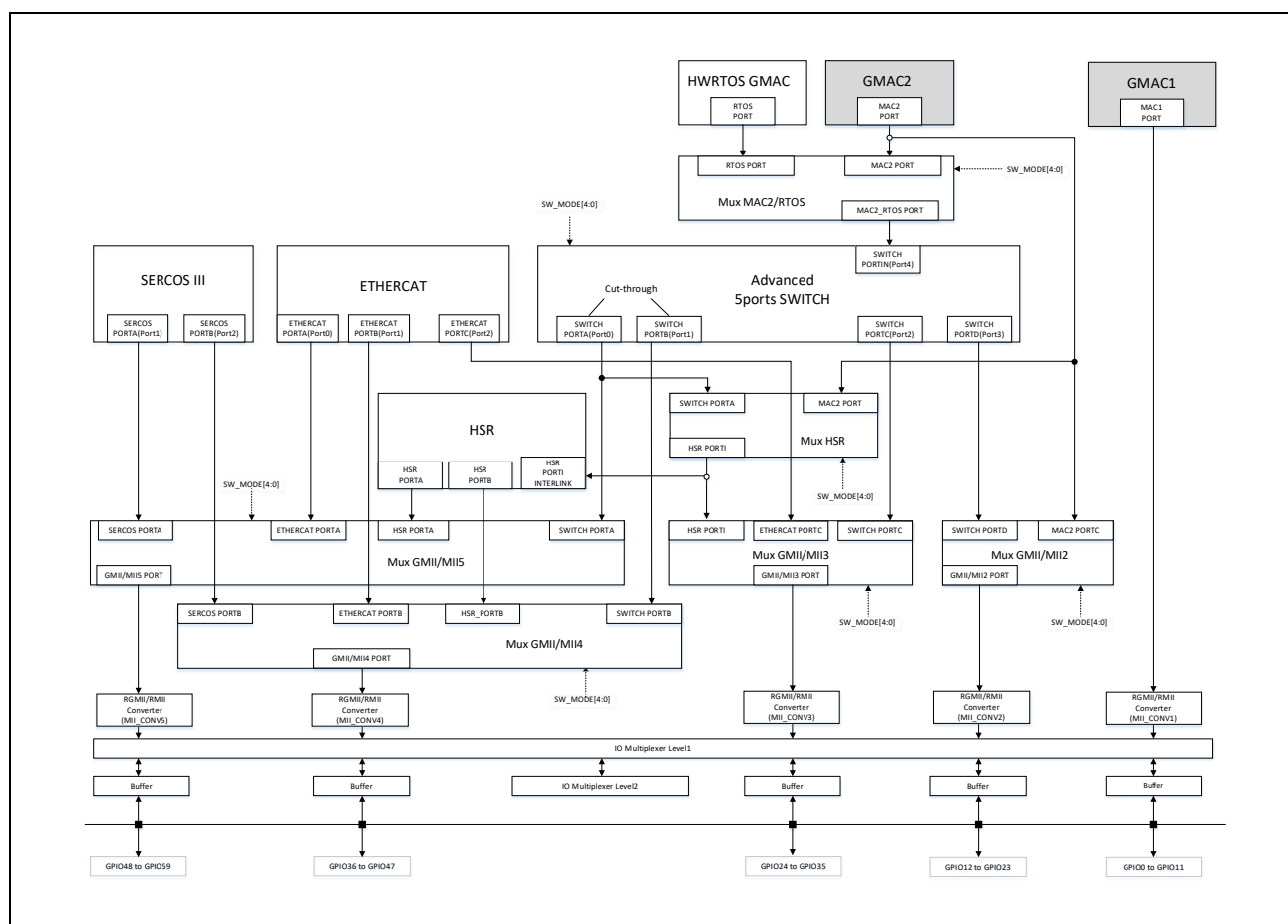
図 6.1 GMAC のブロック図
