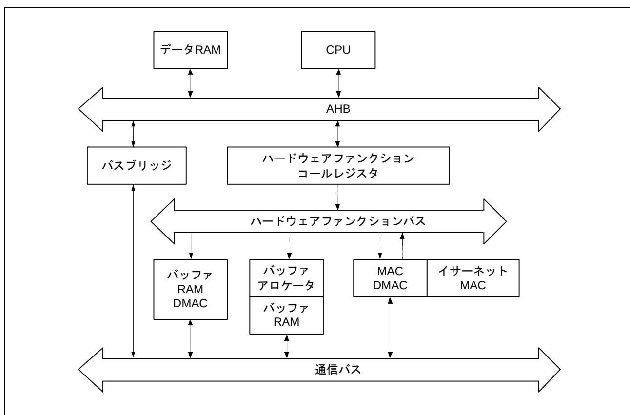
図 3.3 ハードウェアファンクションのブロック図
