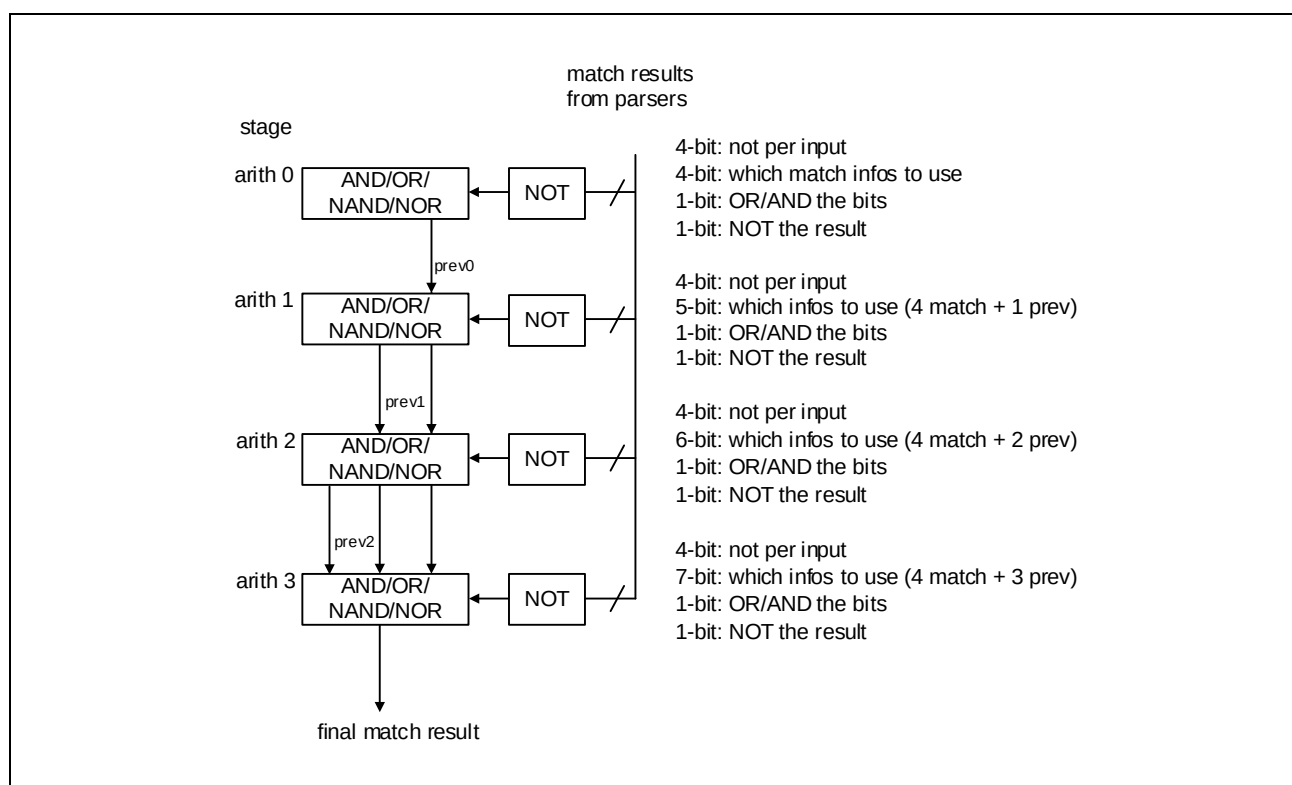
図 4.10 スヌープ演算機能
