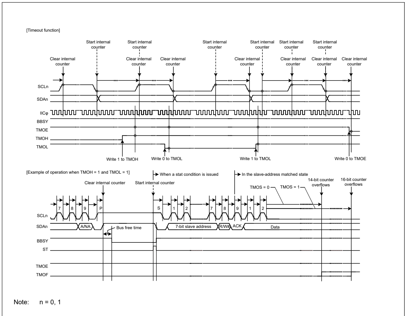
Figure 40.48 Timeout function using the TMOE, TMOS, TMOH, and TMOL bits
