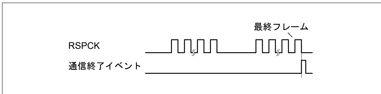
図 28.66 通信終了イベント出力タイミング (受信専用スレーブモード、クロック同期式動作)
