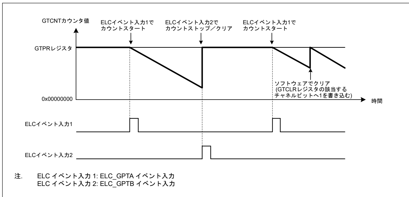
図 20.37 ハードウェア要因によるカウンタクリア動作例（のこぎり波ダウンカウント、ELC_GPTA 入力でスタート、ELC_GPTB 入力でストップ/クリアの場合）
