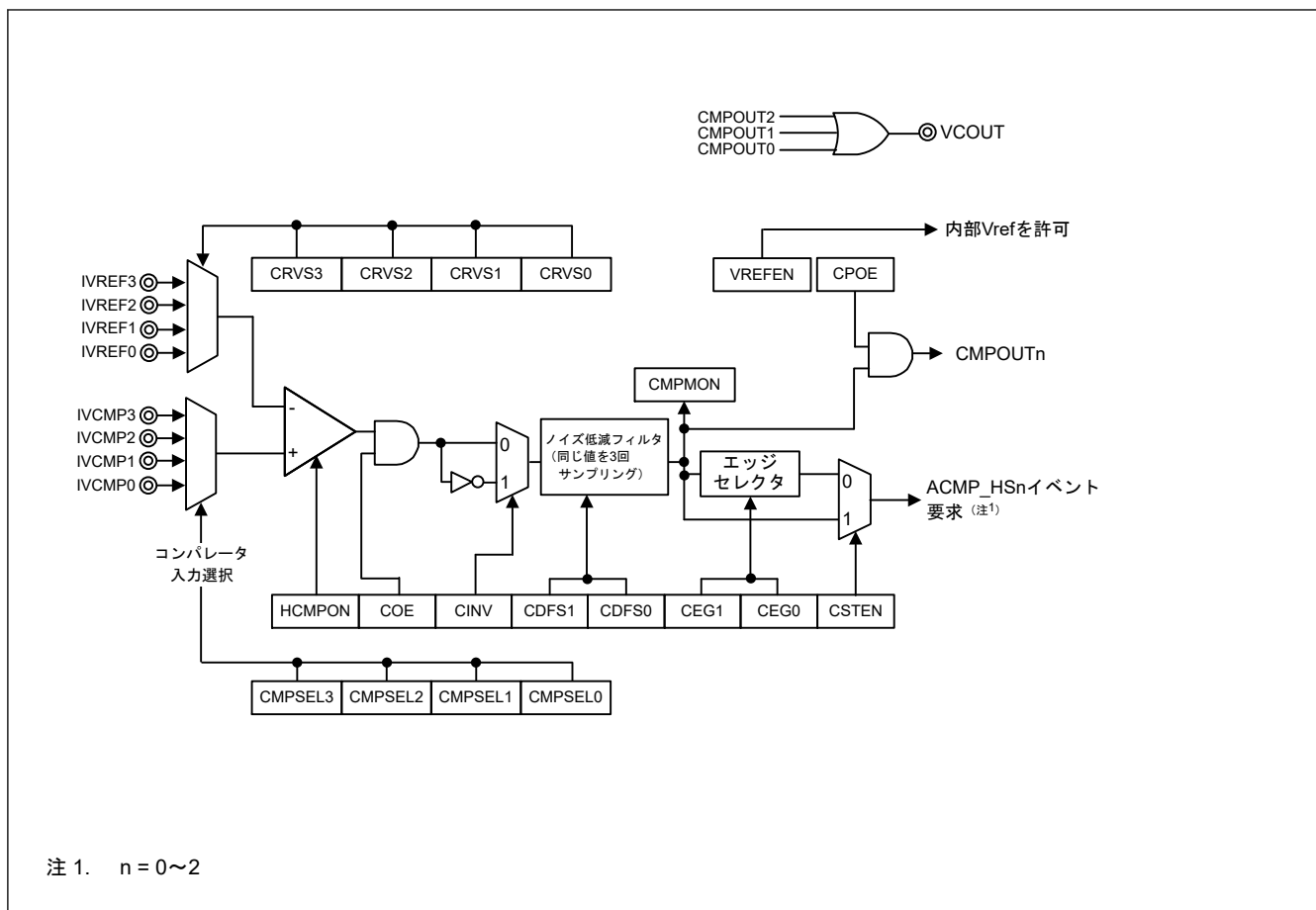
図 35.1 ACMPHS ブロック図
