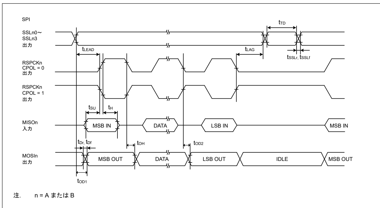
図 41.35 CPHA = 0 の場合におけるマスタの SPI タイミング
