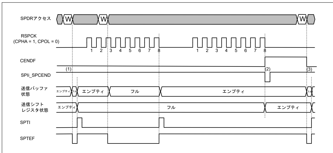
図 28.34 通信終了割り込み動作例（クロック同期式動作時の送受信／送信スレーブモード）
