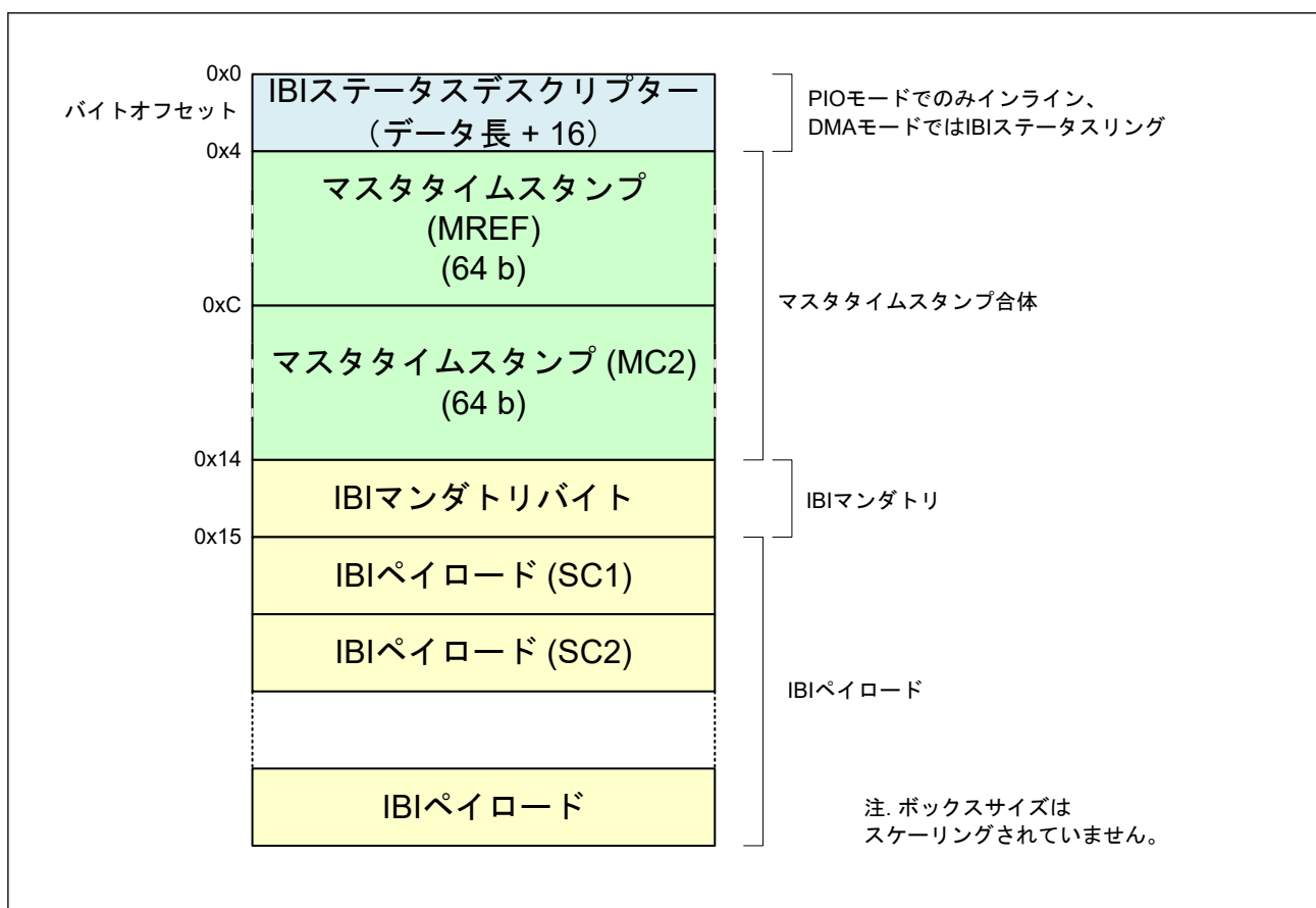
図 25.87 IBI イベント用のマスタタイムスタンプカウンタ
