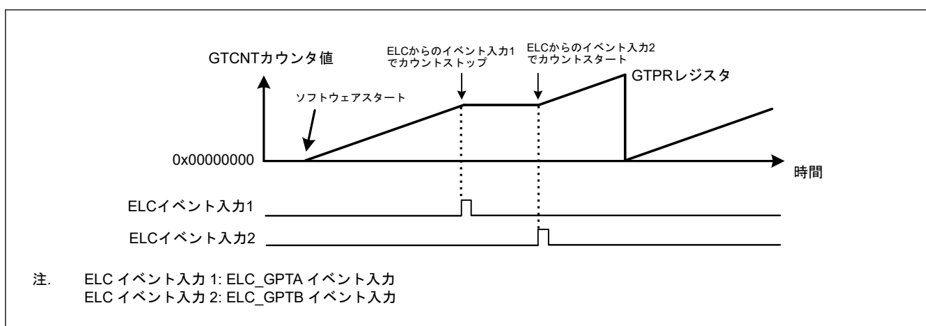
図 20.34 ハードウェア要因によるカウントストップ動作例 (ソフトウェアによるスタート、ELC_GPTA 入力でのストップ、および ELC_GPTB 入力での再スタートの場合)
