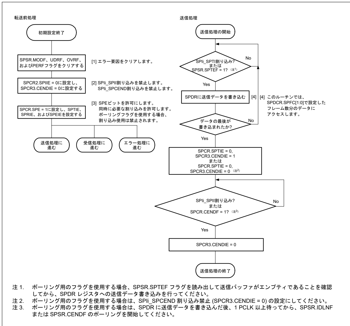
図 28.53 スレーブモードでの送信フロー
