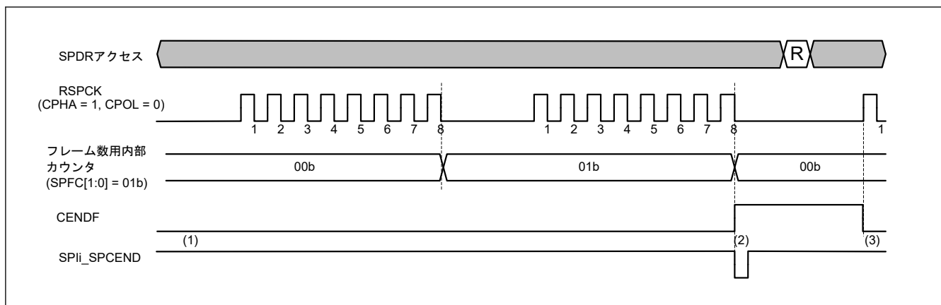
図 28.35 通信終了割り込み動作例（クロック同期式動作時の受信のみスレーブモード）
