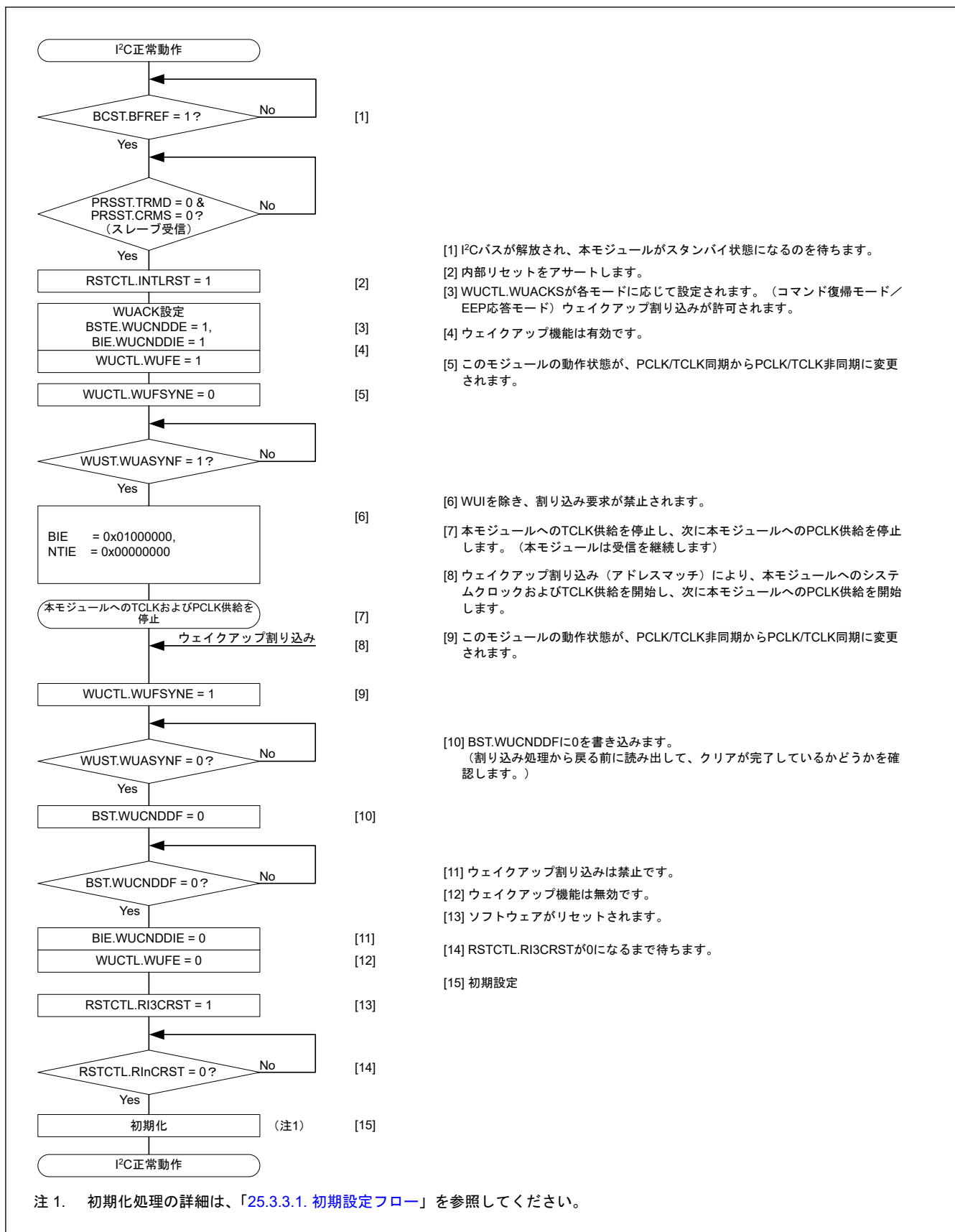
図 25.104 コマンドリカバリモードと EEP 応答モードの使用例 (スレーブアドレス一致に起因するウェイクアップ割り込みによるウェイクアップリカバリの場合)
