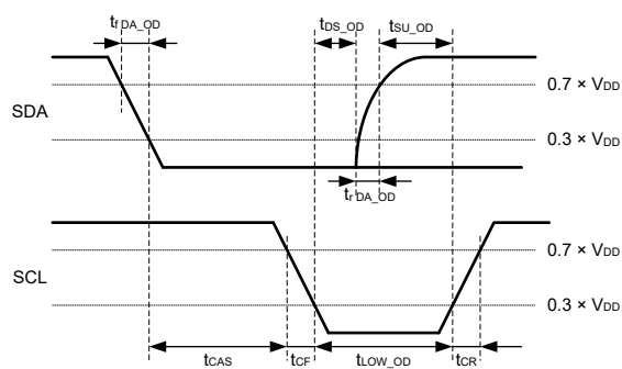
図 41.45 I3C スタートコンディションタイミング
