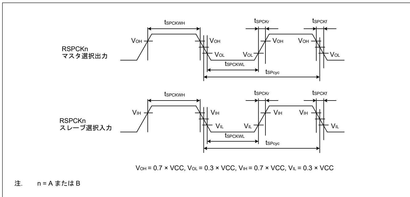
図 41.34 SPI クロックタイミング
