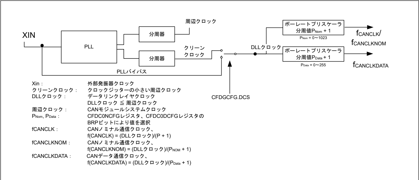
図 26.16 CAN チャネルの通信クロックを生成する回路のブロック図
