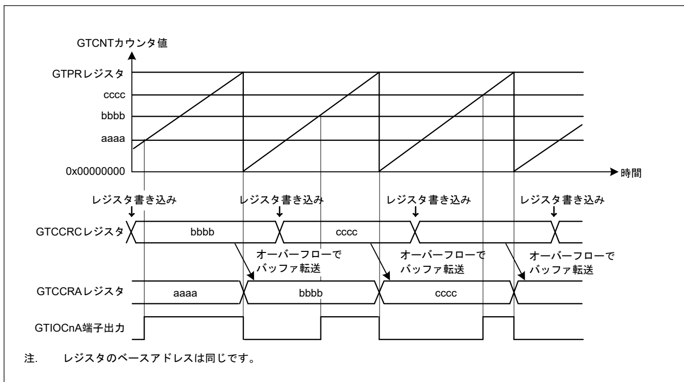
図 20.14 GTCCRA レジスタのバッファ動作例（アウトプットコンペア、アップカウント時ののこぎり波、GTCCRA レジスタのコンペアマッチで High 出力、周期の終わりで Low 出力の場合）
