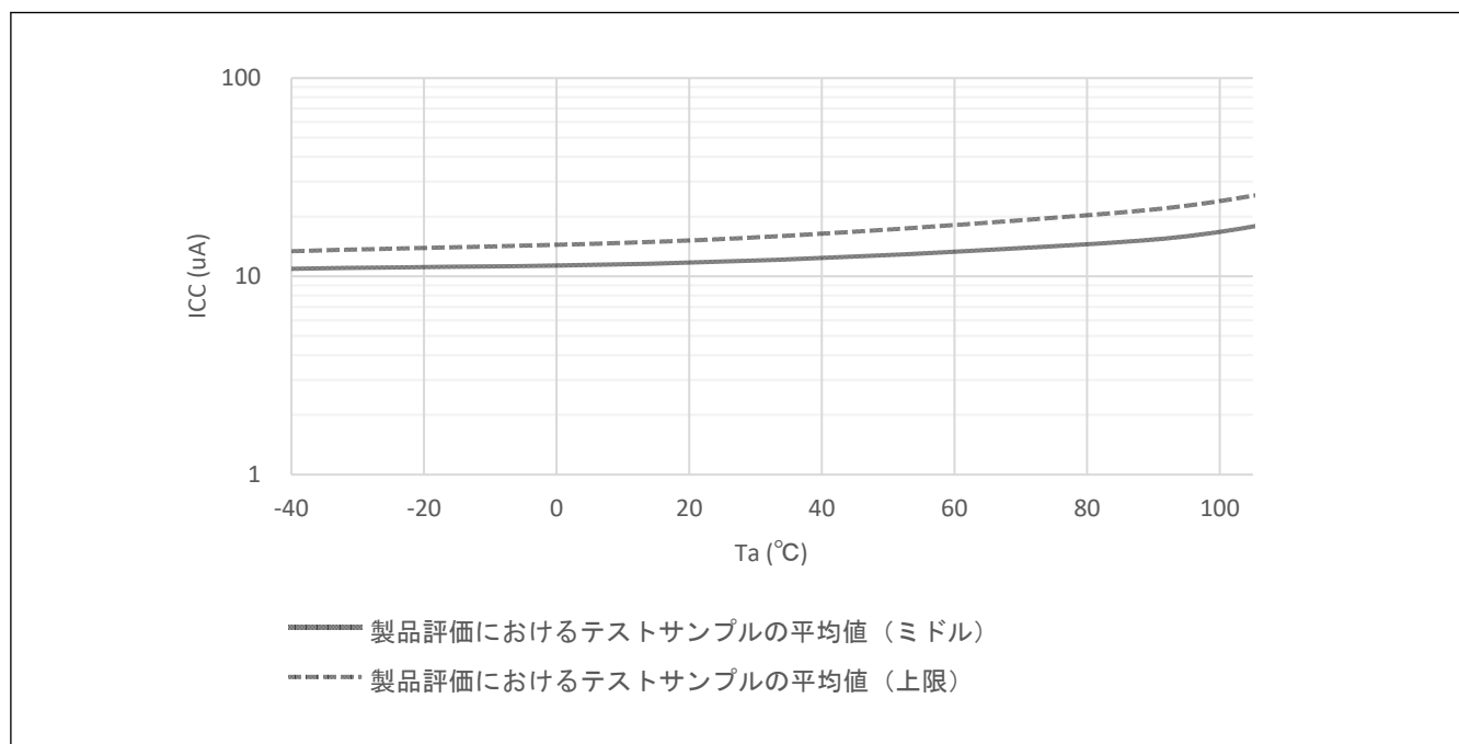
図 41.4 ディープソフトウェアスタンバイモード時の温度依存性、DPSBYCR.DEEPCUT[1:0] = 01b (参考データ)
