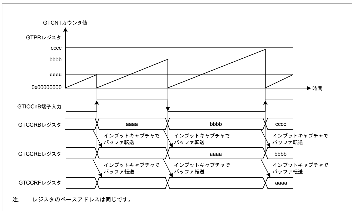
図 20.18 GTCRB レジスタのダブルバッファ動作例 (GTIOCnB 端子入力の両エッジでインプットキャプチャ、のこぎり波でアップカウント、GTIOCnB 端子入力の両エッジで GTCNT カウンタクリアの場合)
