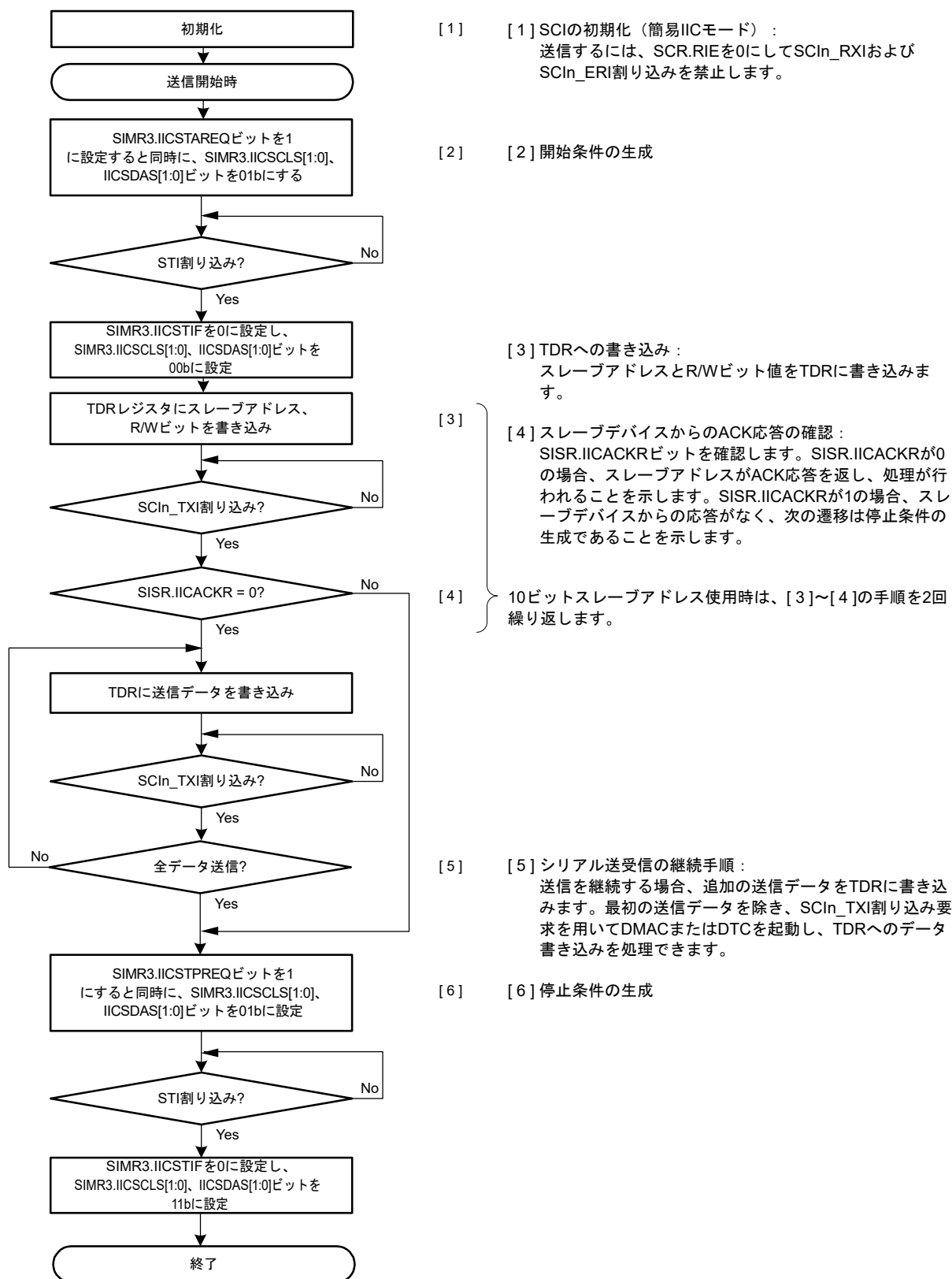
図 24.92 簡易 IIC モードにおけるマスタ送信のフローチャート例（送信割り込み、受信割り込み使用時）
