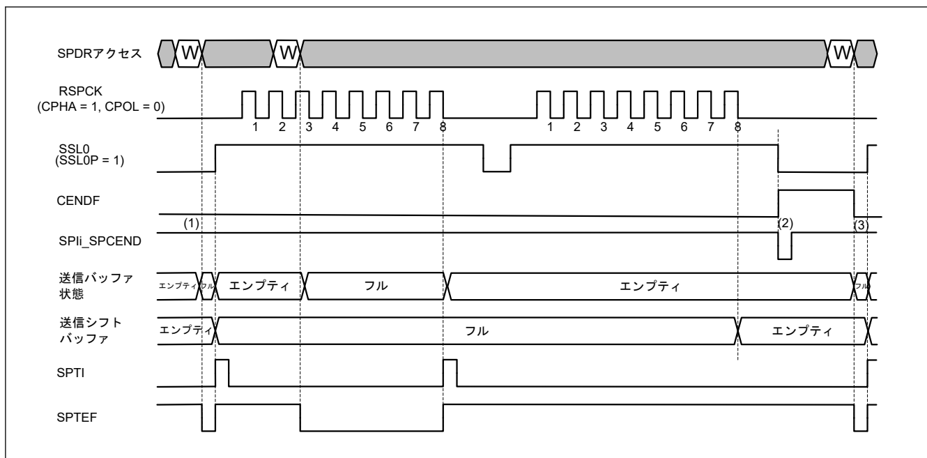
図 28.32 通信終了割り込み動作例 (SPI 動作時の送受信/送信スレーブモード)
