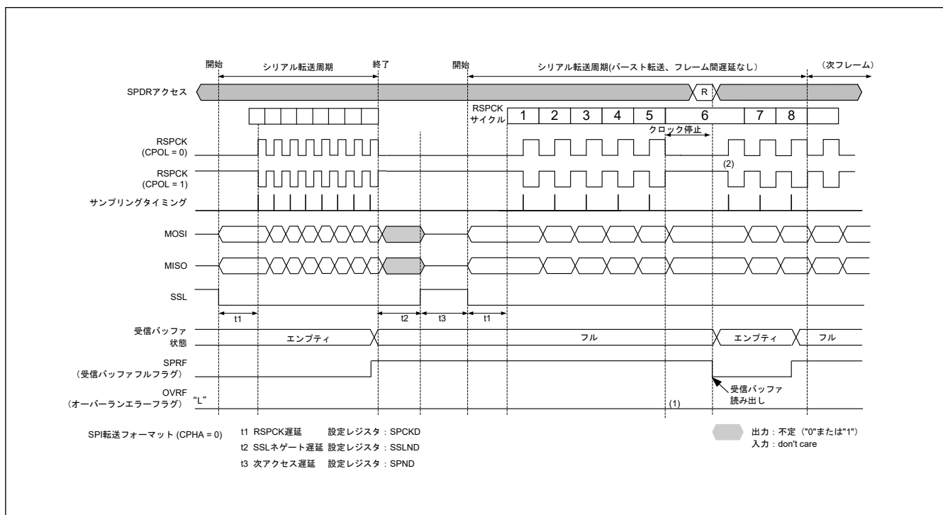
図 28.41 マスタモードの受信バッファフル状態でシリアル転送が継続する場合のクロック停止波形(バースト転送でフレーム間遅延なし、CPHA = 0)
