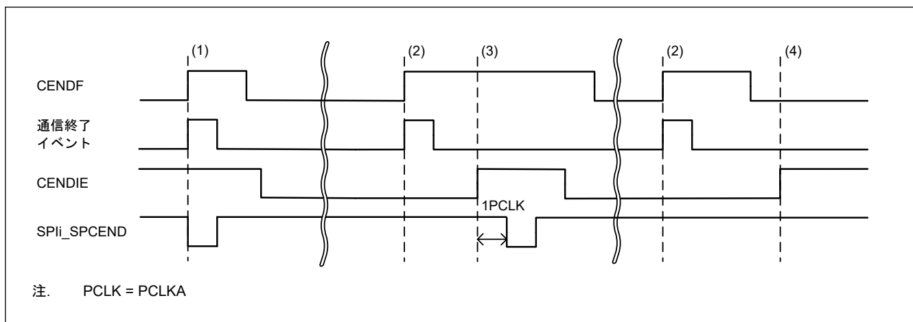
図 28.36 通信終了割り込みの動作例（許可制御）
