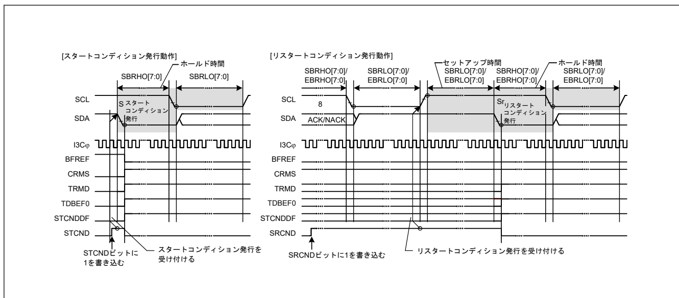
図 25.56 スタートコンディション／繰り返しのスタートコンディション発行動作タイミング (STCND、SRCND ビット)
