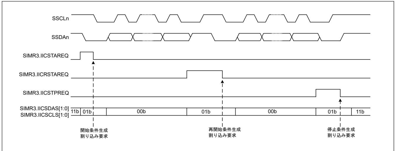
図 24.87 開始条件、再開始条件、停止条件生成の動作タイミング
