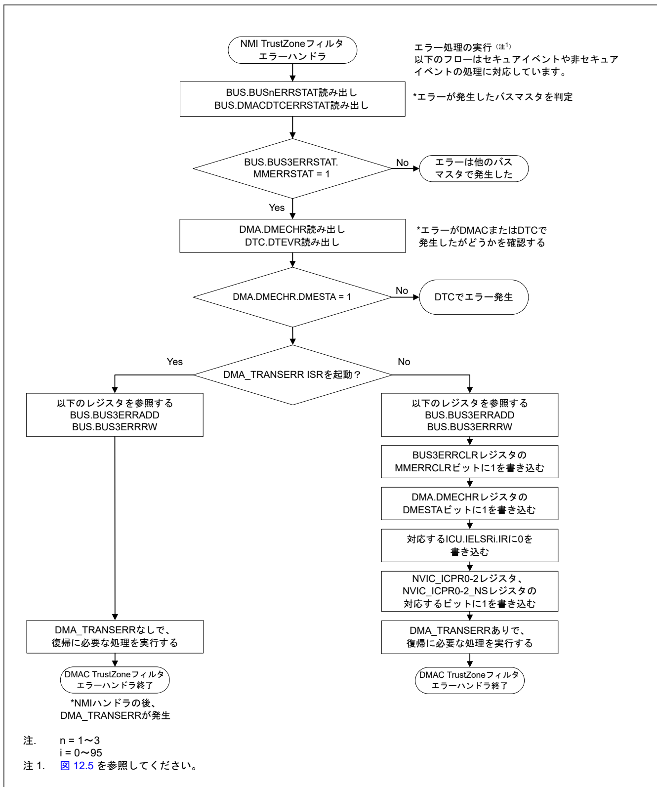
図 15.26 マスタ MPU エラーによる NMI ハンドラの処理
