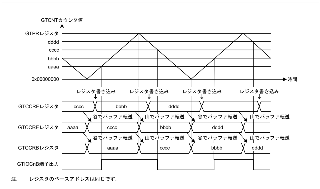
図 20.16 GTCCRB レジスタのダブルバッファ動作例（アウトプットコンペア、三角波、山と谷でバッファ動作、GTCCRB レジスタのコンペアマッチでトグル出力、周期の終わりで出力保持の場合）
