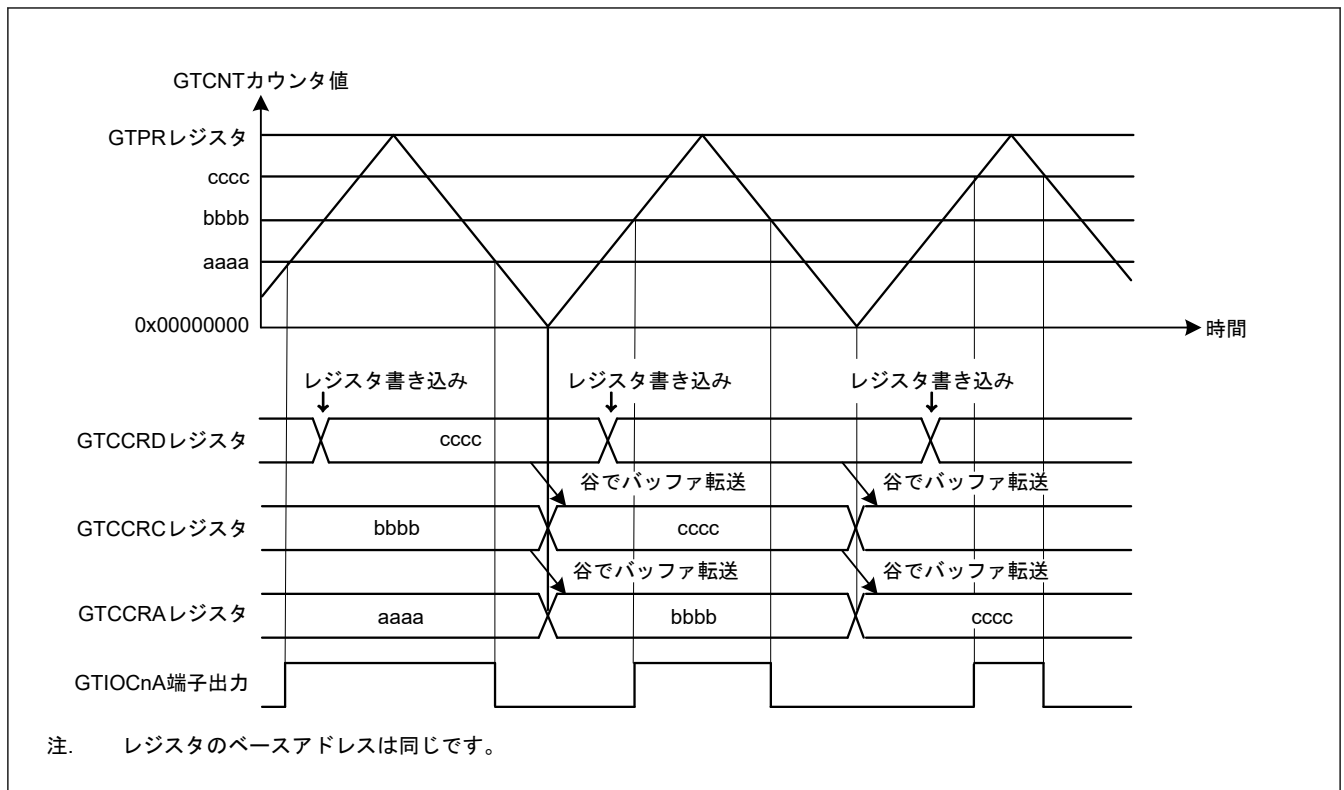
図 20.15 GTCCRA レジスタのダブルバッファ動作例（アウトプットコンペア、三角波、谷でバッファ動作、GTCCRA レジスタのコンペアマッチでトグル出力、周期の終わりで出力保持の場合）
