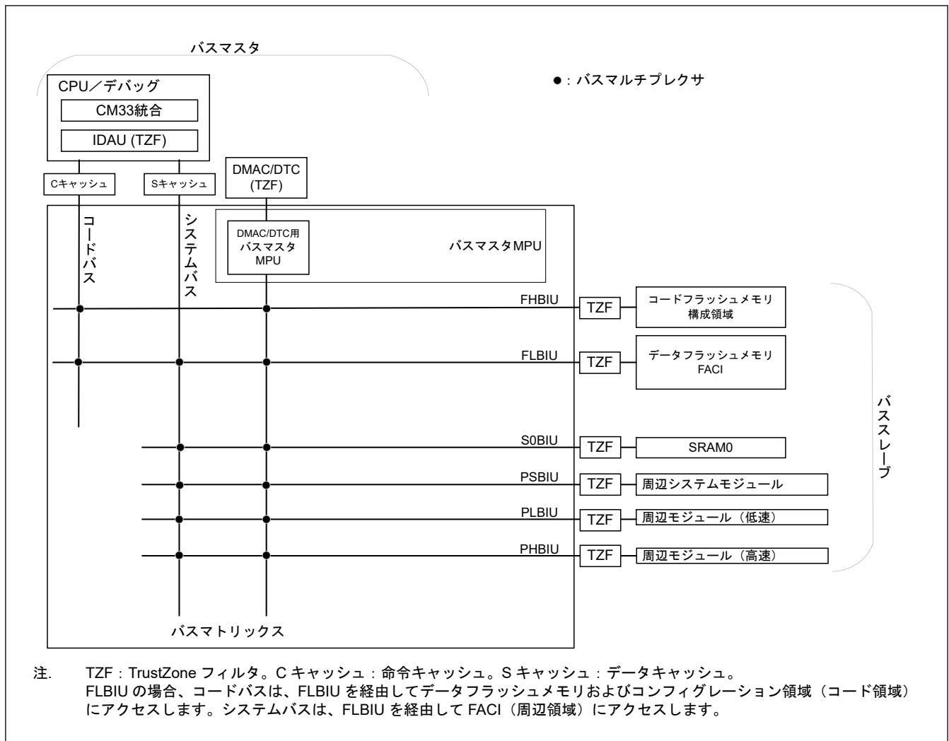
図 13.1 バス接続
