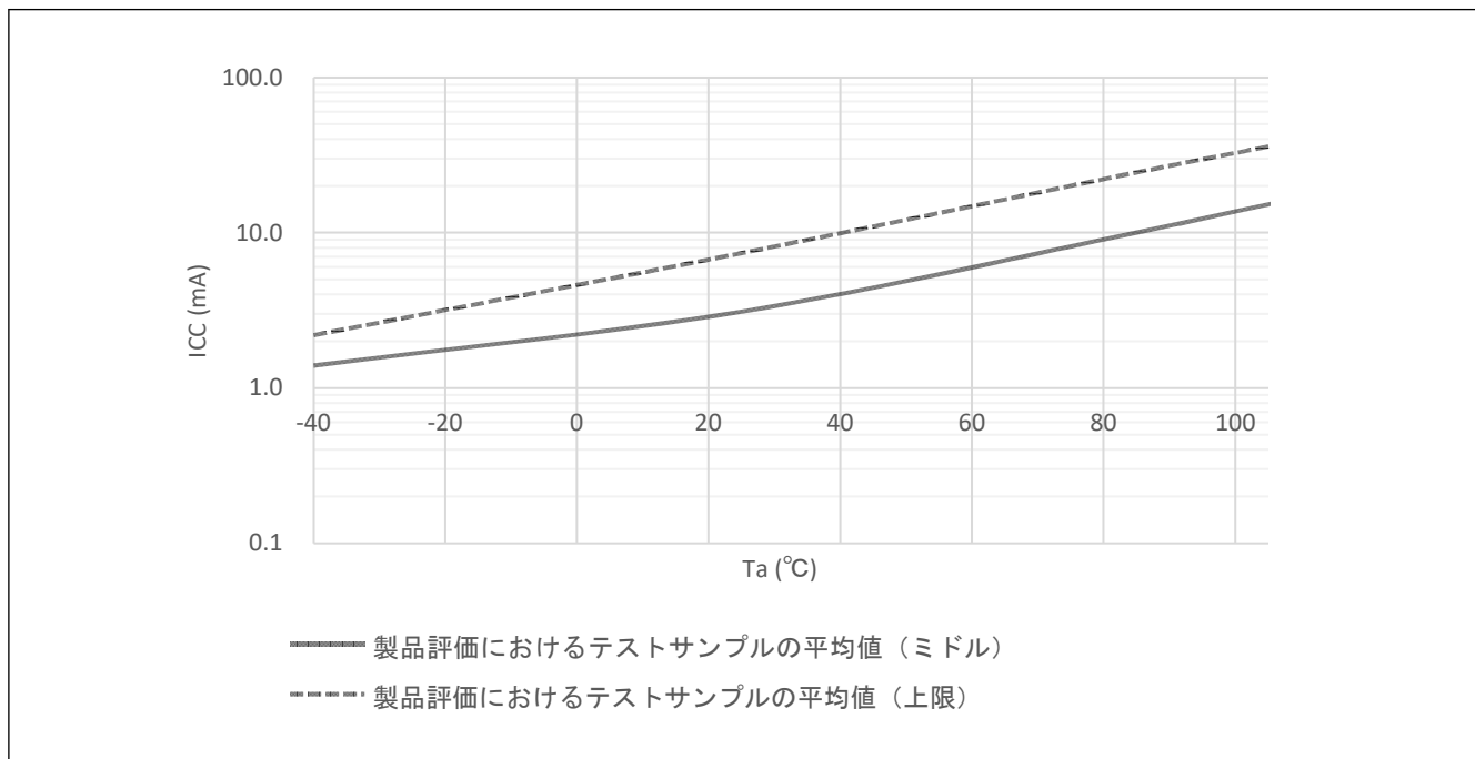
図 41.2 ソフトウェアスタンバイモードにおける温度依存性 (参考データ)
