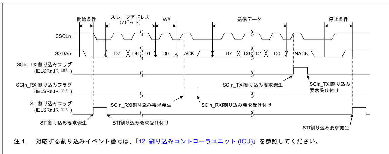
図 24.91 簡易 IIC モードにおけるマスタ送信の動作例 2 (7 ビットスレーブアドレス、ACK 割り込み、NACK 割り込み使用時)
