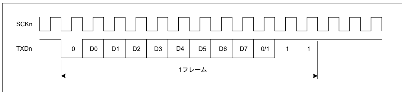
図 27.5 調歩同期式モードにおける出カクロックと送信データの位相関係 (SMR.CHR = 0、PE = 1、MP = 0、および STOP = 1 の場合)
