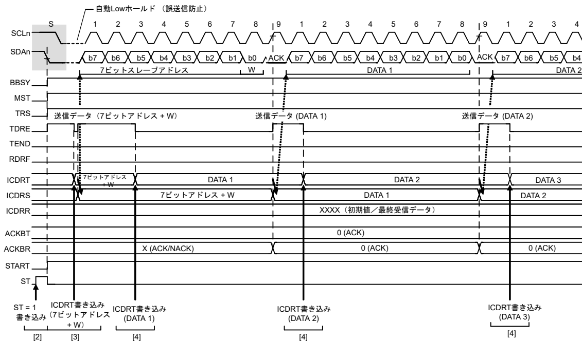
図 28.7 マスタ送信の動作タイミング (1) (7 ビットアドレスフォーマット)
