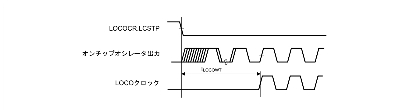
図 43.9 LOCO クロック発振開始タイミング
