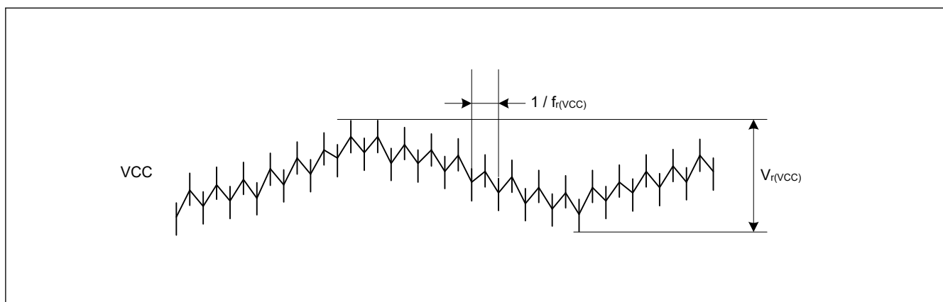
図 43.6 リップル波形
