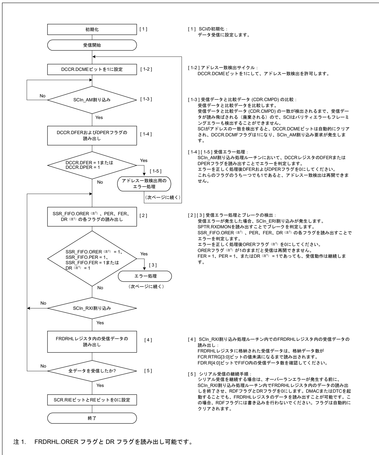
図 27.25 調歩同期式モードにおけるシリアル受信のフローチャート例 (FIFO 選択、アドレス一致検出有効時) (1)
