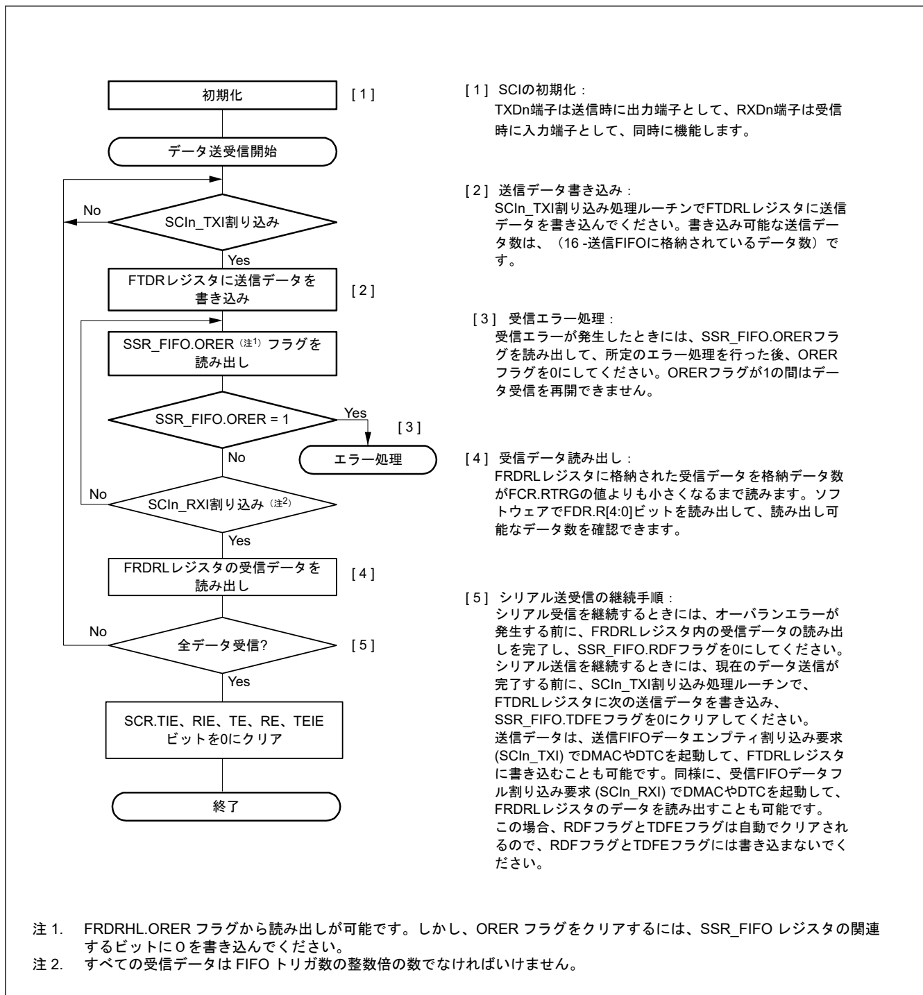
図 27.73 クロック同期式モードにおけるシリアル同時送受信動作のフローチャート例 (FIFO 選択時)
