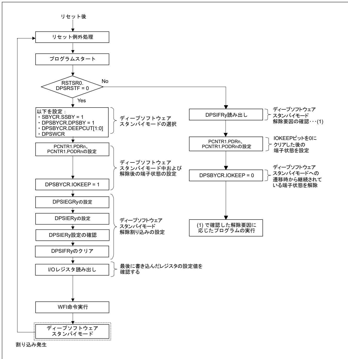
図 10.11 ディープソフトウェアスタンバイモード使用時のフローチャート例
