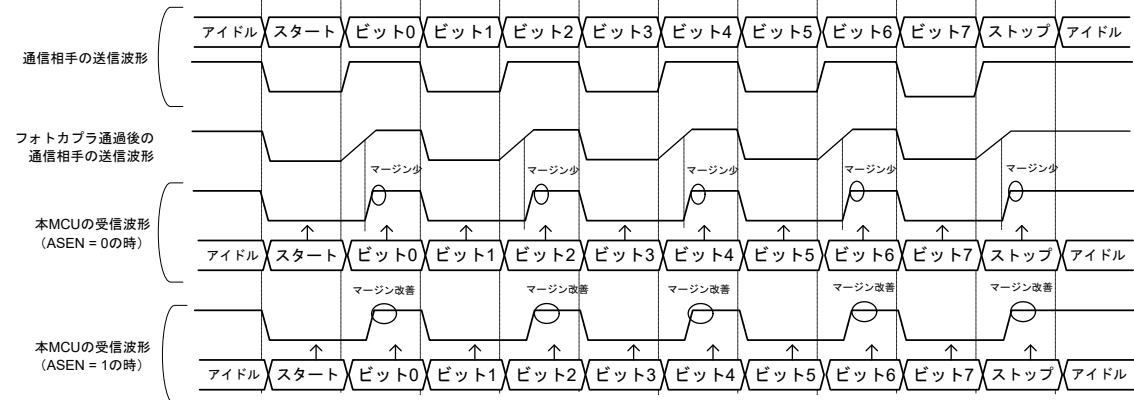
図 27.30 受信サンプリングタイミング調整機能による受信マージン向上の例
