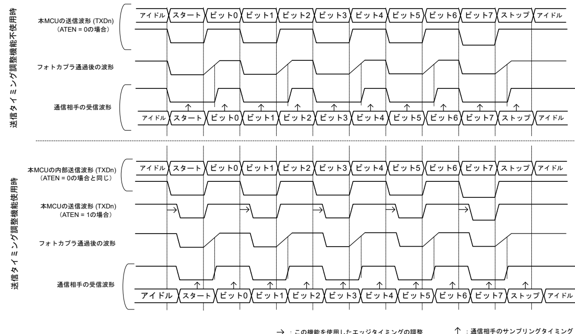
図 27.34 フォトカプラを経由する送信波形の説明
