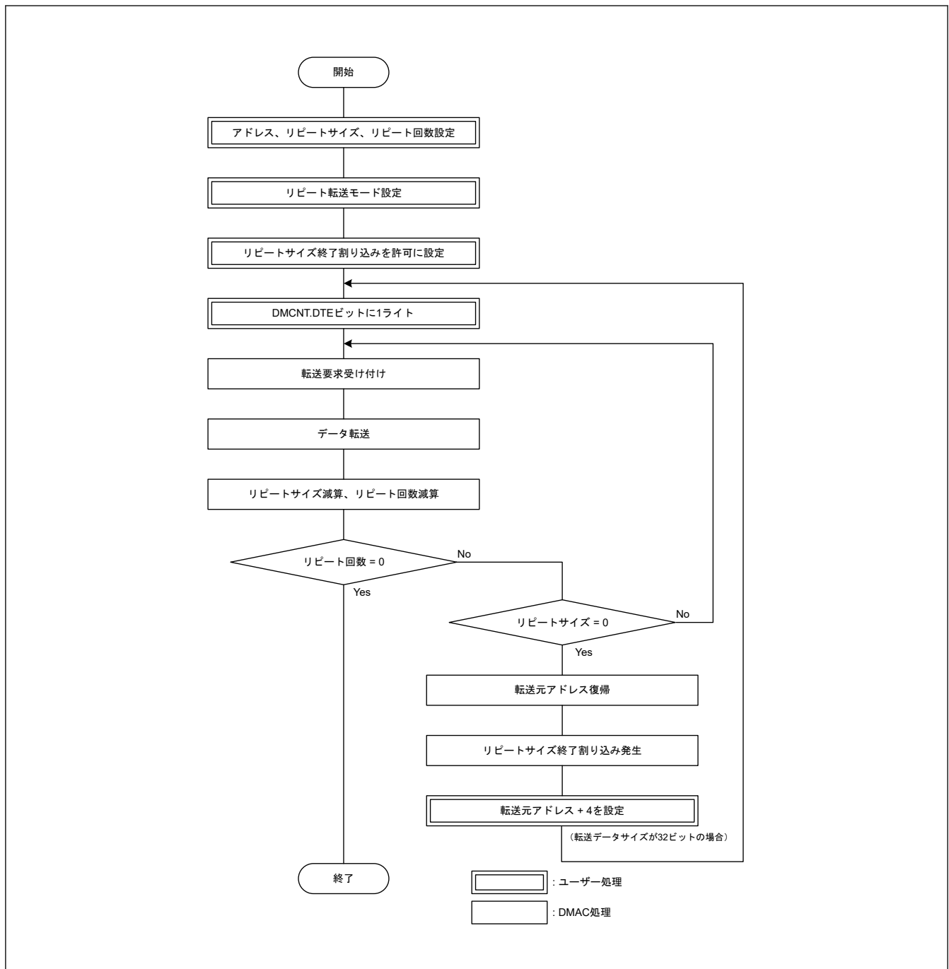
図 16.13 リピート転送モードにおけるオフセット加算による XY 変換フロー
