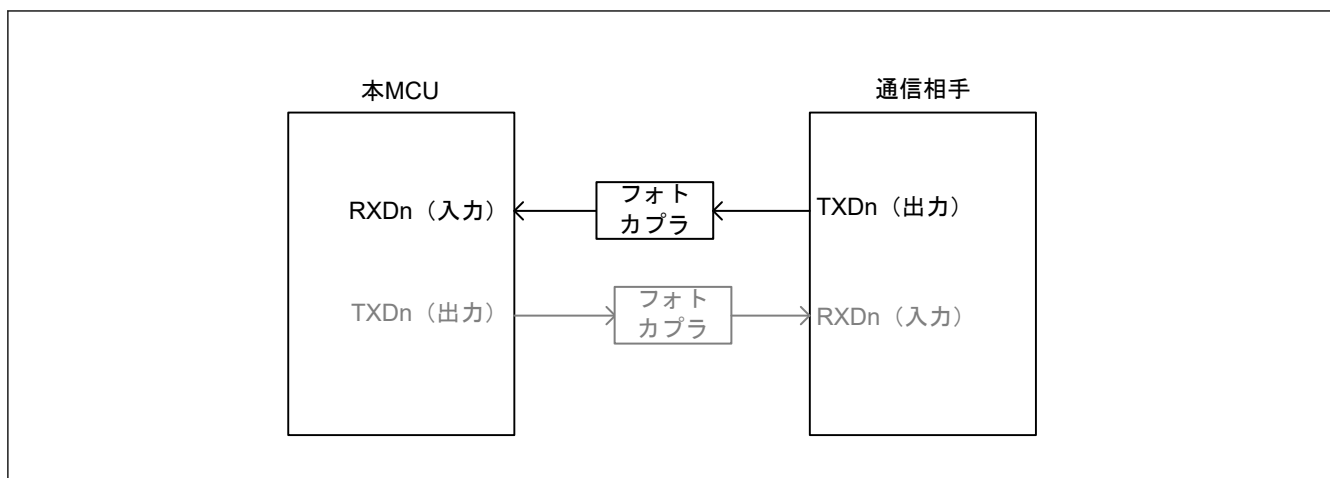
図 27.28 フォトカプラを通過する受信のブロック図イメージ
