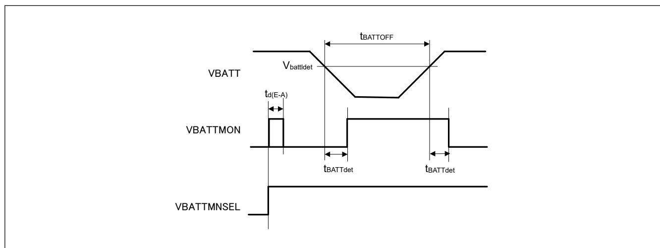
図 43.54 バッテリバックアップ機能特性
