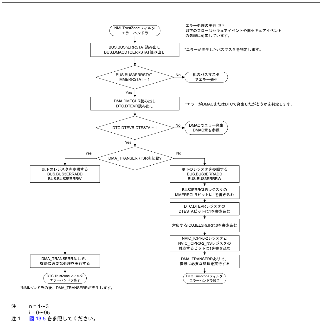
図 17.16 マスタ MPU エラーによる NMI ハンドラでの処理
