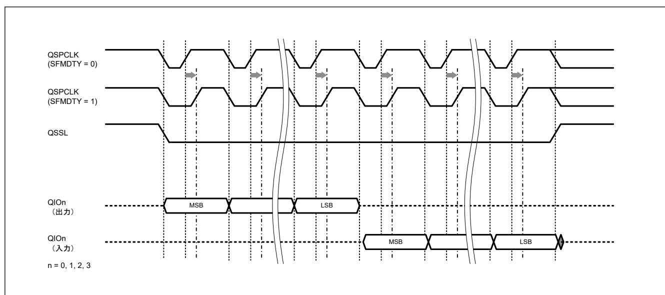
図 31.10 PCLKA を 3 通倍した場合の SFMDTY ビットを使用した QSPCLK 信号デューティー比補正例
