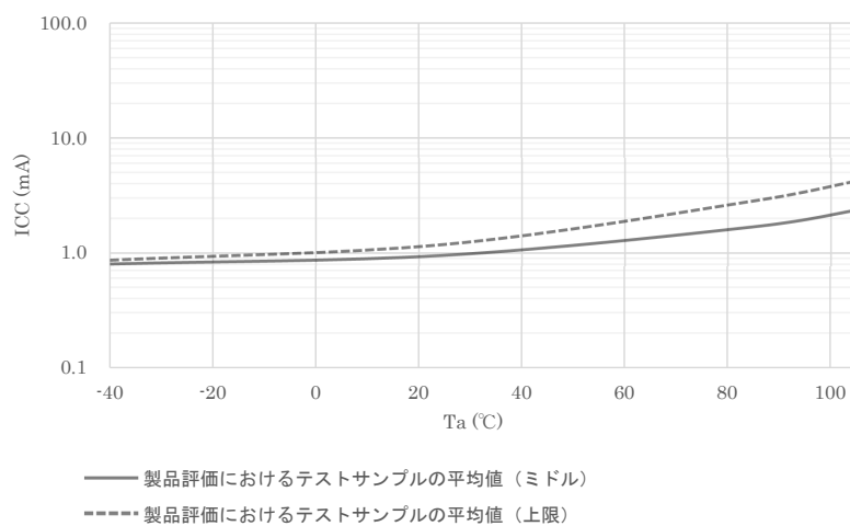
図 43.2 ソフトウェアスタンバイモード時の温度依存性（参考データ）
