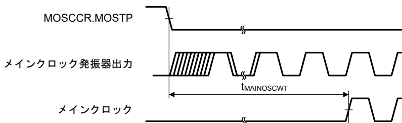
図 43.8 メインクロック発振開始タイミング
