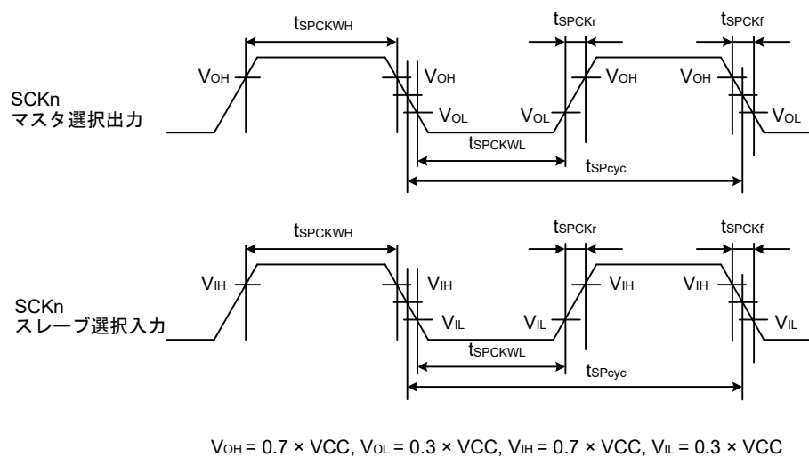
図 43.27 SCI 簡易 SPI モードクロックタイミング
