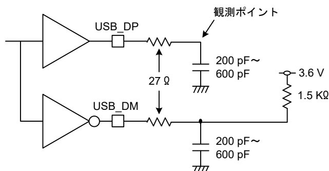
図 43.44 Low-speed モードにおける測定回路
