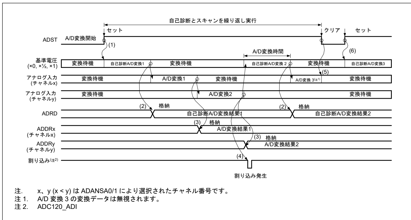
図 35.13 連続スキャンモードの基本動作例（アナログ入力（チャネル x、y）選択+自己診断）
