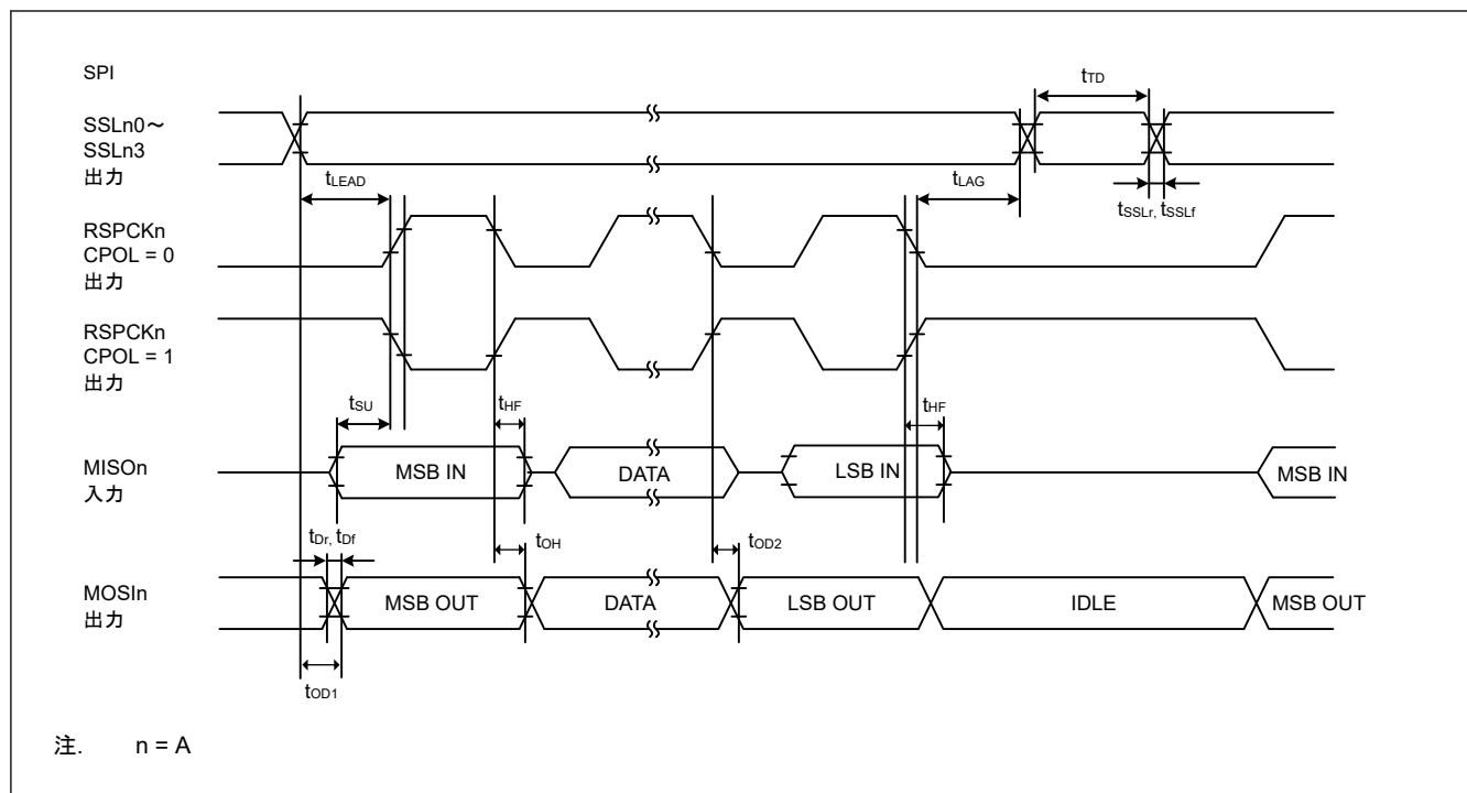
図 43.35 CPHA = 0 でビットレートが PCLKA/2 に設定されている場合におけるマスタの SPI タイミング
