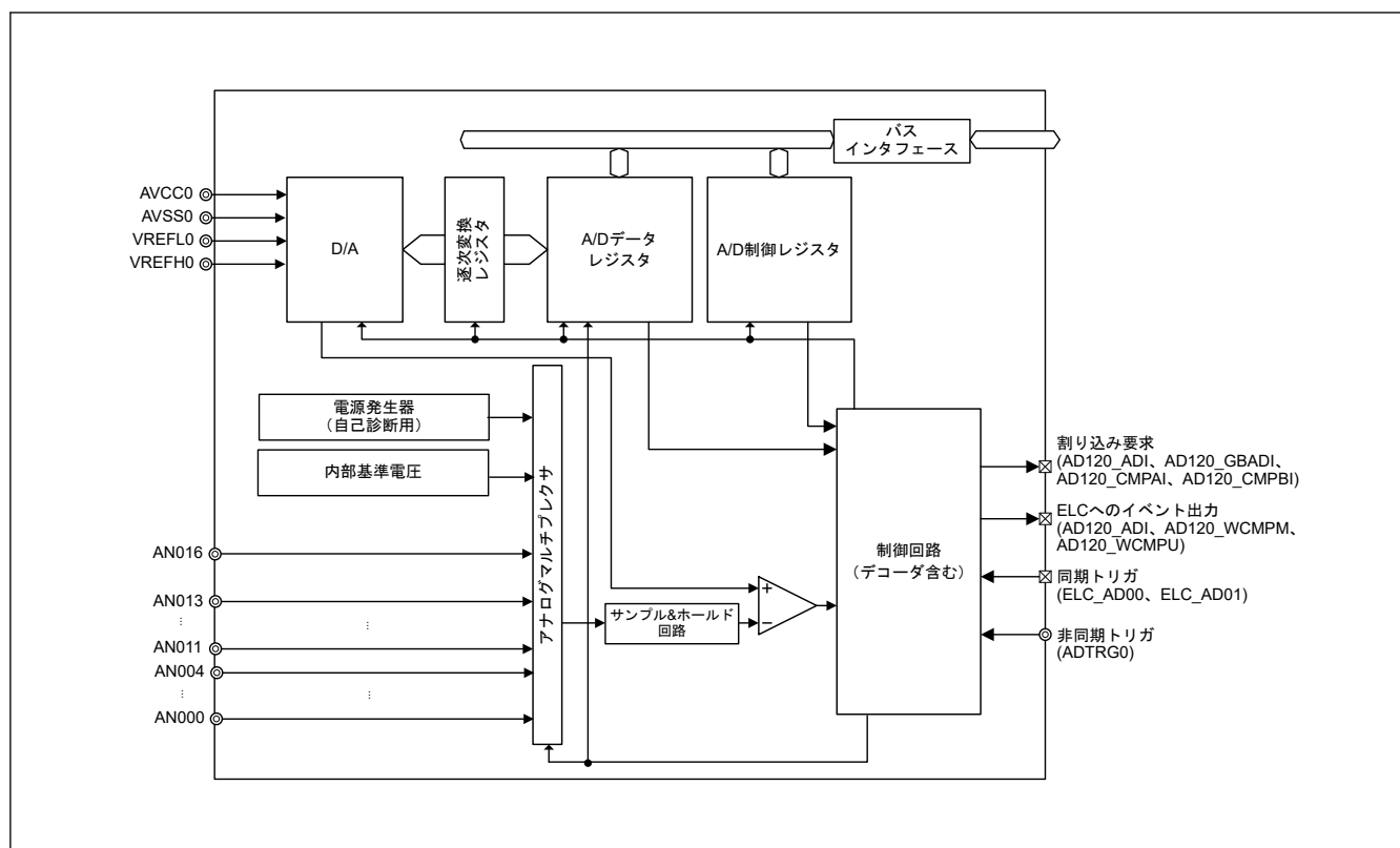
図 35.1 ADC12 のブロック図
