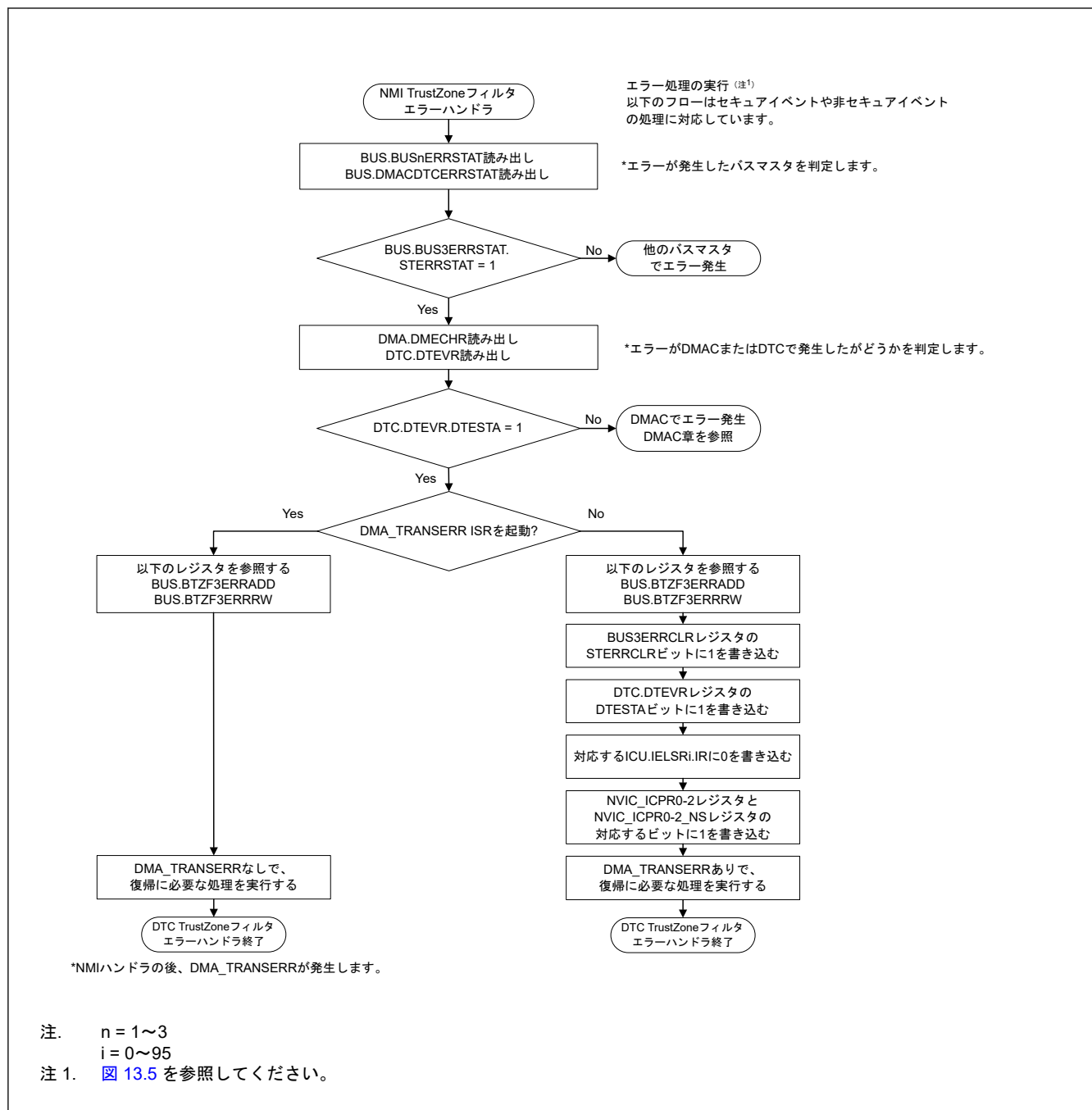
図 17.15 スレーブ TrustZone フィルタエラーの NMI ハンドラにおける処理
