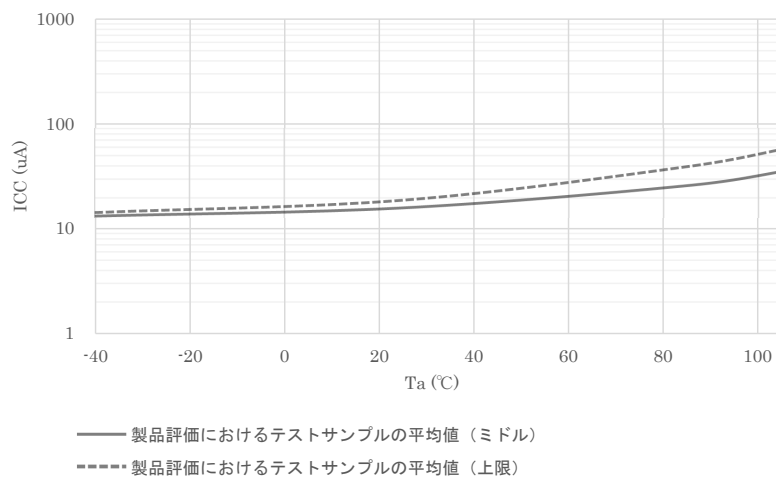
図 43.3 ディープソフトウェアスタンバイモード時の温度依存性、スタンバイ SRAM および USB レジューム検出部への電源供給あり（参考データ）
