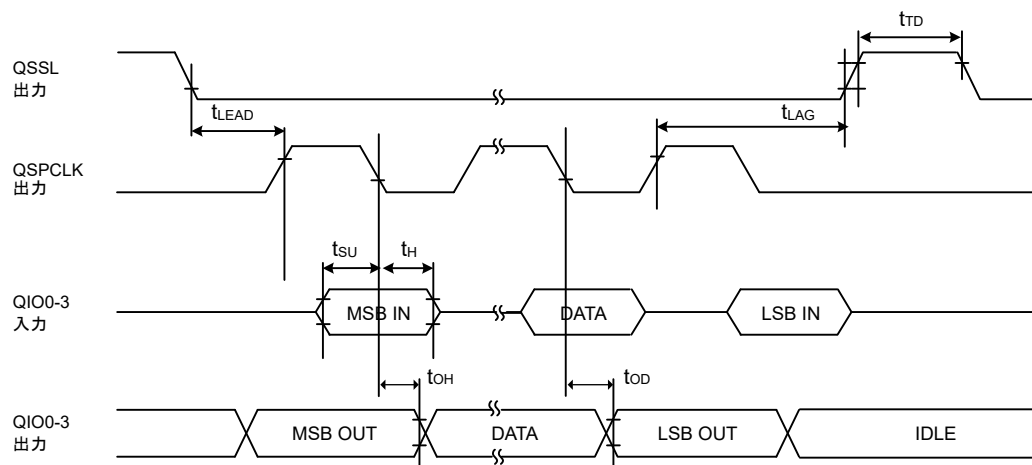
図 43.41 送受信タイミング
