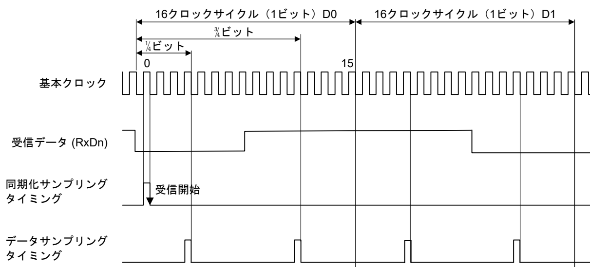
図 27.56 マンチェスタモードでのデータ受信サンプリングタイミング
