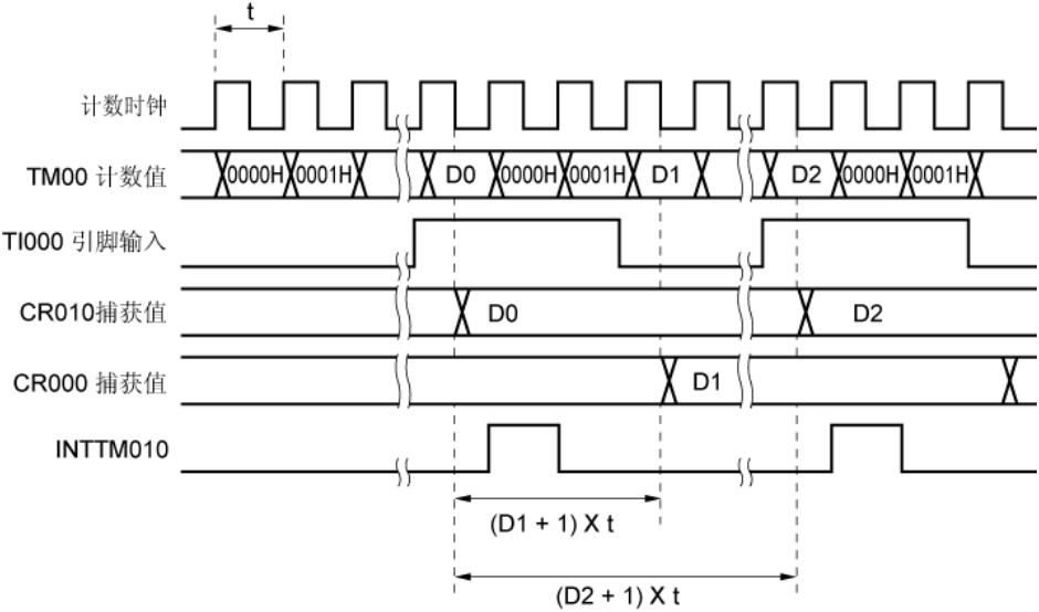
图 6-26. 通过重启进行测量脉冲宽度的时序（指定上升沿有效）
