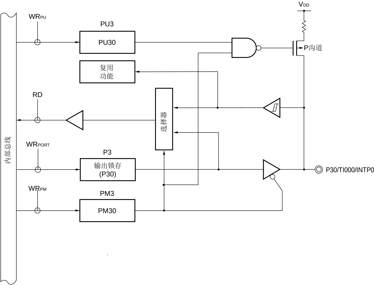
图 4-4 P30 的框图
