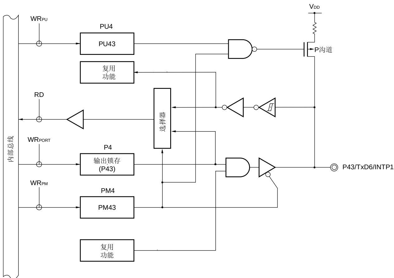
图 4-11 P43 的框图
