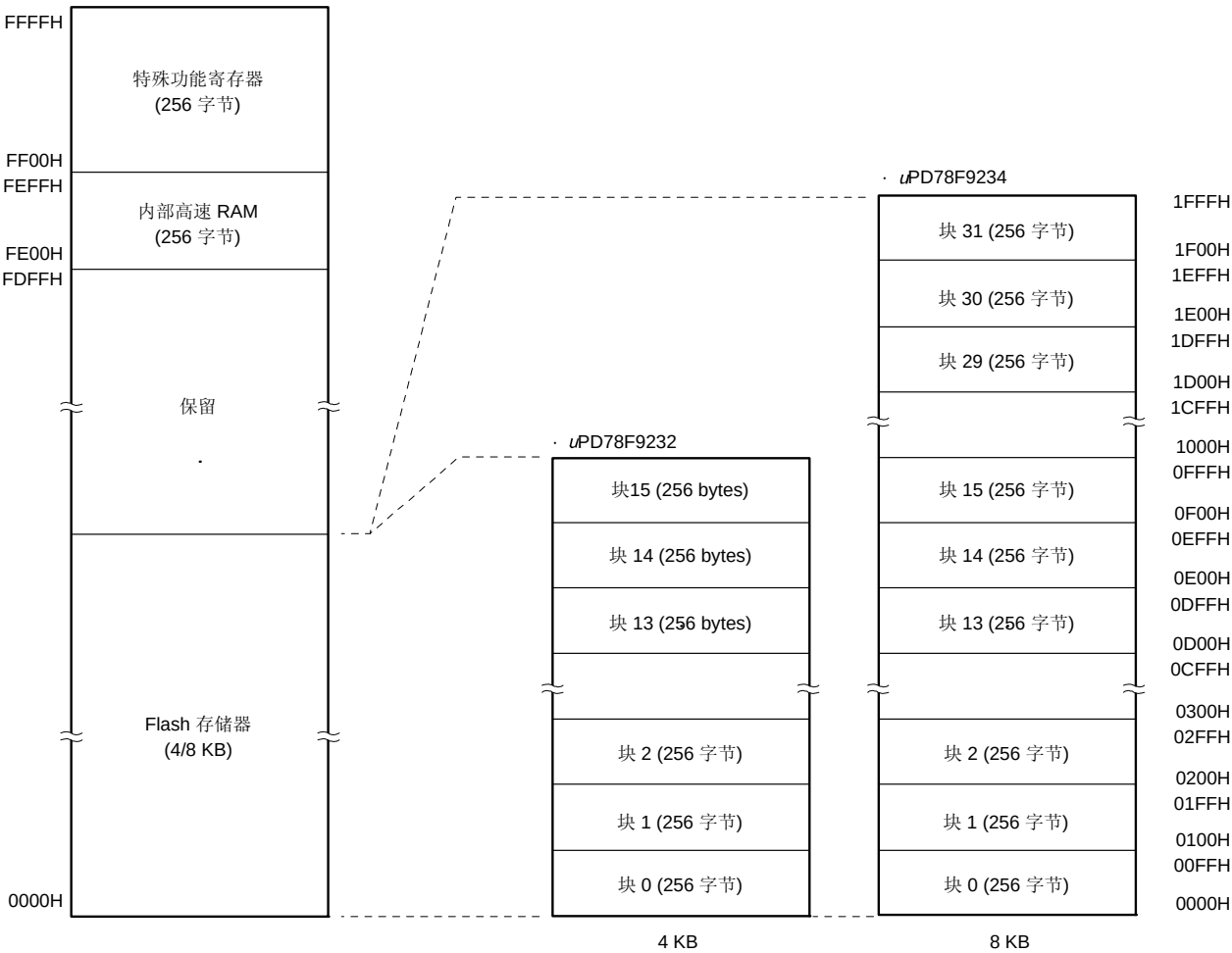
图 19-1. Flash 存储器图表
