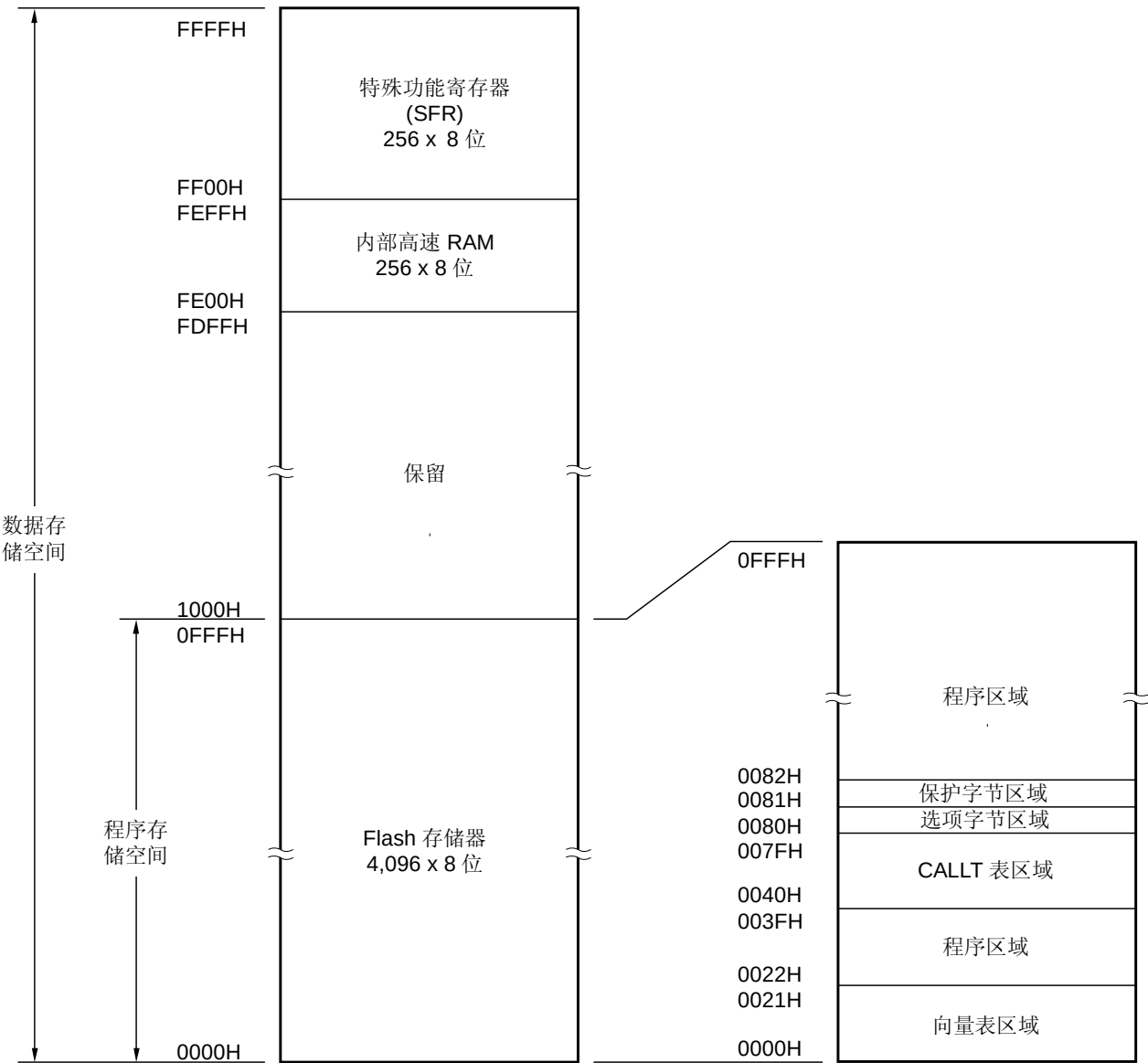
图 3-1. 存储空间映射图 (μPD78F9232)
