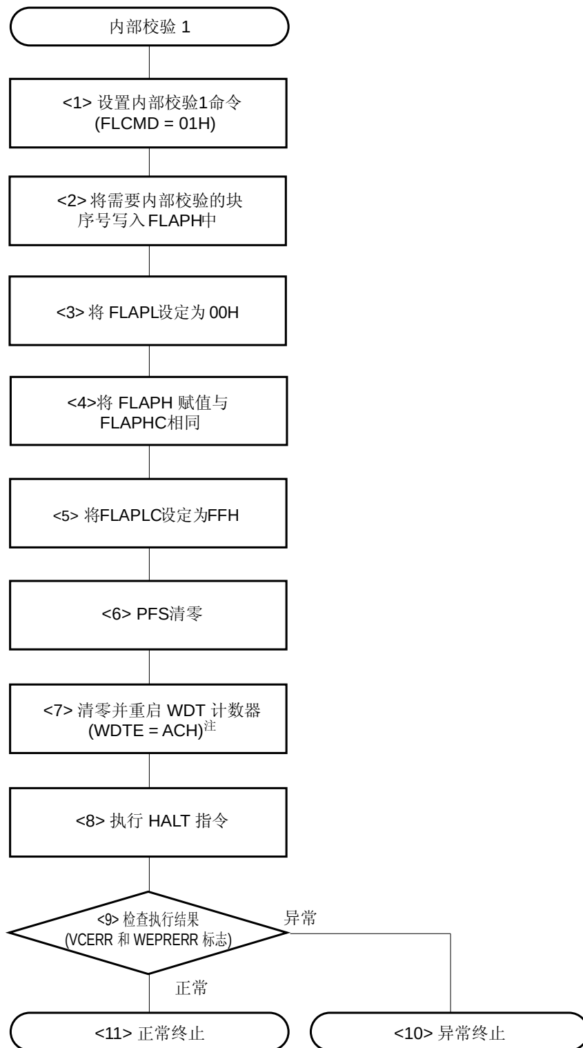
图 19-23. 自编程模式下内部校验 1 流程
