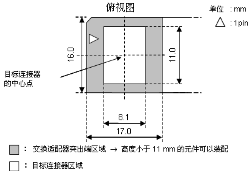
图 B-1. 当使用 78K0S/Kx1+ 仿真探头时 (30 脚 MC 封装)
