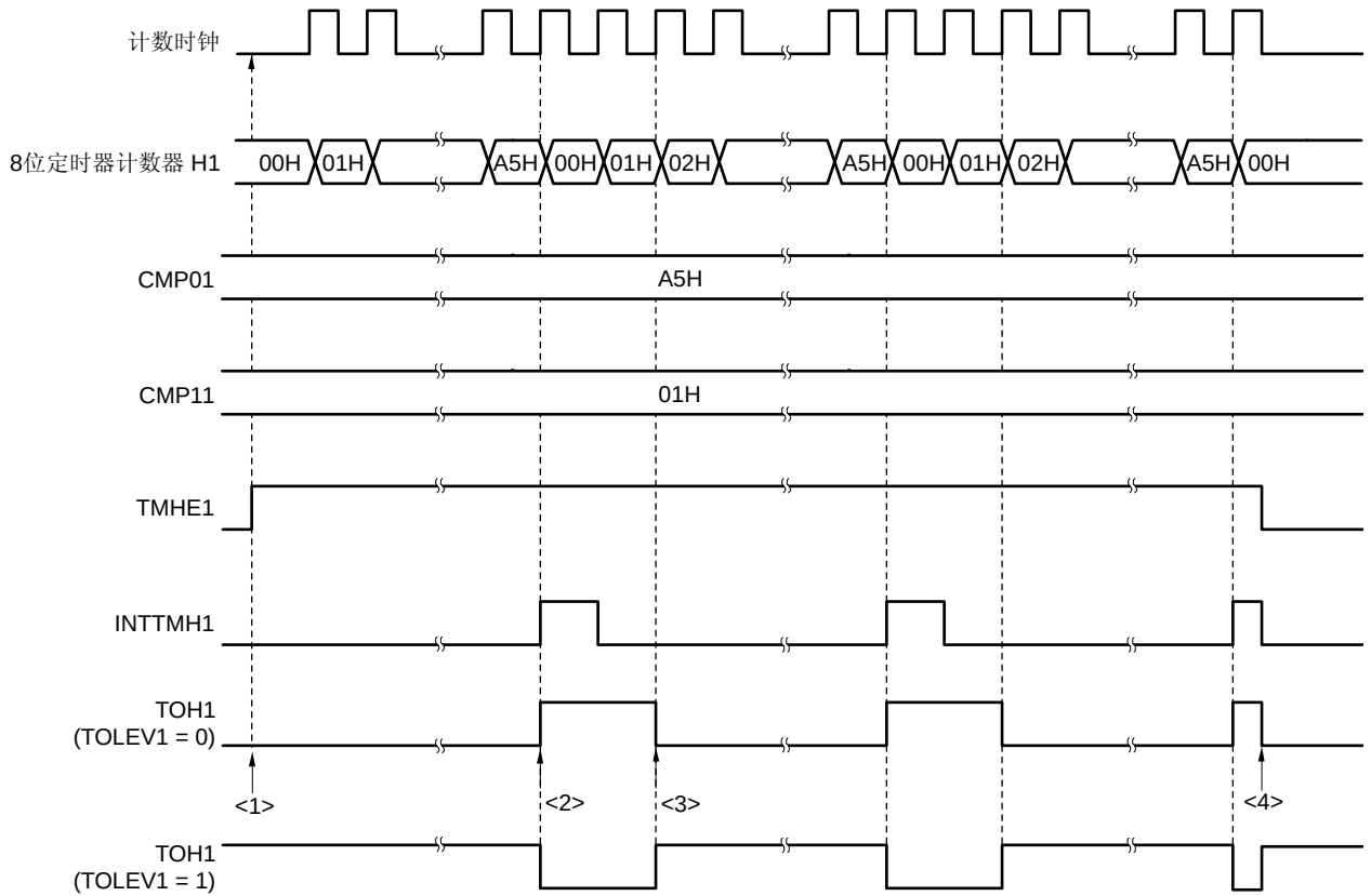
(a) 基本操作 ( 00H < \text{CMP11} < \text{CMP01} < FFH )
