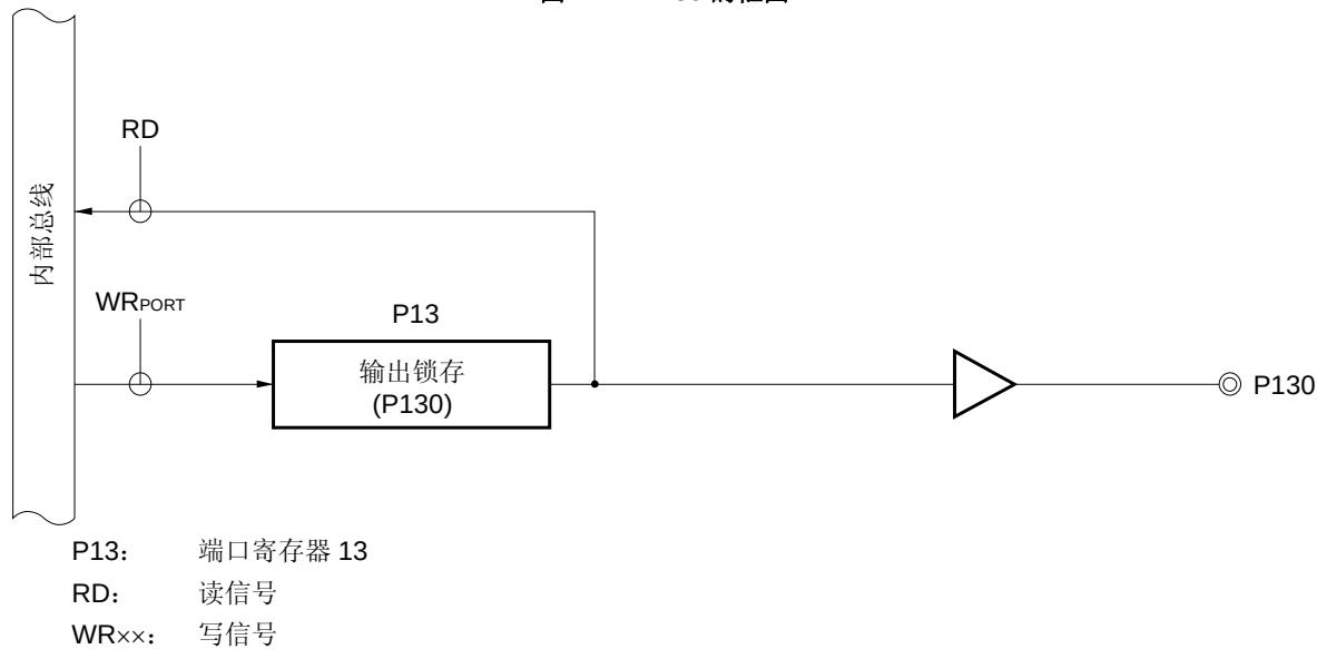
图 4-14 P130 的框图
