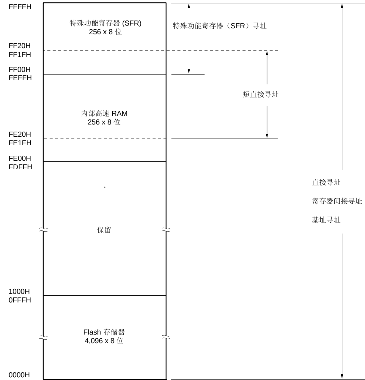
图 3-3. 数据存储寻址（μPD78F9232）
