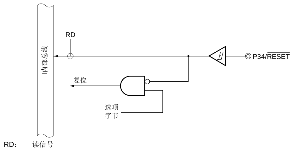
图 4-7 P34 的框图
