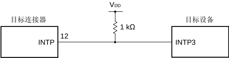
图20-2. 当目标系统未使用INTP3引脚时的线路连接
