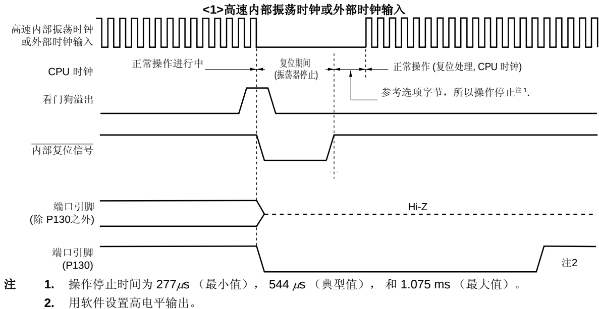
图 15-3. 由看门狗定时器溢出引起的复位时序
