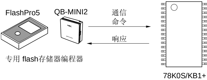
图 19-7. 通讯命令
