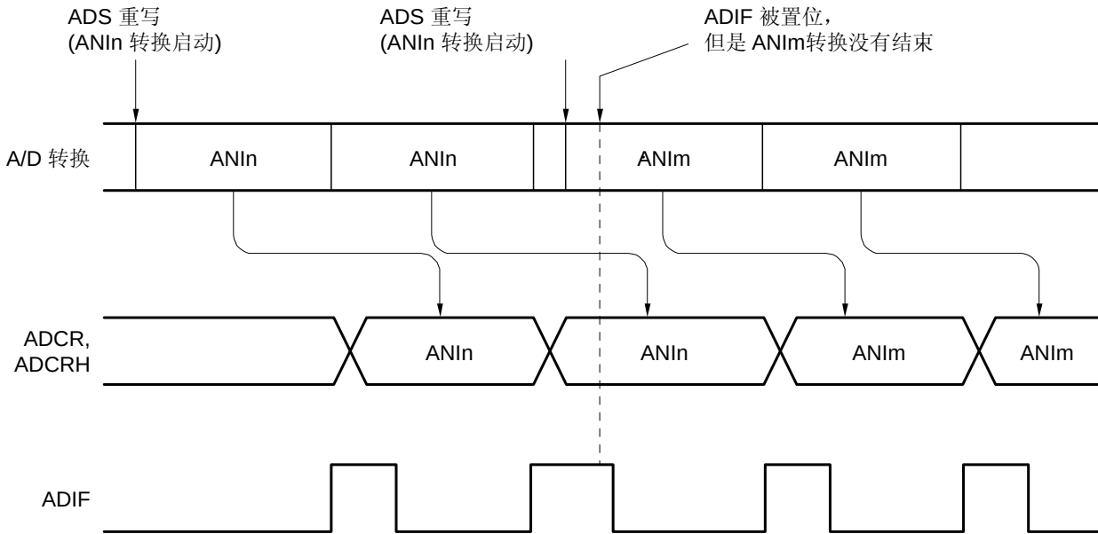
图 10-20. A/D 转换结束中断请求产生的时序
