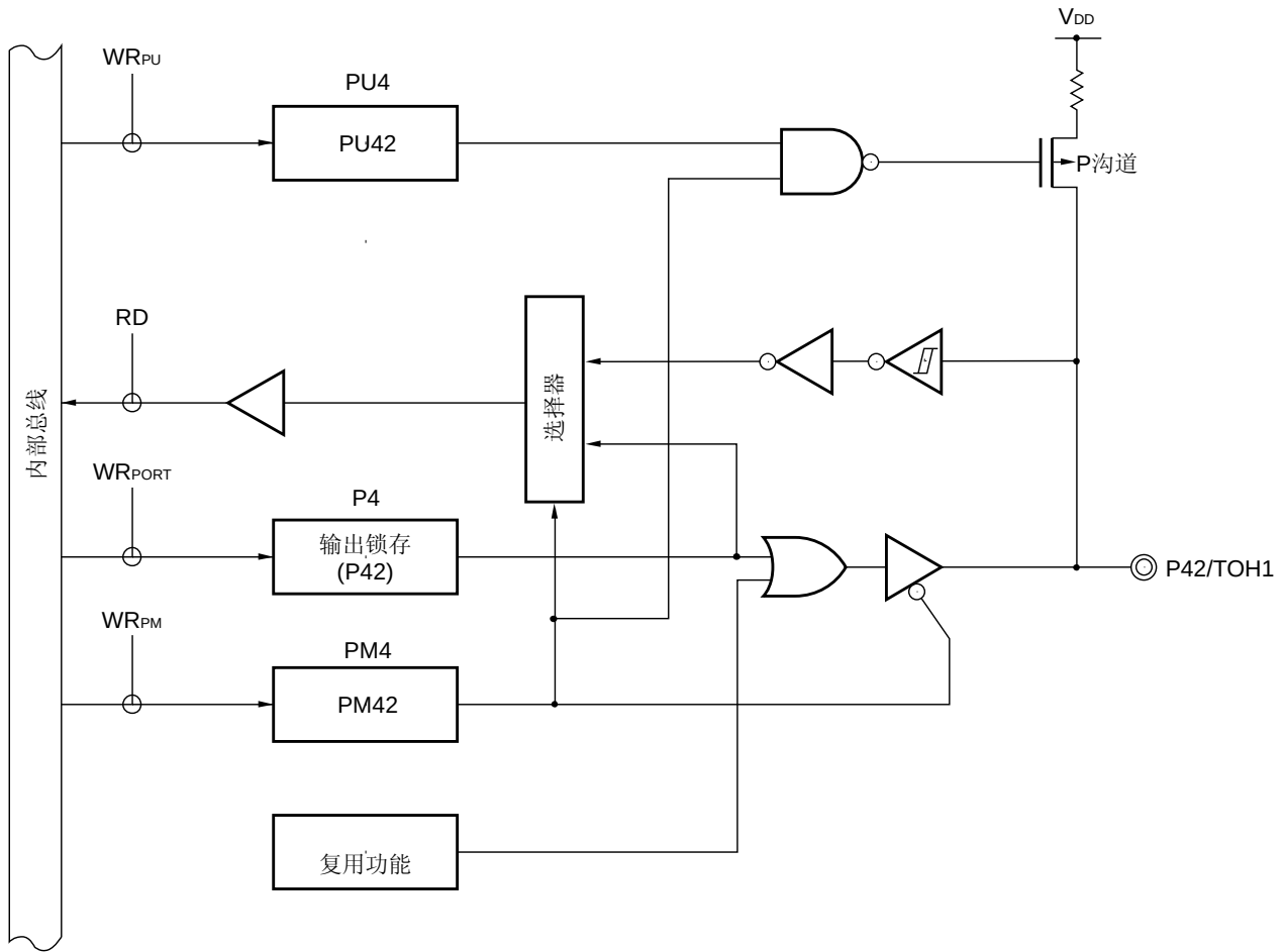
图 4-10 P42 的框图
