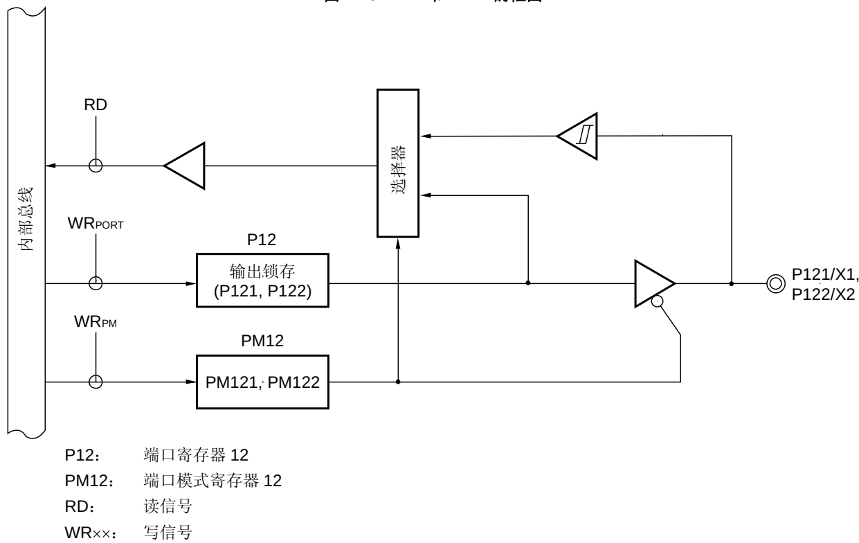
图 4-13 P121 和 P122 的框图
