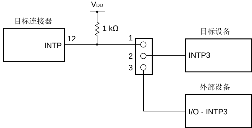
图20-4. QB-MINI2用来调试且INTP3引脚的调试只能通过实际设备来执行时的线路连接
