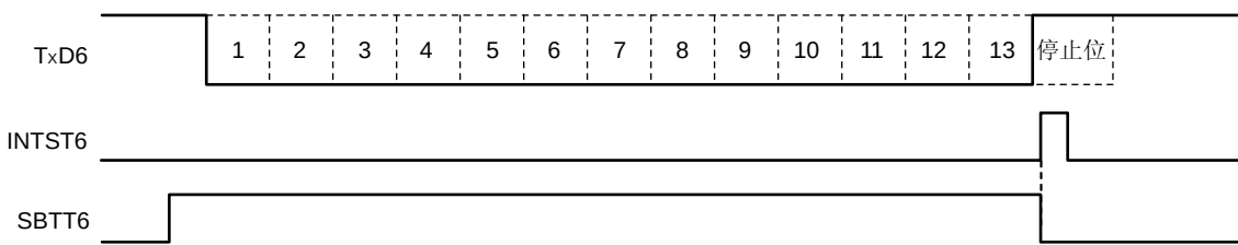
图 11-22. SBF 发送
