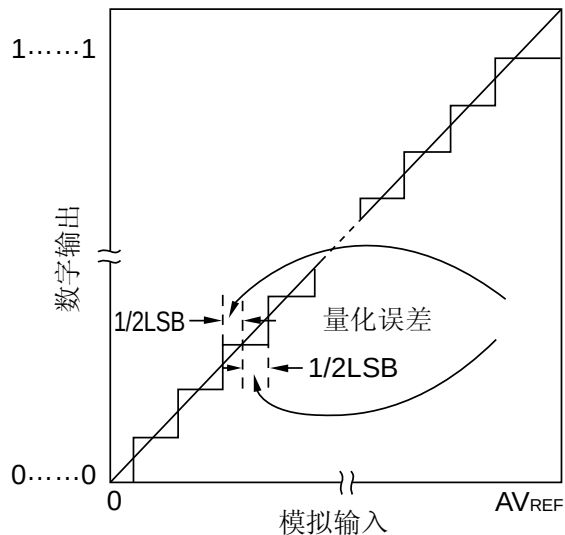
图 10-14. 量化误差
