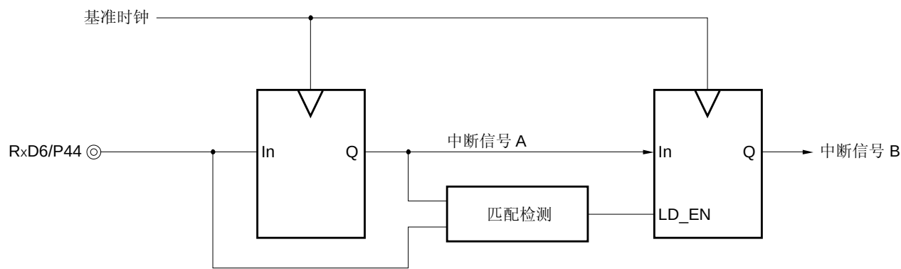
图 11-21. 噪声过滤器电路
