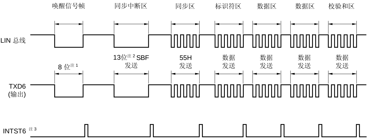
图 11-1. LIN 发送操作
