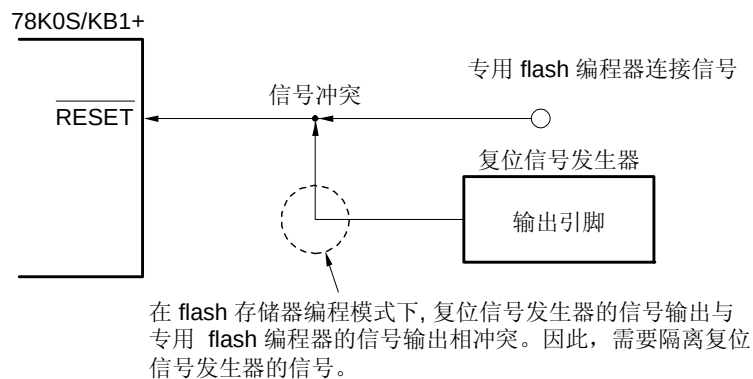
图 19-6. 信号冲突 (RESET 引脚)
