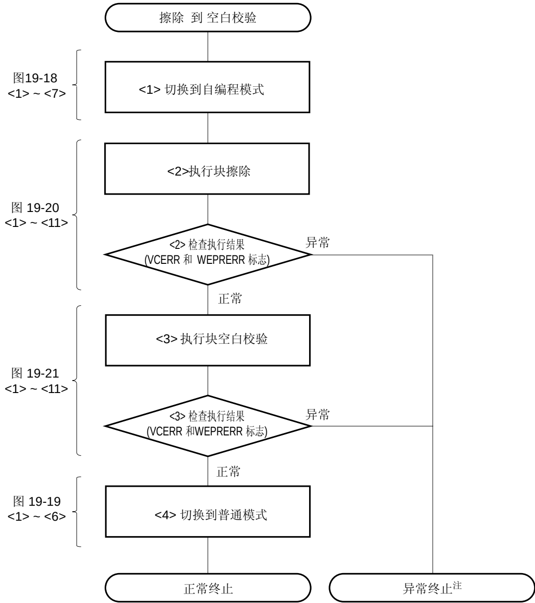
图 19-25 最短命令执行时间的操作流程（从擦除到空白检验）
