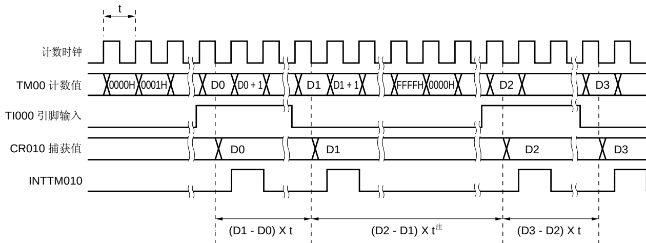
图 6-20. 通过自由运行计数器和一个捕获寄存器（双沿有效）测量脉冲宽度的时序图
