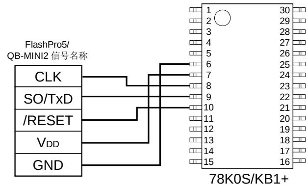
图 19-3. 和 FlashPro5/QB-MINI2 的连线图（30 引脚产品）
