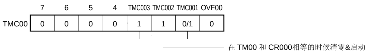
(c) 16 位定时器模式控制寄存器 00 (TMC00)
