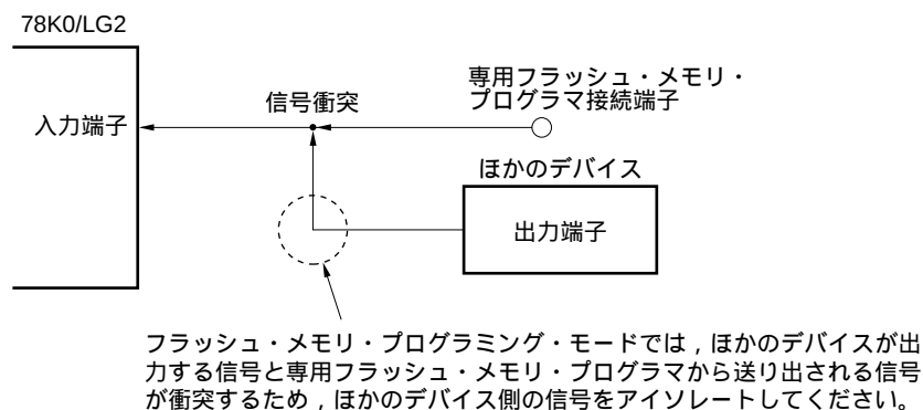
図27 - 9 信号の衝突（シリアル・インタフェースの入力端子）
