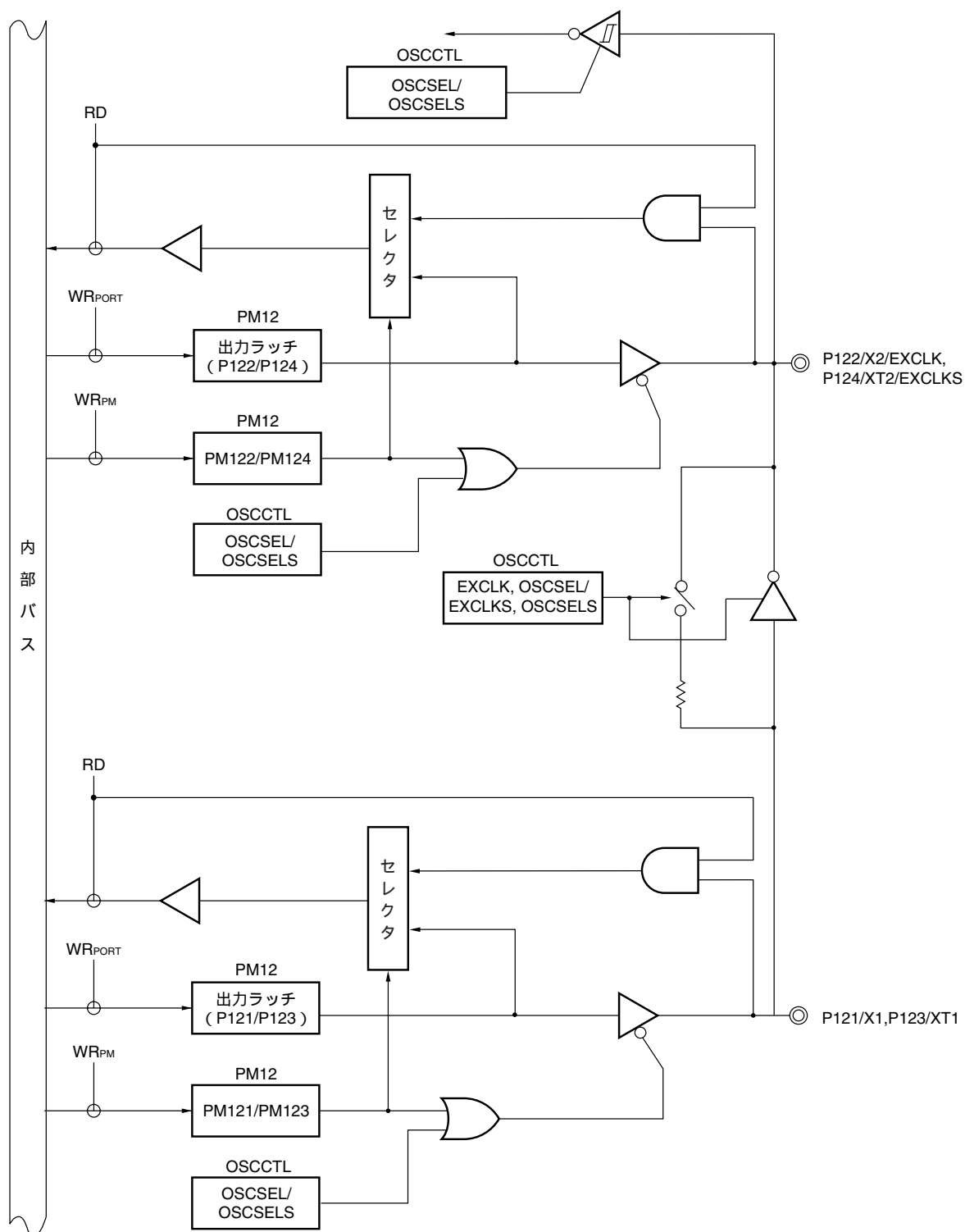
図5 - 19 P121-P124のブロック図
