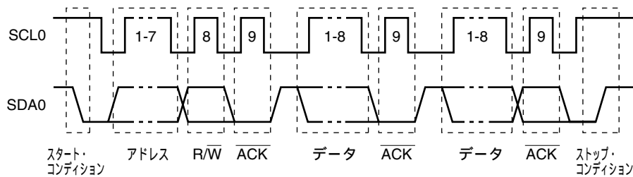
図17-13 I 2 Cバスのシリアル・データ転送タイミング
