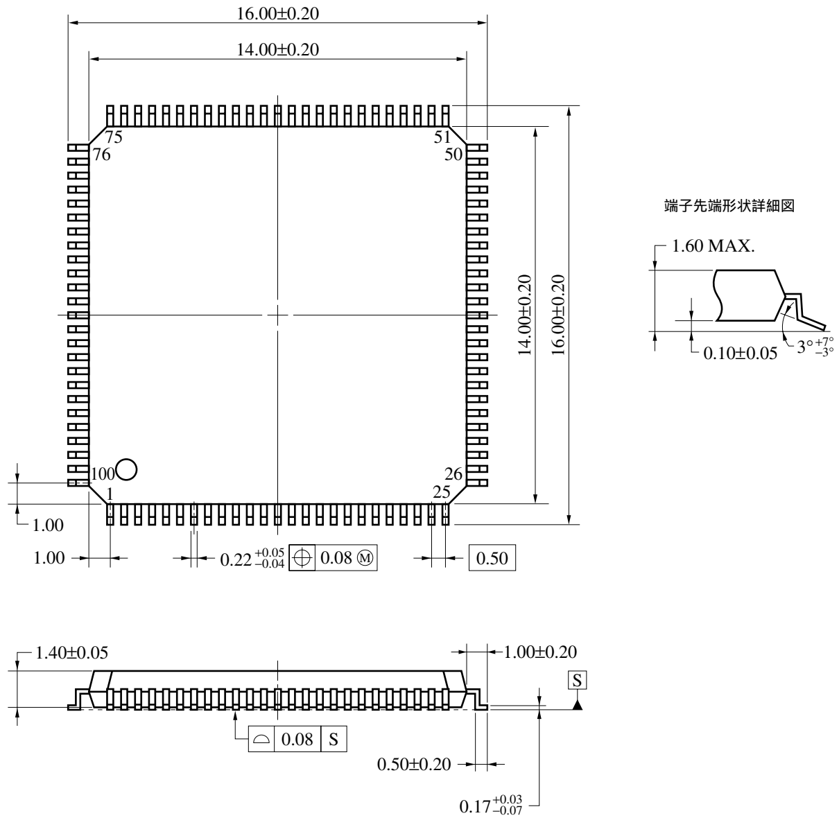
100ピン・プラスチック LQFP (ファインピッチ)(14x14) 外形図 (単位: mm)
