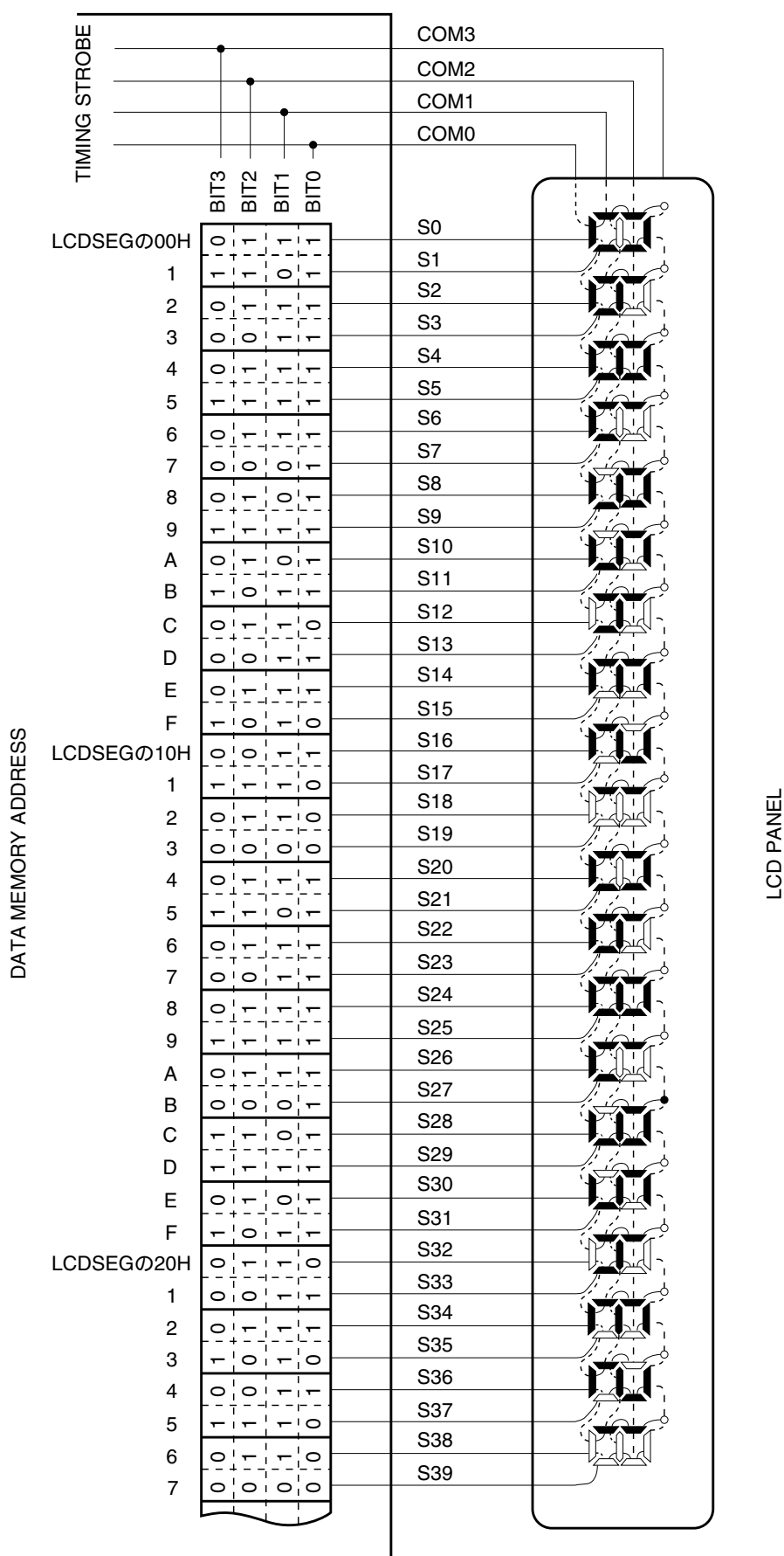
図18 - 25 4時分割LCDパネルの結線例
