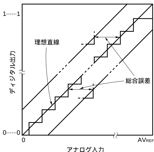
図13 - 14 総合誤差
