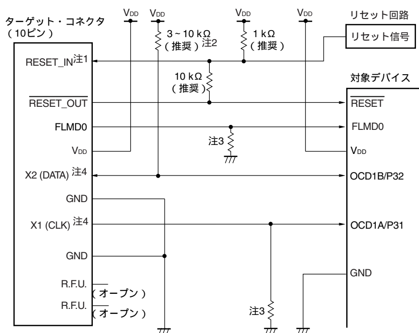
図28 - 2 QB-78K0MINIまたはQB-MINI2とμ PD78F0397Dの接続例 (OCD1A/P31, OCD1B/P32使用時)
