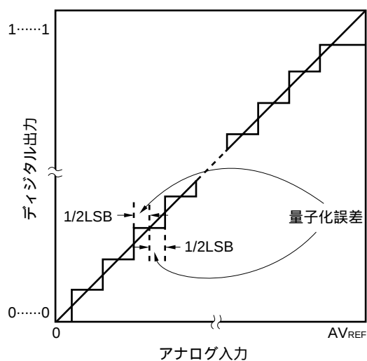
図13 - 15 量子化誤差
