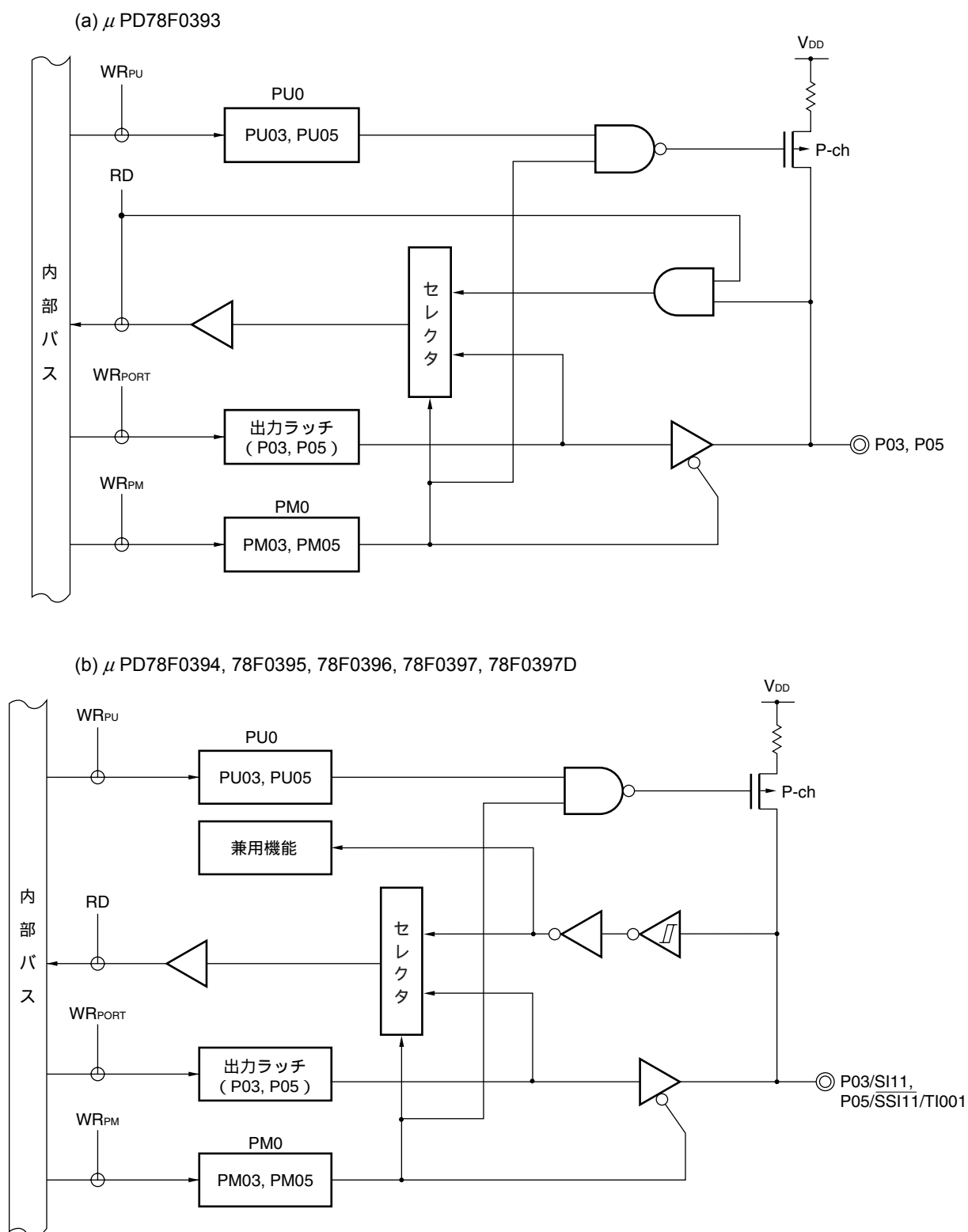
図5 - 5 P03, P05のブロック図
