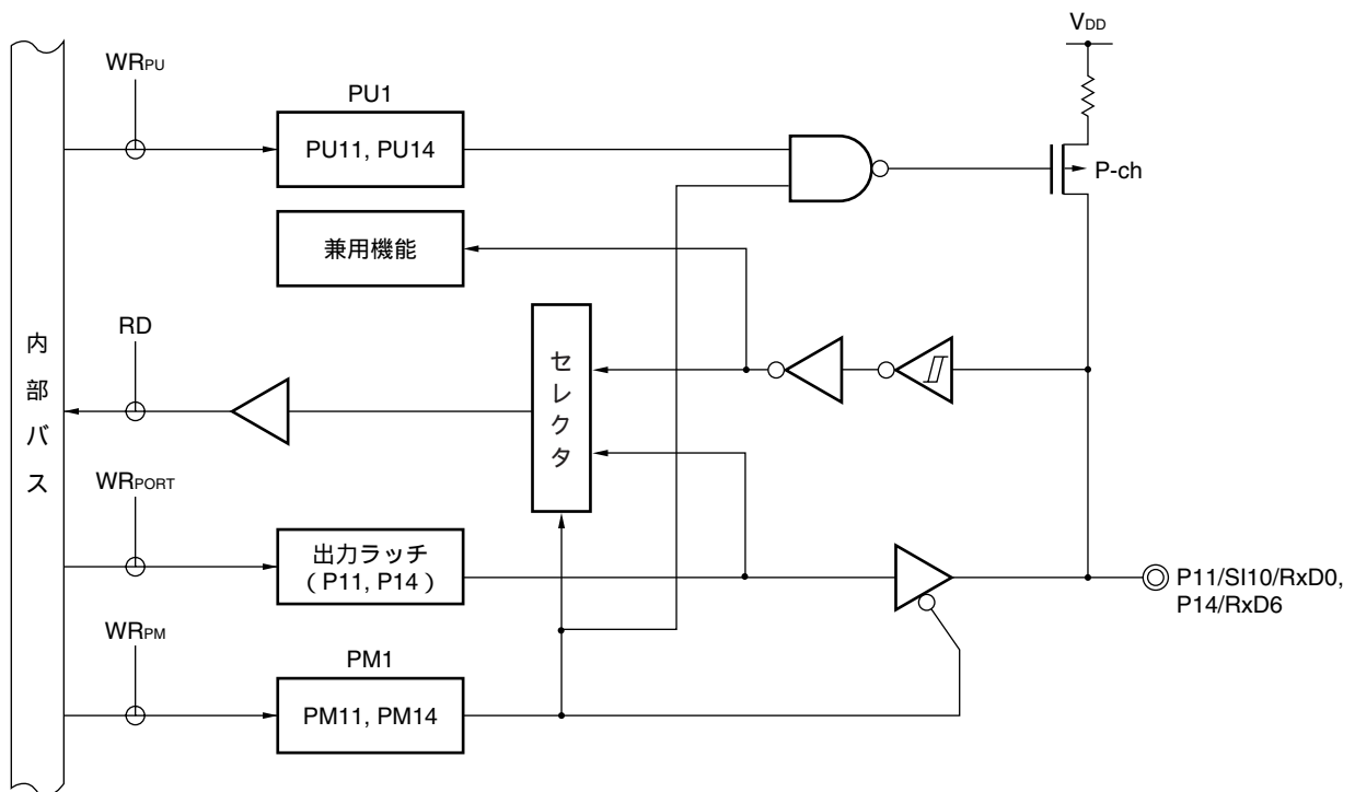
図5 - 9 P11, P14のブロック図
