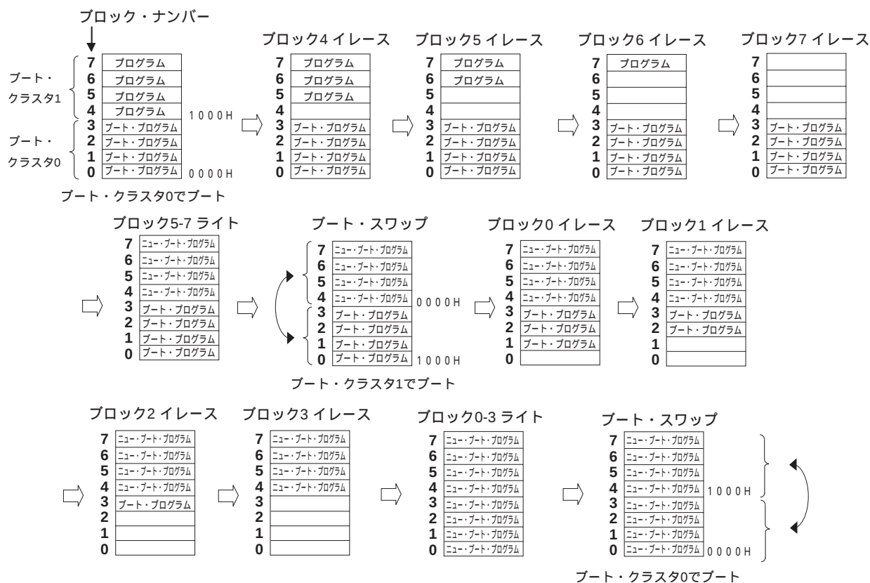
図27 - 18 ブート・スワップの実行例
