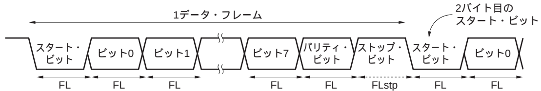
図15 - 26 連続送信時のデータ・フレーム長
