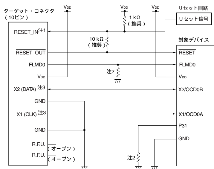
図28 - 1 QB-78K0MINIまたはQB-MINI2と \mu PD78F0397Dの接続例 (OCD0A/X1, OCD0B/X2使用時)
