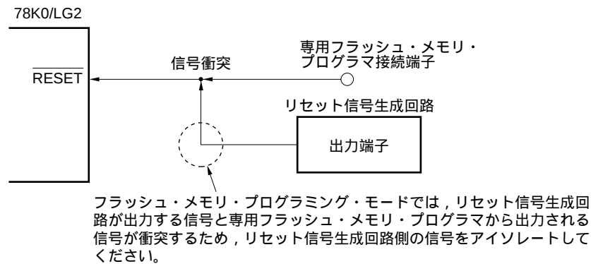
図27 - 11 信号の衝突 (RESET端子)
