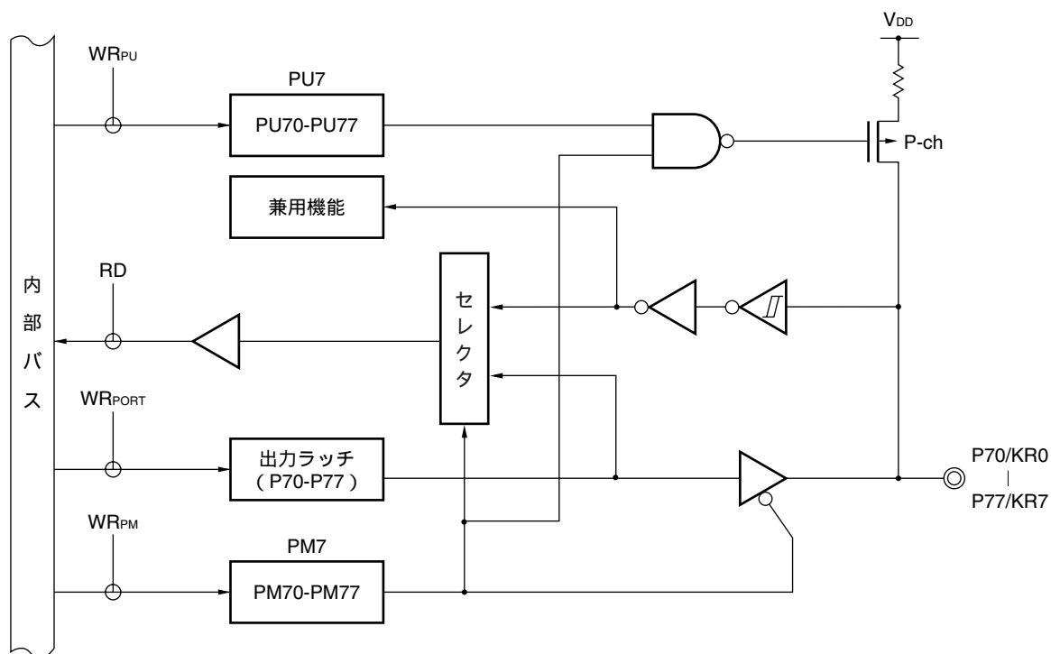
図5 - 17 P70-P77のブロック図
