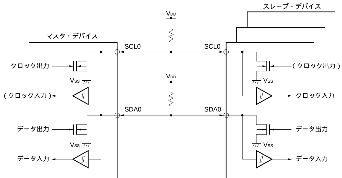
図17 - 12 端子構成図
