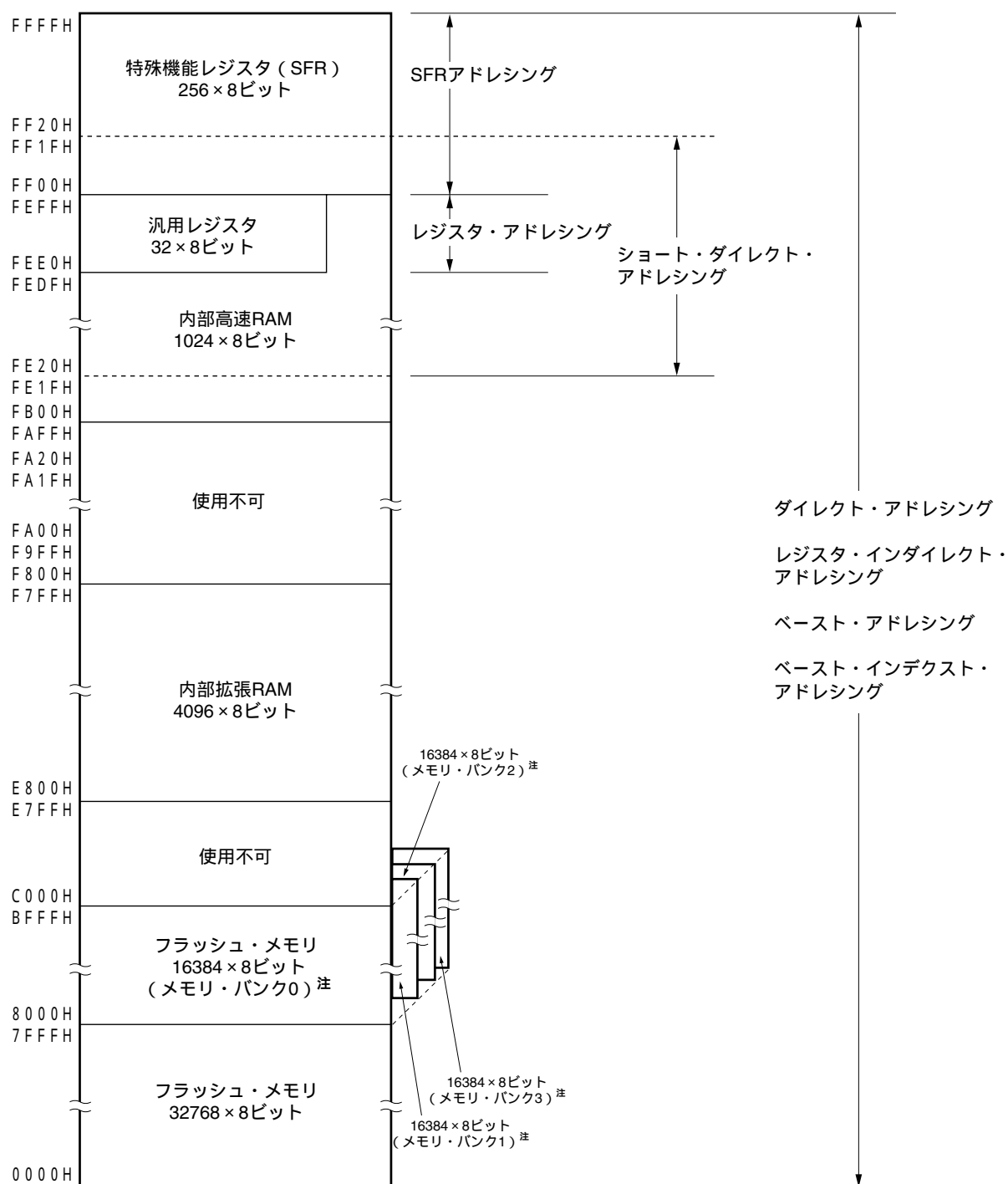
図3 - 10 データ・メモリとアドレッシングの対応 (μ PD78F0396)
