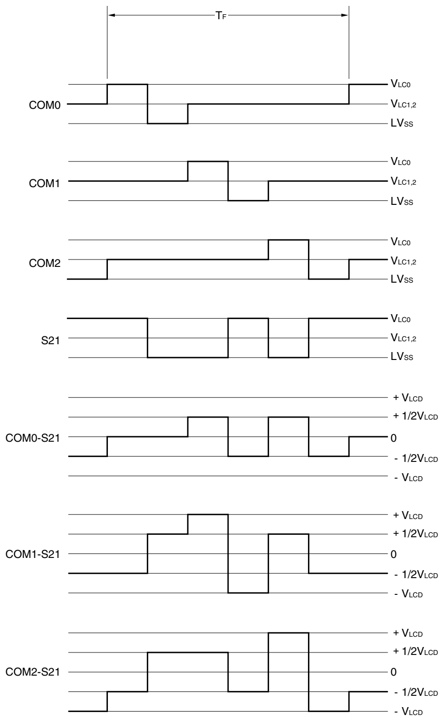
図18 - 22 3時分割LCD駆動波形例（1/2バイアス法）
