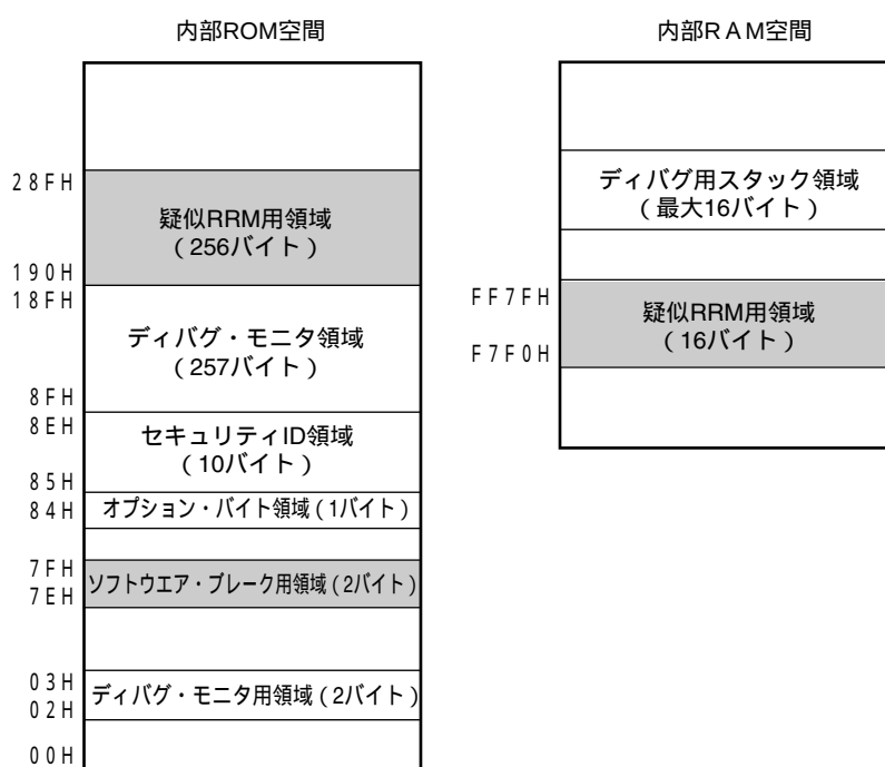
図28 - 4 QB-78K0MINI, QB-MINI2が使用する予約領域
