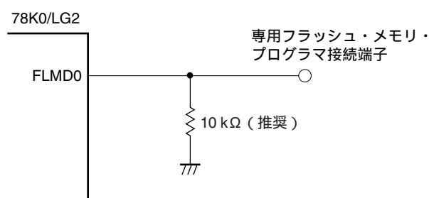
図27 - 8 FLMD0端子の接続例
