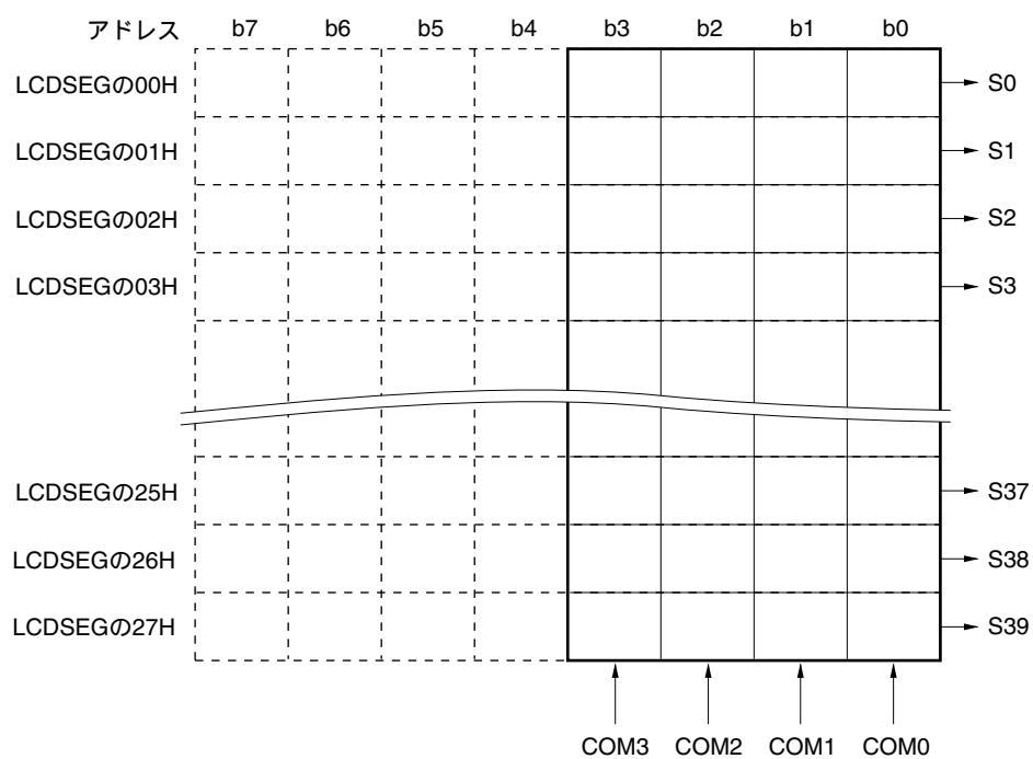
図18 - 11 LCD表示データ・メモリの内容とセグメント出力/コモン出力の関係
