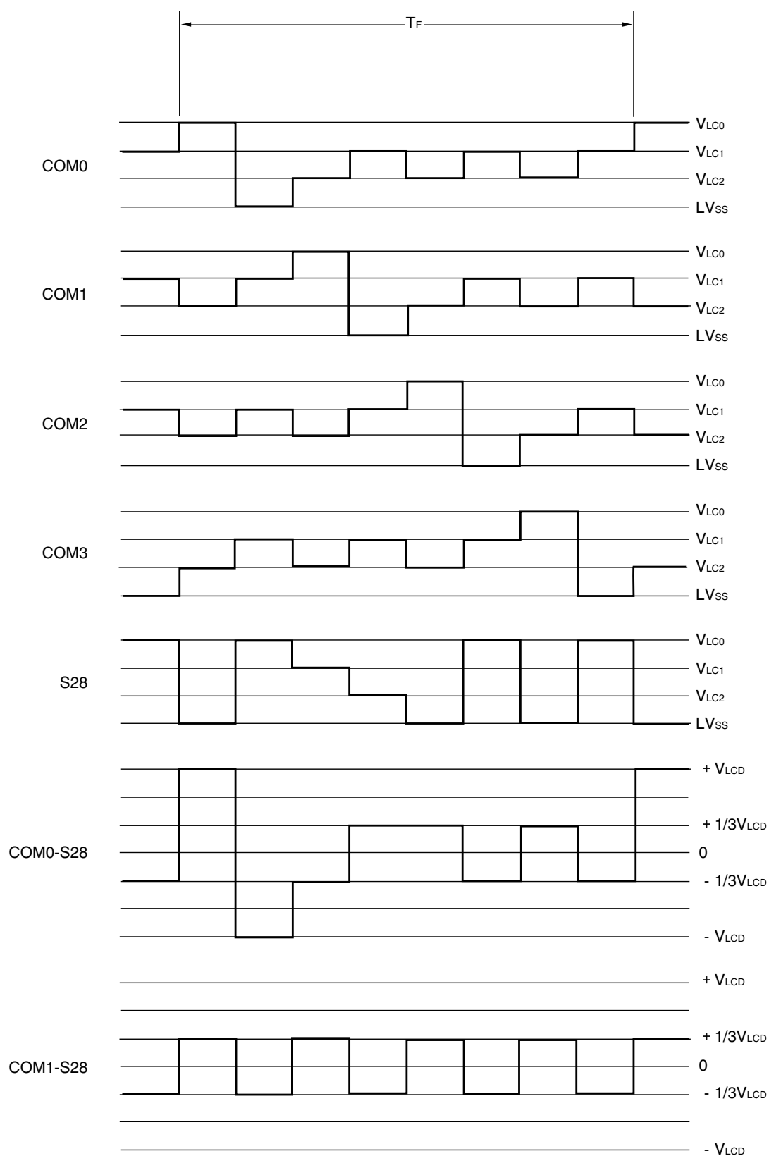
図18 - 26 4時分割LCD駆動波形例（1/3バイアス法）
