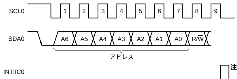
図17 - 15 アドレス
