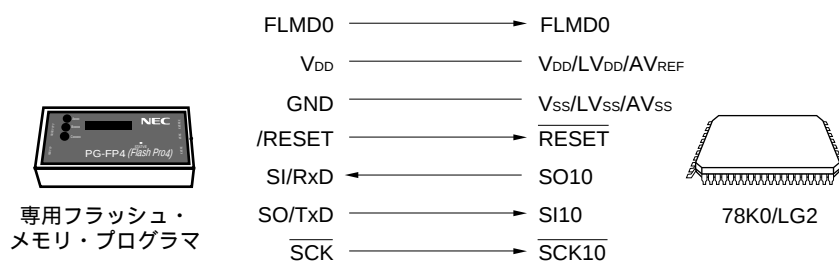
図27 - 6 専用フラッシュ・メモリ・プログラマとの通信（CSI10）
