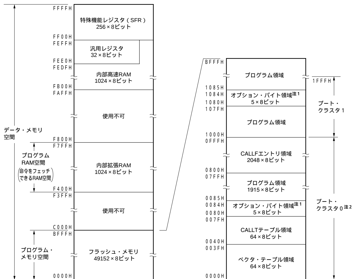
図3 - 2 メモリ・マップ (μ PD78F0394)
