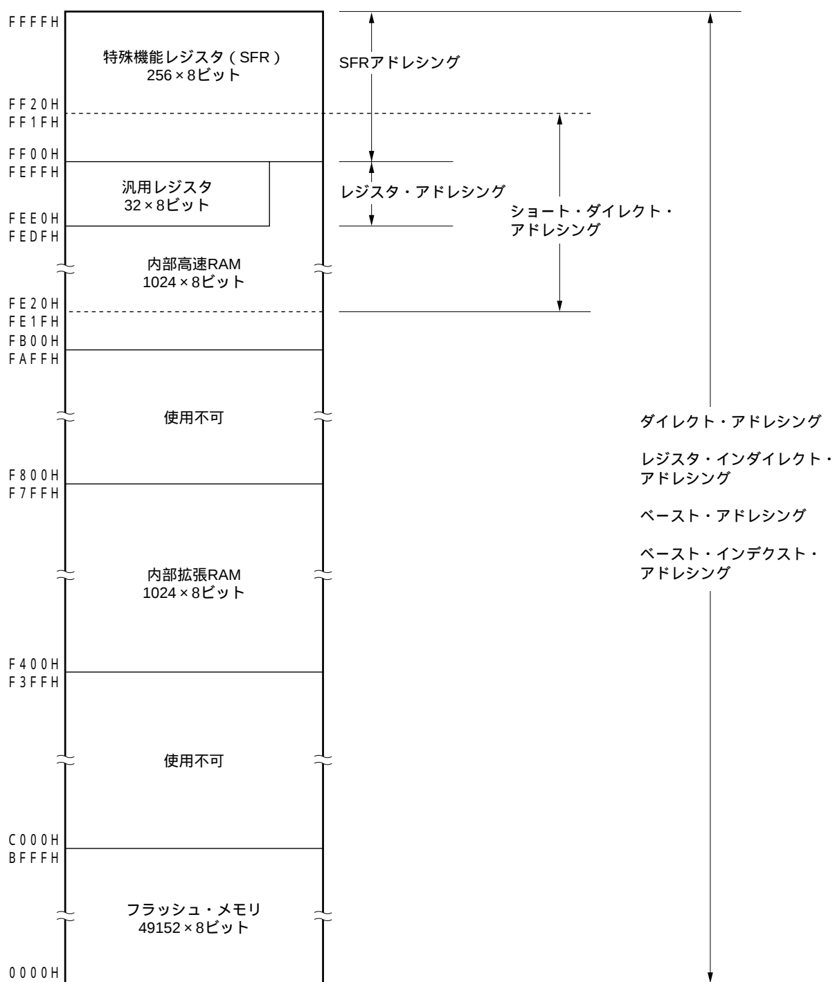
図3 - 8 データ・メモリとアドレッシングの対応 (μ PD78F0394)
