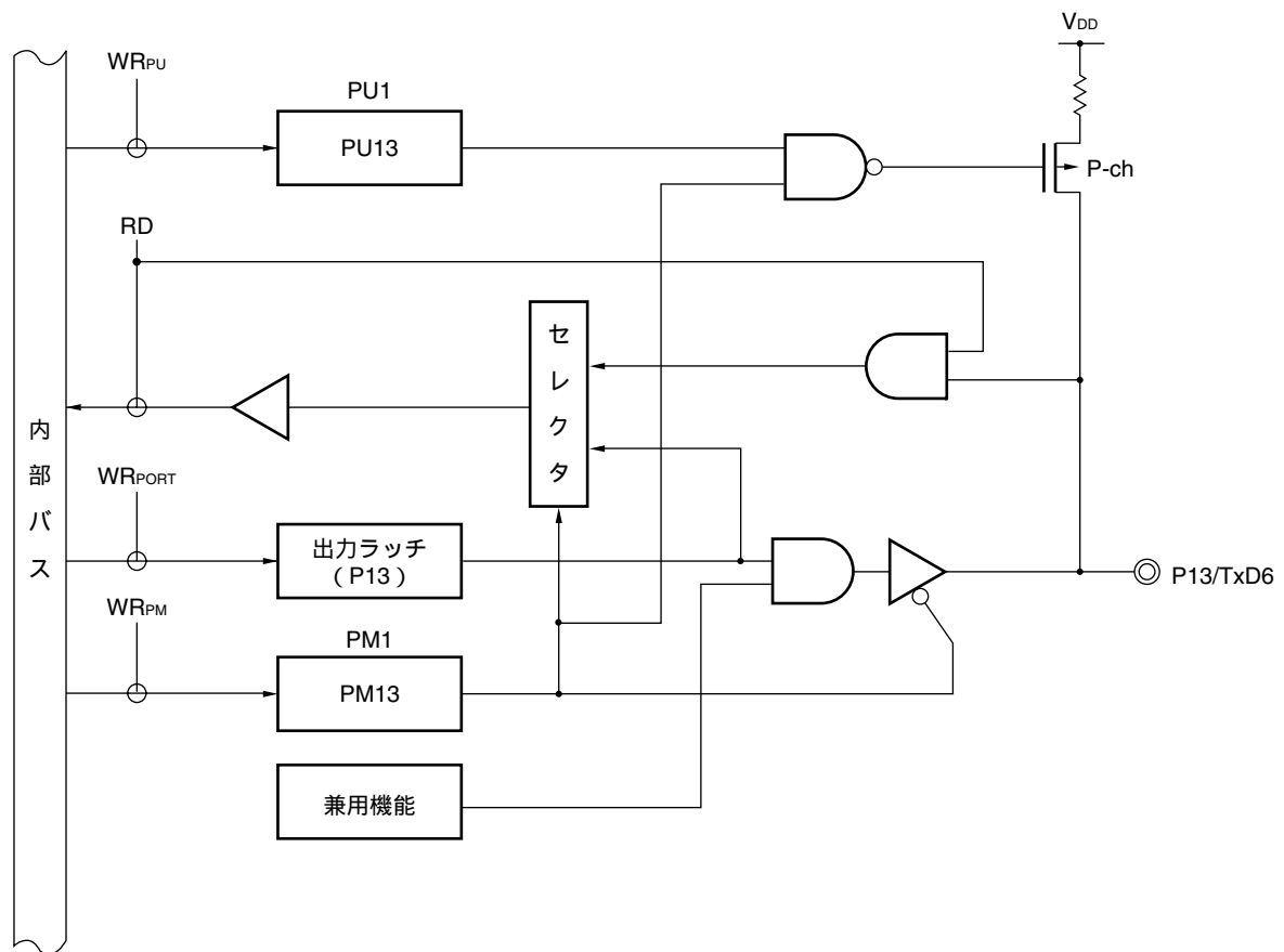
図5 - 11 P13のブロック図
