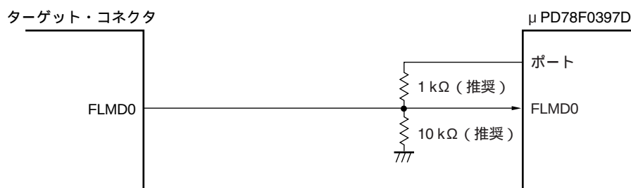
図28 - 3 オンチップ・ディバグでセルフ・プログラミングを行う場合のFLMD0端子の処理
