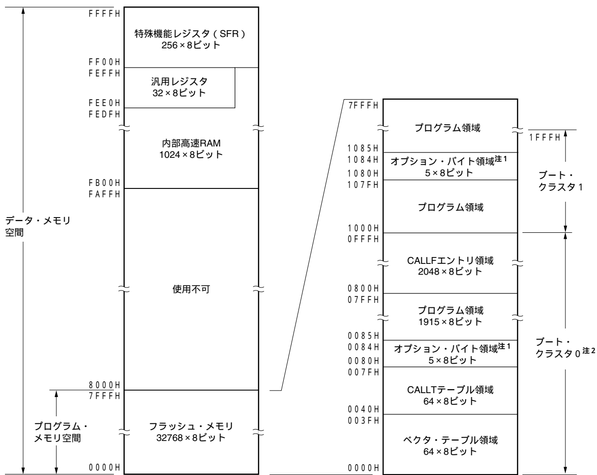
図3 - 1 メモリ・マップ (μ PD78F0393)
