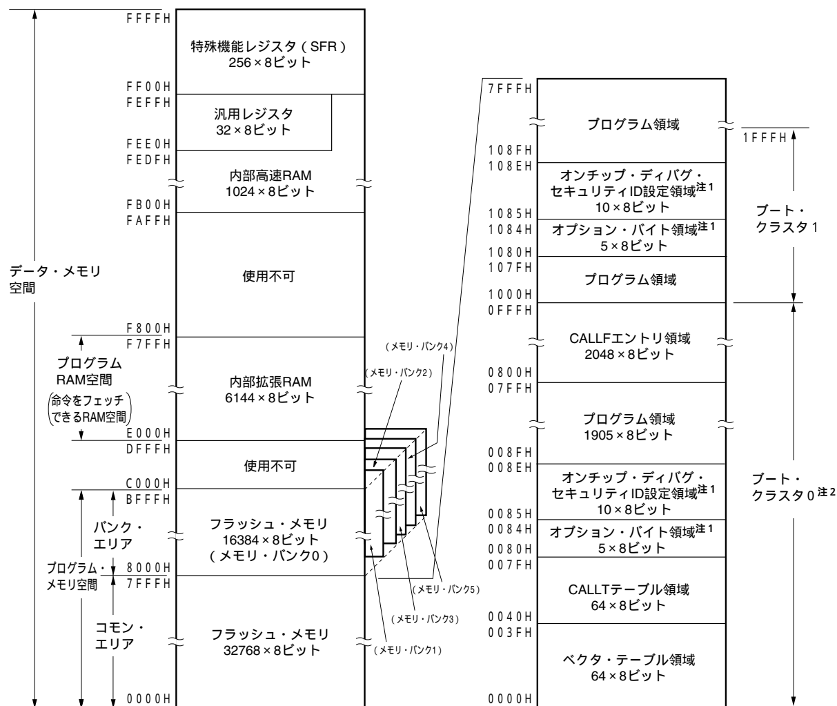
図3 - 6 メモリ・マップ (μPD78F0397D)
