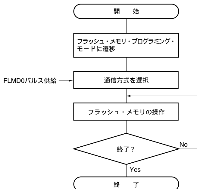
図27 - 12 フラッシュ・メモリの操作手順
