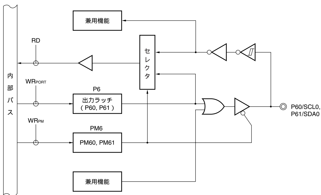
図5 - 16 P60, P61のブロック図
