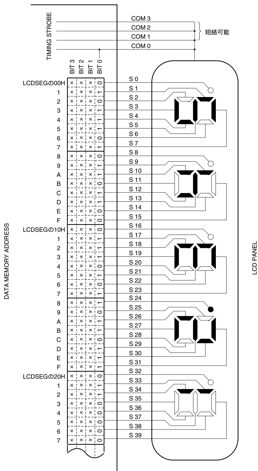
図18 - 15 スタティックLCDパネルの結線例
