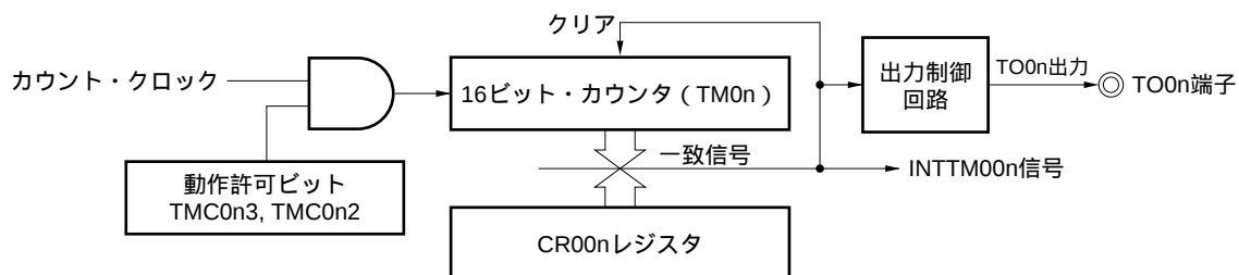
図7 - 20 方形波出力動作のブロック図
