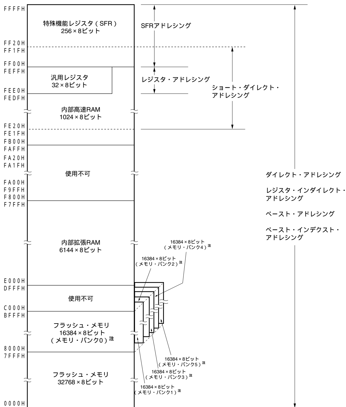
図3 - 11 データ・メモリとアドレッシングの対応 (μ PD78F0397, 78F0397D)
