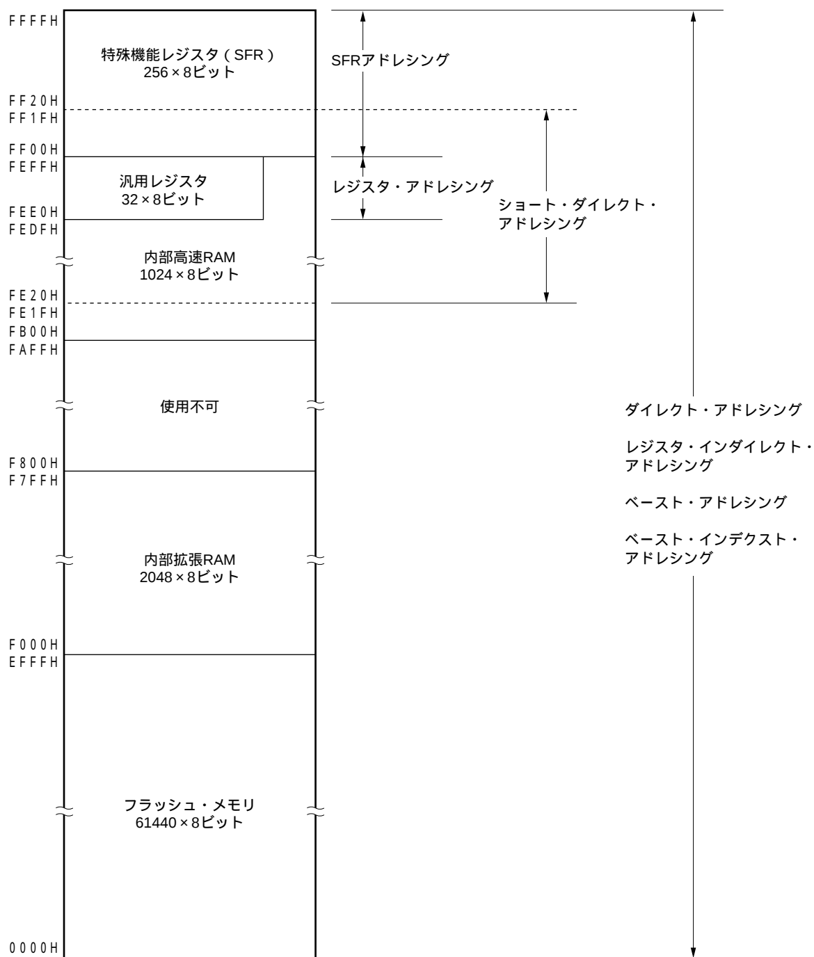
図3 - 9 データ・メモリとアドレッシングの対応 (μ PD78F0395)
