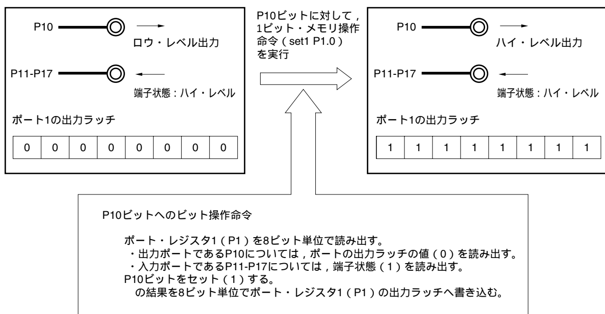
図5-24 1ビット・メモリ操作命令（P10の場合）
