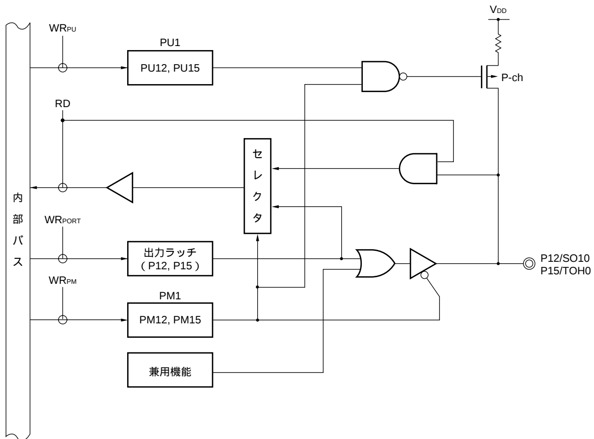
図5 - 10 P12, P15のブロック図
