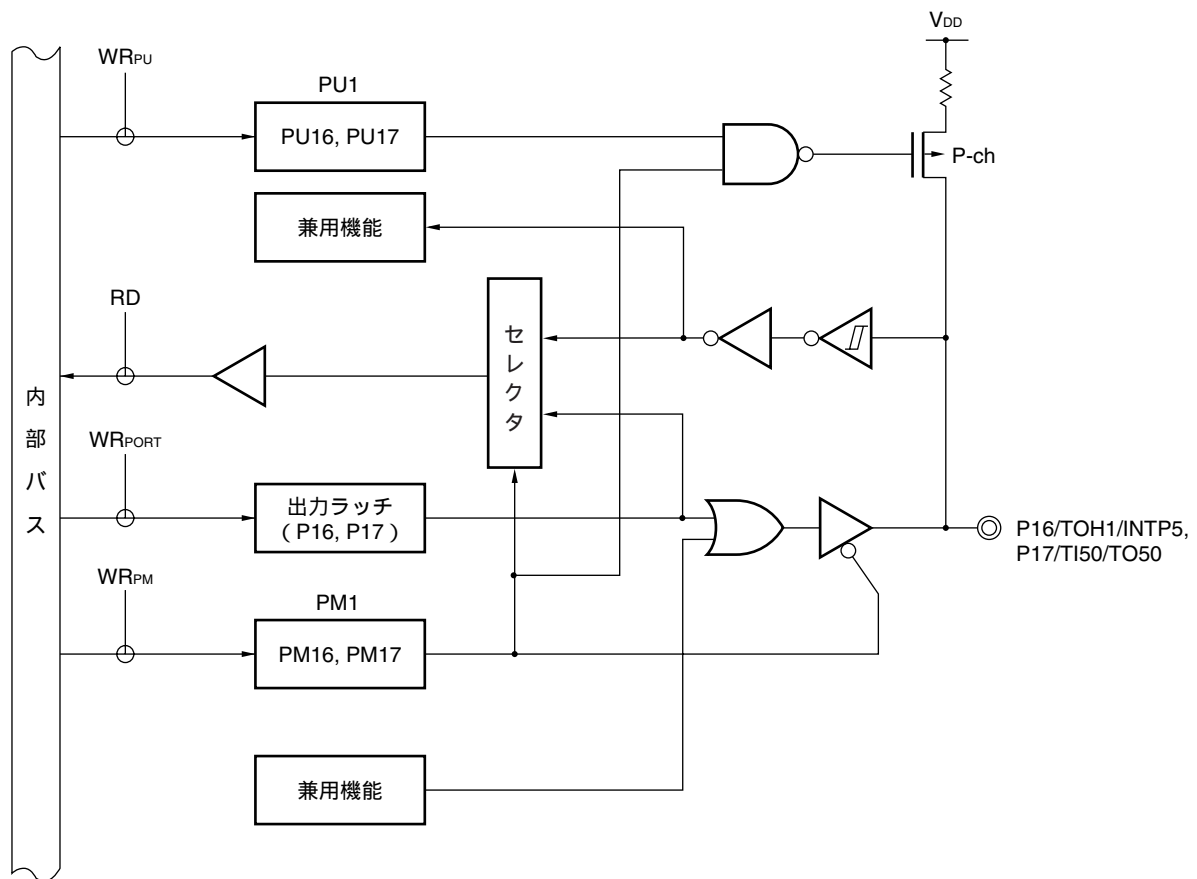
図5 - 12 P16, P17のブロック図
