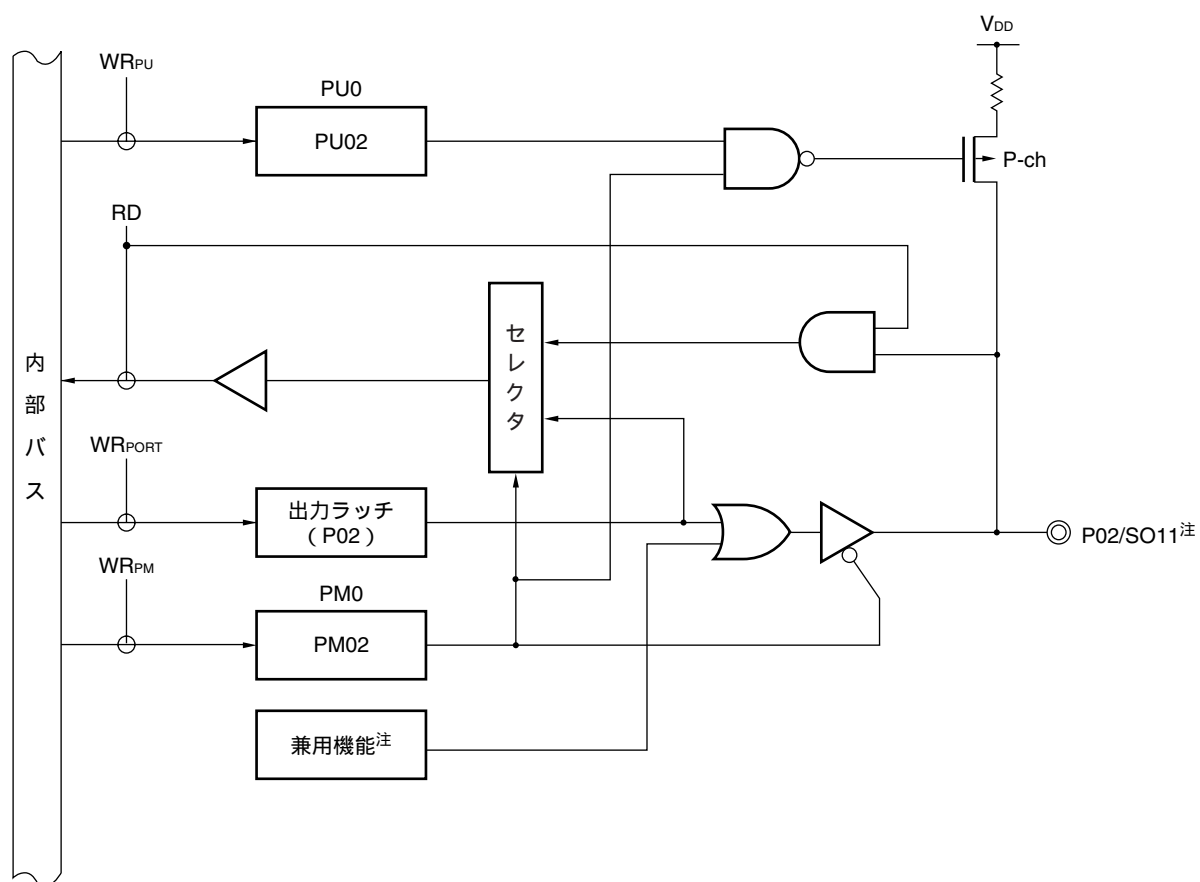
図5 - 4 P02のブロック図
