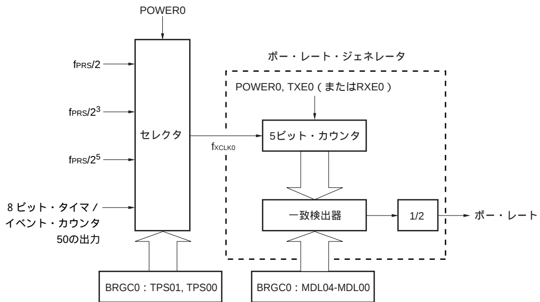
図14 - 11 ボー・レート・ジェネレータの構成
