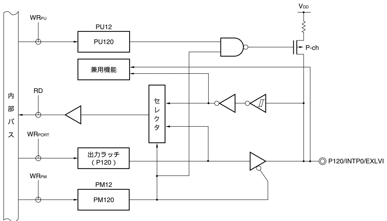
図5 - 18 P120のブロック図
