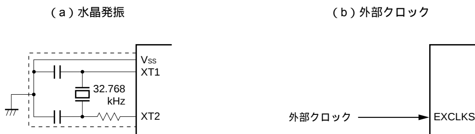
図6 - 10 XT1発振回路の外付け回路例
