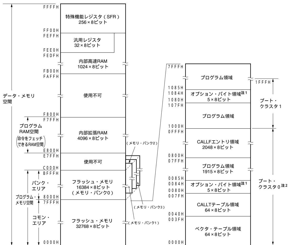
図3-4 メモリ・マップ(μ PD78F0396)
