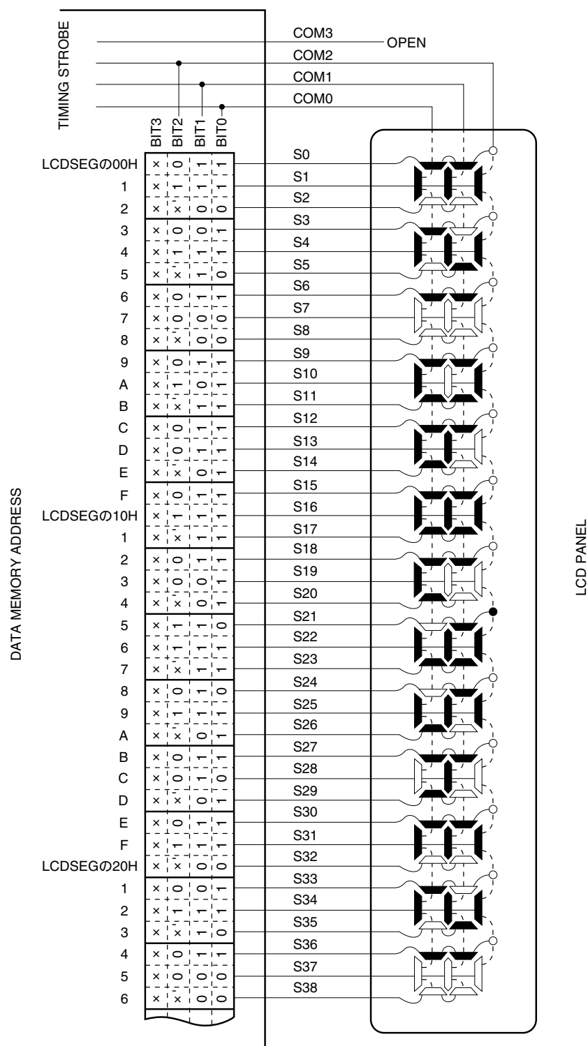
図18 - 21 3時分割LCDパネルの結線例
