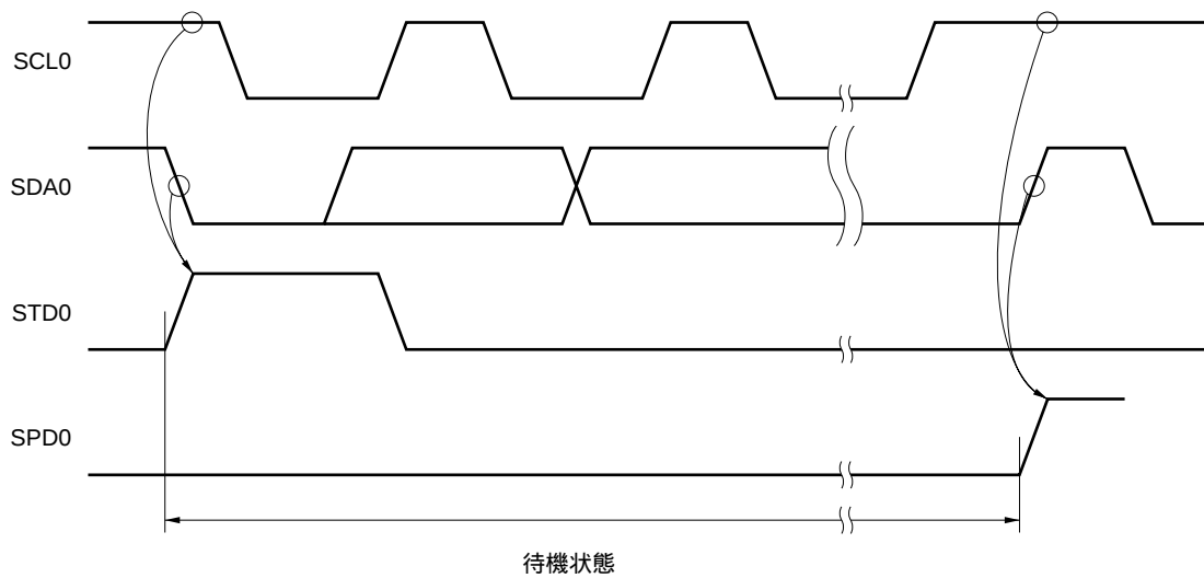
図17 - 22 通信予約受け付けタイミング
