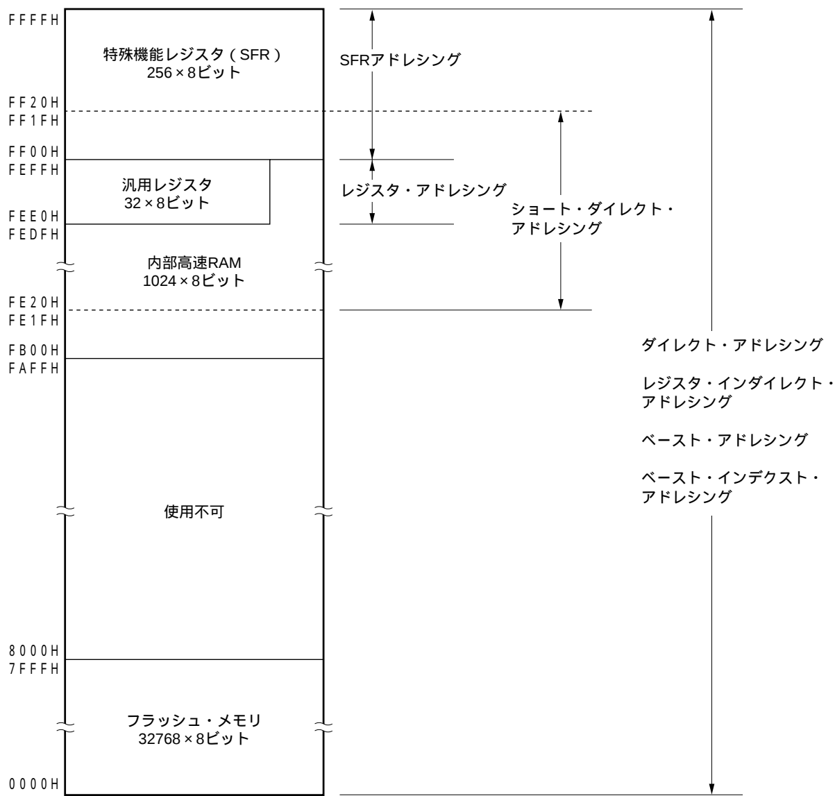
図3 - 7 データ・メモリとアドレッシングの対応 (μ PD78F0393)
