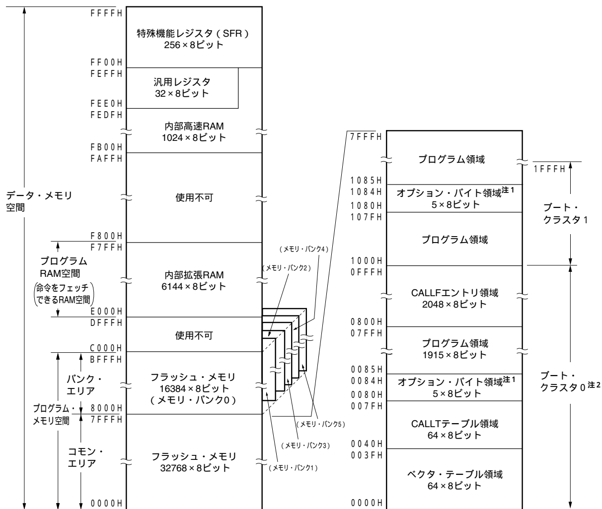
図3 - 5 メモリ・マップ (μ PD78F0397)
