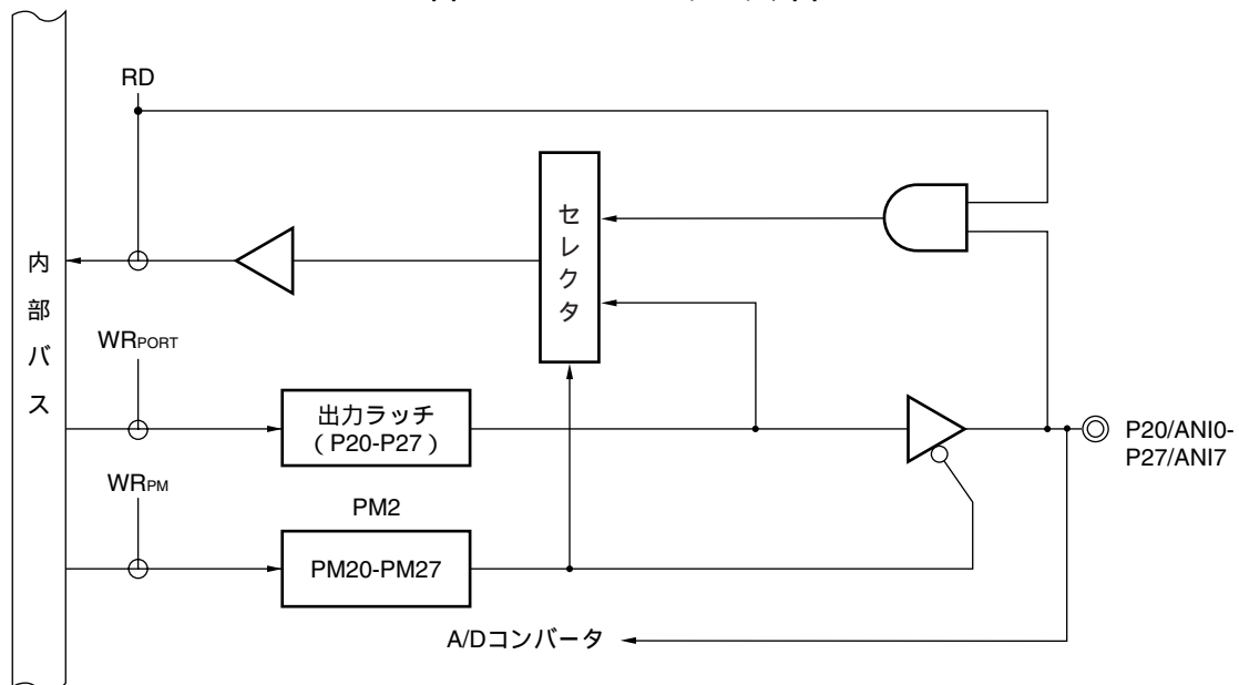
図5 - 13 P20-P27のブロック図
