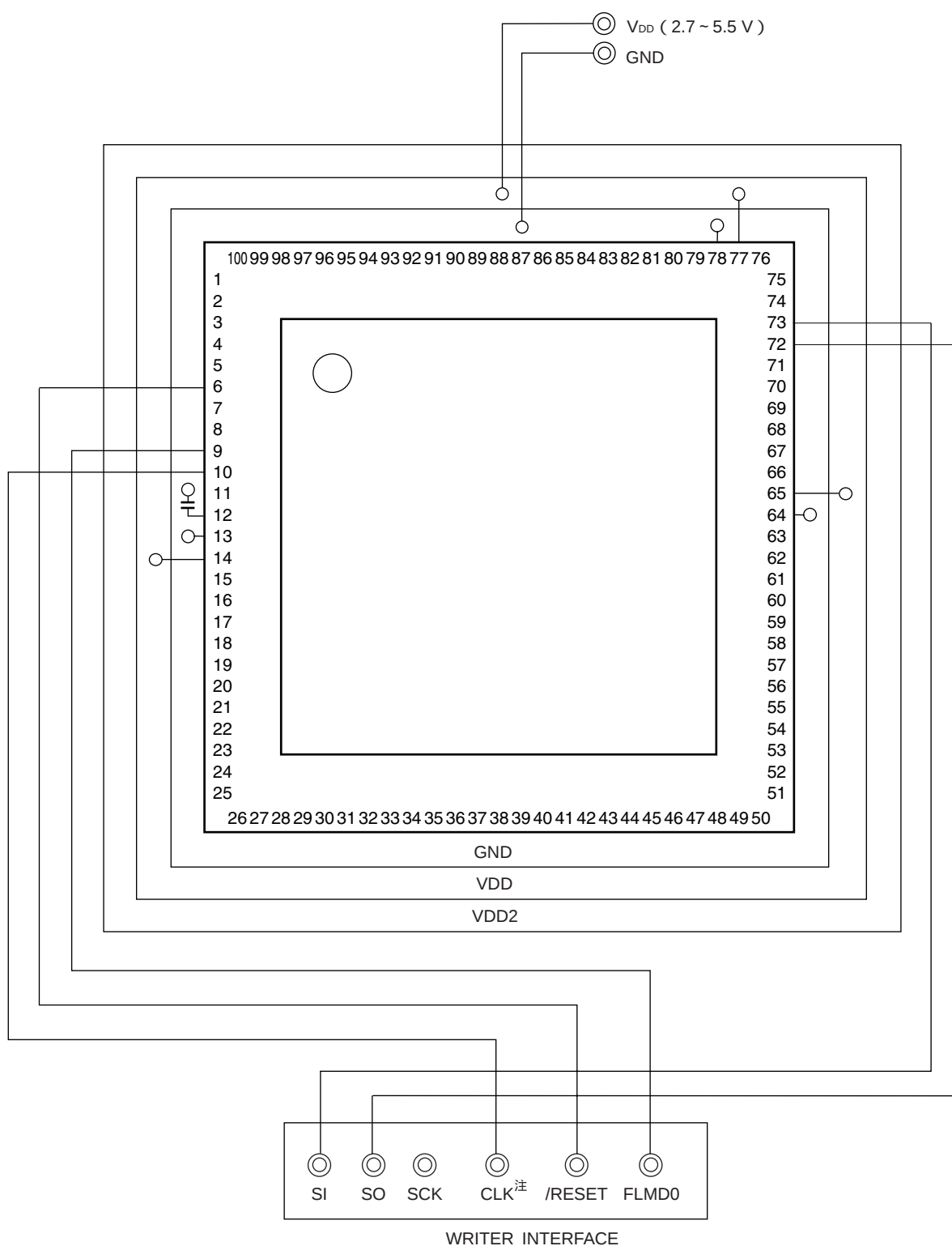
図27 - 4 UART (UART6) 方式でのフラッシュ書き込み用アダプタ配線例
