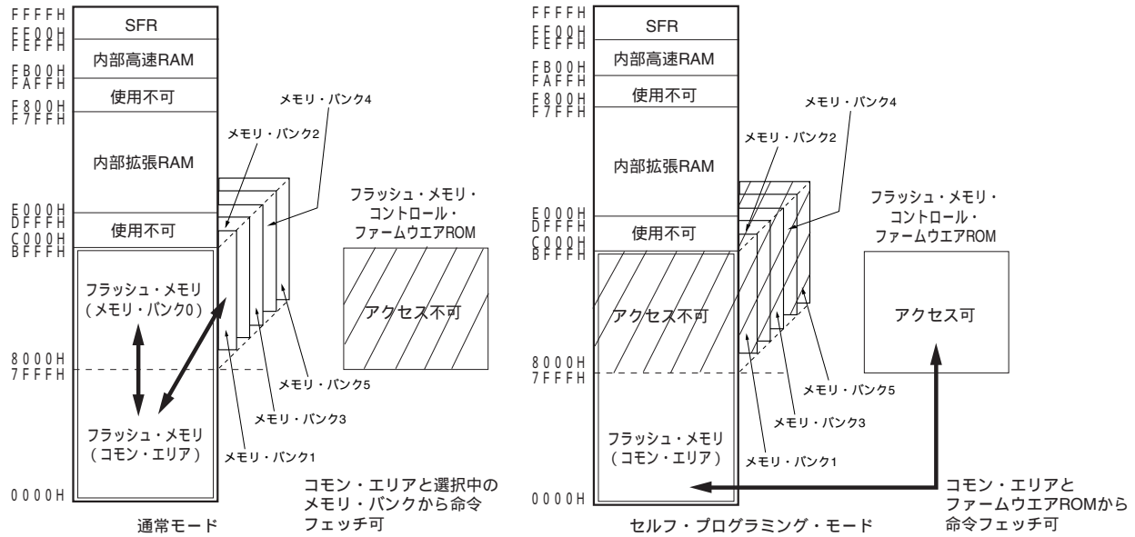
図27 - 15 セルフ・プログラミングの動作モードとメモリ・マップ (μ PD78F0397の場合)
