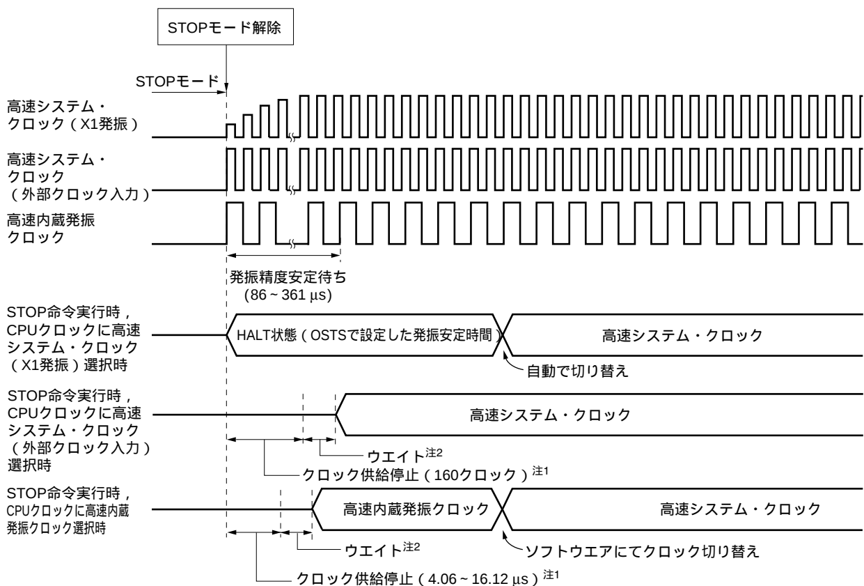
図22 - 5 STOPモード解除時の動作タイミング
