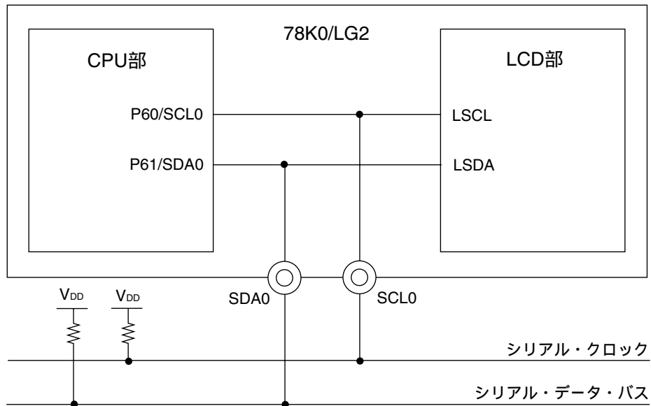
図17 - 30 システム構成
