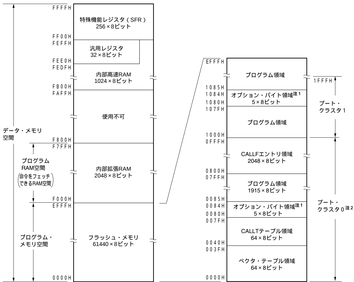
図3 - 3 メモリ・マップ (μ PD78F0395)
