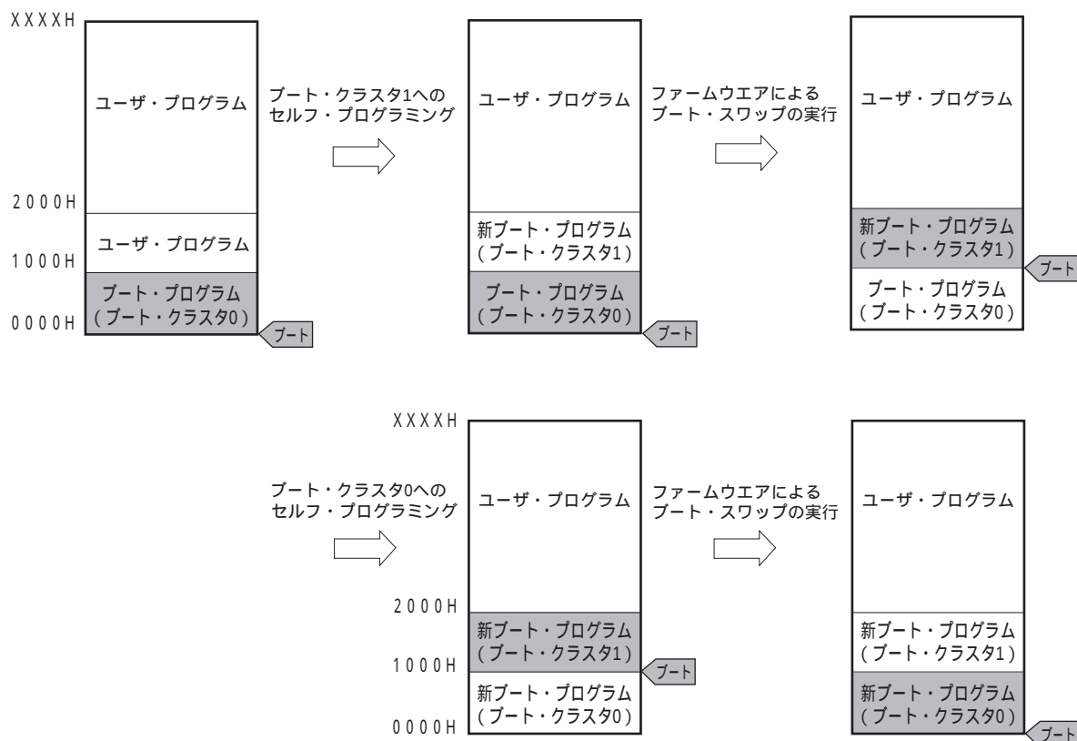
図27 - 17 ブート・スワップ機能
