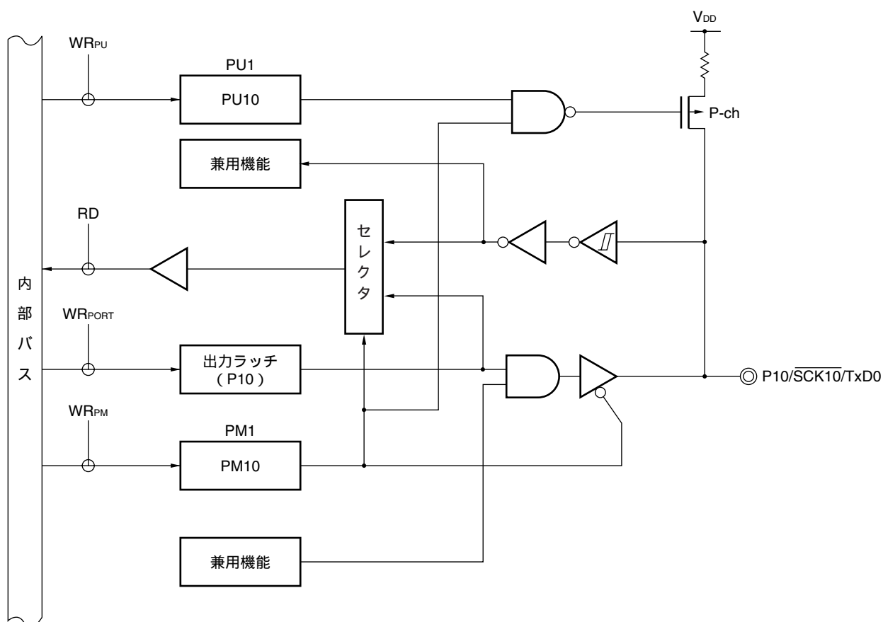
図5 - 8 P10のブロック図
