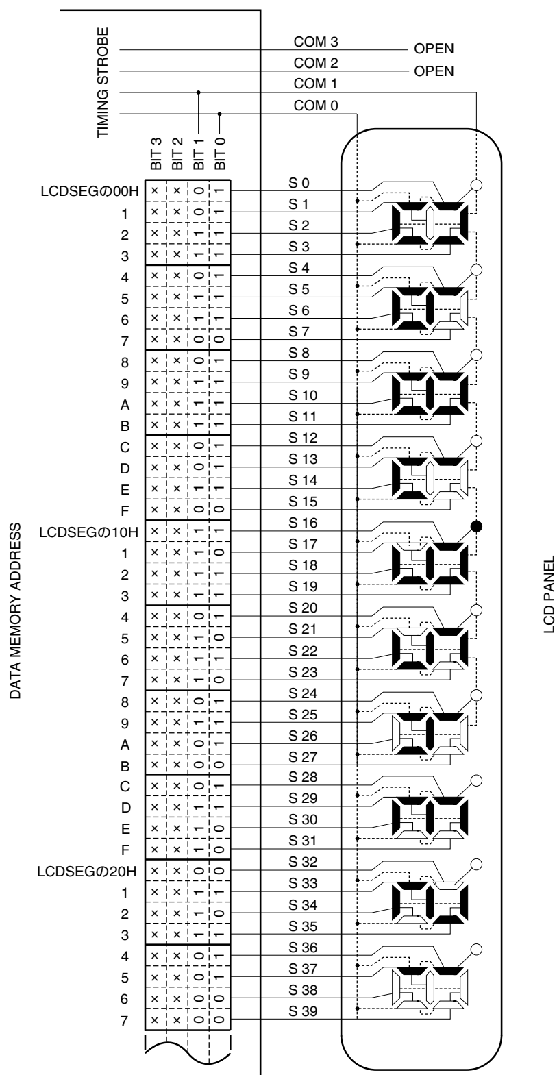
図18 - 18 2時分割LCDパネルの結線例
