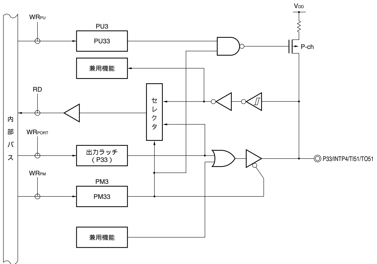
図5 - 15 P33のブロック図
