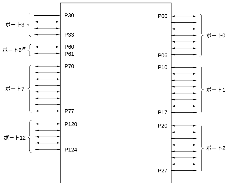
図5 - 1 ポートの種類
