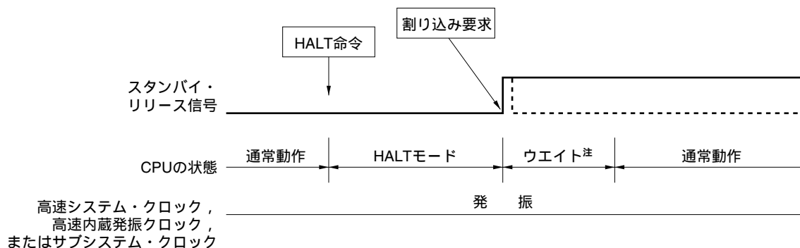
図22 - 3 HALTモードの割り込み要求発生による解除
