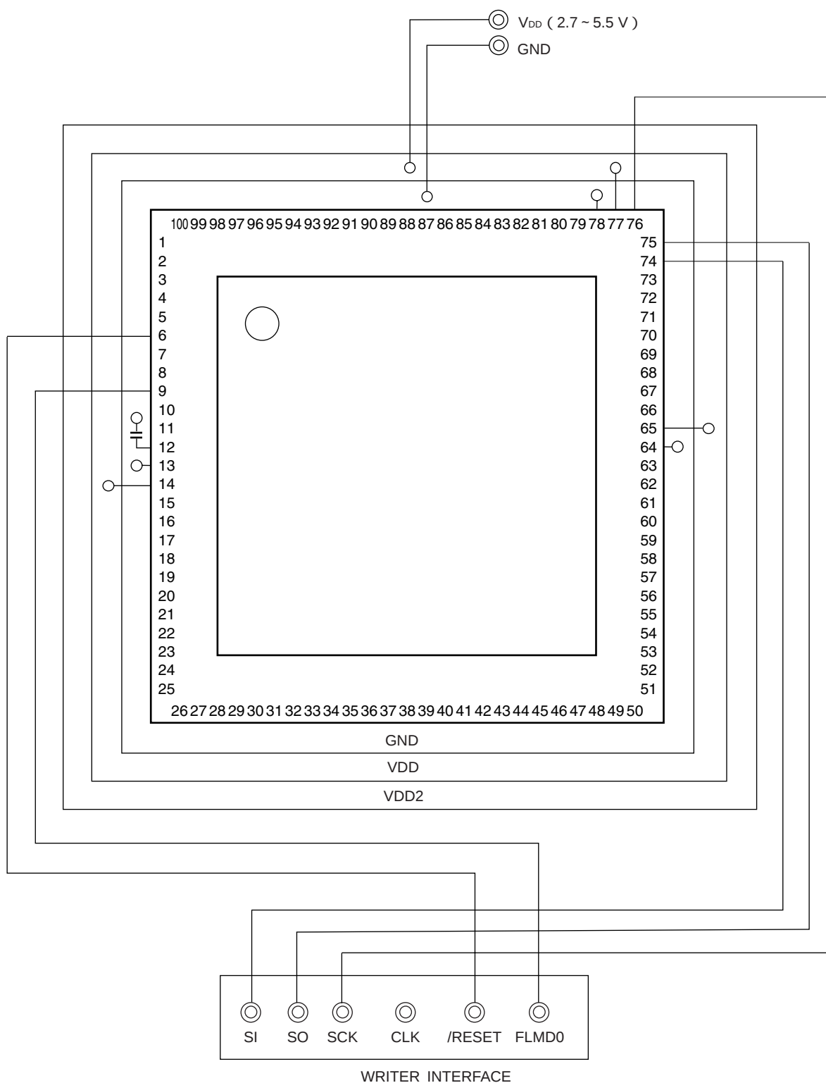
図27 - 3 3線式シリアルI/O (CSI10) 方式でのフラッシュ書き込み用アダプタ配線例
