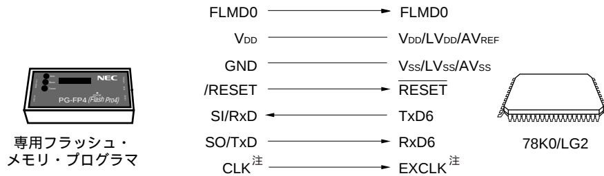
図27 - 7 専用フラッシュ・メモリ・プログラマとの通信 (UART6)
