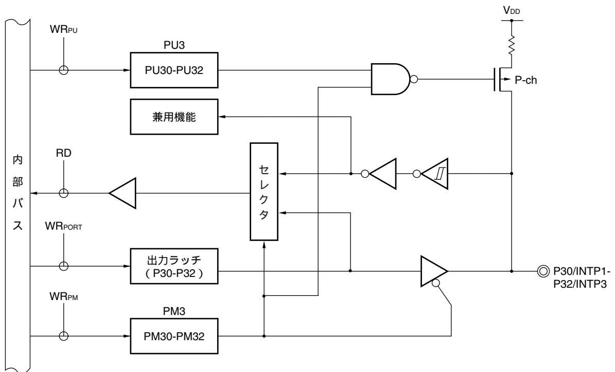
図5 - 14 P30-P32のブロック図
