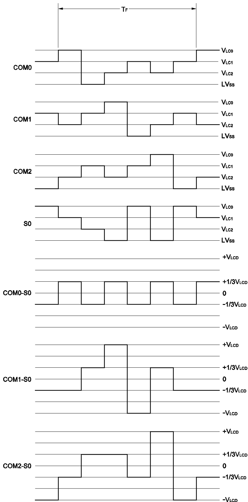
图 17-24. 3 分时 LCD 驱动波形举例 (1/3 偏压模式)
