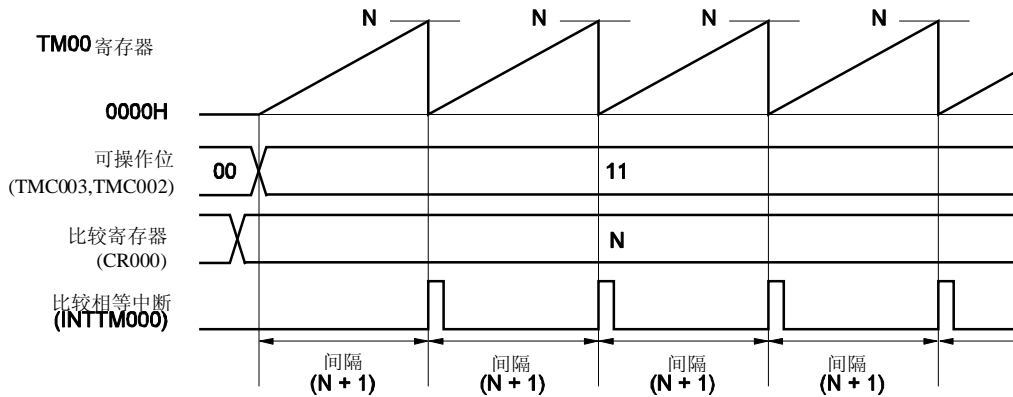
图 6-12. 间隔定时器操作的基本时序示例
