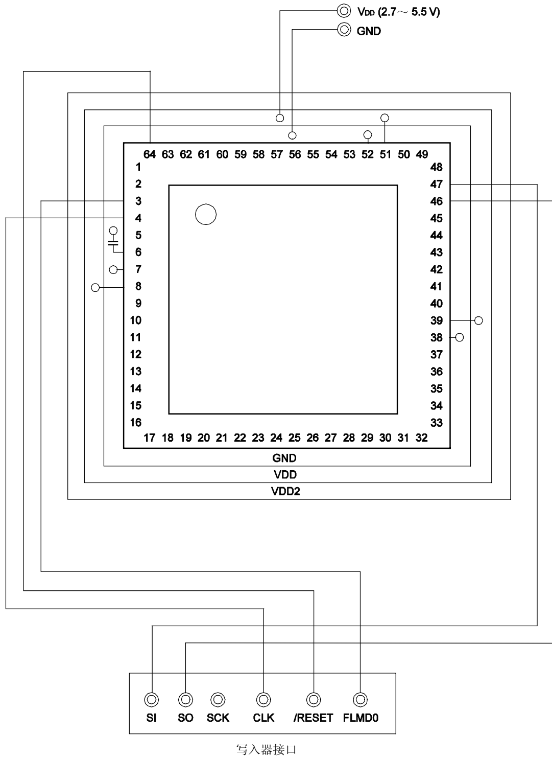
图 24-3. UART (UART6) 模式下使用适配器对 Flash 存储器进行写操作示例
