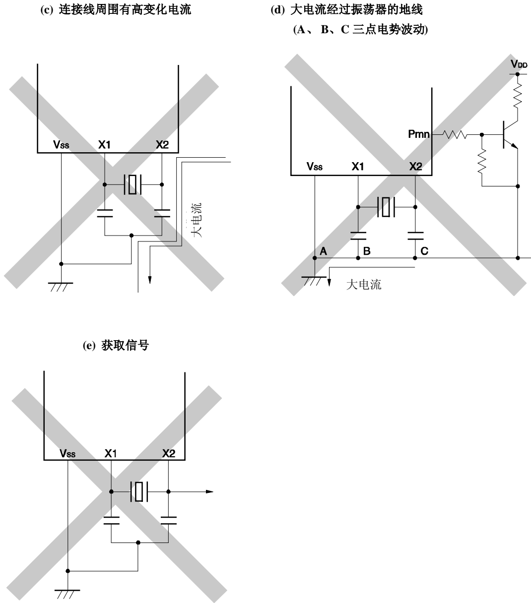
图 5-11. 不正确的振荡器连接示例 (2/2)
