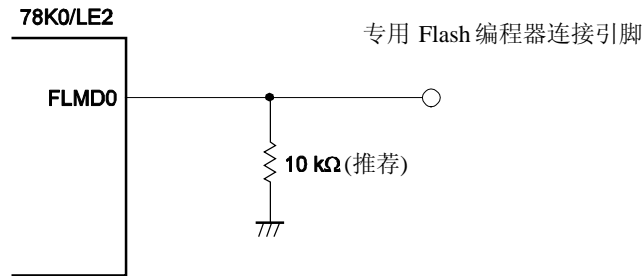
图 24-7. FLMD0 引脚连接示例
