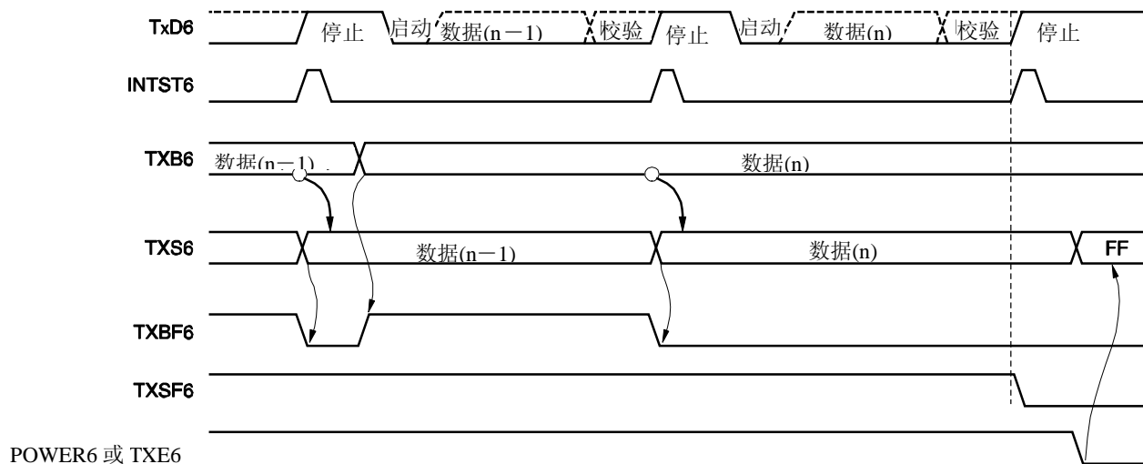
图 14-18. 结束连续发送操作的时序
