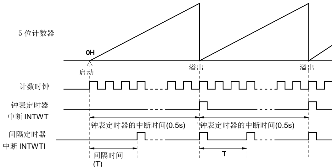
图 9-3. 钟表定时器/间隔定时器的操作时序
