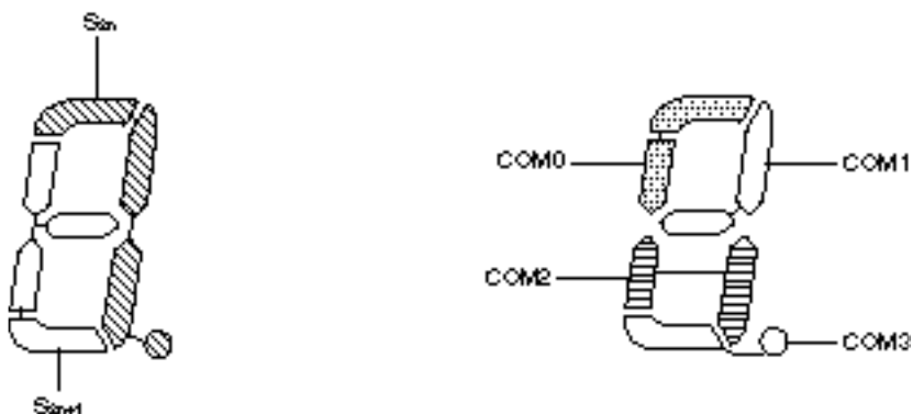
图 17-25. 4 分时 LCD 显示模式和电极连接
