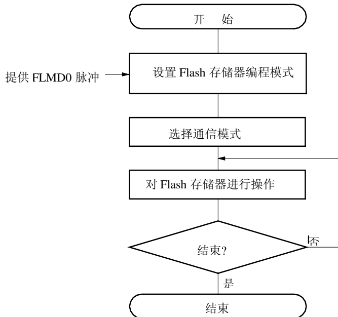
图 24-11. Flash 存储器操作过程
