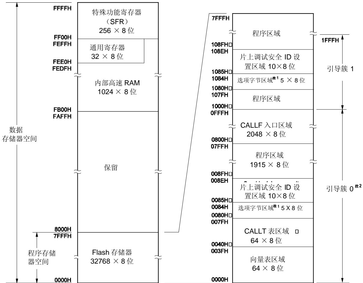
图 3-4. 存储空间映射图 (μPD78F0363D)
