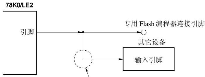
图 24-9. 其它设备的故障
