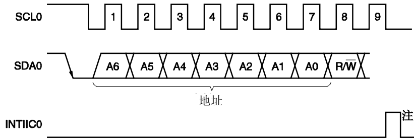
图 16-14. 地址
