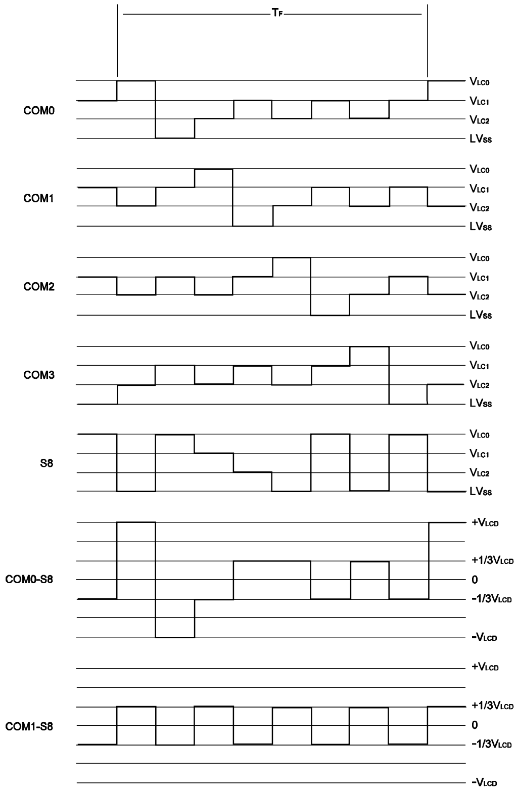
图 17-27. 4 分时 LCD 驱动波形举例 (1/3 偏压模式)
