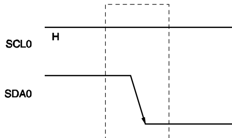
图 16-13. 起始条件
