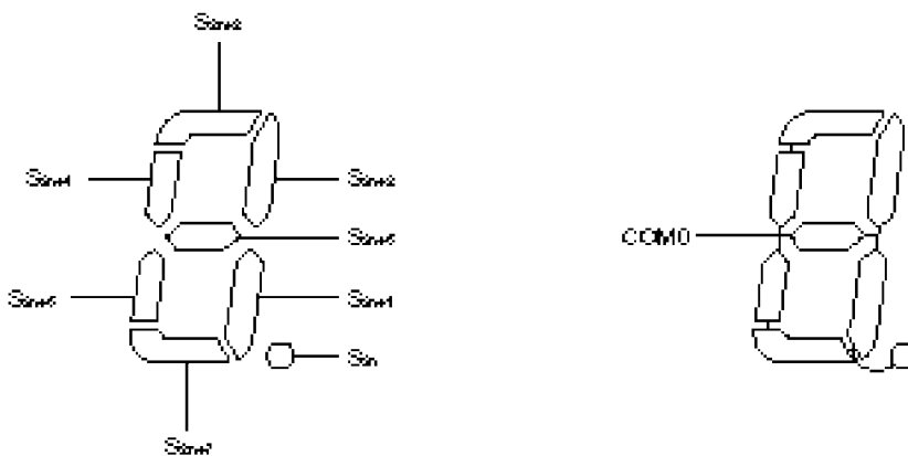
图 17-15. 静态 LCD 显示模式和电极连接
