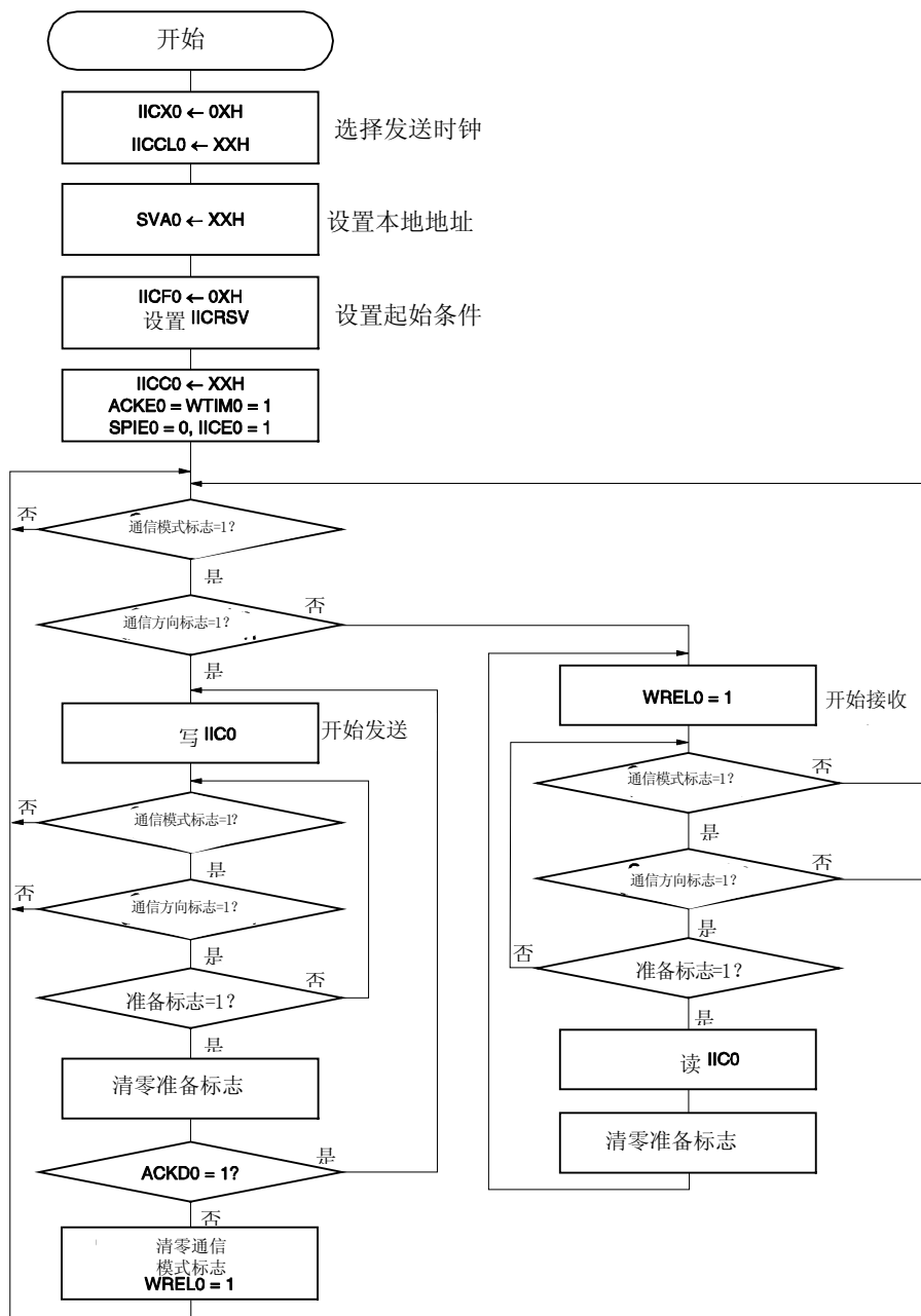
图 16-25. 从设备操作流程图中 (1)
