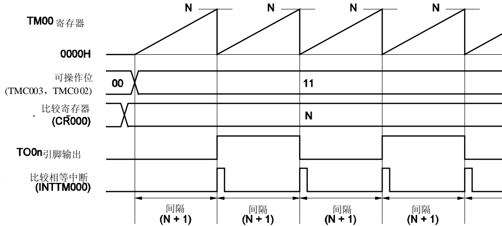
图 6-16. 方波输出操作的基本时序示例
