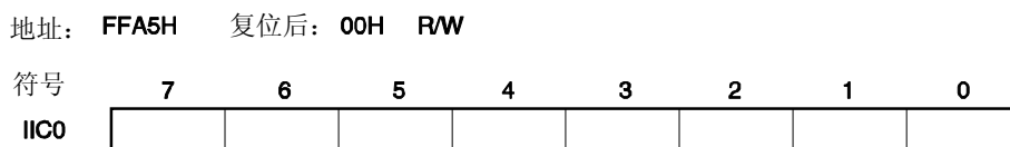
图 16-3. IIC 移位寄存器 0 的格式 (IIC0)
