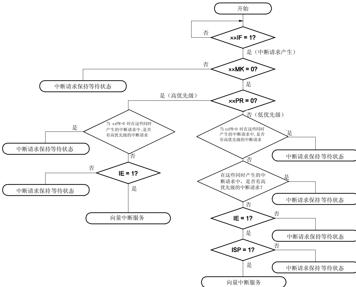
图 18-7. 中断请求响应处理
