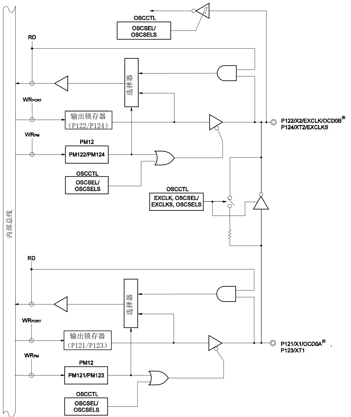
图 4-14. P121 ~ P124 的框图
