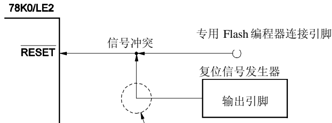
图 24-10. 信号冲突（RESET 引脚）
