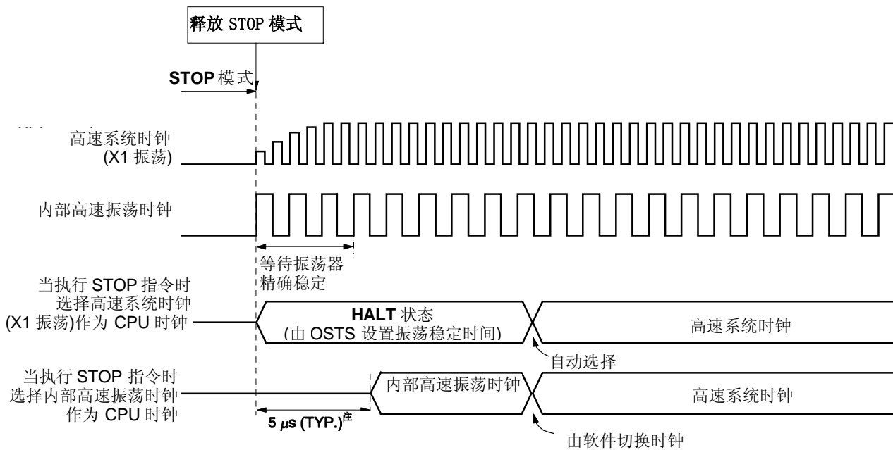
图 19-5. 释放 STOP 模式时的操作时序
