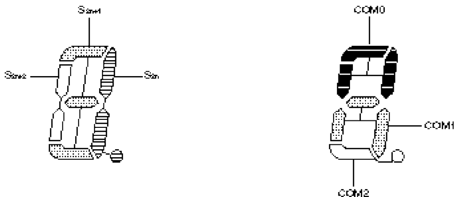
图 17-21. 3 分时 LCD 显示模式和电极连接
