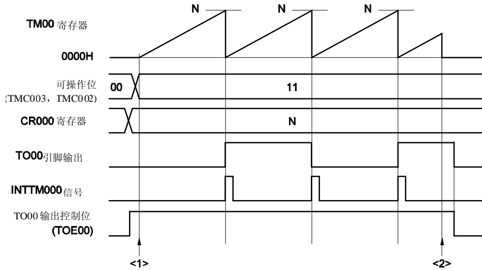
图 6-18. 方波输出功能软件处理示例
