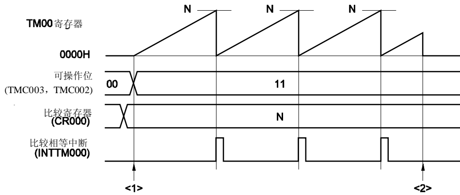
图 6-21. 外部事件计数器模式下的软件处理示例
