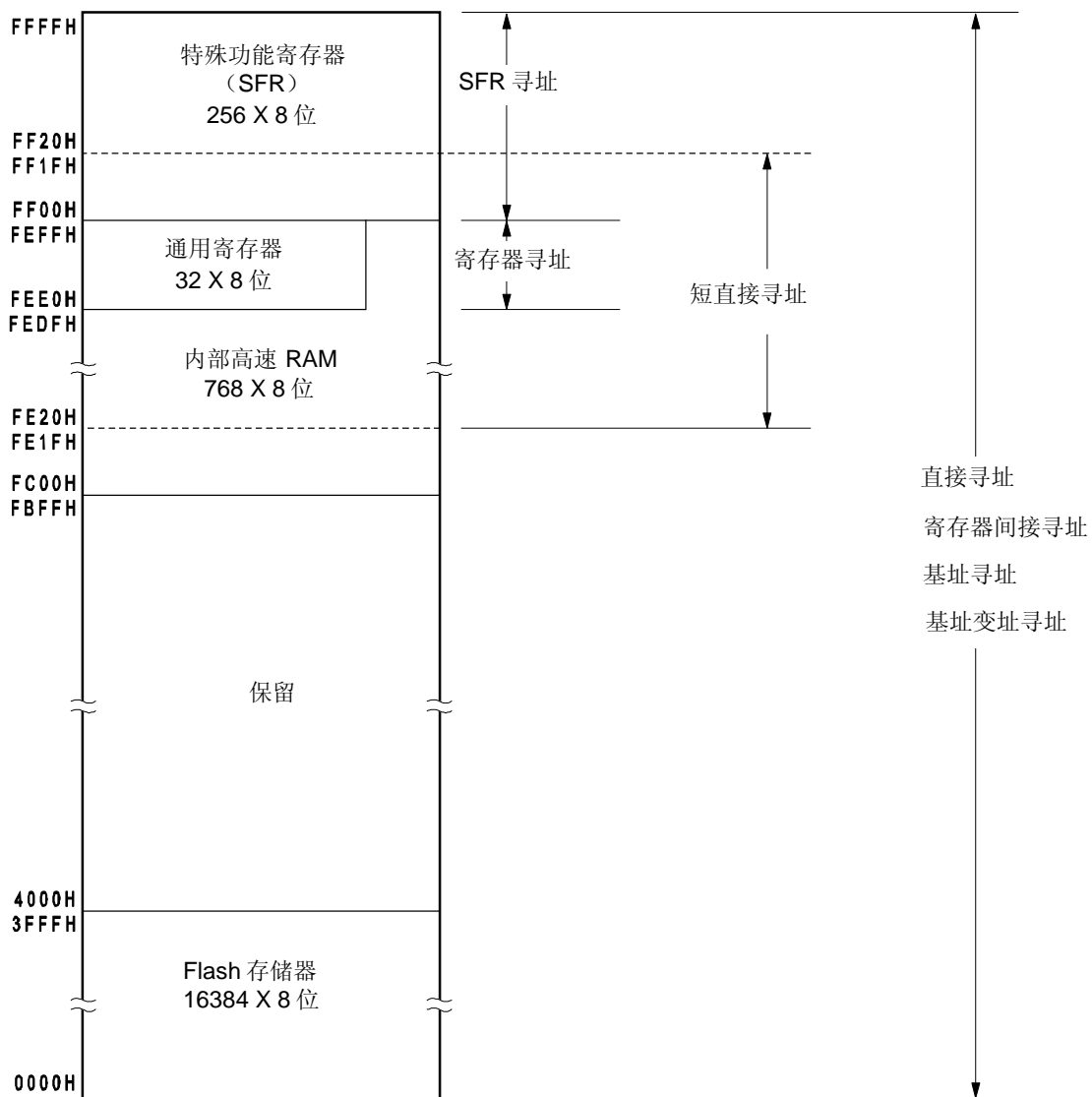
图 3-5. 数据存储寻址与寻址方式的对应关系 (μPD78F0361)
