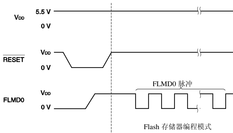
图 24-12. Flash 存储器编程模式
