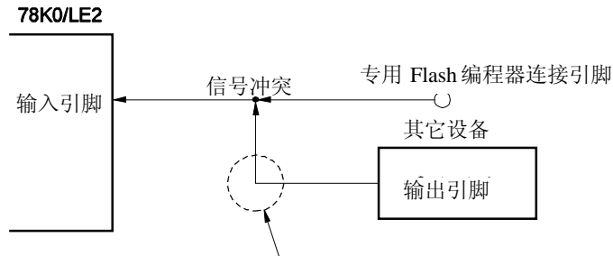
图 24-8. 信号冲突（串行接口的输入引脚）
