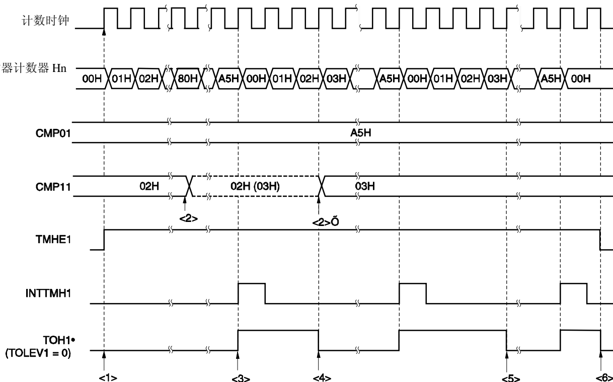
(e) 修改 CMP1n 的时序操作 (CMP1n = 02H → 03H, CMP0n = A5H)
