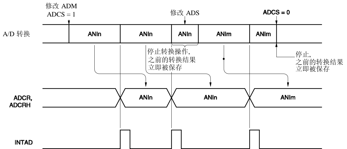
图 12-13. A/D 转换操作
