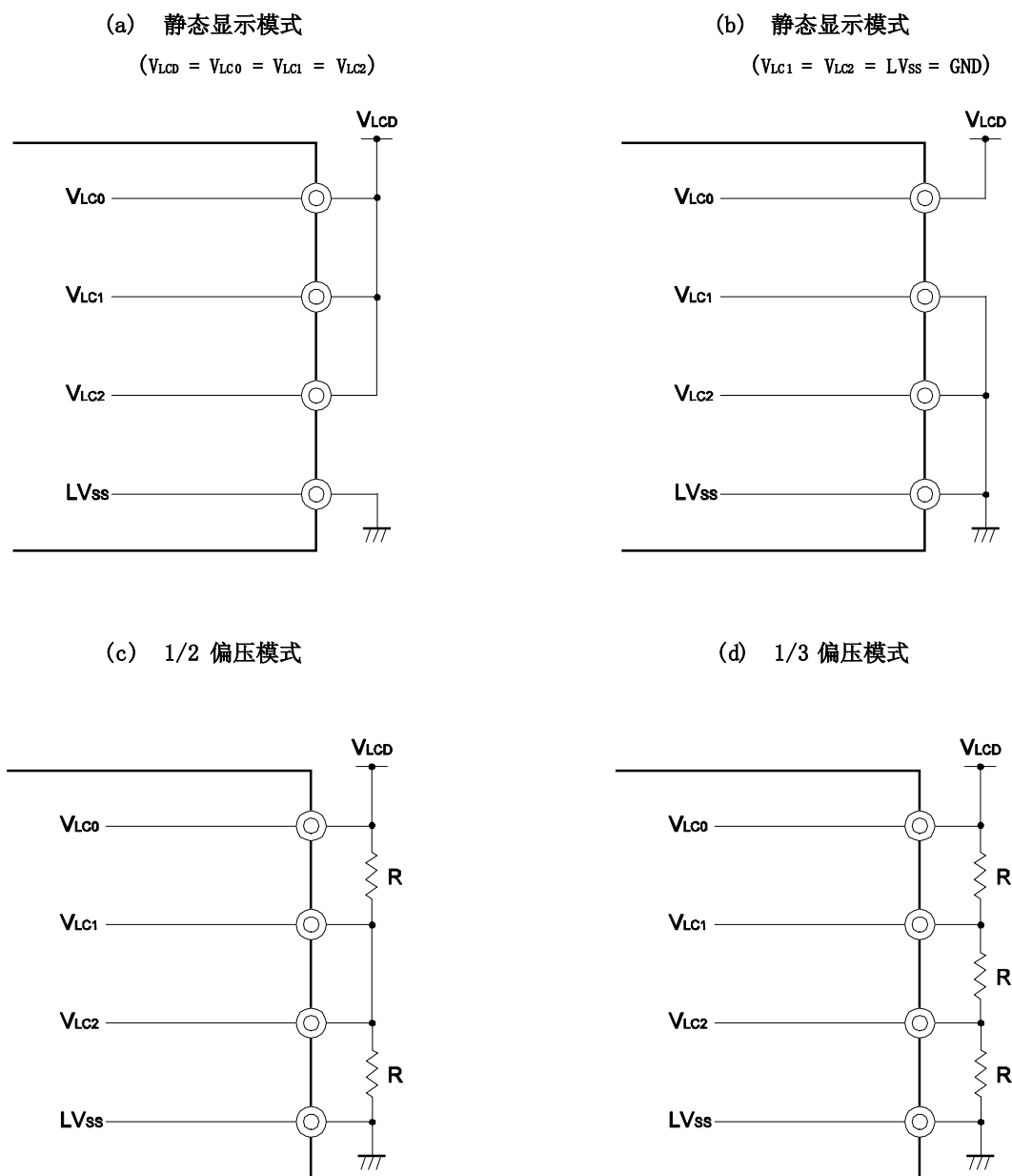
图 17-29. LCD 驱动电压连接举例 (外部电阻分压模式)
