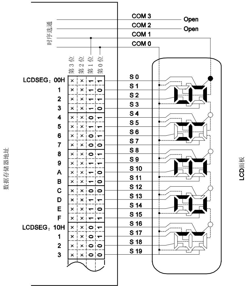
图 17-19. 2 分时 LCD 面板连接举例
