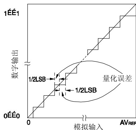
图 12-15. 量化误差
