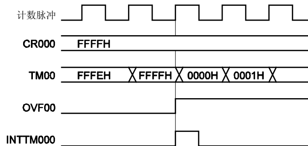
图 6-57. OVF00 标志操作时序
