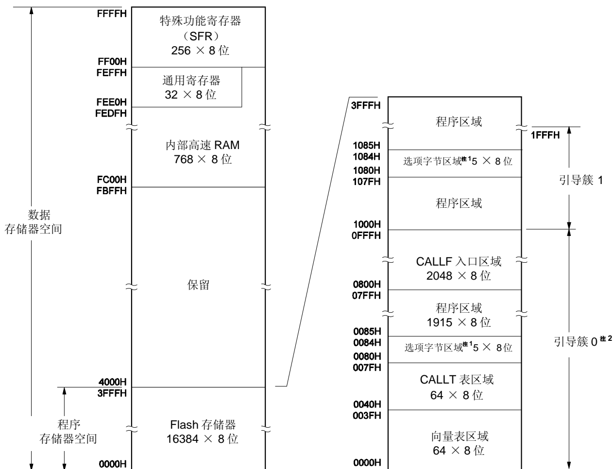
图 3-1. 存储空间映射图 (μPD78F0361)
