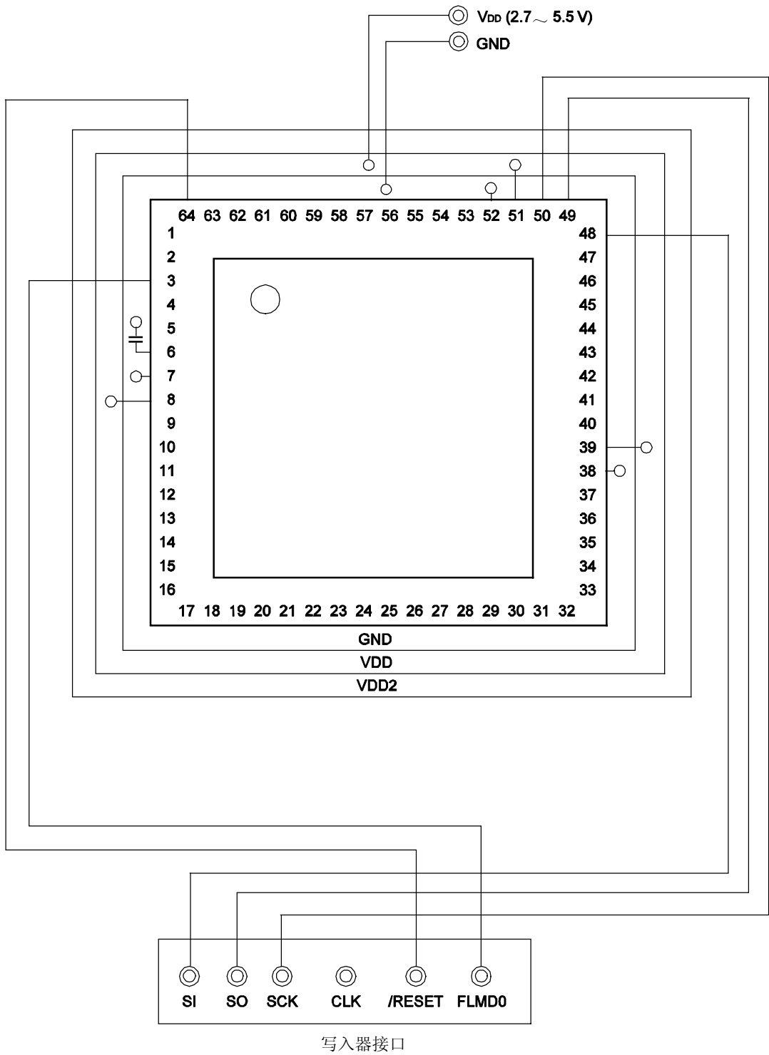
图 24-2. 3 线串行 I/O (CSI10) 模式下使用适配器对 Flash 存储器进行写操作示例
