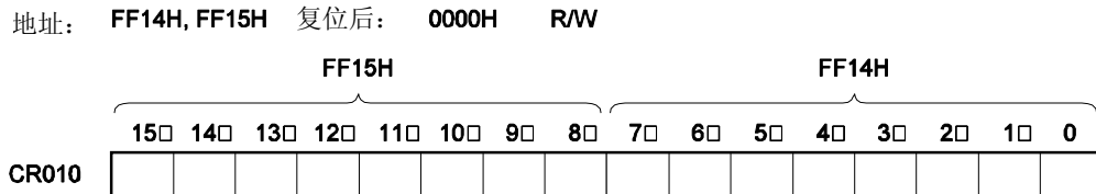
图 6-4. 16 位定时器捕捉/比较寄存器 010 (CR010)的格式
