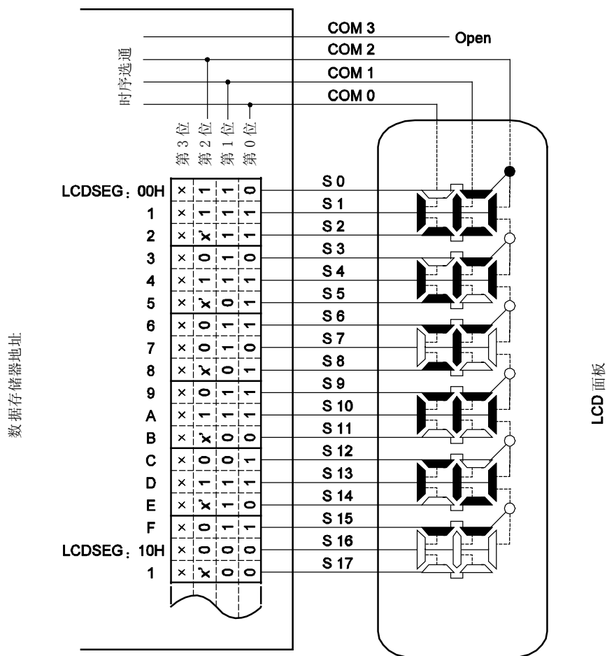
图 17-22. 3 分时 LCD 面板连接举例
