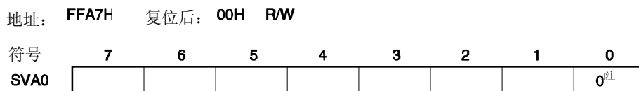
图 16-4. 从地址寄存器 0 的格式 (SVA0)
