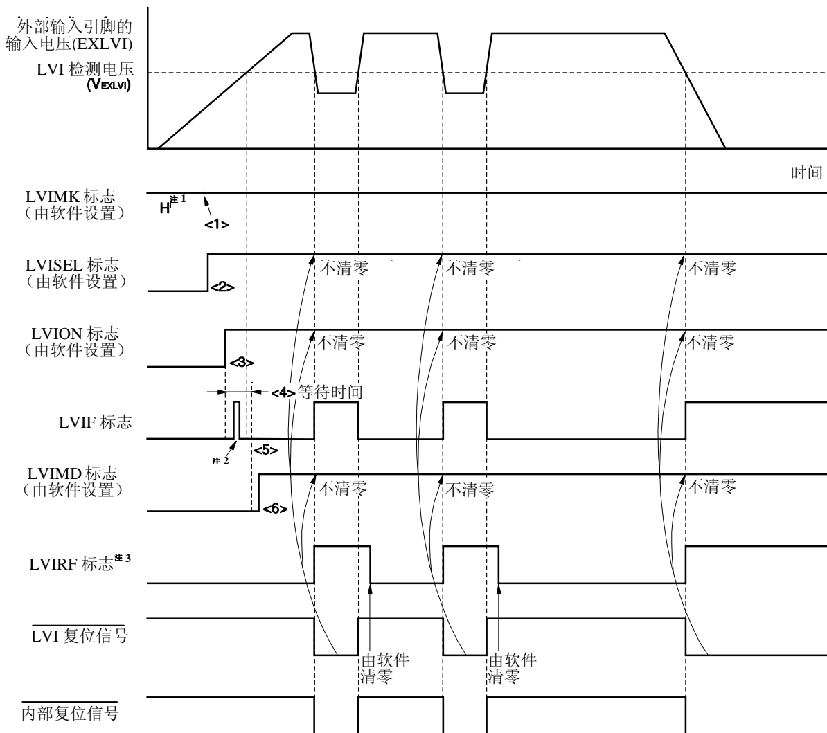
图 22-6. 低电压检测电路内部复位信号产生时序 (检测外部输入引脚的输入电压(EXLVI)的等级)
