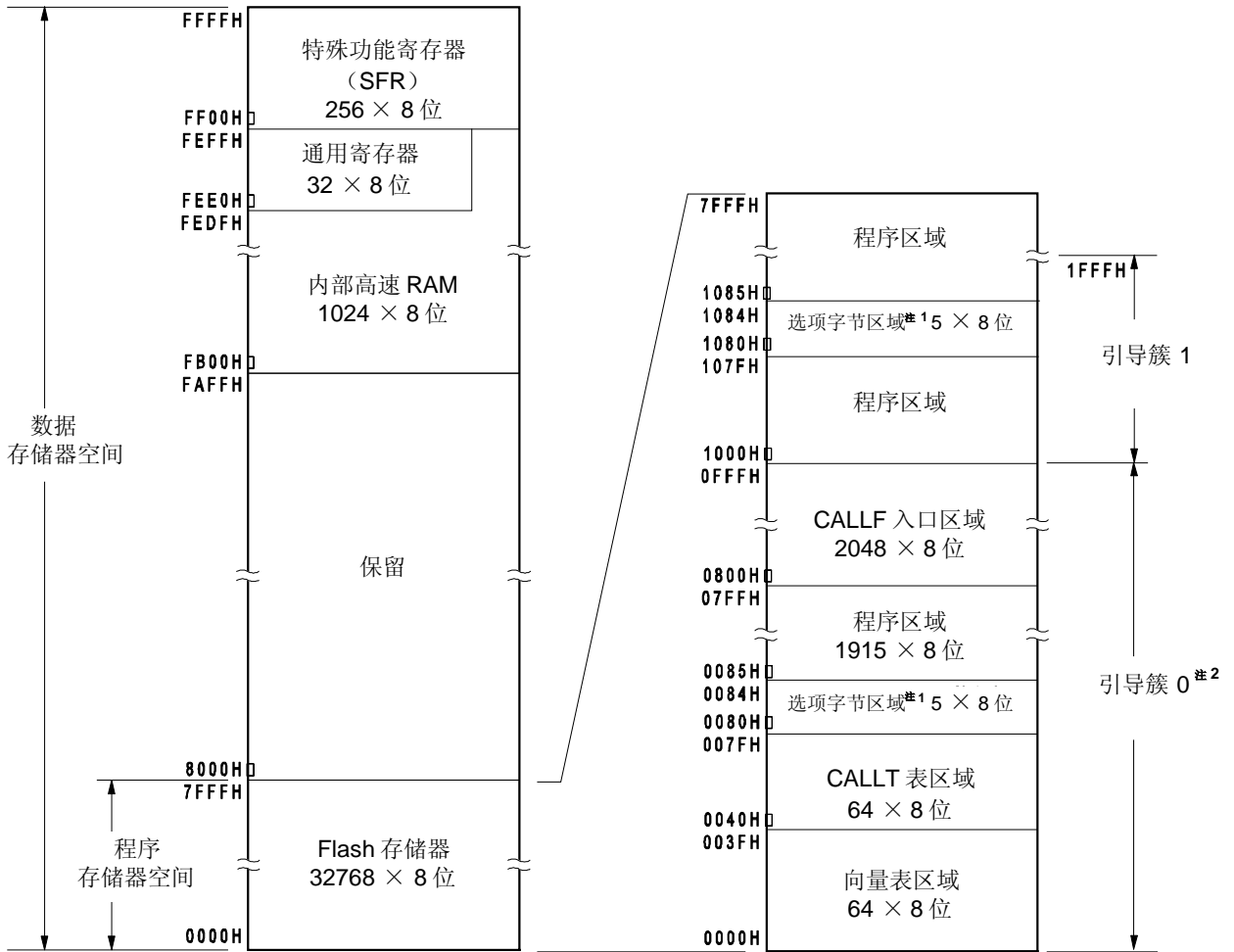
图 3-3. 存储空间映射图 (μPD78F0363)
