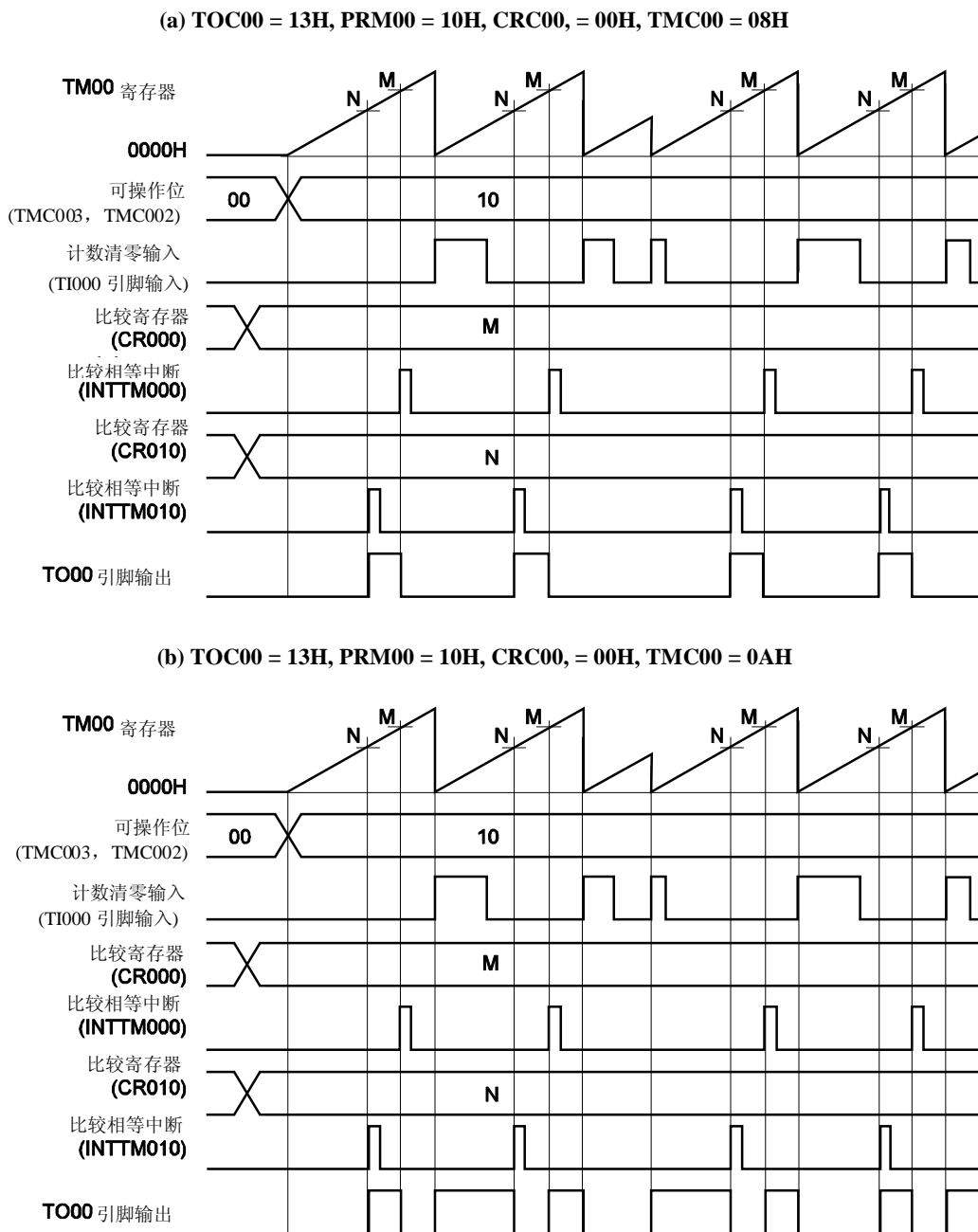
图 6-23. 清零&启动模式(通过 TI000 引脚有效沿输入进入)时序示例 (CR000: 比较寄存器, CR010: 比较寄存器)
