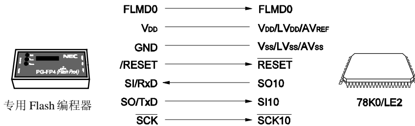
图 24-5. 专用 Flash 编程器的通信 (CSI10)
