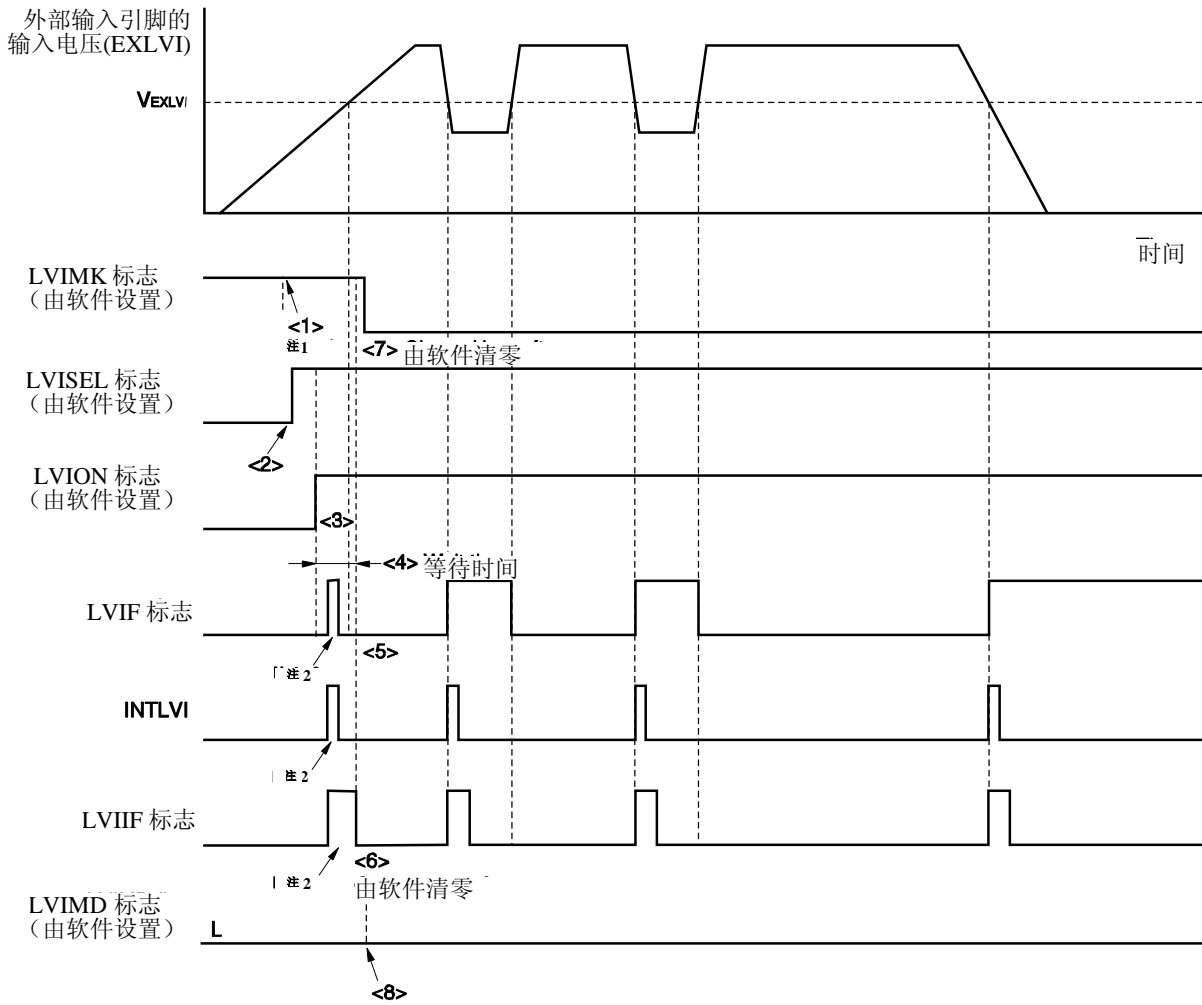
图 22-8. 低电压检测电路中中断信号产生时序 (检测外部输入引脚的输入电压 (EXLVI) 等级)
