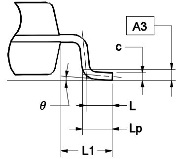
引脚端详图
