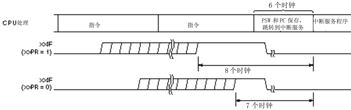
图 18-8. 中断请求响应时序 (最短时间)
