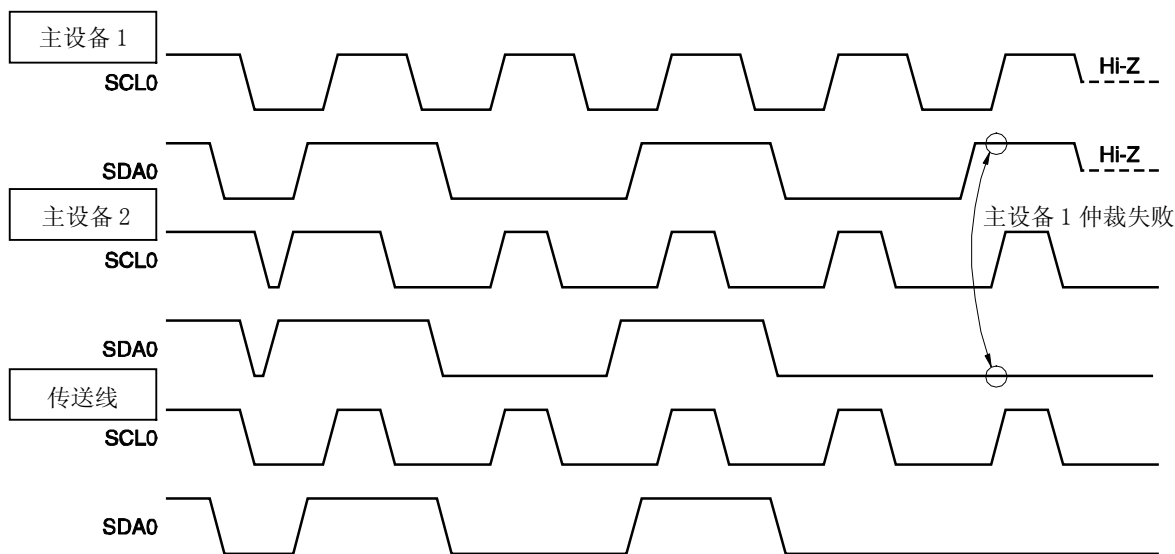
图 16-19. 仲裁时序举例
