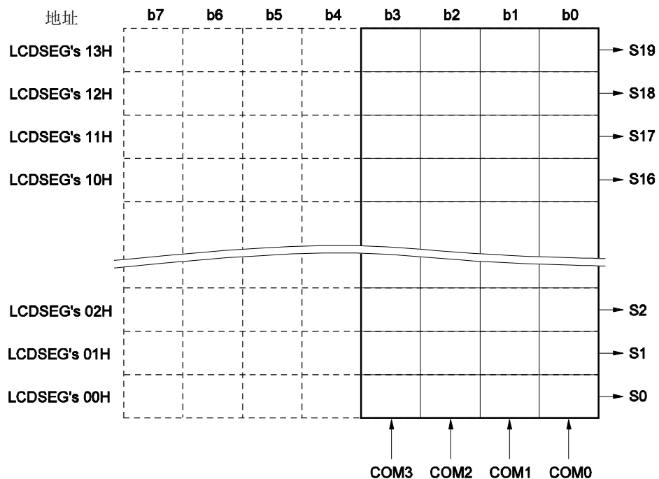
图 17-12. LCD 显示数据存储的内容和 segment/common 输出的关系
