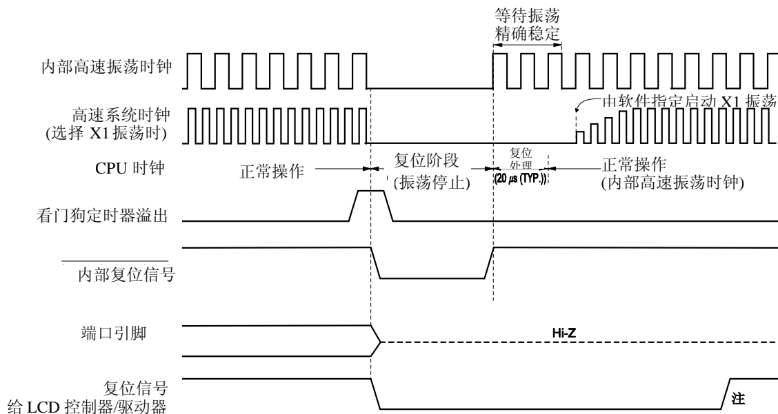
图 20-3. 由于看门狗定时器溢出进行复位的时序
