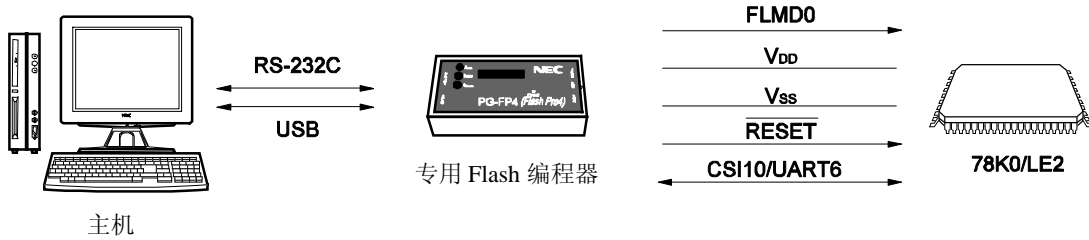
图 24-4. Flash 存储器编程环境
