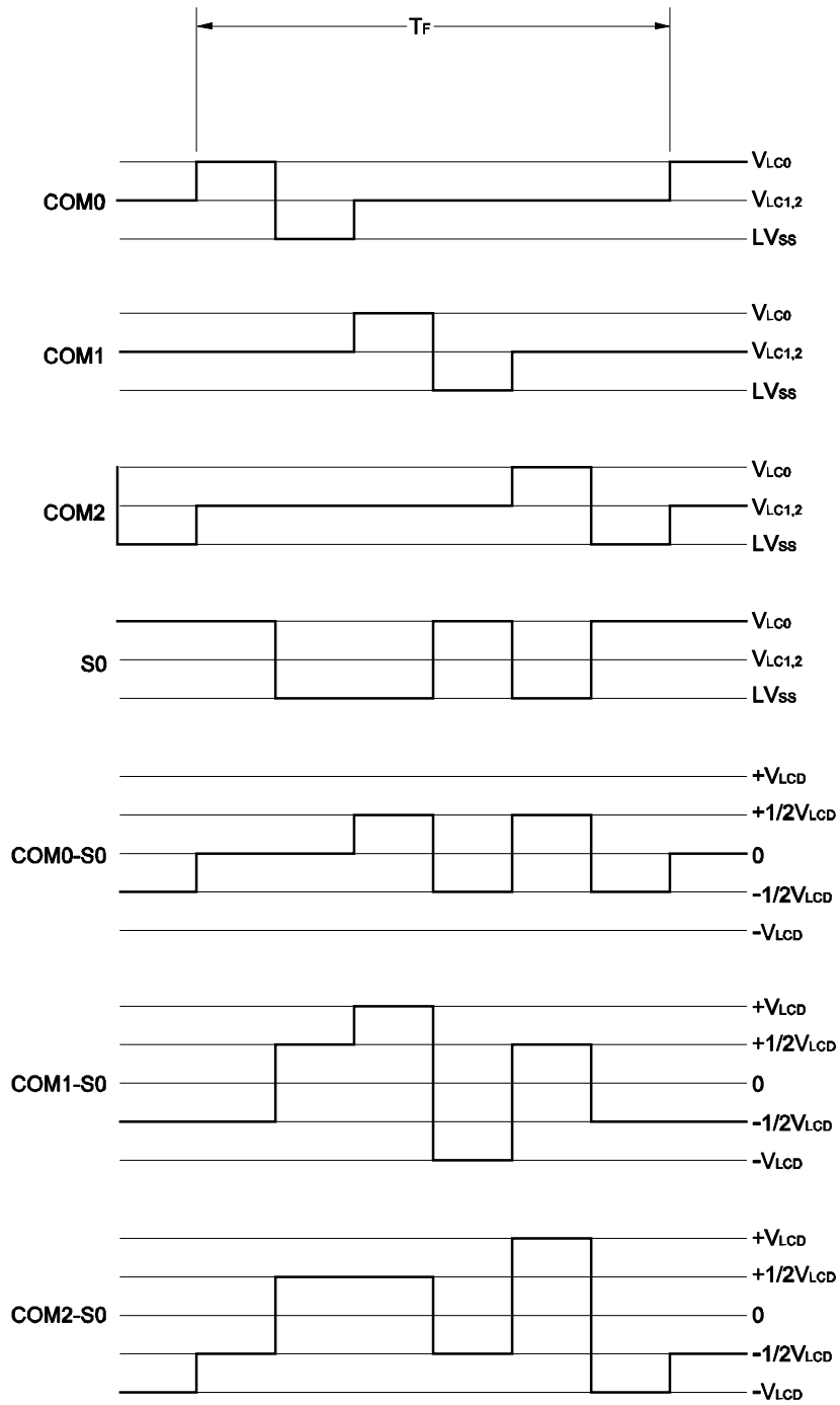
图 17-23. 3 分时 LCD 驱动波形举例 (1/2 偏压模式)
