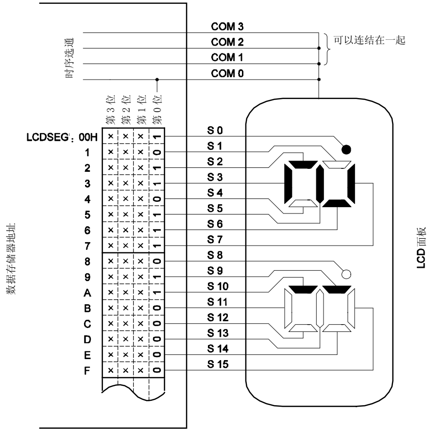
图 17-16. 静态 LCD 面板连接举例
