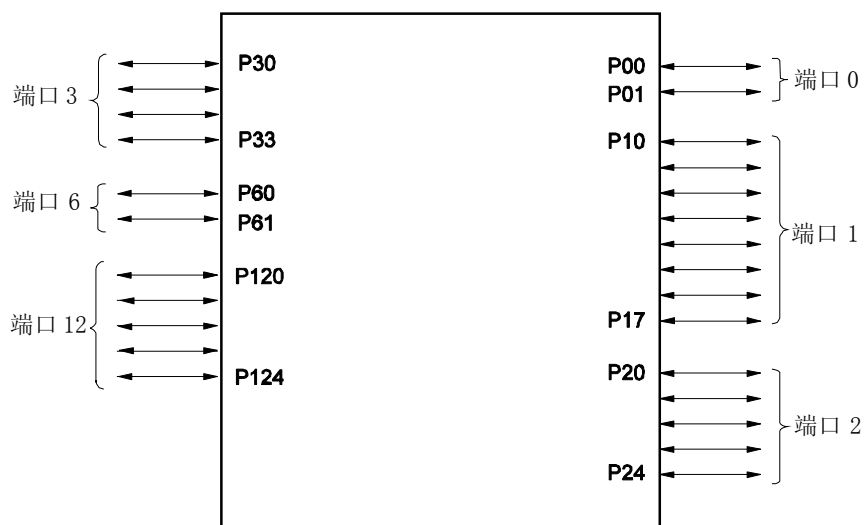
图 4-1. 端口类型
