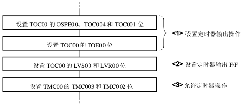
图 6-53. LVS00 和 LVR00 设置流程示例
