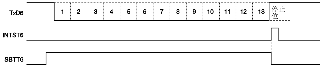
图 14-22. SBF 发送
