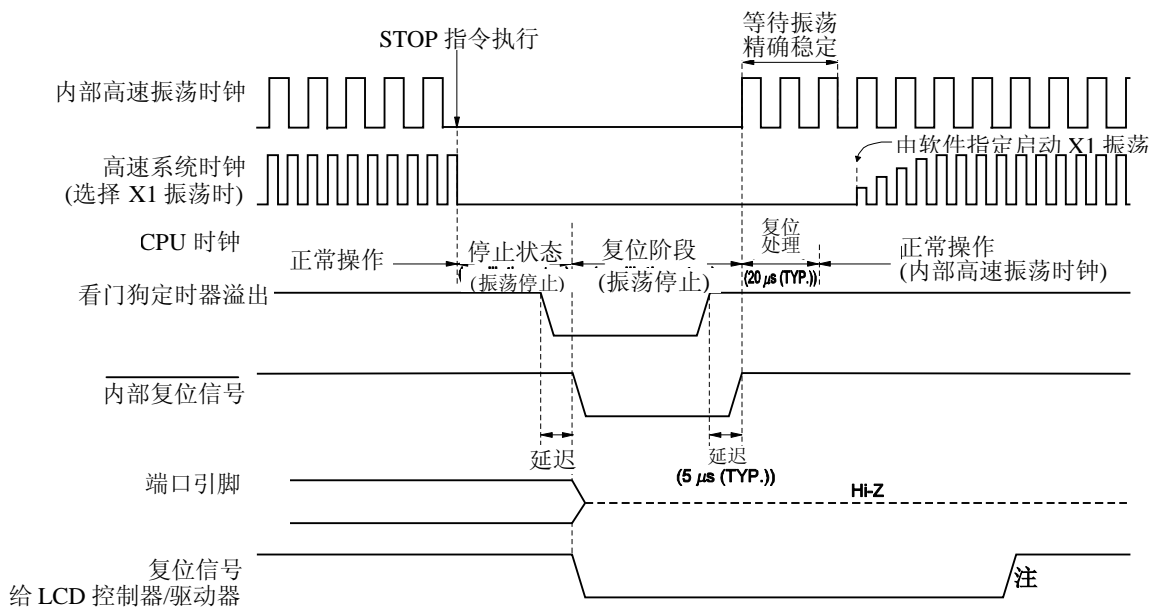
图 20-4. 在 STOP 模式下通过 RESET 输入进行复位的时序
