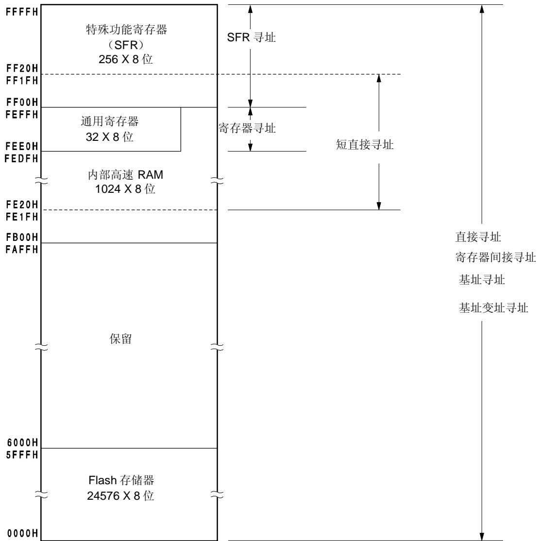
图 3-6. 数据存储与寻址方式的对应关系 (μPD78F0362)
