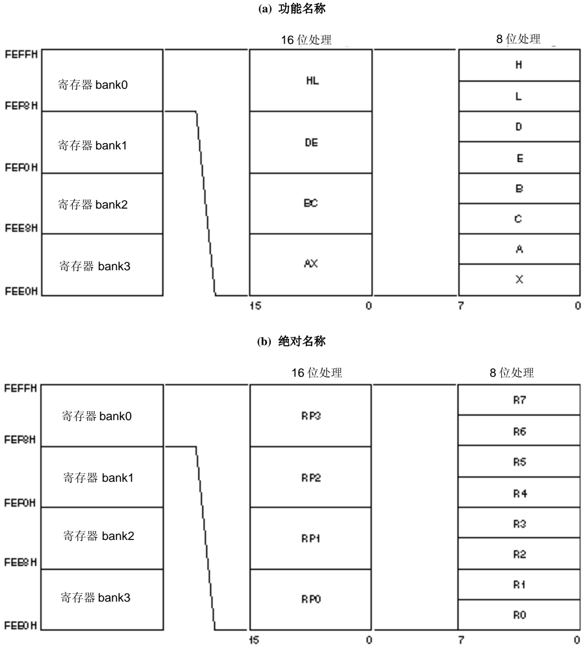
图 3-13. 通用寄存器结构
