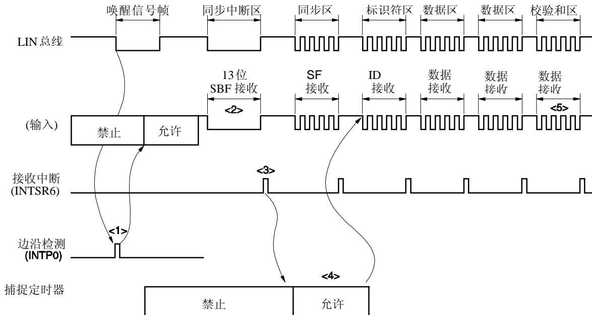
图 14-2. LIN 接收操作
