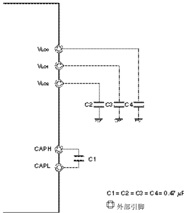
图 17-30. LCD 驱动器引脚连接举例
