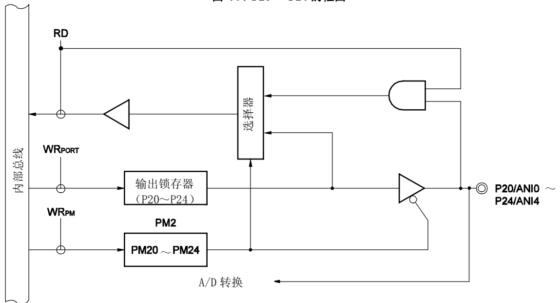
图 4-9. P20 ~ P24 的框图
