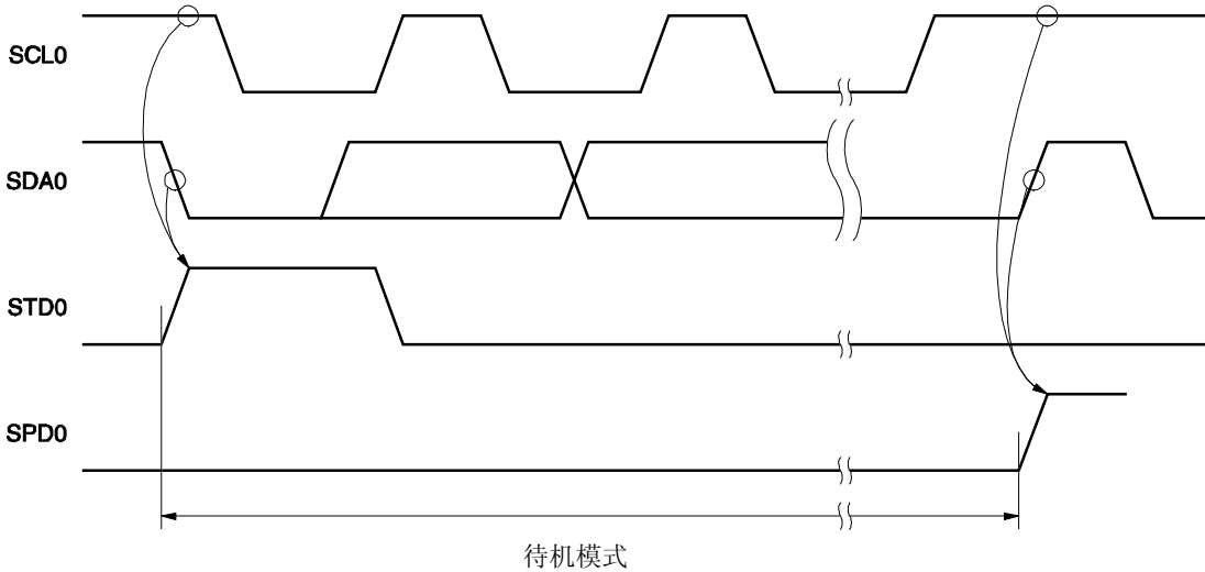
图 16-21. 接受通信预约的时序
