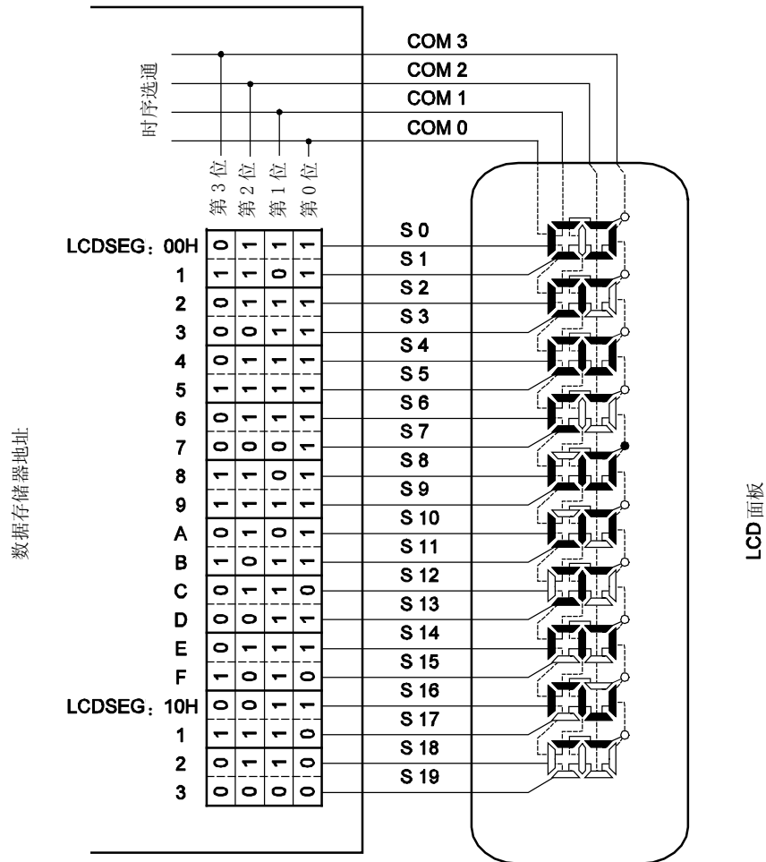
图 17-26. 4 分时 LCD 面板连接举例
