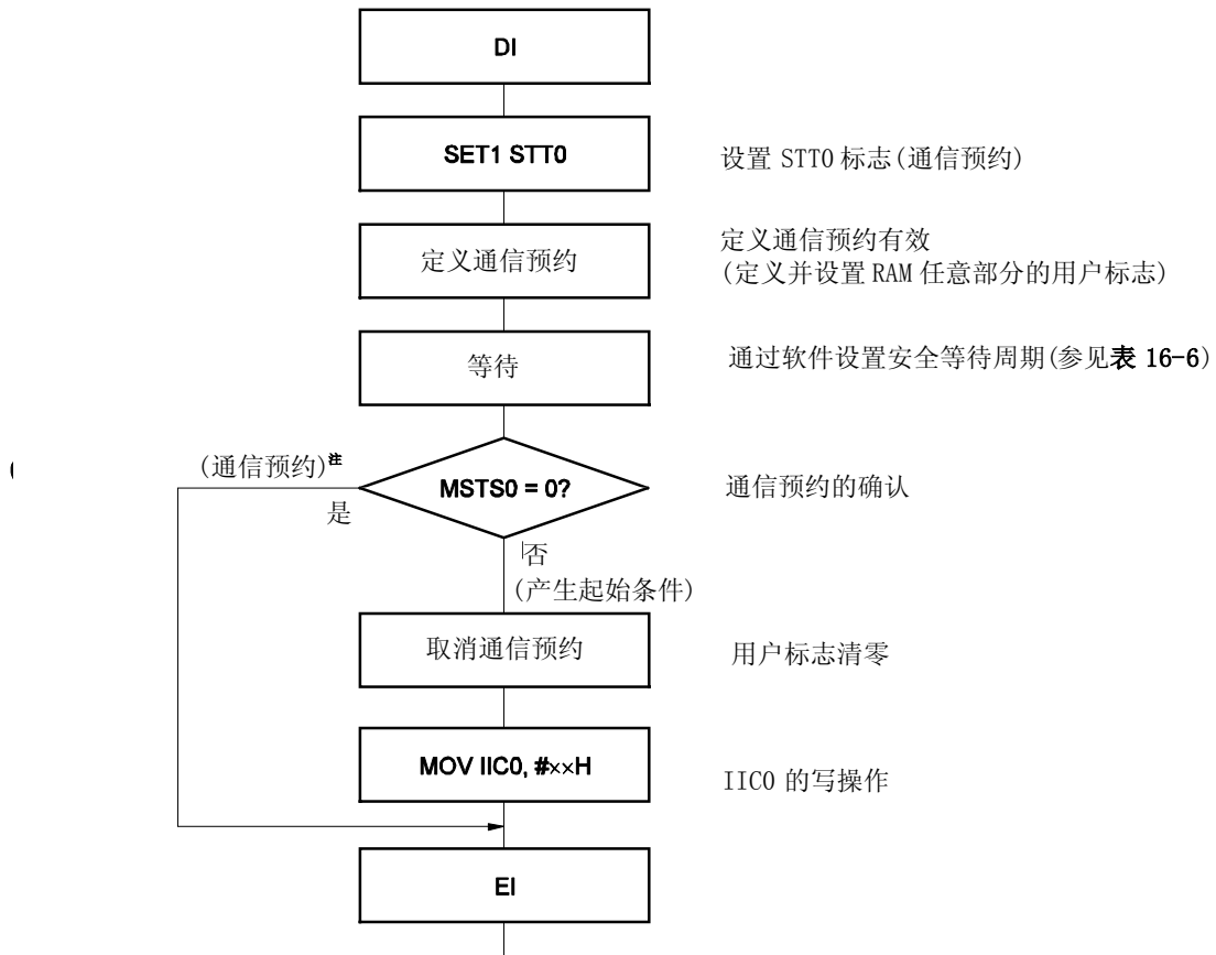
图 16-22. 通信预约协议
