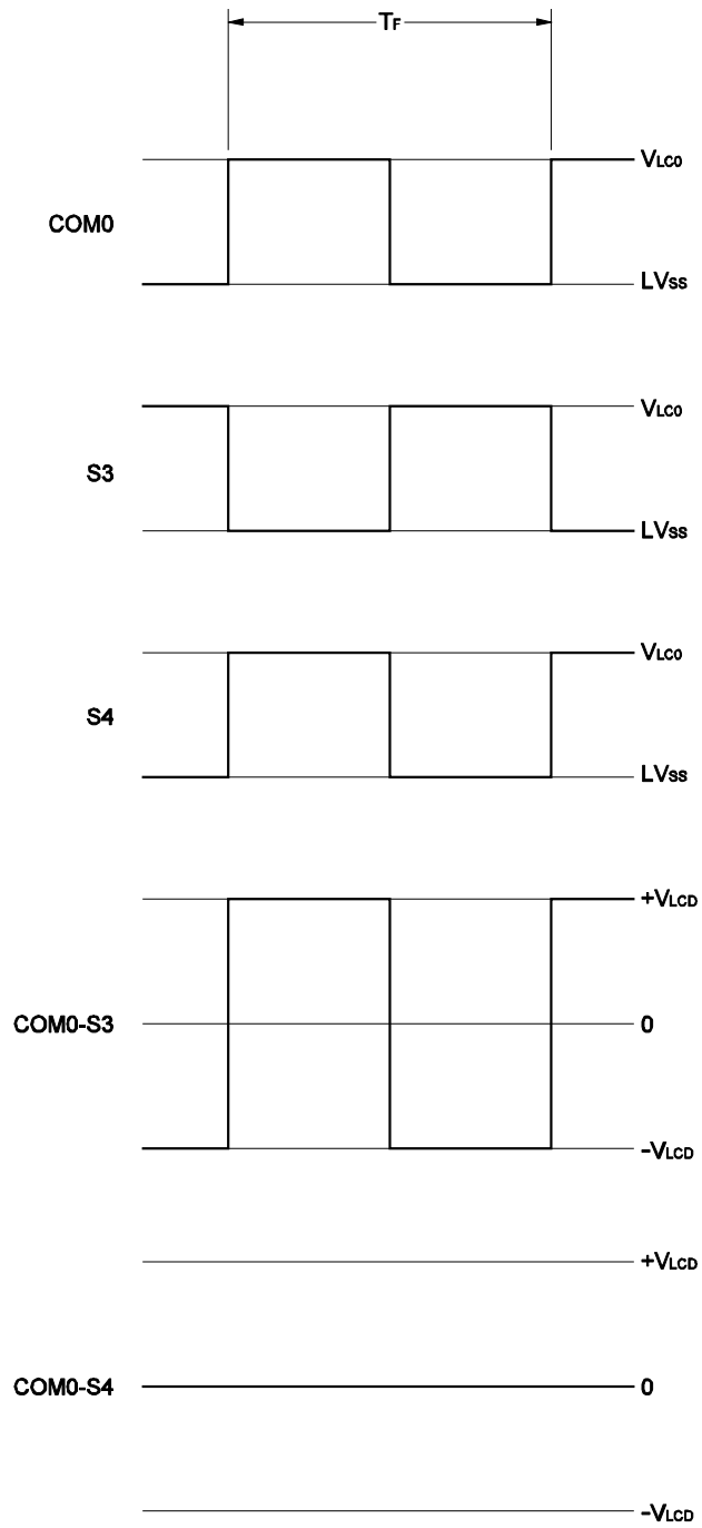
图 17-17. 静态LCD 驱动波形举例
