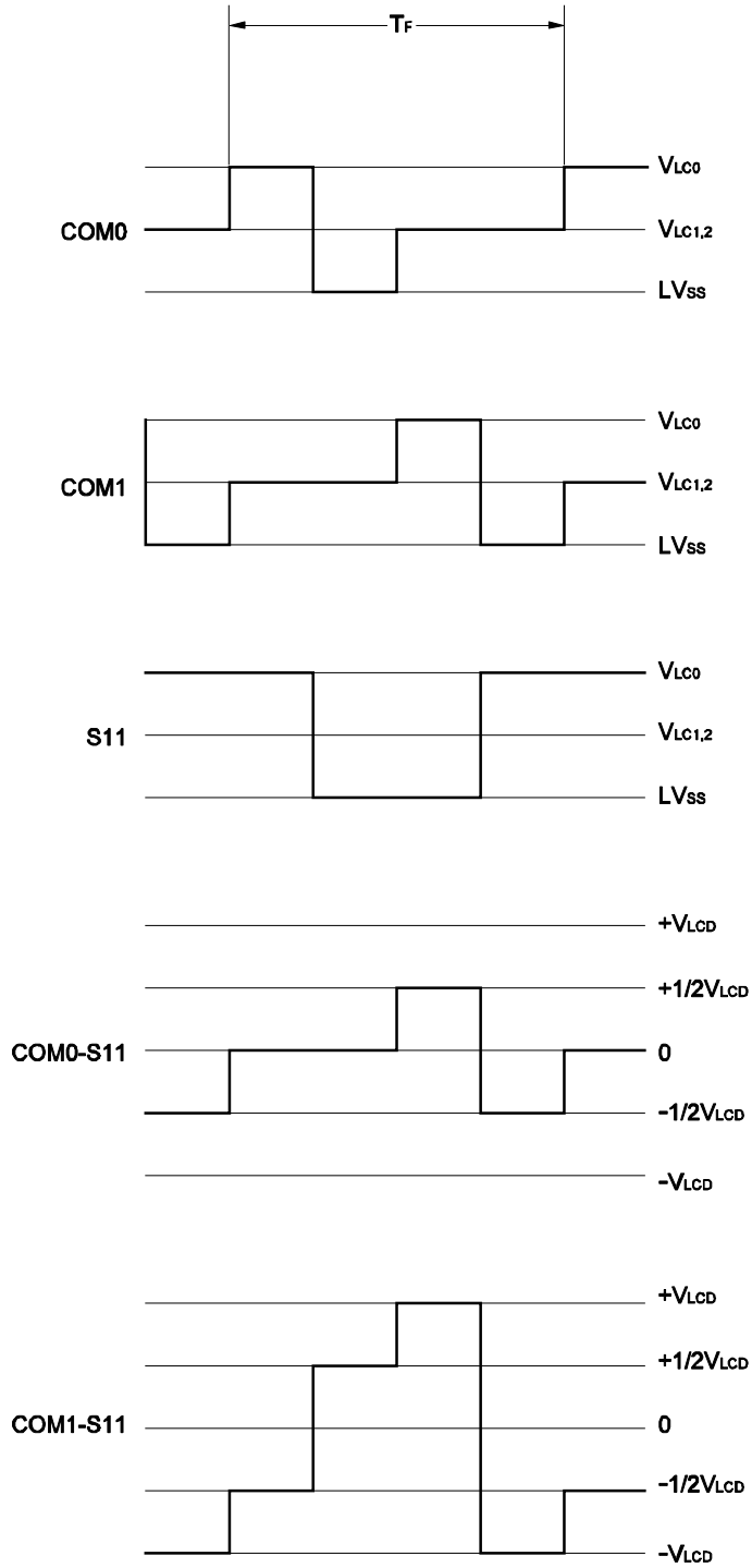
图 17-20. 2 分时 LCD 驱动波形举例 (1/2 偏压模式)
