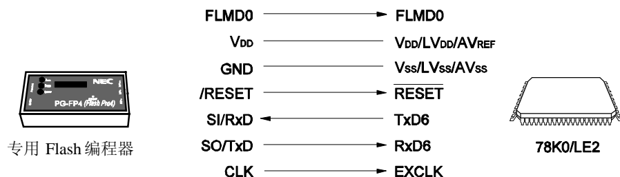
图 24-6. 专用 Flash 编程器的通信 (UART6)
