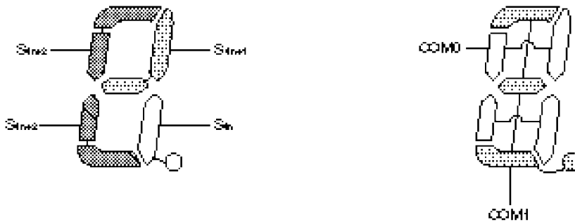
图 17-18. 2 分时 LCD 显示模式和电极连接
