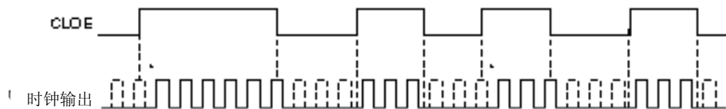
图 11-4. 时钟输出应用举例
