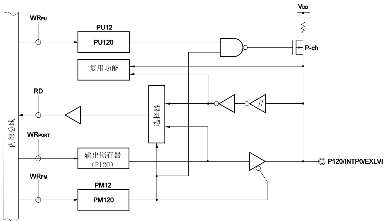
图 4-13. P120 的框图
