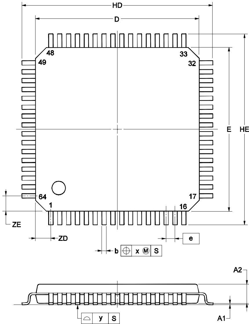
64引脚塑封LQFP (12x12)
