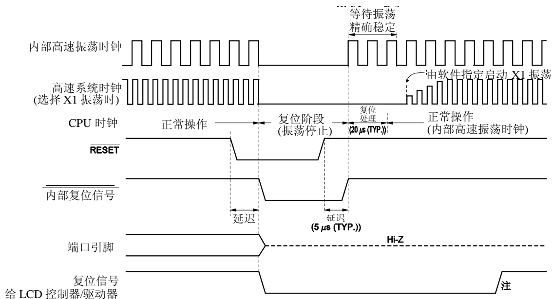
图 20-2. 由 RESET 输入进行复位的时序
