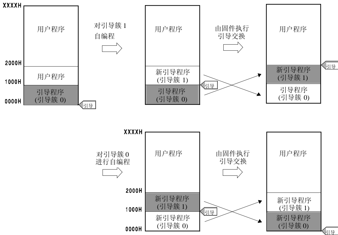
图 24-15. 引导交换功能
