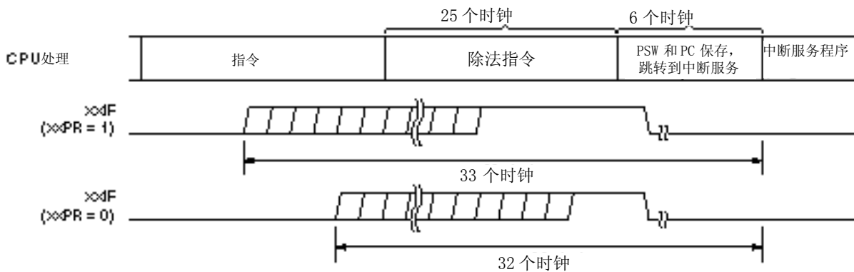
图 18-9. 中断请求响应时序 (最长时间)
