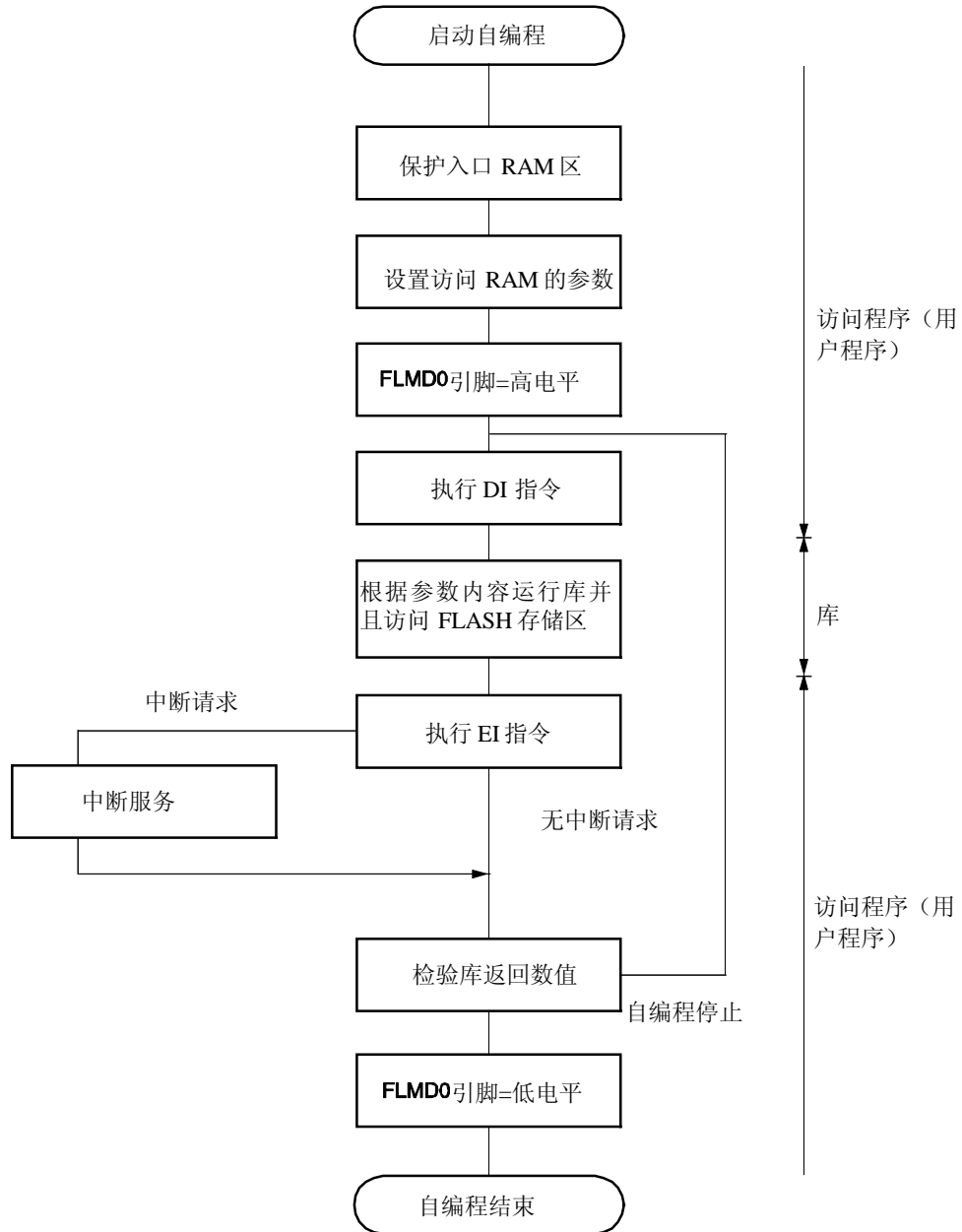
图 24-14. 自编程流程
