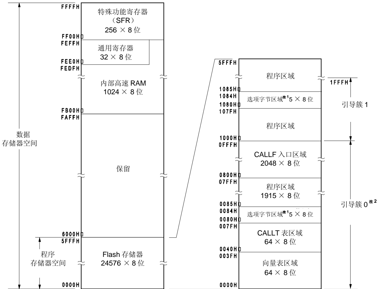
图 3-2. 存储空间映射图 (μPD78F0362)
