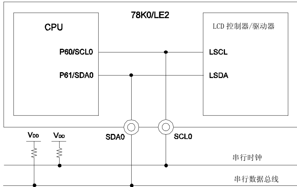
图 16-29. 系统结构
