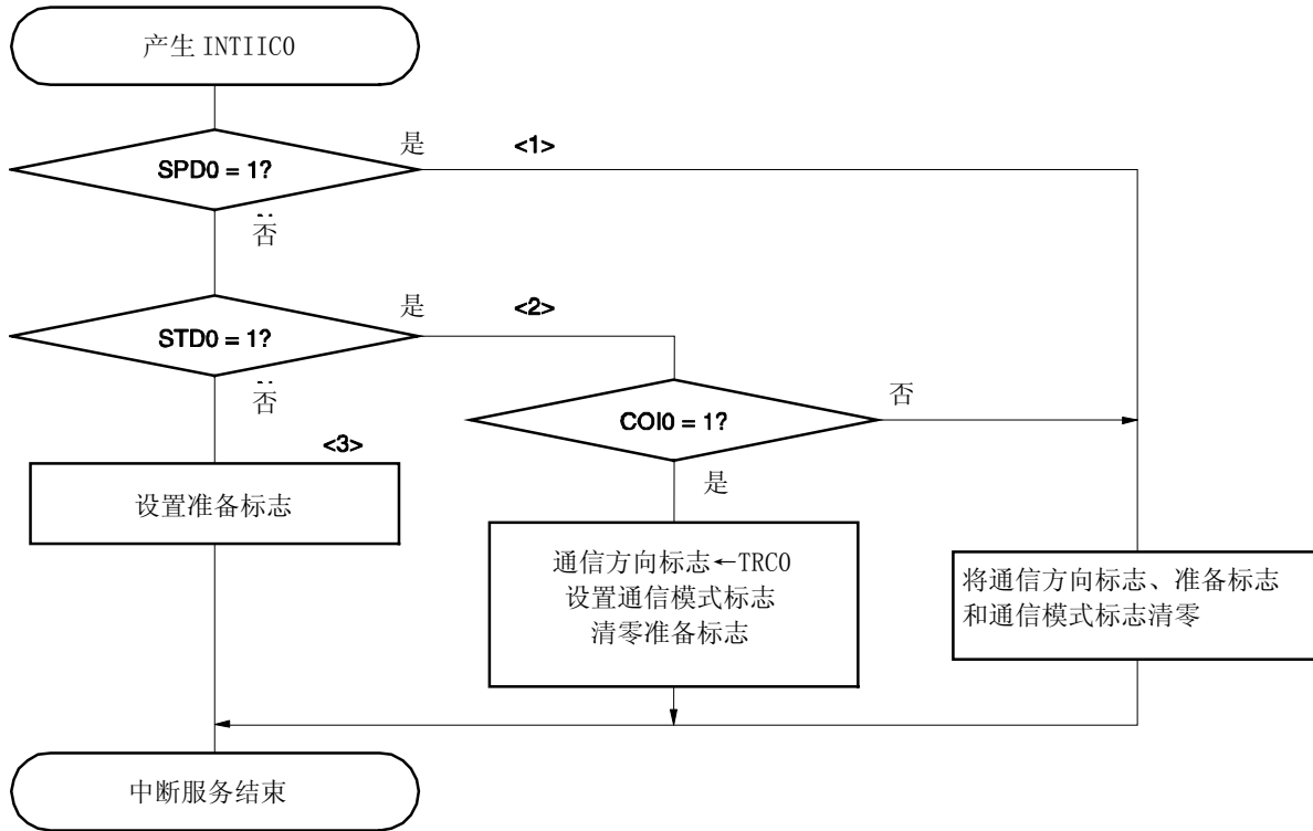
图 16-26. 从设备操作流程(2)
