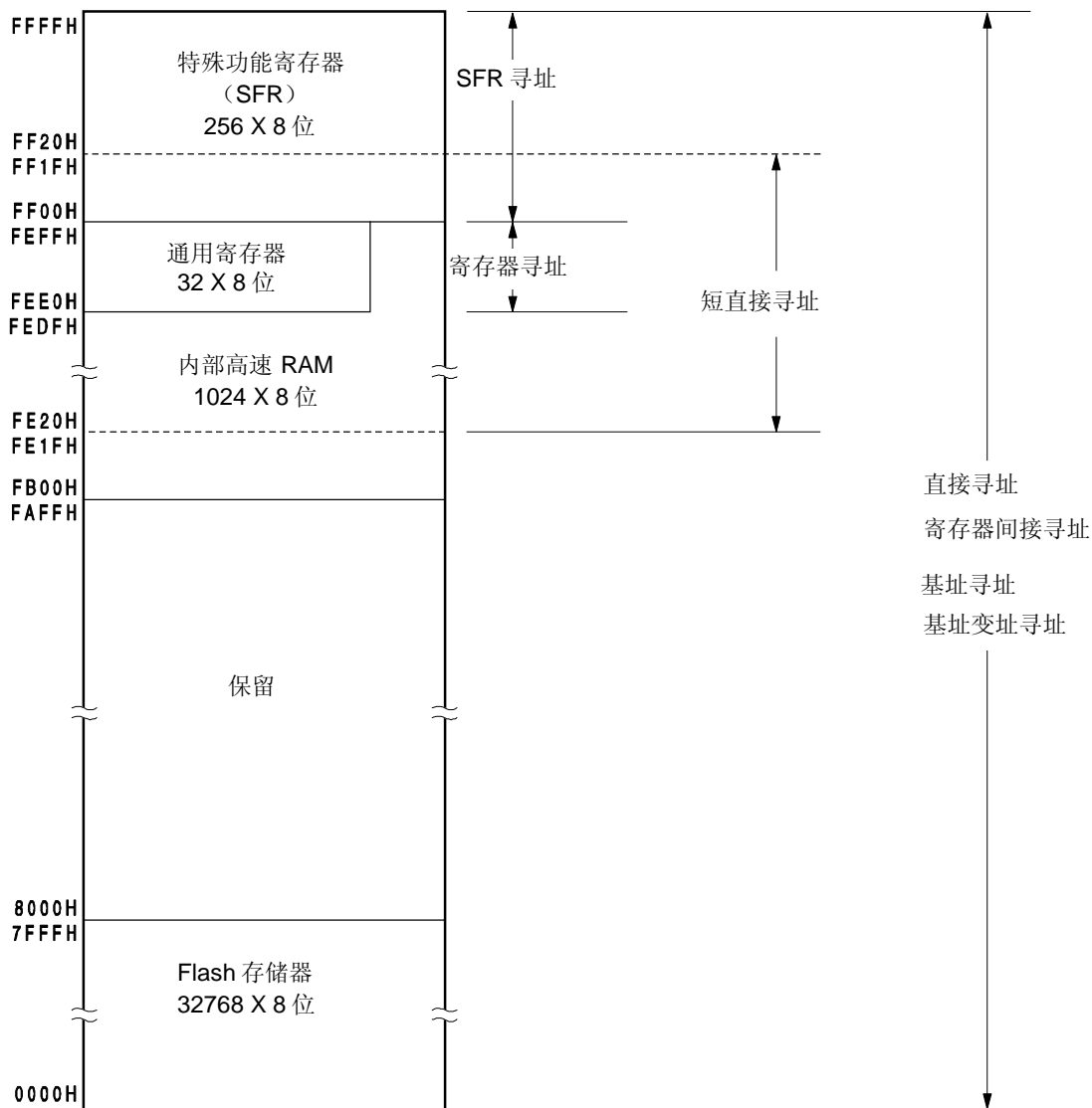
图 3-7. 数据存储器与寻址方式的对应关系 ( \mu PD78F0363, 78F0363D)
