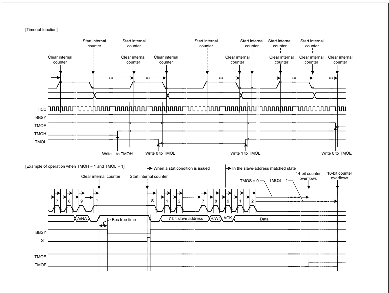
Figure 25.48 Timeout function using the TMOE, TMOS, TMOH, and TMOL bits
