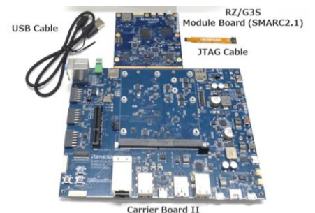
RZ/G3S-EVKit
