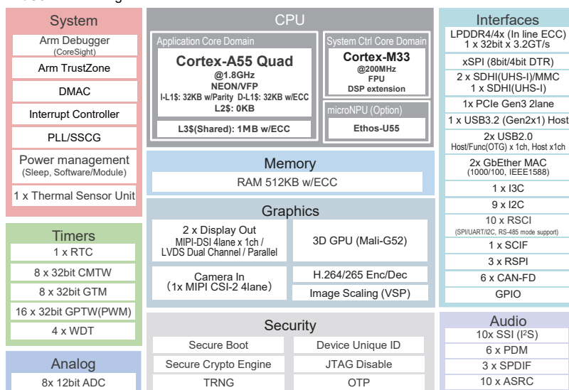
RZ/G3E Block Diagram
