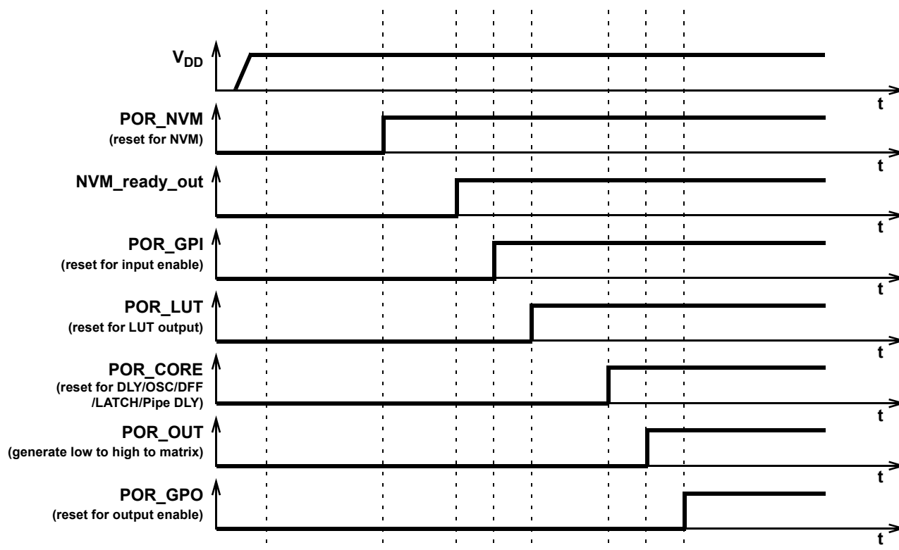
Figure 84. POR Sequence
