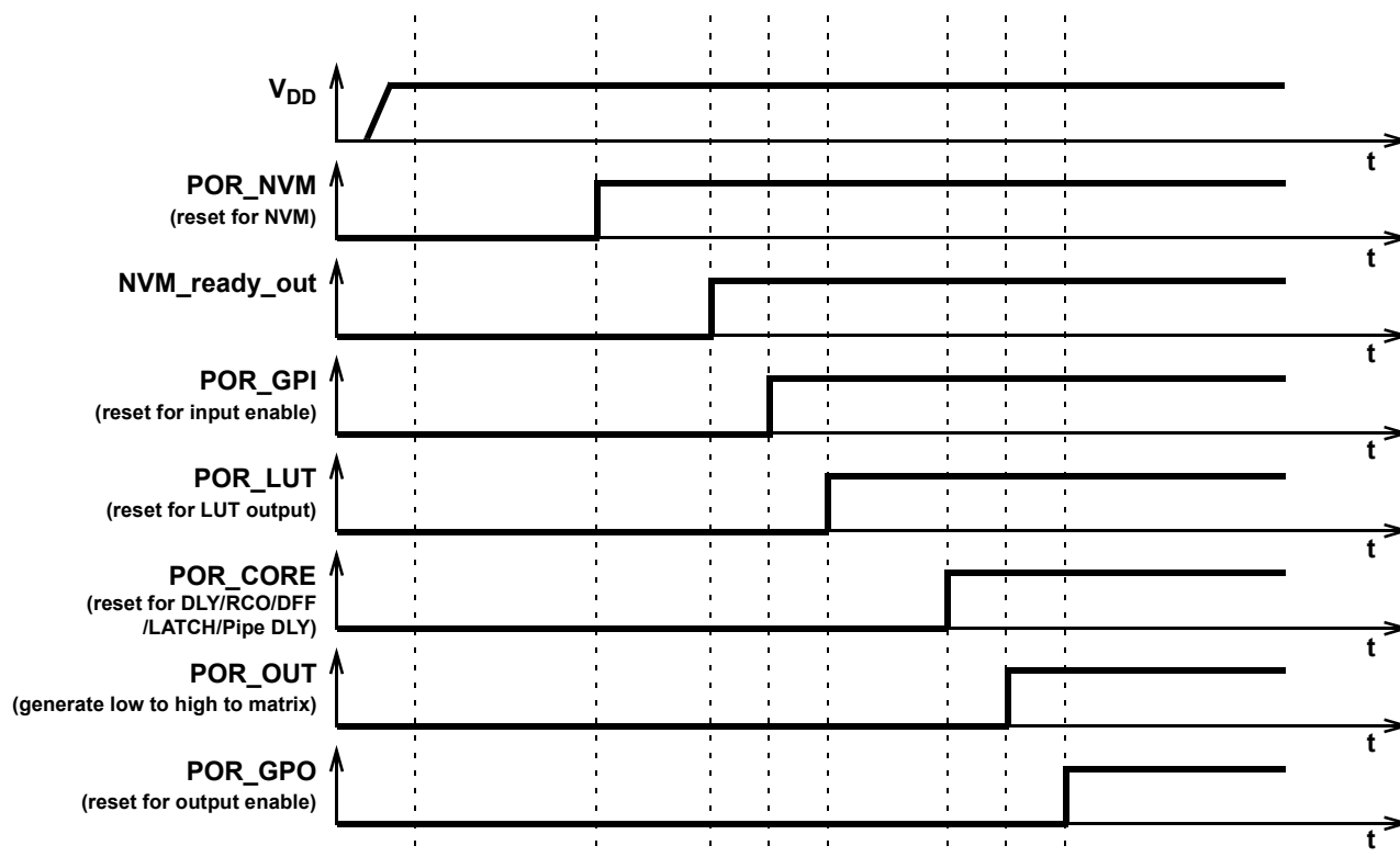
Figure 92. POR Sequence
