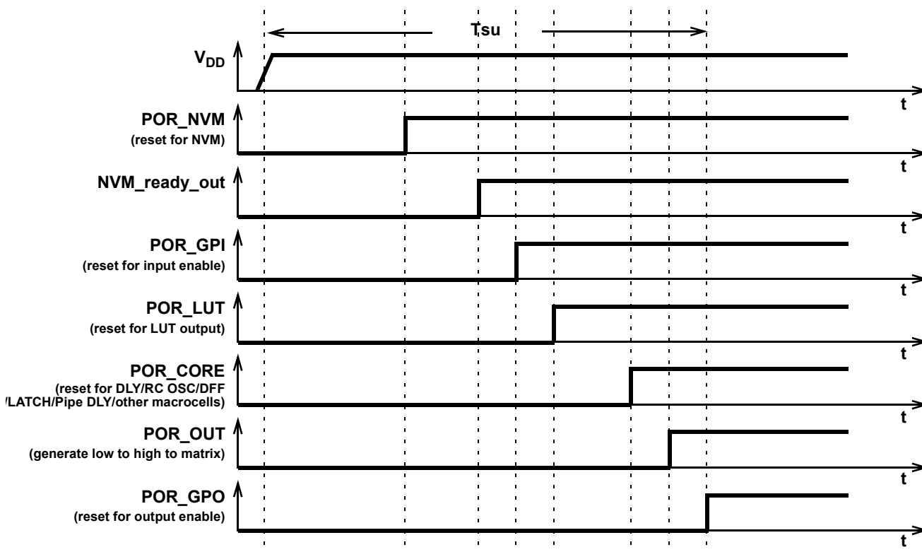
Figure 39. POR Sequence
