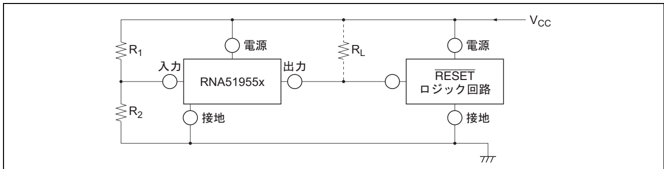
図 1 RNA51955 のリセット回路への応用
