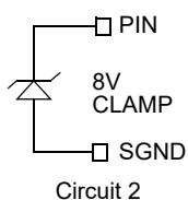
ESD Circuits
