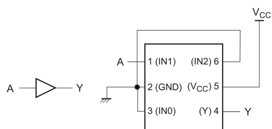
図 7. Non-Invert Buffer
