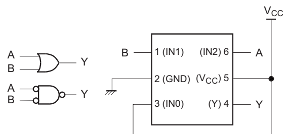
図 5. 2-inputs OR Gate
