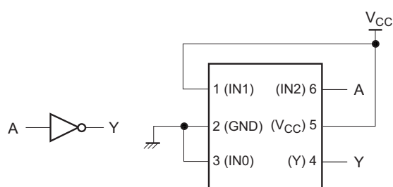
図 6. Inverter
