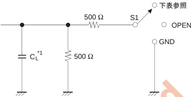
負荷回路
