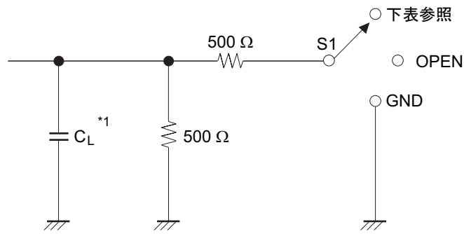
負荷回路
