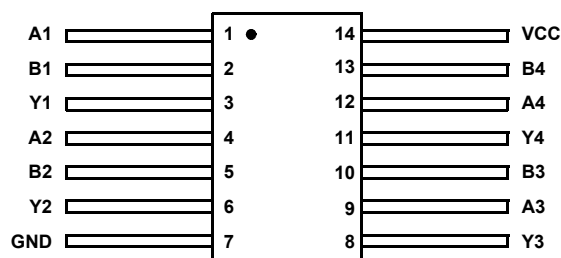
TRUTH TABLE
