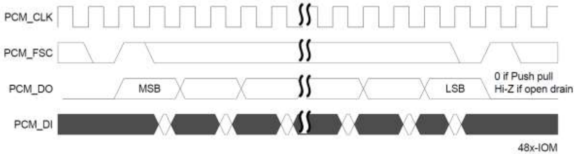
Figure 67. IOM format
