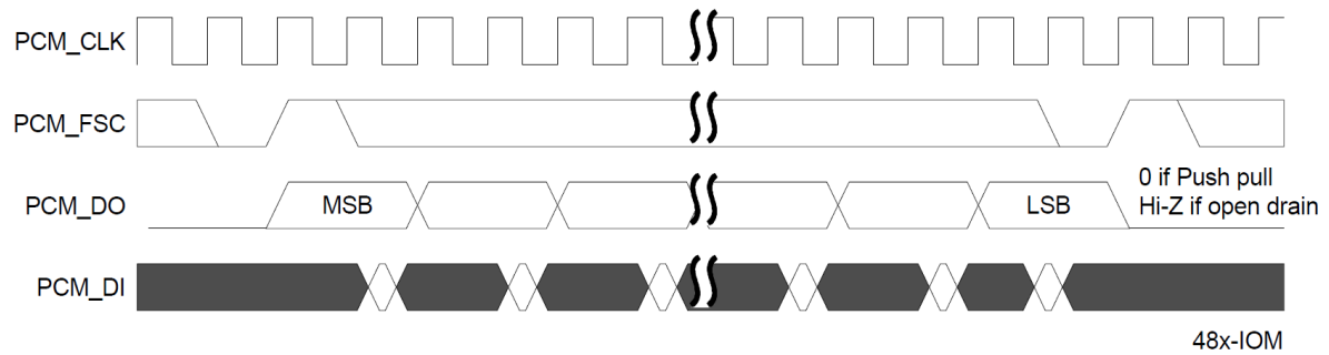
Figure 68: IOM format
