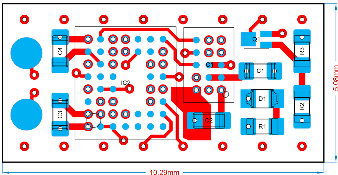
Figure 24. Reference Design 2: Mini Module - Assembly View TOP
