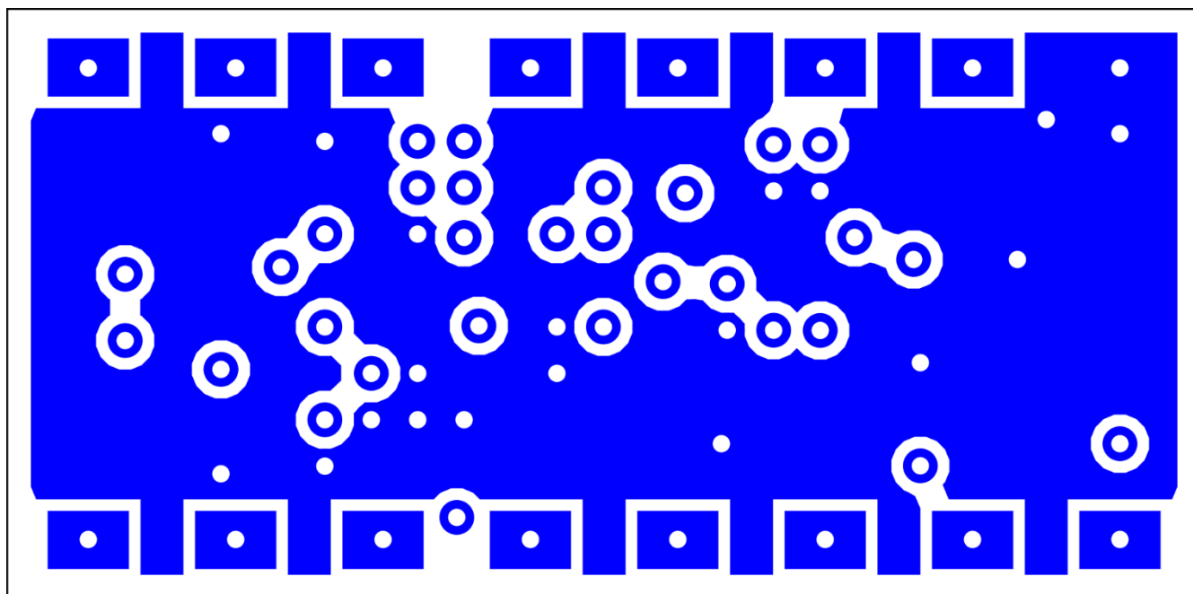
Figure 23. Reference Design 2: Mini Module - BOT Layer
