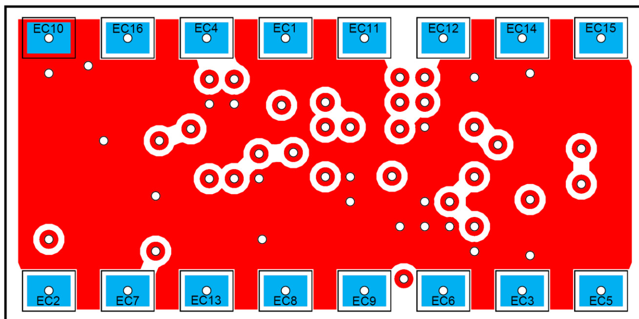
Figure 25. Reference Design 2: Mini Module - Assembly View BOT
