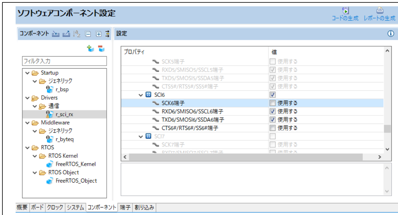
図 3-11 SCI チャンネル 6 の端子設定
