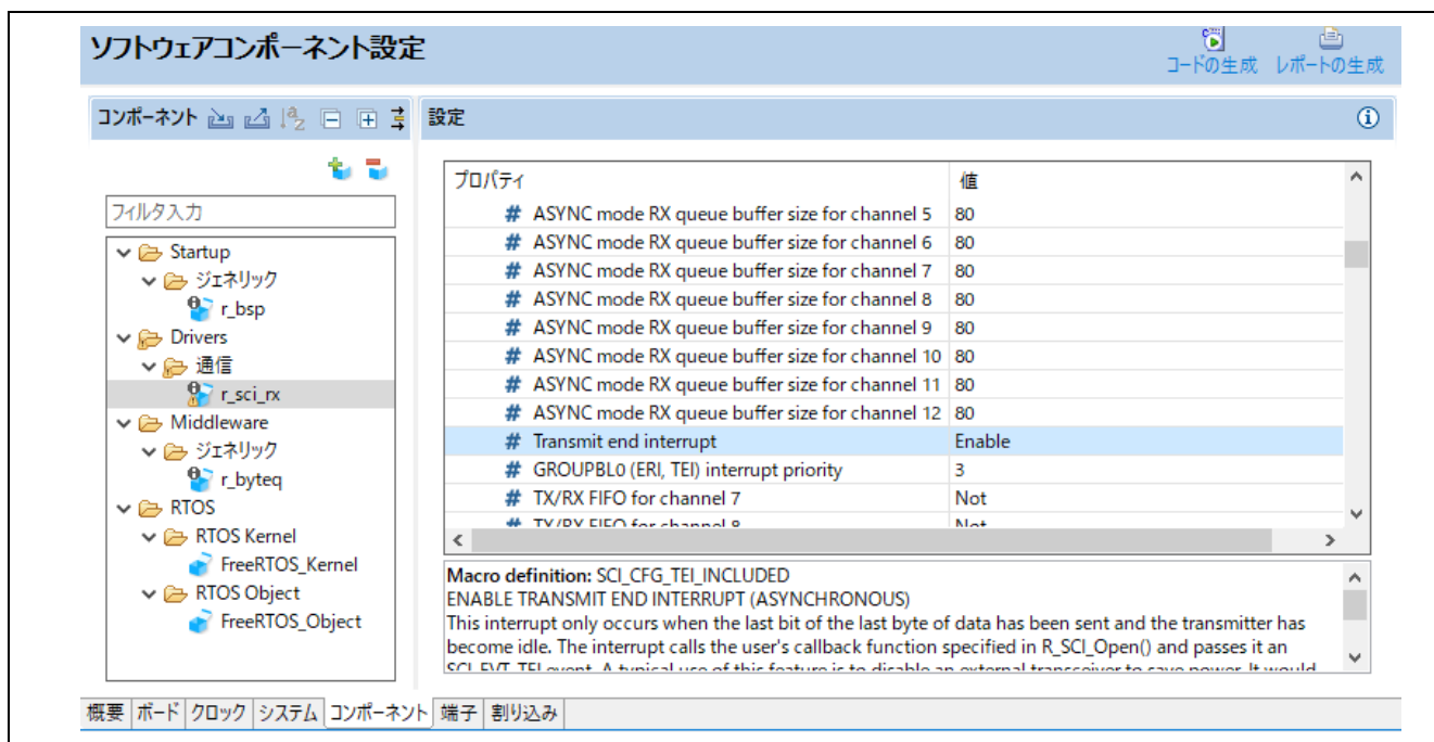
図 3-10 SCI チャンネル 6 の割り込みの設定
