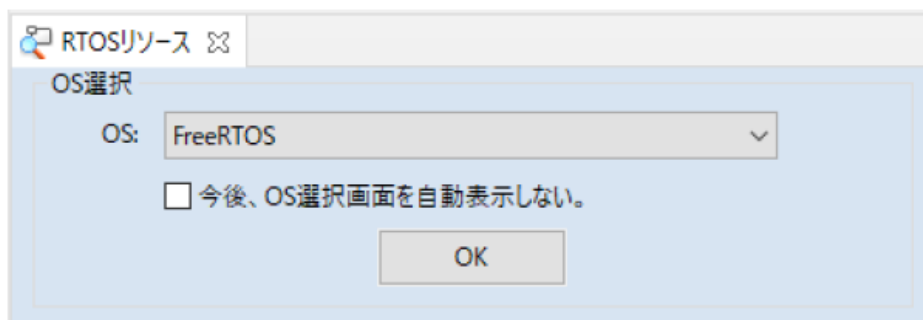
図 3-22 OS の選択
