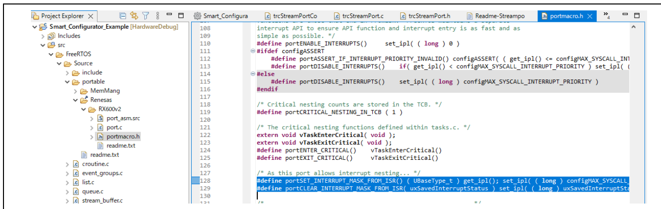
図 3-15 portmacro.h
