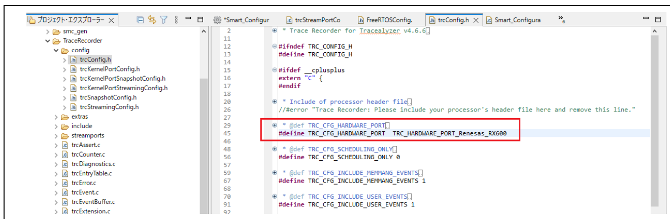
図 3-5 trcConfig.h の修正
