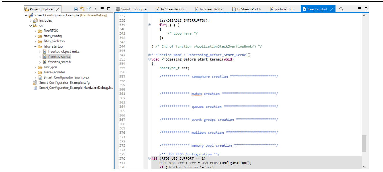
図 3-16 freertos_start.c
