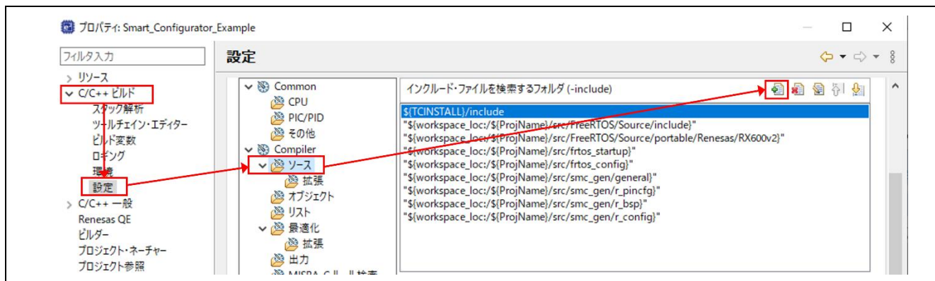
図 3-14 パスの追加
