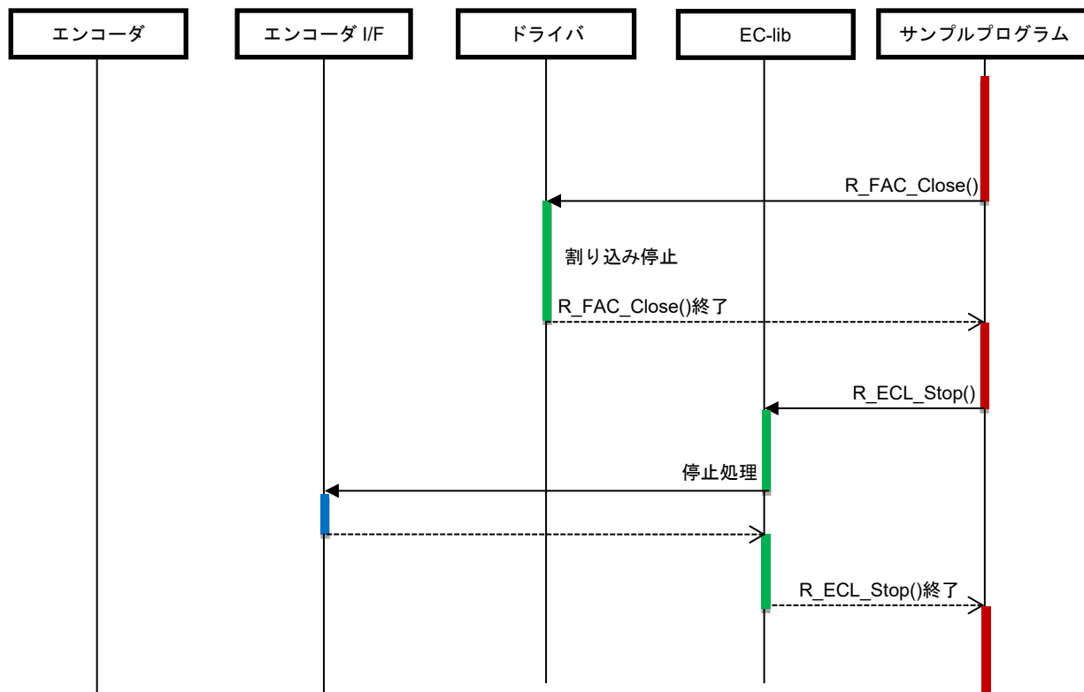
図 4-21 停止シーケンス図
