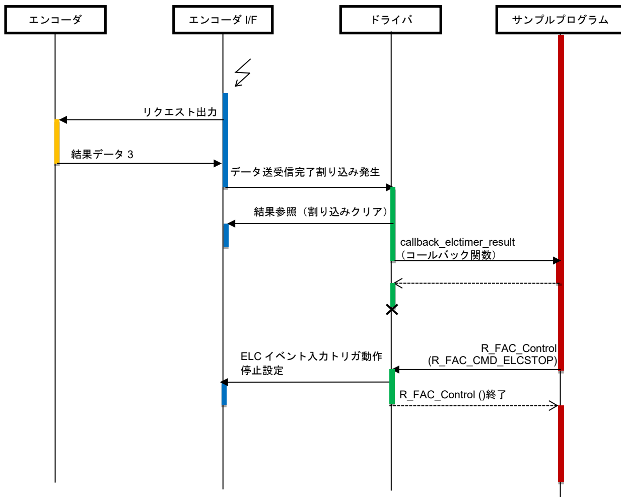
図 4-20 ELC イベント入カトリガ動作のシーケンス図
