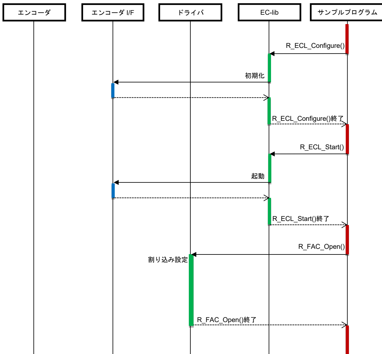
図 4-18 開始シーケンス図
