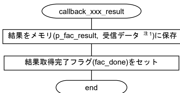
図 4-16 callback_xxx_result 関数のフローチャート
