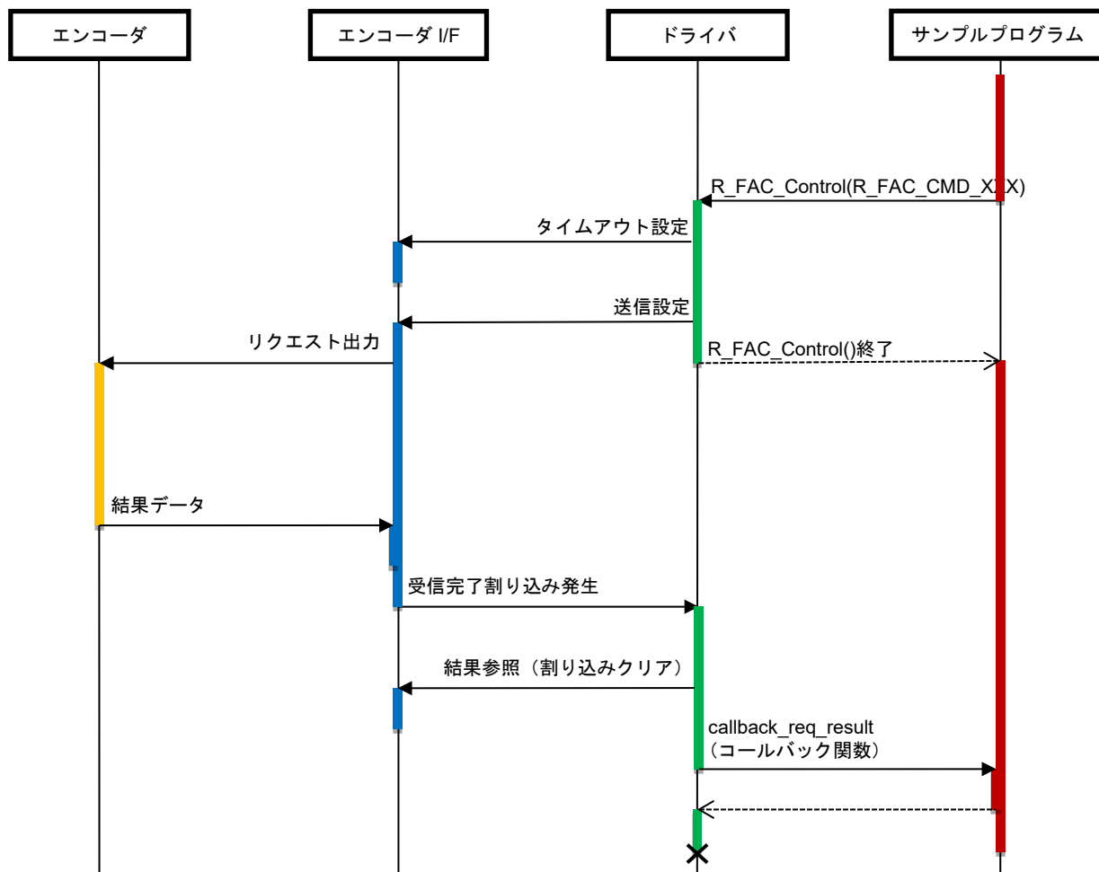
図 4-19 リクエスト・データ受信シーケンス図
