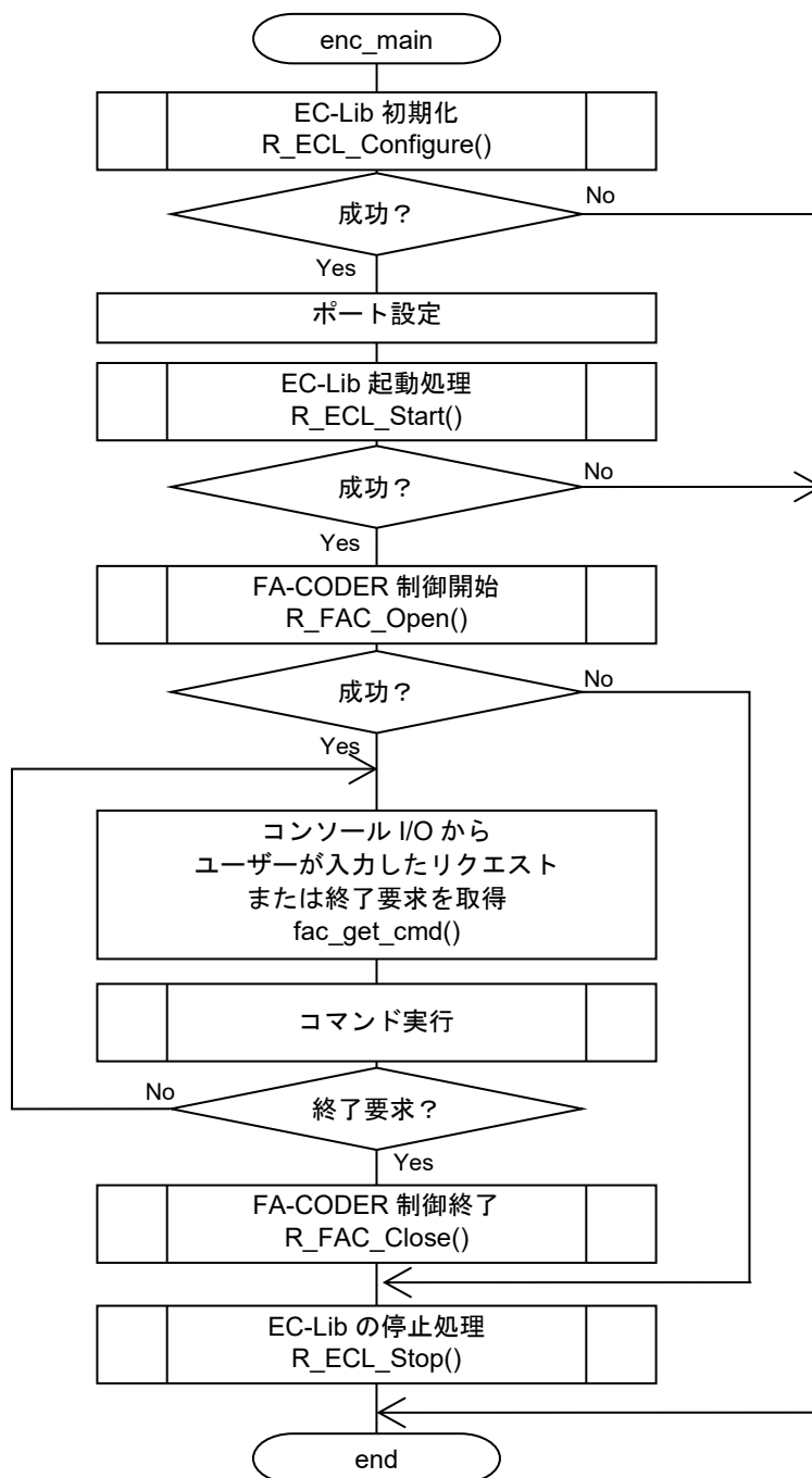
図 4-3 enc_main 関数のフローチャート
