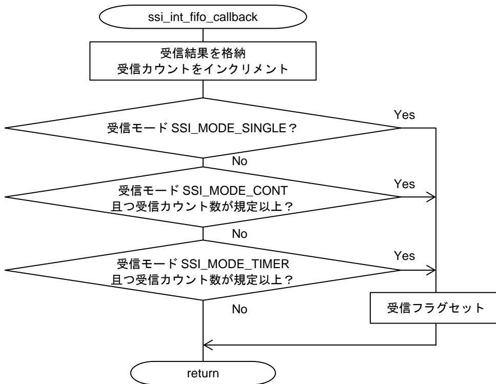
図 4-11 ssi_int_fifo_callback 関数のフローチャート
