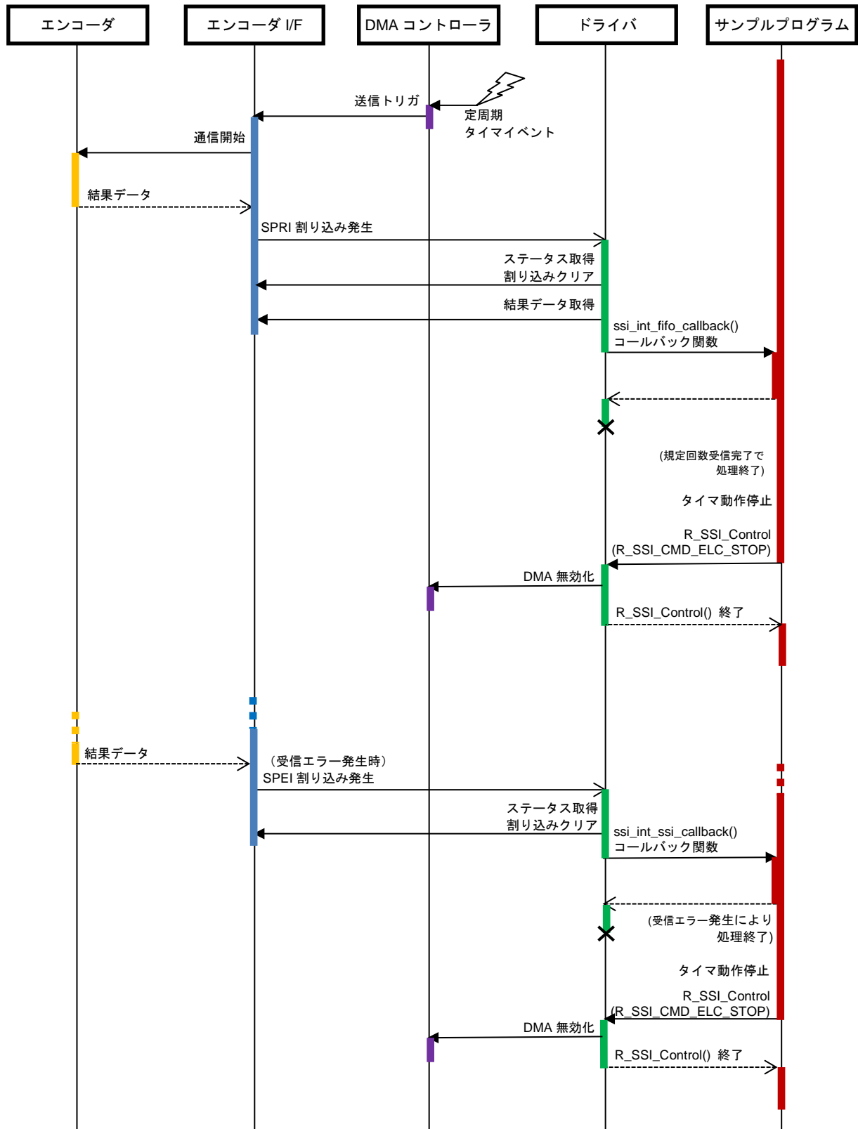
図 4-21 データ受信(タイマイベント同期動作)のシーケンス図
