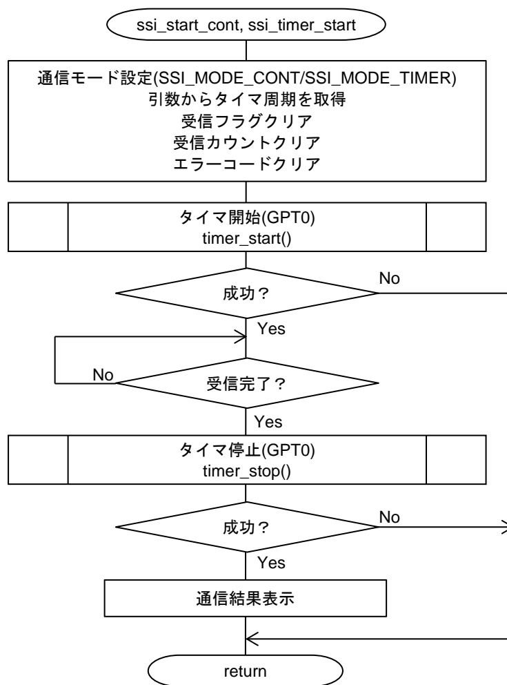
図 4-7 ssi_start_cont, ssi_timer_start 関数のフローチャート
