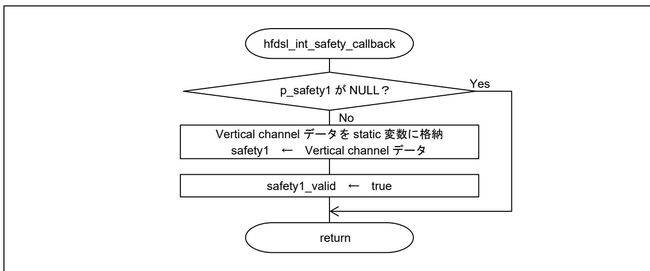
図 4-12 hfdsl_int_safety_callback 関数のフローチャート
