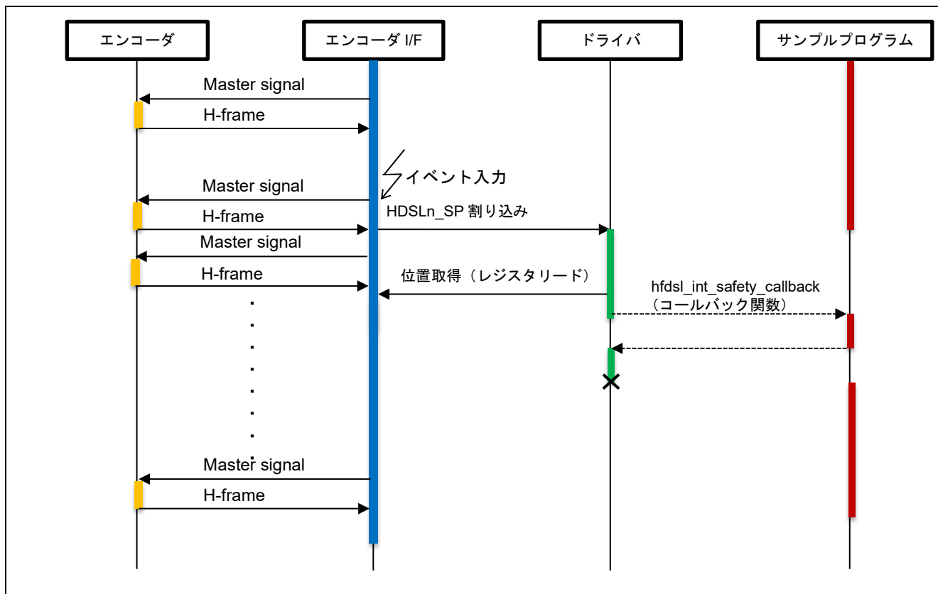
図 4-17 Vertical channel データ取得のシーケンス図
