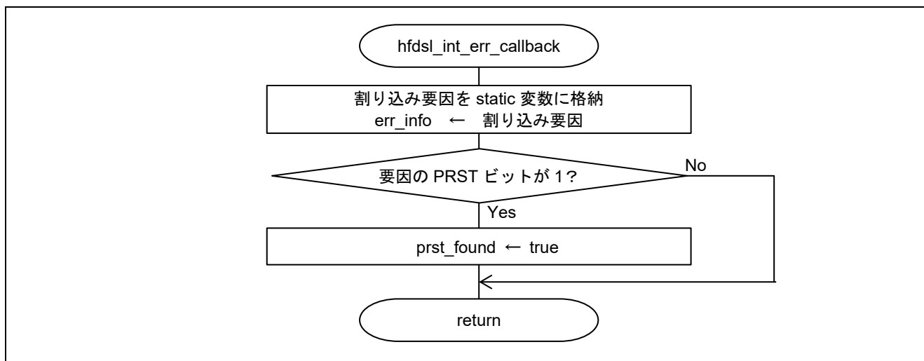
図 4-11 hfdsl_int_err_callback 関数のフローチャート
