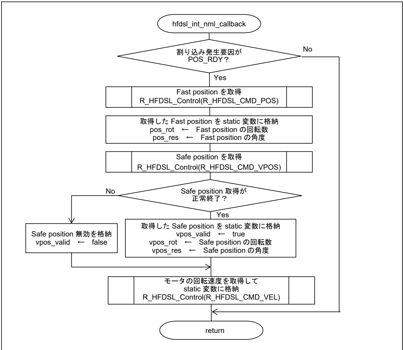
図 4-10 hfdsl_int_nml_callback 関数のフローチャート
