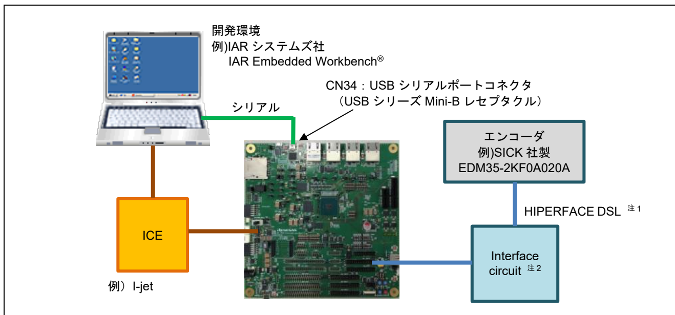
図 1-1 動作環境
