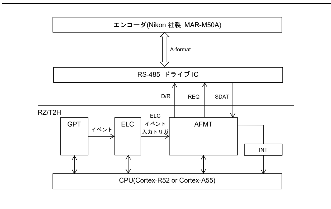
図 4-1 システムブロック図
