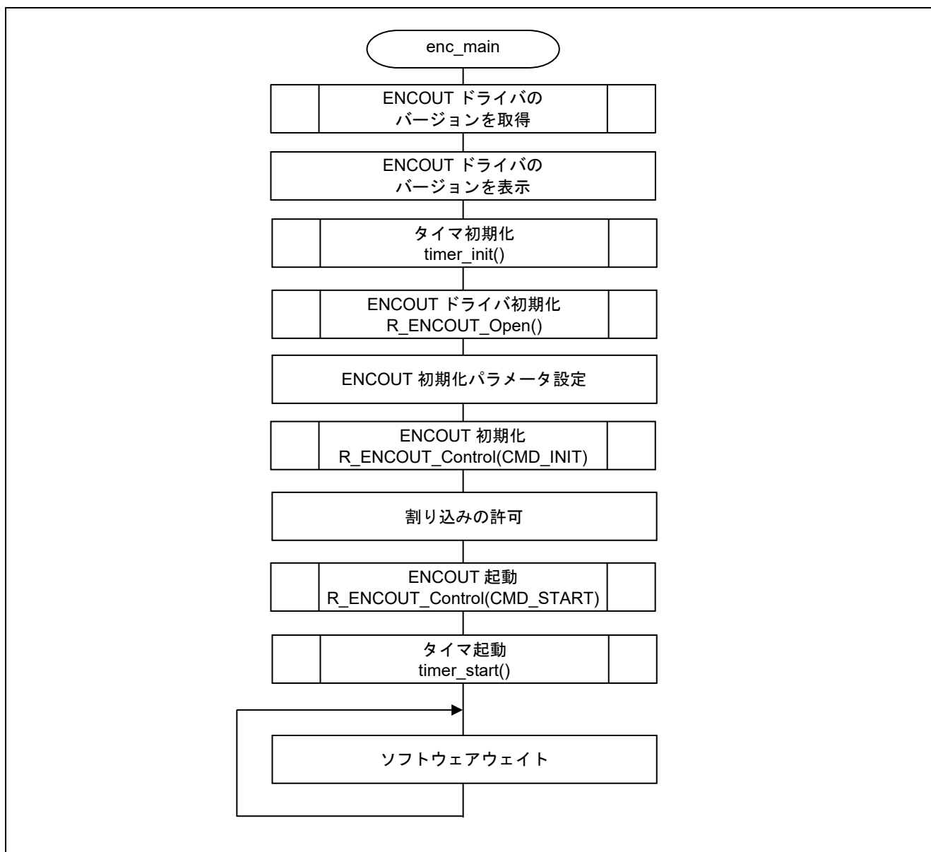
図 4-3 enc_main 関数のフローチャート
