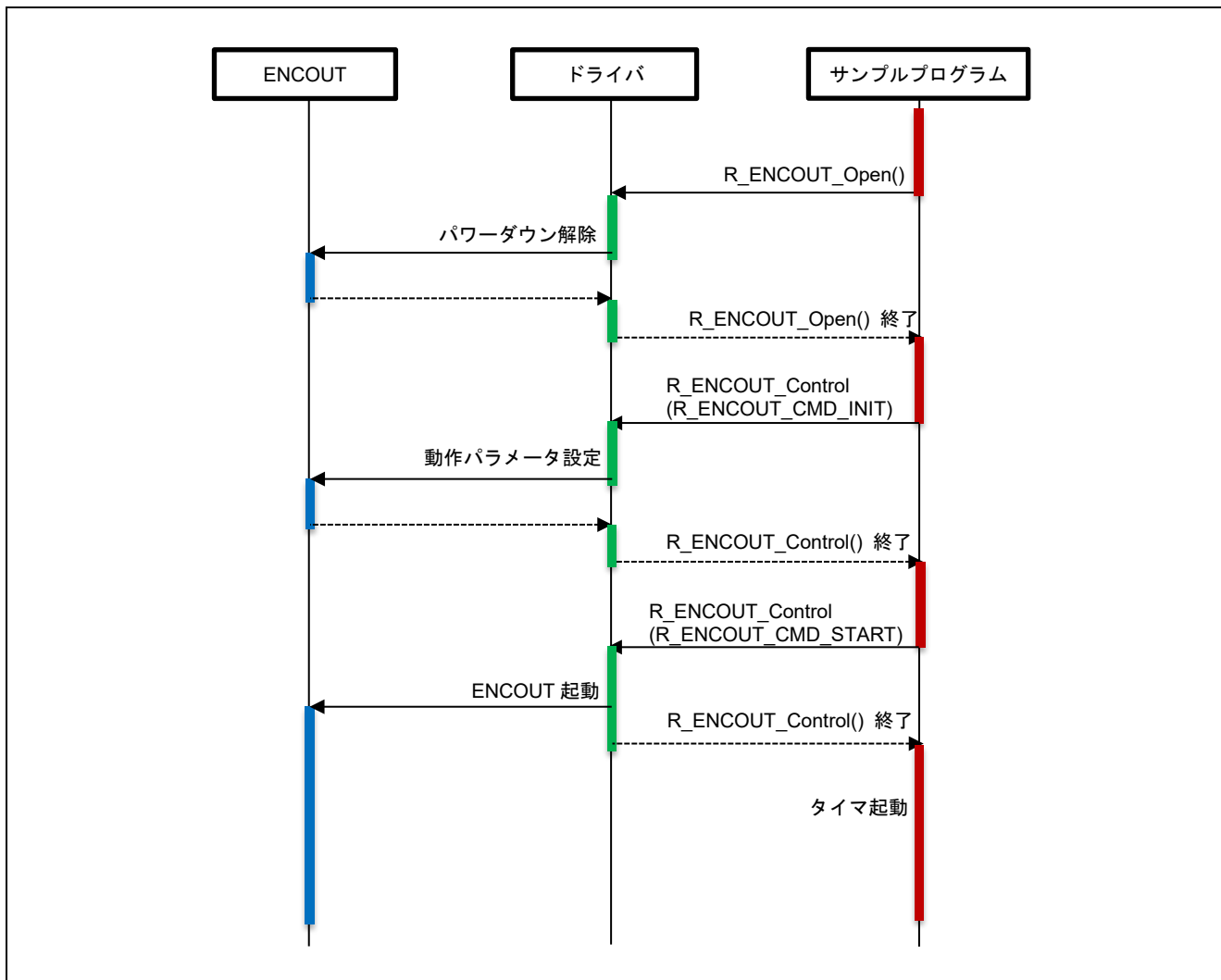
図 4-5 開始シーケンス図
