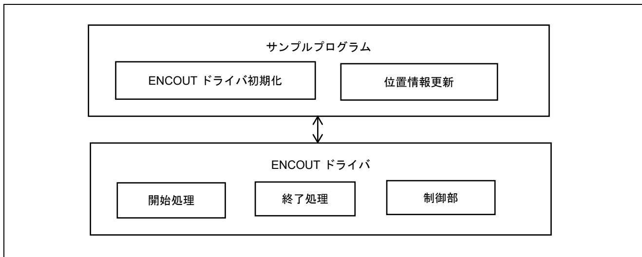
図 4-2 ソフトウェア構成図
