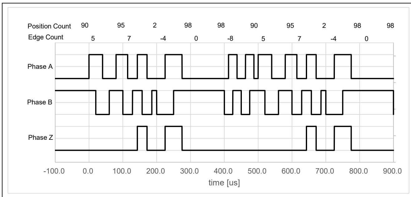
図 4-7 ABZ 相出力信号
