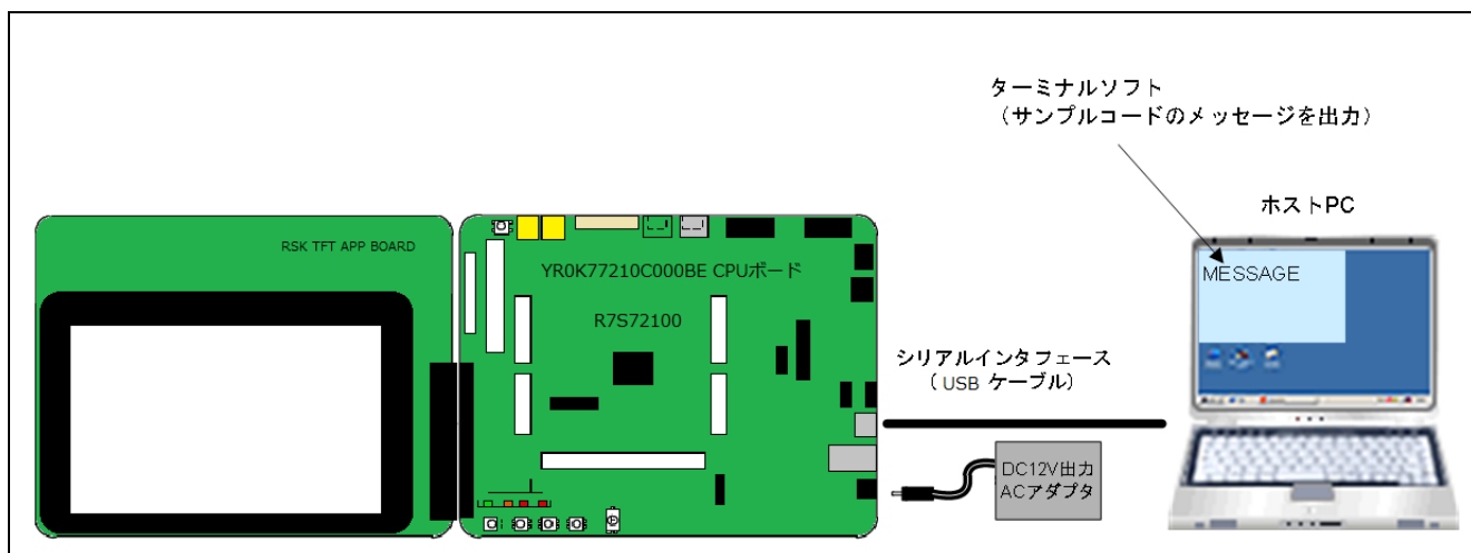
図 1.1 動作環境
