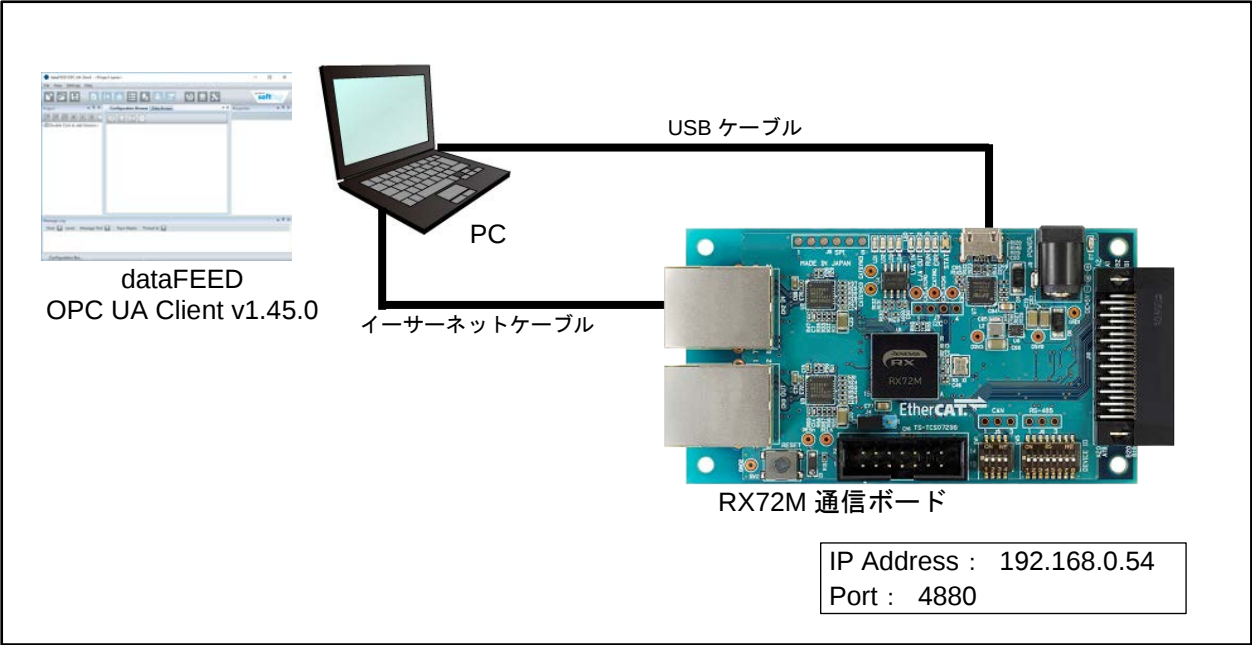
図 7.1 接続構成
