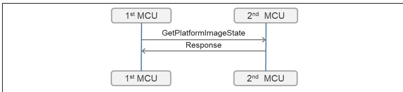
図 3-5 2 nd MCU の ImageState を問い合わせる通信
