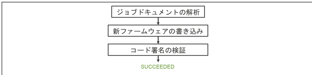
図 3-3 fileType ≠ configOTA_FIRMWARE_UPDATE_FILE_TYPE_ID の場合の OTA Agent 動作
