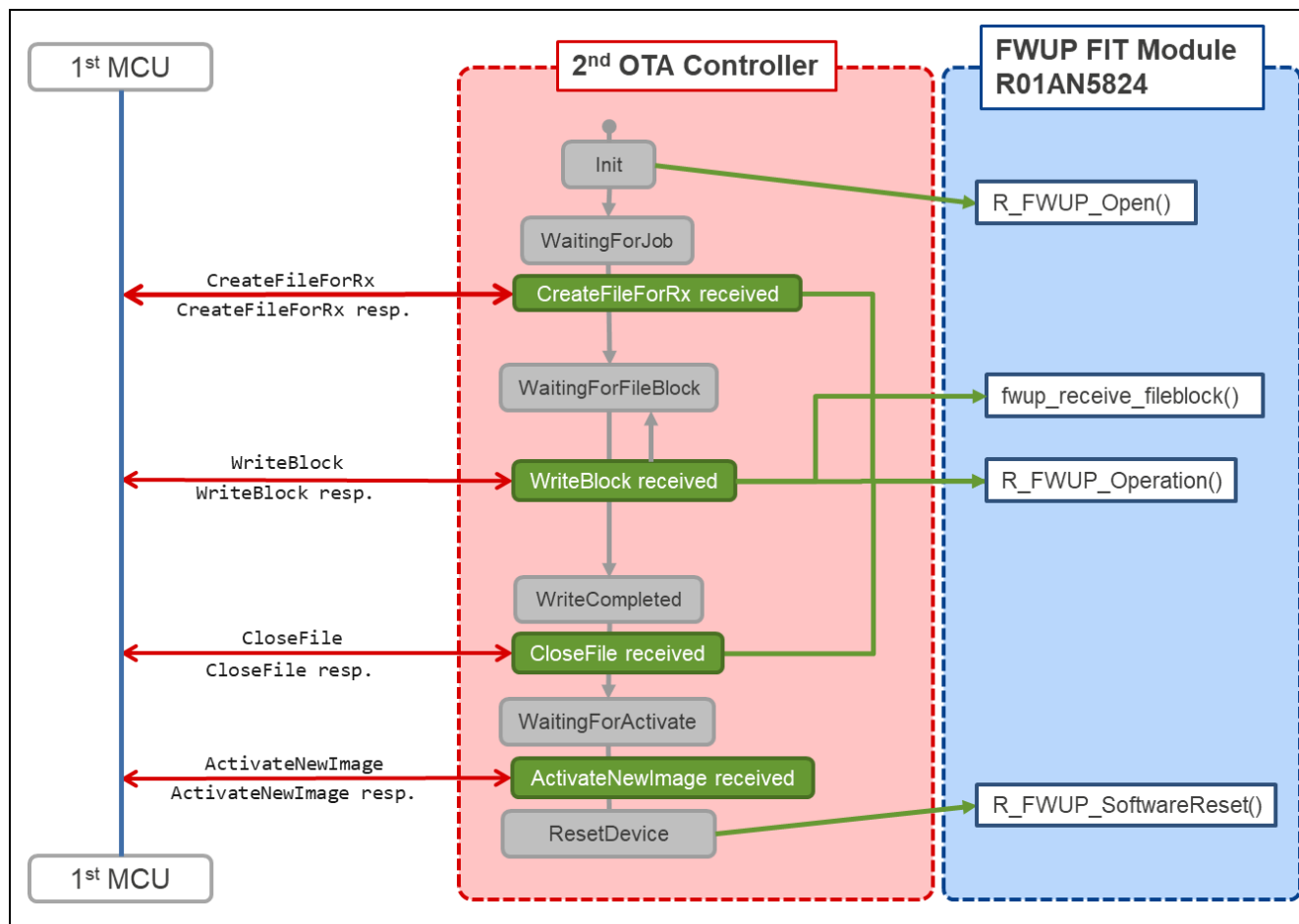
図 5-1 2 nd OTA Controller の状態遷移設計例
