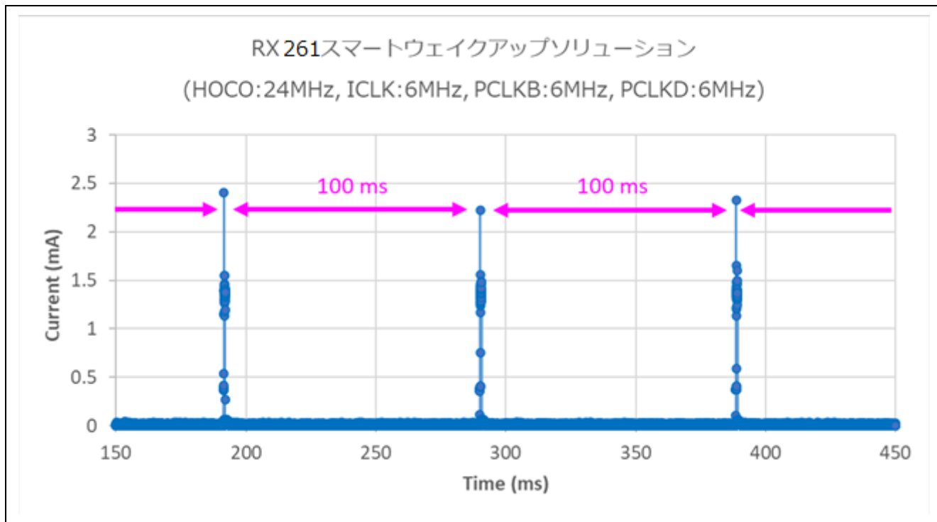
図 6.5 スタンバイモードの消費電流波形 (1/2)
