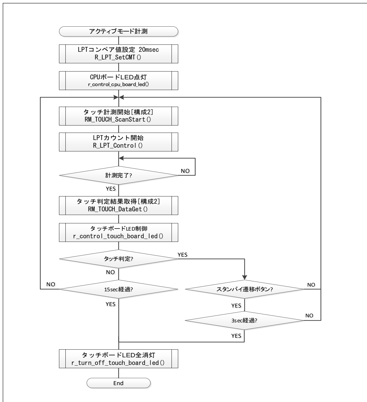
図 4.7 アクティブモード計測処理のフローチャート
