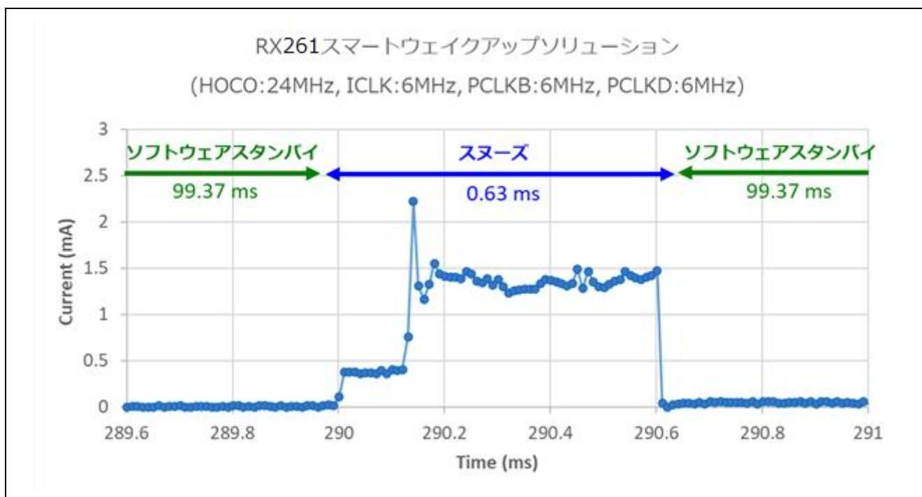
図 6.6 スタンバイモードの消費電流波形 (2/2)
