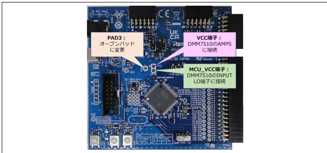
図 6.1 RX261 CPU ボード・前面
