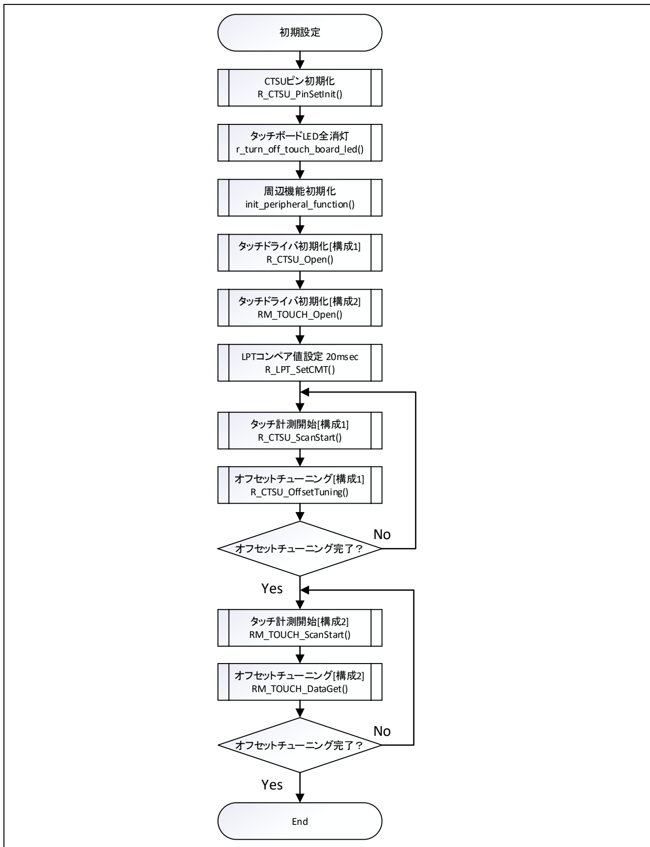
図 4.4 初期設定処理のフローチャート
