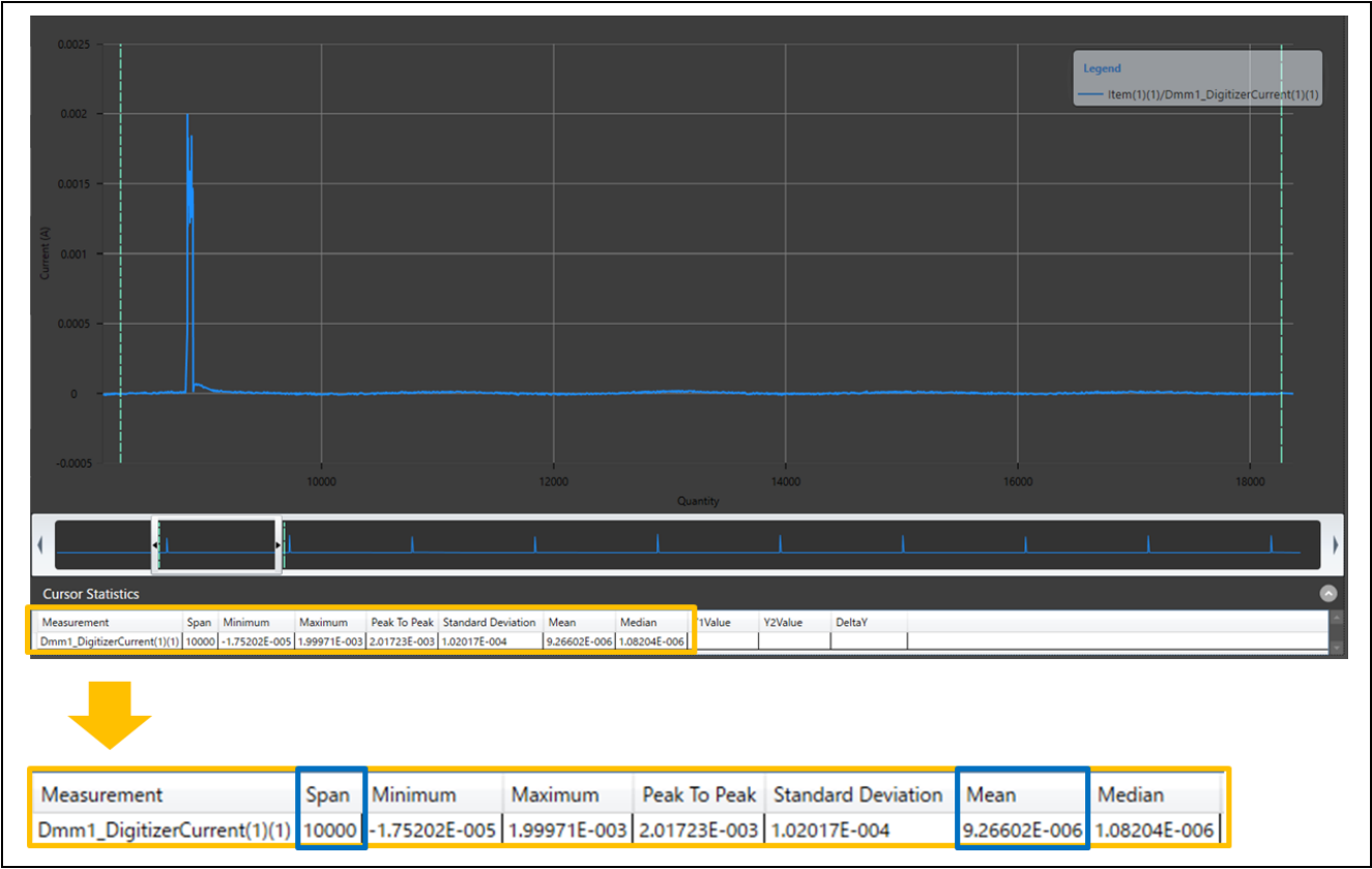
図 6.7 スタンバイモードの消費電流結果
