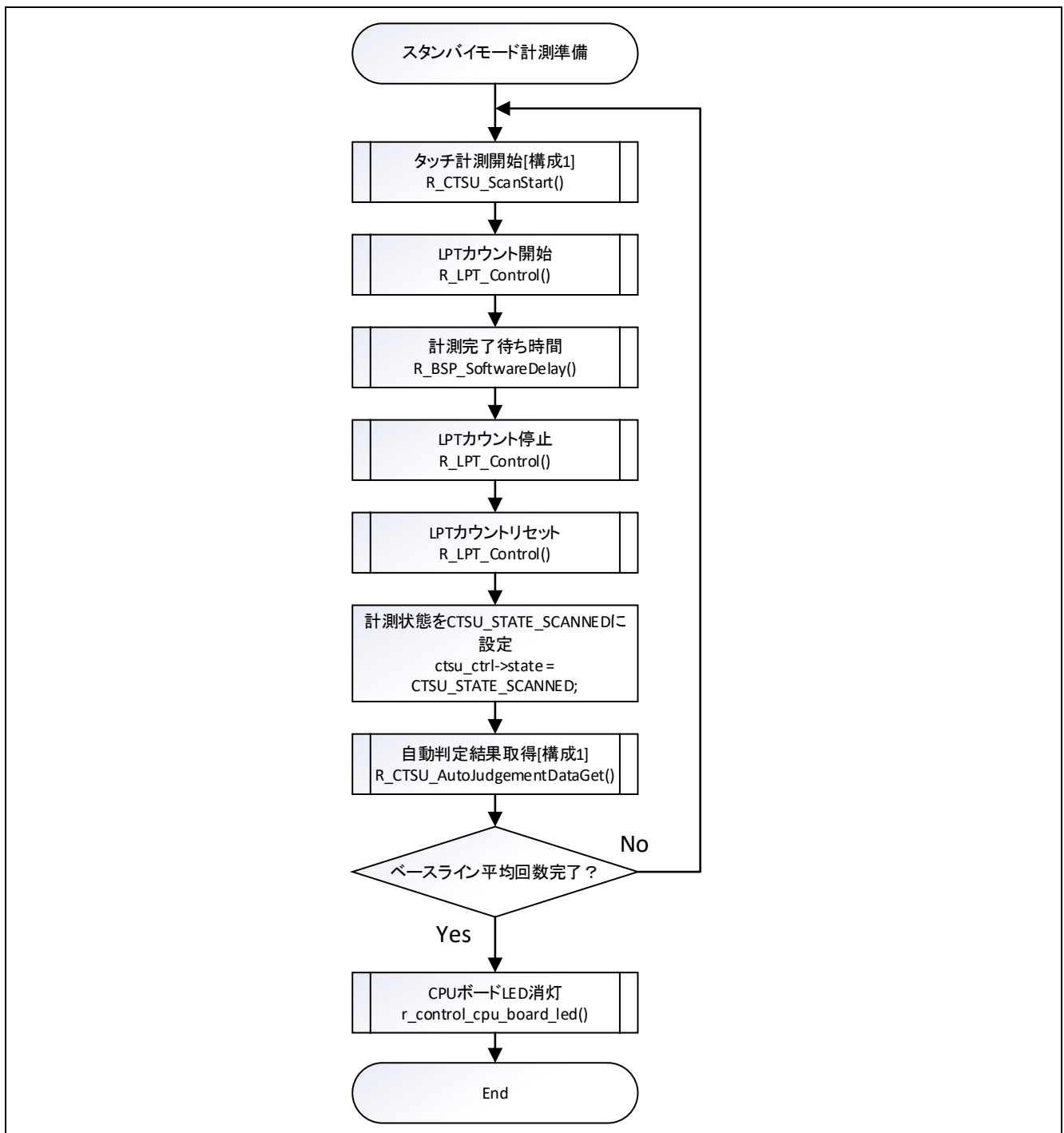
図 4.5 スタンバイモード計測準備処理のフローチャート
