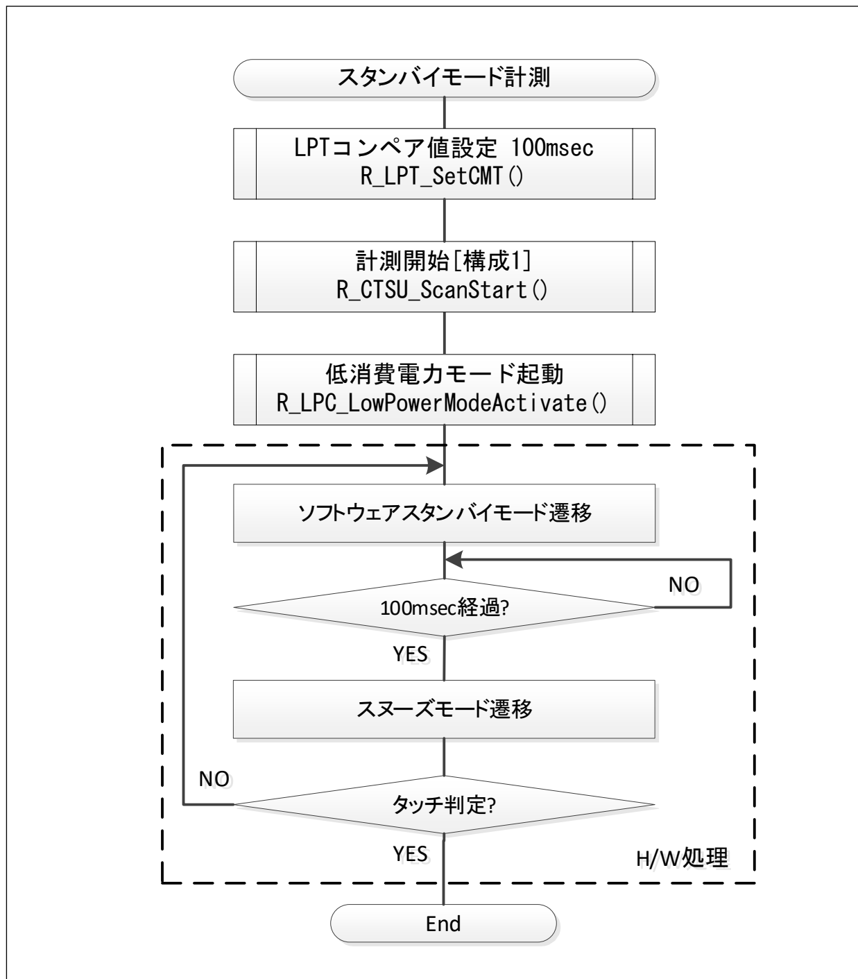
図 4.6 スタンバイモード計測処理のフローチャート
