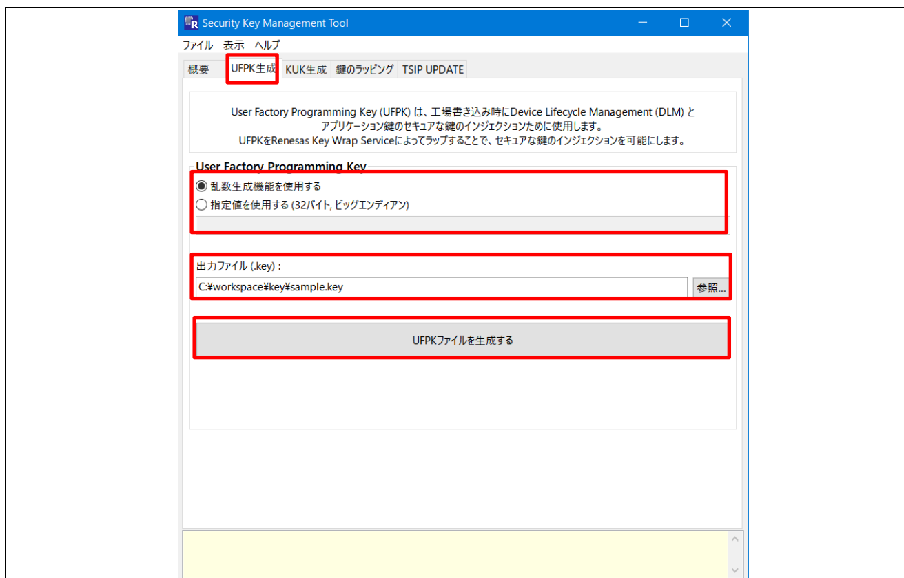
図 2-33 UFPK の生成
