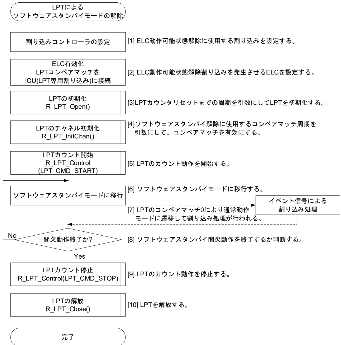
図 1.1 LPT FIT モジュールの処理例
