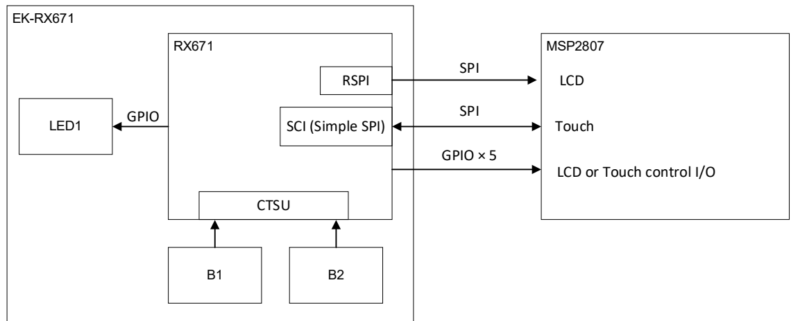
図 5.1 ハードウェアの構成
