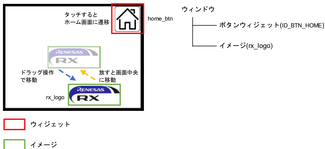
図 6.5 RX ロゴ表示画面の構成
