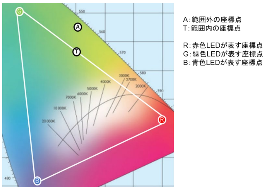
図 4-12 各 LED 座標点による範囲と範囲外座標点/範囲内座標点の例
