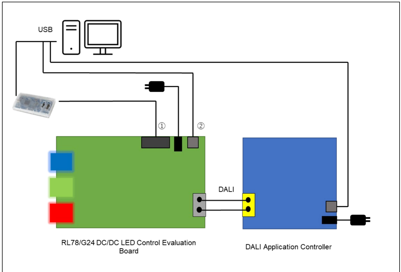
図 4-2 接続図
