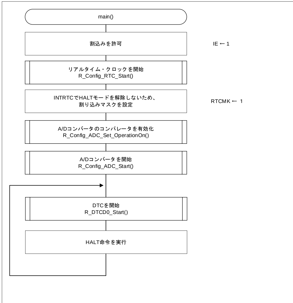
図 4-1 メイン処理
