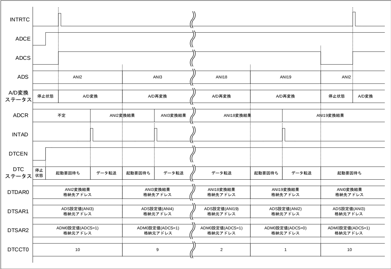
図 1-2 DTC による A/D 変換結果転送概要 (タイミングチャート)
