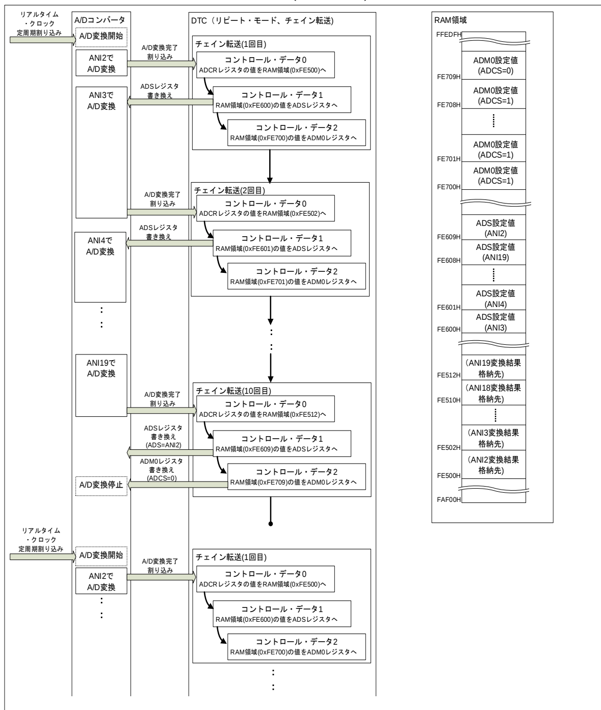
図 1-1 DTC による A/D 変換結果転送概要 (ブロック図)
